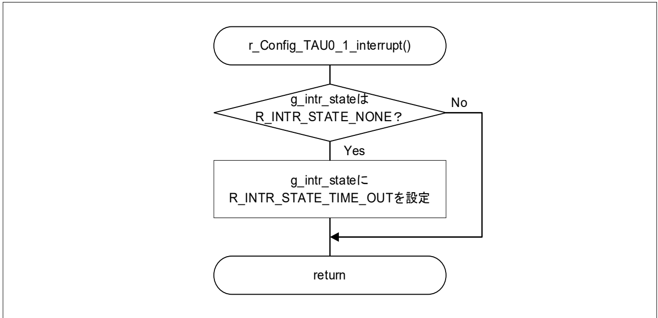
図 4-5 STOP モード移行用タイマ割り込み
