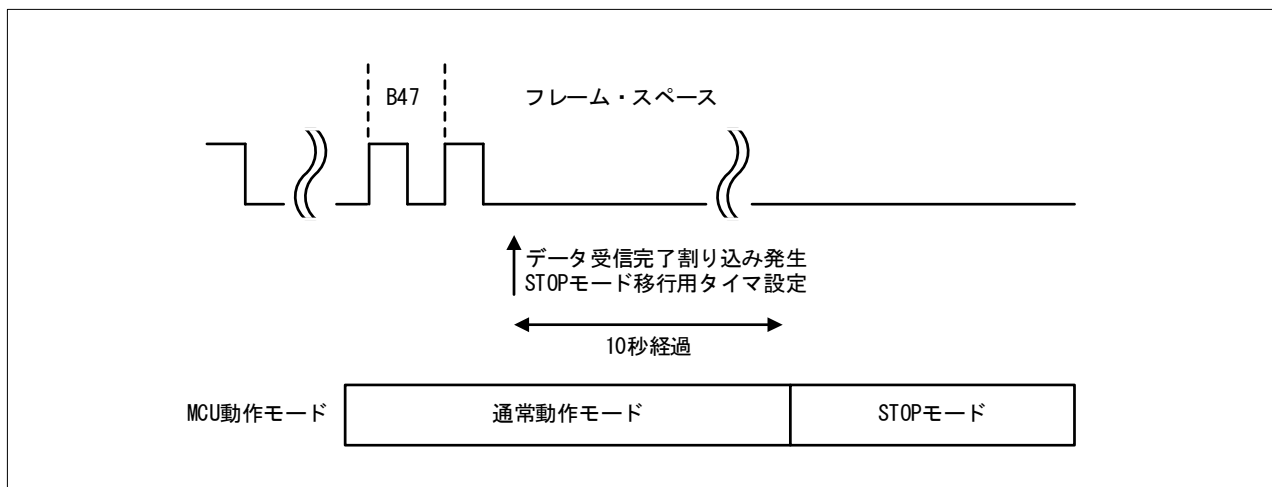
図 1-3 STOP モードへ移行するタイミング
