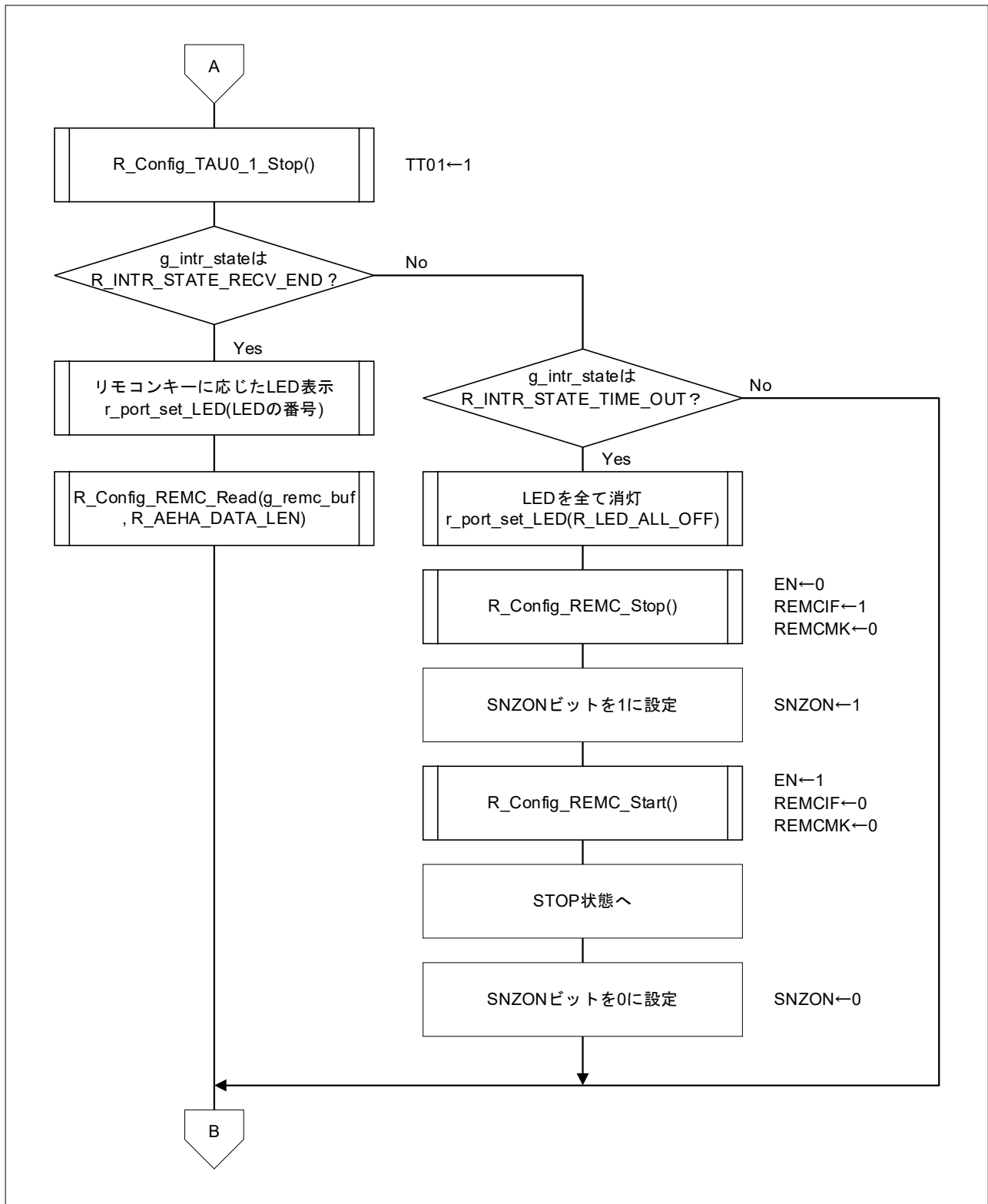
図 4-2 メイン処理 (2/2)
