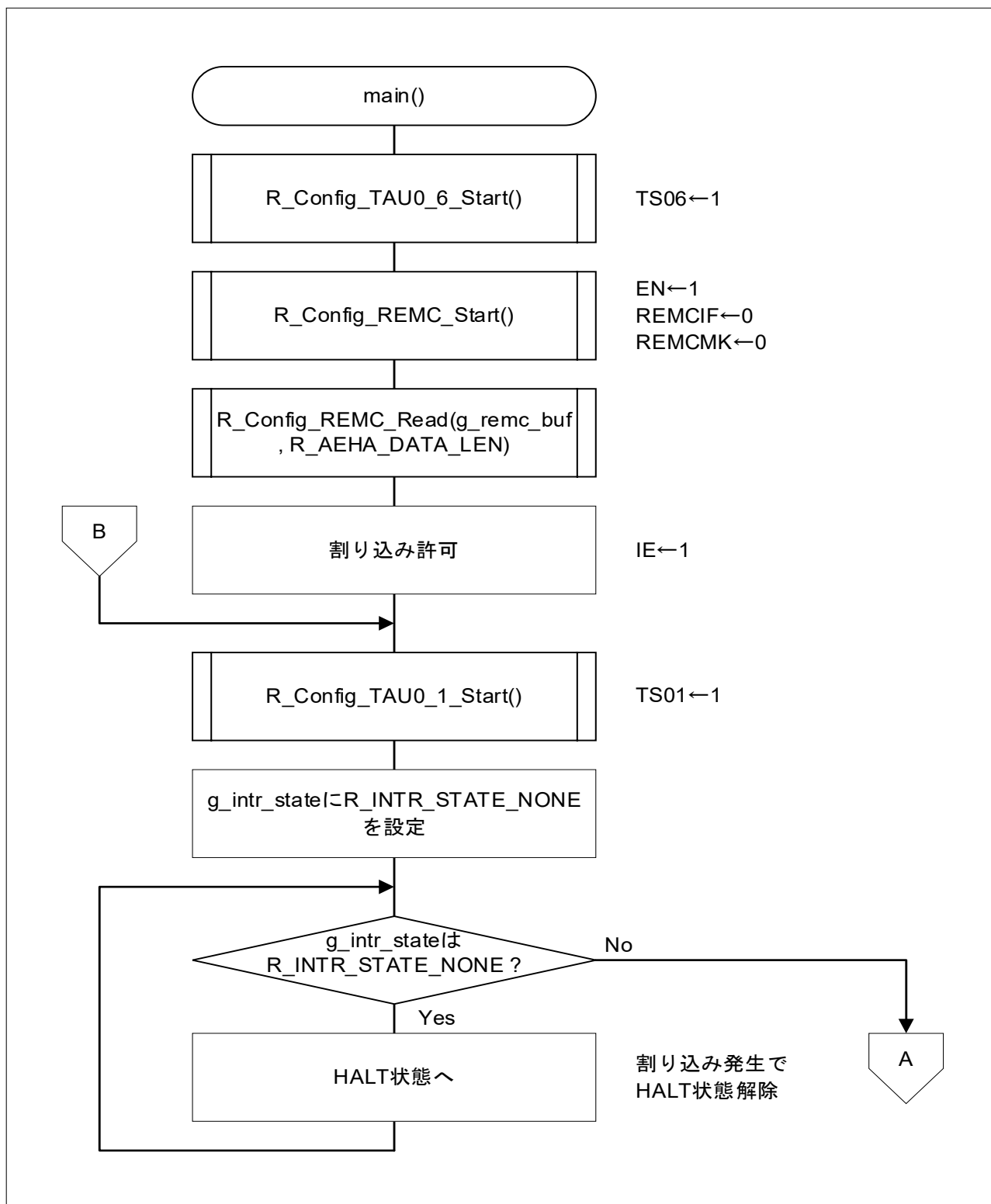
図 4-1 メイン処理 (1/2)
