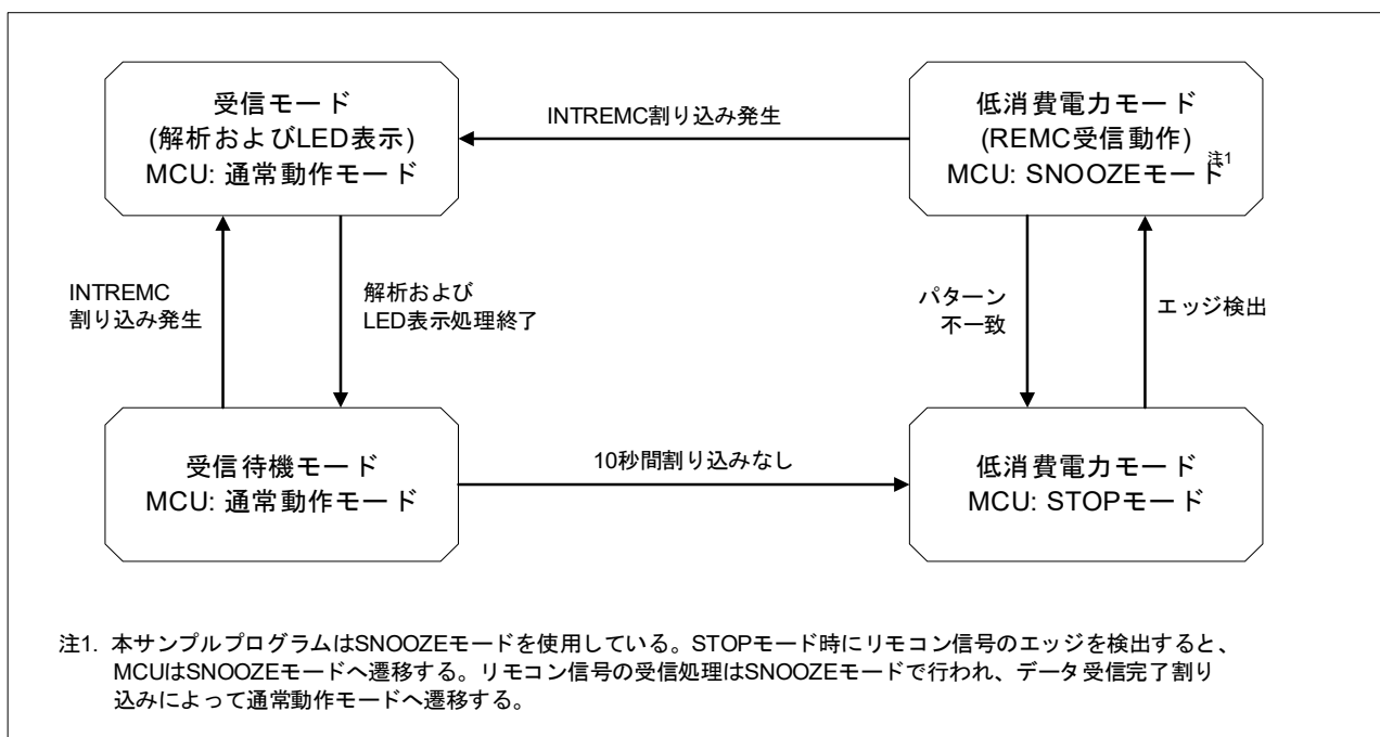
図 1-4 リモコン受信ソフトウェア状態遷移図
