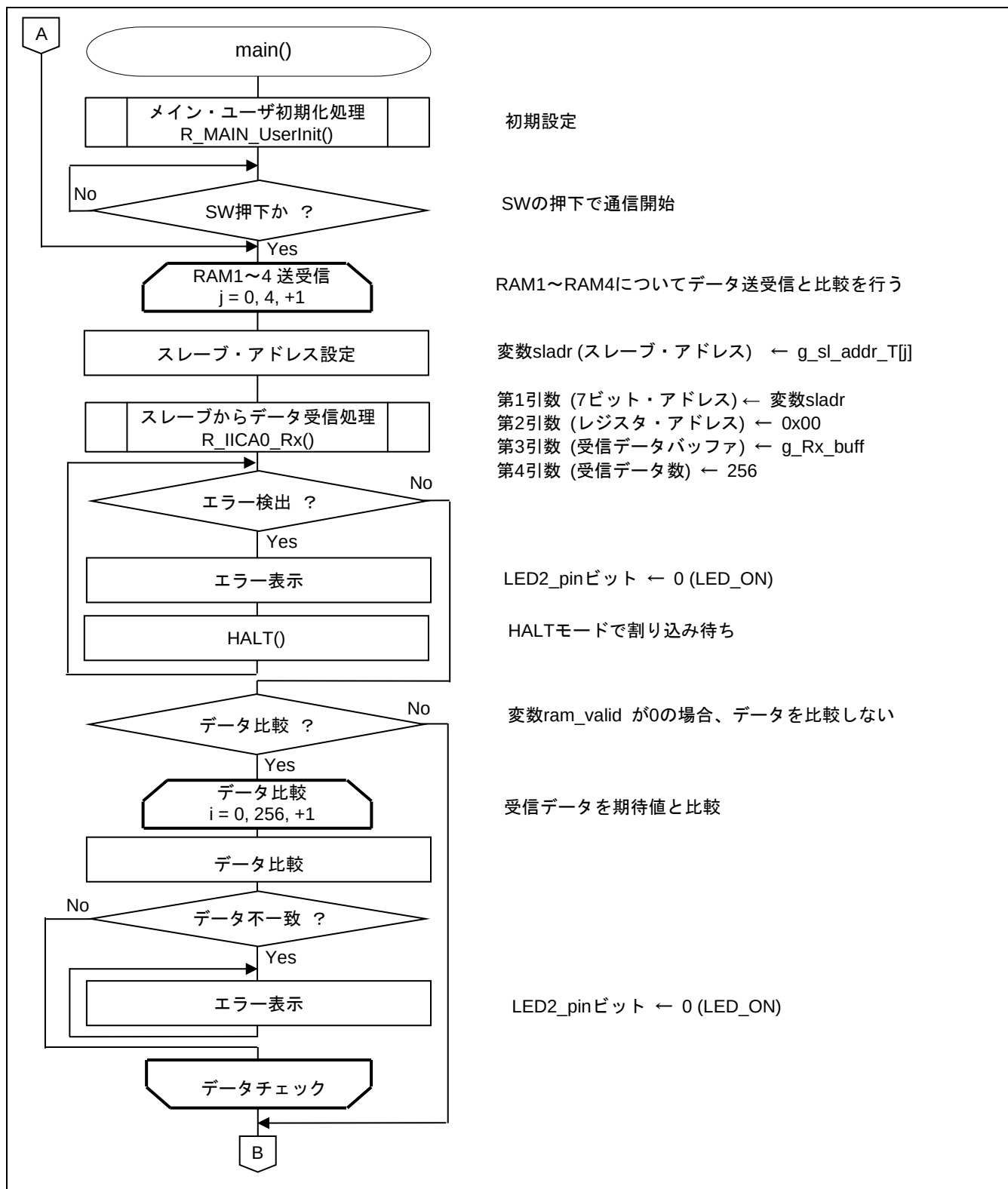
図 4-1 メイン処理 (1/3)
