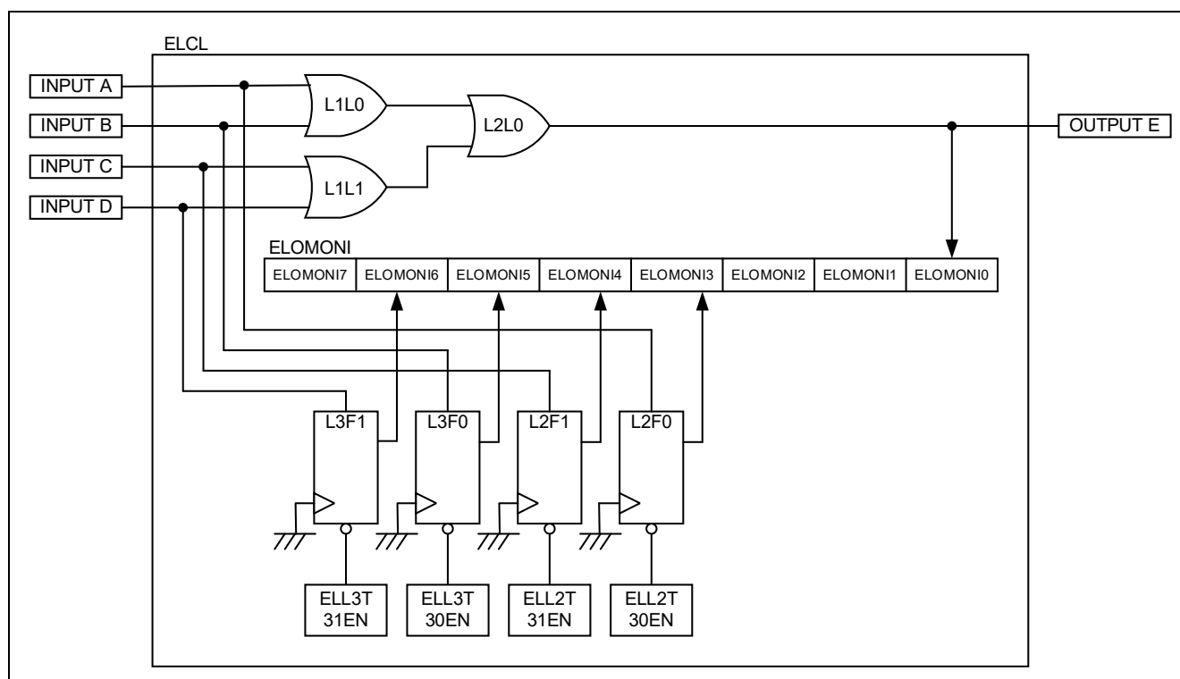
図 1-1 ELCL の構成
