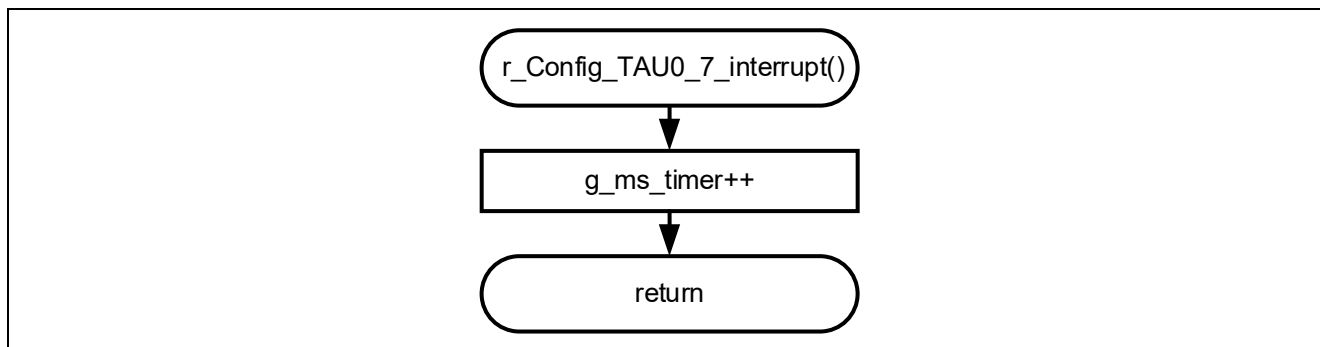
図 4-12 TAU0 チャンネル 7 割り込み処理
