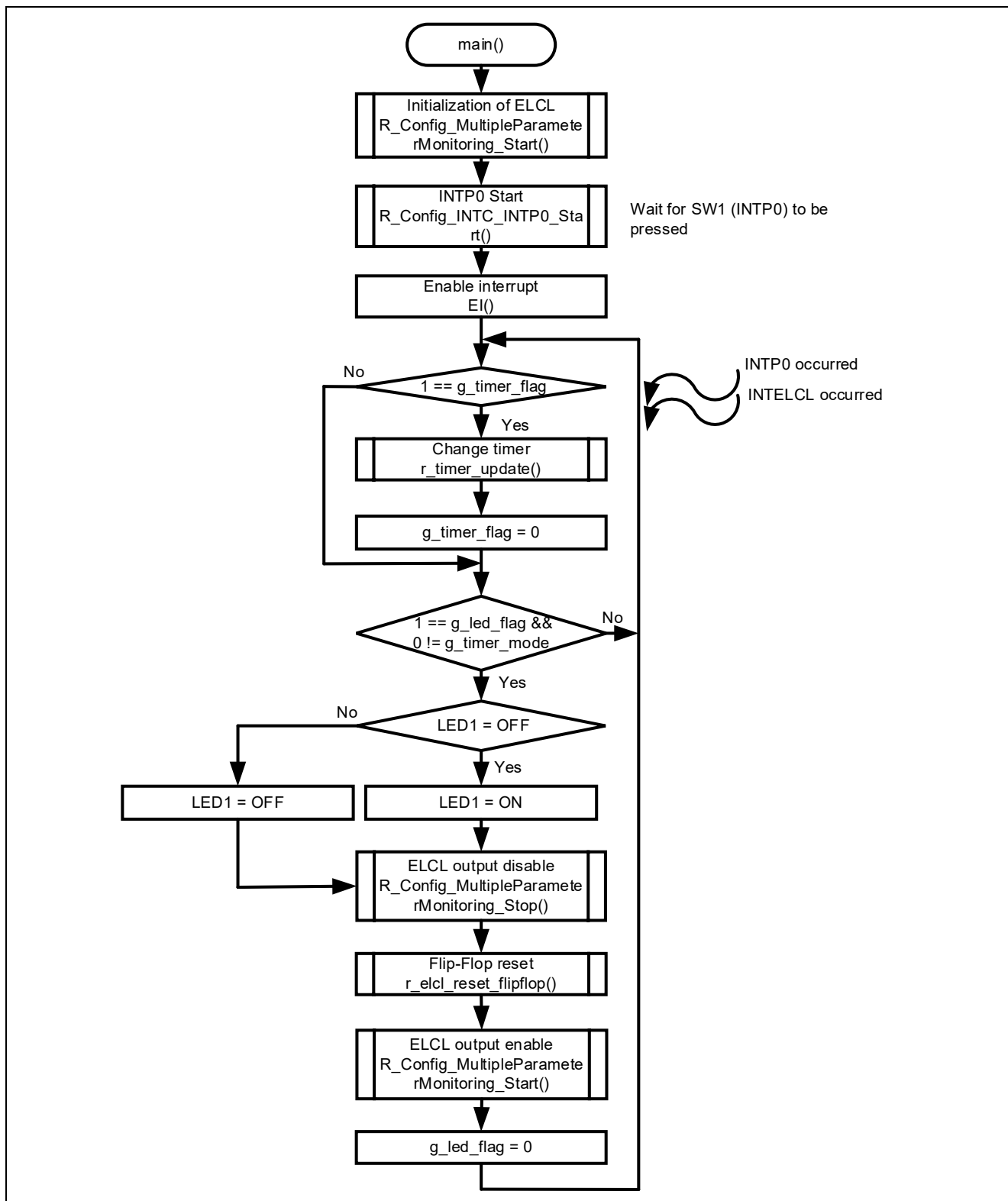
図 4-4 メイン処理
