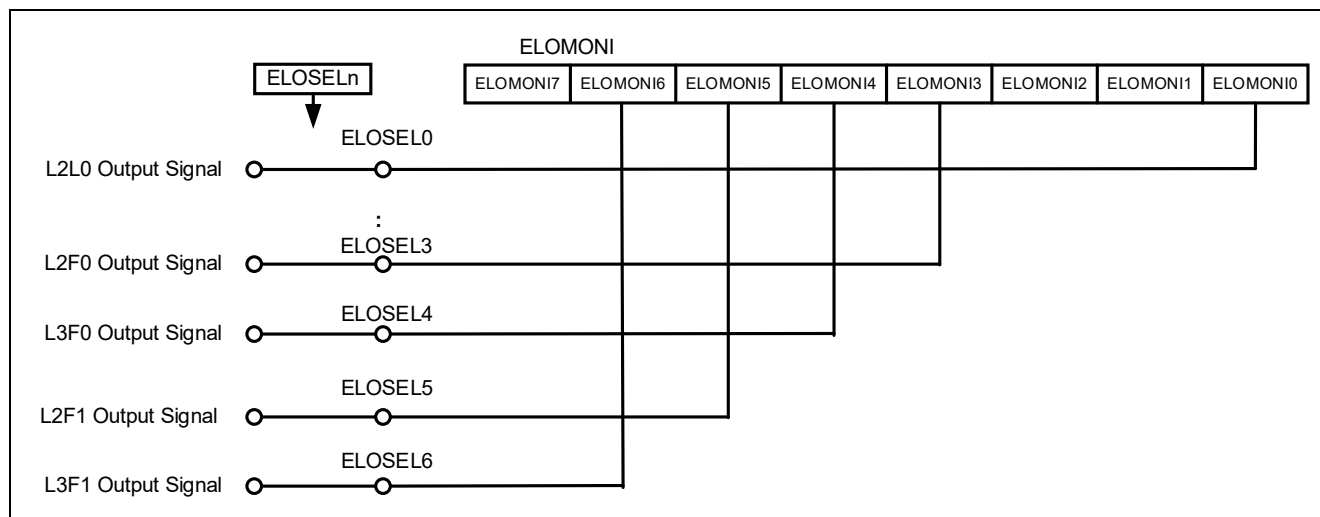
図 5-9 ELCL の出力設定
