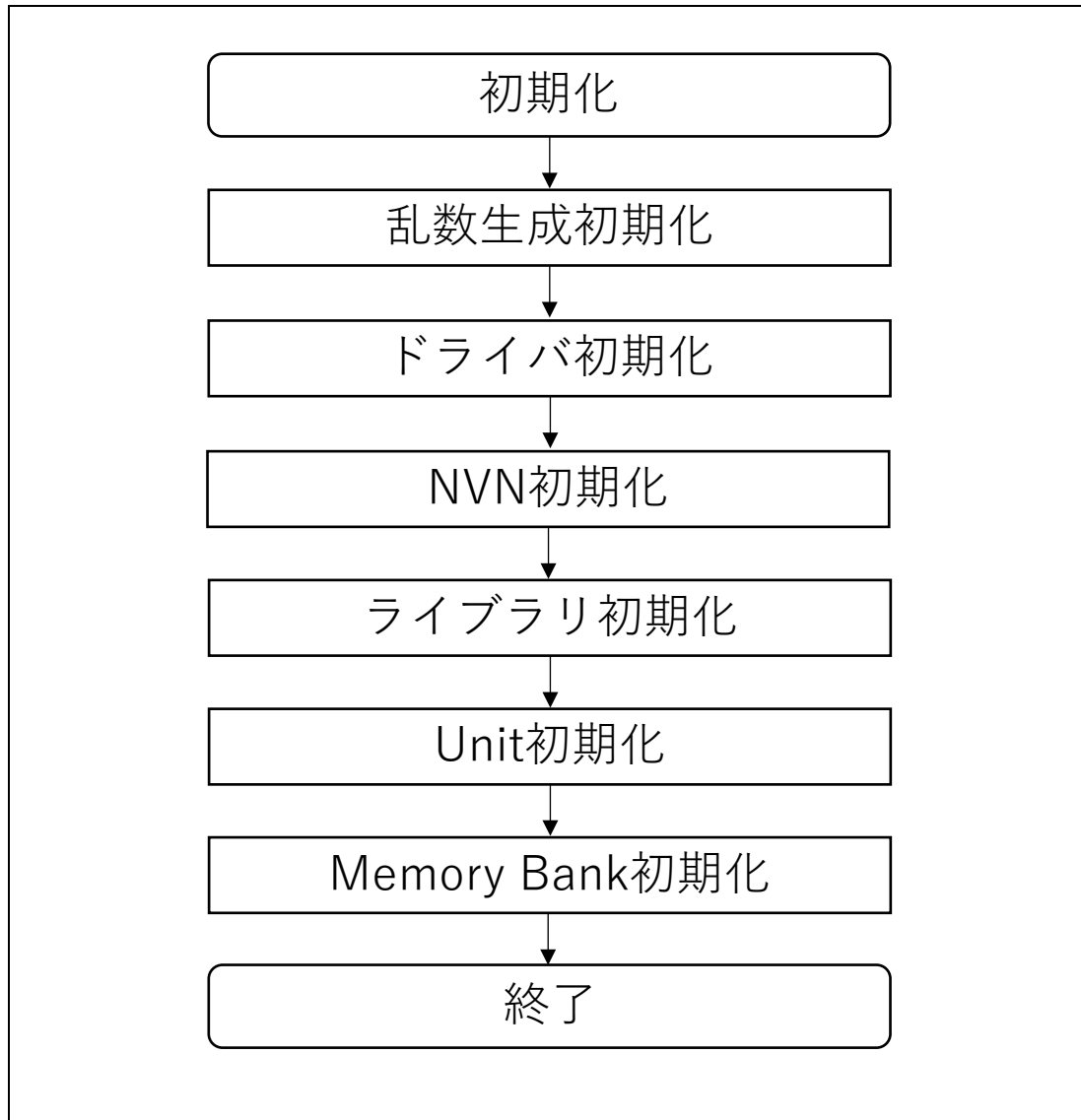
図 4-14 初期化処理フロー図
