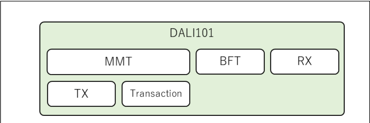
図 4-12 DALI101 通信ドライバ構成
