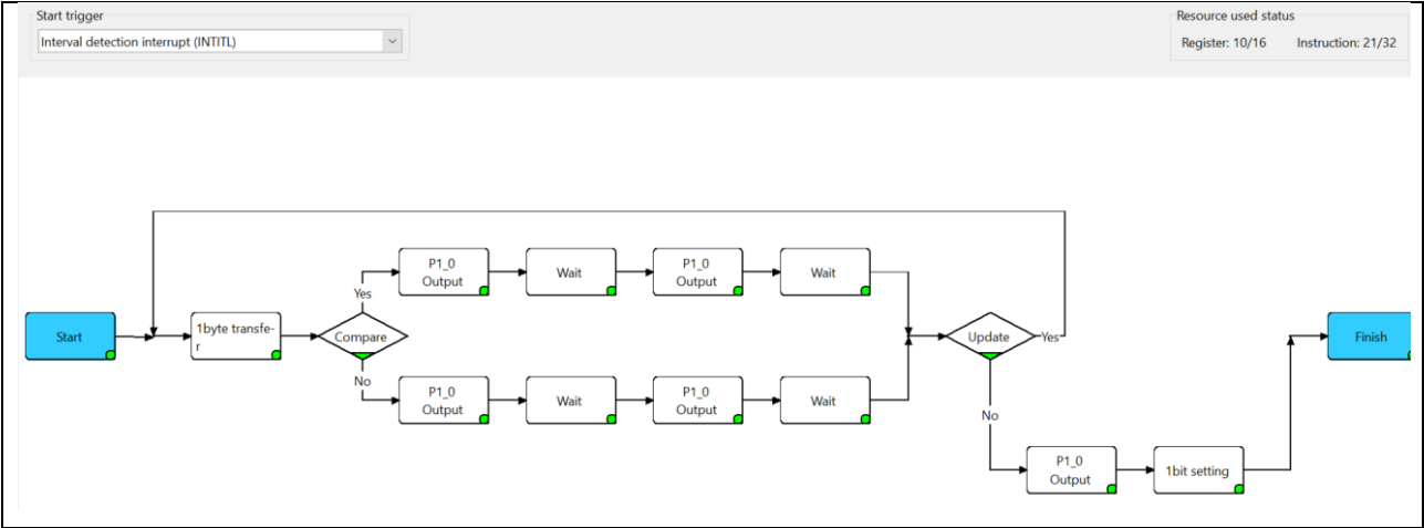
図 4-11 SMS 設定
