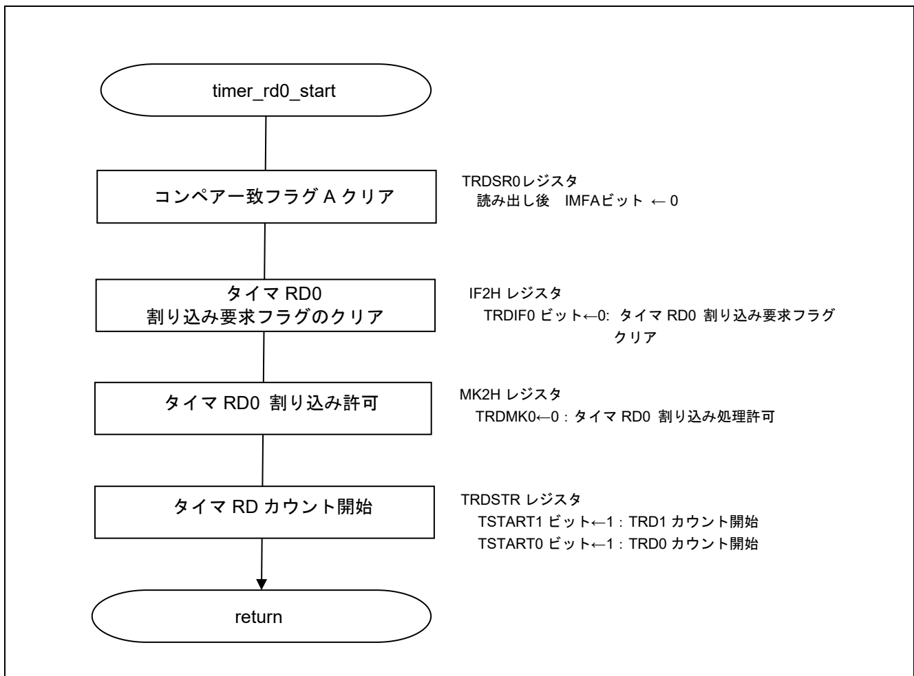
図 4.28 タイマ RD カウント開始設定
