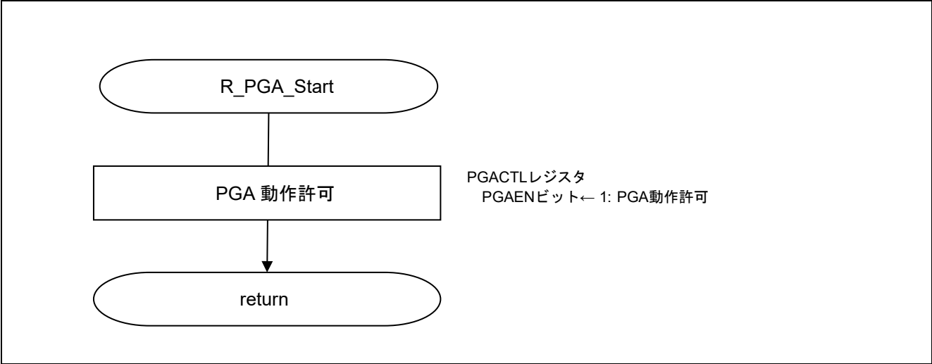
図 4.27 PGA 起動
