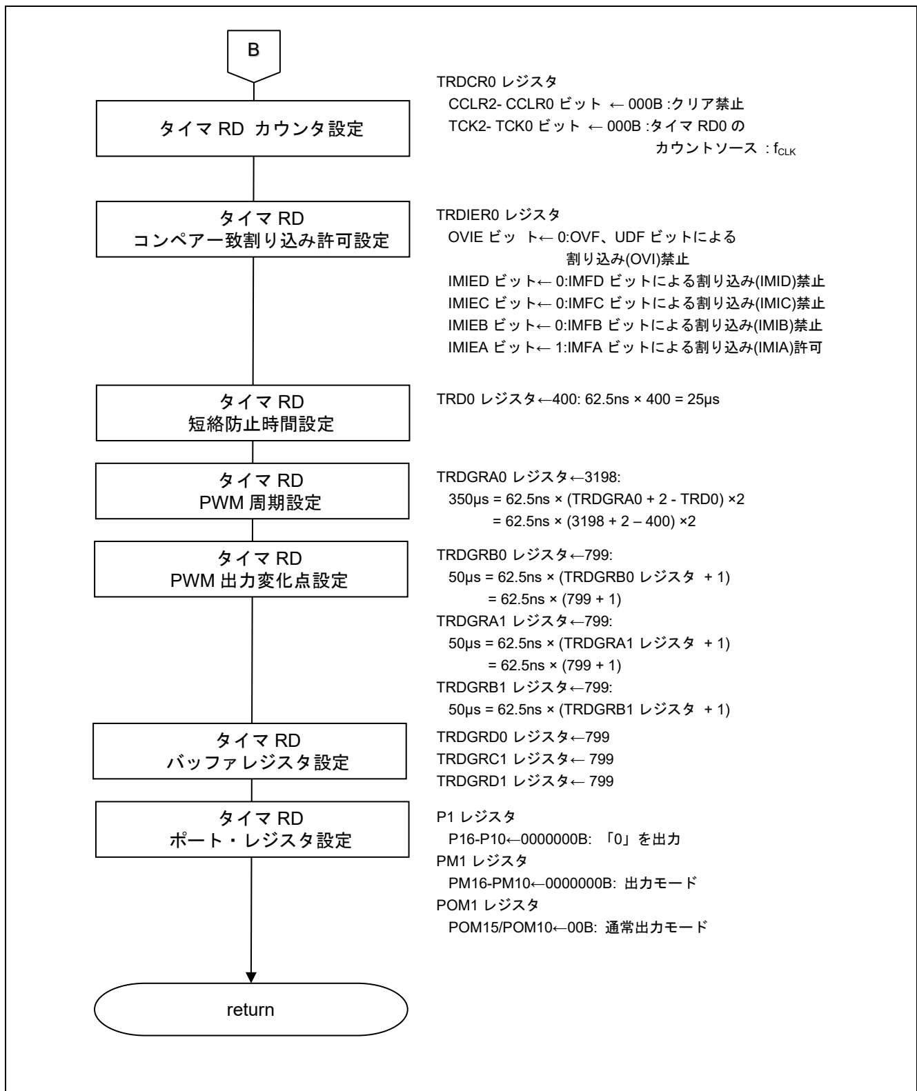
図 4.21 タイマ RD 初期設定(3/3)
