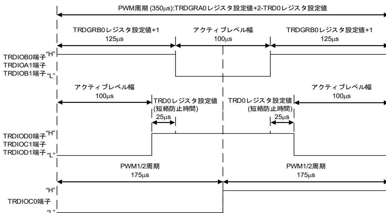
図 4.2 PWM 波形 2
