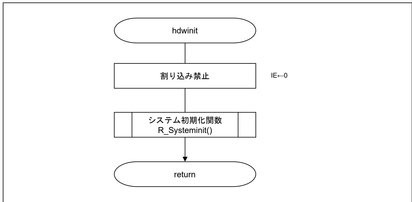
図 4.15 初期設定
