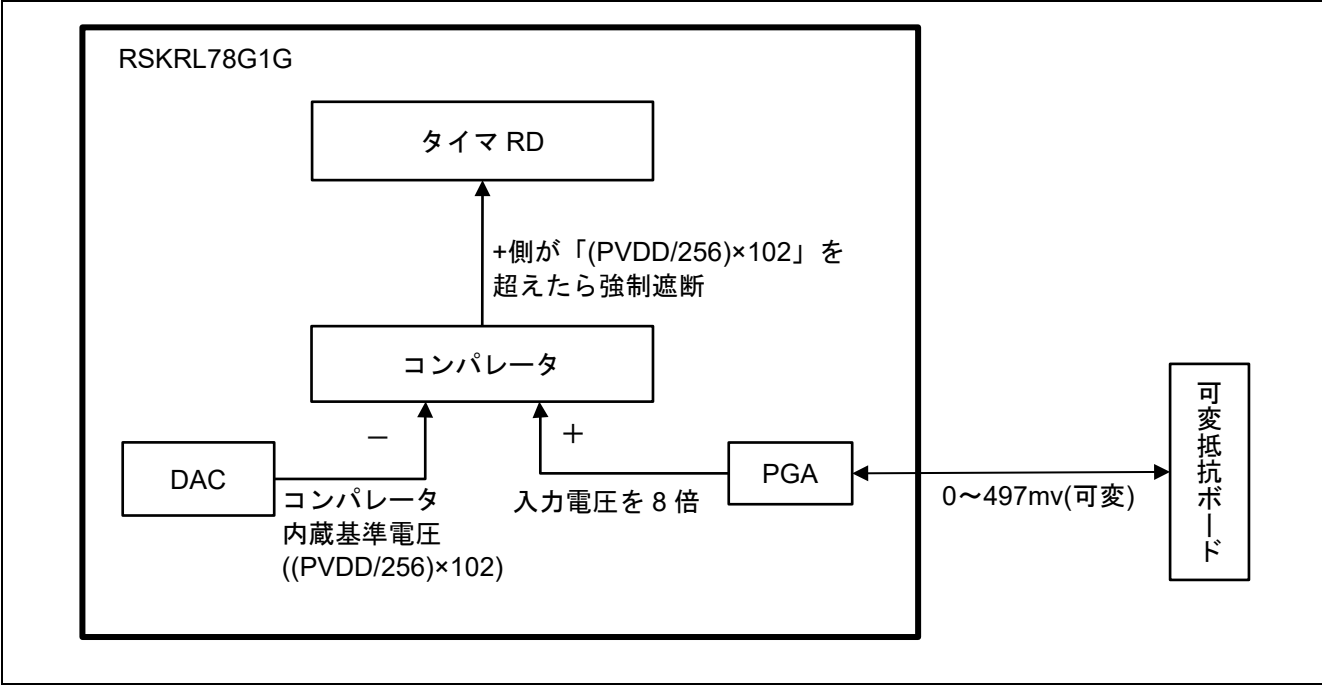
図 1.1 動作概要
