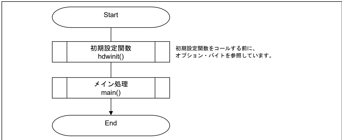
図 4.14 全体フロー
