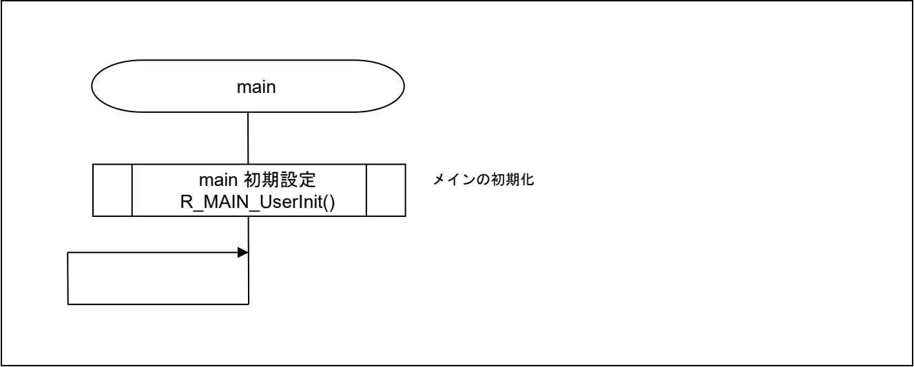
図 4.23 メイン処理
