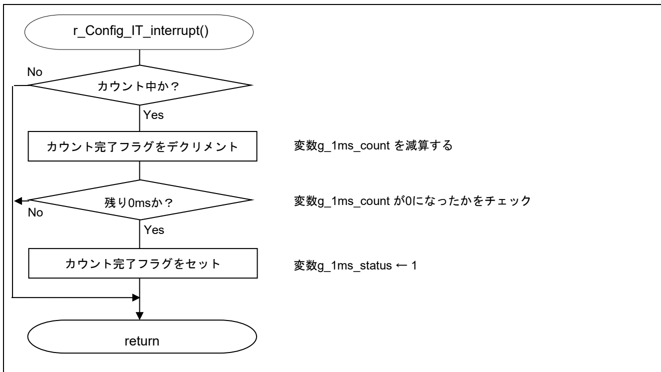
図 5.7 12 ビット・インターバル・タイマ割り込み処理
