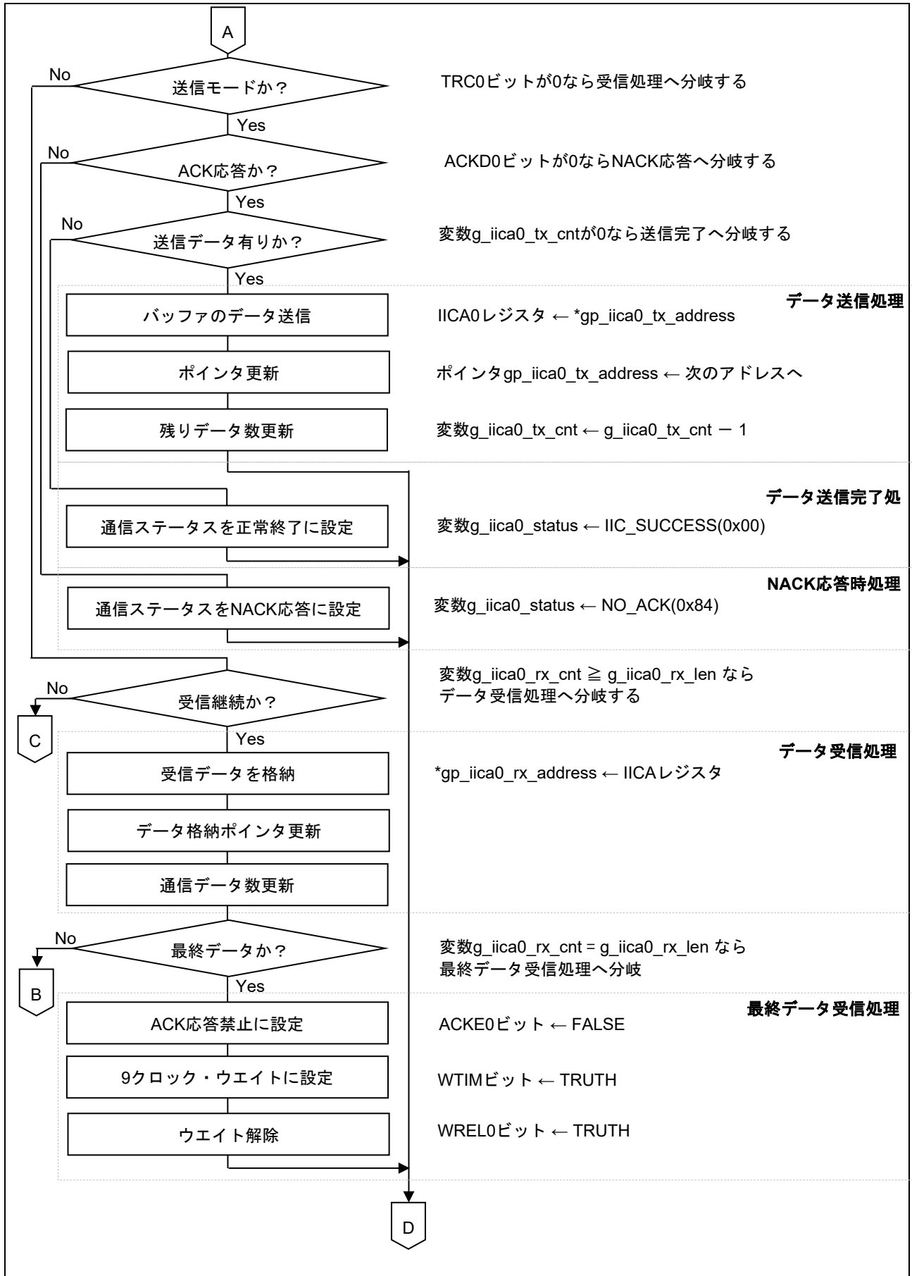
図 5.19 IICA0 割り込み処理 (2/3)
