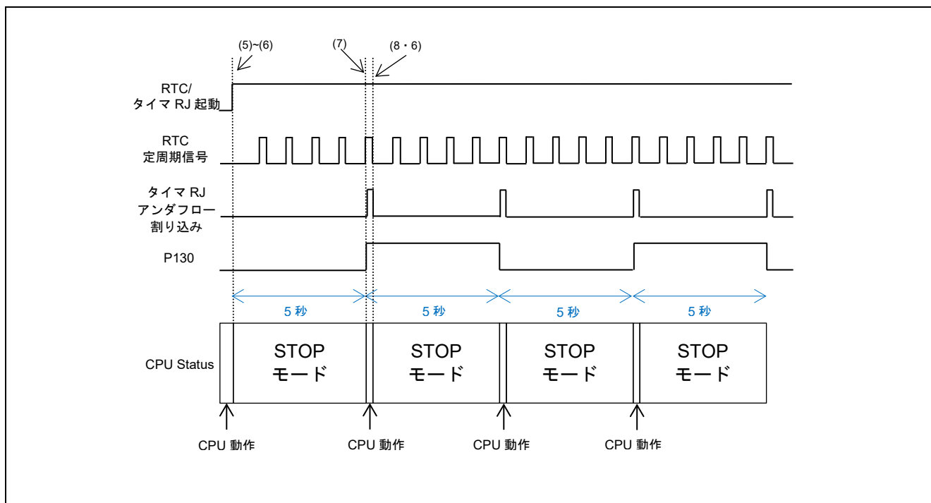
図 5.3 タイミングチャート
