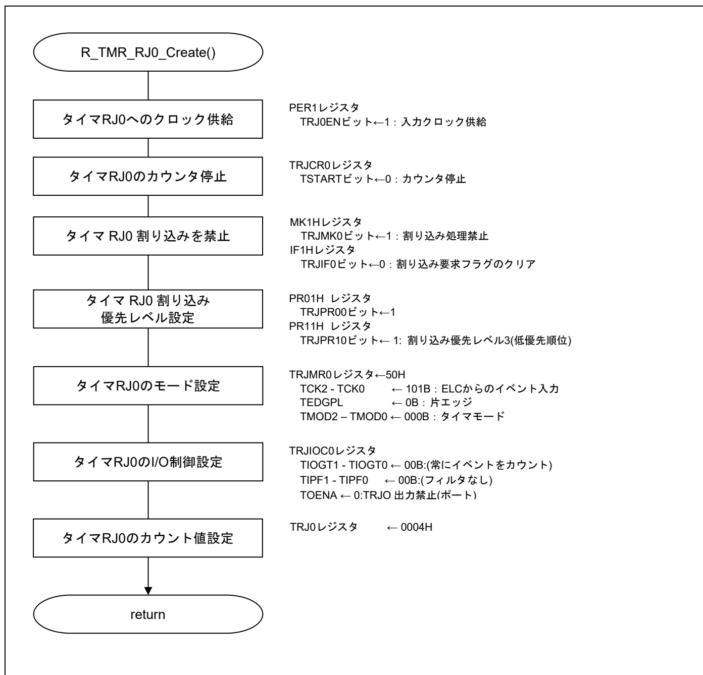
図 5.10 タイマ RJ 初期設定
