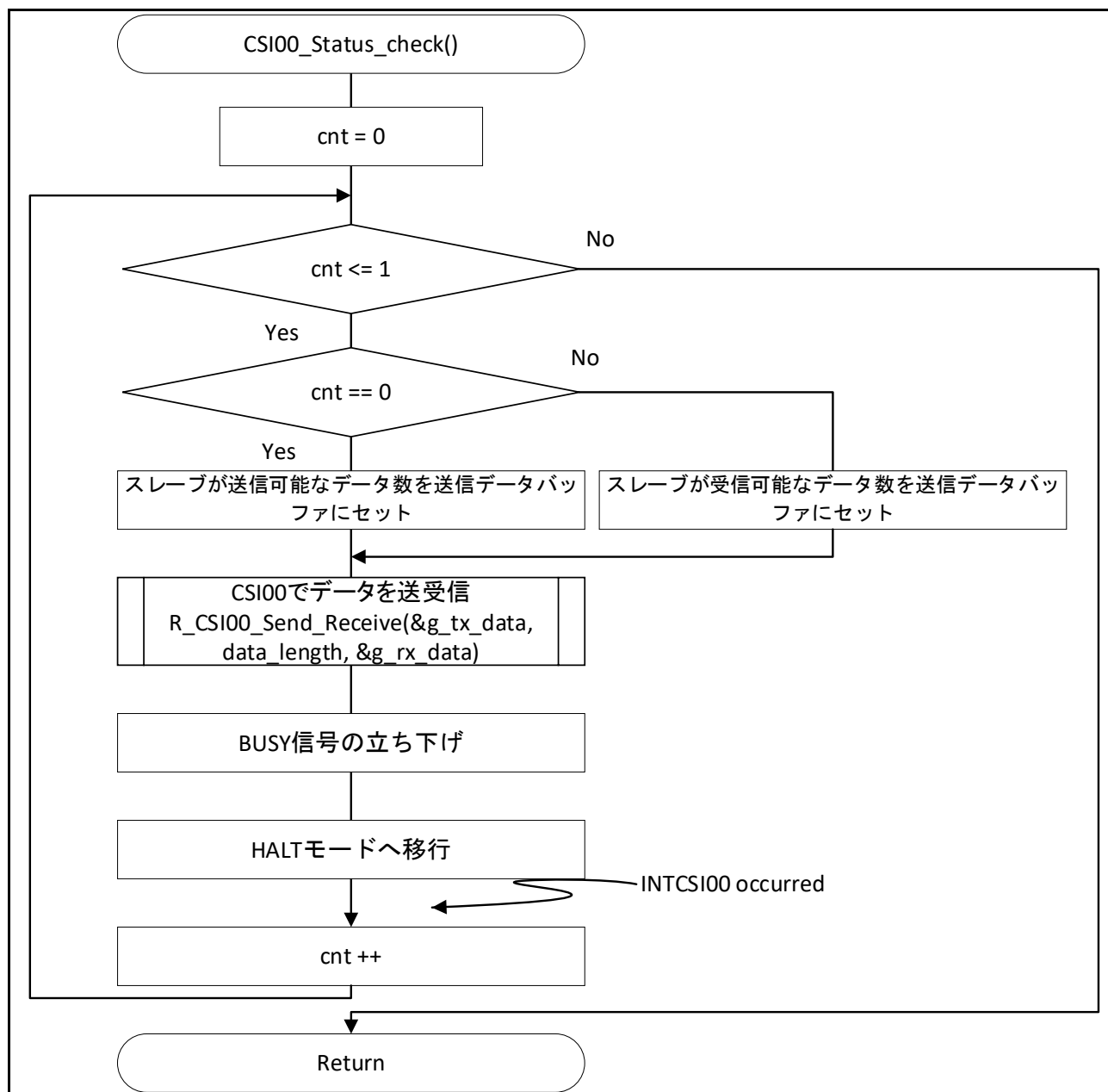
図 5-14 CSI ステータス確認処理
