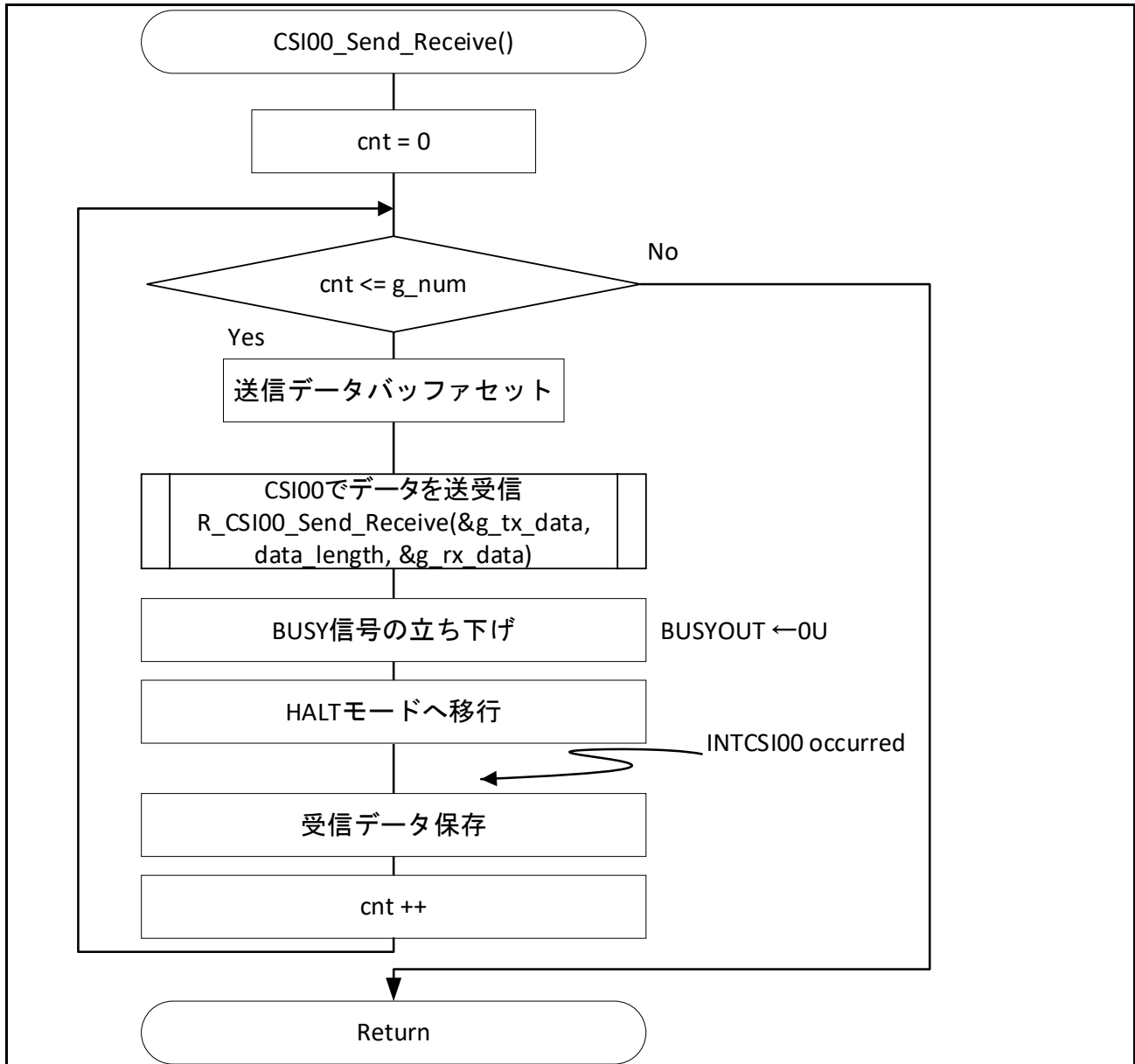
図 5-15 CSI 送受信処理
