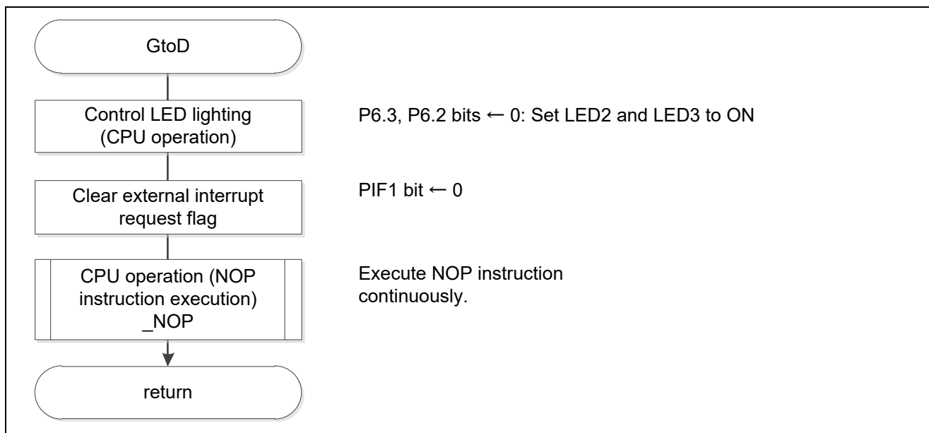
Figure 5.15 Status Transition GtoD
