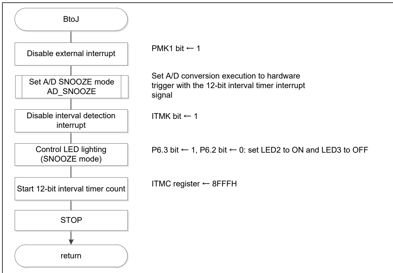
Figure 5.34 Status Transition BtoJ
