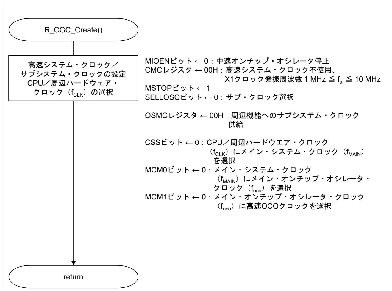
図 5.5 CPU クロックの設定
