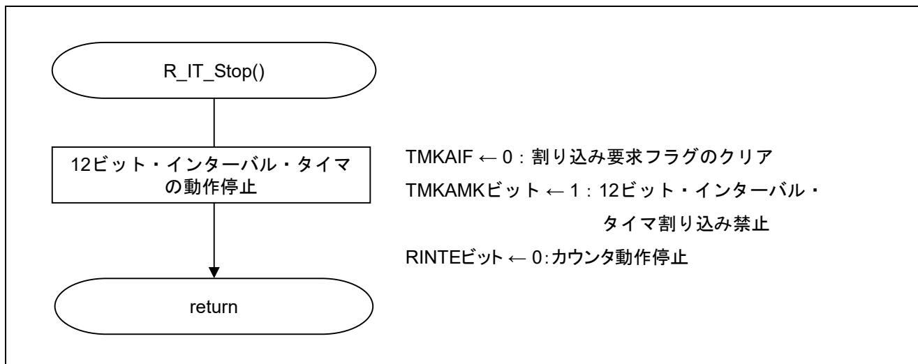
図 5.16 12 ビット・インターバル・タイマ停止処理関数
