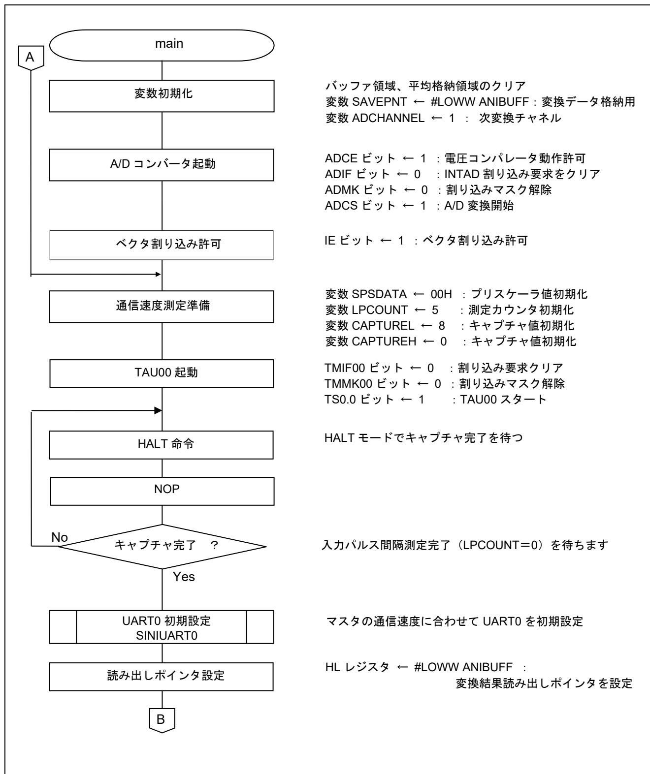
図 5.8 メイン処理(1/3)
