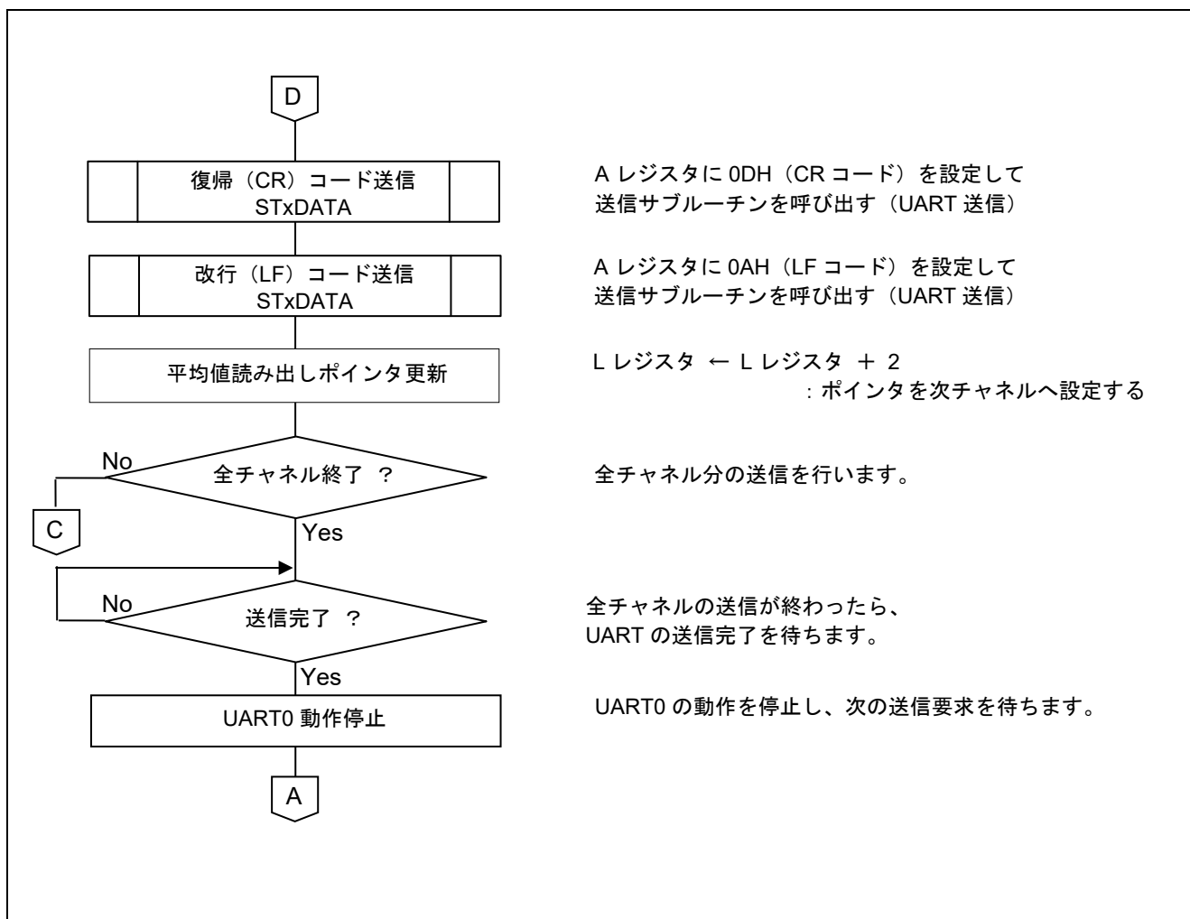
図 5.10 メイン処理(3/3)
