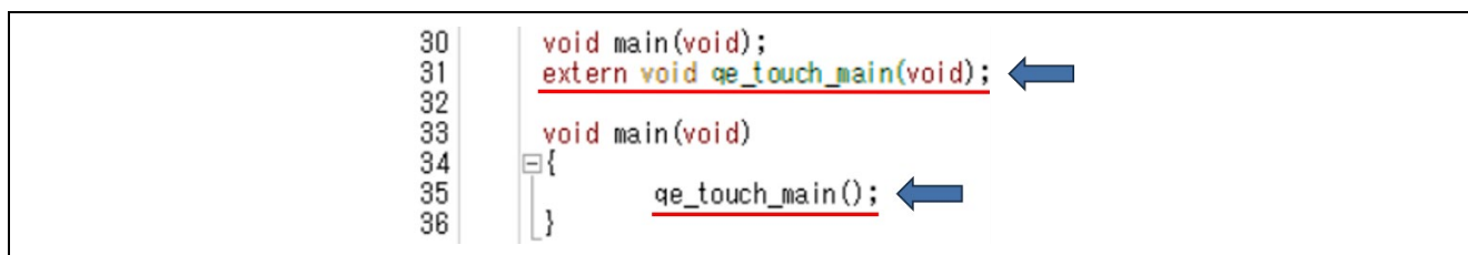
図 8-26 main.c
