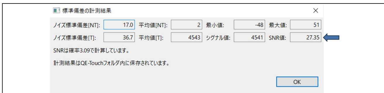
図 8-51 SNR 値
