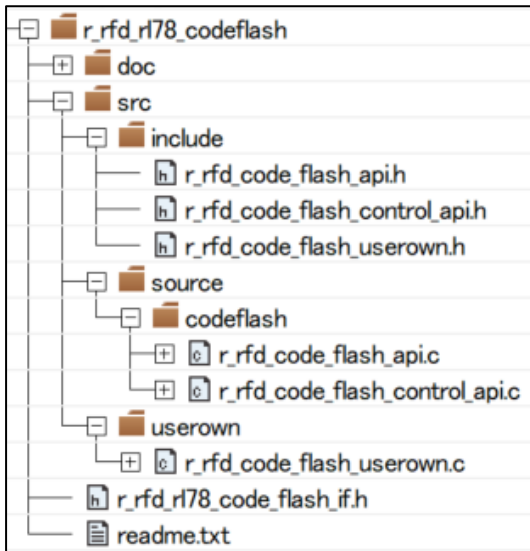
展開時の r_rfd_rl78_codeflash フォルダ
