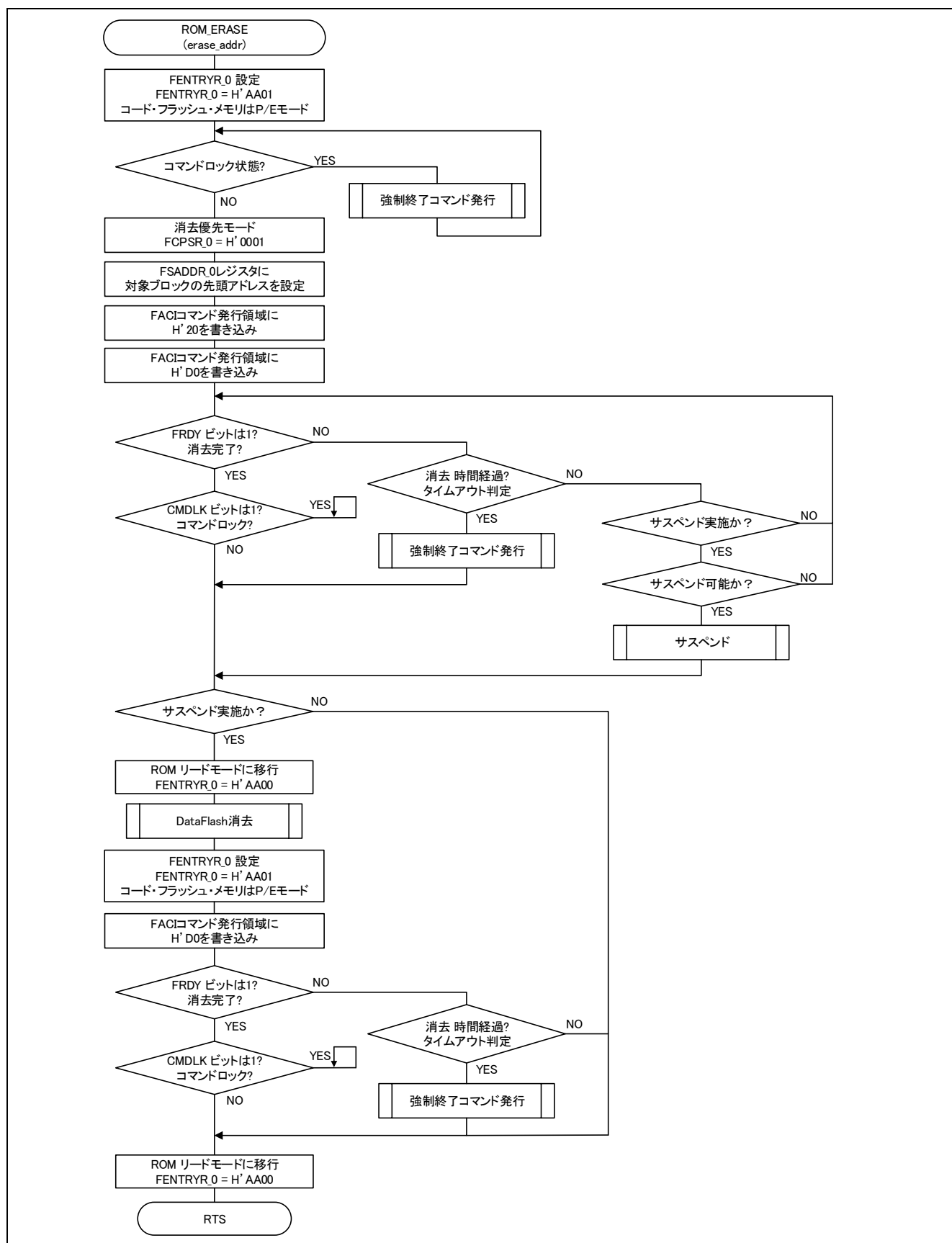
図 3-8 「Code Flash_ERASE()関数」のフローチャート
