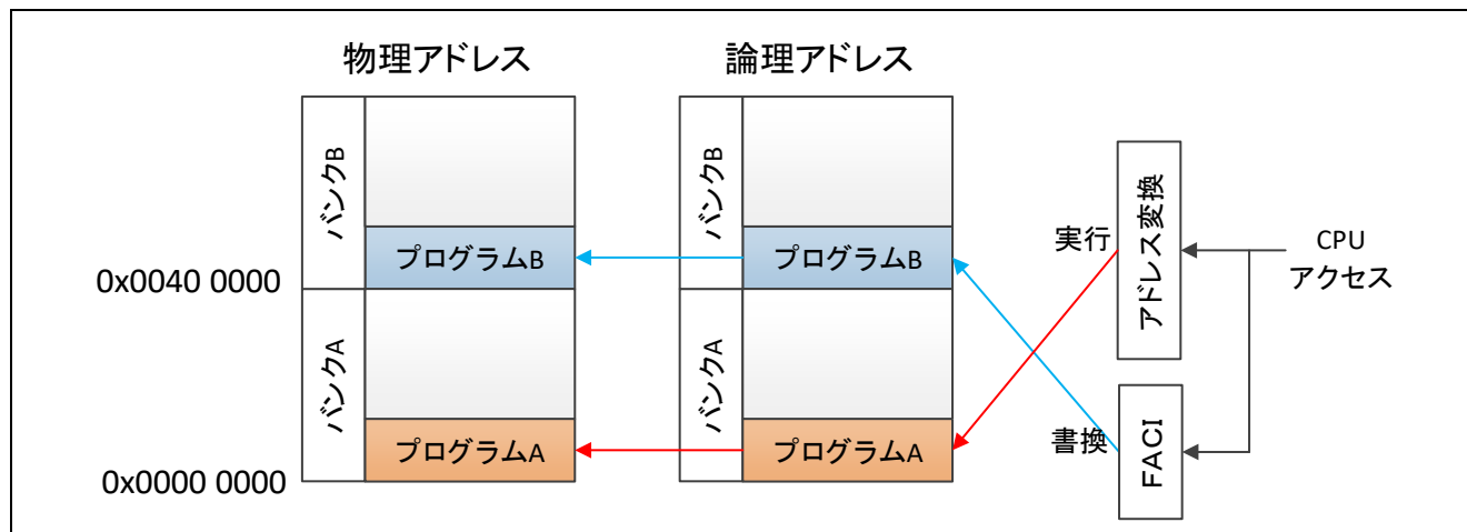
図 1-3 プログラム A 起動での書き込み動作
