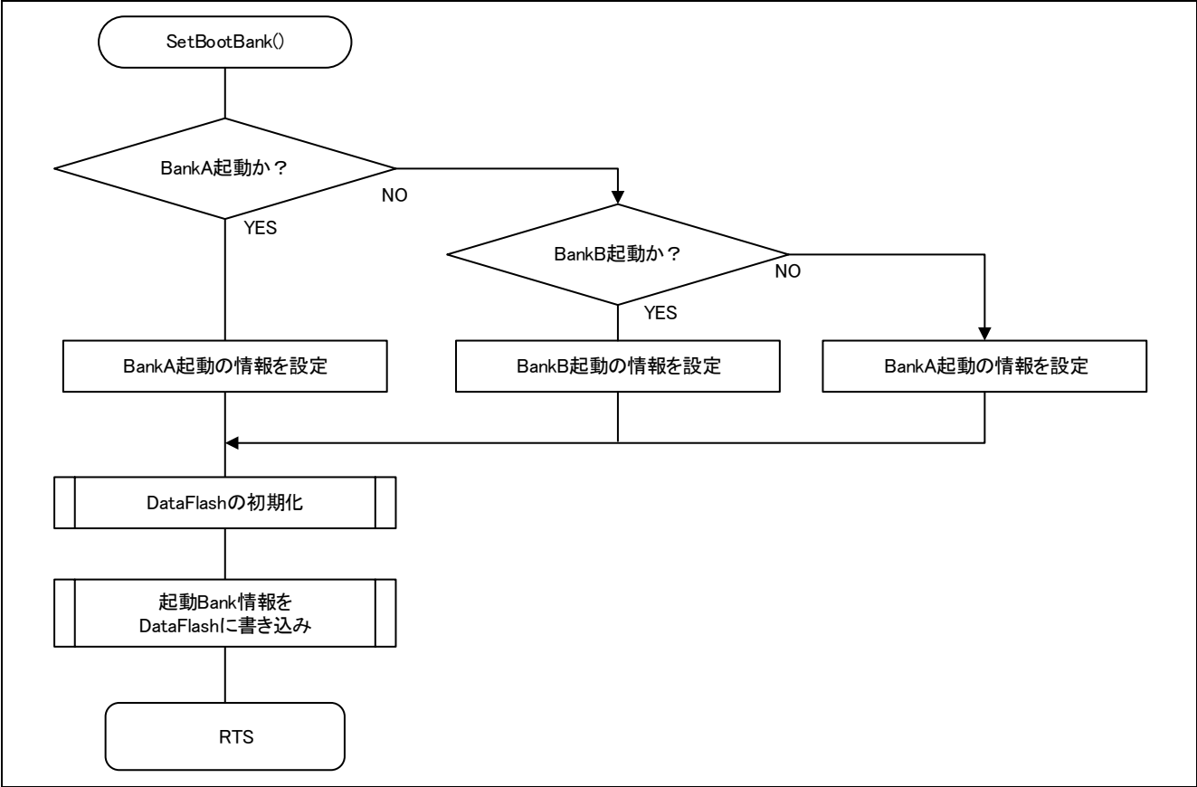
図 3-12 「SetBootBank ()関数」のフローチャート 「動作手順⑦」
