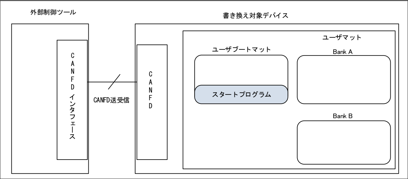
図 3-1 スタートアッププログラム動作
