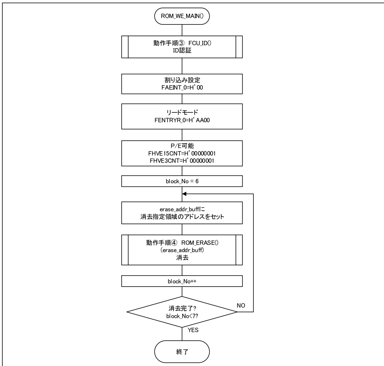
図 3-6 「Code Flash_WE_MAIN()関数」のフローチャート
