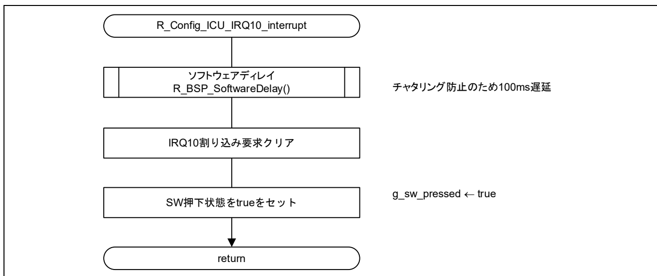
図 4-11 IRQ10 割り込み処理
