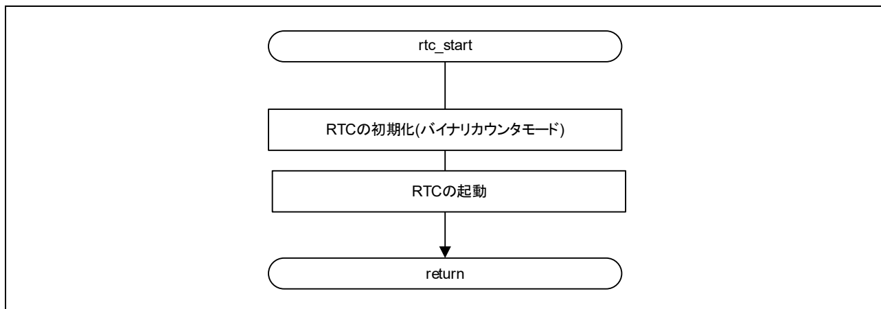
図 4-9 RTC の初期設定
