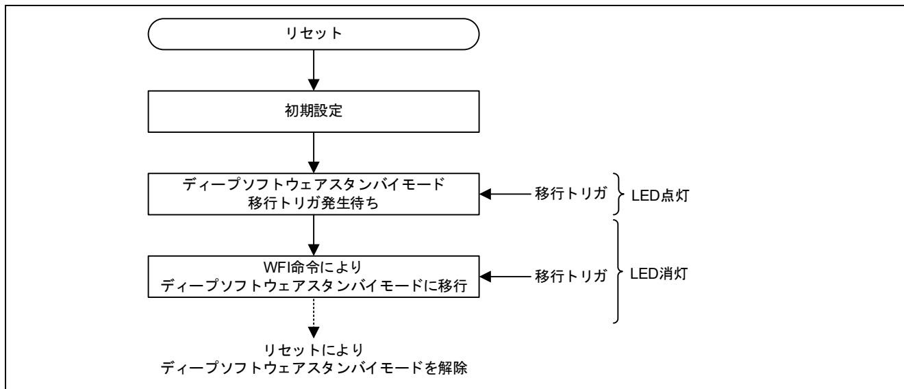
図 4-3 ディープソフトウェアスタンバイモードの動作概要(リセットによるモード解除)
