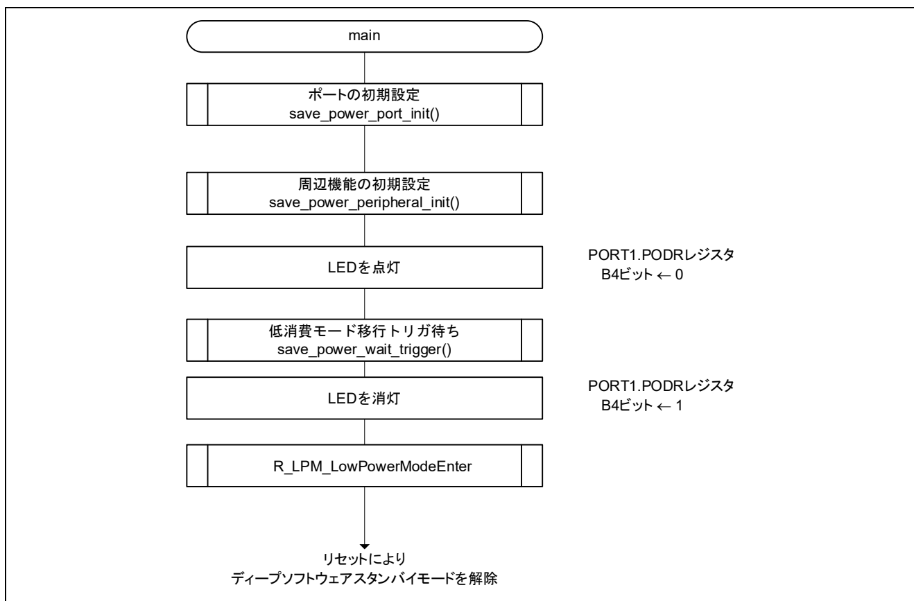
図 4-7 ディープソフトウェアスタンバイモードに遷移するサンプルプログラムのメイン処理
