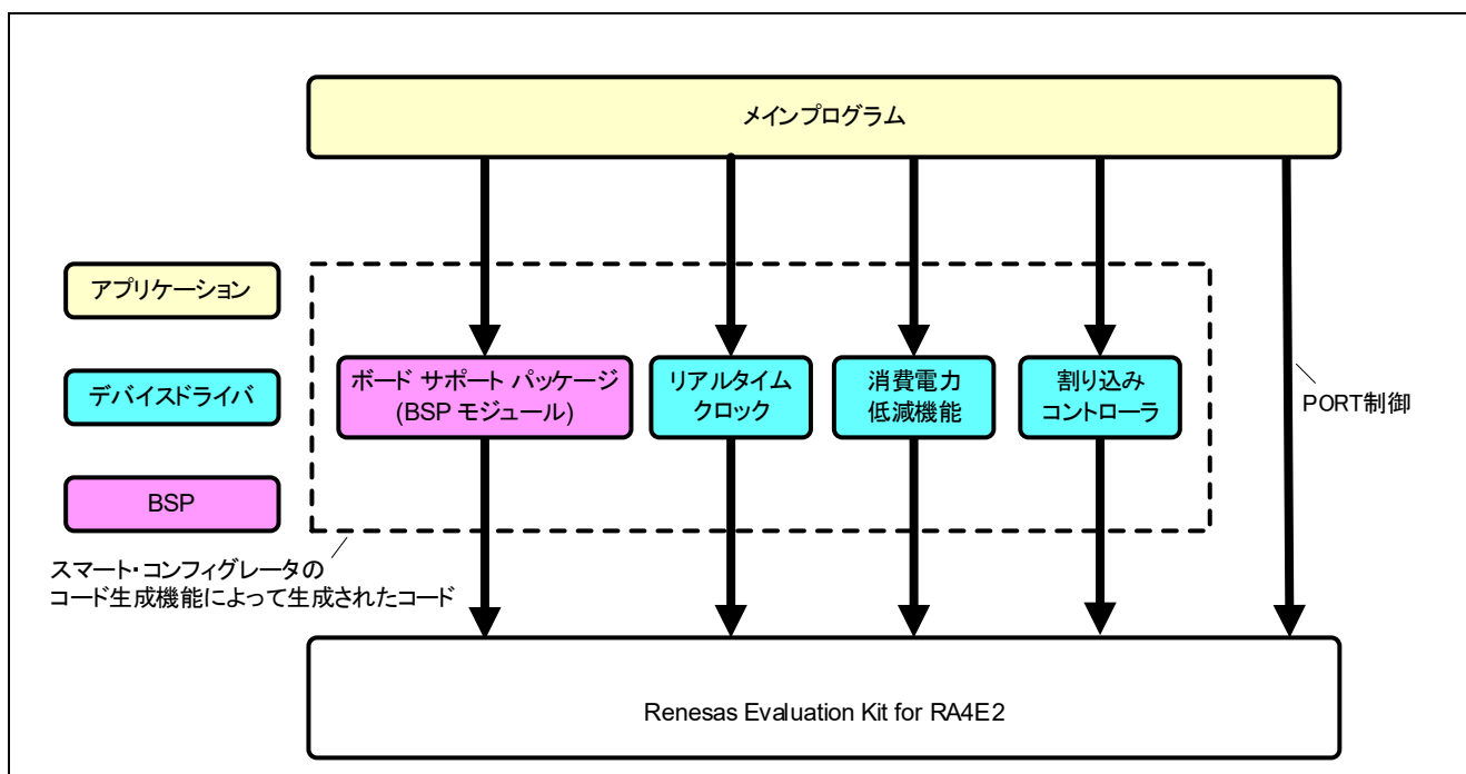
図 4-4 モジュール構成
