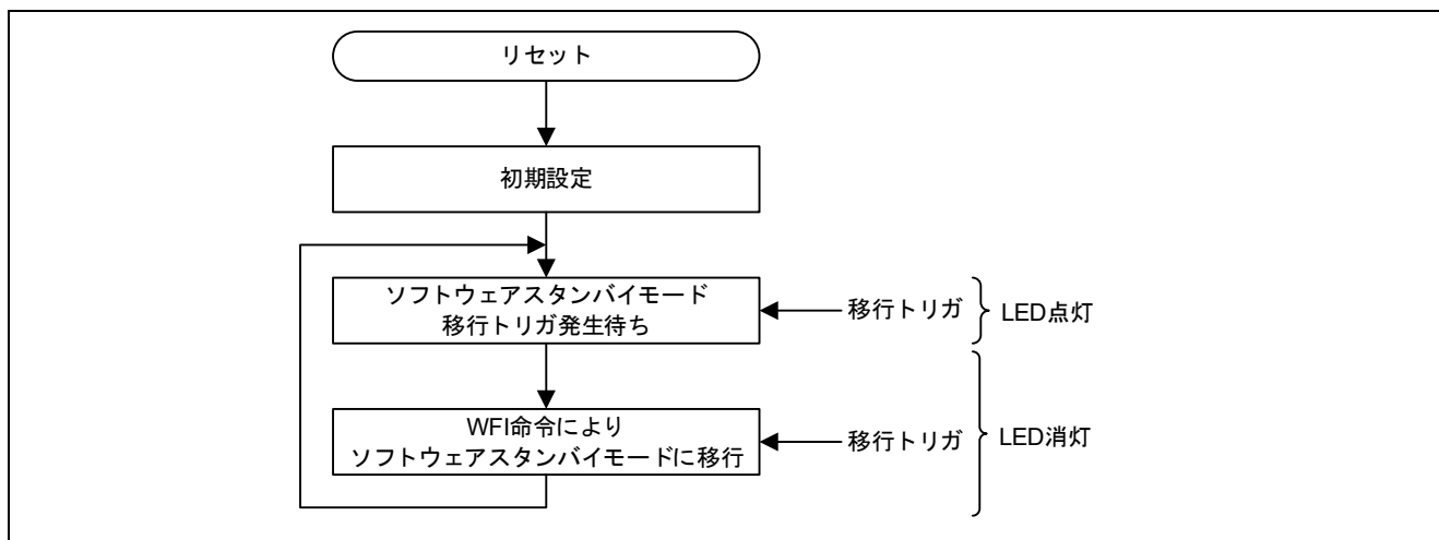
図 4-2 ソフトウェアスタンバイモードの動作概要
