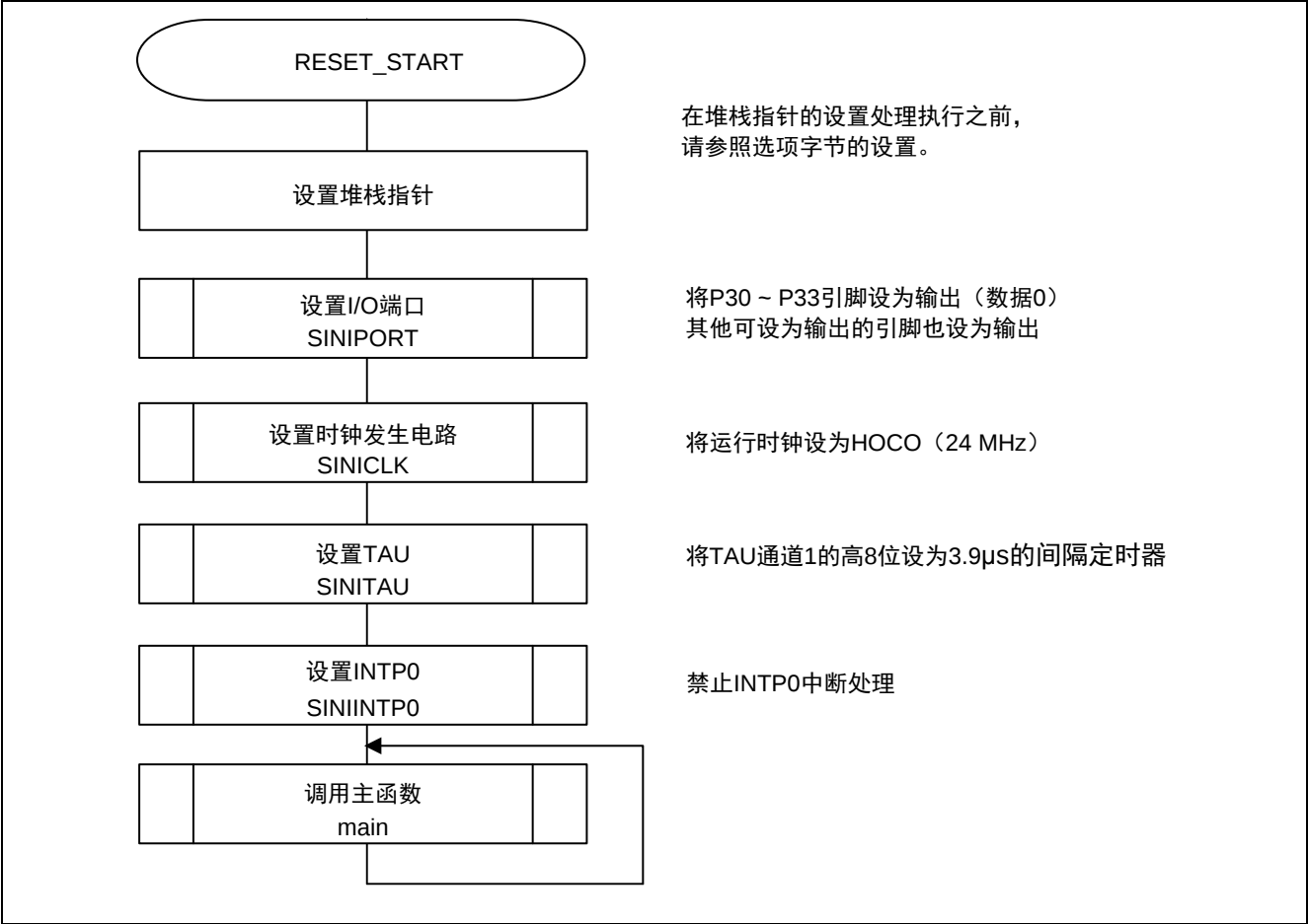
图 4.2 整体流程图
