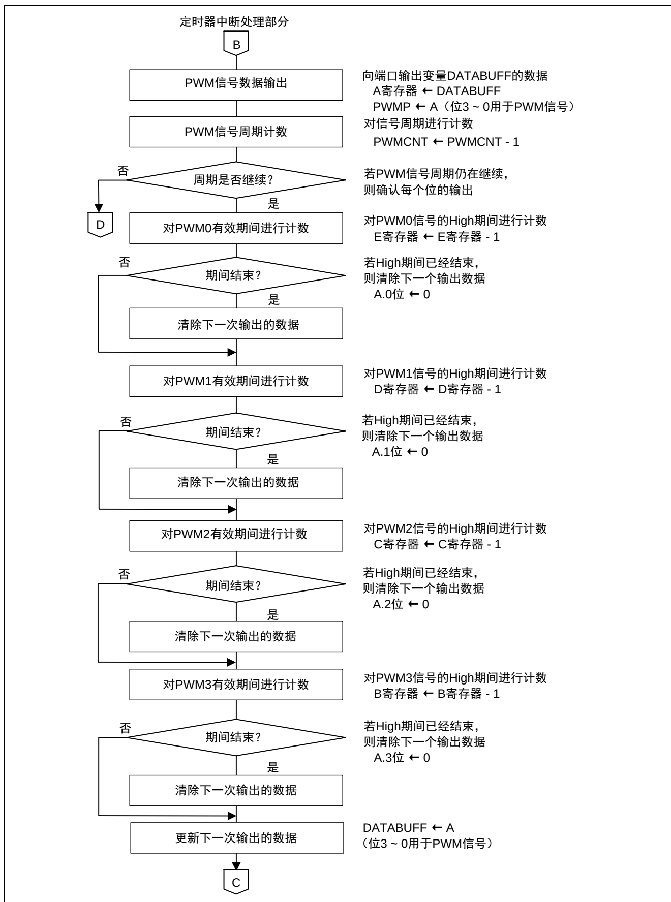
图 4.8 主函数处理 (2/3)
