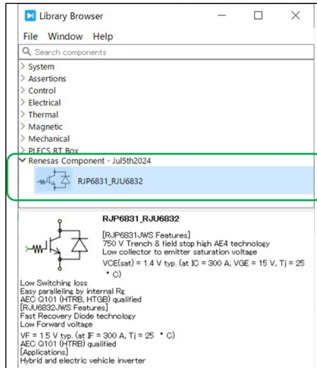
図 1-1 PLECS モデル
