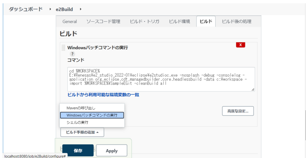
図 21 「ビルド」タブ
