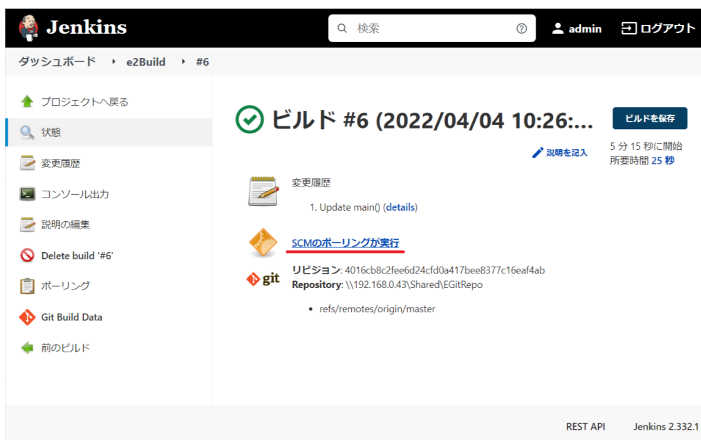
図 25 Git リポジトリ更新後のビルド結果
