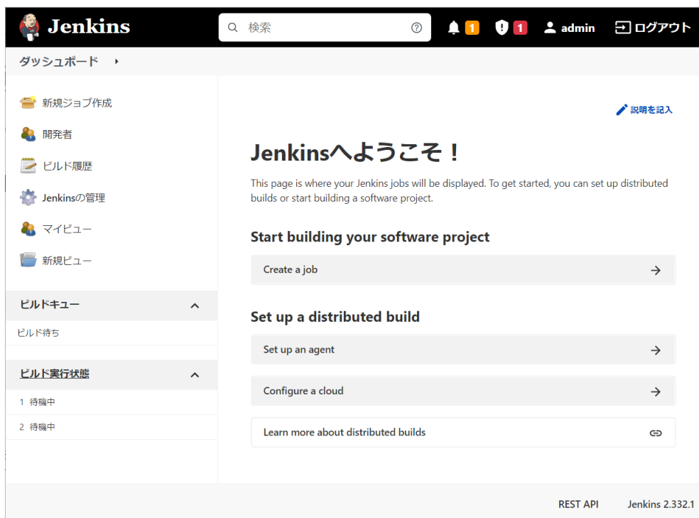
図 5 [Jenkins] ページ
