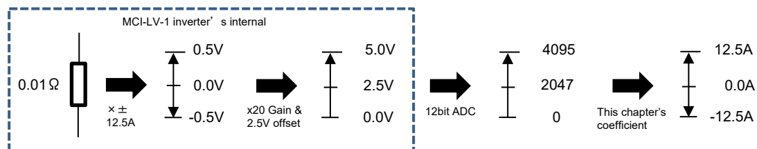
図 9-1 電流検出の計算の流れ
