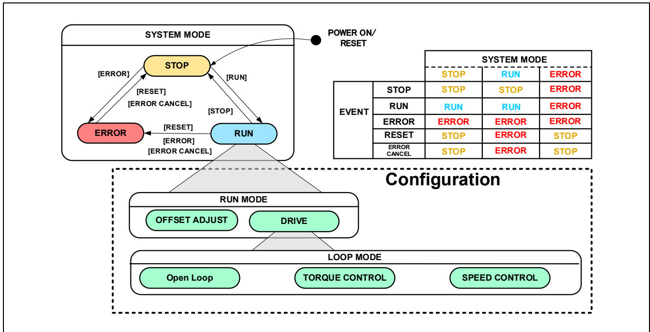
図 8-3 ホールセンサベクトル制御ソフトウェアの状態遷移図
