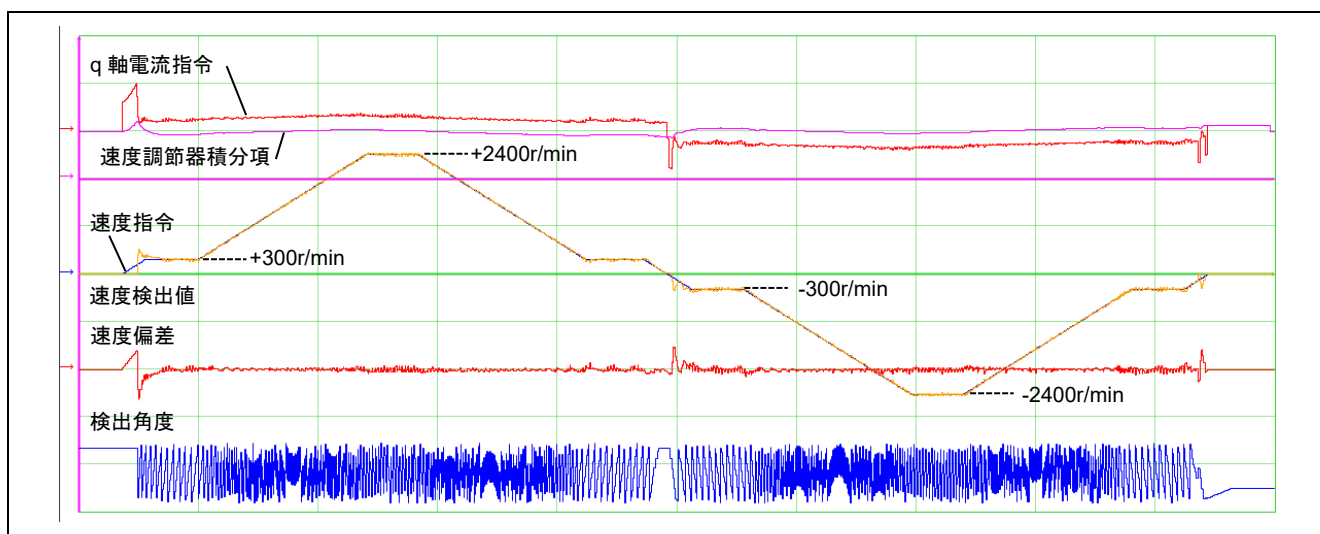
図 1-1 加減速および正転逆転特性
