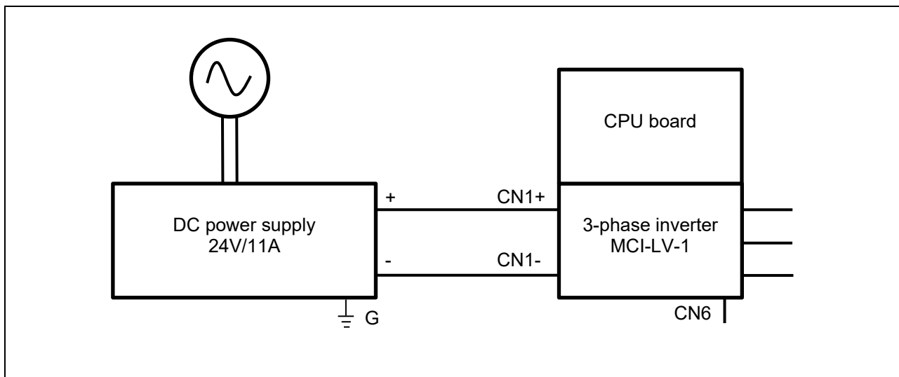
図 4-7 電源～インバータ間の配線
