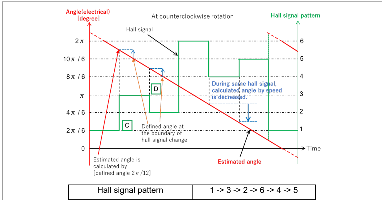
図 7-12 電気角度推定 (逆方向回転時)
