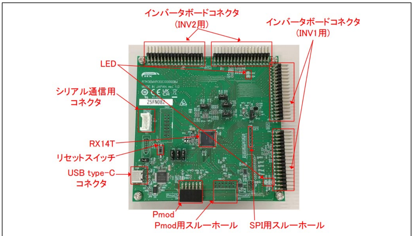
図 4-3 RX14T CPU ボードとインタフェース
