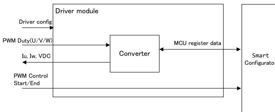
図 8-6 ドライバモジュール構成図
