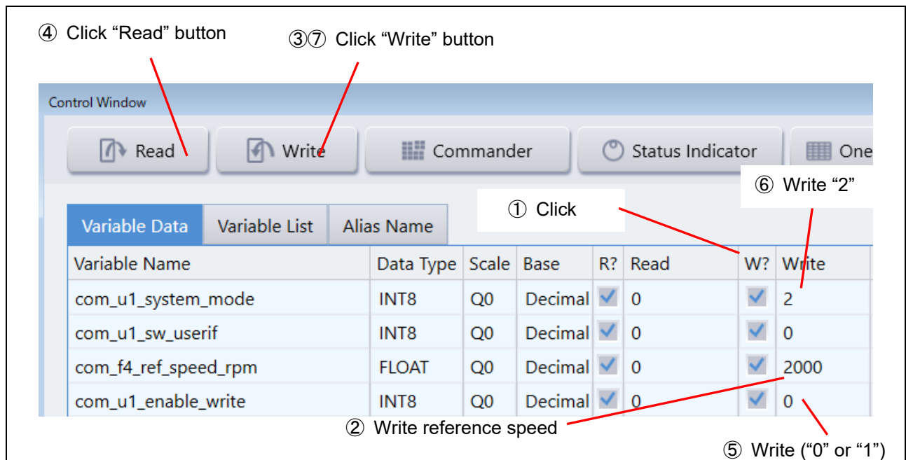
図 6-6 モータ回転の手順
