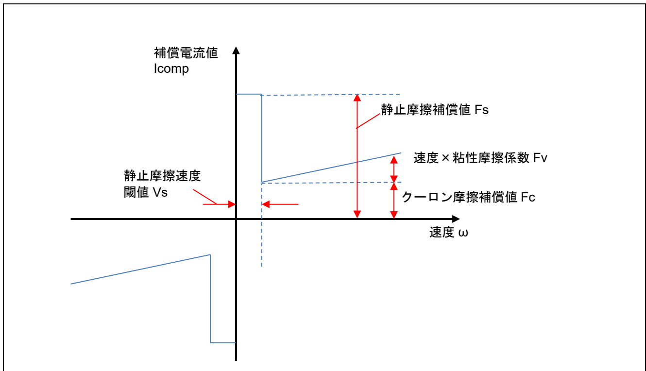
図 7-14 摩擦補償の概念図
