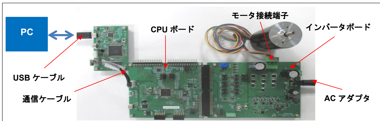
図 4-4 キットの接続例
