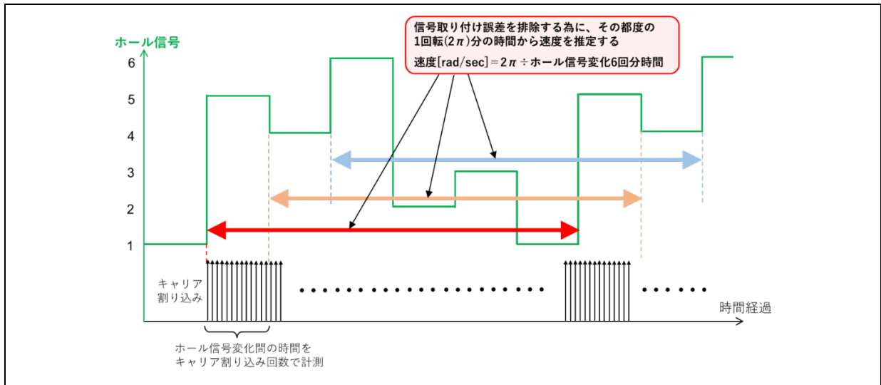
図 7-10 速度推定概念図
