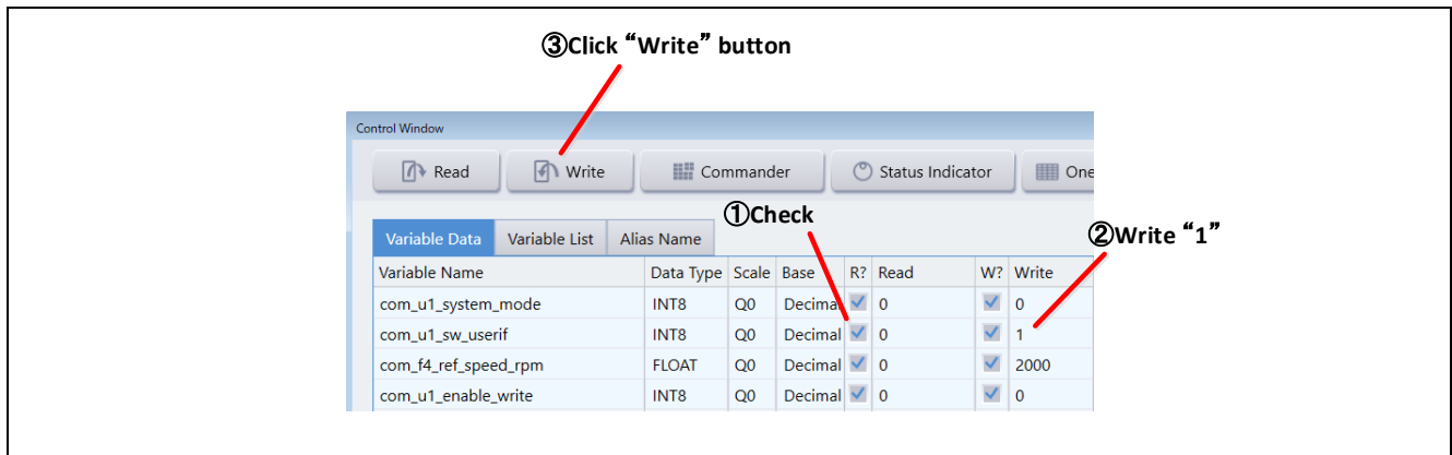
図 6-9 RMW・ボード UI の切り替えの手順
