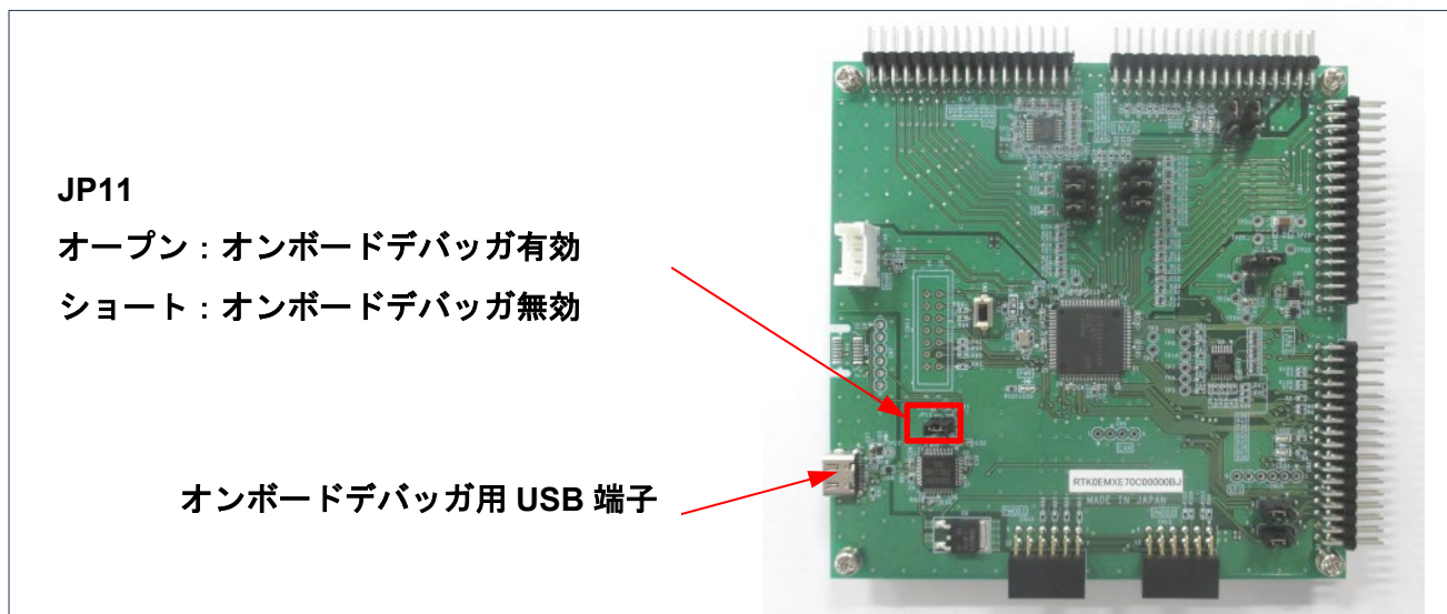
図 6-1 オンボードデバッグ(RX26T)
