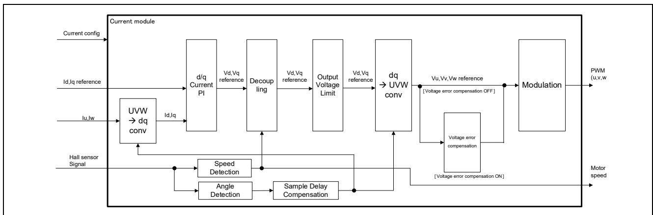
図 7-6 電流制御の機能ブロック図
