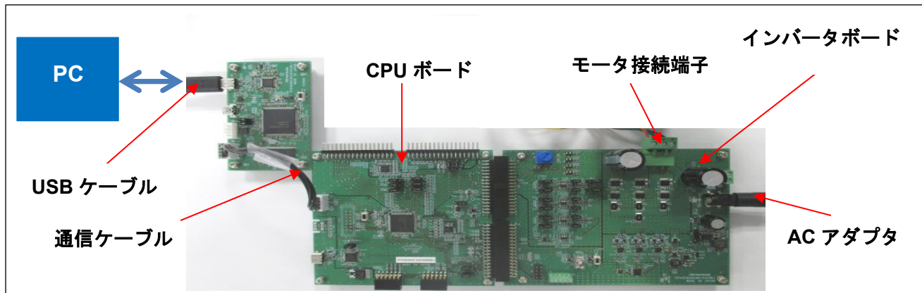
図 6-3 運転操作時の接続例
