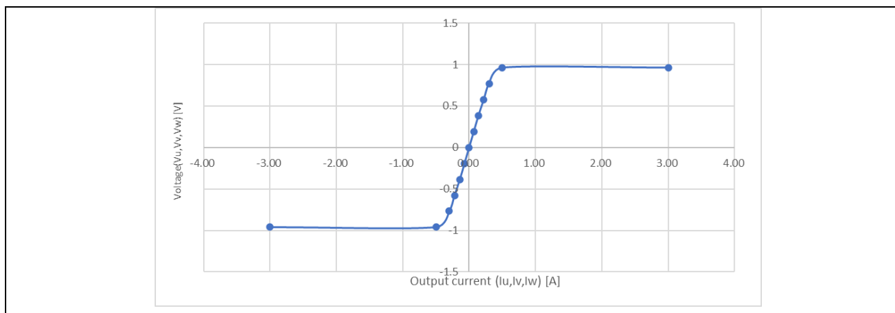
図 7-16 電圧誤差の電流依存性(一例)
