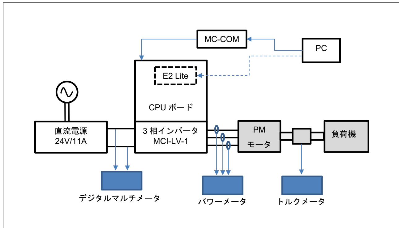
図 4-9 測定器の追加例
