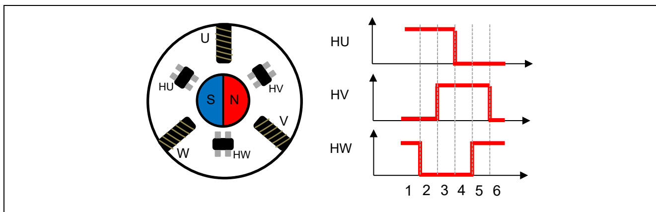
図 7-9 ホールセンサ配置とホールセンサ信号
