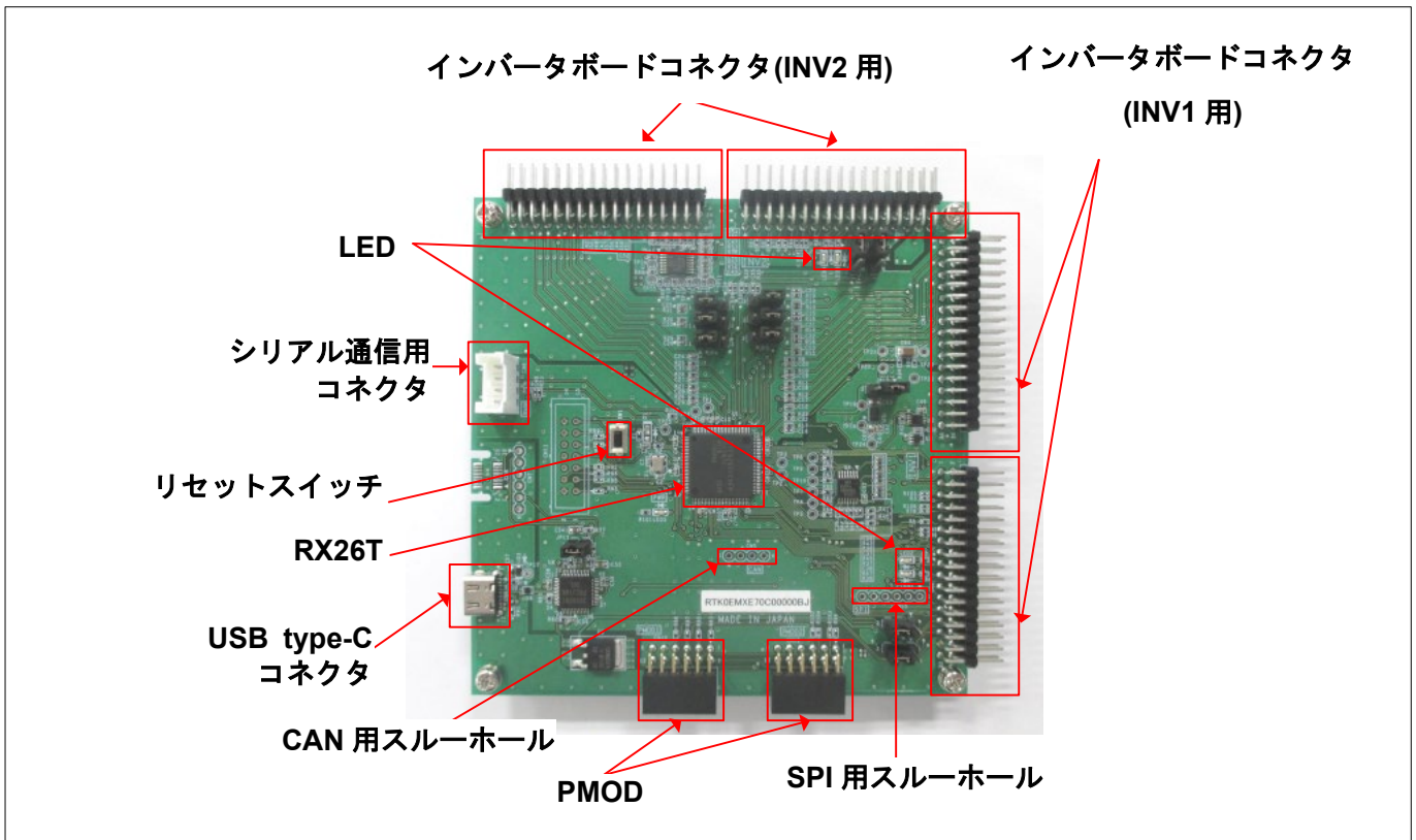
図 4-2 RX26T CPU ボードとインタフェース
