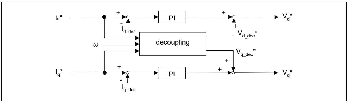
図 7-7 非干渉制御の機能ブロック図
