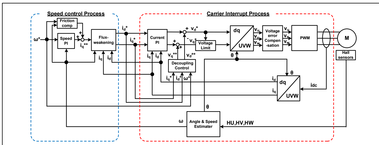
図 7-1 ホールセンサベクトル制御概略ブロック図
