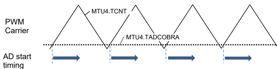
図 10-1 AD 検出開始タイミング
