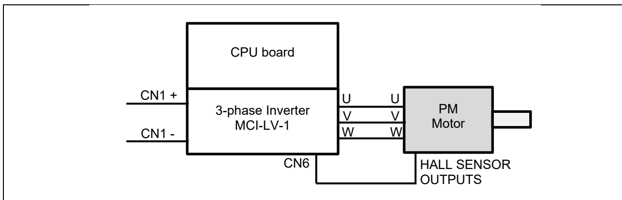
図 4-8 インバータ～モータ間の配線
