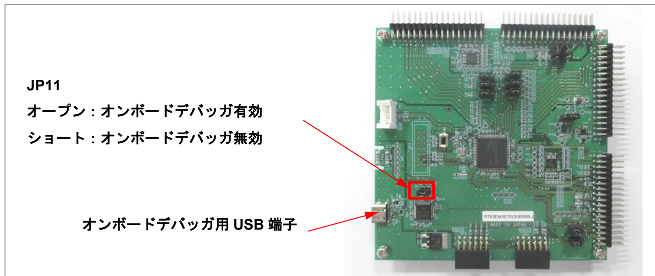
図 4-5 オンボードデバッグ(RX26T)
