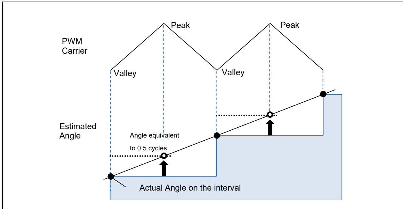
図 7-15 PWM キャリア周期で進む角度量の例
