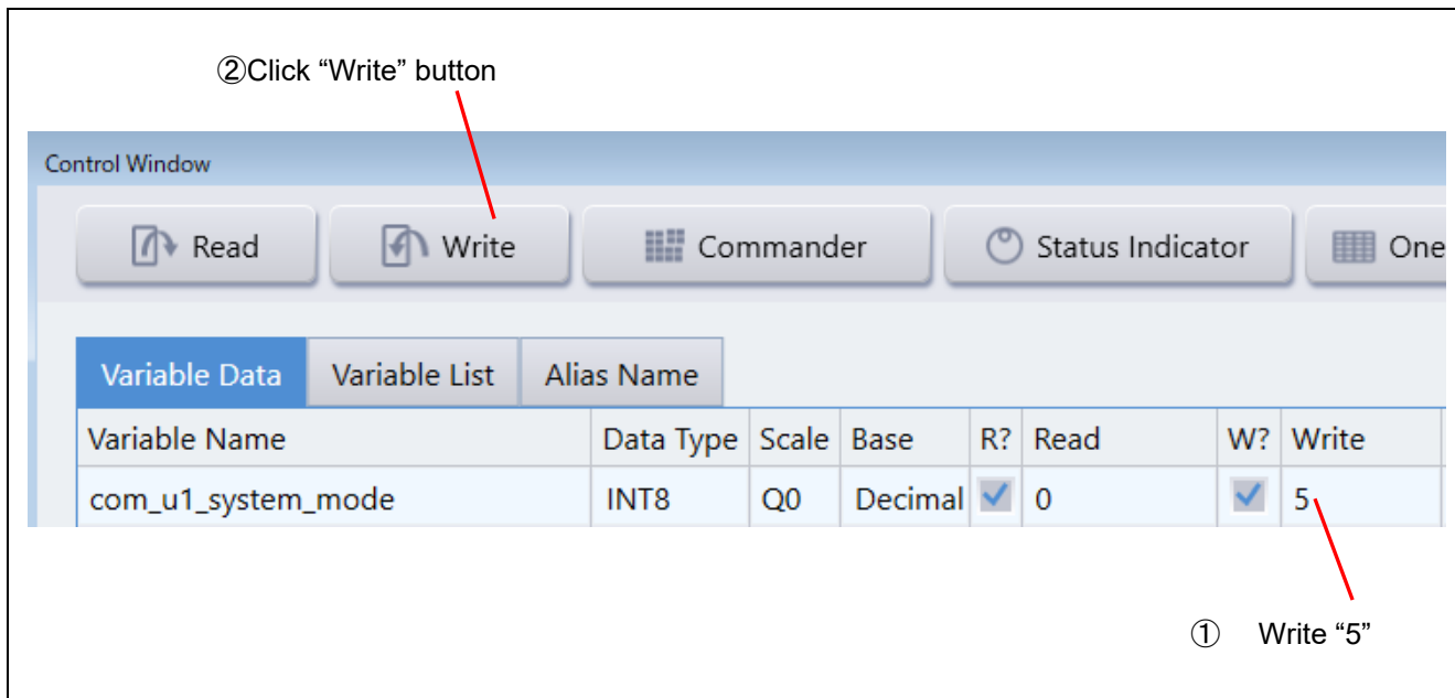
図 6-8 エラー解除の手順
