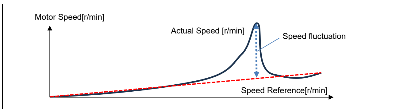
図 7-8 始動時の速度変動
