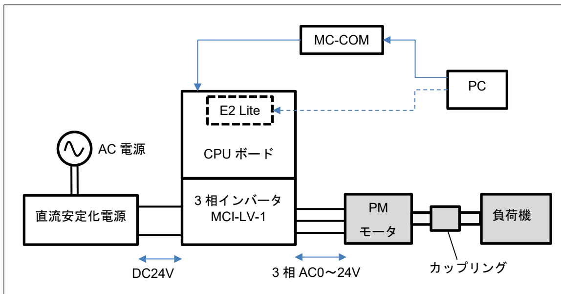
図 4-1 ハードウェア構成例
