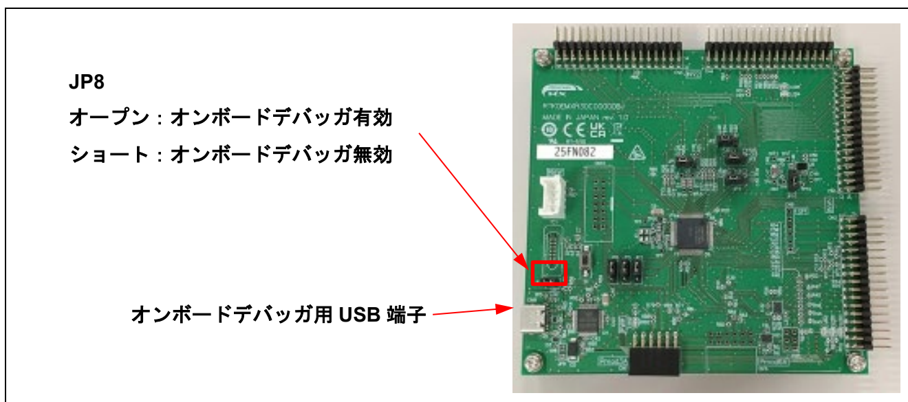
図 6-2 オンボードデバッグ(RX14T)
