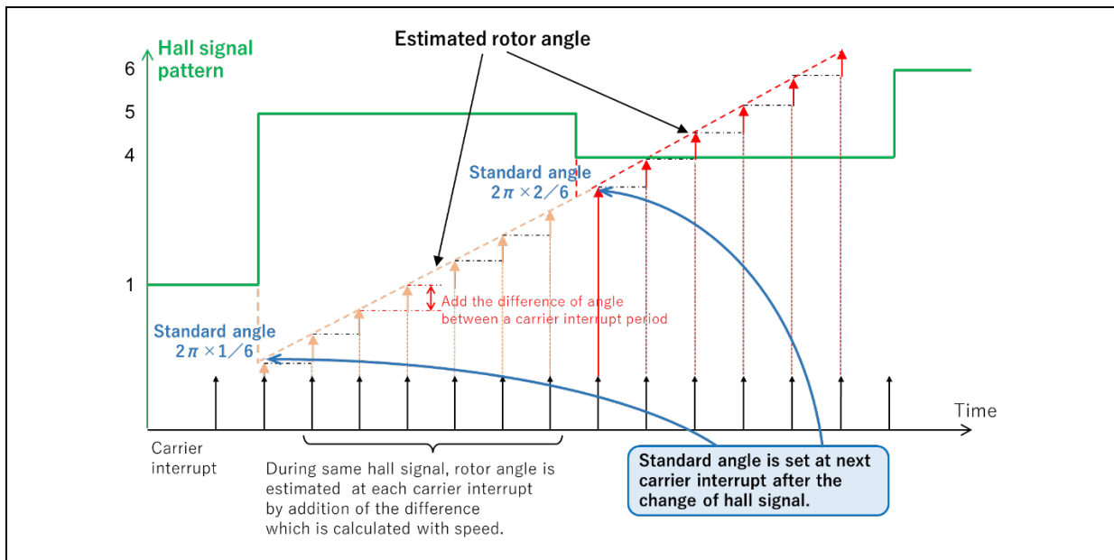
図 7-13 ホール信号内角度推定概念図(正方向回転時)
