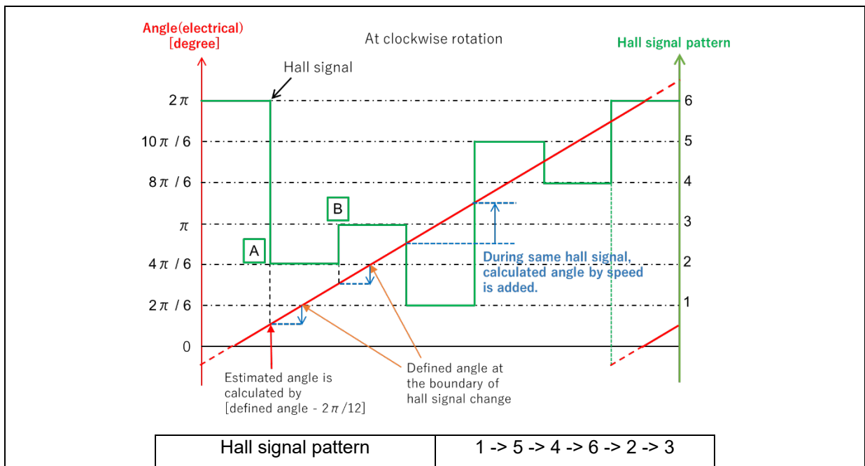
図 7-11 電気角度推定 (正方向回転時)
