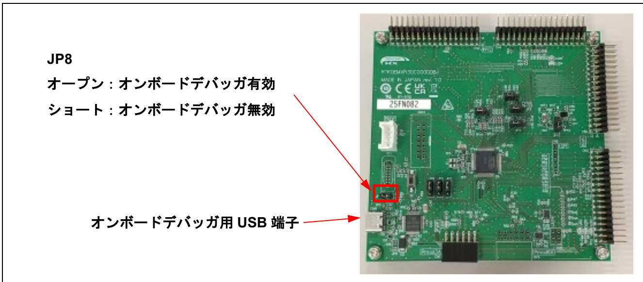
図 4-6 オンボードデバッグ(RX14T)
