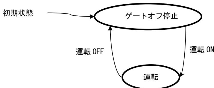
図 8-4 運転シーケンスの状態遷移図
