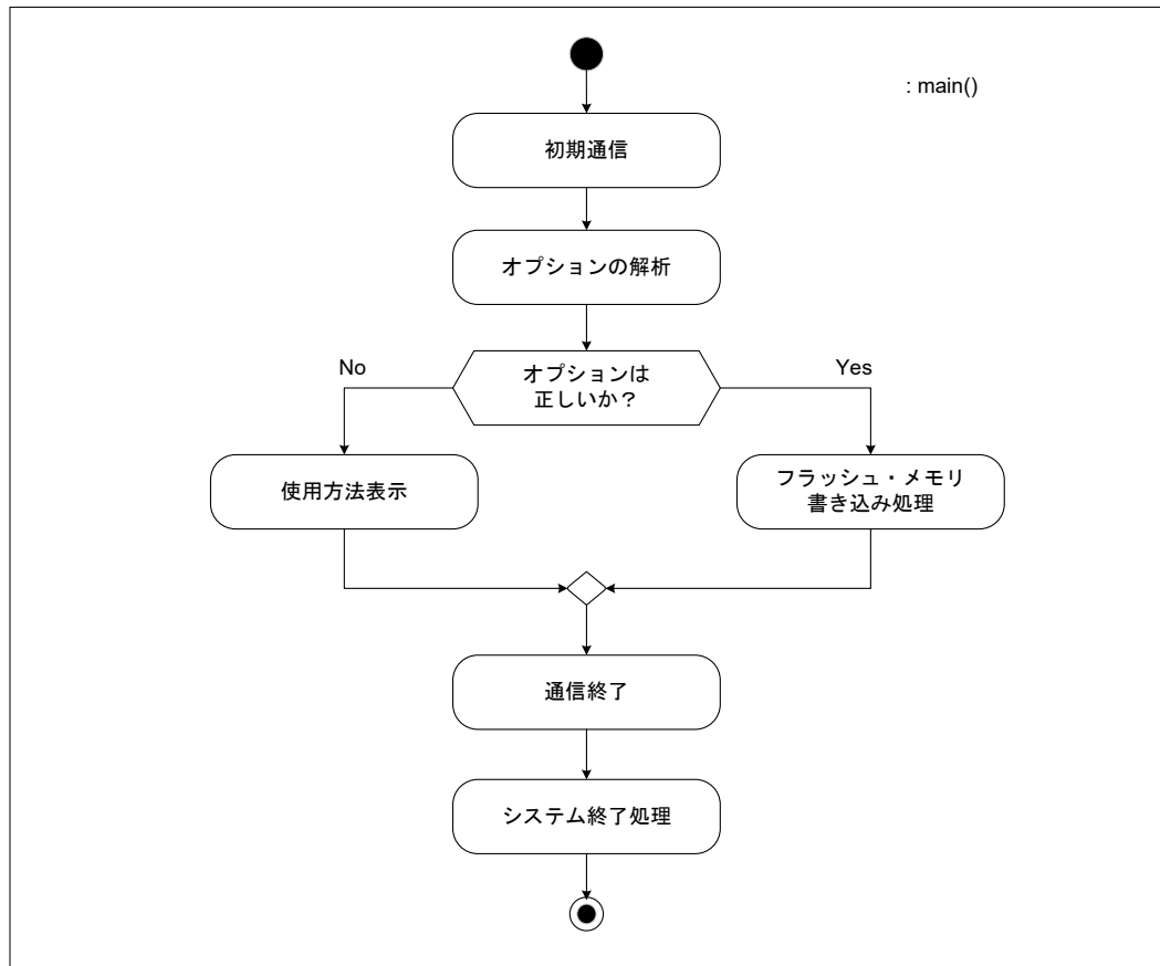
図 4-3 メインルーチン
