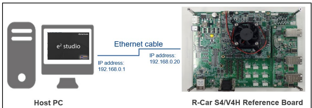
図 2-1 Host PC と Reference Board の接続図
