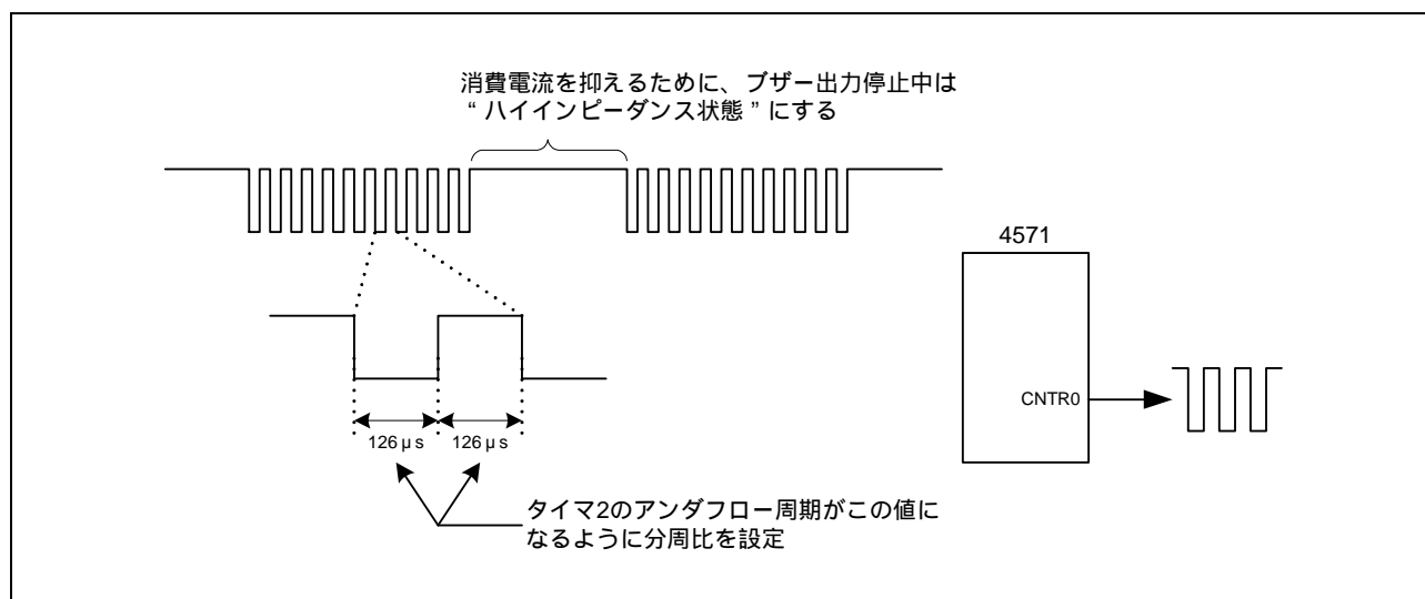
図 4.1 周辺回路例
