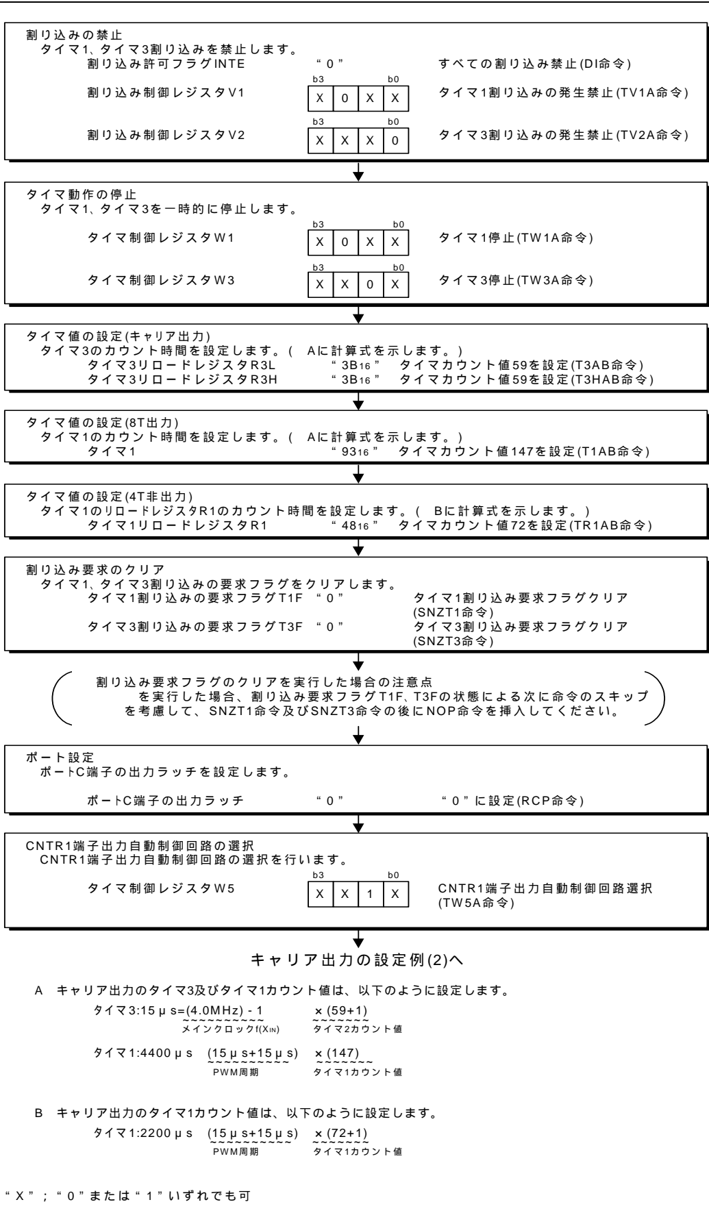
図 4.2 キャリア出力の設定例 (1)
