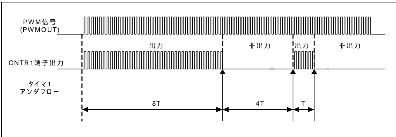
図 4.1 CNTR1 出力自動制御
