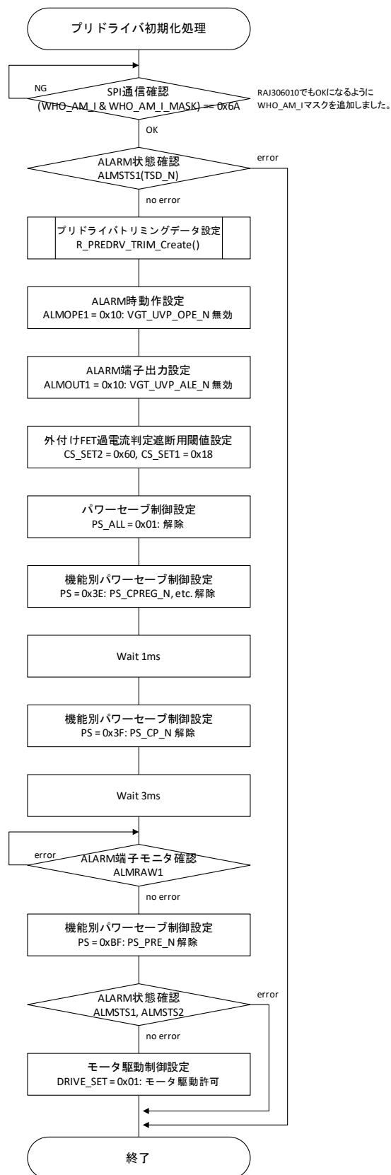
Figure 3-7 フローチャート(プリドライバ初期化処理)
