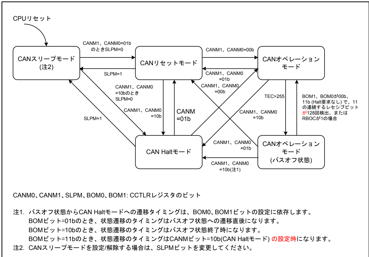
図 24.12 CAN 動作モード間の遷移
