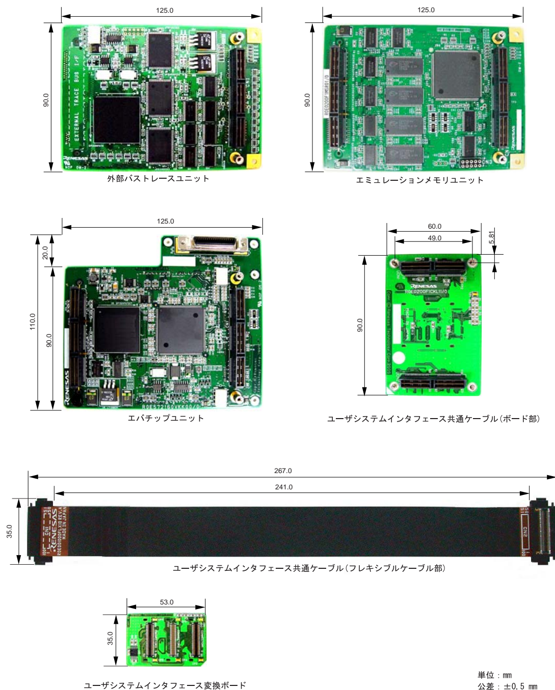
図 12 外部バストレースユニット、エミュレーションメモリユニット、エパチップユニット、ユーザシステムインタフェース共通ケーブル、およびボード本体部の外形寸法
