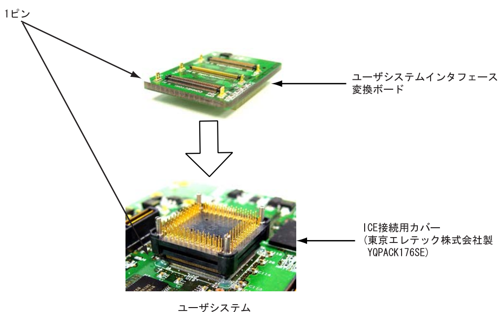
図7 ユーザシステムへの接続
