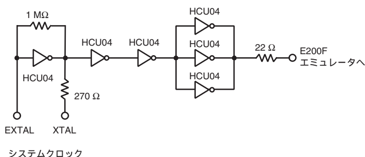
図 18 クロック発振回路
