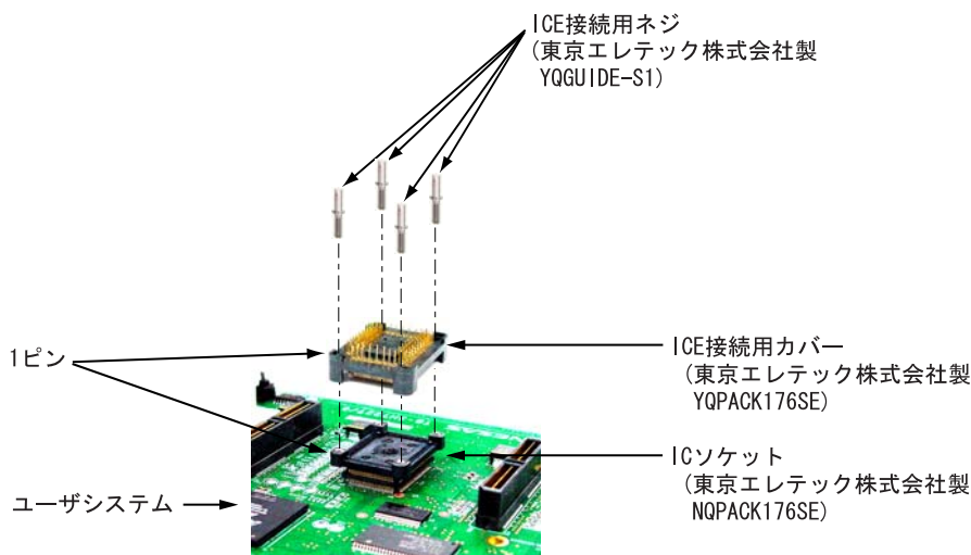
図2 ユーザシステムへの接続
