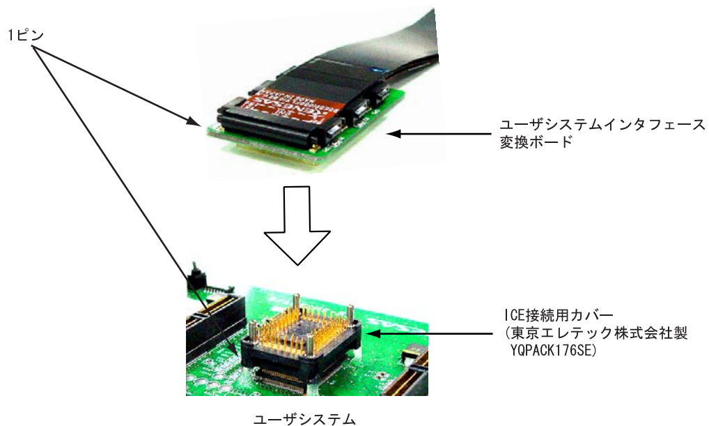
図 6 ユーザシステムへの接続
