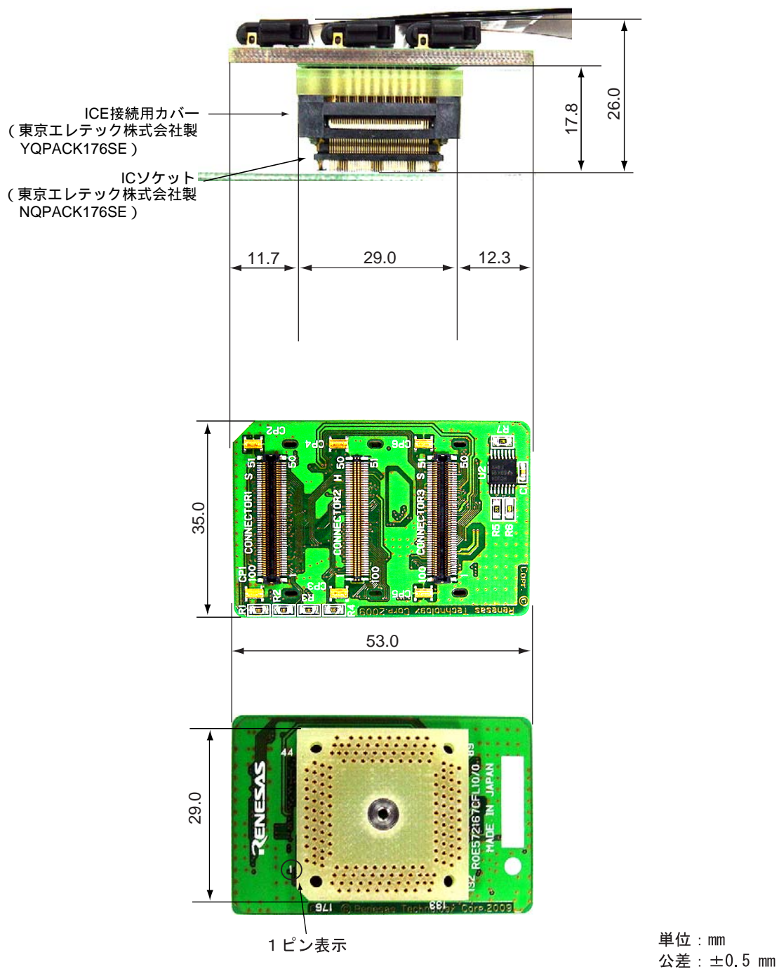
図 13 ユーザシステムインタフェース変換ボード接続時のユーザシステムとの寸法 (フレキシブルケーブル接続時)
