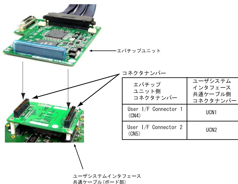
図 10 エバチップユニットとの接続
