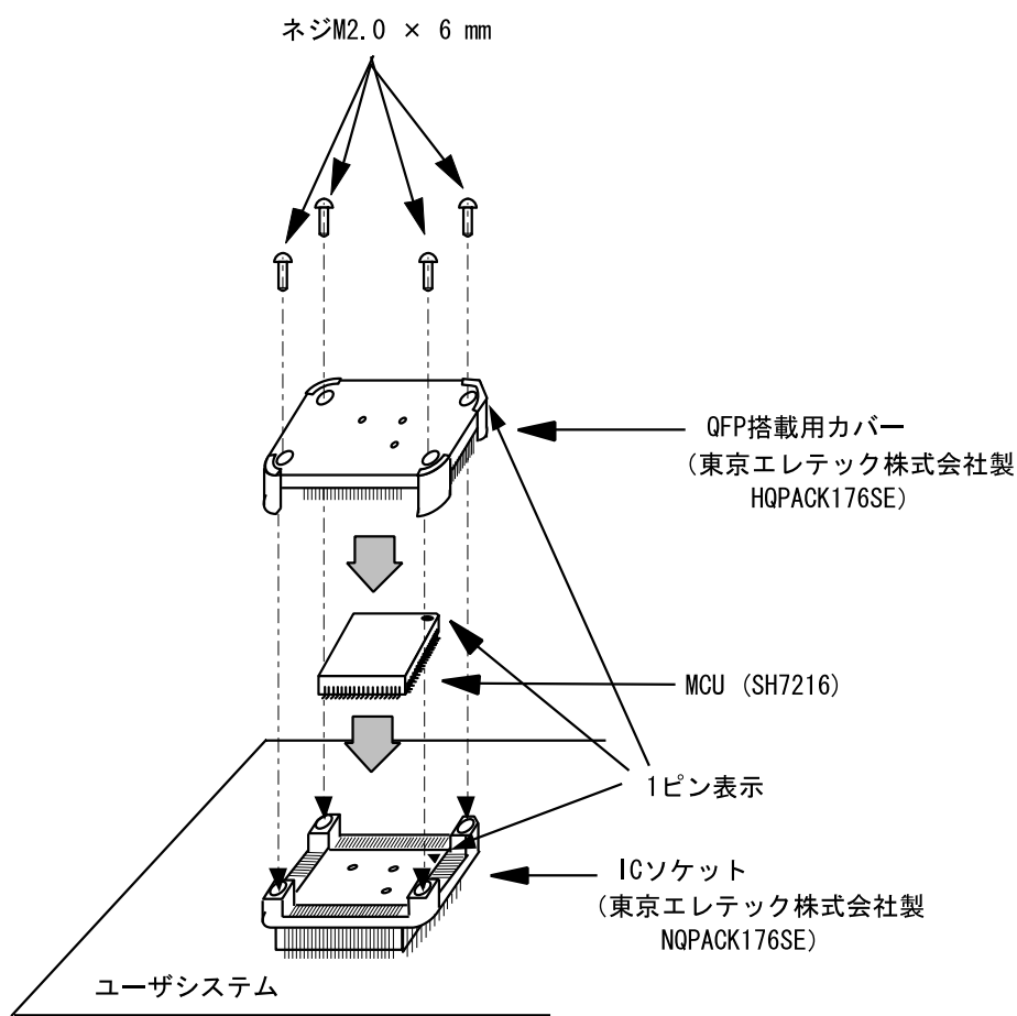
図 17 MCU をユーザシステムに実装する場合
