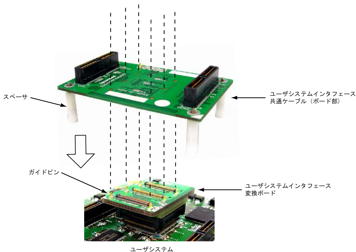
図8 ユーザシステムインタフェース共通ケーブル(ボード部)の接続
