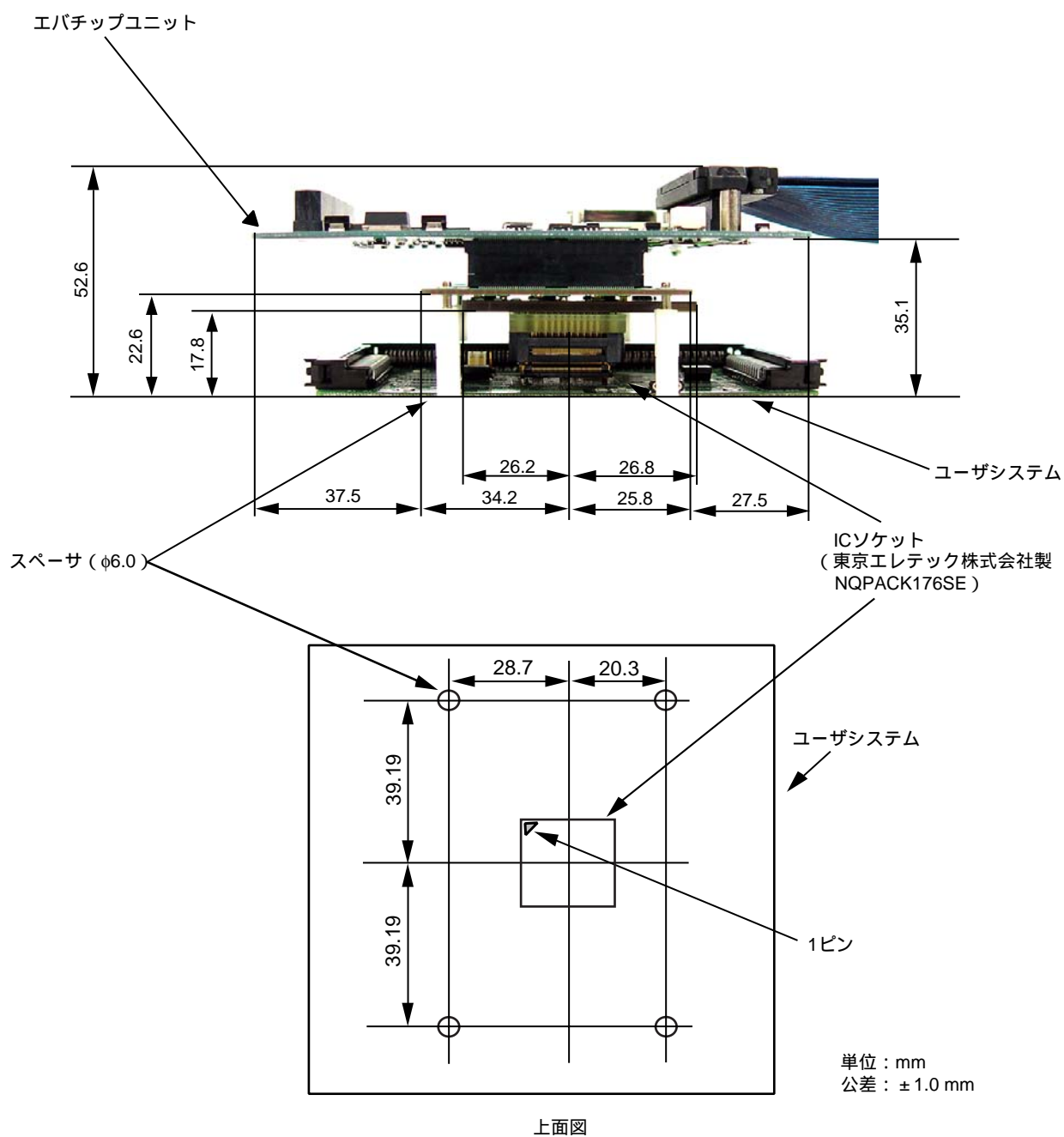
図 16 ユーザシステムインタフェース変換ボード接続時のユーザシステムとの寸法 (エバチップユニット接続時)
