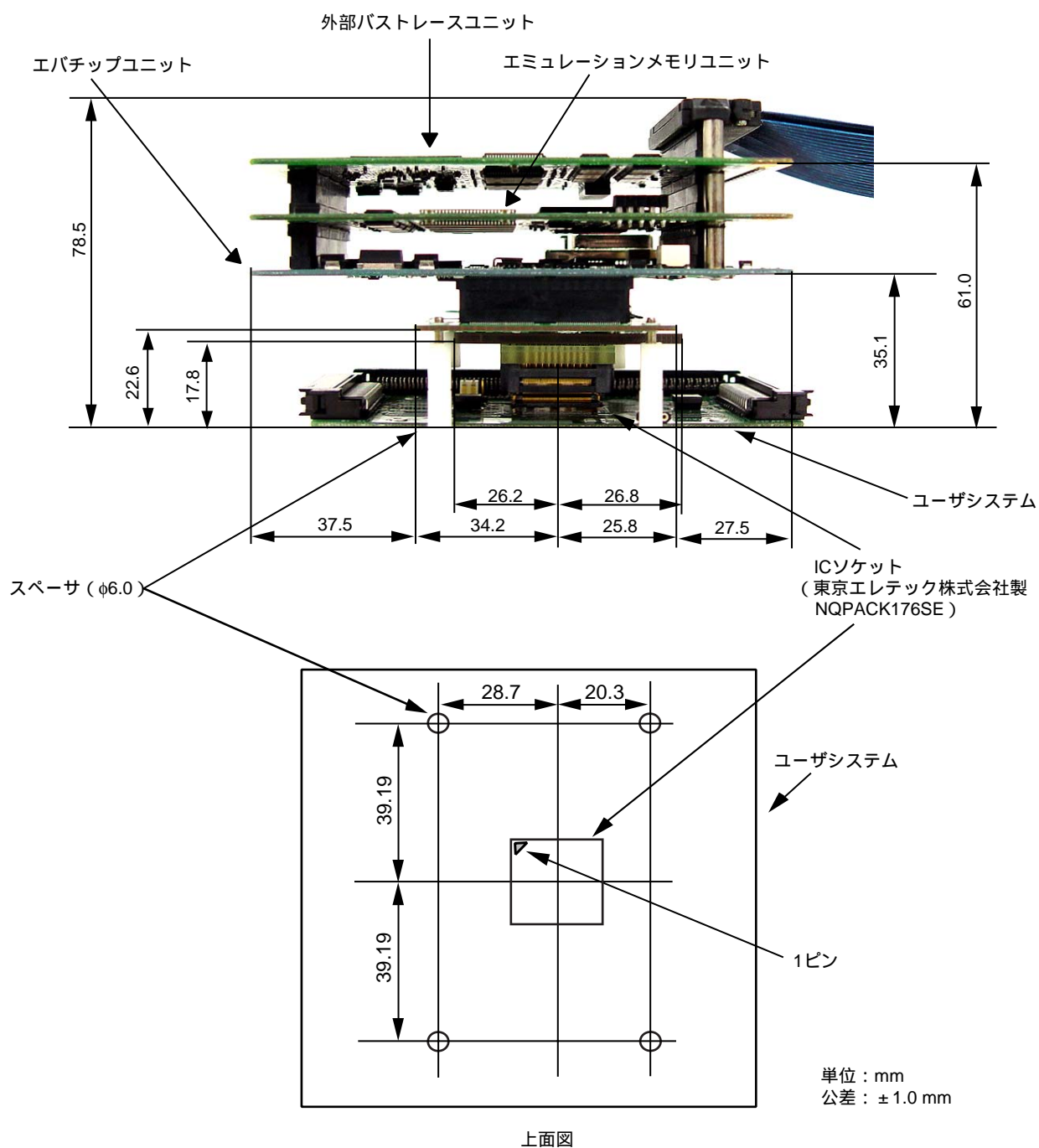
図 14 ユーザシステムインタフェース変換ボード接続時のユーザシステムとの寸法 (外部バストレースユニット、エミュレーションメモリユニット、エパチップユニット接続時)
