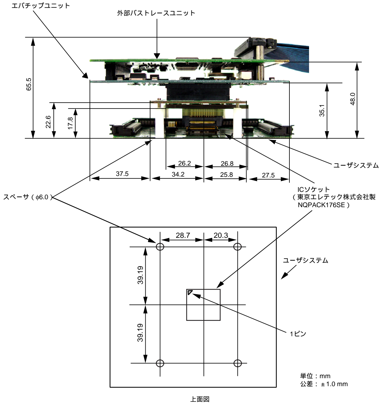
図 15 ユーザシステムインターフェース変換ボード接続時のユーザシステムとの寸法 (外部バストレースユニット、エバチップユニット接続時)
