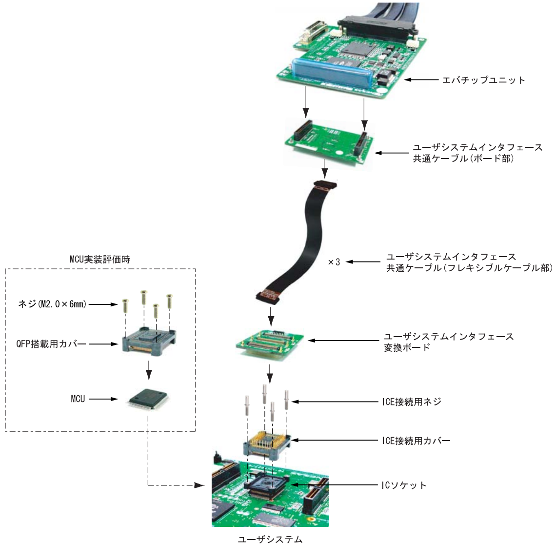
図 1 SH7216 グループ PLQP0176LB-A 用ユーザシステムインタフェース変換ボード外観イメージ
