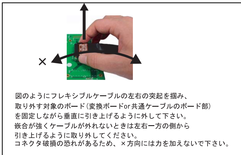
図4 フレキシブルケーブルの取り外しについて
