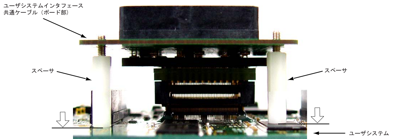
図9 スペーサ位置の調整
