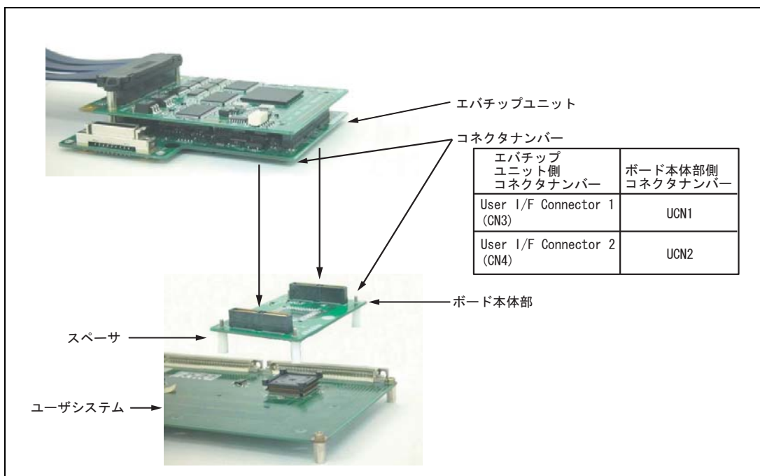
図 2.9 ユーザシステムインタフェースボード使用時のエバチップユニット接続方法
