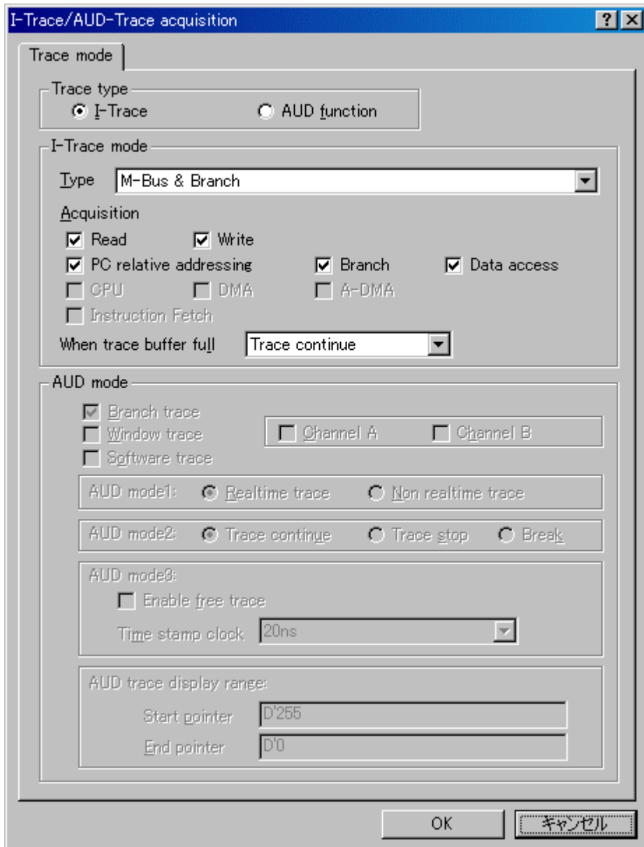
図 3.2 [I-Trace/AUD-Trace acquisition]ダイアログボックス (内蔵トレース機能)
