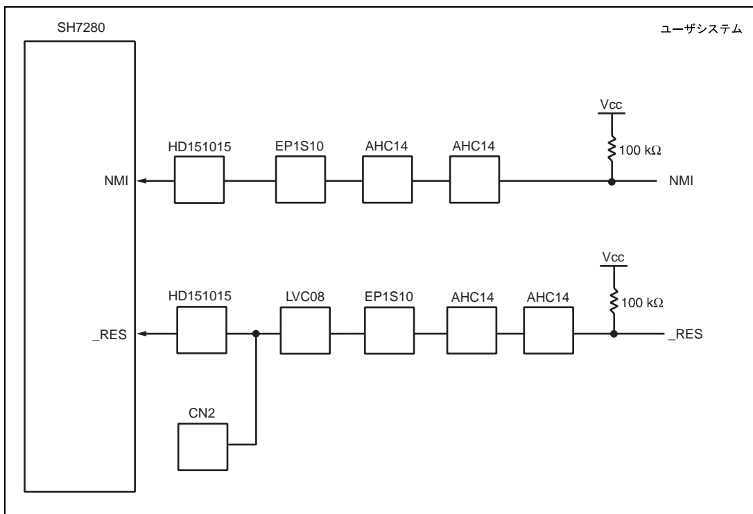
図 4.3 ユーザインタフェース回路(3)
