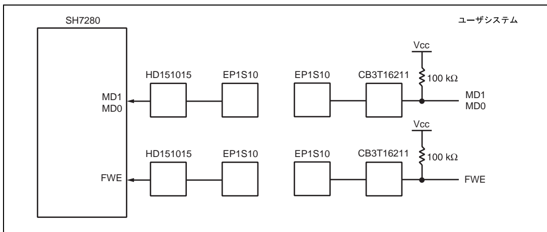
図 4.1 ユーザインタフェース回路(1)
