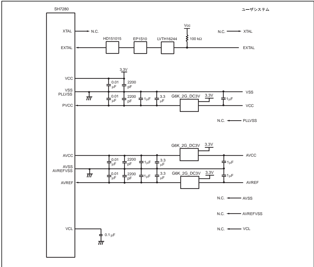
図 4.4 ユーザインタフェース回路(4)
