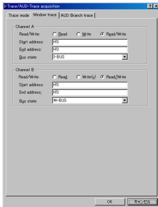
図 3.5 [Window trace]ページ
