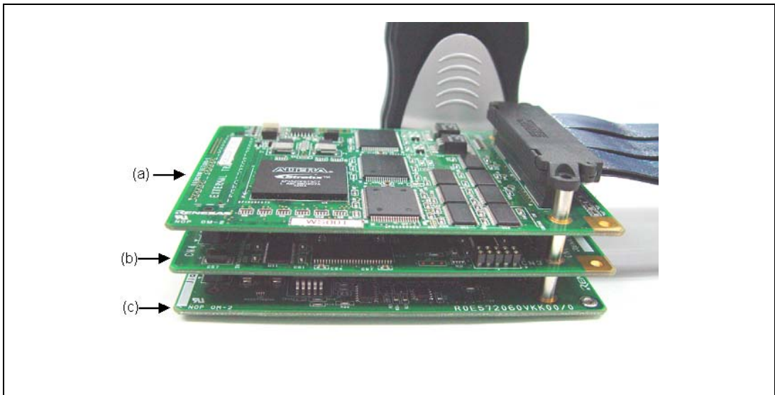
図 2.8 外部バストレーユニット、エミュレーションメモリユニット、およびエバチップユニットの接続方法
