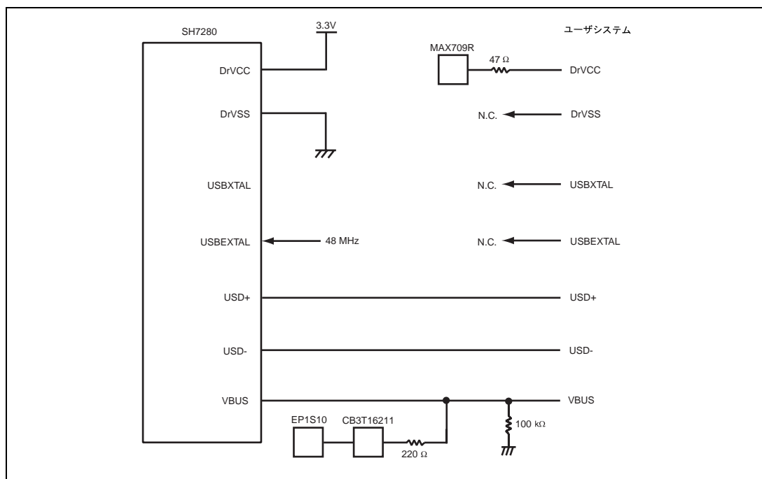
図 4.7 ユーザインタフェース回路(7)
