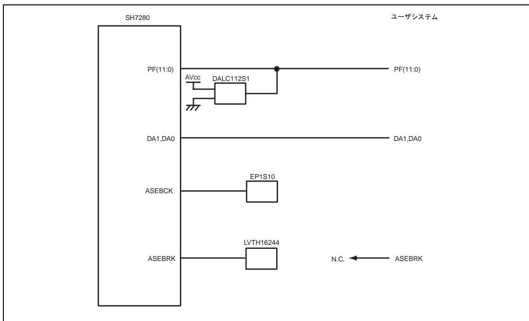
図 4.5 ユーザインタフェース回路(5)
