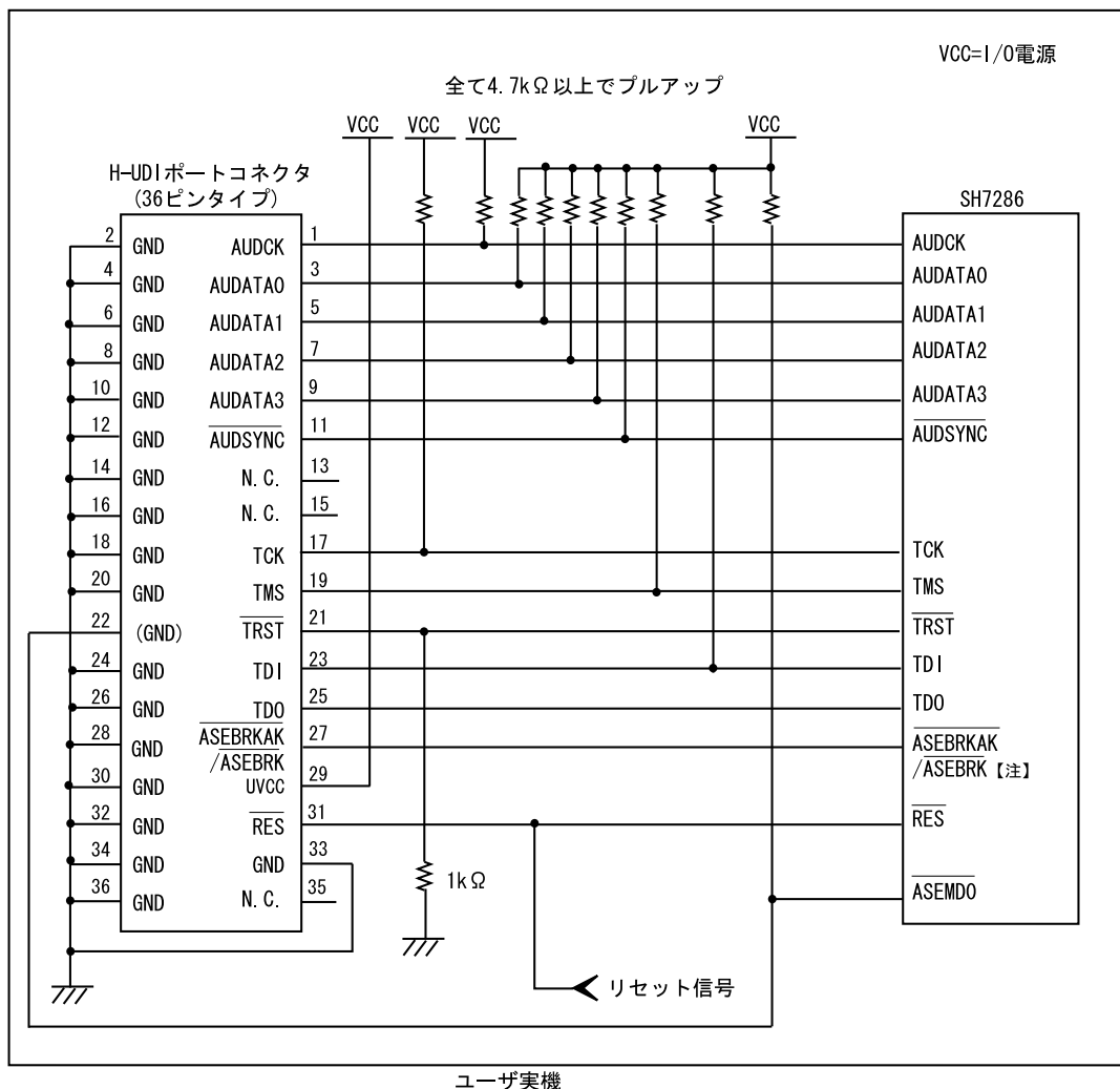
図 2.12 E200F 使用時の H-UDI ポートコネクタ - チップ間の推奨接続例(36 ピンタイプ) (1)
