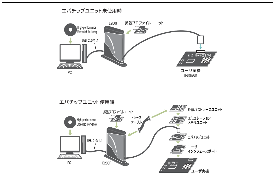
図 1.1 E200F エミュレータを使用したシステム構成外観
