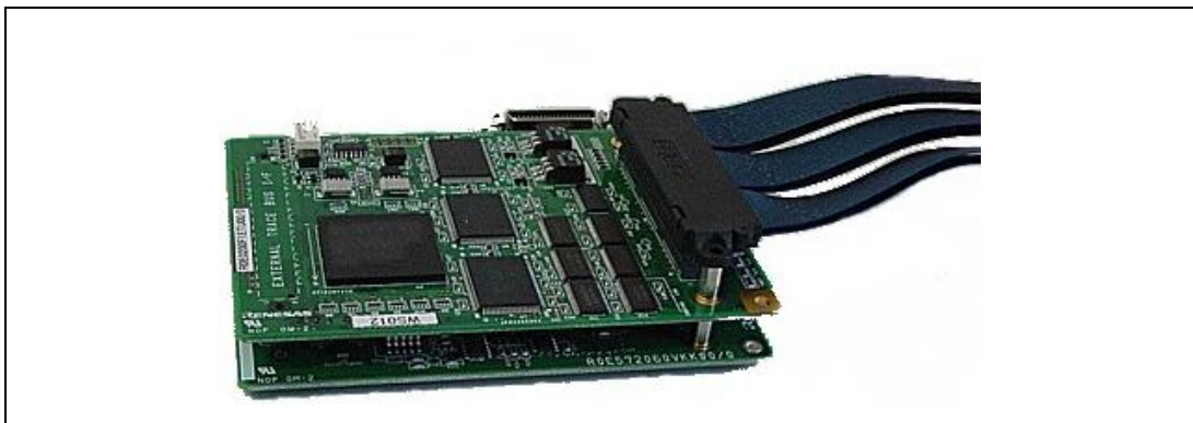
図 2.4 外部バストレースユニット、エバチップユニット、およびトレースケーブルの接続方法
