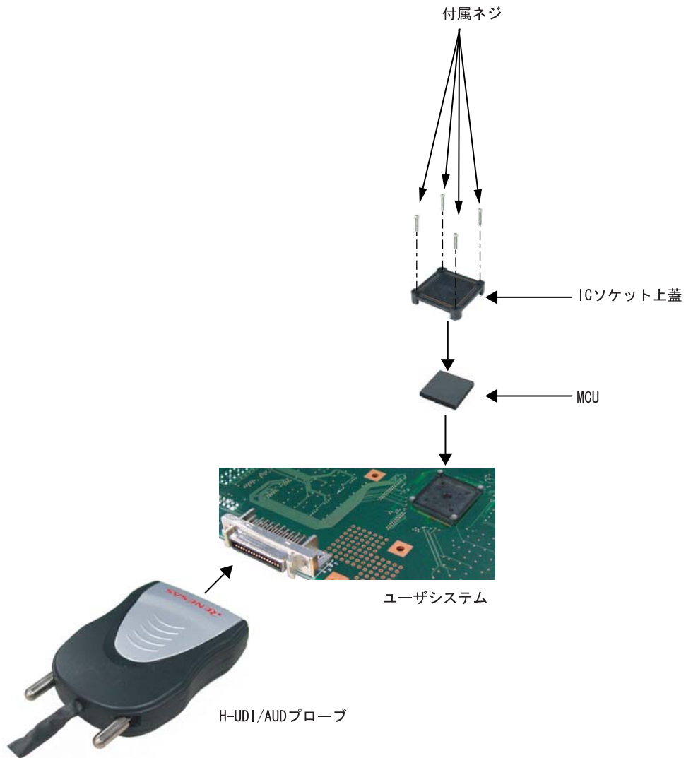
図 2.14 SH7286/SH7285/SH7243 でのオンチップ接続構成外観
