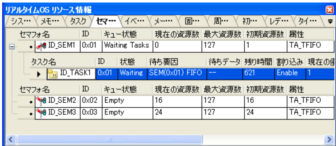
図 A—6 [セマフォ] タブ (待ちタスク情報)
