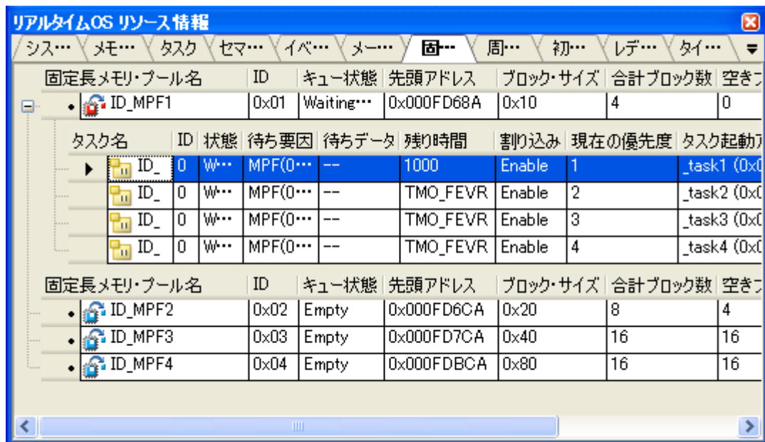
図 A—13 [固定長メモリ・プール] タブ (待ちタスク情報)
