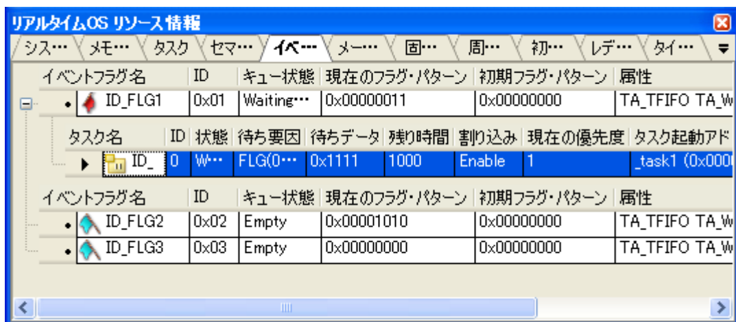
図 A—8 [イベントフラグ] タブ (待ちタスク情報)
