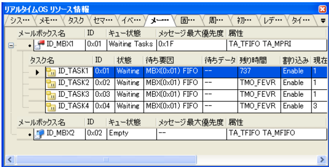
図 A—10 [メールボックス] タブ (待ちタスク情報)
