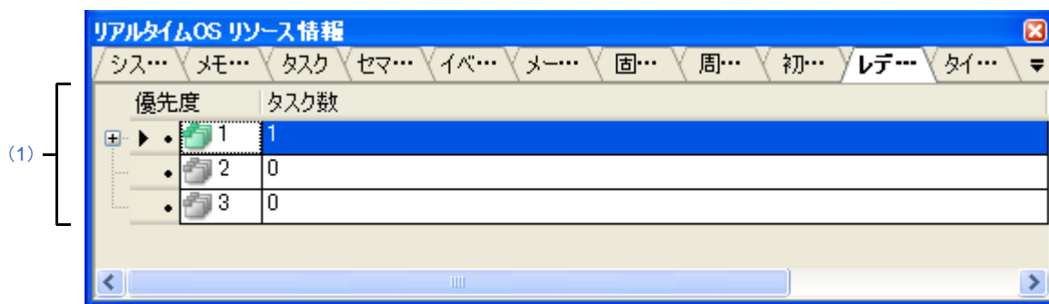
図 A—16 [レディ・キュー] タブ
