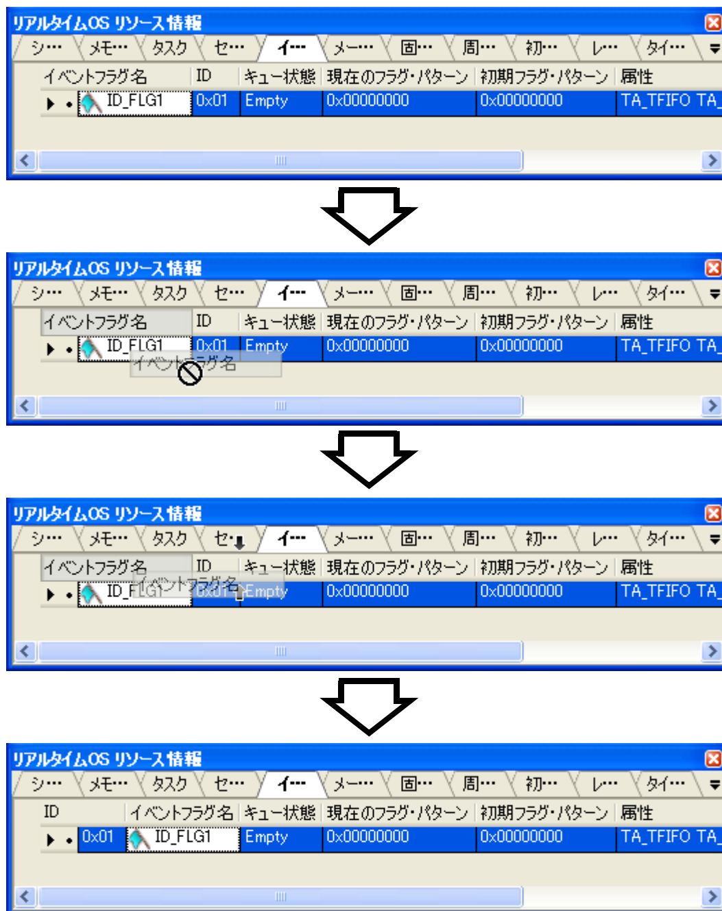
図 2—2 表示順序の変更 (ID 列の移動)
