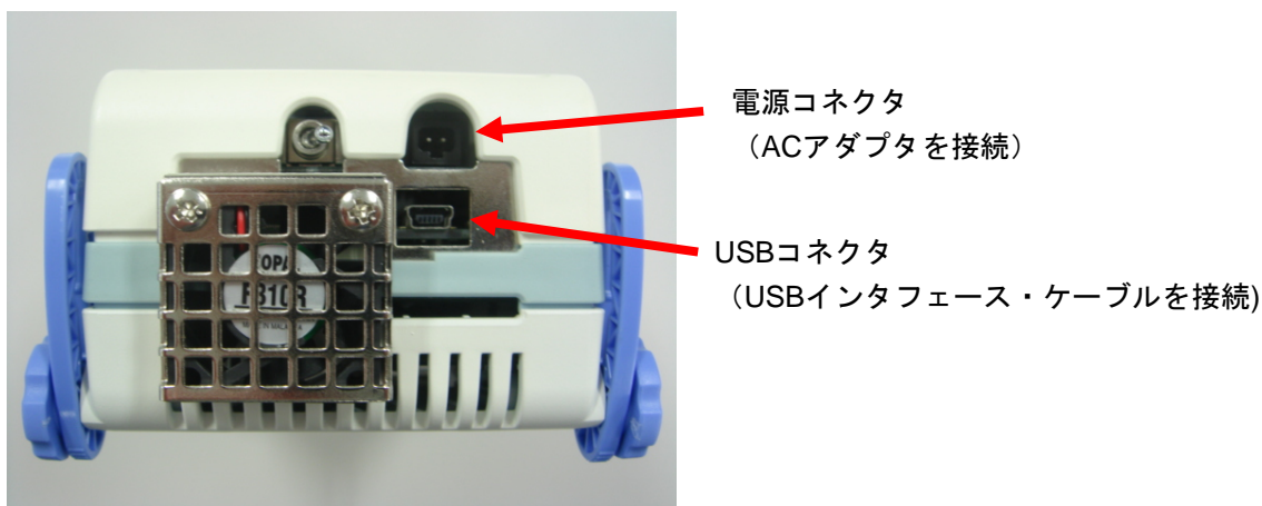
図2-8 コネクタ位置
