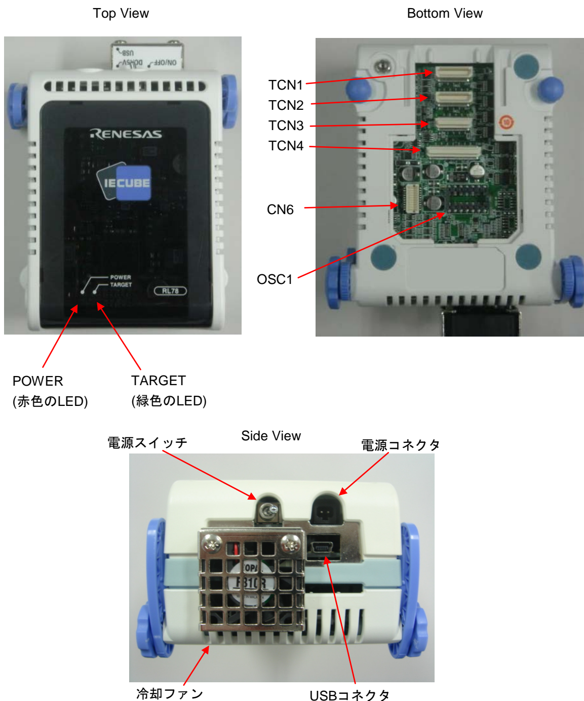
図1-1 QB-RL78L1Cの各部の名称
