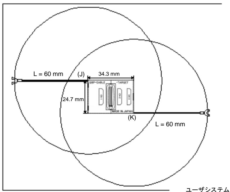
図2-7 GND線接続可能箇所
