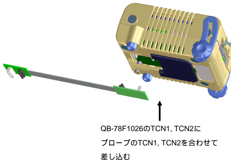
図2 - 5 QB-78F1026とプローブの接続
