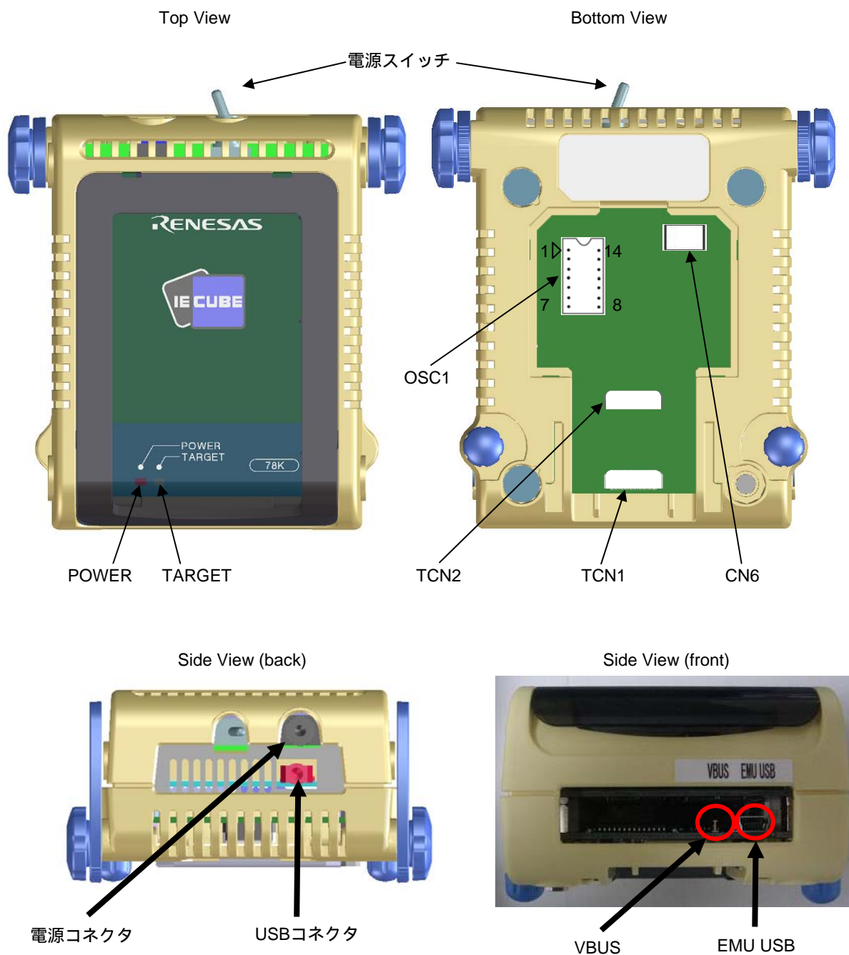
図2 - 1 QB-78F1026の各部の名称
