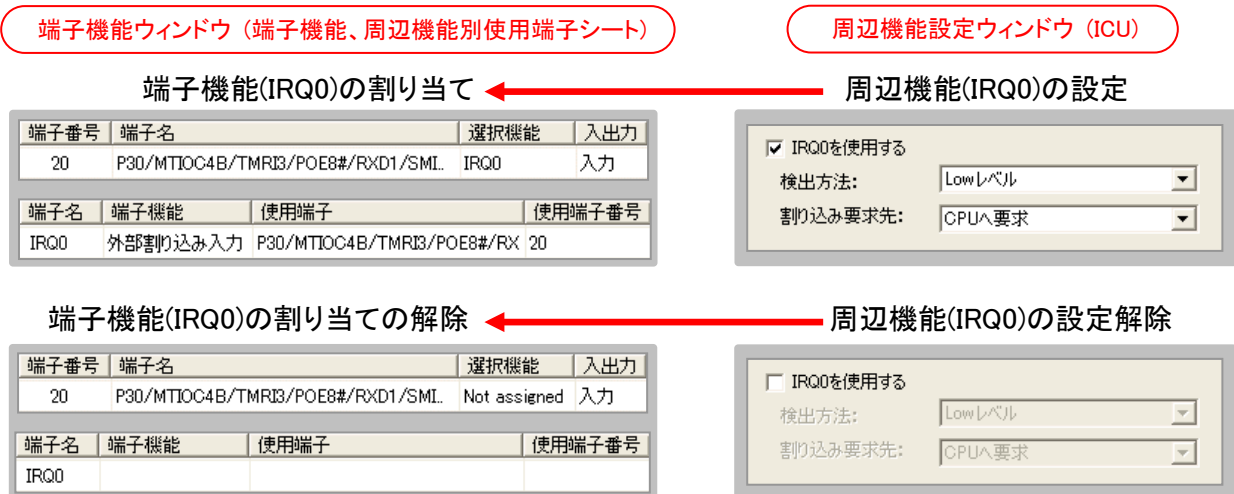
図 3.19 周辺機能の設定と端子機能の割り当て
