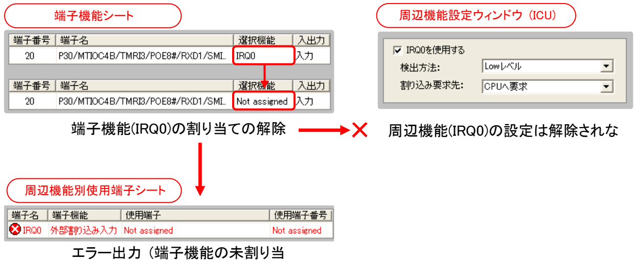
図 3.20 端子機能の割り当て解除とエラー表示
