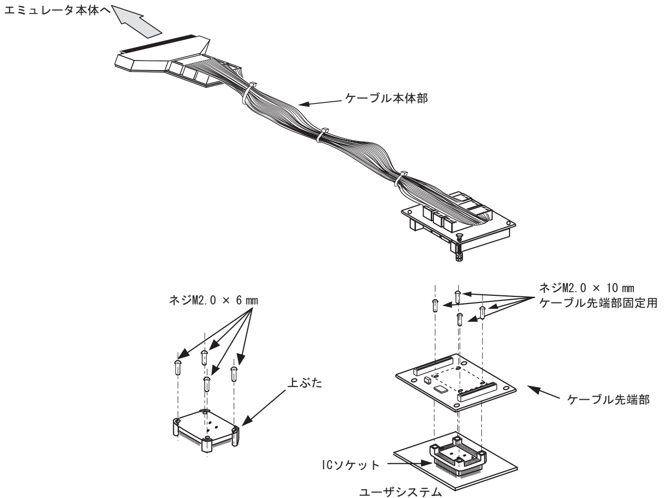
図1 HS1582ECH61H ユーザシステムインタフェースケーブル
