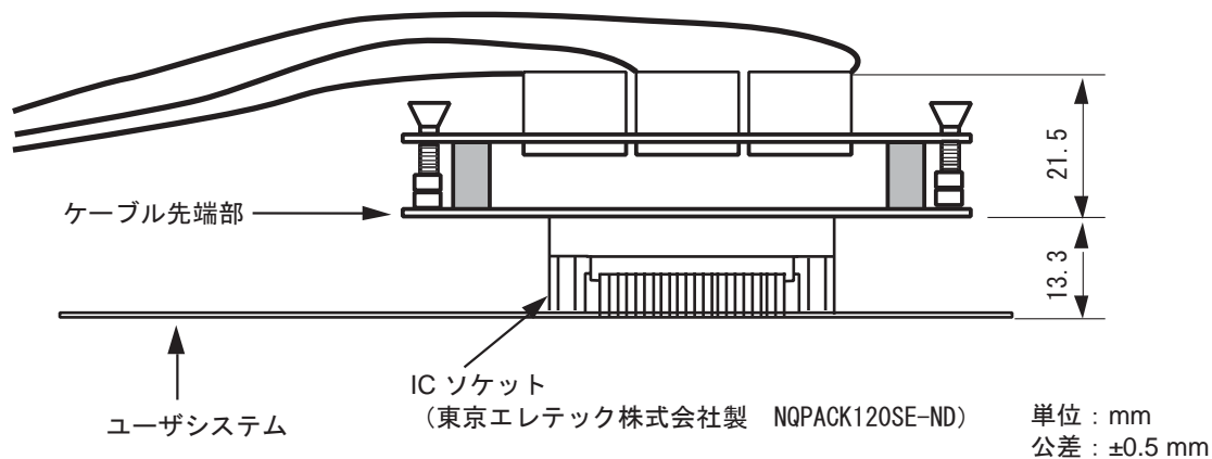
図8 ケーブル接続時のユーザシステムとの寸法
