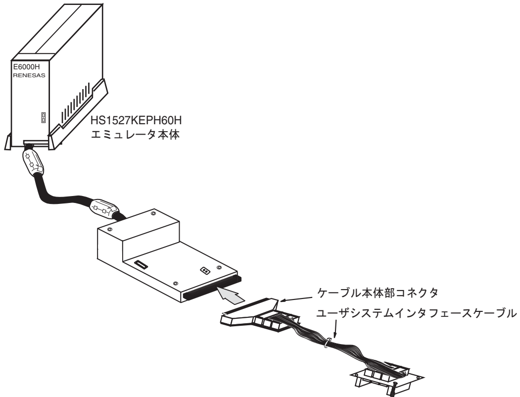
図2 HS1527KEPH60H エミュレータ本体への接続
