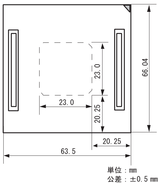
図7 ケーブル先端部の寸法
