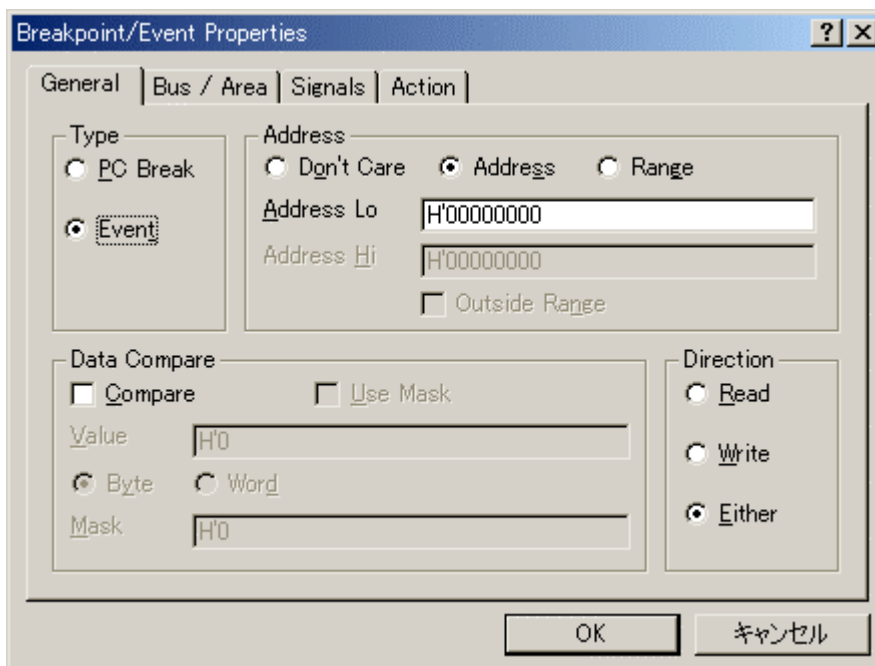
図 5-64 Breakpoint/Event Properties ダイアログボックス (General ページ)
