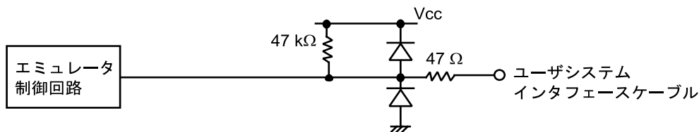
図 7-3 RESET 信号回路
