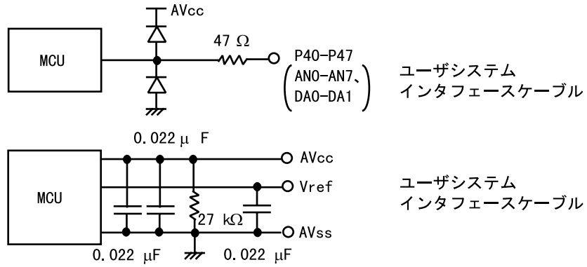
図 7-4 P40-P47、AVcc、AVss、Vref 信号回路
