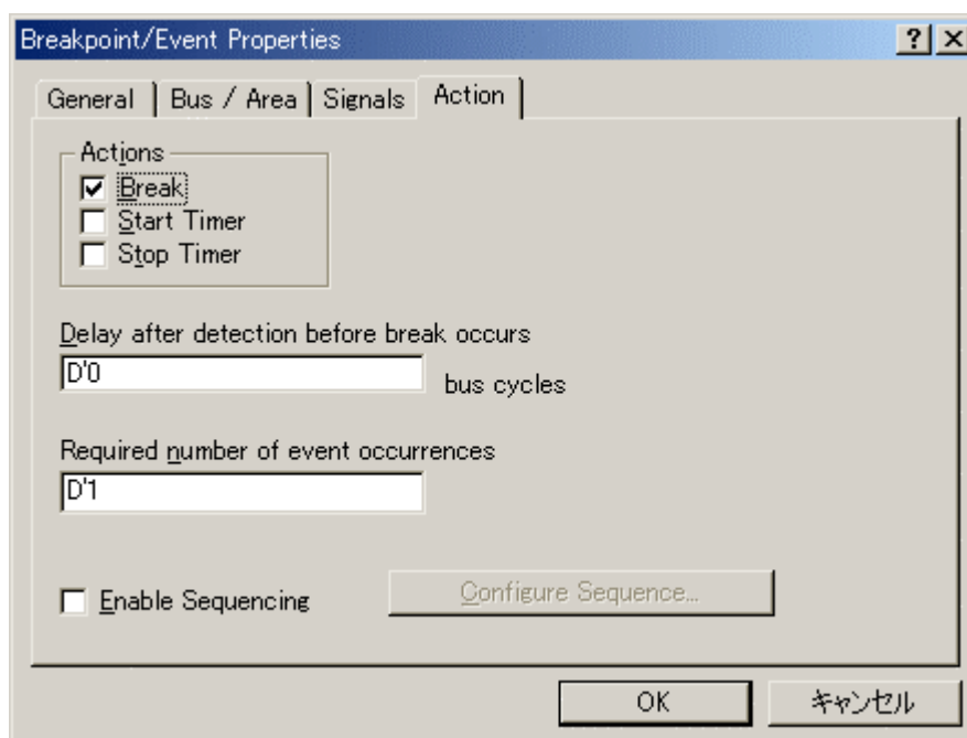
図 5-67 Breakpoint/Event Properties ダイアログボックス (Action ページ)
