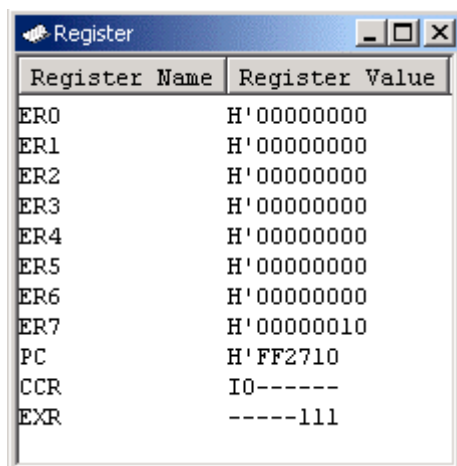
図 6-5 [Register]ウィンドウ
