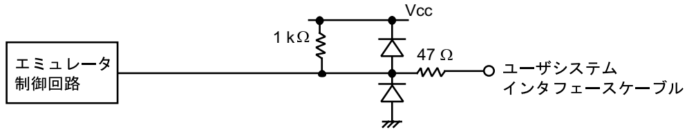
図 7-4 RESET 信号回路
