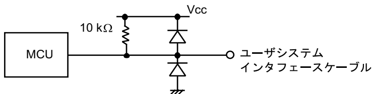
図 7-2 ユーザインタフェース信号回路(2)
