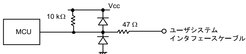
図 7-1 ユーザインタフェース信号回路(1)
