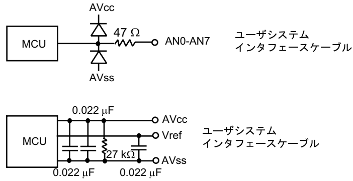
図 7-5 AN0-AN7、AVcc、AVss、Vref 信号回路
