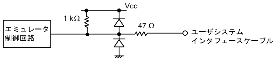
図 7-3 モード端子, NMI 信号回路
