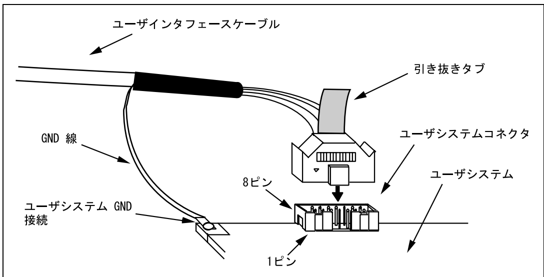
図 1.1 14ピンストレータイプコネクタ使用時のユーザシステム側のユーザインタフェースケーブル接続方法
