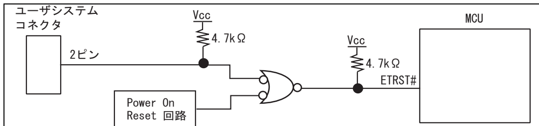
図 1.8 ETRST#端子の考慮 (参考)
