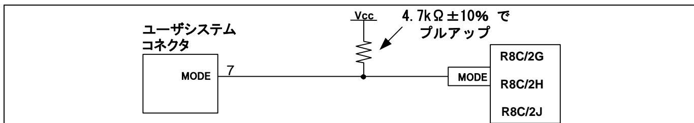
図5.2 E8a エミュレータと MODE 端子の接続
