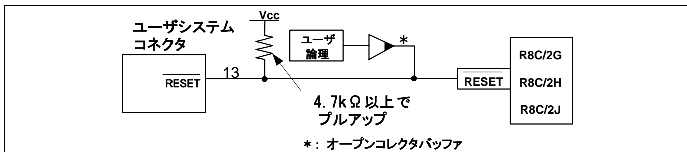
図5.3 リセット回路例
