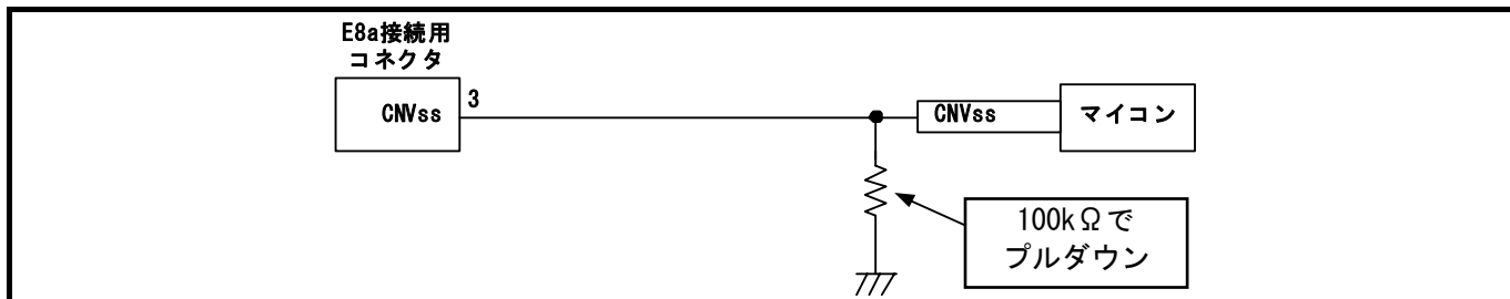
図 4.7 E8aエミュレータとCNVss端子の接続
