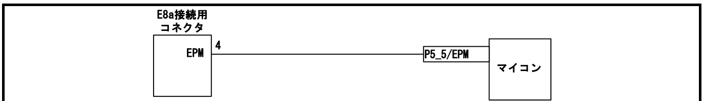
図 4.6 E8aエミュレータとP5_5端子の接続
