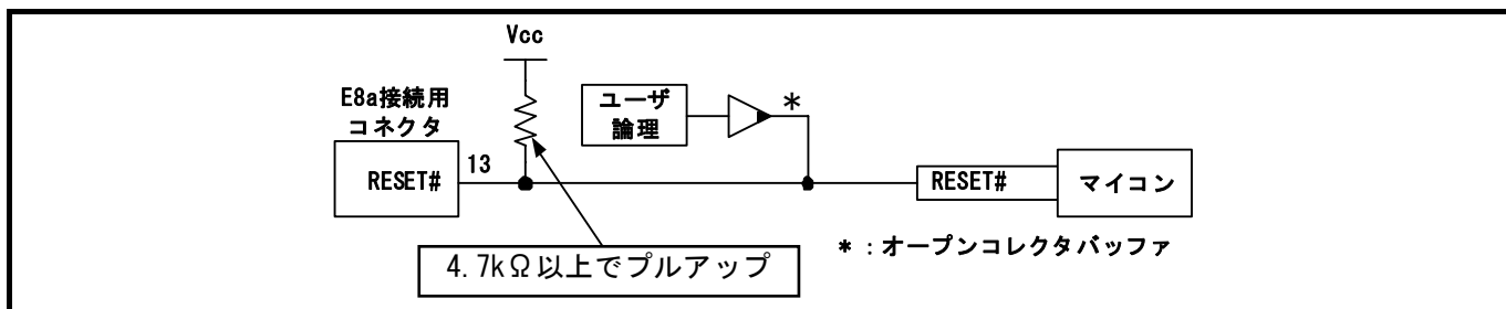
図 4.8 リセット回路例
