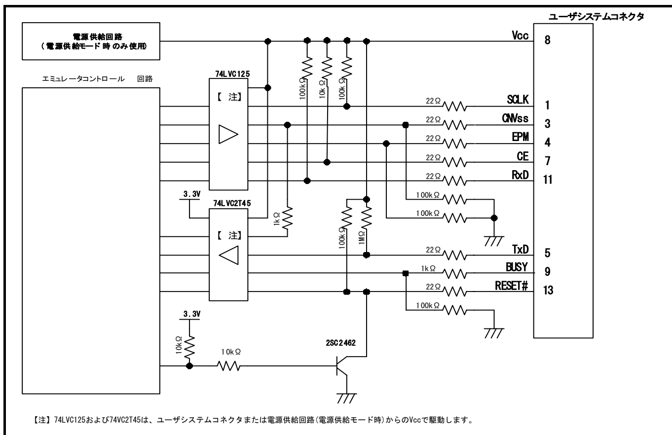
図 4.9 E8aエミュレータ内インタフェース回路 (参考)
