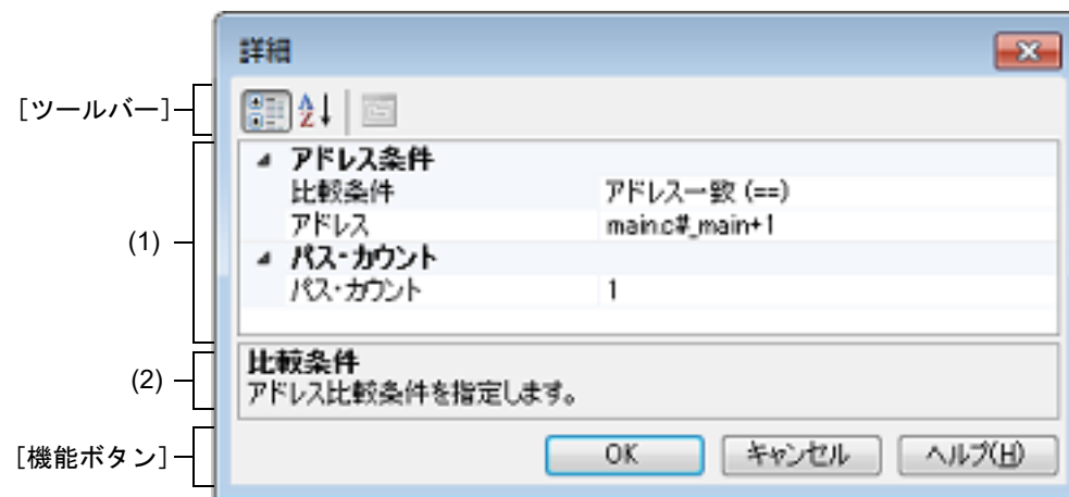
図 A.36 詳細 ダイアログ (実行イベント)【E1】【E20】【EZ Emulator】【COM Port】
