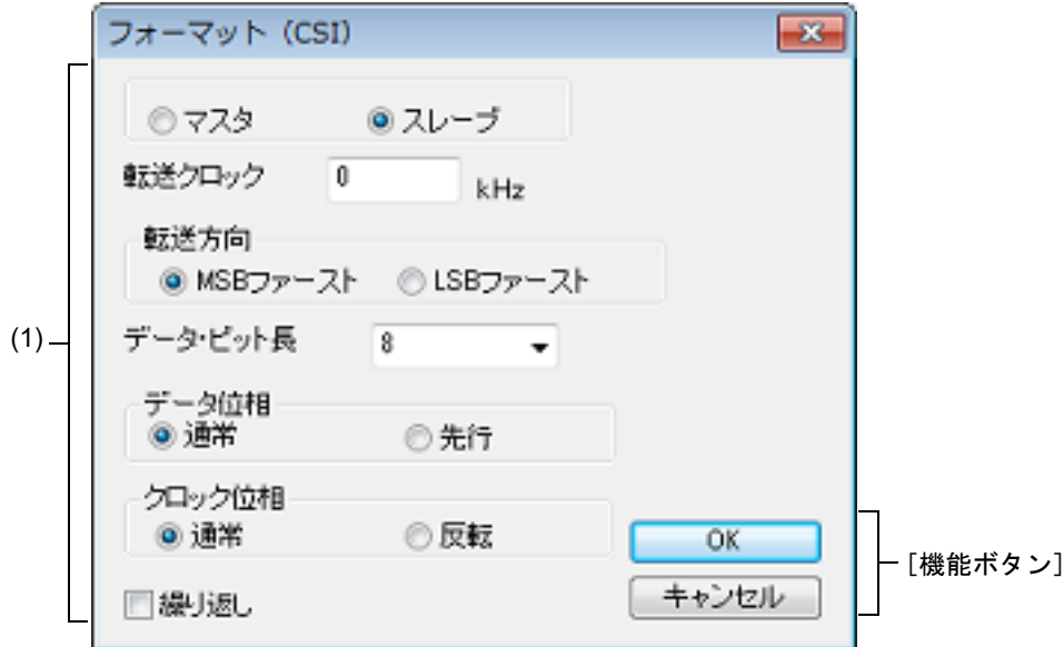
図 A.96 フォーマット (CSI) ダイアログ
