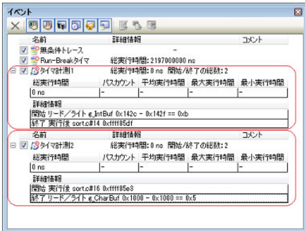
図 2.162 タイマ計測イベント（タイマ開始イベント／タイマ終了イベント）の測定結果例【E1】【E20】
