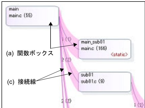
図 A.18 コール・グラフの構成要素 【全体表示】
