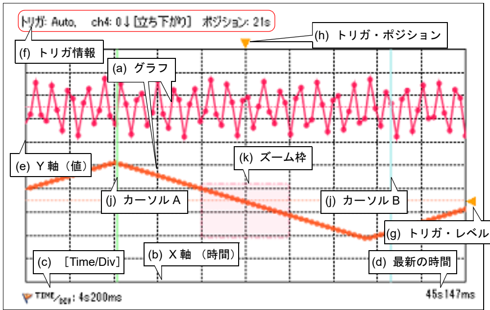
図 A.11 グラフ表示エリア
