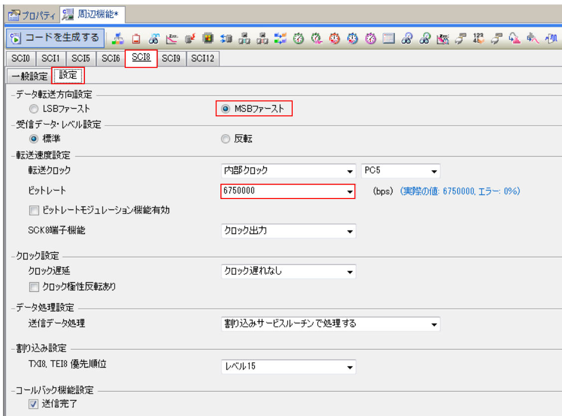
図 4-10: SCI8 設定
