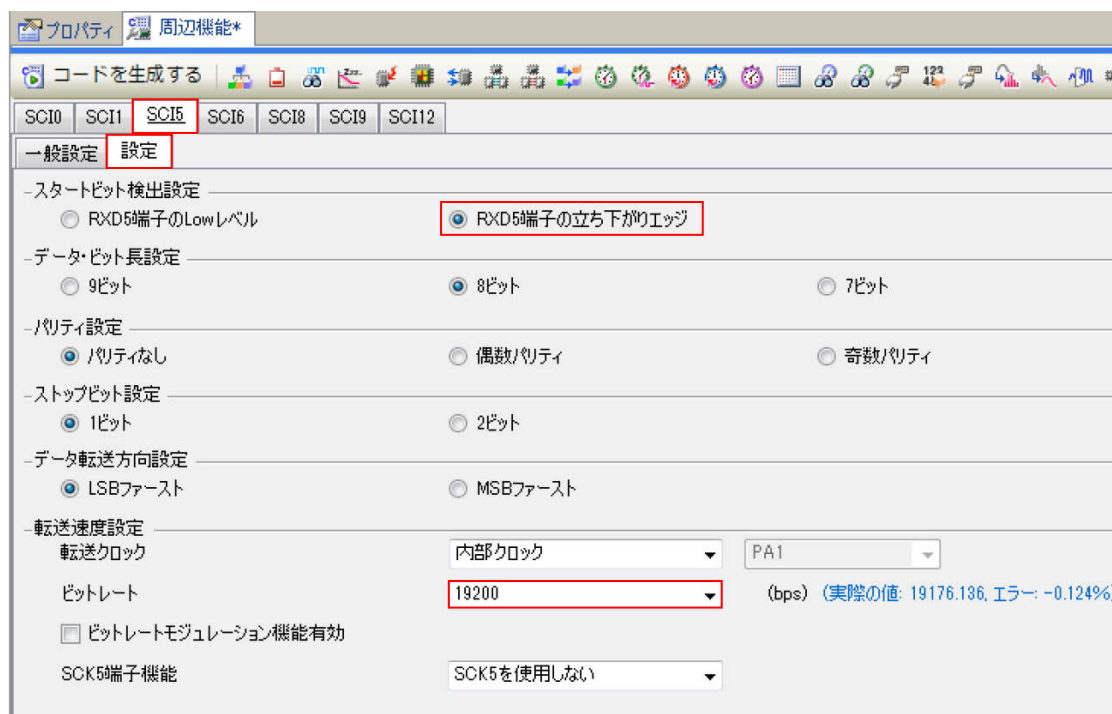
図 4-12: SCI5 設定
