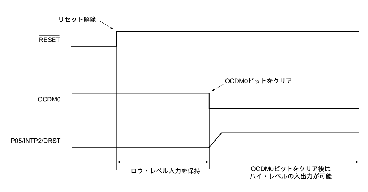
図30 - 1 オンチップ・ディバグ機能未使用時のタイミング
