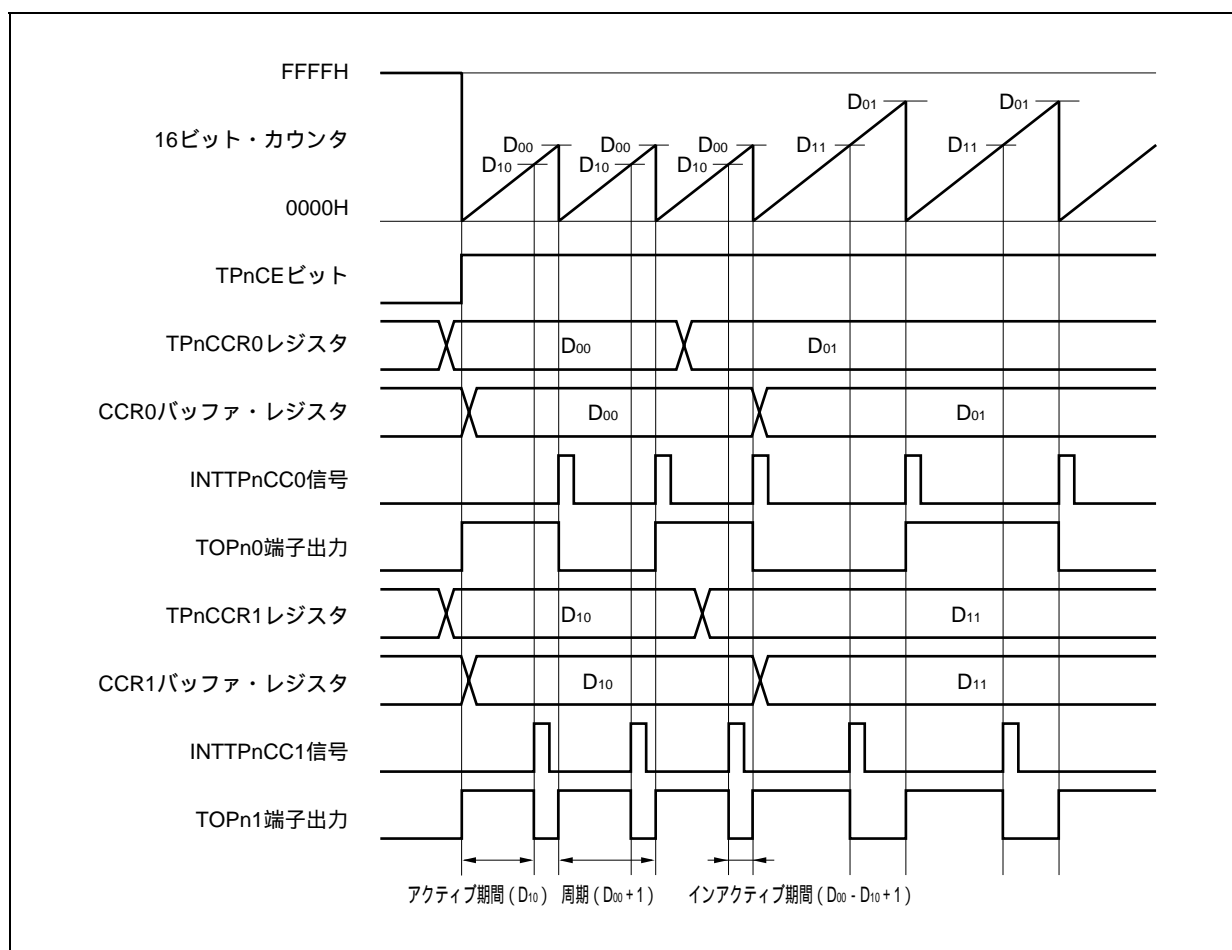
図7-25 PWM出力モードの基本タイミング
