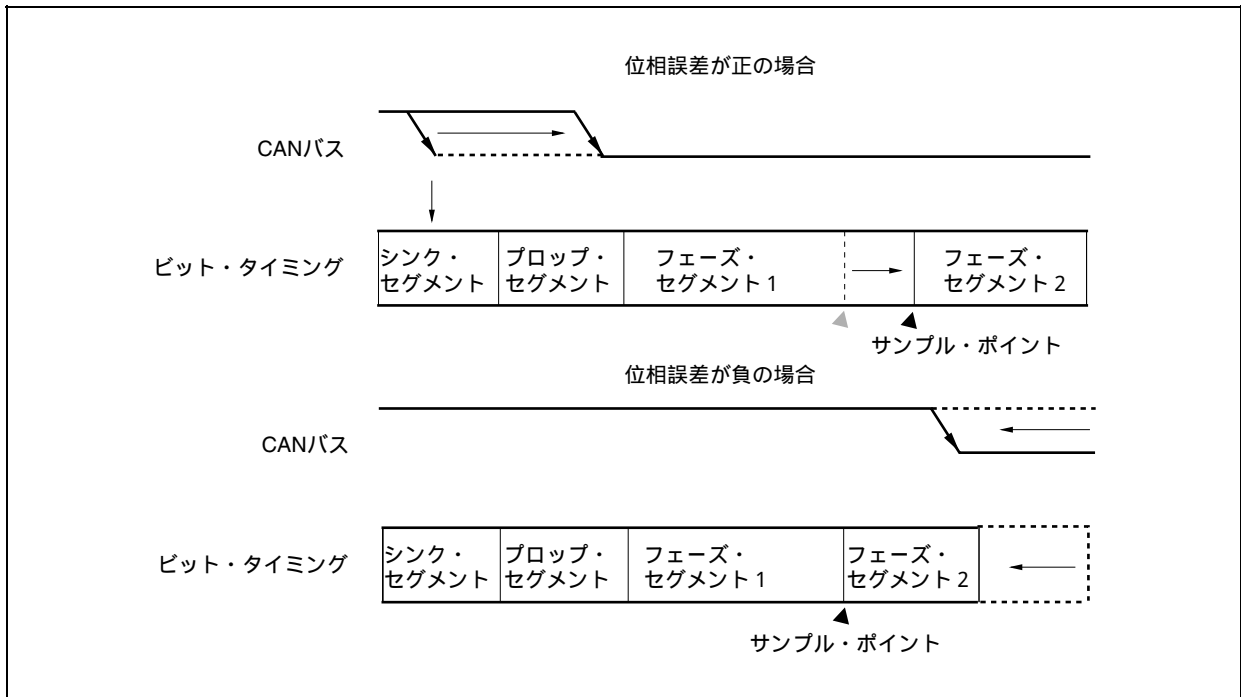
図19 - 21 再同期
