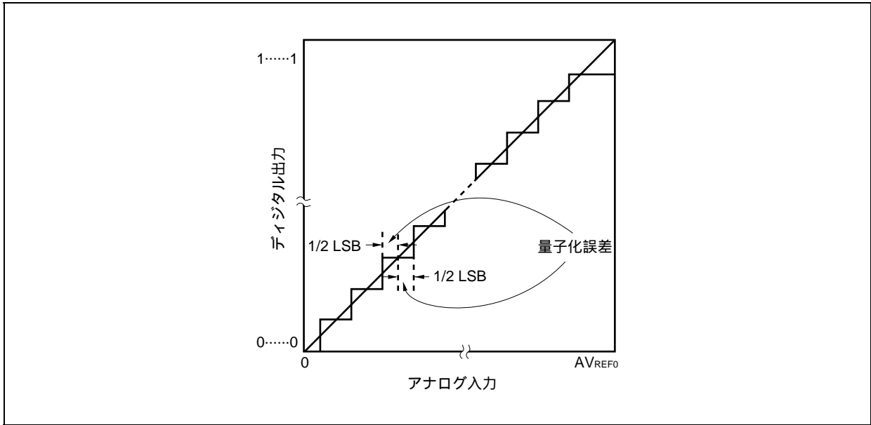
図13 - 17 量子化誤差
