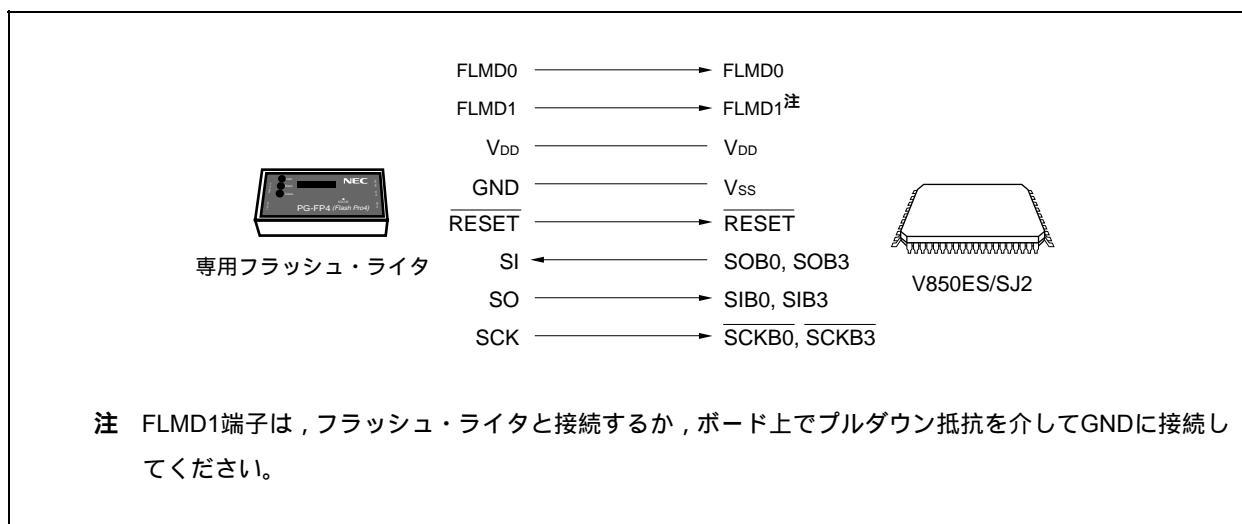
図29-4 専用フラッシュ・ライタとの通信 (CSIB0, CSIB3)
