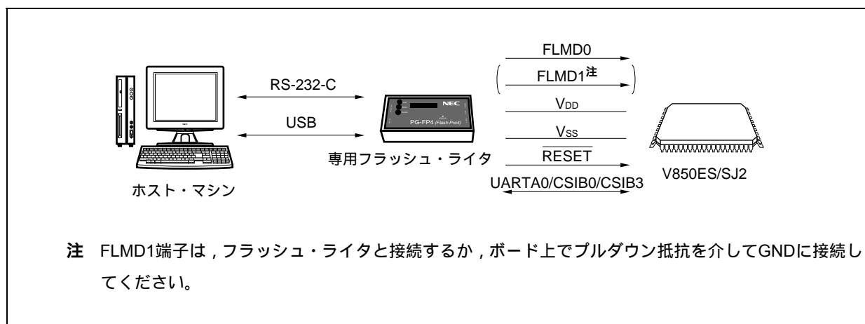
図29-2 フラッシュ・メモリにプログラムを書き込むための環境
