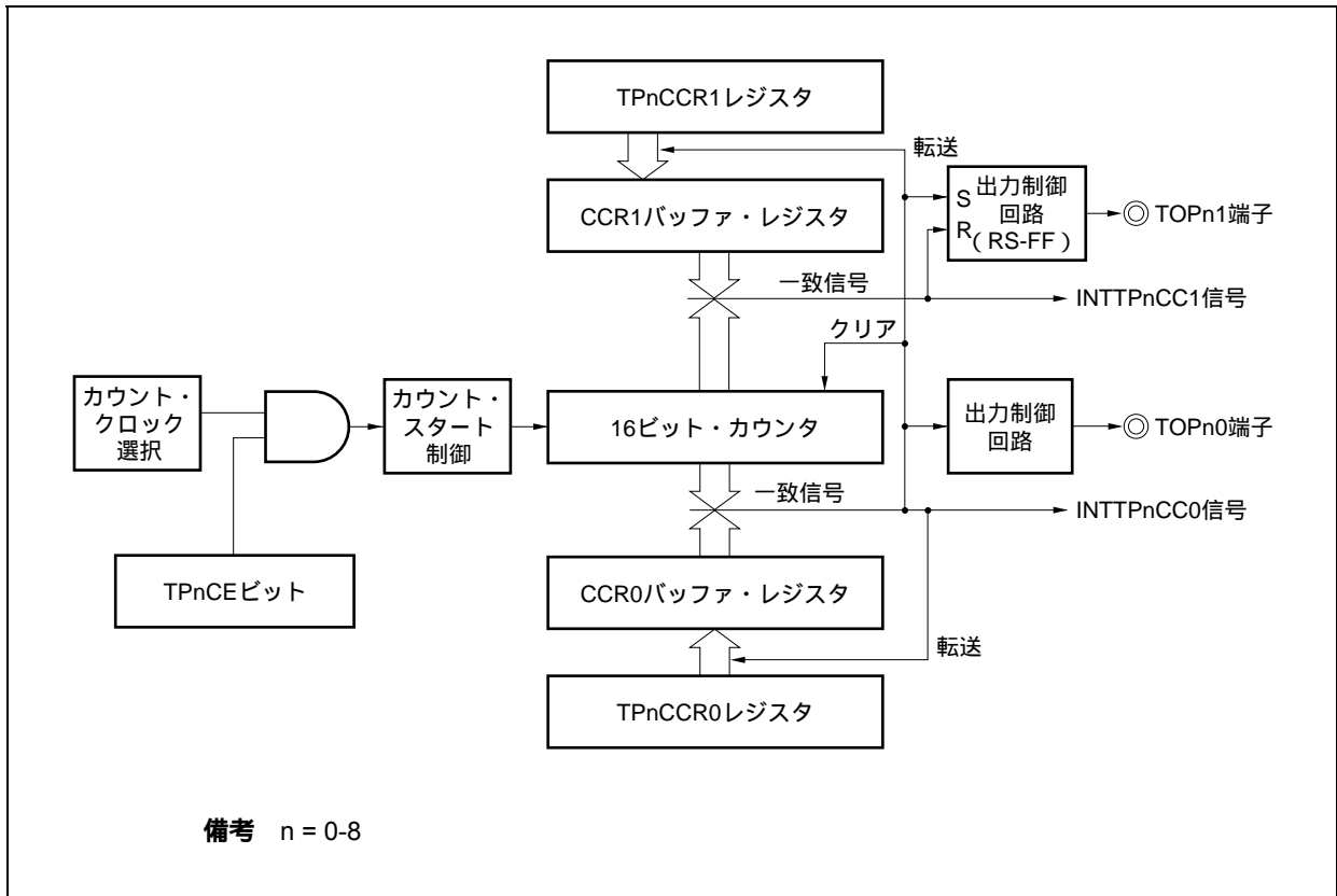
図7-24 PWM出力モードの構成図
