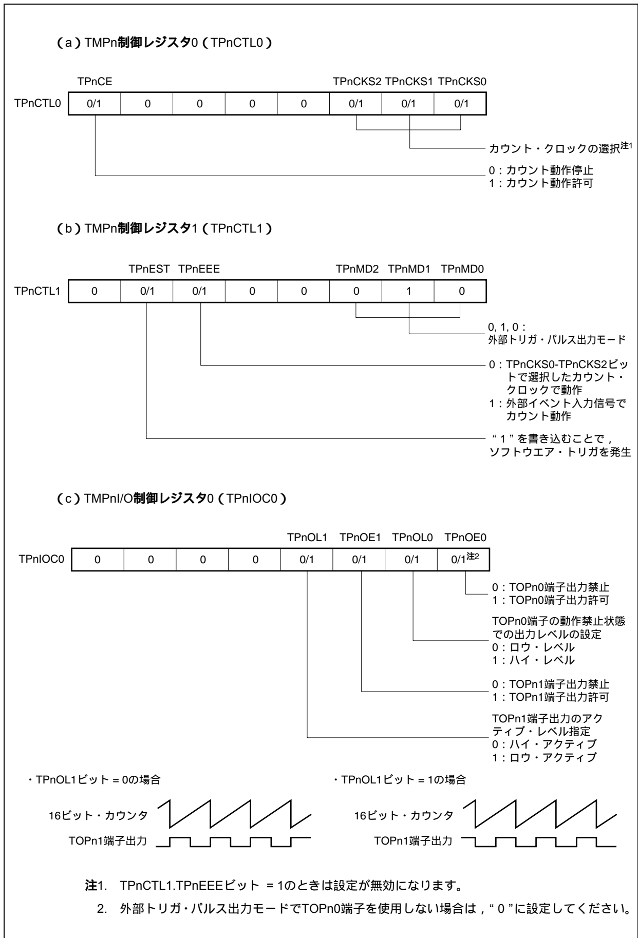
図7 - 18 外部トリガ・パルス出力モード動作時のレジスタ設定内容 (1/2)
