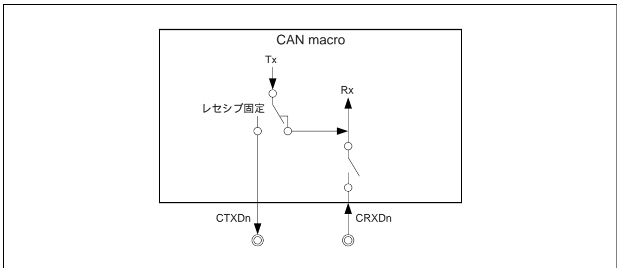
図19 - 33 セルフ・テスト・モードにおけるCAN端子接続
