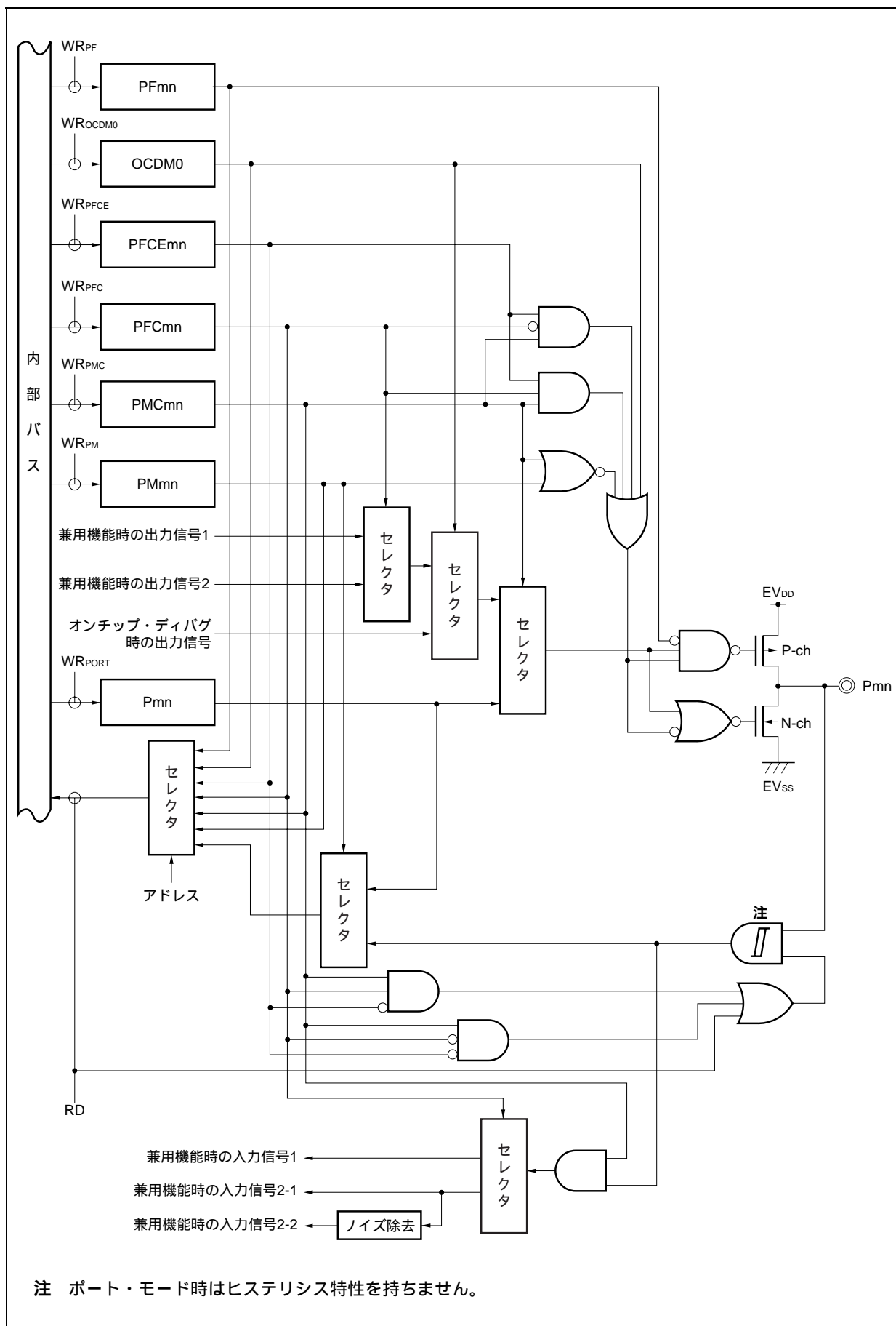
図4 - 31 タイプU - 7のブロック図
