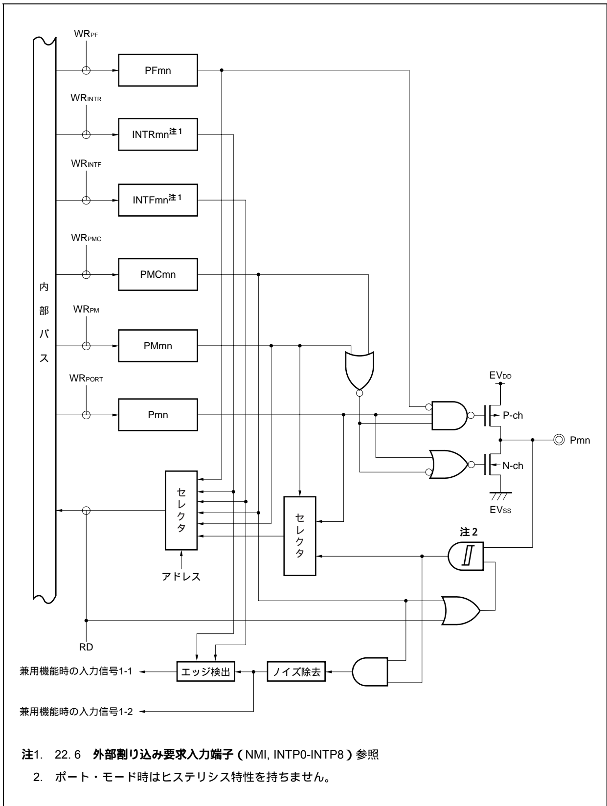
図4-21 タイプL-2のブロック図
