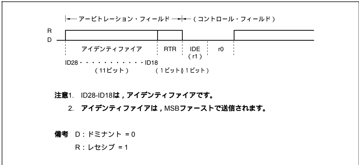
図19-6 アービトレーション・フィールド(標準フォーマット・モード時)
