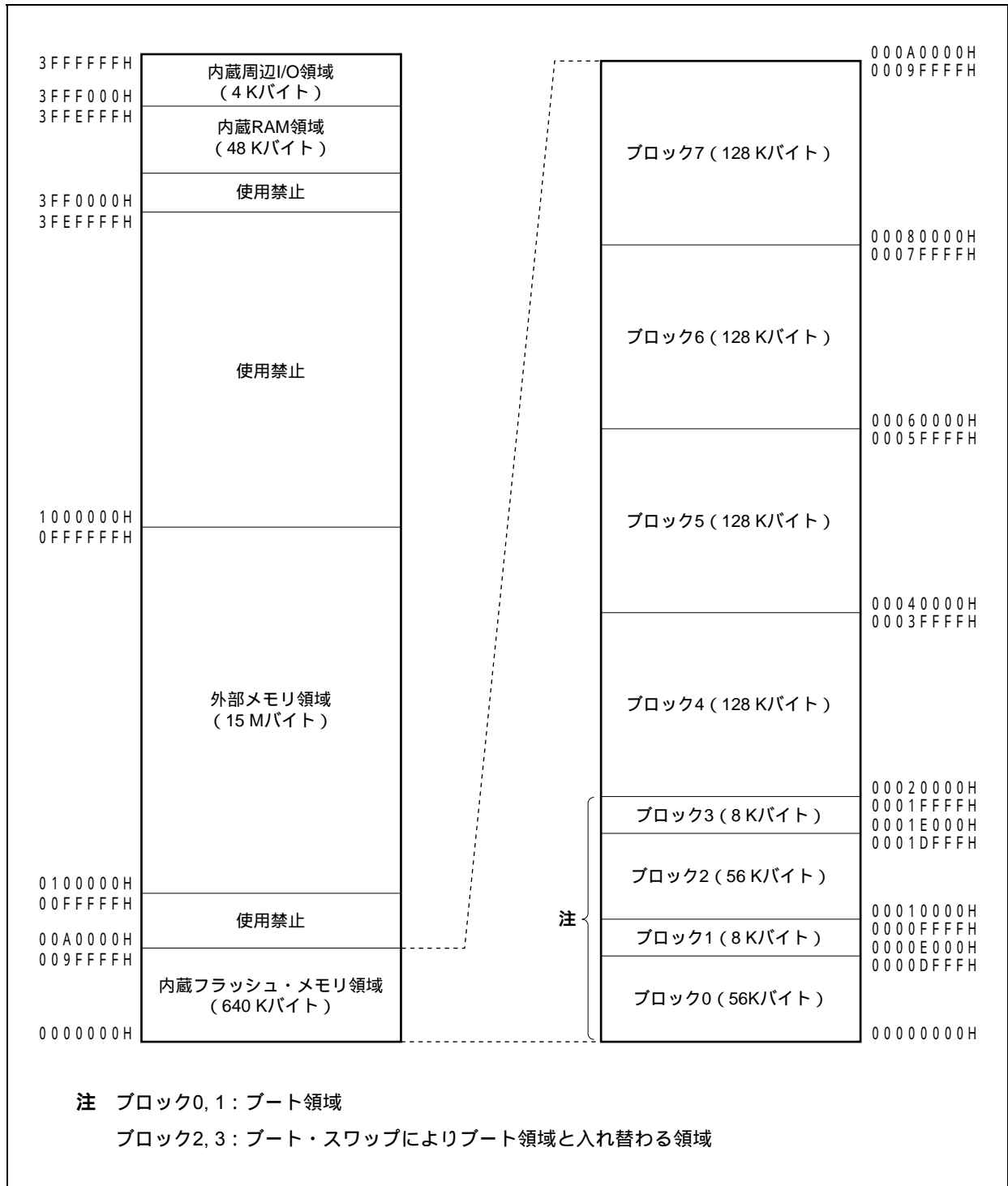
図29-1 フラッシュ・メモリ・マッピング
