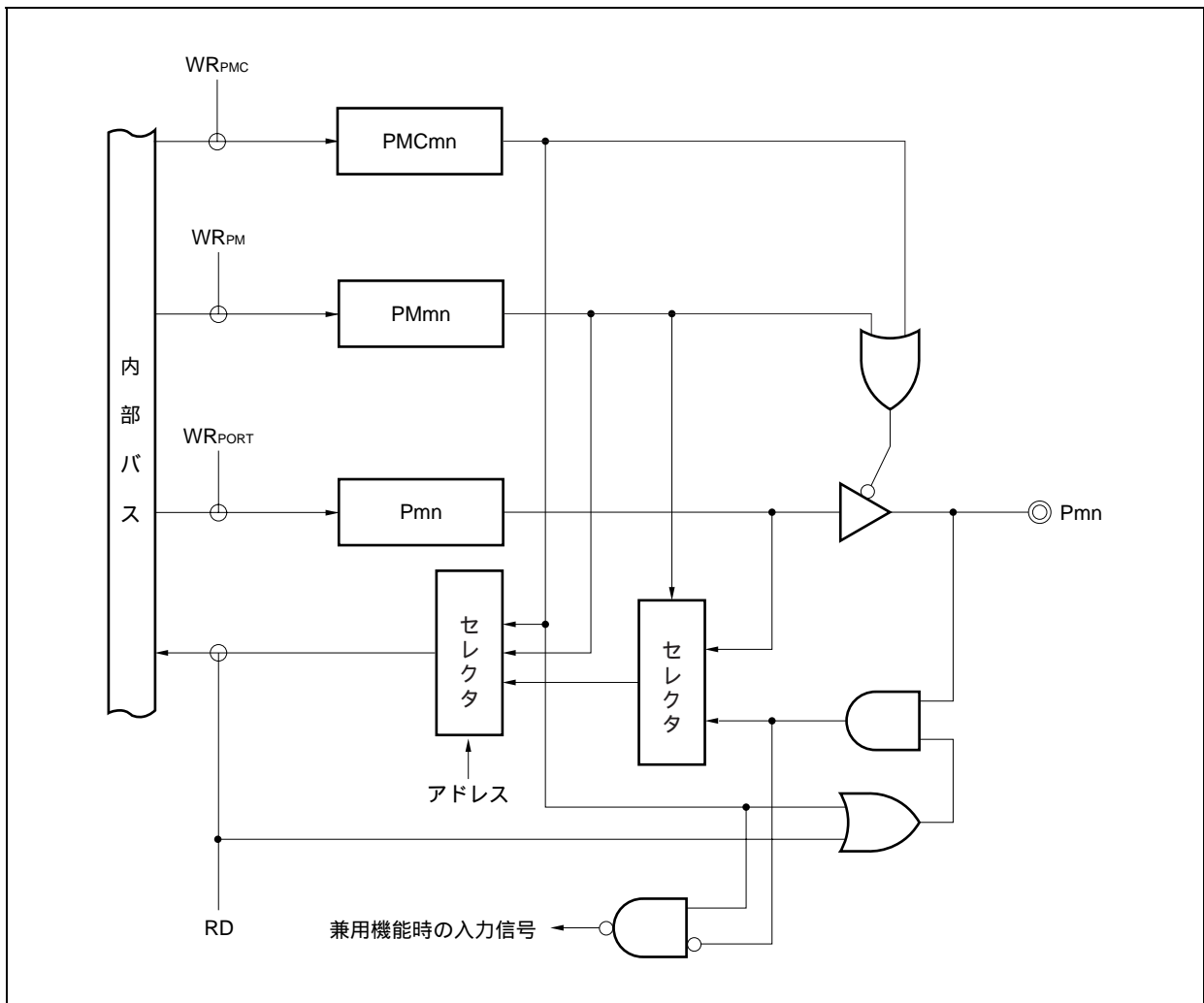
図4-7 タイプD-1のブロック図
