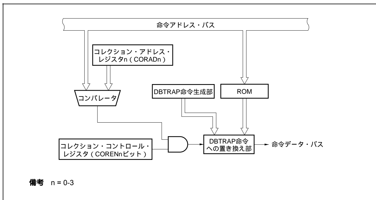
図28 - 1 ROMコレクションのブロック図
