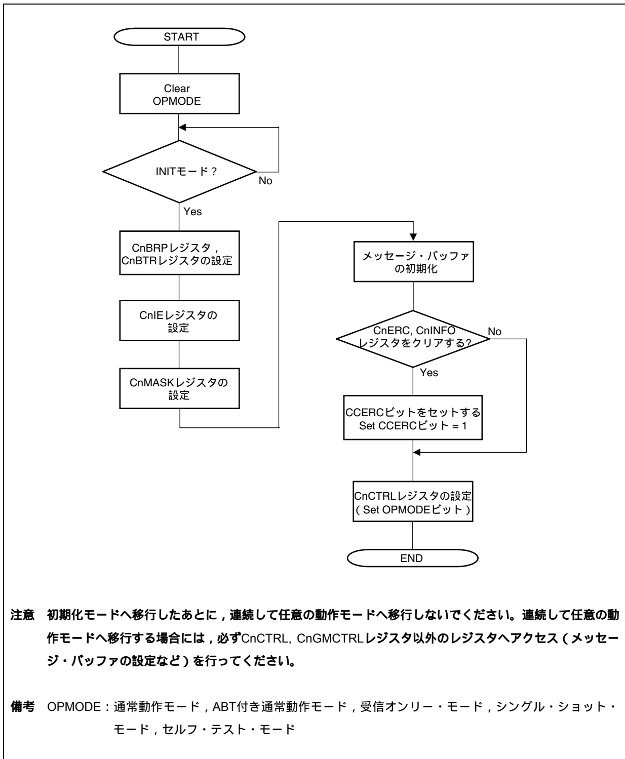
図19 - 36 再初期化
