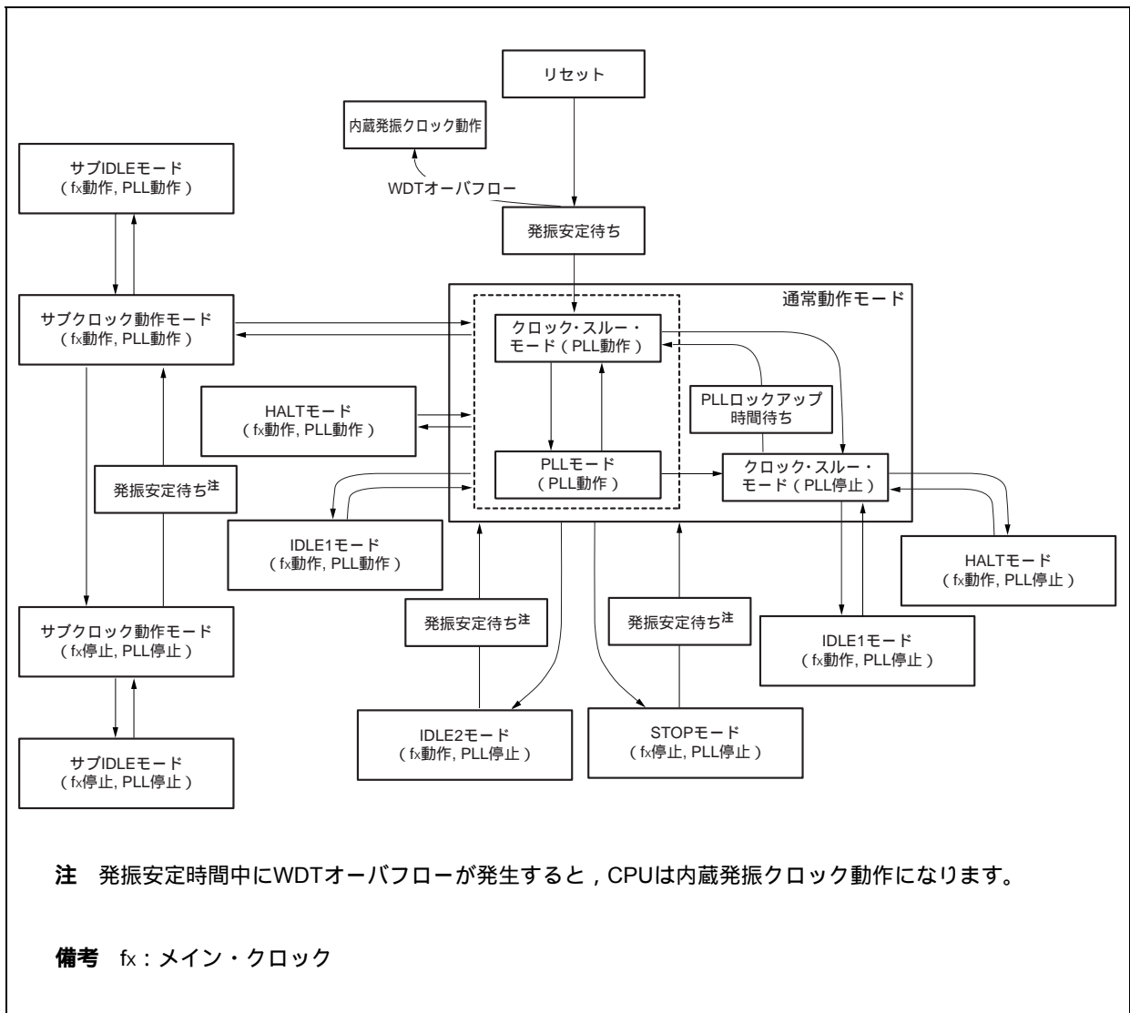
図24 - 1 状態遷移図
