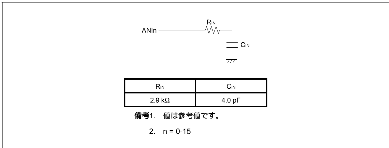
図13 - 14 ANIn端子内部等価回路
