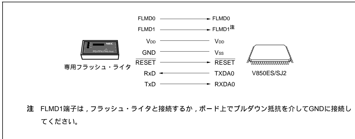
図29-3 専用フラッシュ・ライタとの通信 (UARTA0)
