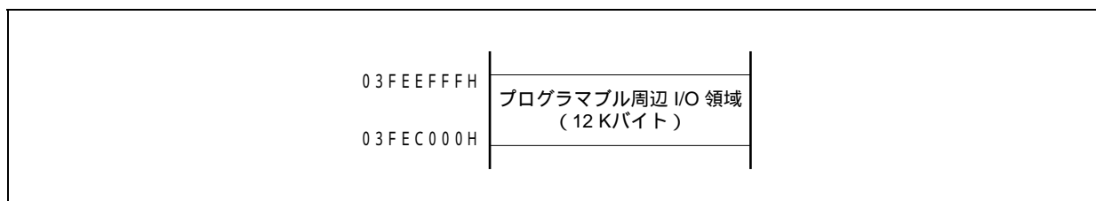
図3 - 9 プログラマブル周辺I/O領域
