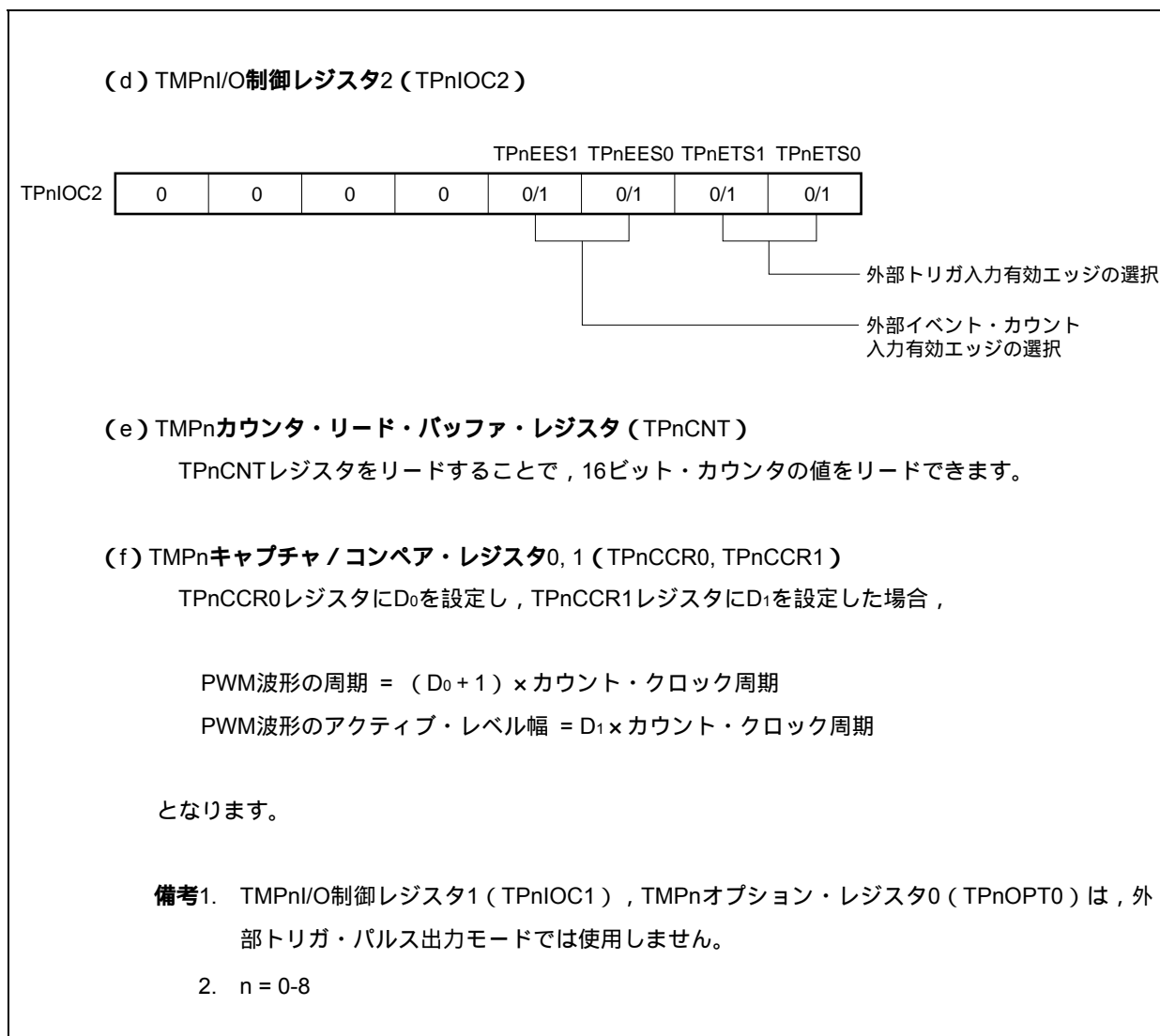
図7 - 18 外部トリガ・パルス出力モード動作時のレジスタ設定内容 (2/2)
