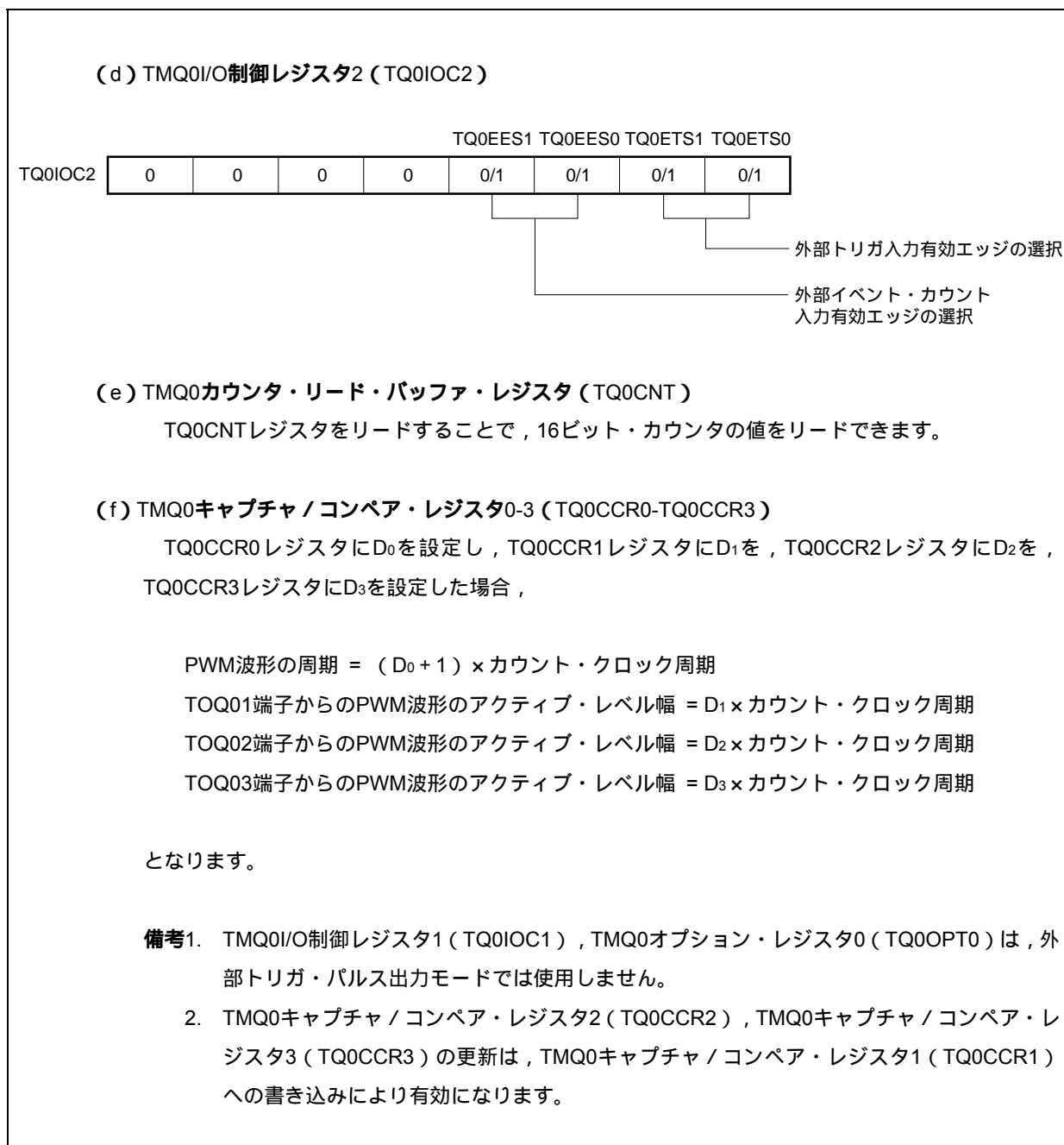
図8 - 18 外部トリガ・パルス出力モード動作時のレジスタ設定内容 (3/3)
