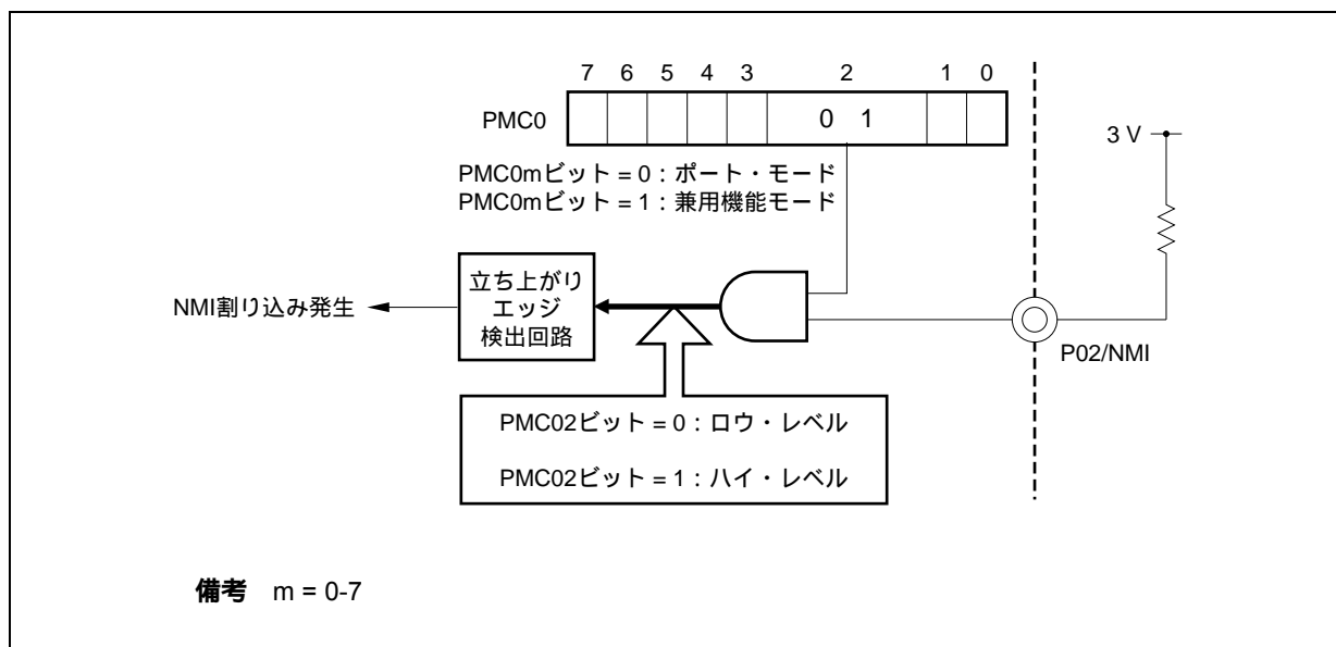
図4 - 41 P02端子からNMI端子への切り替え（悪い例）
