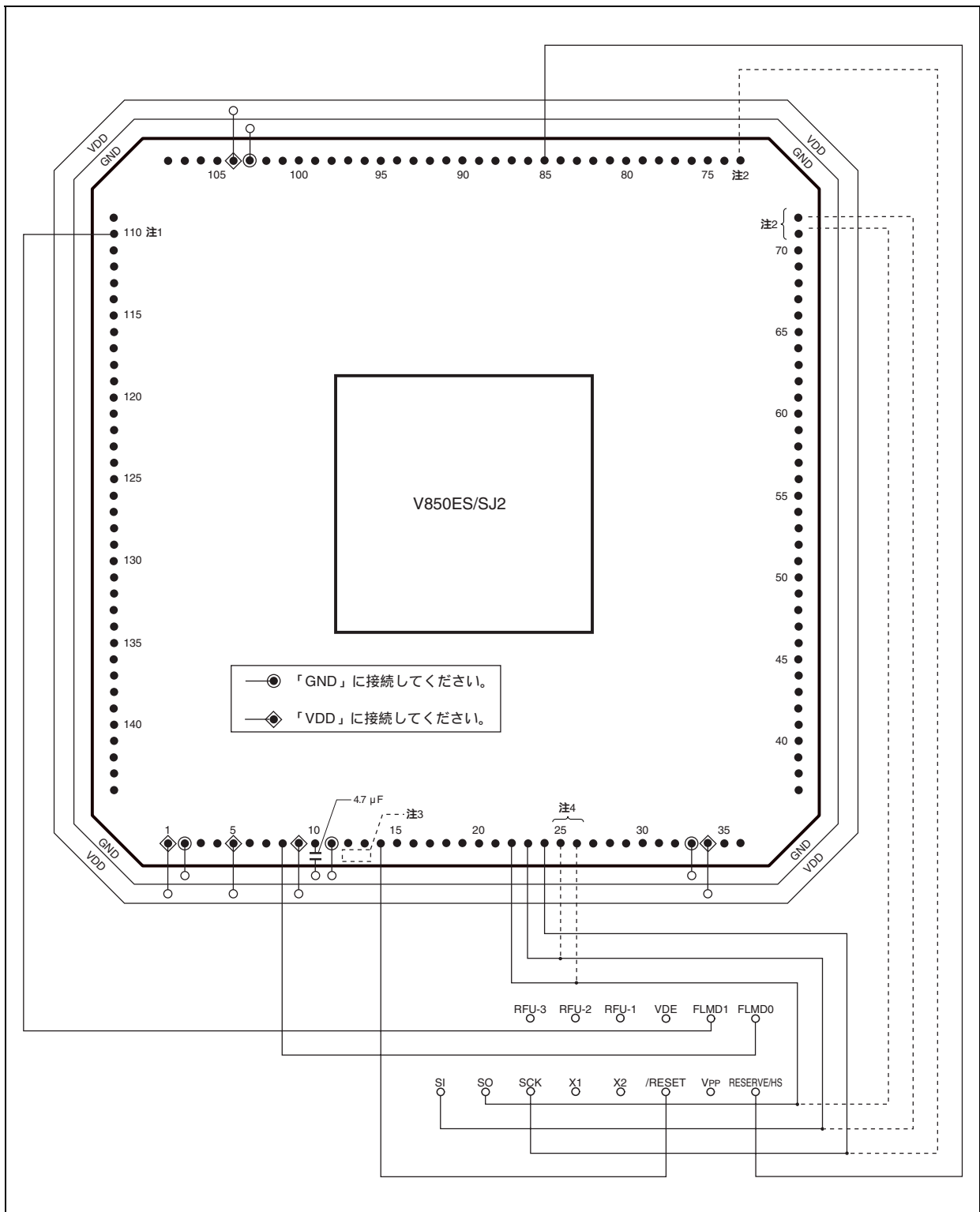
図29 - 6 V850ES/SJ2フラッシュ書き込み用アダプタ (FA-144GJ-UEN) の配線例 (CSIB0 + HSモード時) (1/2)
