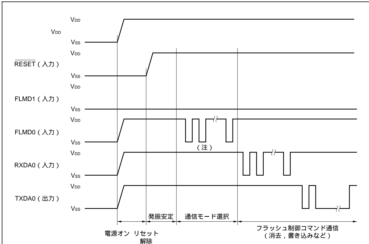
図29 - 8 通信方式の選択
