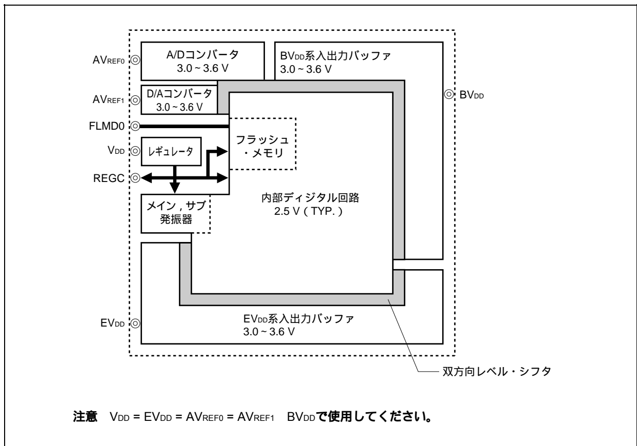
図27 - 1 レギュレータ
