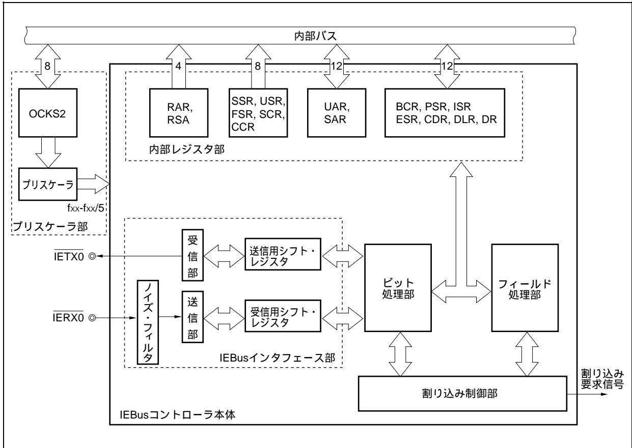
図18 - 10 IEBusコントローラのブロック図
