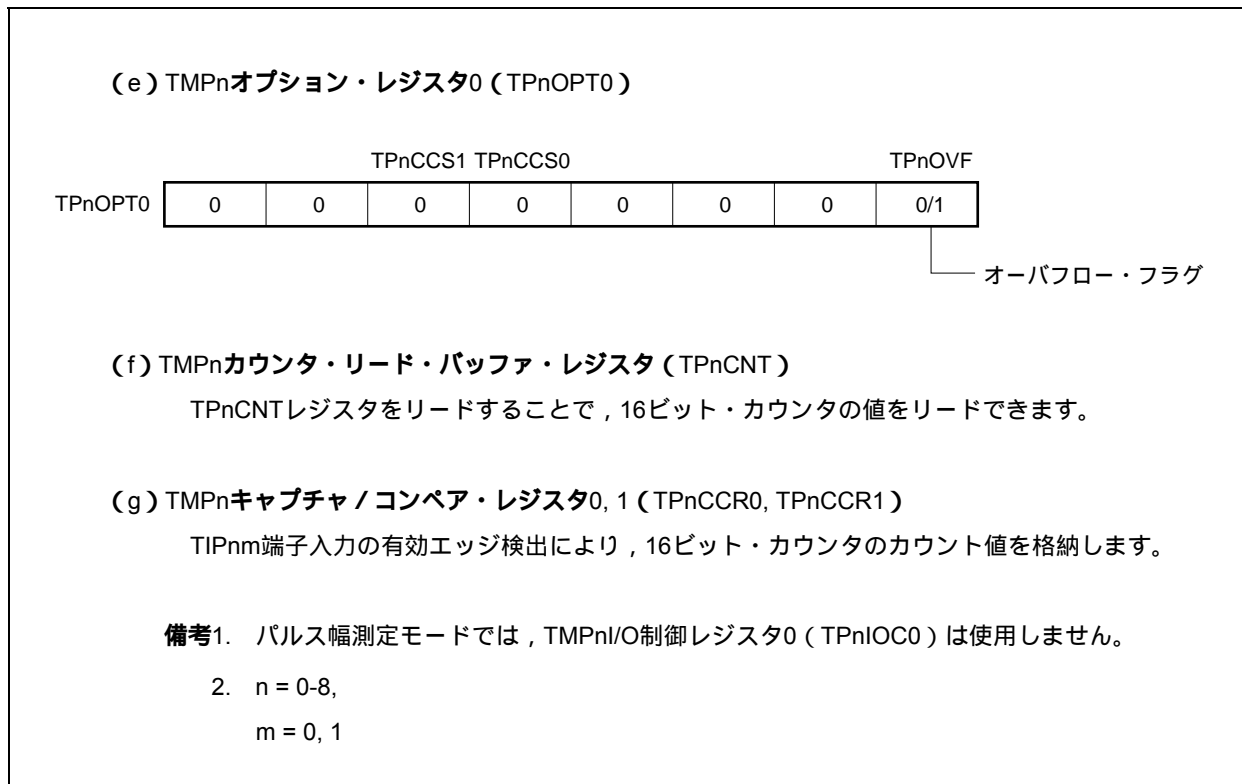
図7 - 36 パルス幅測定モード動作時のレジスタ設定内容 (2/2)
