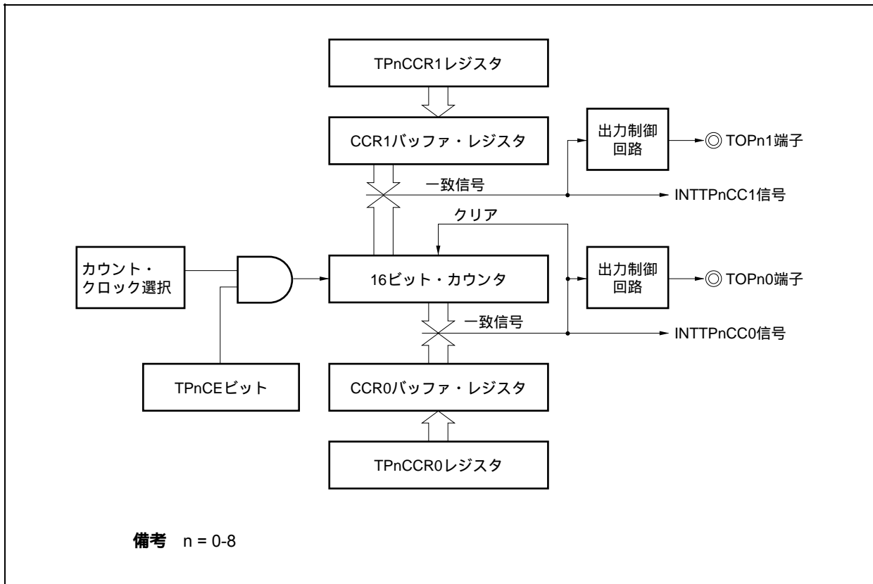
図7-6 TPnCCR1レジスタの構成図
