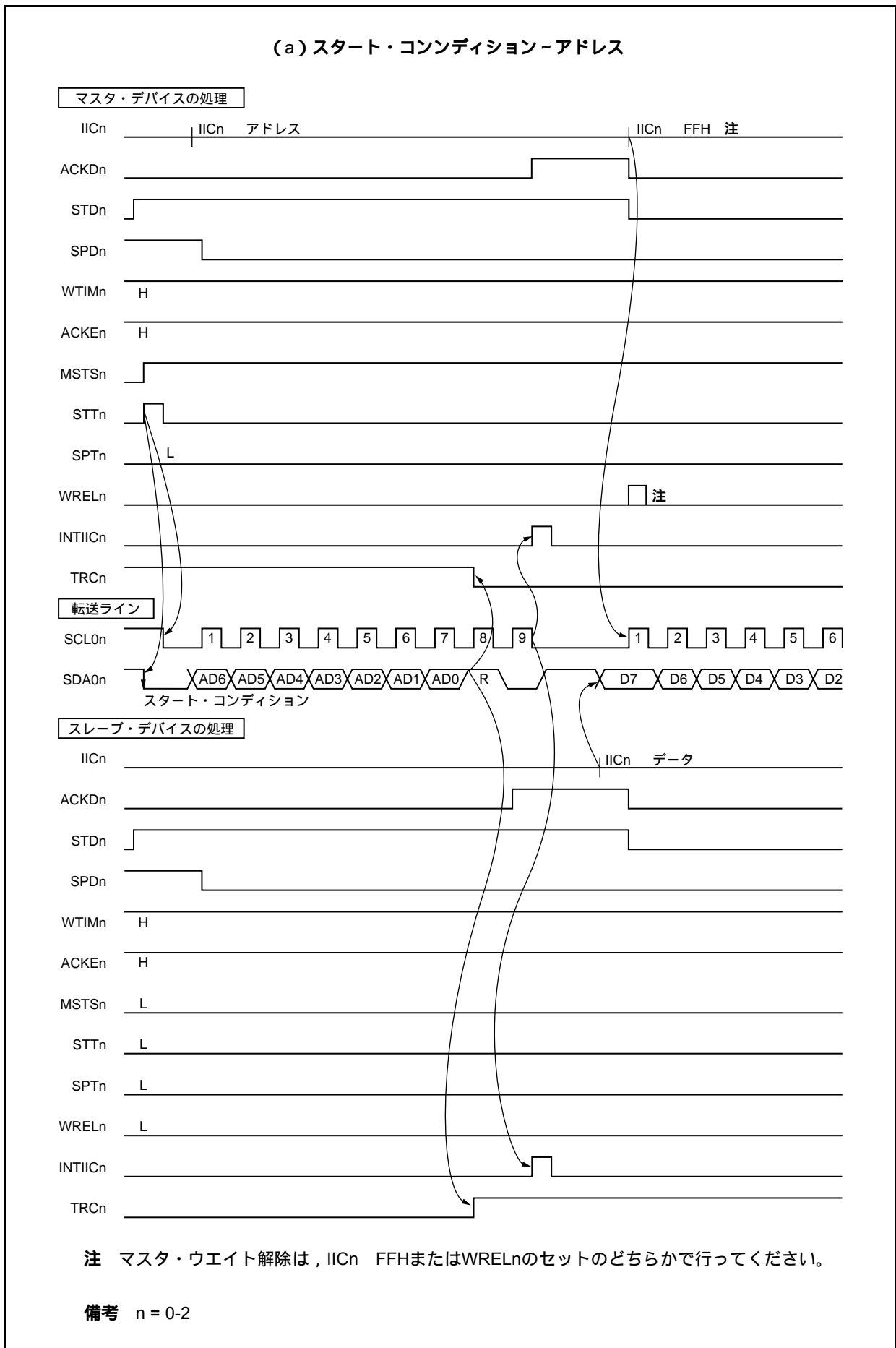
図17-24 スレーブ マスタ通信例 (マスタ, スレーブとも9クロック・ウエイト選択時) (1/3)
