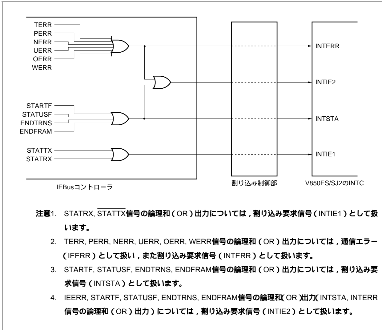
図18 - 20 割り込み制御部の構成
