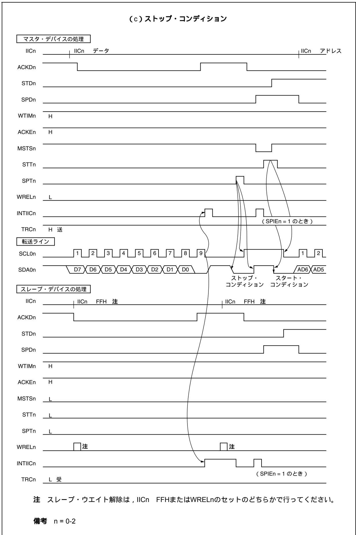
図17-23 マスタ スレーブ通信例 (マスタ, スレーブとも9クロック・ウエイト選択時) (3/3)
