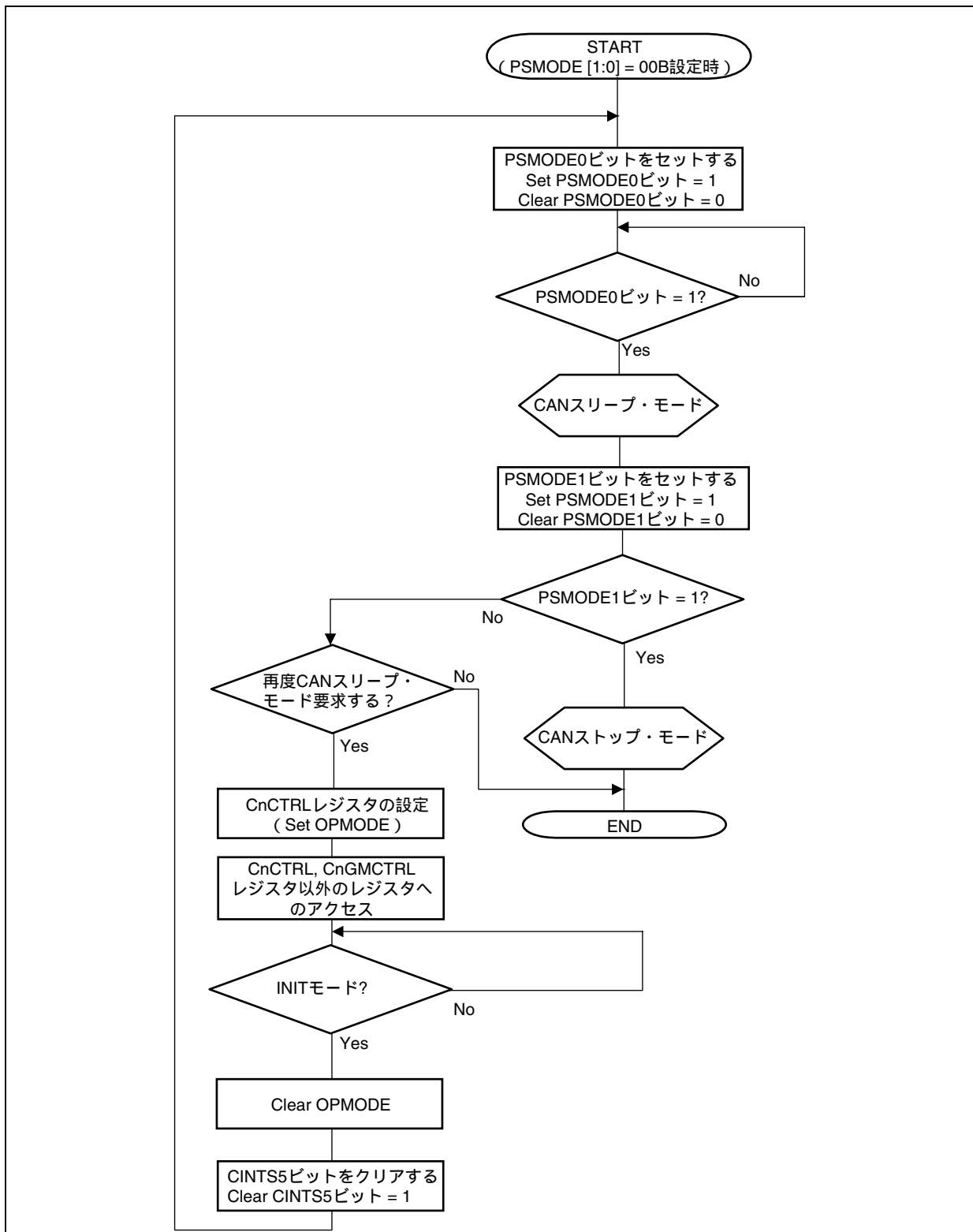
図19 - 51 CANスリープ・モード/CANストップ・モードの設定
