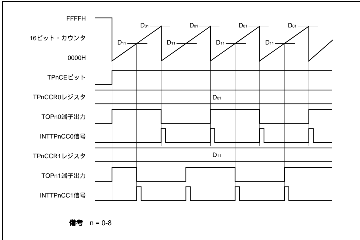
図7-7 D 01 D 11 の場合のタイミング図
