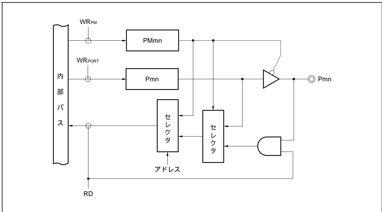
図4-6 タイプC-1のブロック図
