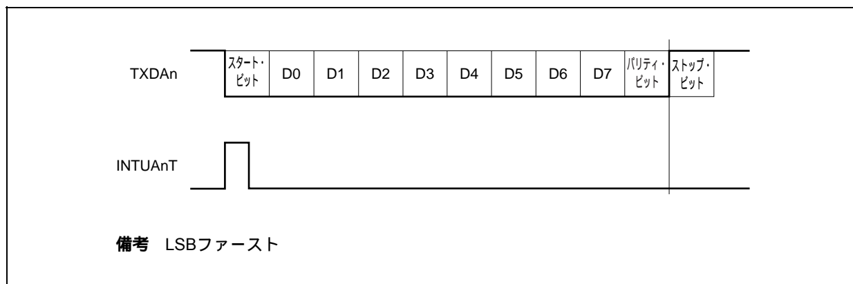
図15 - 10 UART送信
