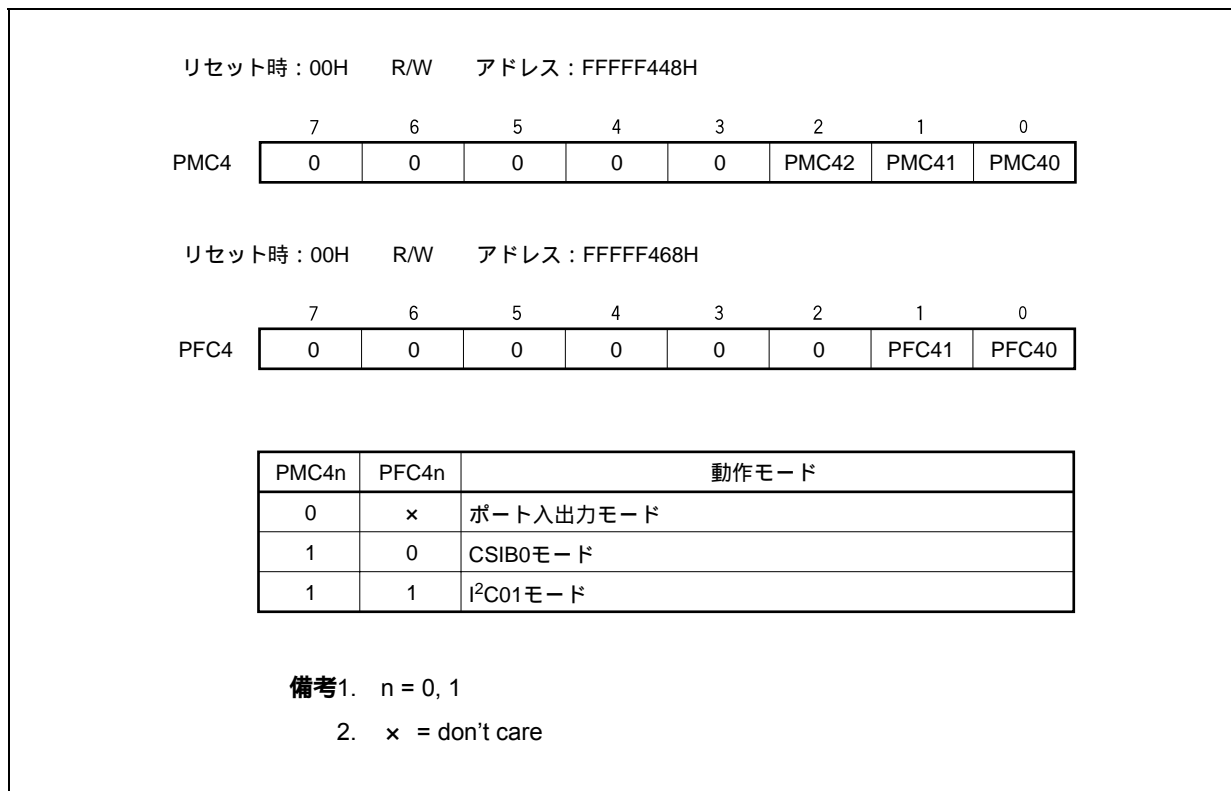
図16 - 2 CSIB0とI 2 C01のモード切り替え設定
