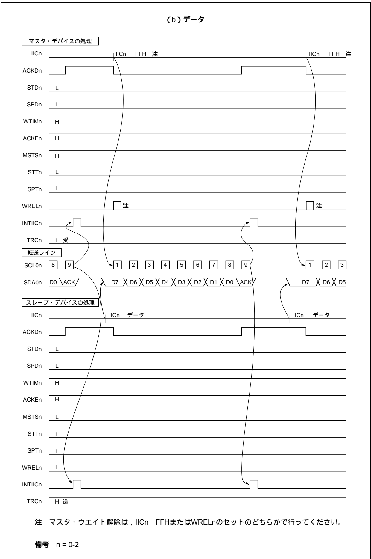
図17-24 スレーブ マスタ通信例 (マスタ, スレーブとも9クロック・ウエイト選択時) (2/3)
