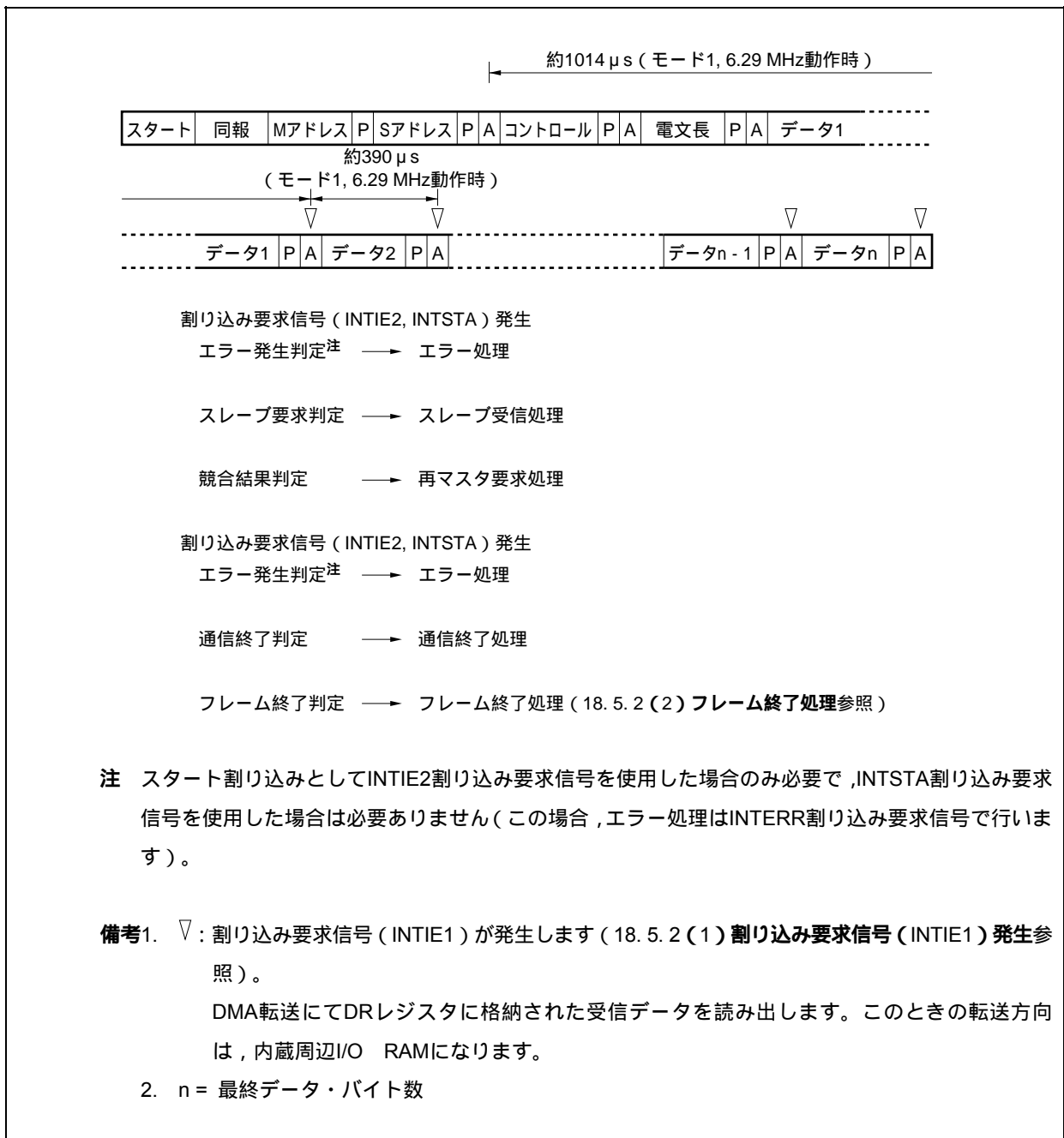
図18 - 27 マスタ受信
