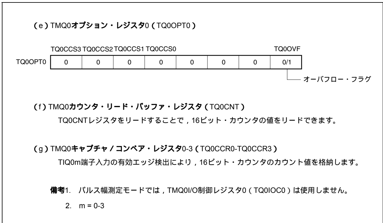
図8 - 36 パルス幅測定モード動作時のレジスタ設定内容 (2/2)
