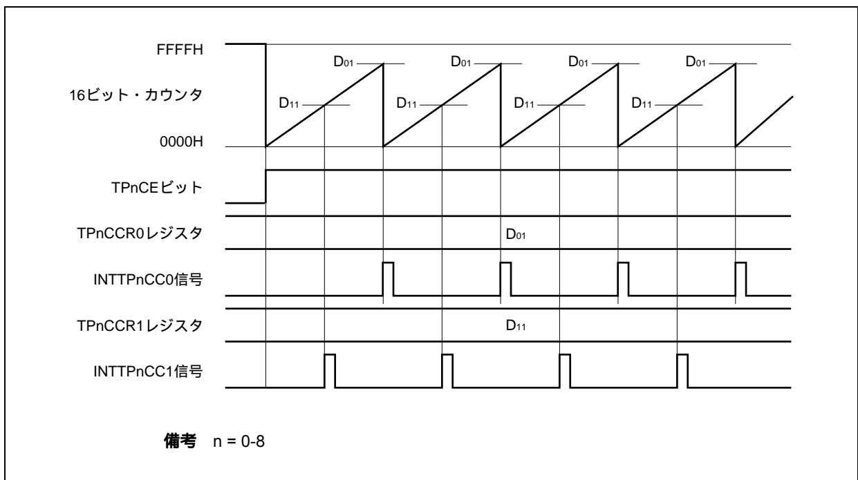
図7 - 14 D 01 D 11 の場合のタイミング図
