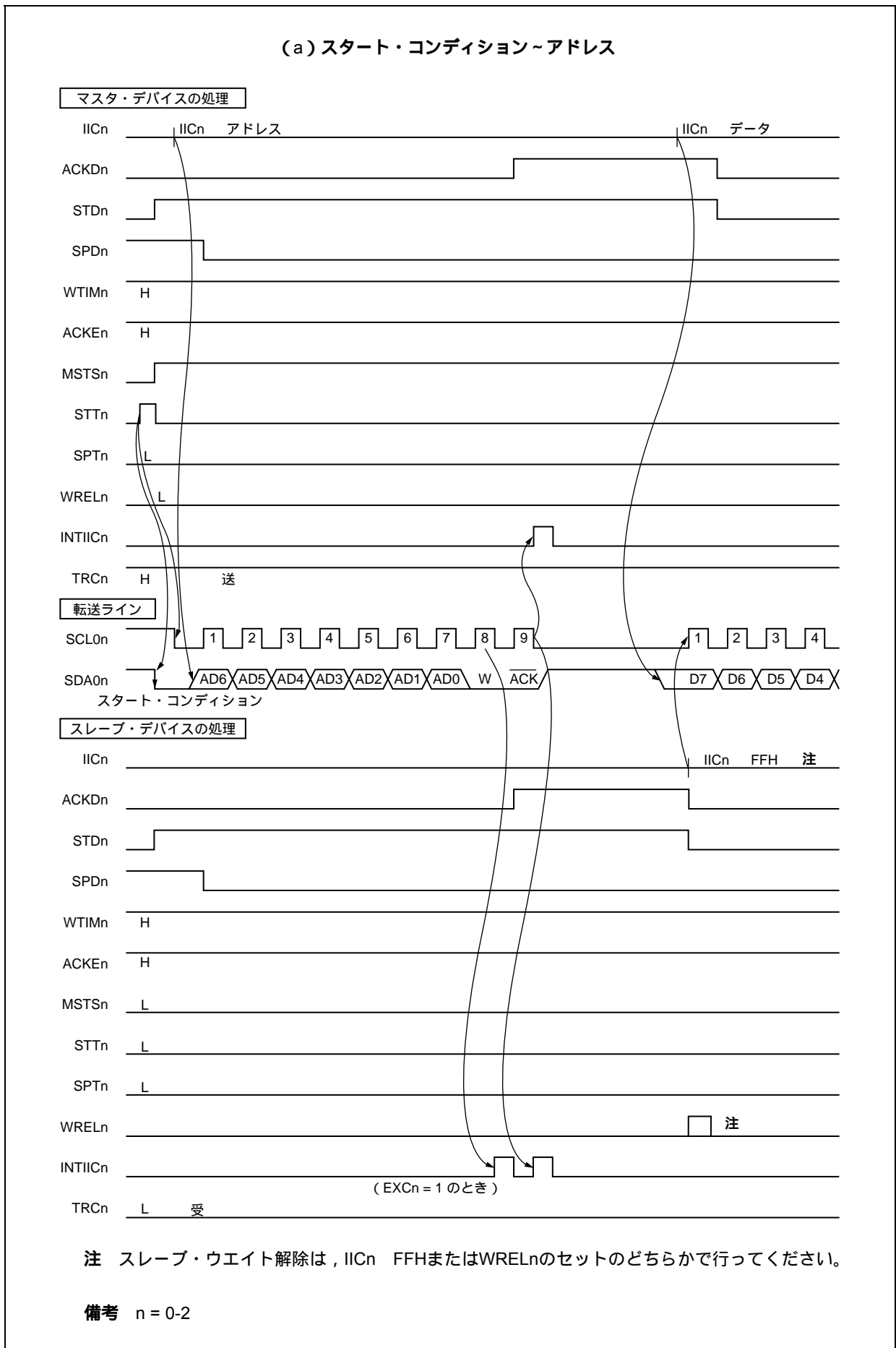
図17-23 マスタ スレーブ通信例 (マスタ, スレーブとも9クロック・ウエイト選択時) (1/3)
