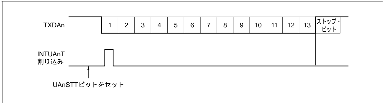
図15 - 8 SBF送信
