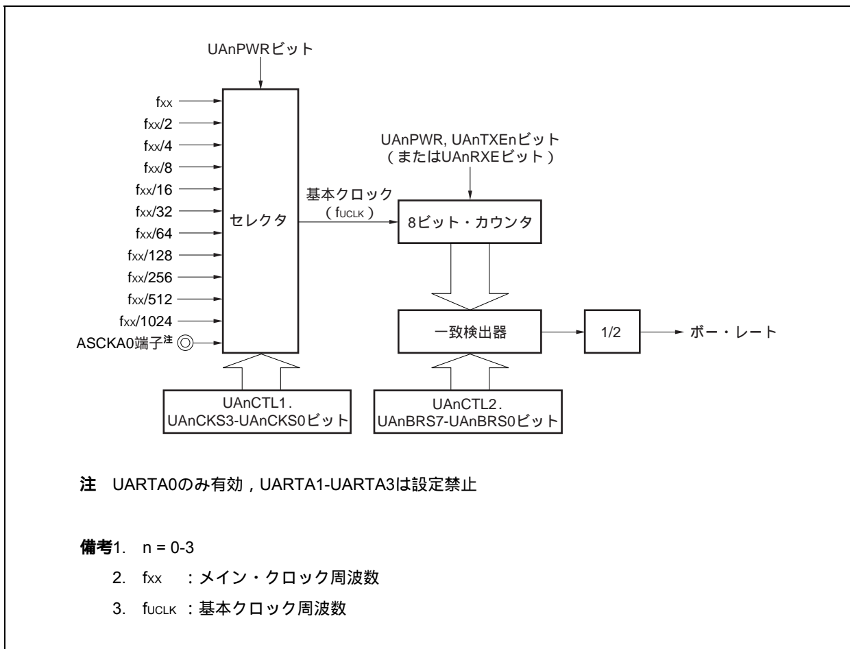
図15-16 ポー・レート・ジェネレータの構成
