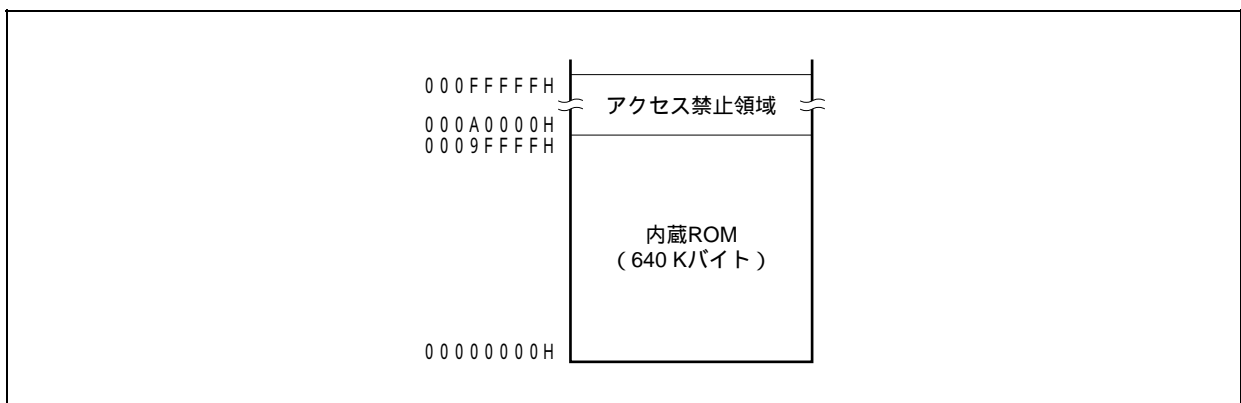
図3 - 5 内蔵ROM領域 (640 Kバイト)
