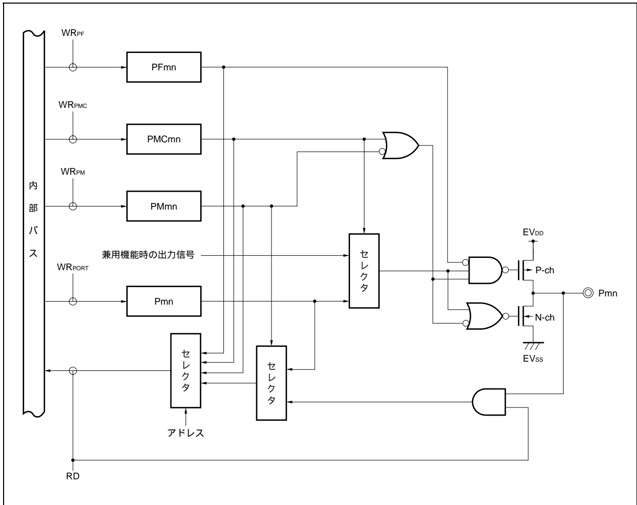
図4 - 11 タイプE - 2のブロック図
