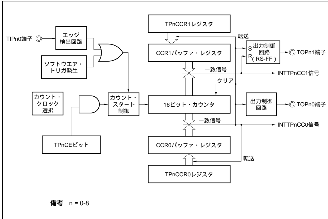
図7 - 16 外部トリガ・パルス出力モードの構成図
