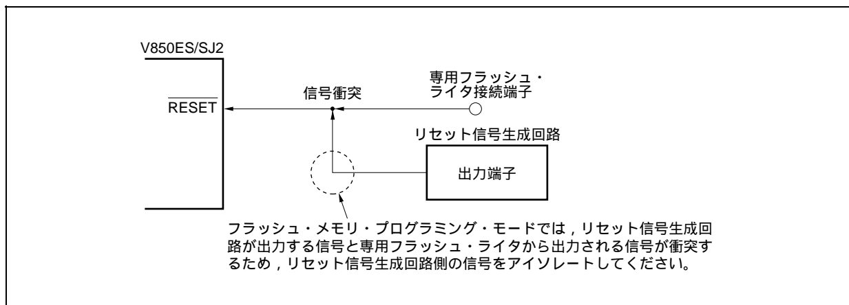
図29 - 14 信号の衝突 (RESET端子)
