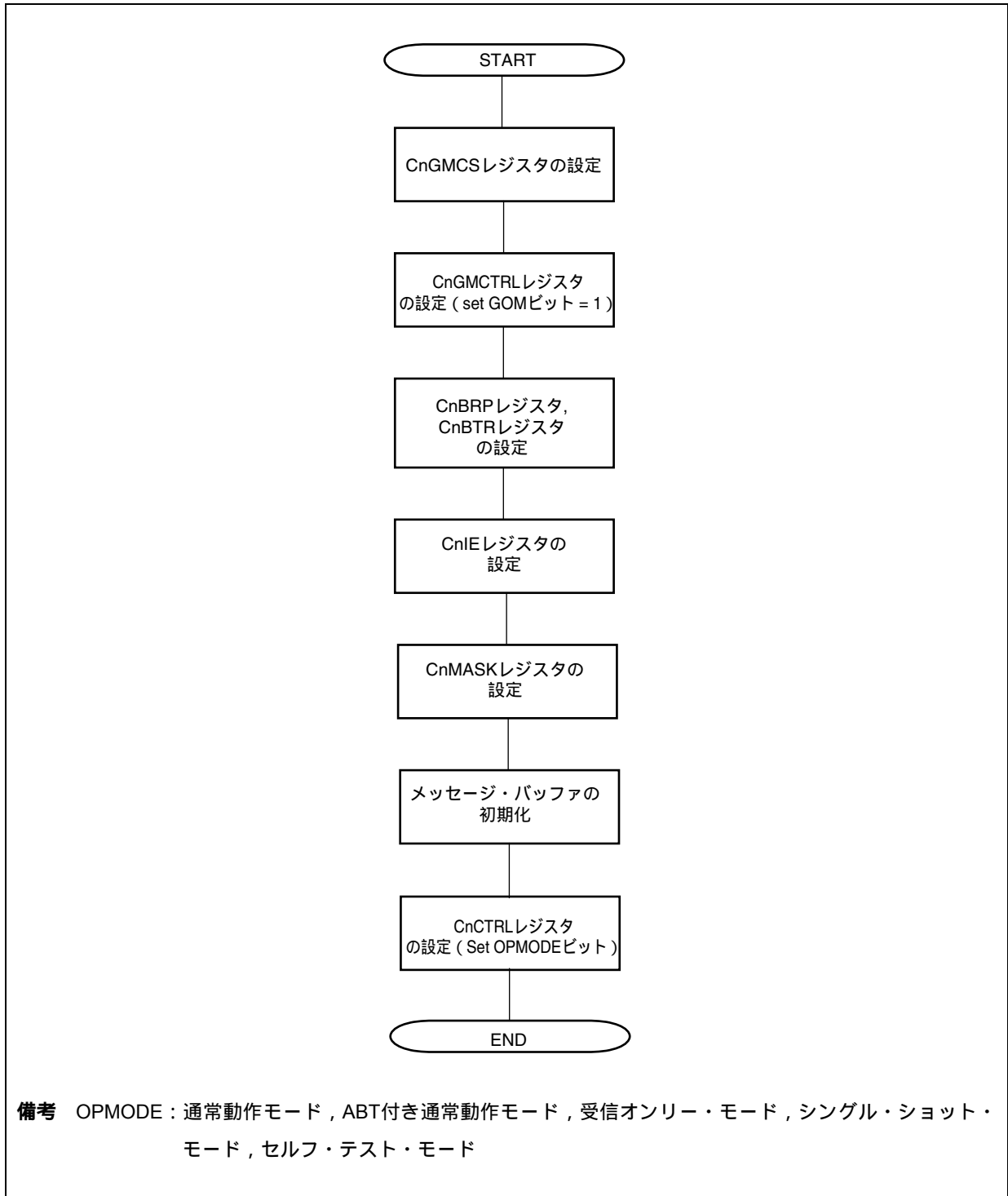
図19 - 35 初期化
