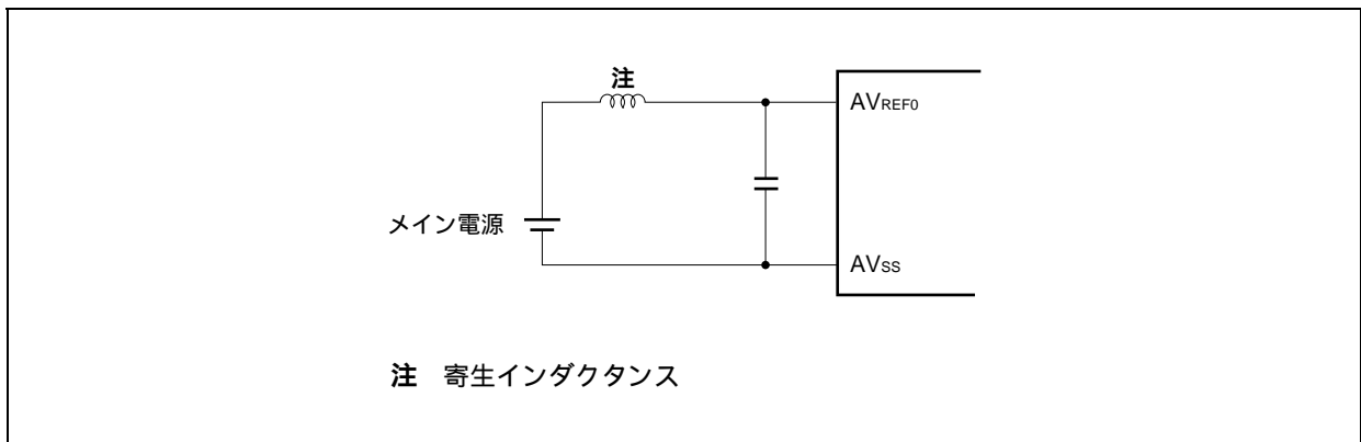
図13 - 15 AV REF0 端子の処理例
