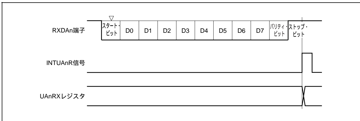
図15 - 13 UART受信
