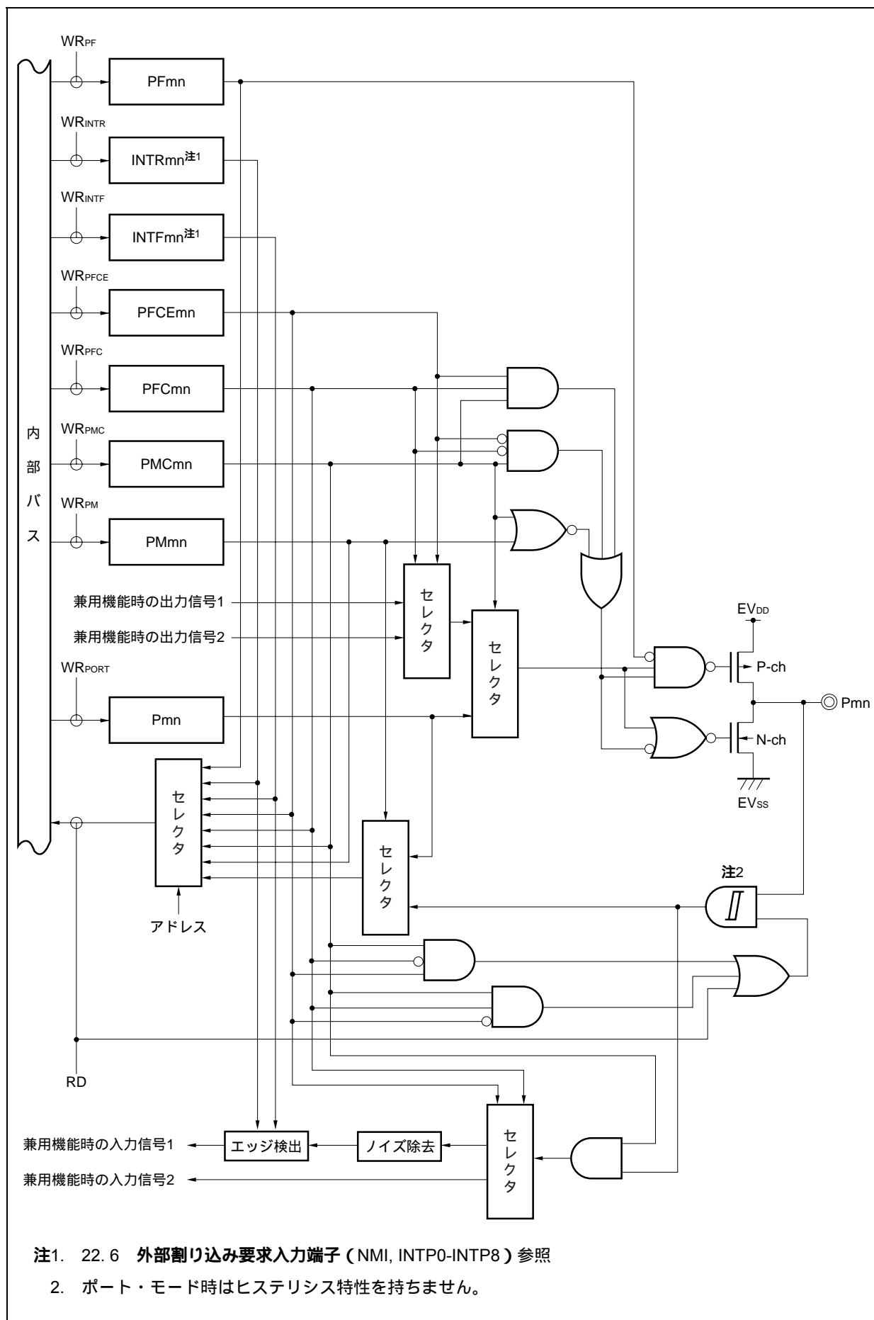
図4 - 39 タイプU - 15のブロック図
