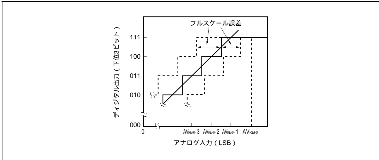
図13 - 19 フルスケール誤差
