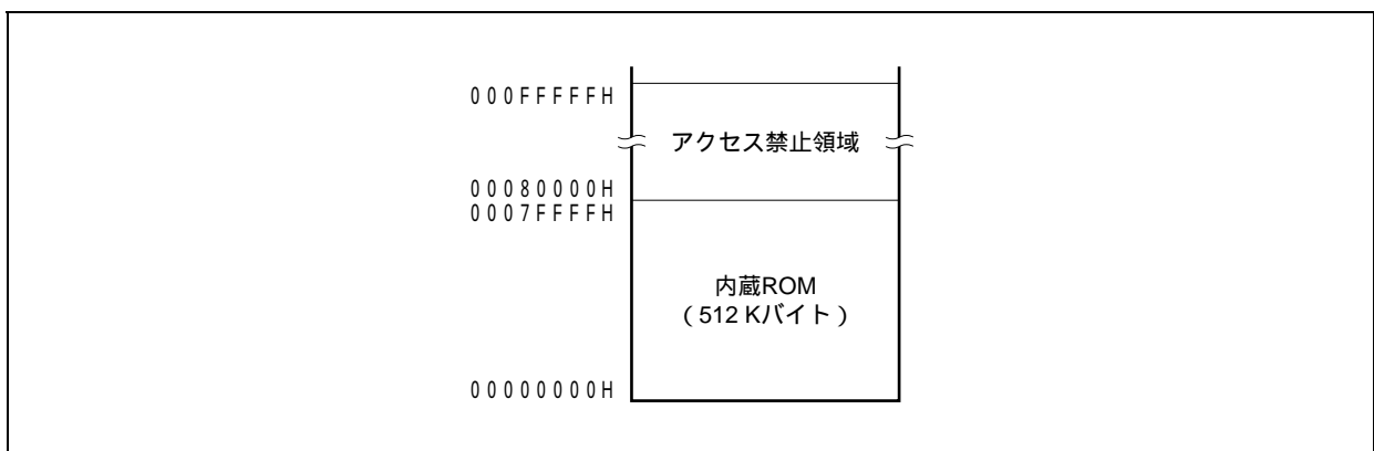
図3 - 4 内蔵ROM領域 (512 Kバイト)
