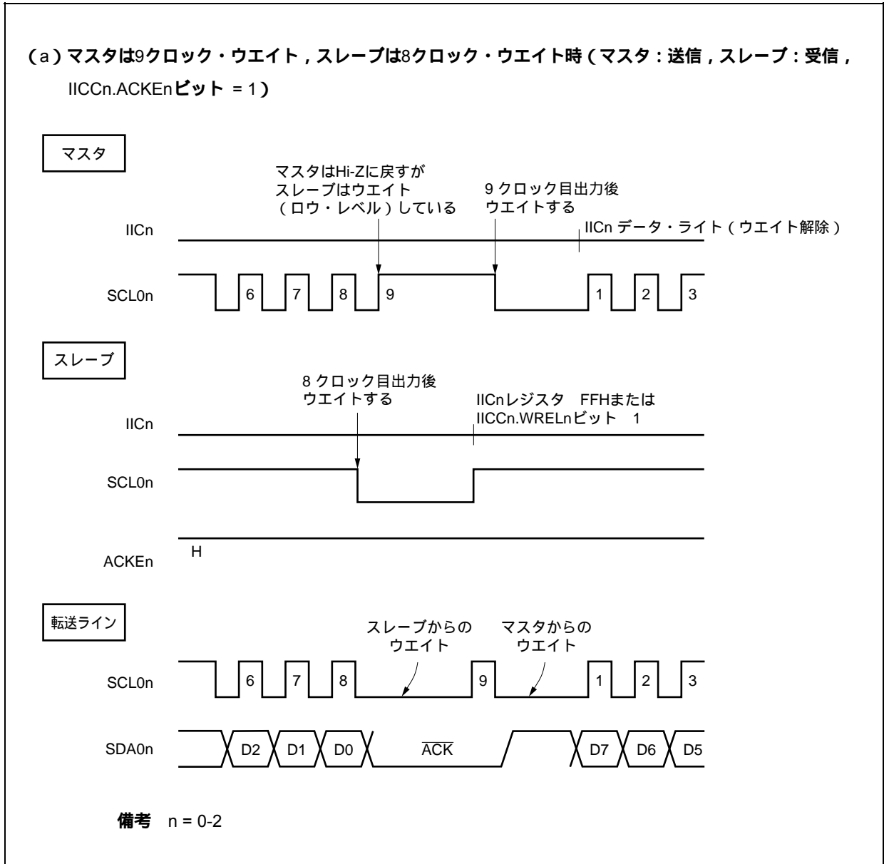
図17 - 13 ウェイト（1/2）
