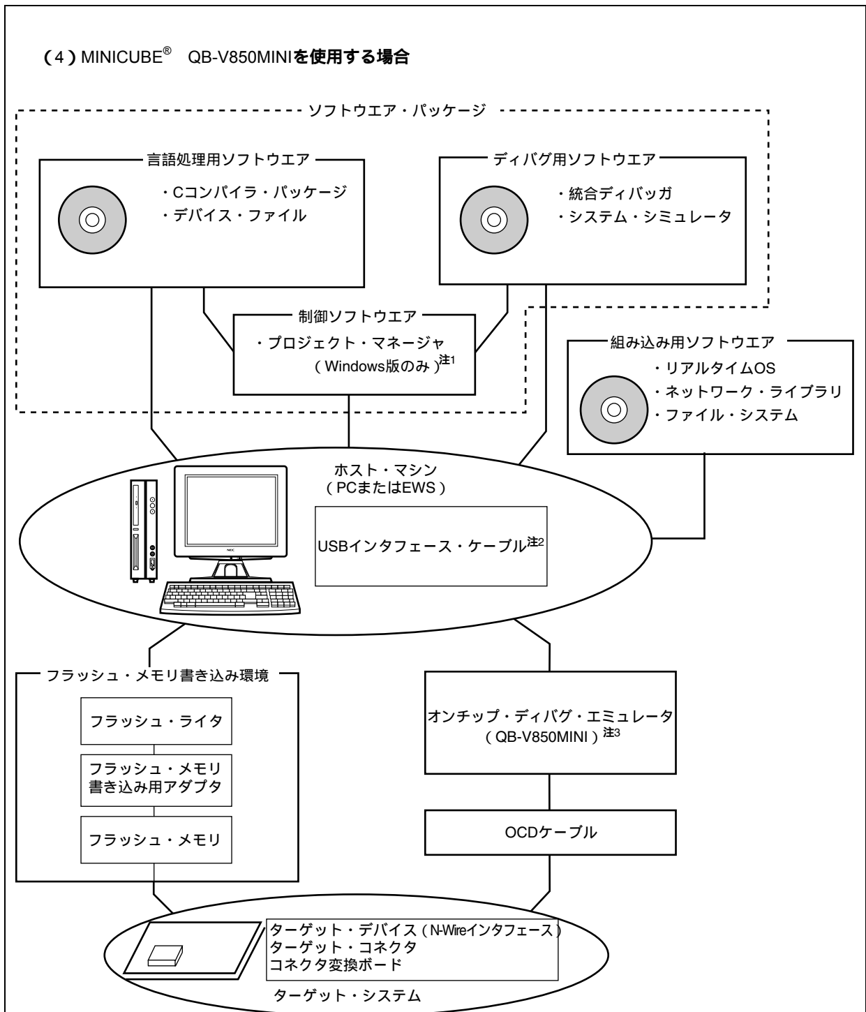
図A - 1 開発ツール構成 (4/4)
