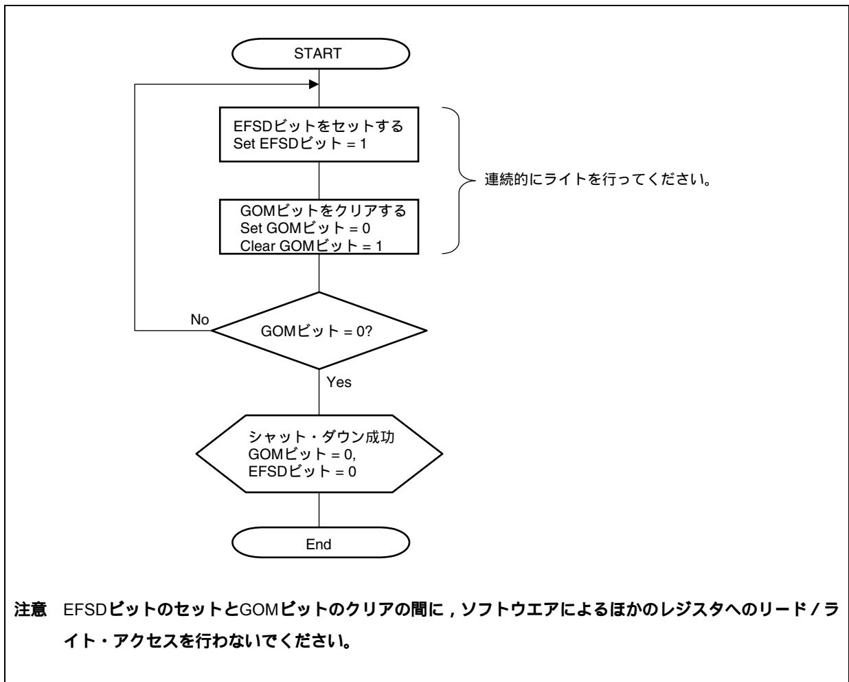
図19 - 55 強制シャット・ダウン処理
