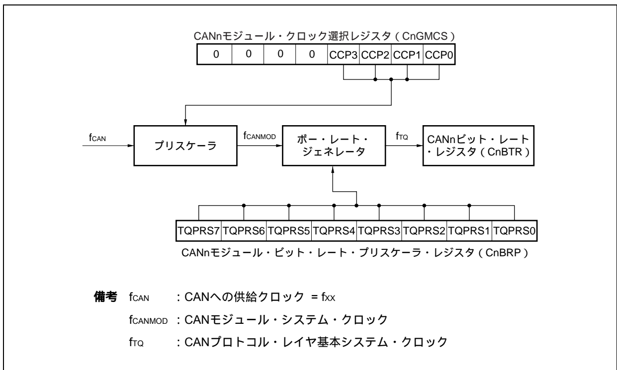
図19 - 23 CANモジュールのクロック
