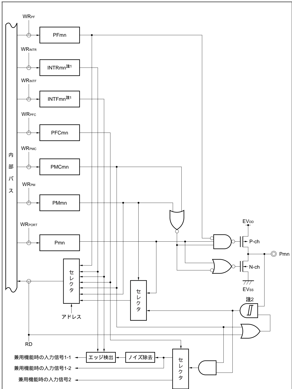
図4 - 24 タイプN - 3のブロック図
