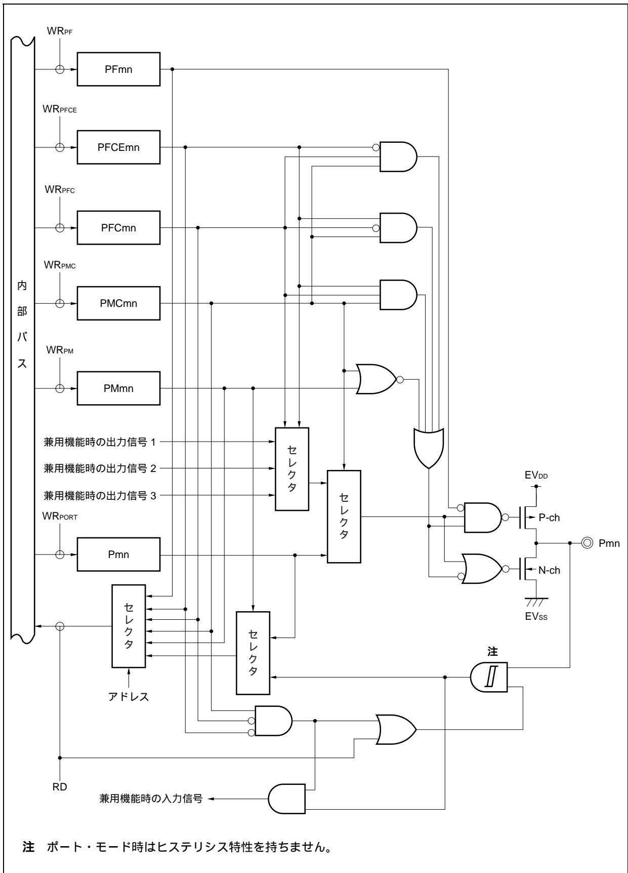
図4 - 26 タイプU - 2のブロック図
