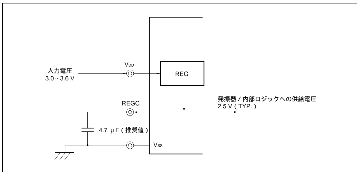
図27 - 2 REGC端子の接続
