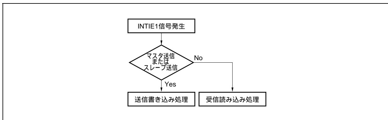
図18 - 24 INTIE1信号の割り込み判定例 (INTIE1, INTIE2信号使用時)
