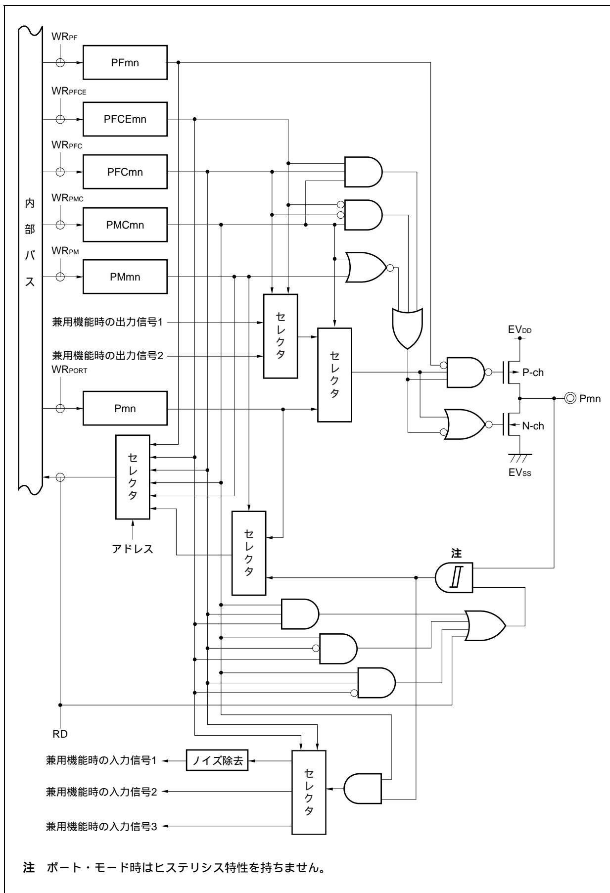
図4 - 35 タイプU - 11のブロック図
