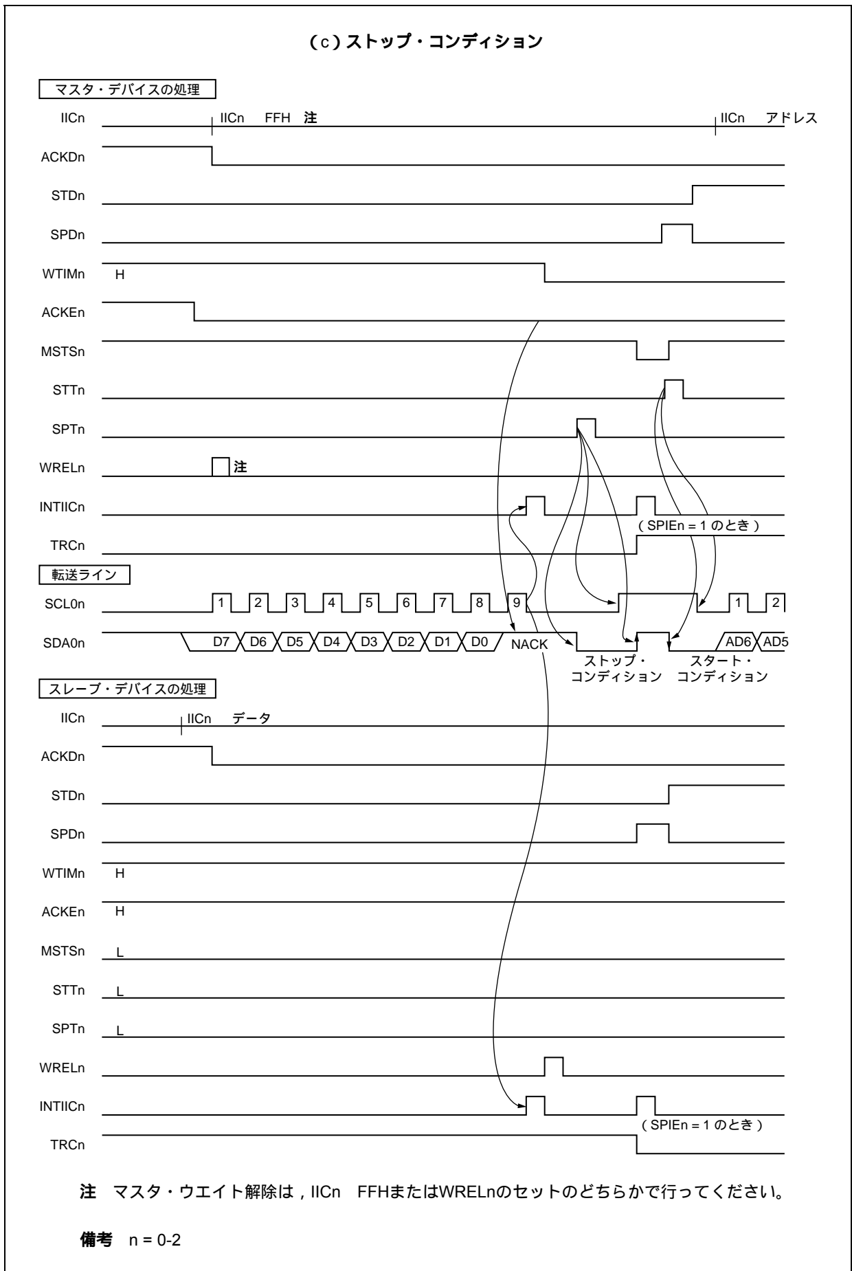
図17-24 スレーブ マスタ通信例 (マスタ, スレーブとも9クロック・ウエイト選択時) (3/3)
