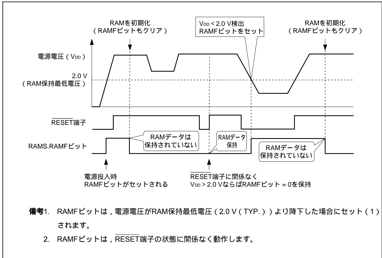
図25 - 7 RAM保持電圧検出機能の動作タイミング
