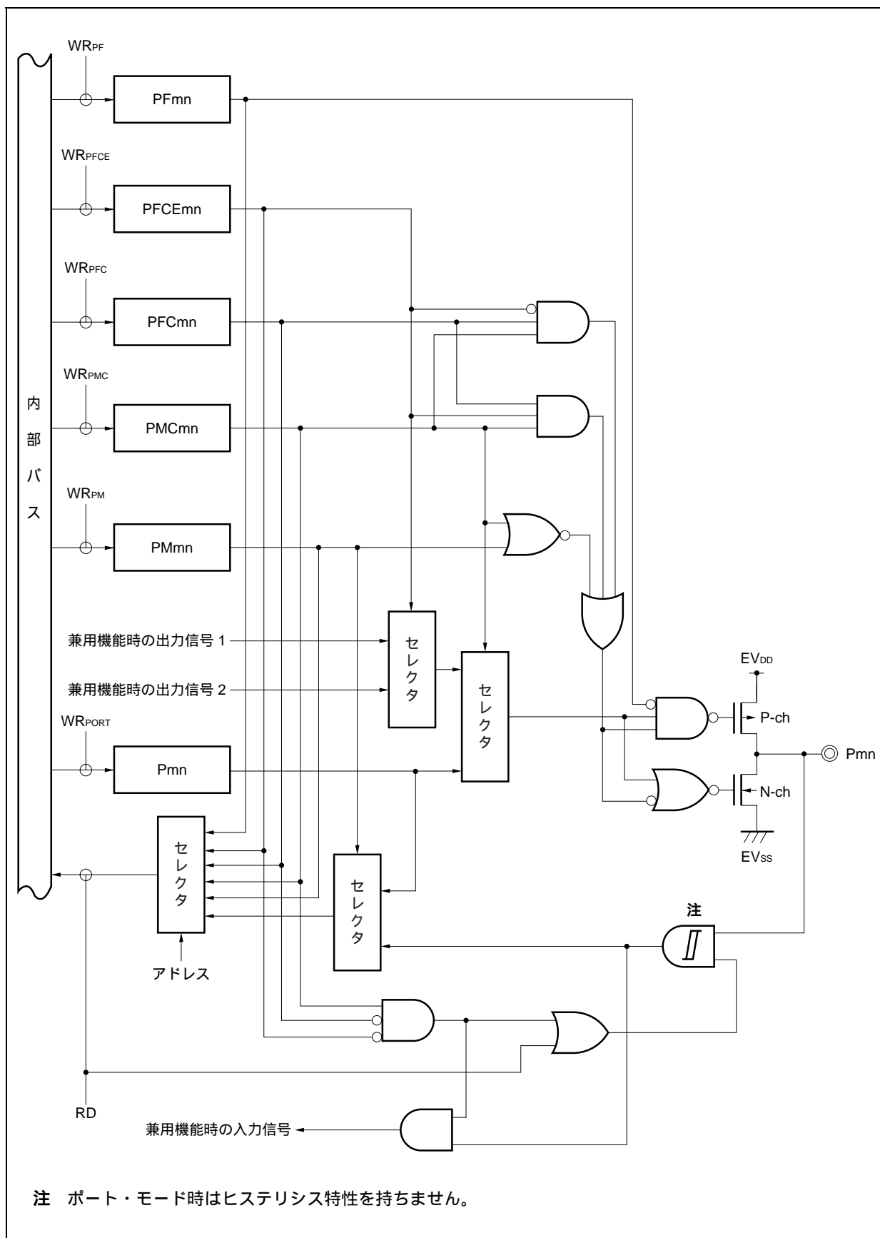
図4 - 28 タイプU - 4のブロック図
