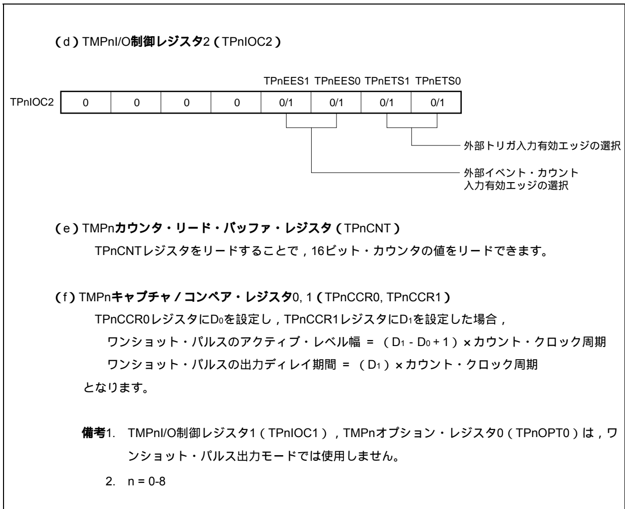
図7 - 22 ワンショット・パルス出力モード動作時のレジスタ設定内容 (2/2)
