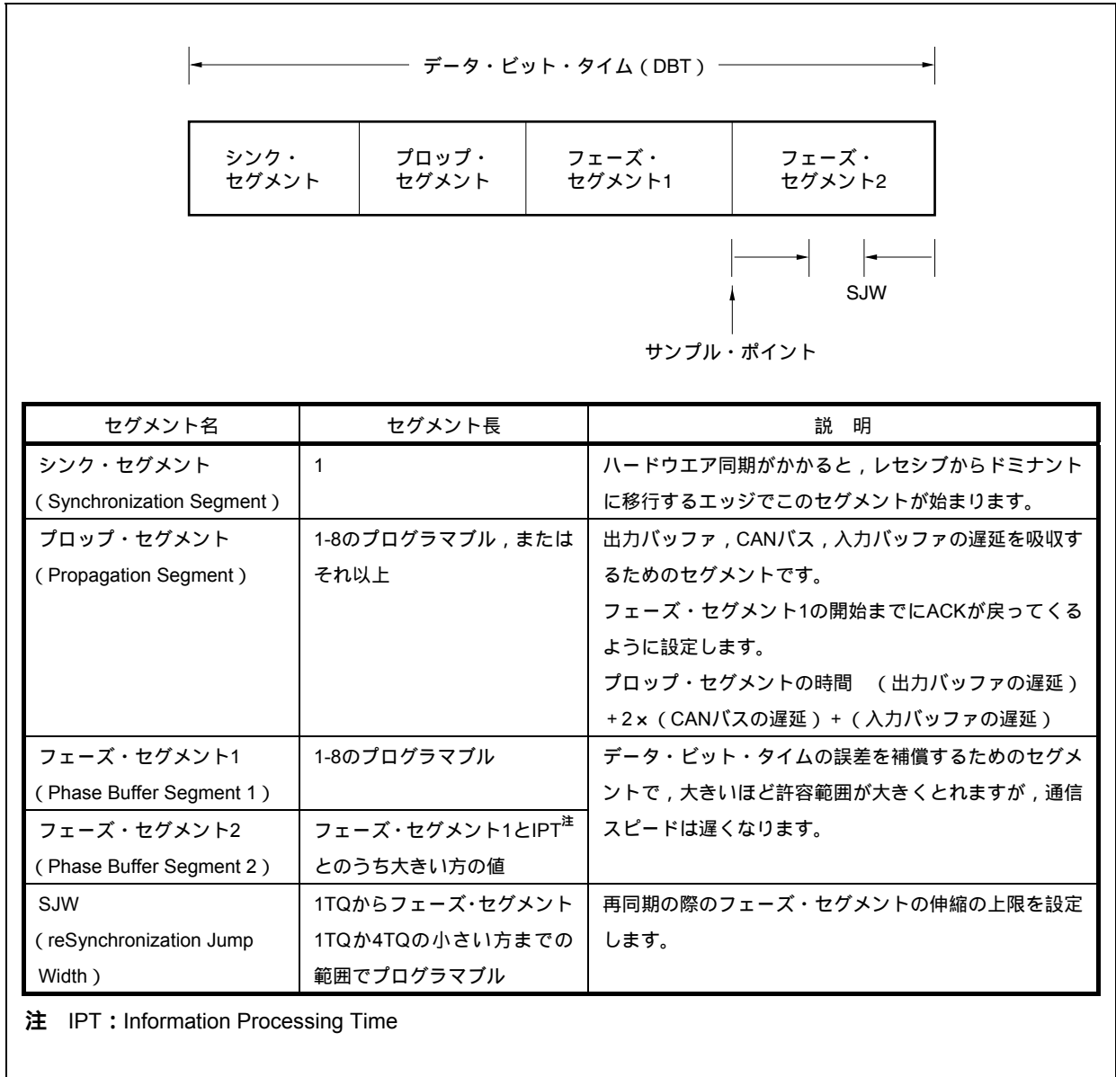
図19 - 19 CANスペック上でのデータ・ビット・タイムの構成
