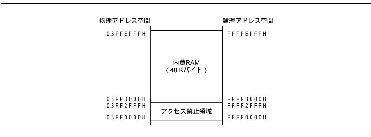
図3 - 7 内蔵RAM領域 (48 Kバイト)
