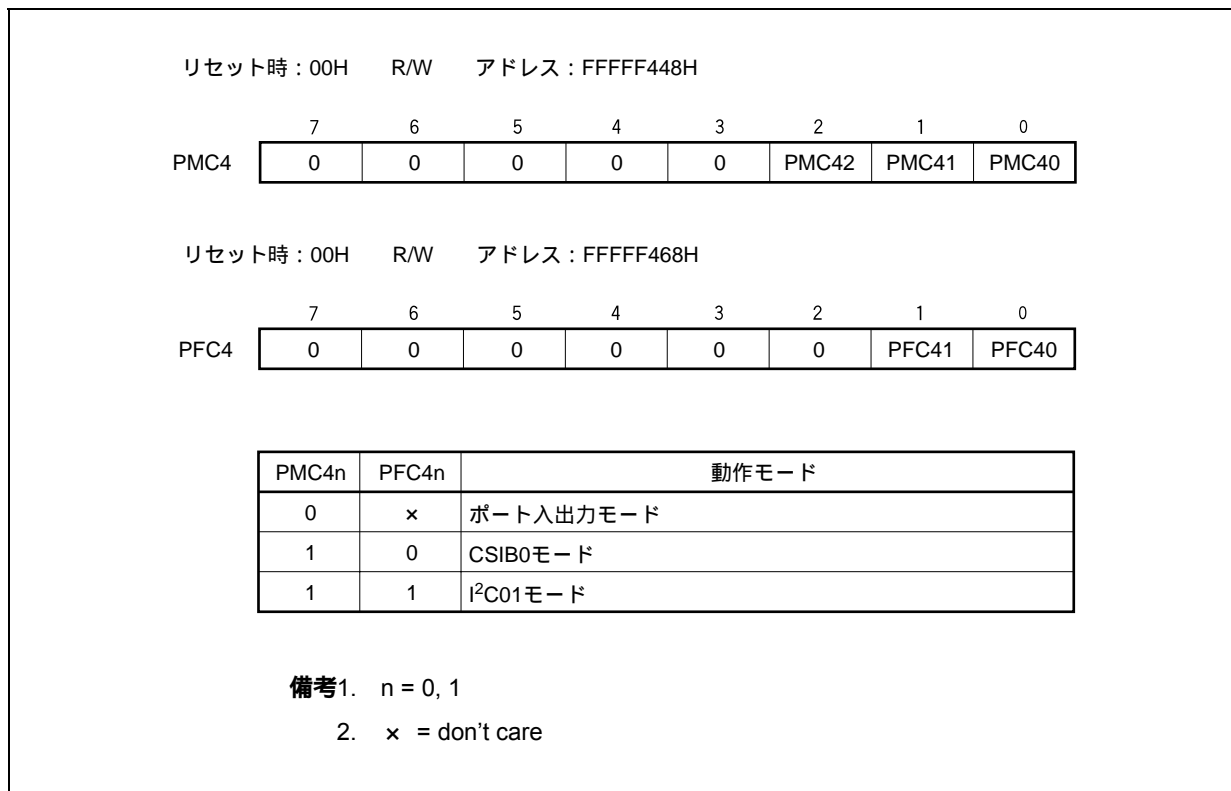
図17-2 CSIB0とI 2 C01のモード切り替え設定
