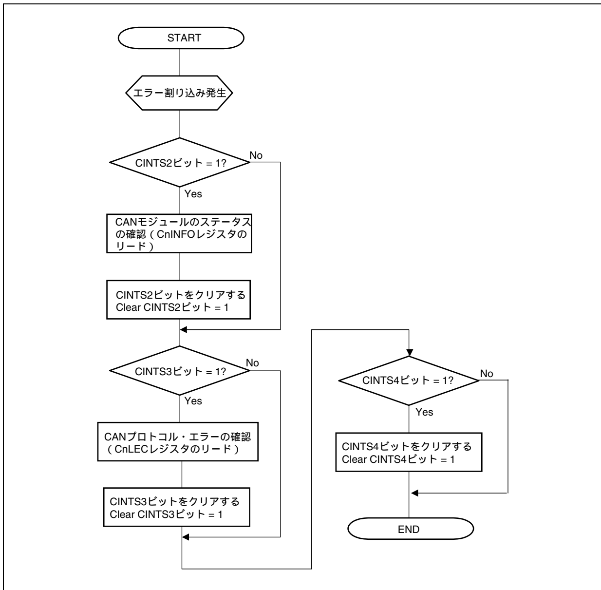
図19 - 56 エラー処理
