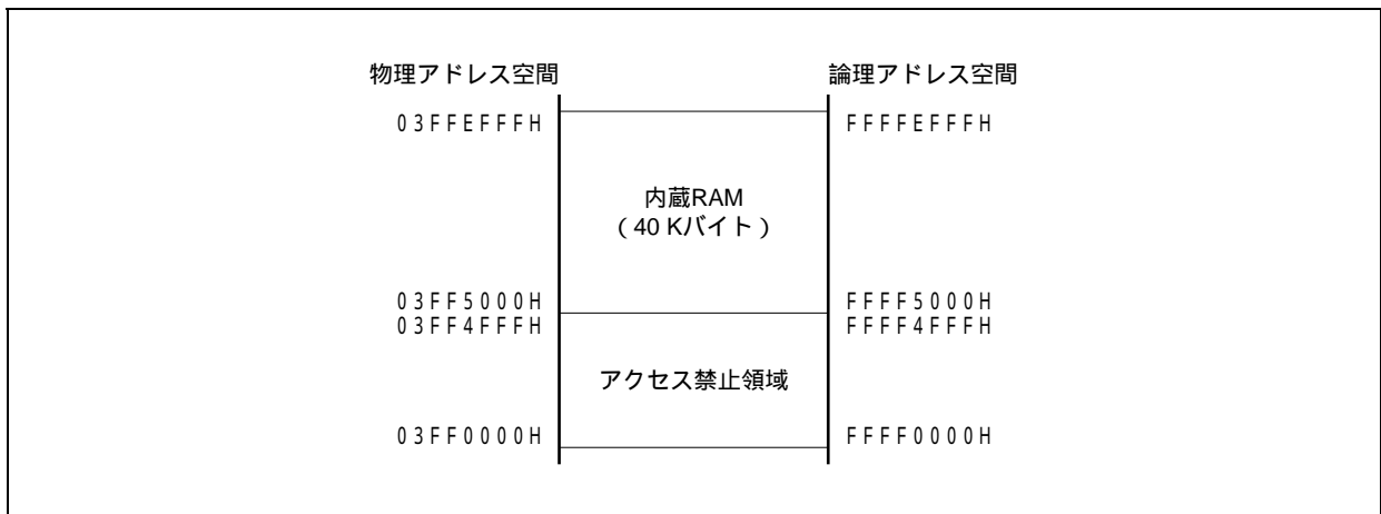
図3 - 6 内蔵RAM領域 (40 Kバイト)
