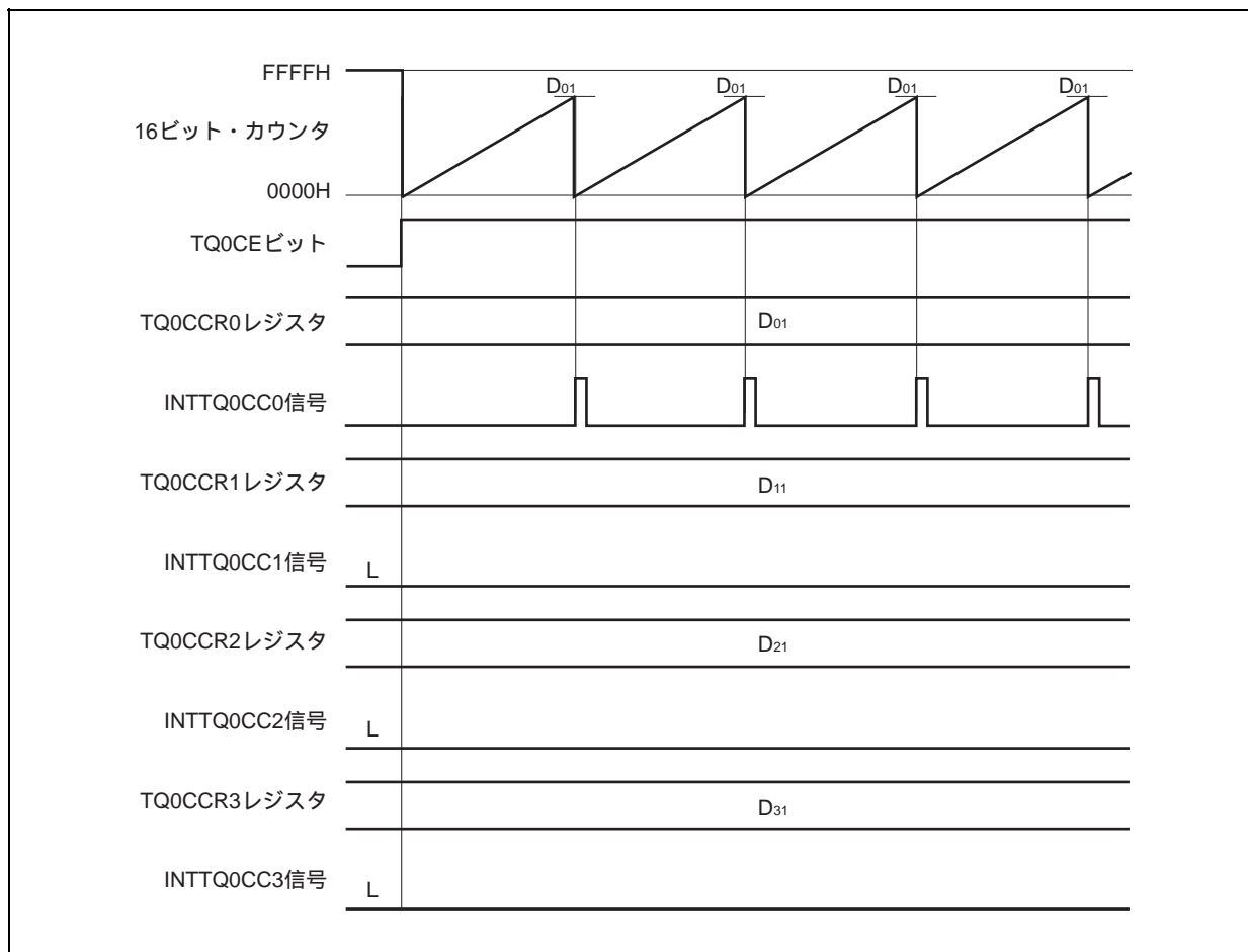
図8 - 15 D 01 < D k1 の場合のタイミング図
