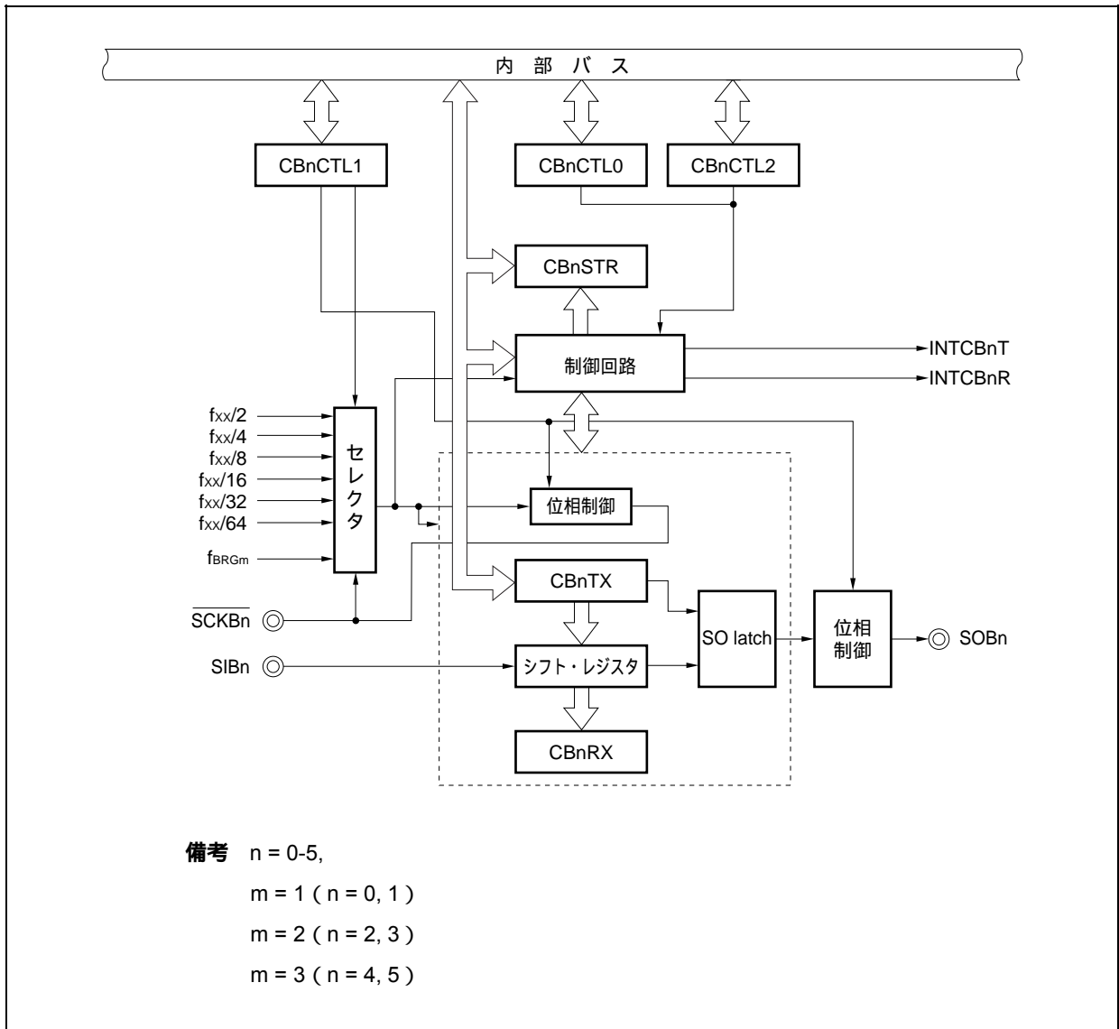
図16-3 CSIBnのブロック図
