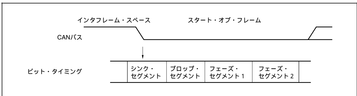
図19 - 20 データ・ビットの同期の調整
