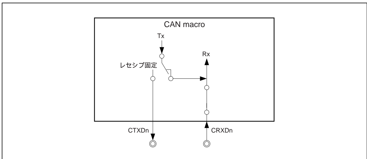
図19 - 32 受信オンリー・モードにおけるCAN端子接続
