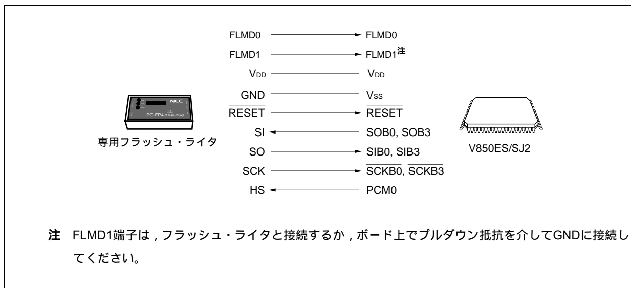
図29 - 5 専用フラッシュ・ライタとの通信 (CSIB0 + HS, CSIB3 + HS)
