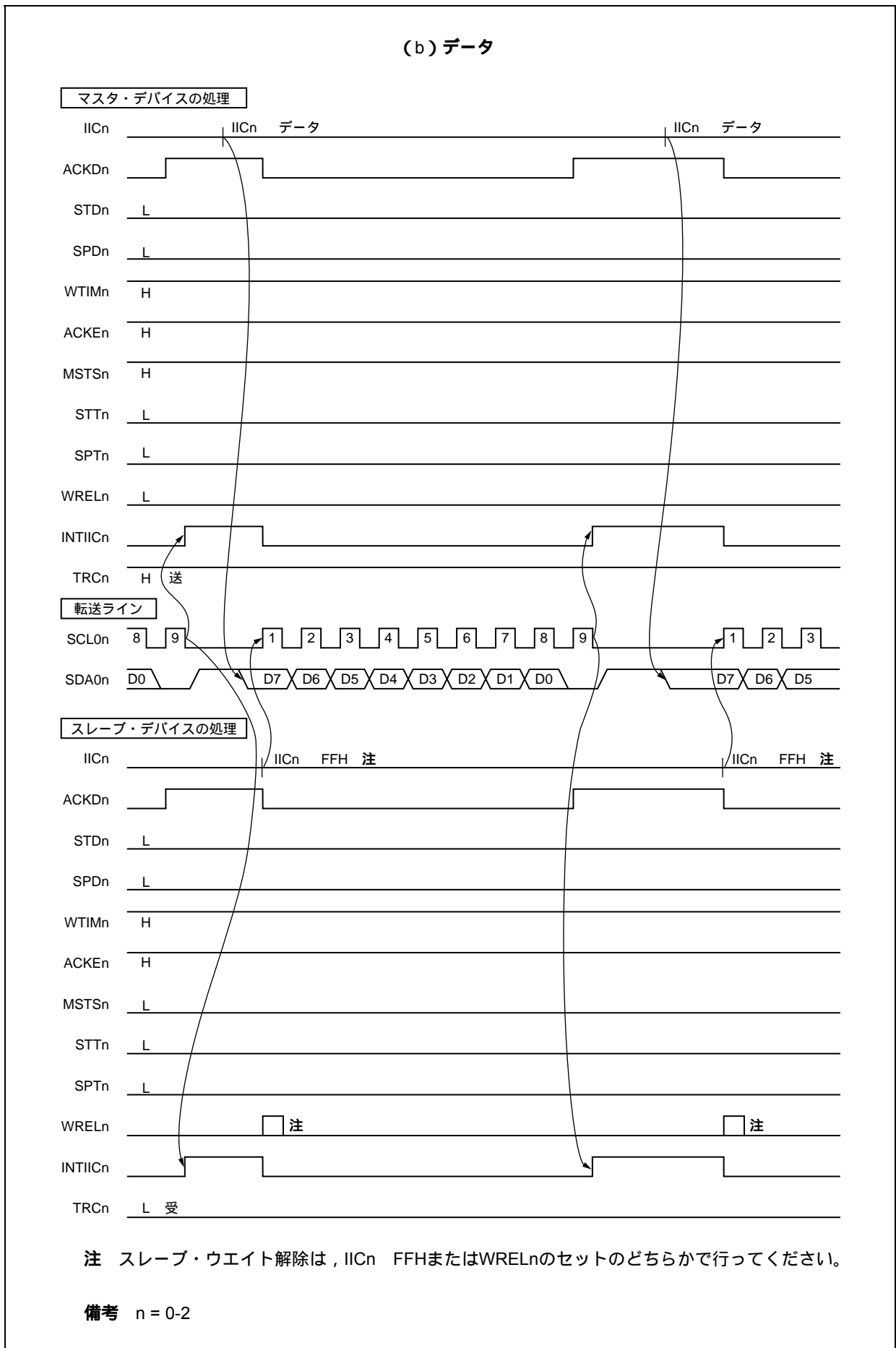
図17-23 マスタ スレーブ通信例 (マスタ, スレーブとも9クロック・ウエイト選択時) (2/3)
