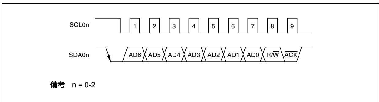
図17 - 11 アクノリッジ
