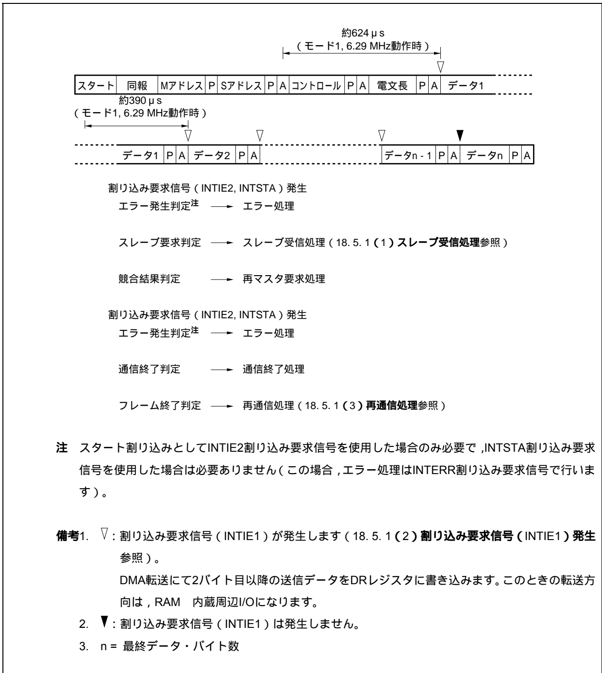
図18 - 26 マスタ送信
