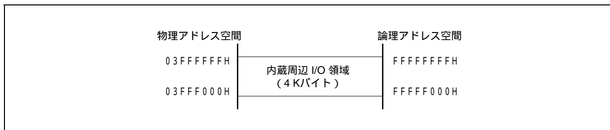
図3 - 8 内蔵周辺I/O領域
