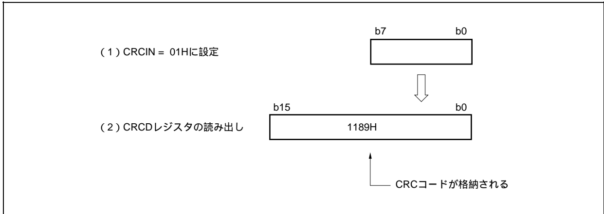
図21 - 2 CRC演算回路の演算例 (LSBファースト)
