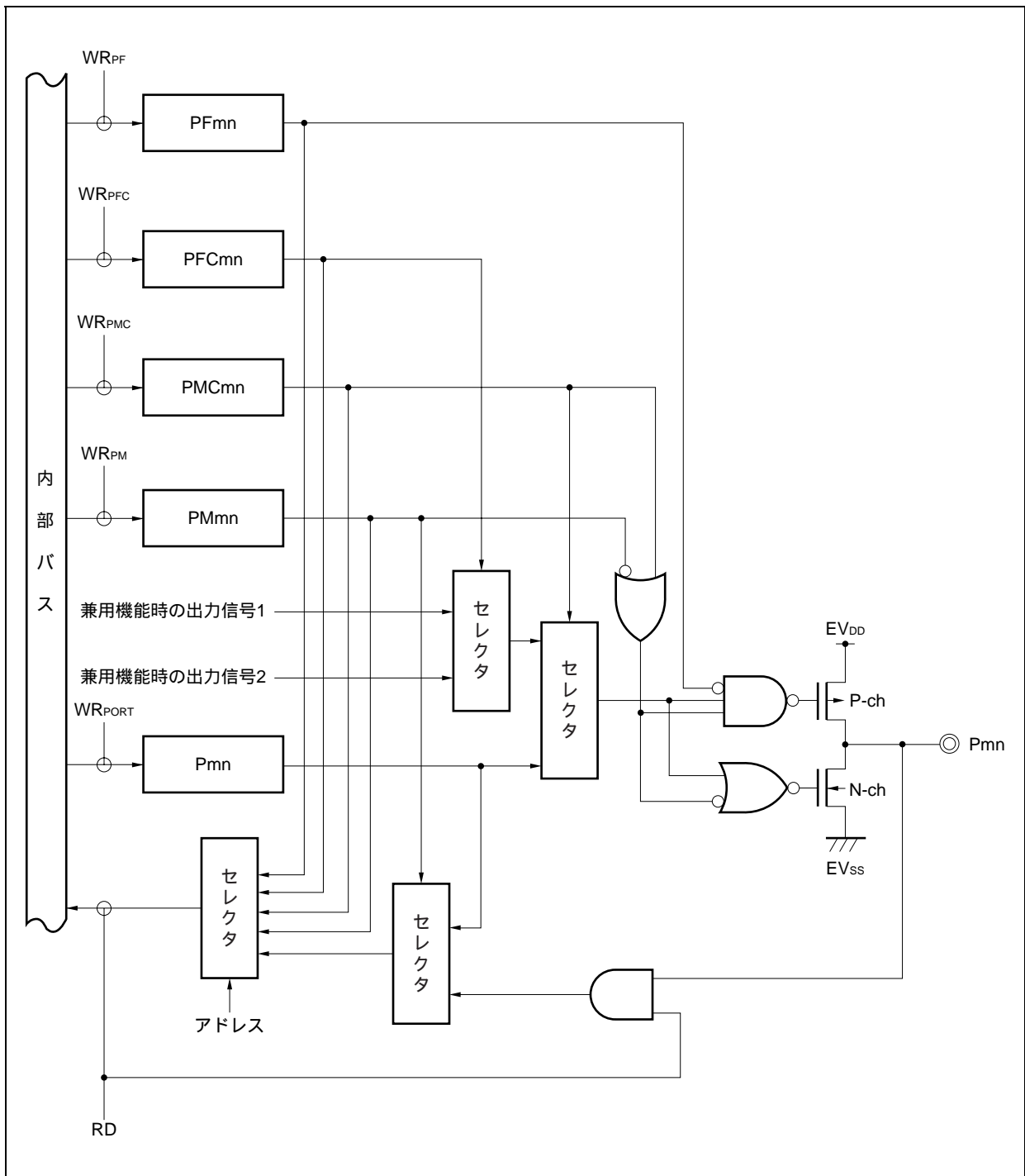
図4 - 15 タイプG - 3のブロック図
