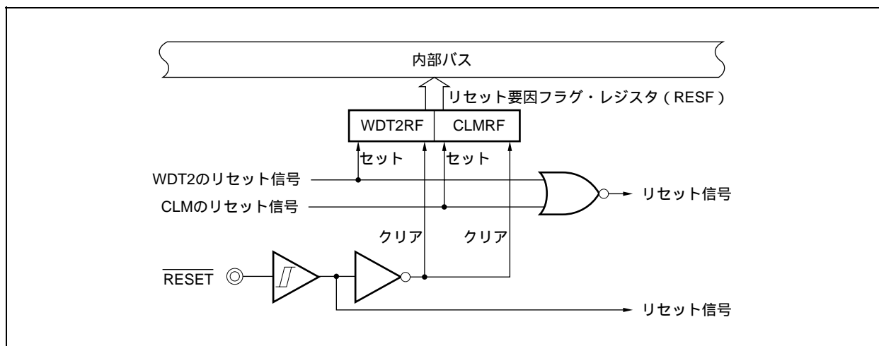
図25 - 1 リセット機能のブロック図
