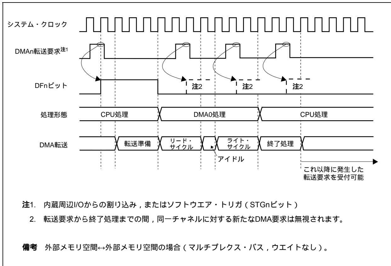
図20 - 3 DMAの転送要求が無視される期間 (1)
