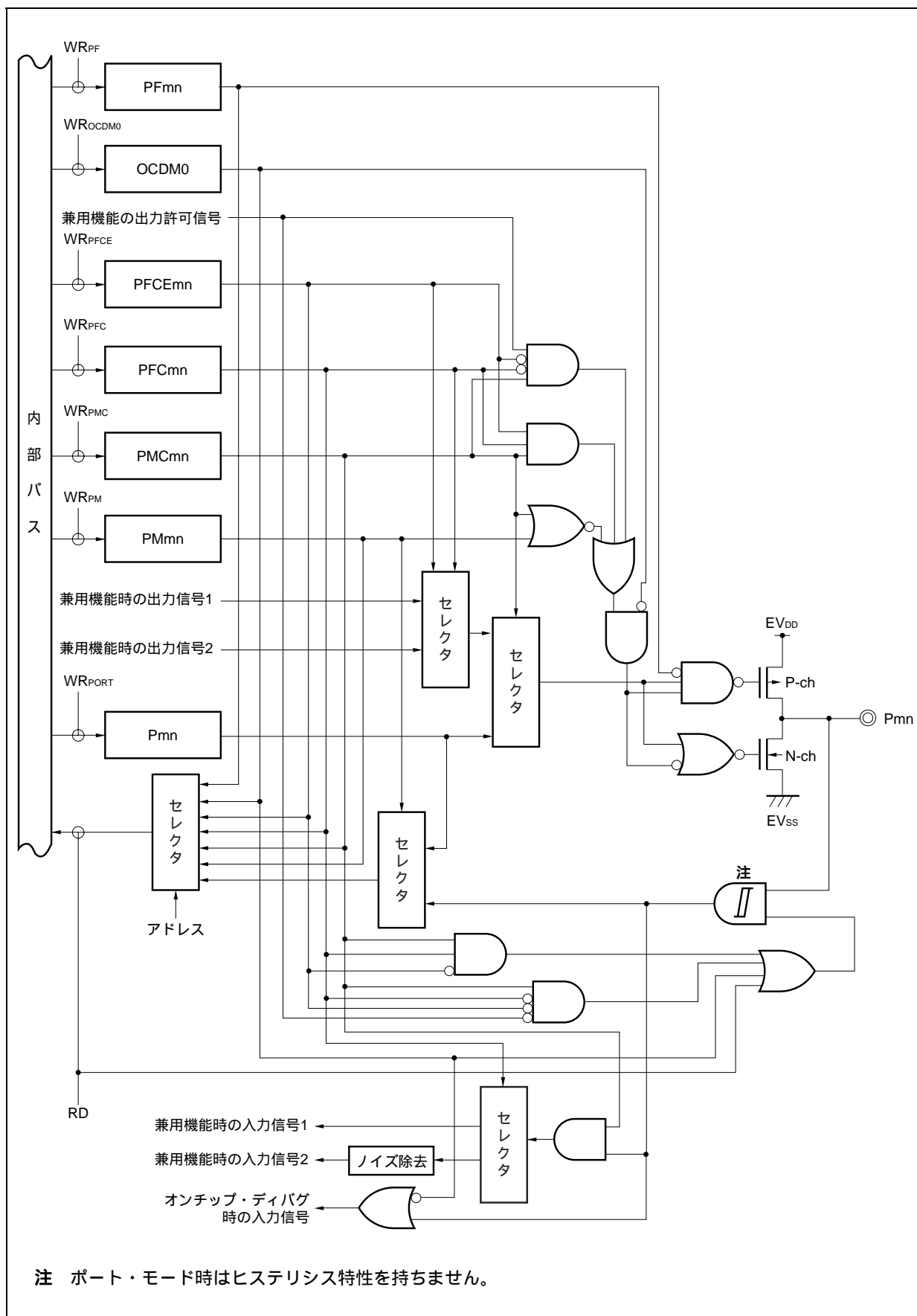
図4 - 33 タイプU - 9のブロック図
