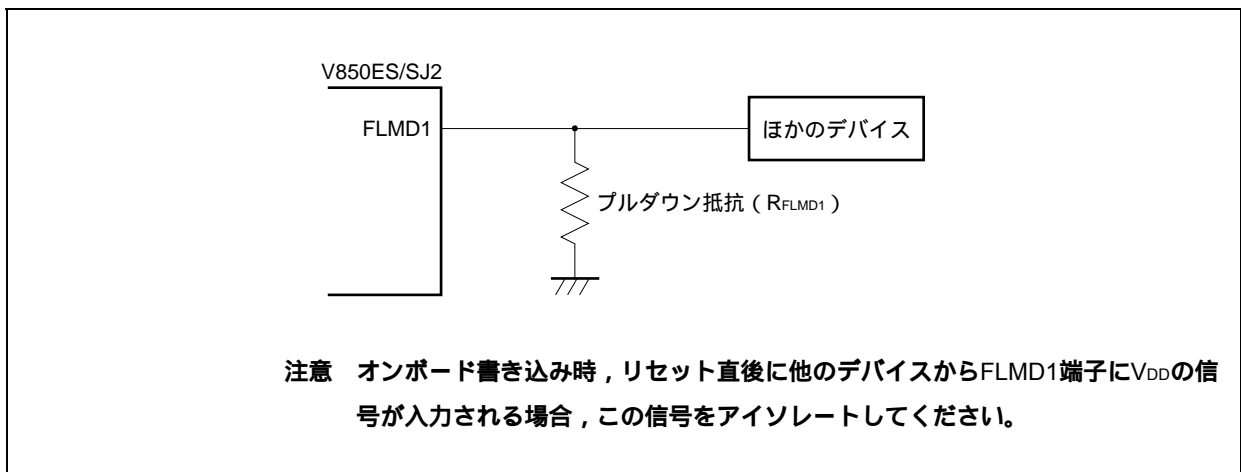
図29 - 11 FLMD1端子の接続例
