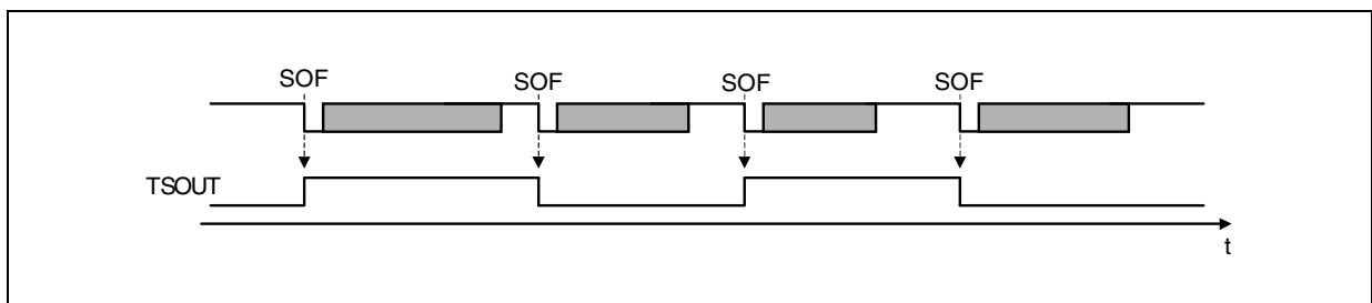
図19 - 34 キャプチャ用信号TSOUTのタイミング図
