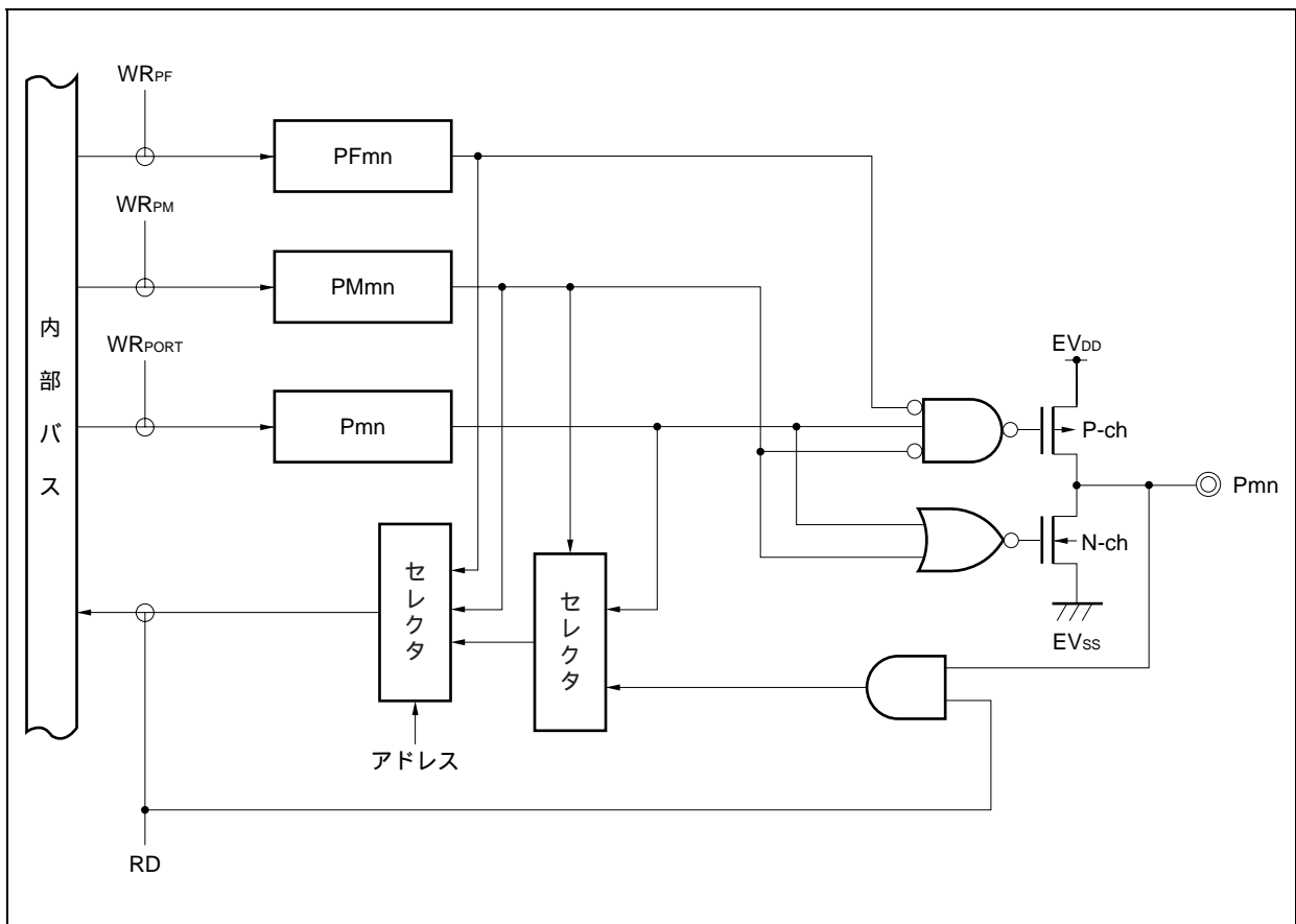
図4-6 タイプC-1のブロック図
