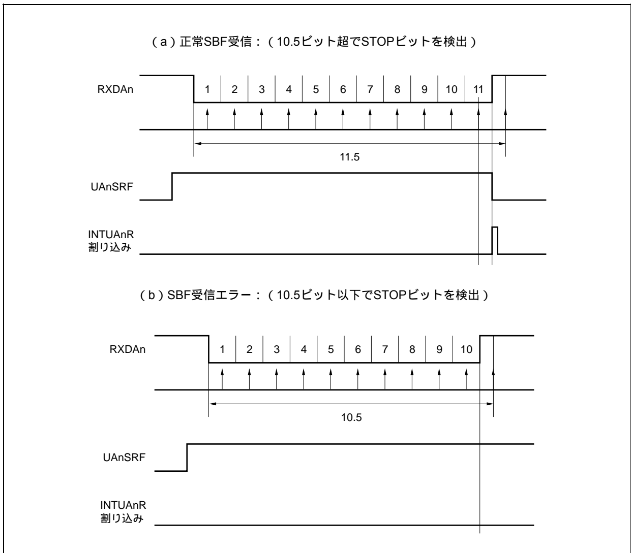
図15 - 9 SBF受信
