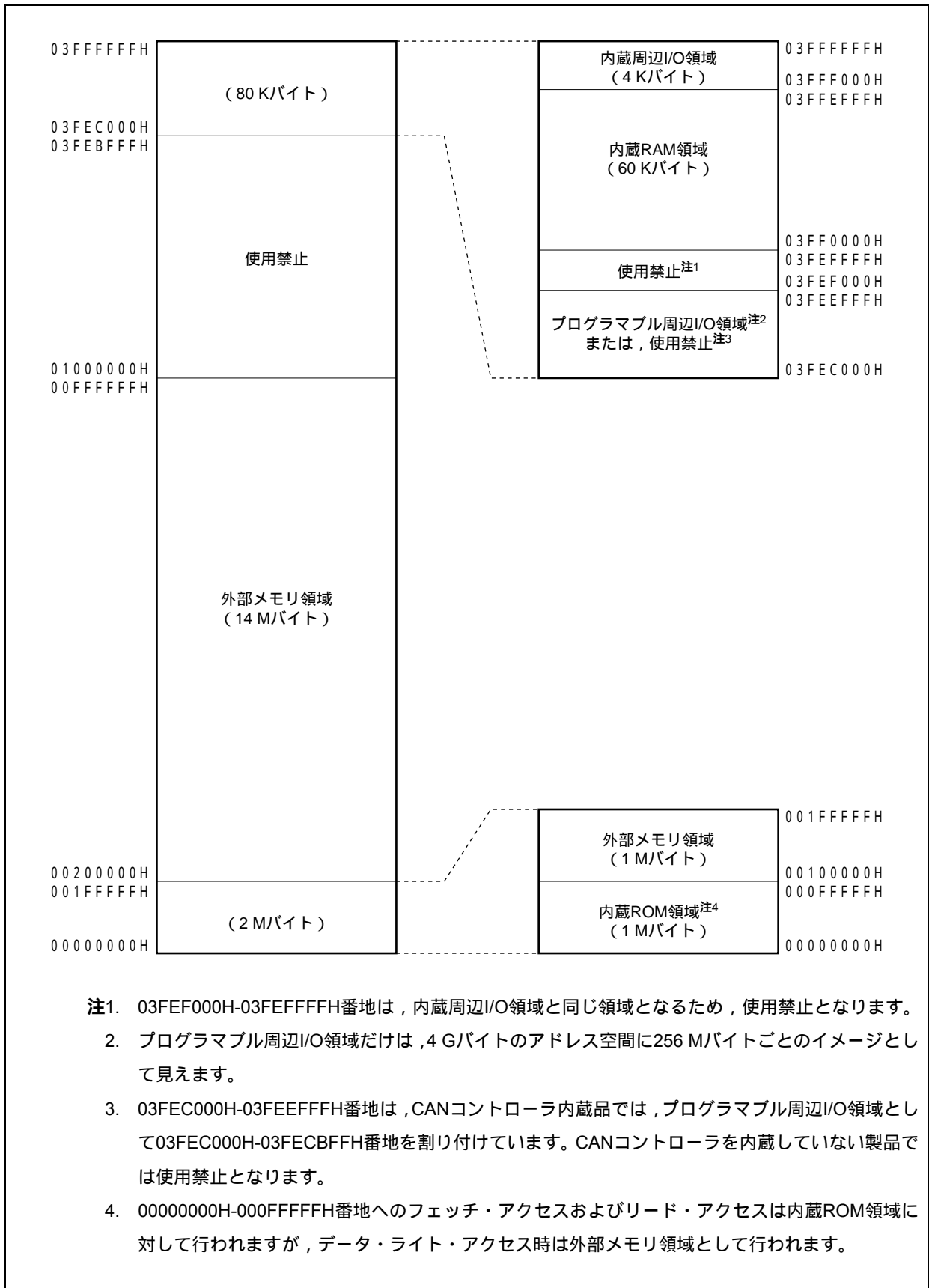
図3-2 データ・メモリ・マップ(物理アドレス)
