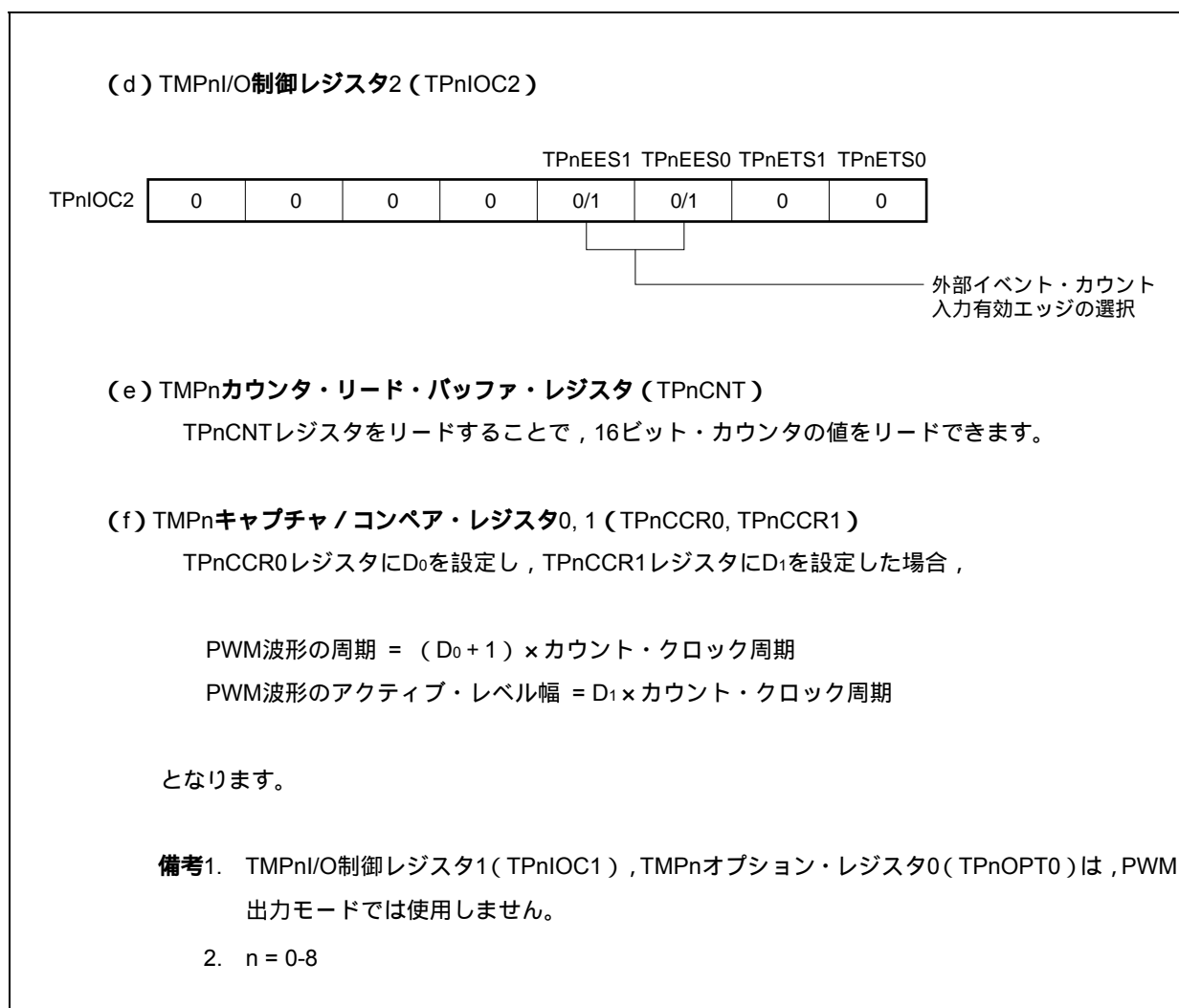
図7 - 26 PWM出力モード動作時のレジスタ設定内容 (2/2)
