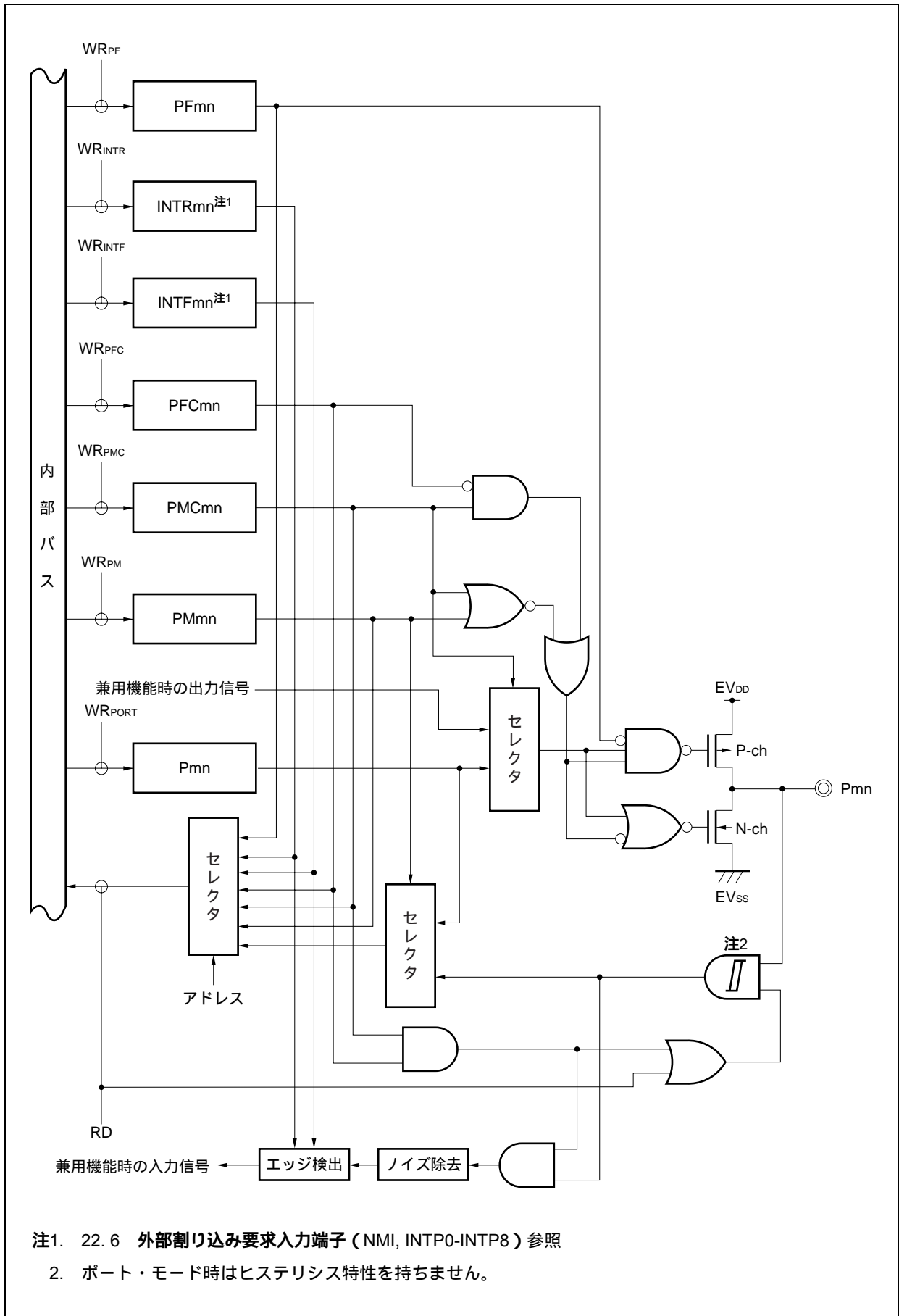
図4 - 23 タイプN - 2のブロック図
