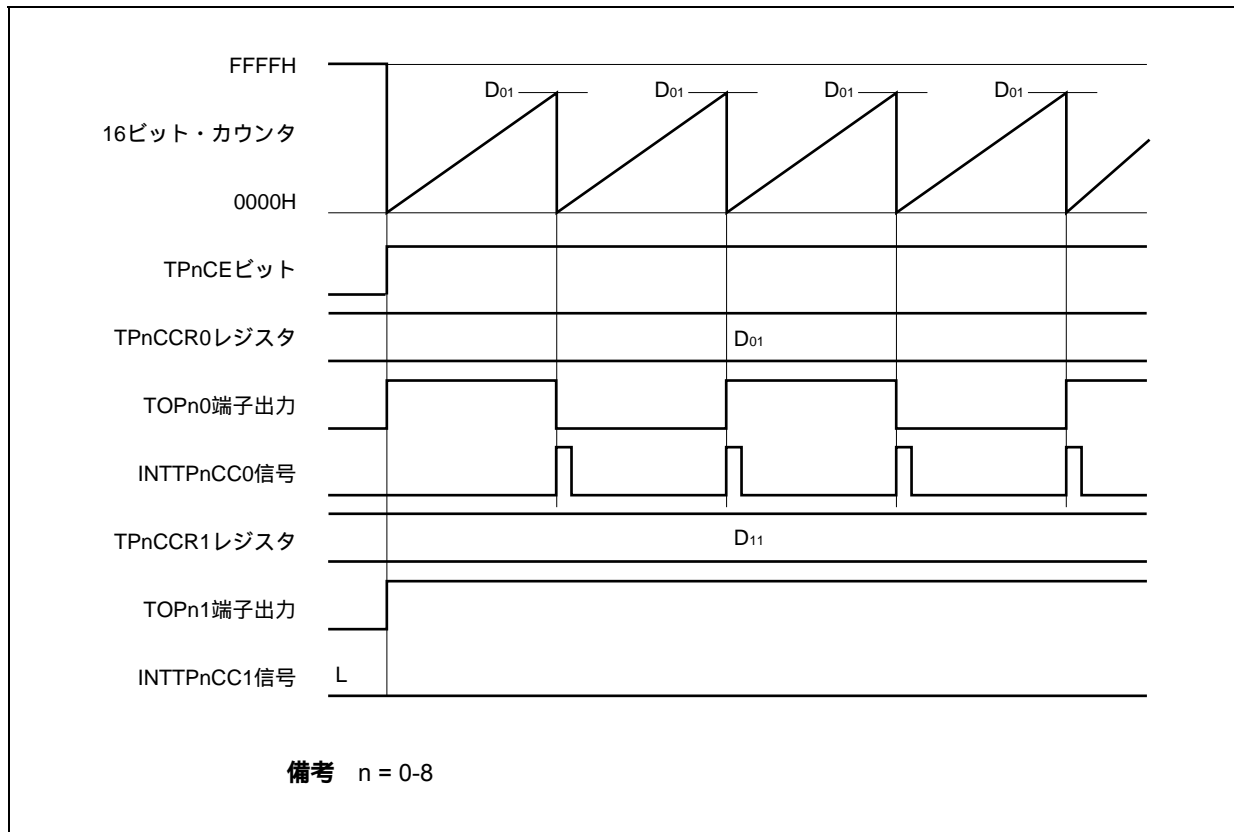
図7 - 8 D 01 < D 11 の場合のタイミング図
