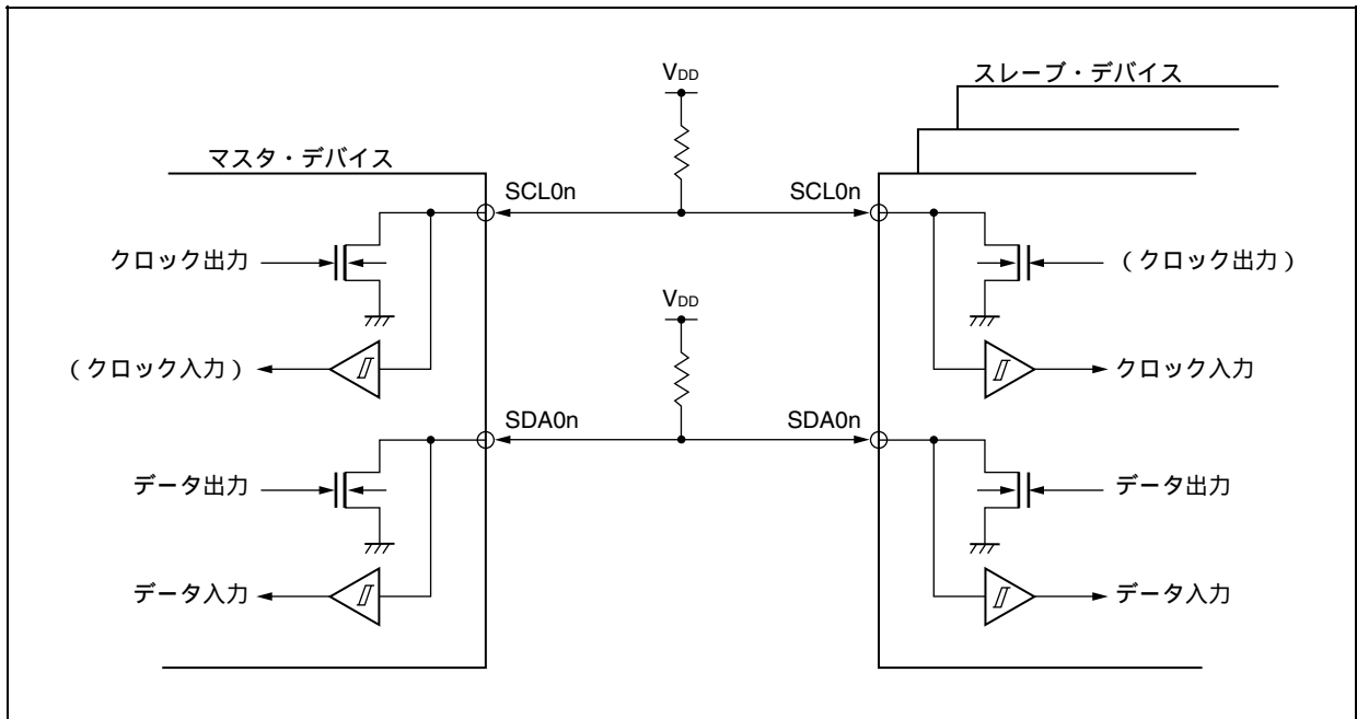
図17-6 端子構成図
