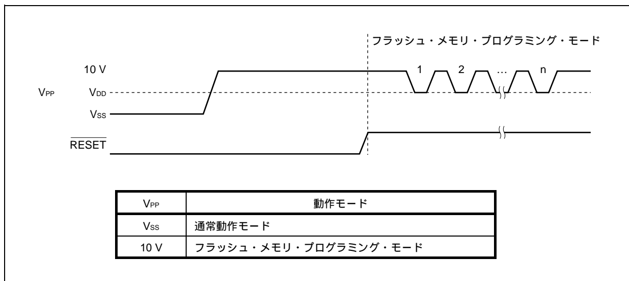
図26 - 11 フラッシュ・メモリ・プログラミング・モード
