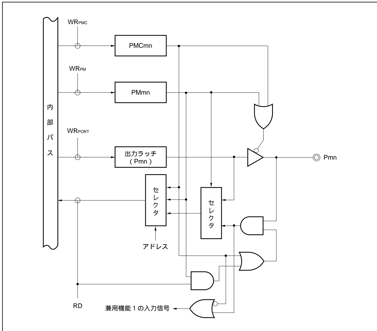
図4 - 3 タイプC-1のブロック図
