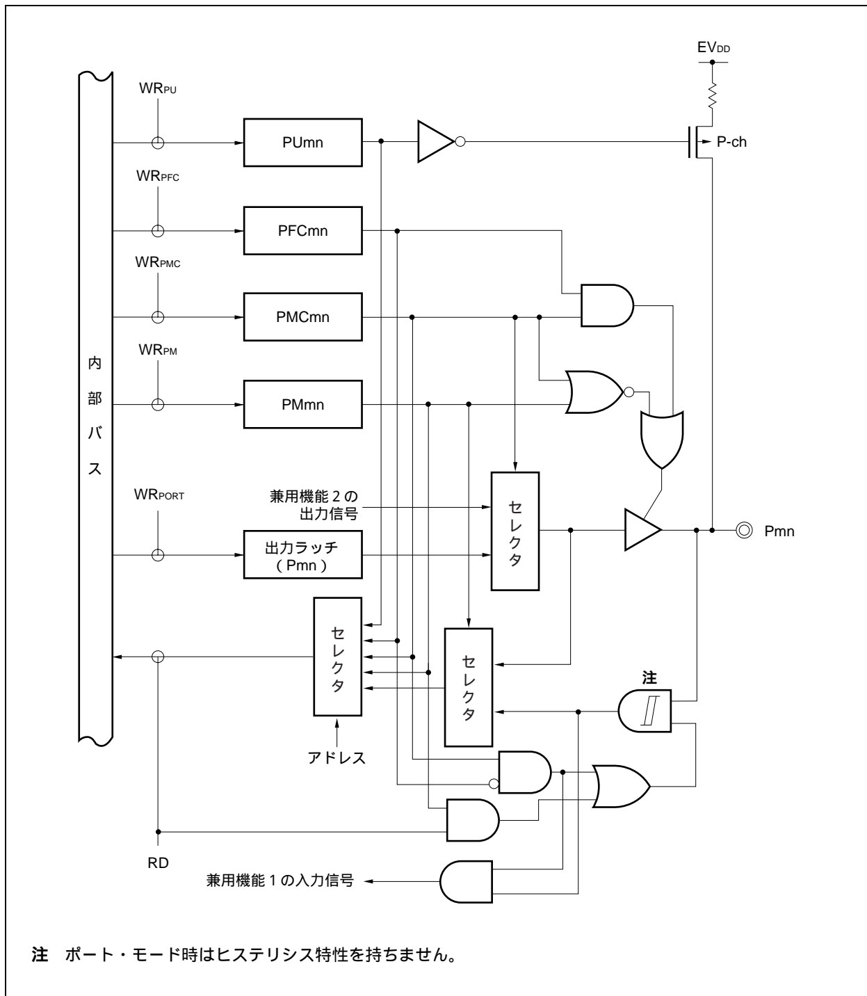
図4 - 12 タイプE-6のブロック図
