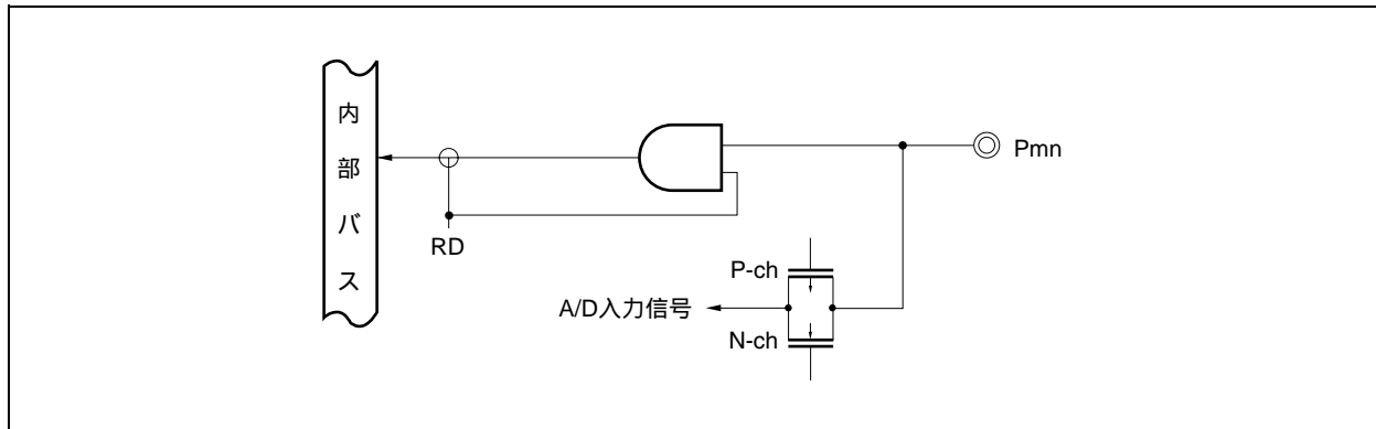
図4 - 3 タイプC-1のブロック図
