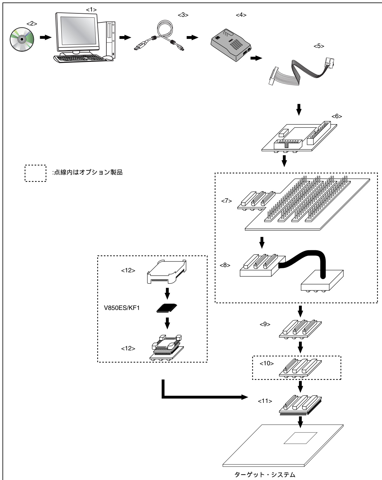
図A - 3 QB-V850ESKX1-DAを使用したシステム構成（オプション製品を使用する場合）
