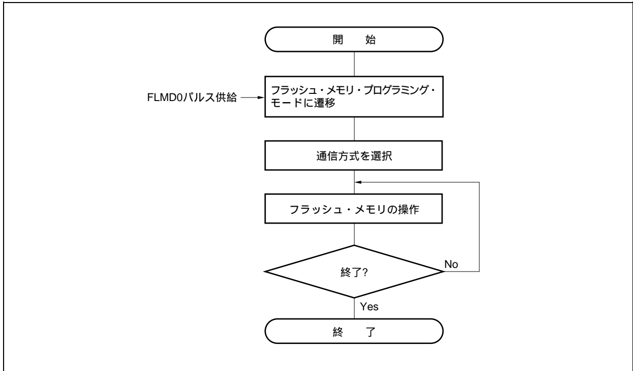
図25 - 7 フラッシュ・メモリの操作手順
