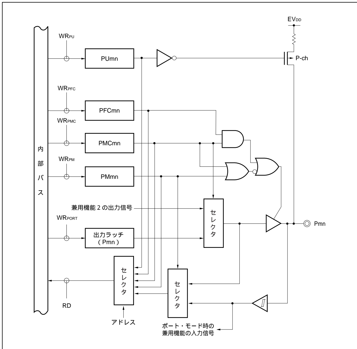
図4 - 15 タイプE-9のブロック図
