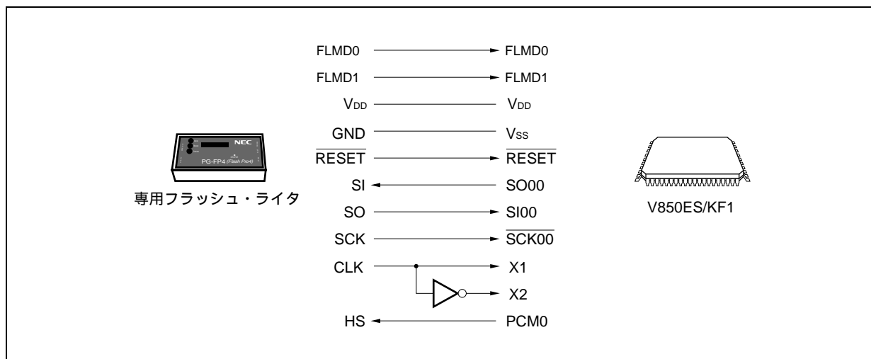
図25 - 5 専用フラッシュ・ライタとの通信 (CSI00 + HS)
