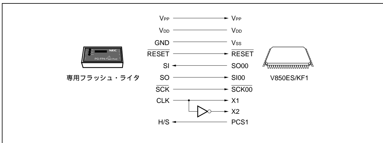
図26 - 5 専用フラッシュ・ライタとの通信 (CSI00 + H/S)
