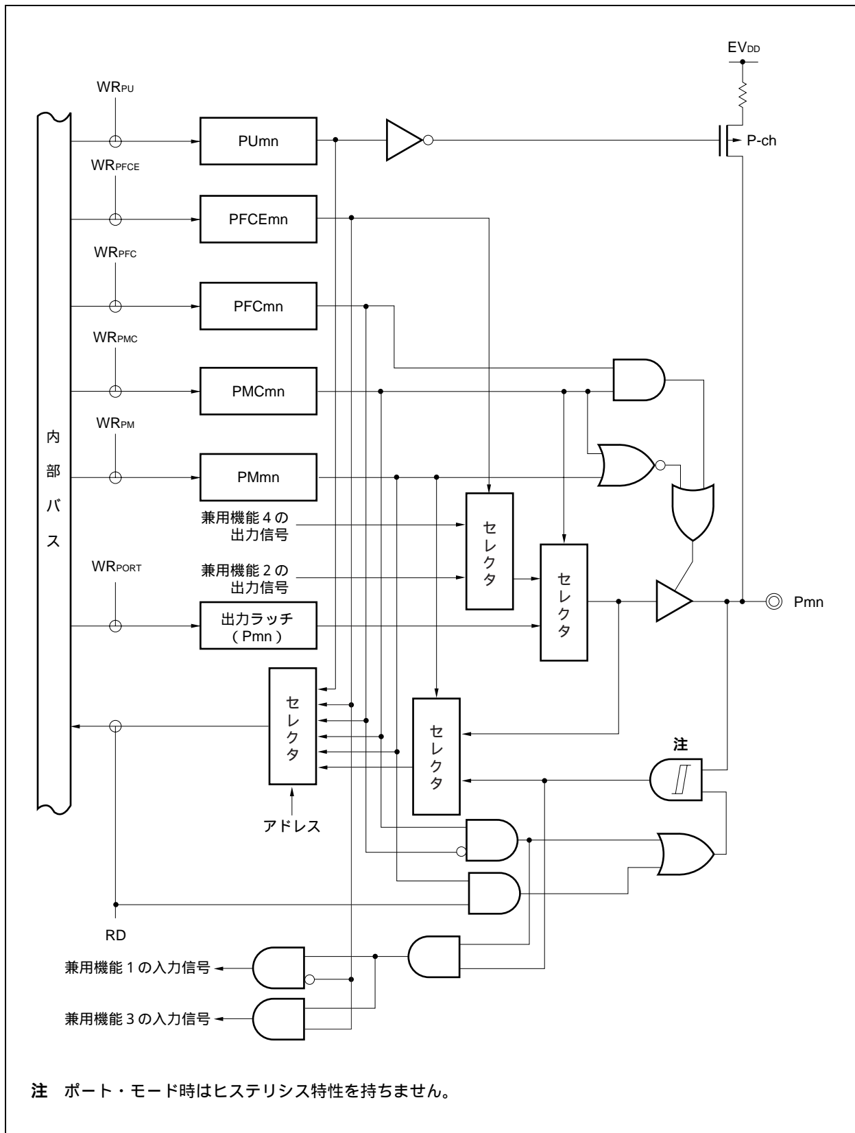
図4 - 20 タイプG-7-1のブロック図
