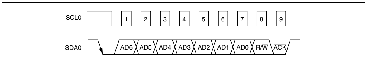
図18-8 アクノリッジ ( \overline{\text{ACK}} )
