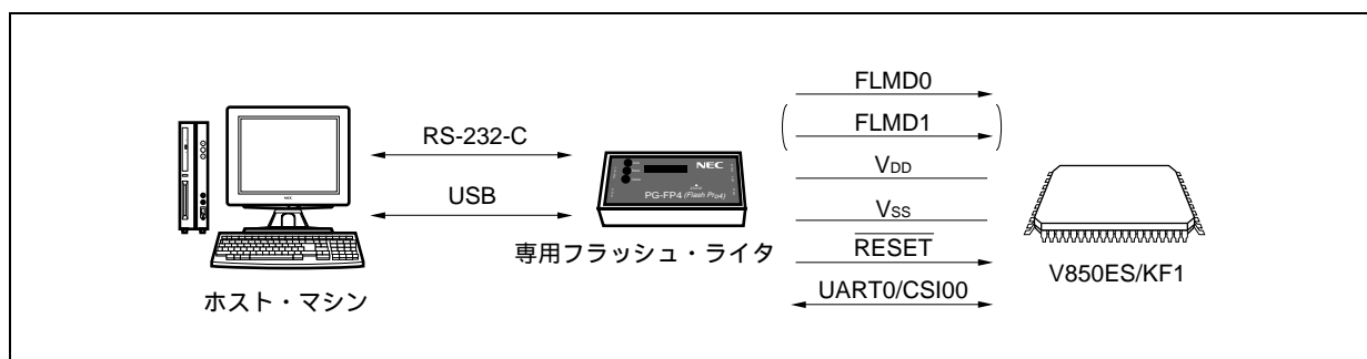
図25 - 2 フラッシュ・メモリにプログラムを書き込むための環境
