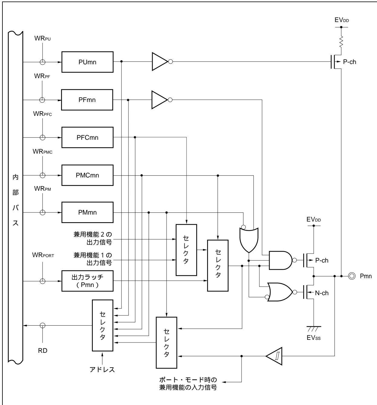
図4 - 18 タイプG-1のブロック図
