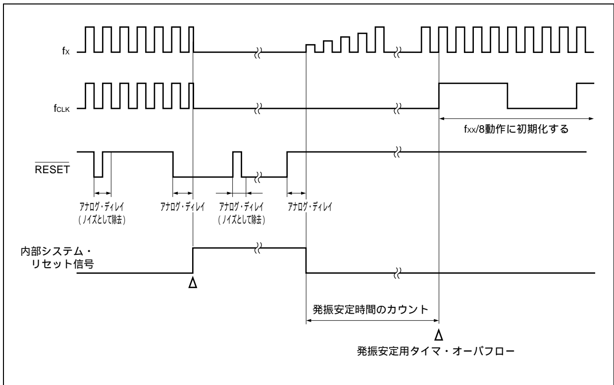
図22 - 3 パワーオン時の動作
