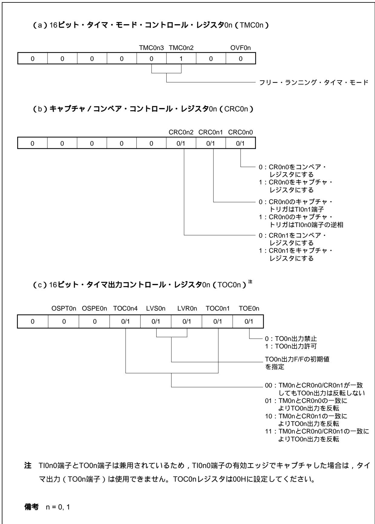
図8 - 29 フリー・ランニング・タイマ・モード動作時のレジスタ設定内容例 (1/2)
