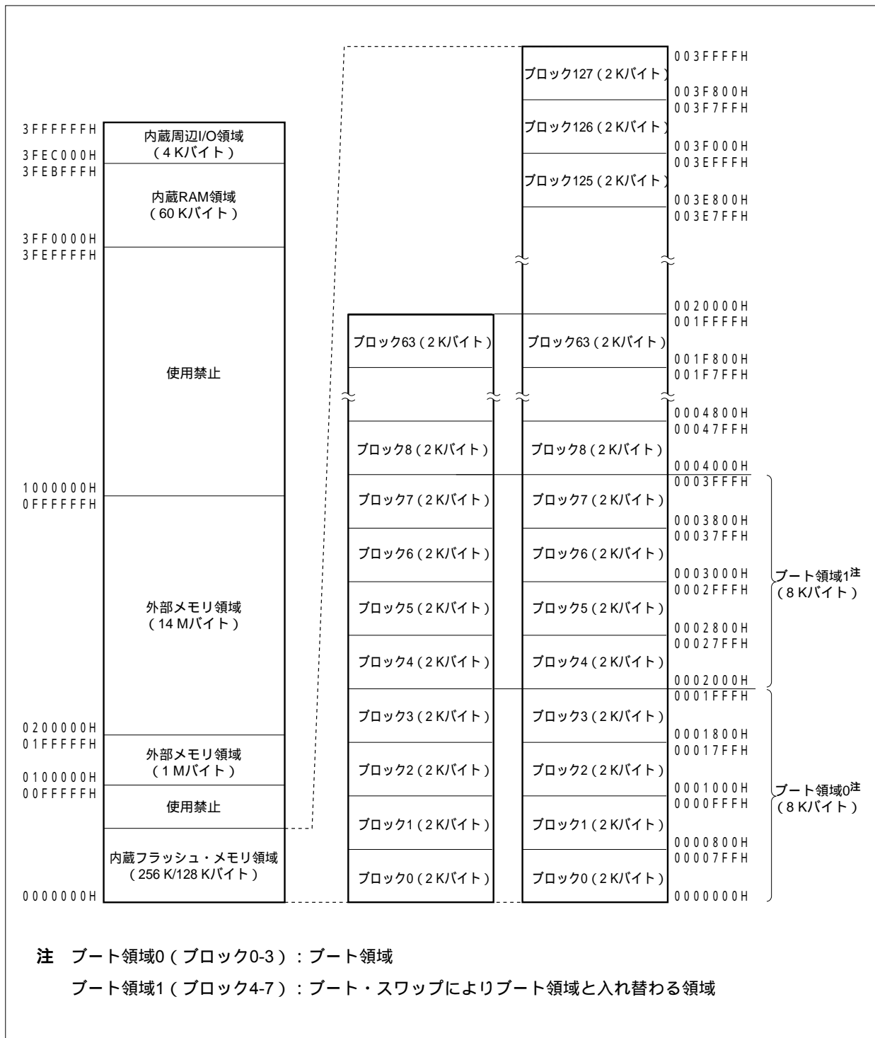
図25 - 1 フラッシュ・メモリ・マッピング
