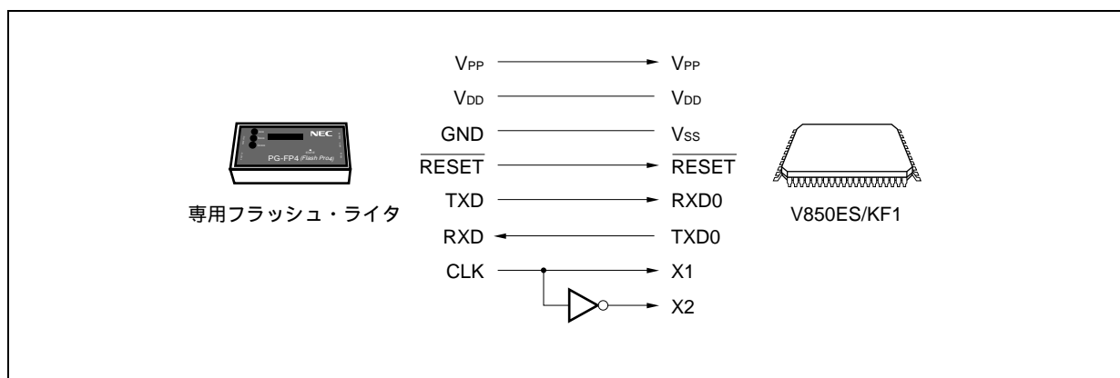
図26 - 3 専用フラッシュ・ライターとの通信（UART0）
