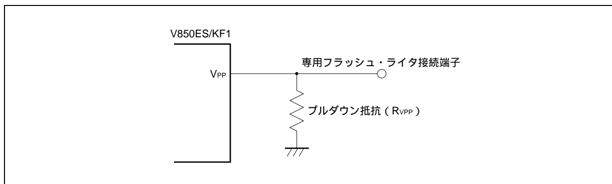
図26 - 6 V PP 端子の接続例
