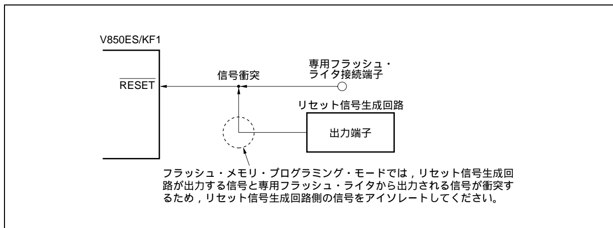
図26 - 9 信号の衝突（ \overline{\text{RESET}} 端子）
