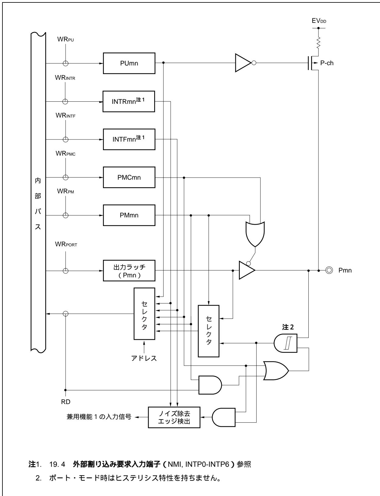
図4-24 タイプH-1のブロック図
