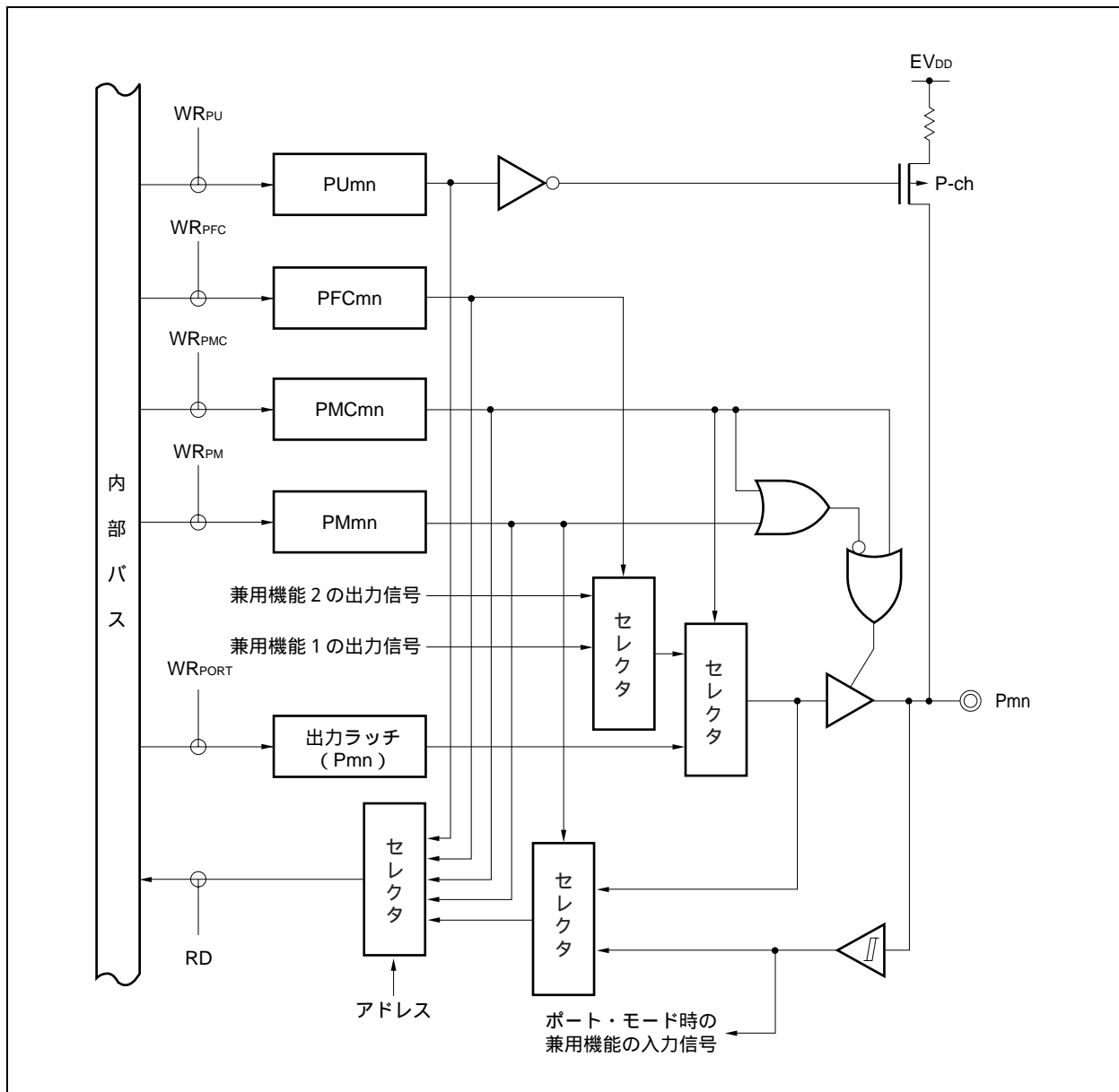
図4 - 10 タイプE-4のブロック図
