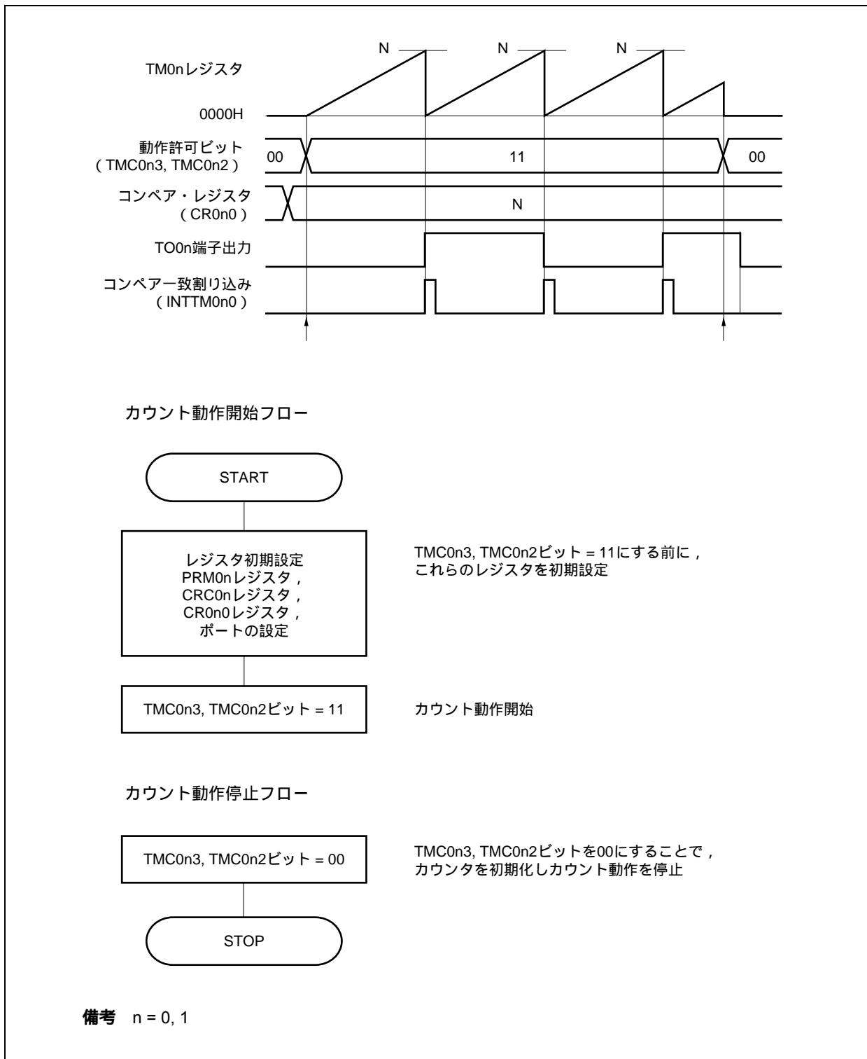
図8 - 12 外部イベント・カウンタ・モード動作時のソフトウェア処理例
