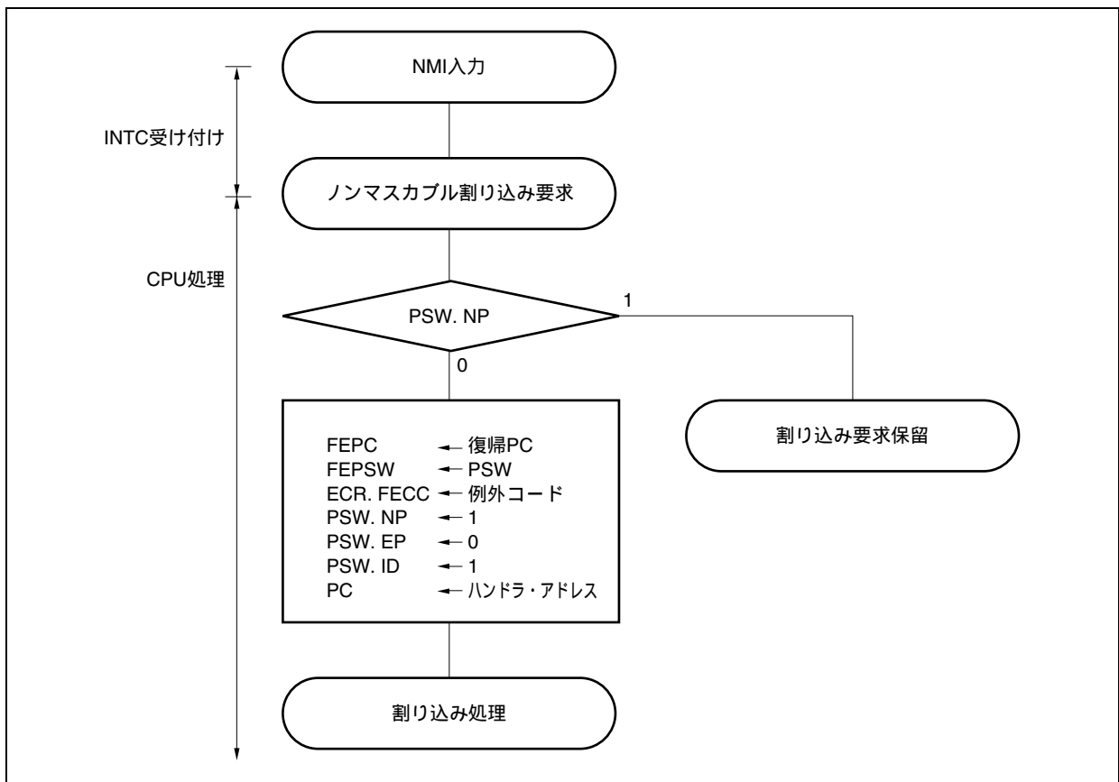
図19-2 ノンマスクブル割り込みの処理形態
