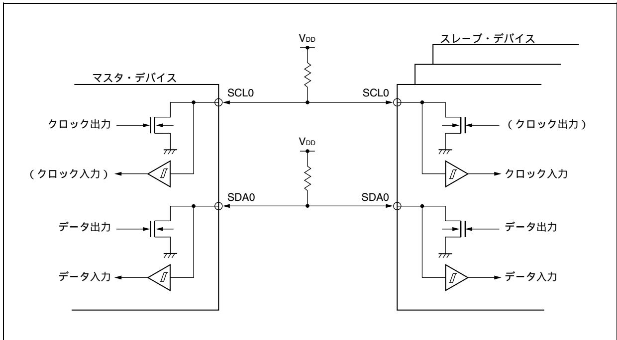
図18-3 端子構成図
