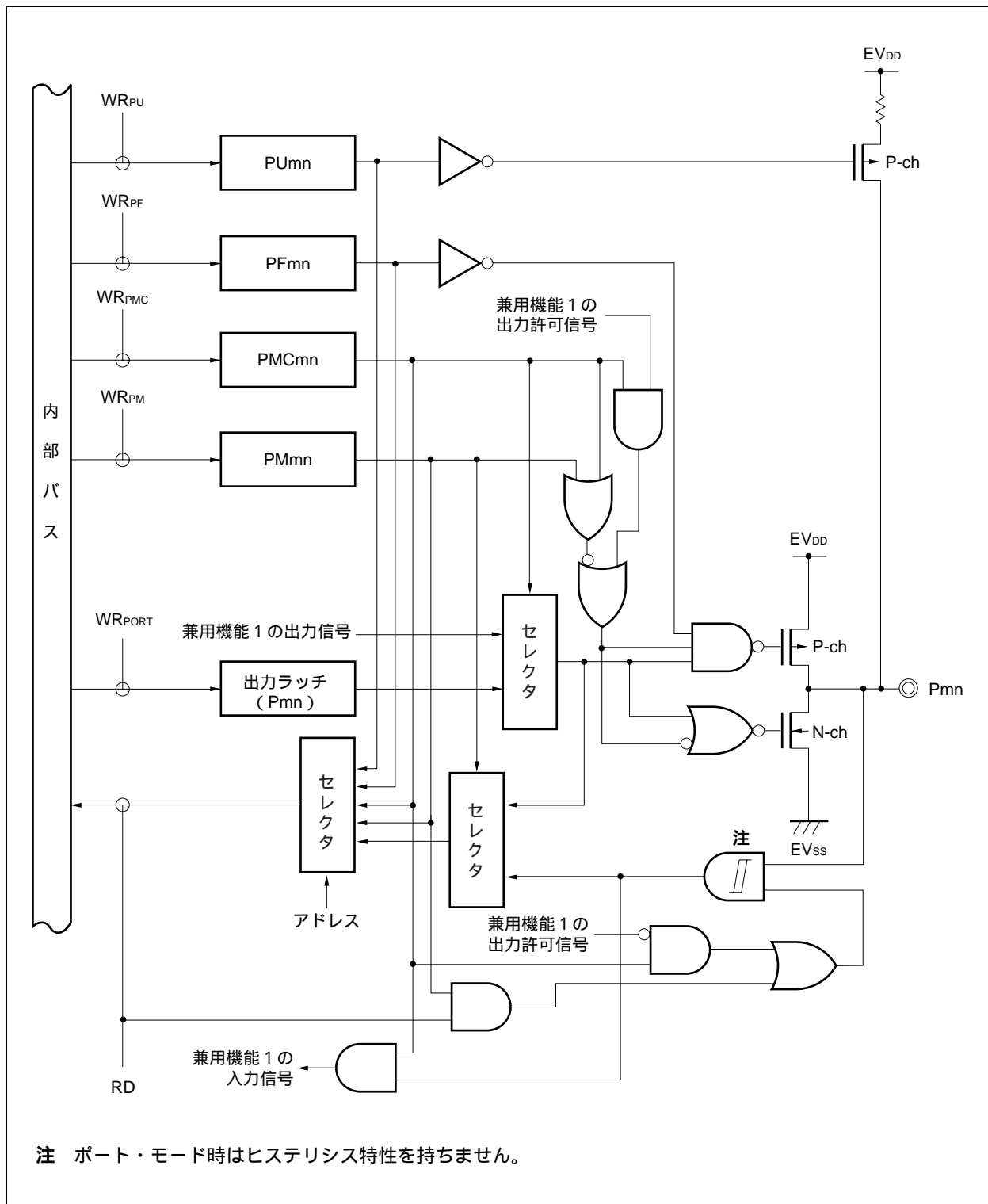
図4 - 17 タイプF-2のブロック図
