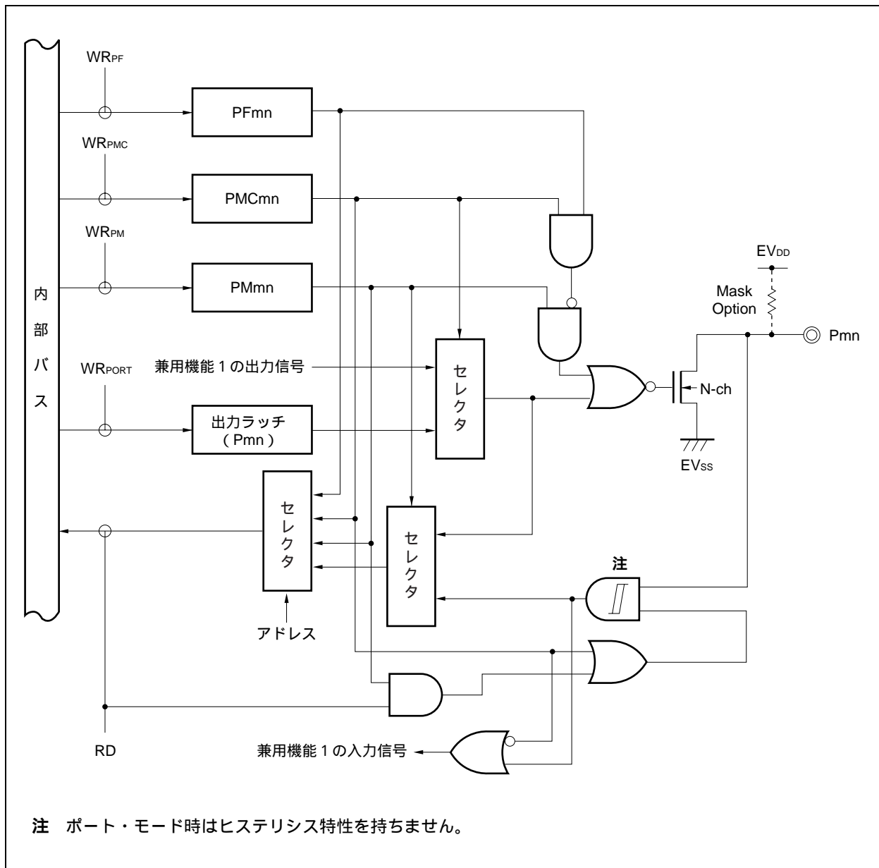
図4 - 26 タイプKのブロック図
