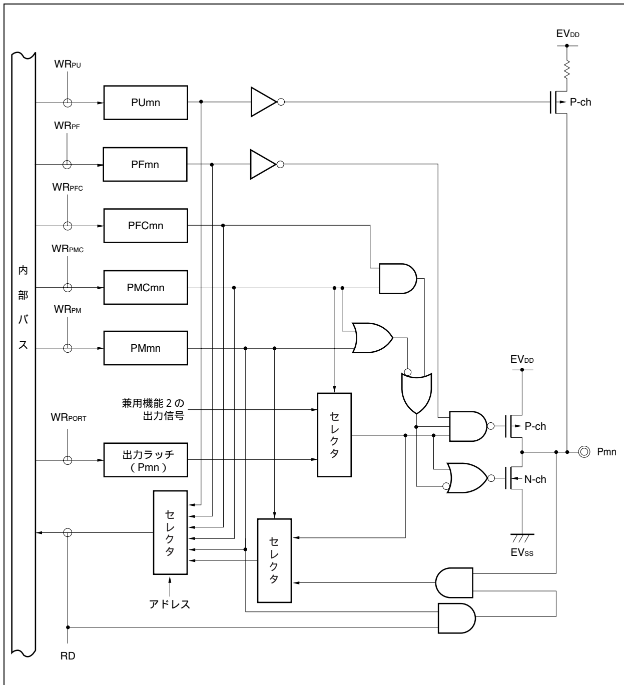
図4 - 23 タイプG-9のブロック図
