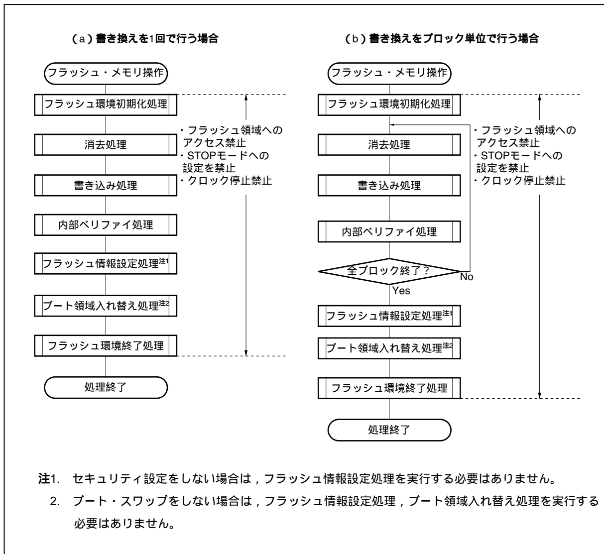
図25 - 17 標準セルフ・プログラミング・フロー
