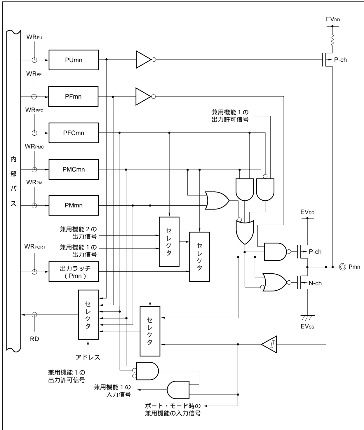
図4-19 タイプG-2のブロック図
