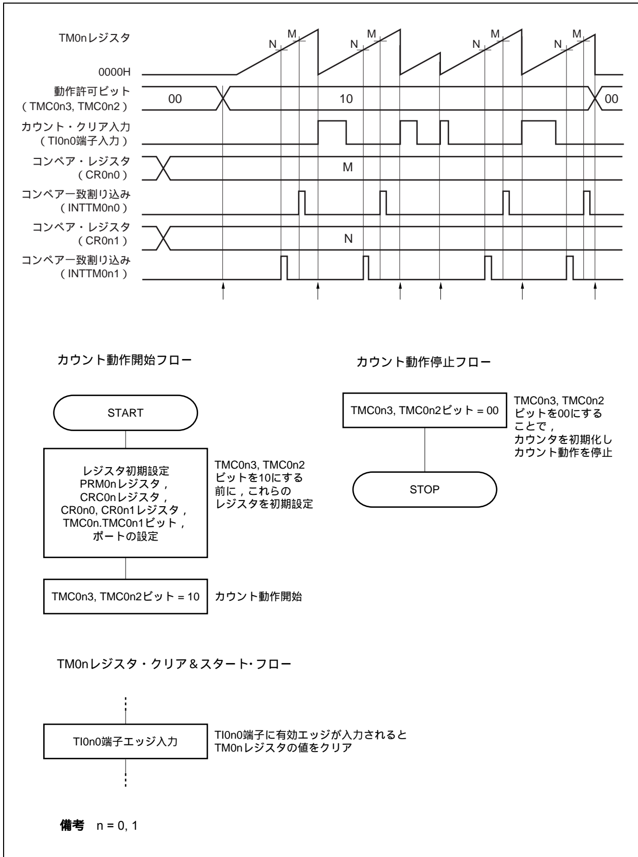
図8-22 T10n0端子の有効エッジ入力によるクリア&スタート・モード動作時のソフトウェア処理例
