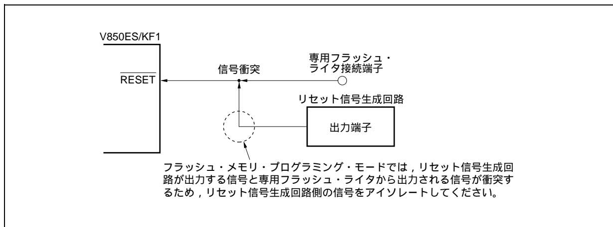
図25 - 14 信号の衝突（RESET端子）
