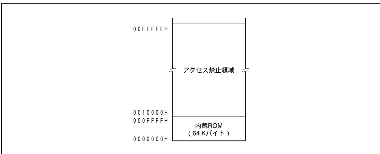
図3 - 7 内蔵ROM (64 Kバイト)
