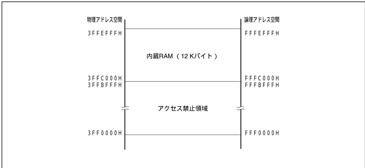
図3 - 8 内蔵RAM (12 Kバイト)
