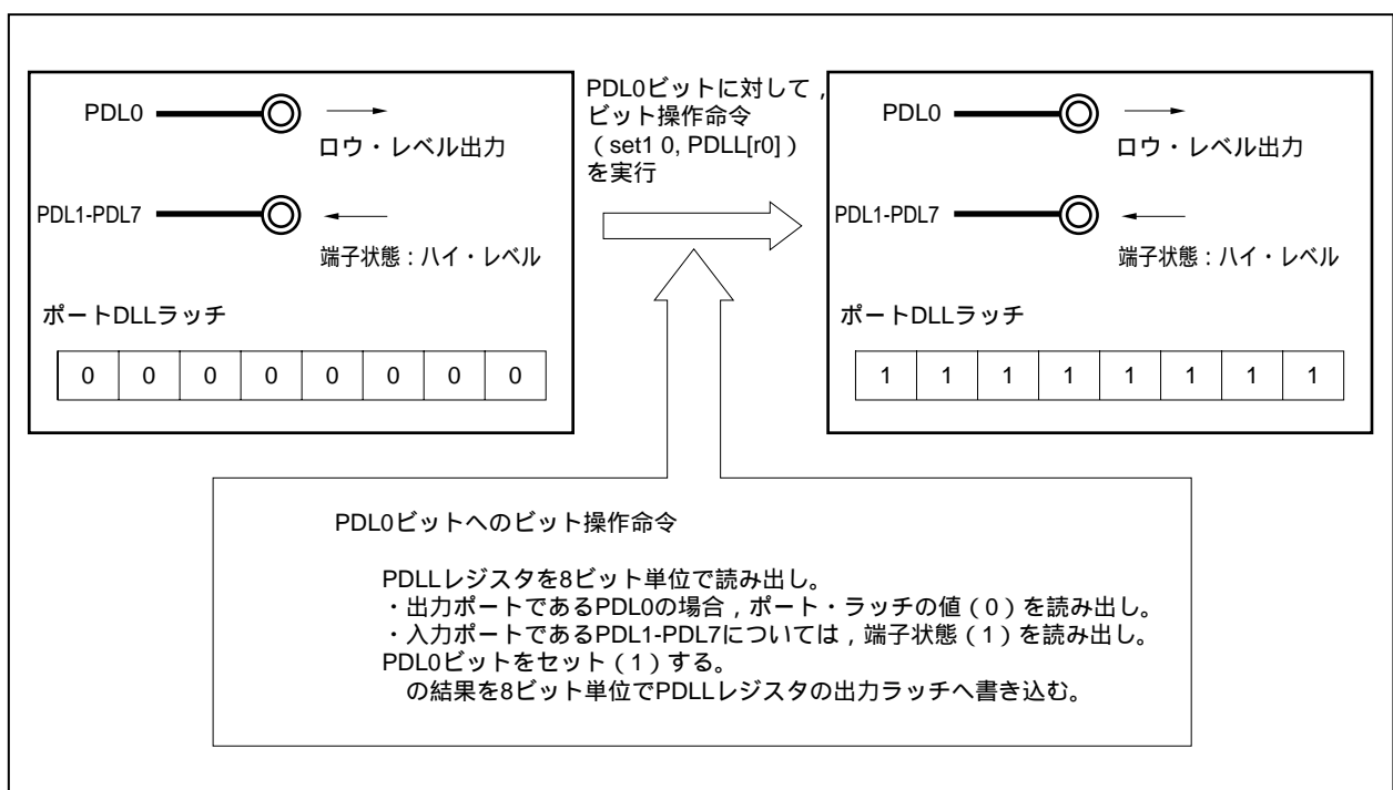
図4 - 27 ビット操作命令 (PDL0の場合)
