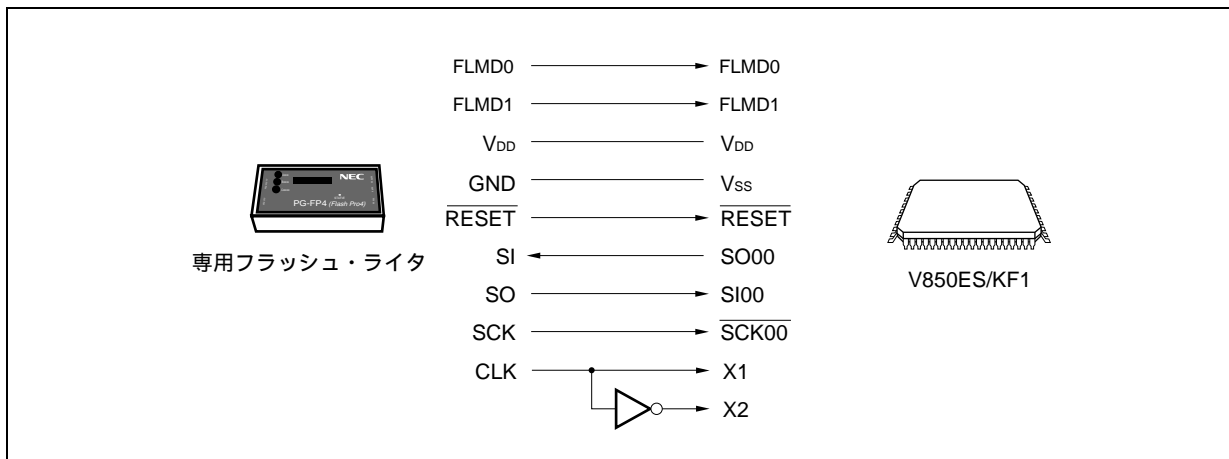
図25 - 4 専用フラッシュ・ライタとの通信 (CSI00)
