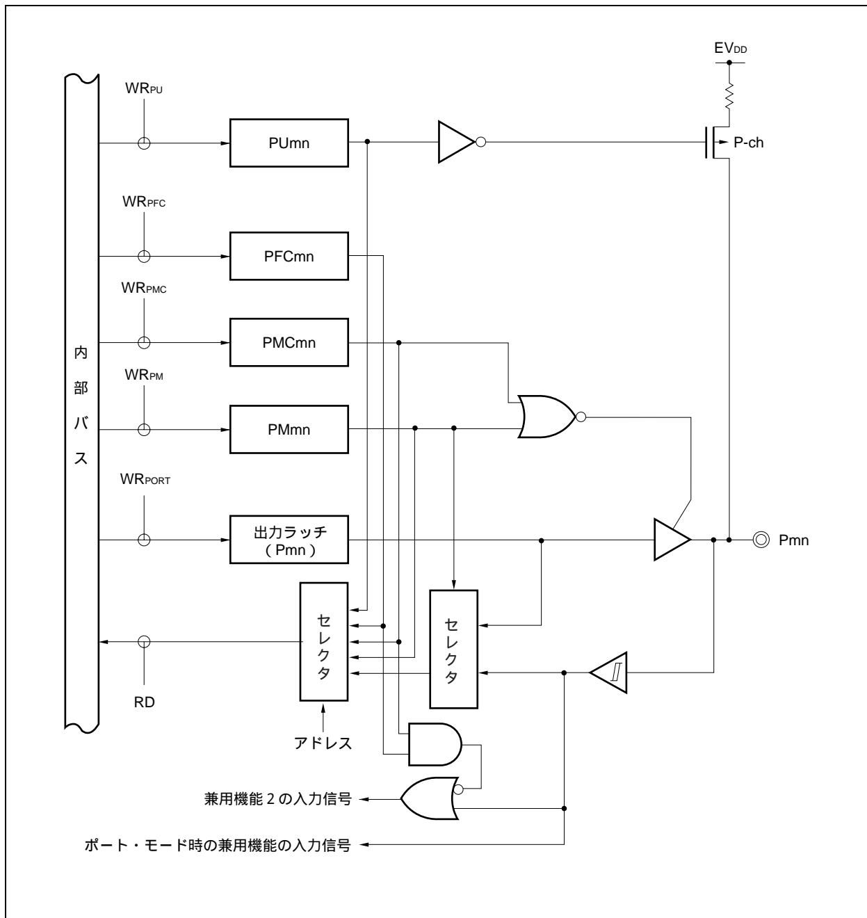
図4 - 13 タイプE-7のブロック図
