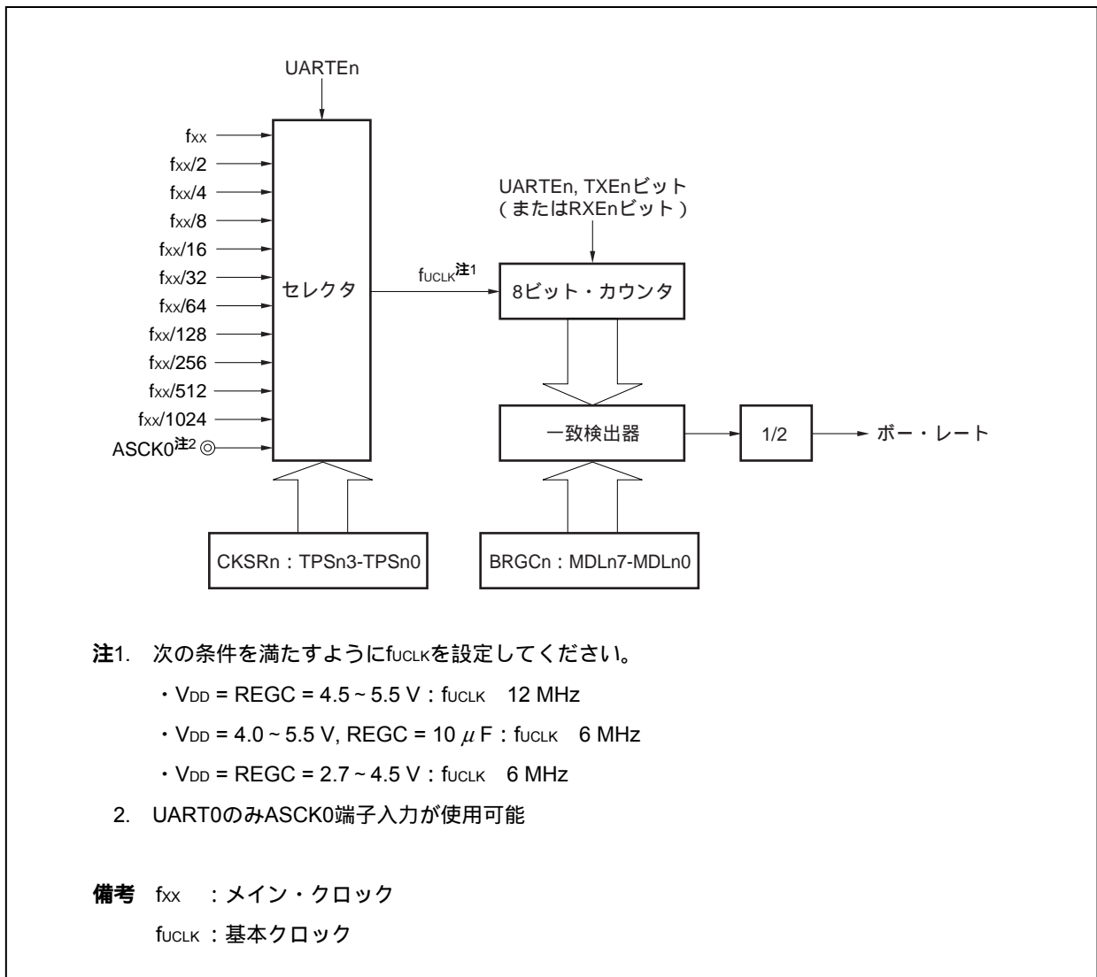
図15-12 ポー・レート・ジェネレータ n (BRG n ) の構成
