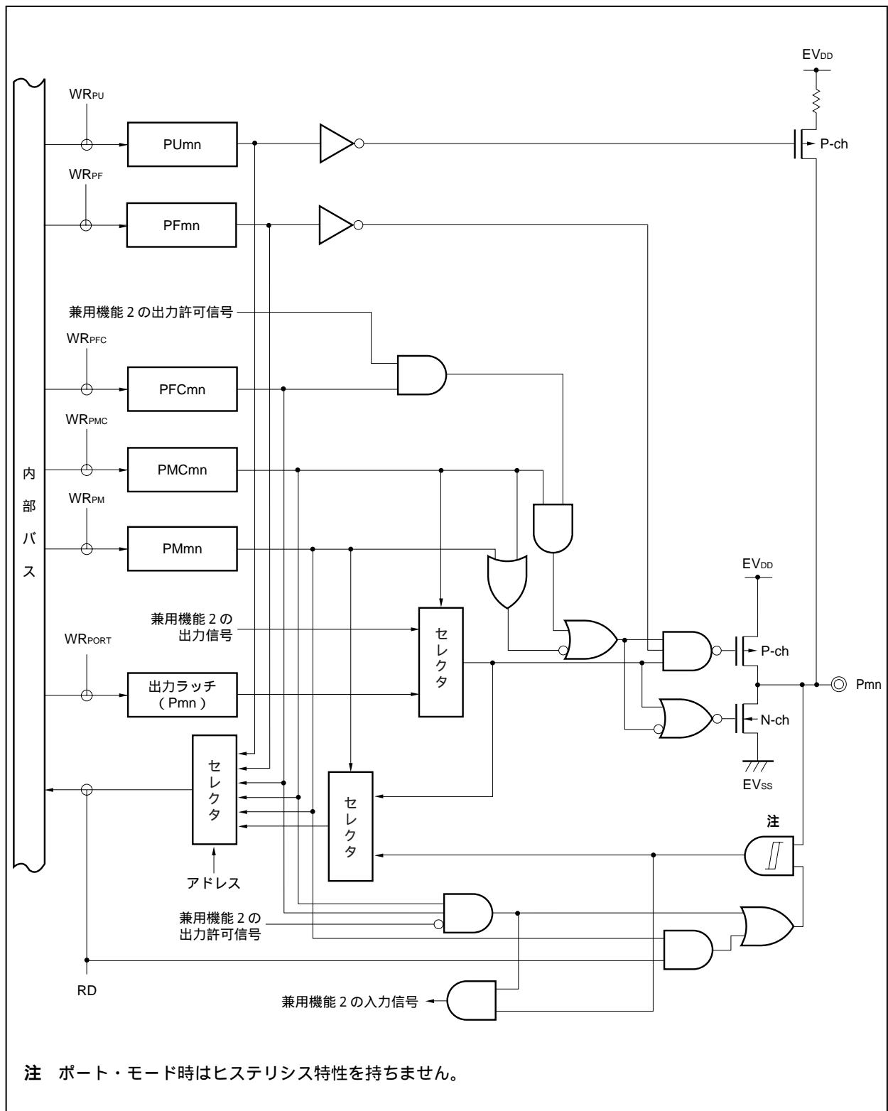
図4-22 タイプG-8のブロック図
