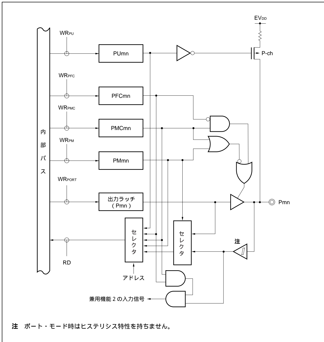
図4 - 14 タイプE-8のブロック図
