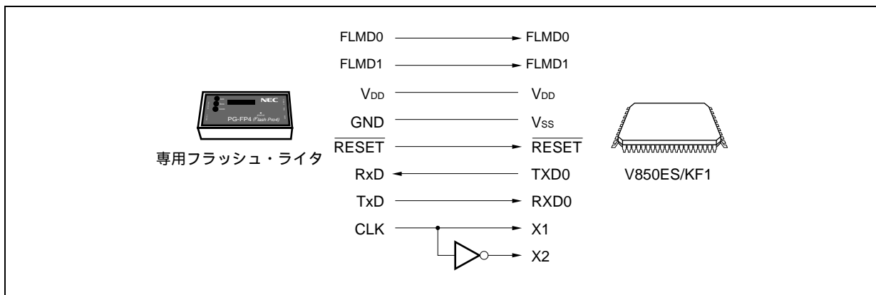
図25 - 3 専用フラッシュ・ライタとの通信 (UART0)
