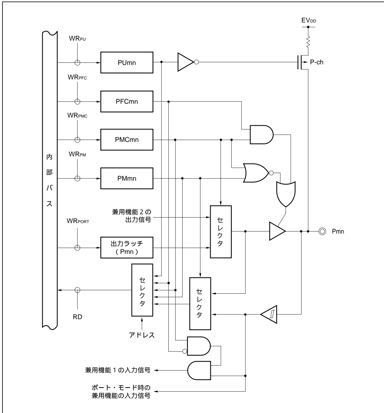
図4 - 11 タイプE-5のブロック図
