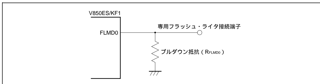
図25 - 10 FLMD0端子の接続例
