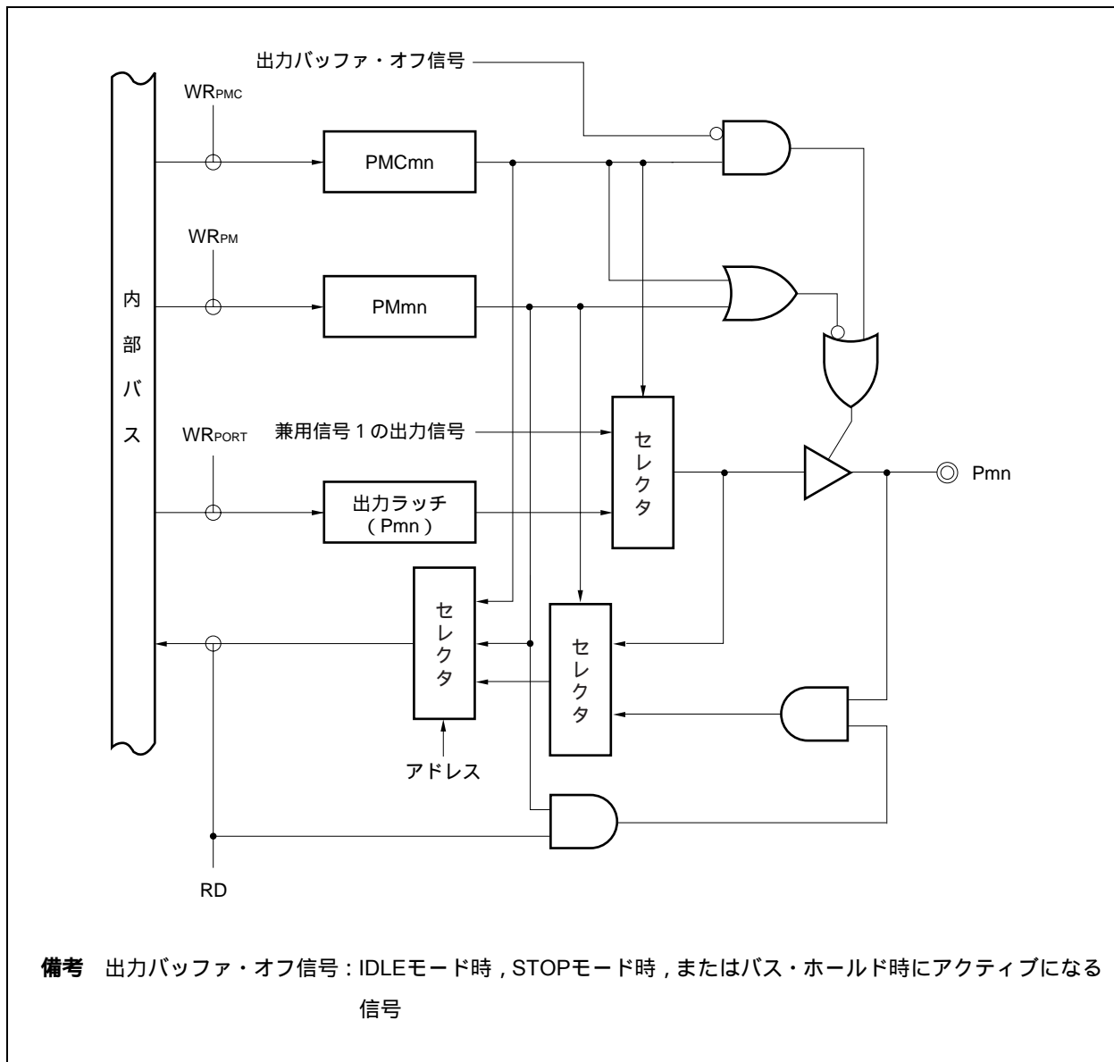
図4 - 5 タイプC-3のブロック図
