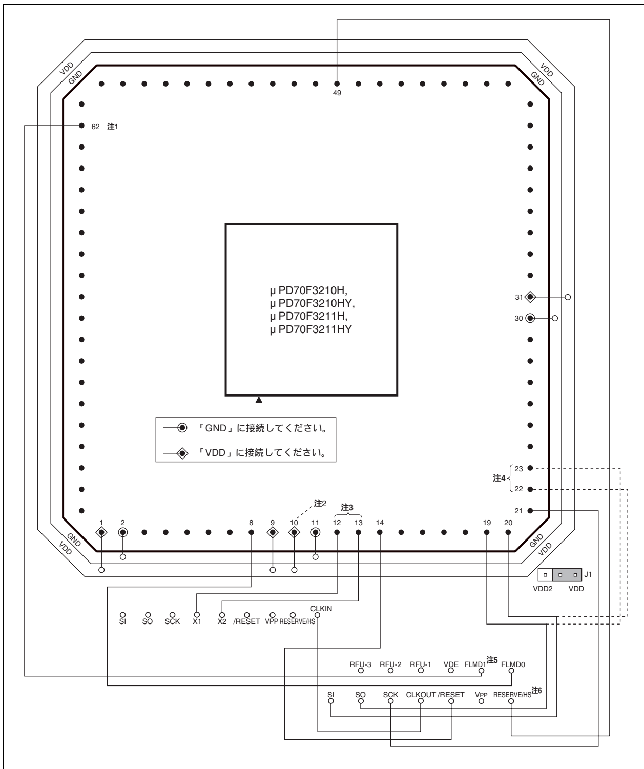
図25 - 6 V850ES/KF1フラッシュ書き込み用アダプタ (FA-80GC-8BT-A, FA-80GK-9EU-A) の配線例 (1/2)
