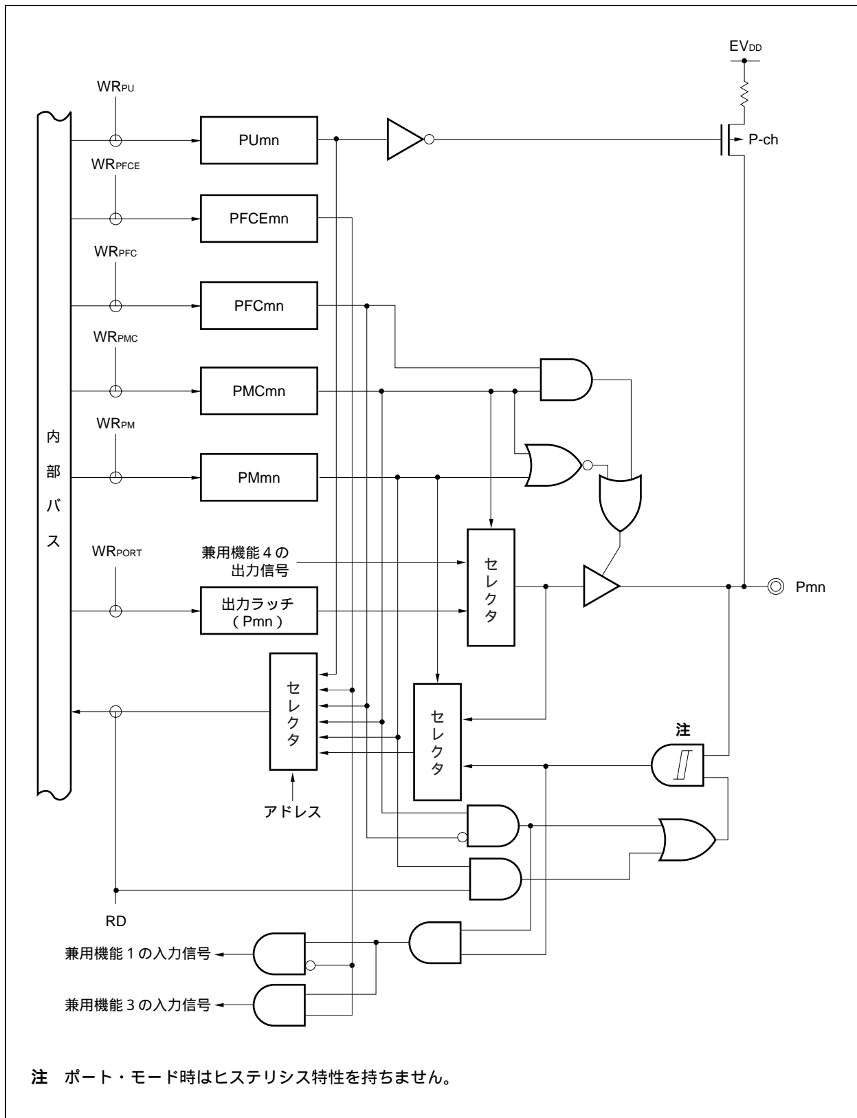
図4 - 21 タイプG-7-2のブロック図
