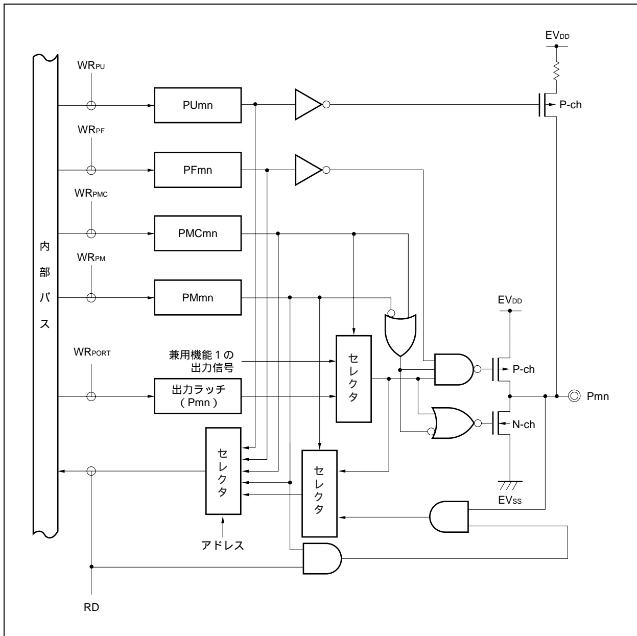
図4 - 16 タイプF-1のブロック図
