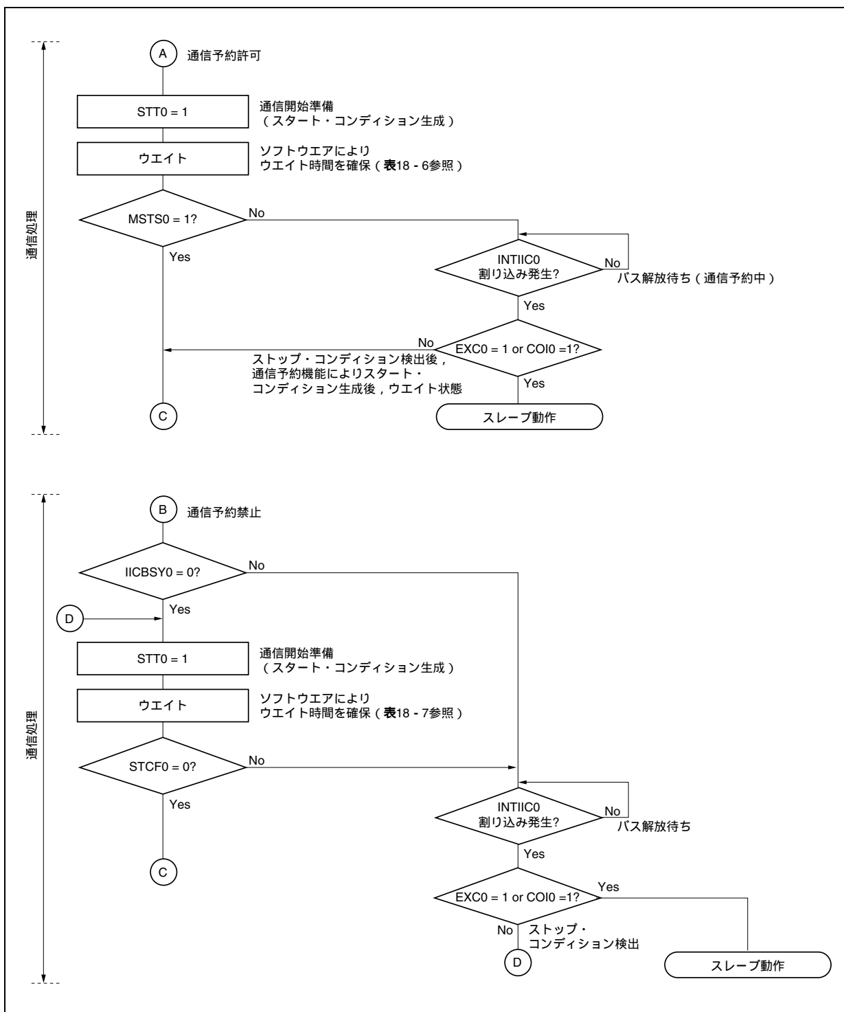
図18 - 16 マルチマスタ・システムでのマスタ動作 (2/3)
