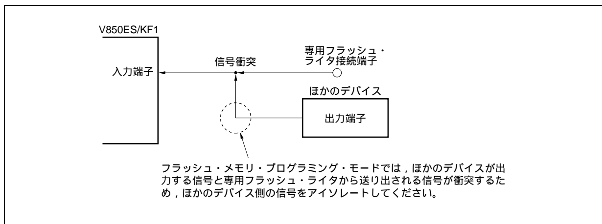
図25 - 12 信号の衝突（シリアル・インタフェースの入力端子）
