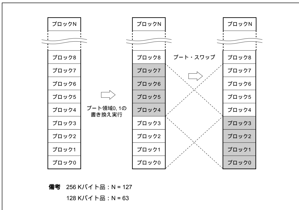
図25 - 16 全メモリ領域の書き換え (ブート・スワップ対応)
