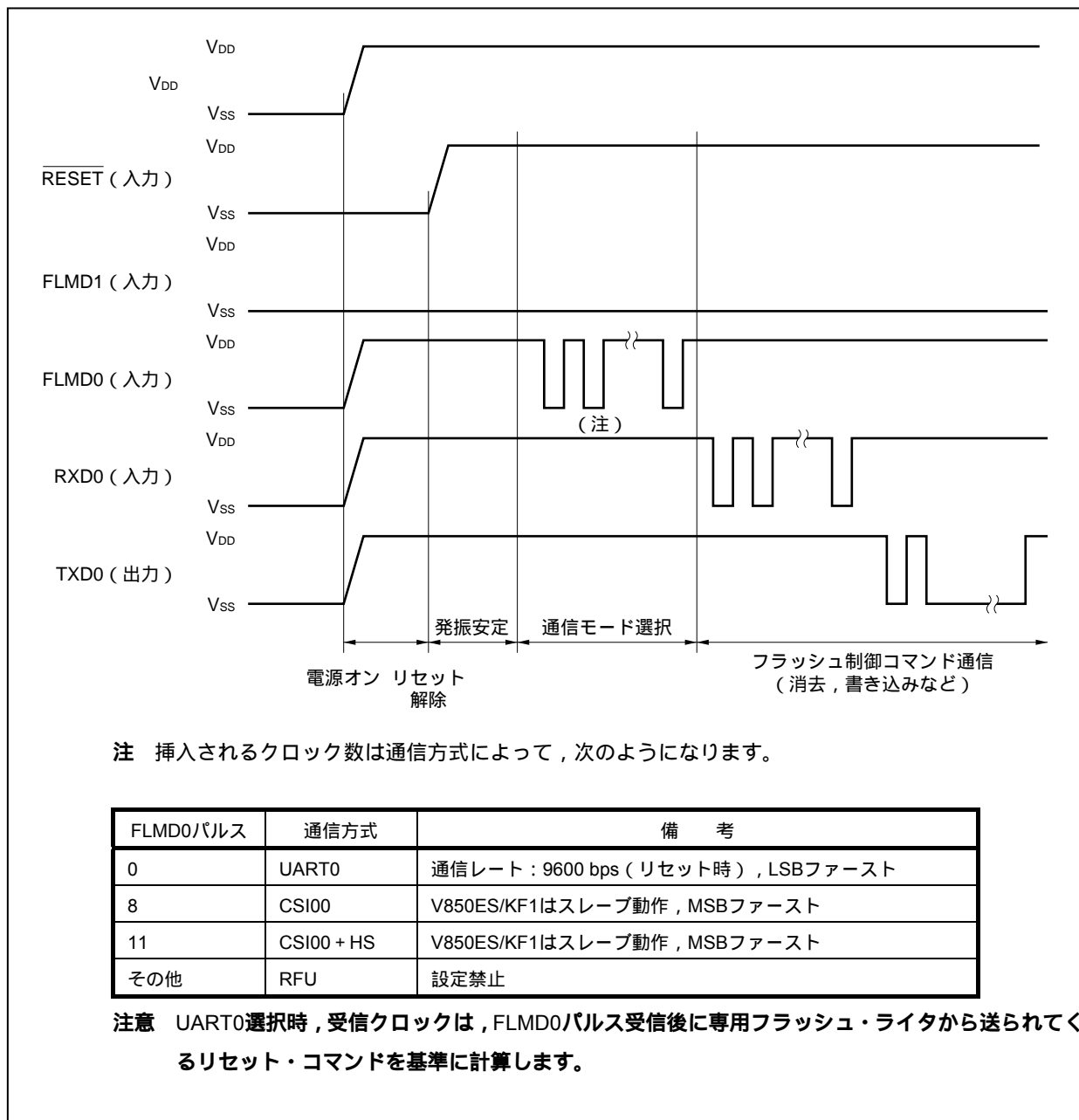
図25-8 通信方式の選択
