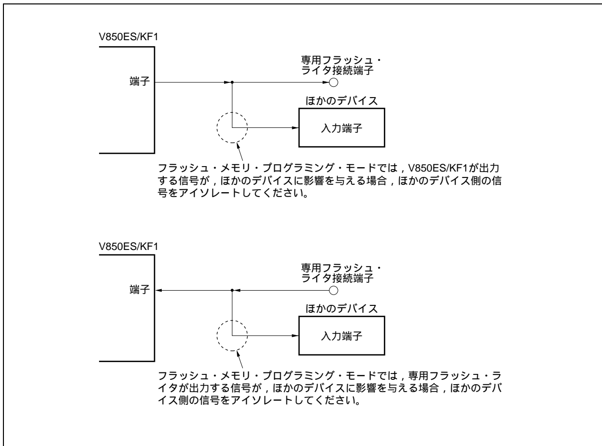
図26 - 8 ほかのデバイスの異常動作
