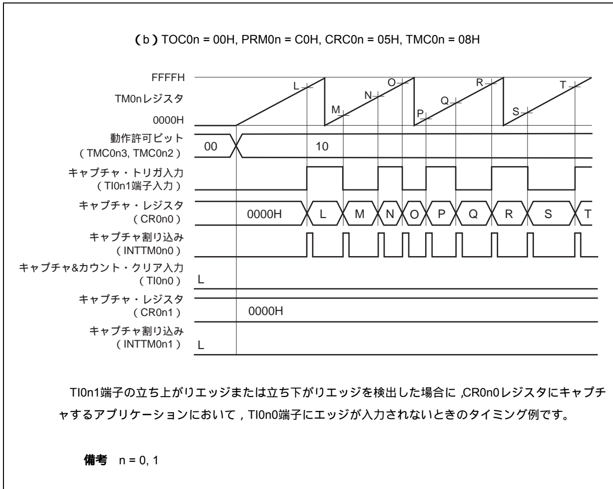
図8 - 20 TI0n0端子の有効エッジ入力によるクリア&スタート・モードのタイミング例 (CR0n0レジスタ：キャプチャ・レジスタ/CR0n1レジスタ：キャプチャ・レジスタ) (2/3)
