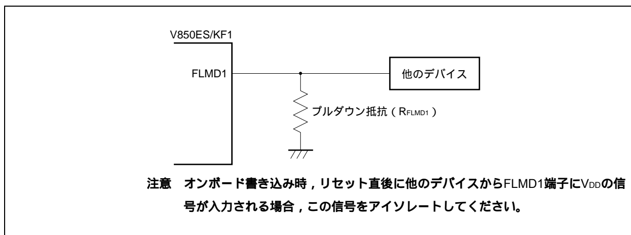
図25 - 11 FLMD1端子の接続例
