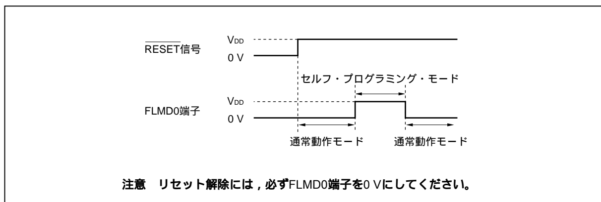
図25 - 18 モード切り替わりタイミング
