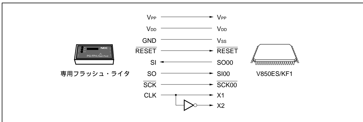
図26 - 4 専用フラッシュ・ライタとの通信 (CSI00)
