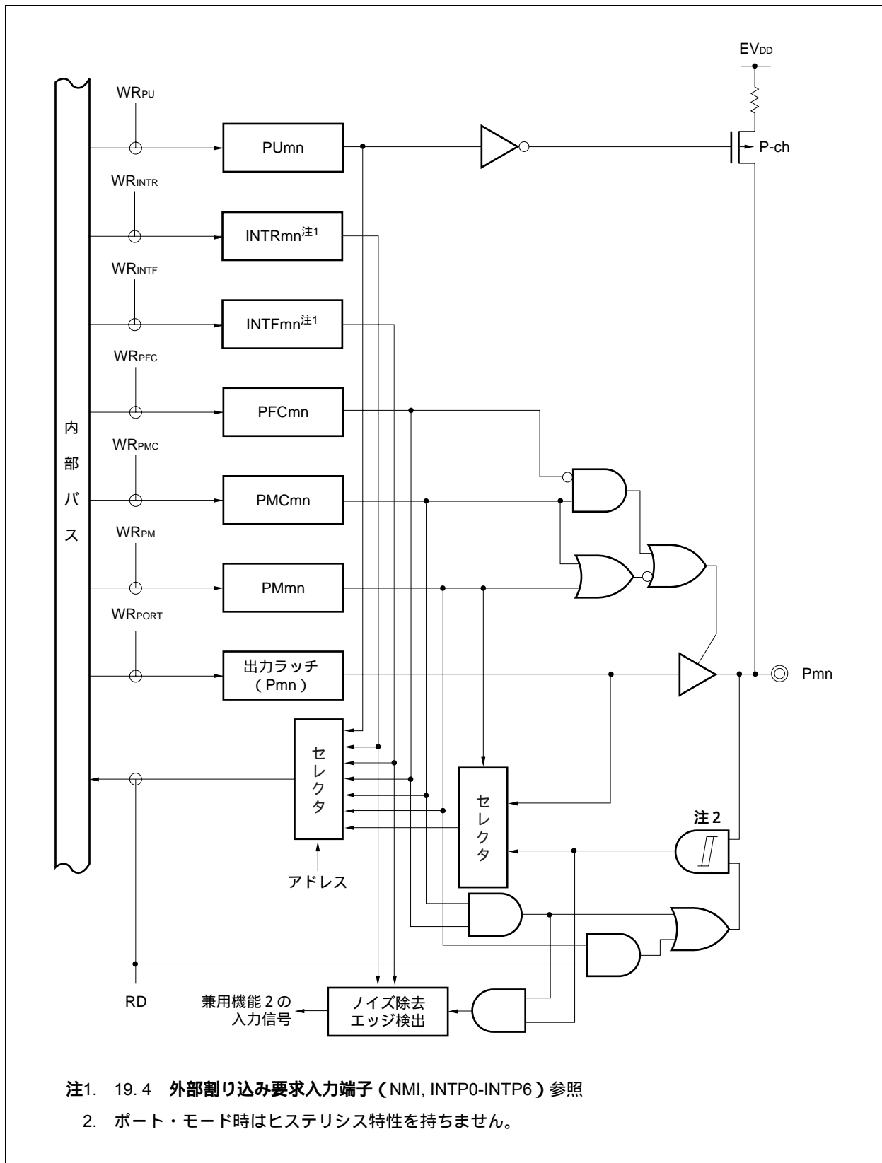
図4 - 25 タイプH-3のブロック図
