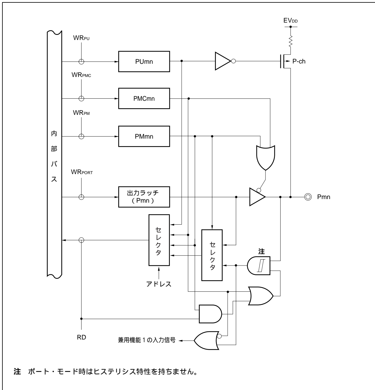
図4-7 タイプD-1-1のブロック図
