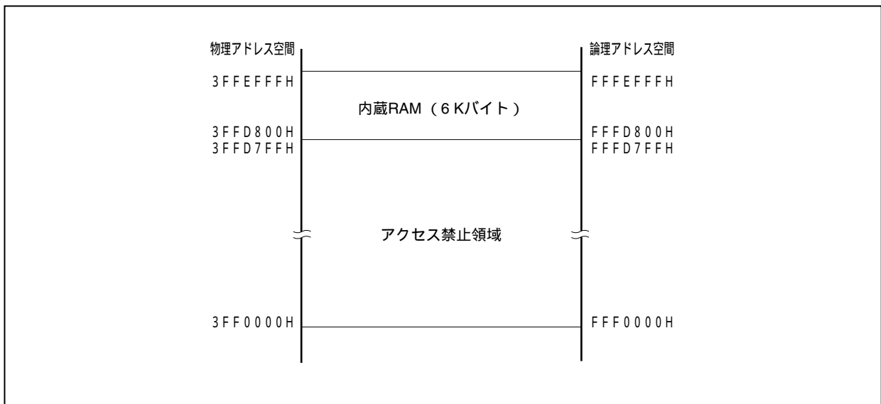
図3 - 9 内蔵RAM (6 Kバイト)
