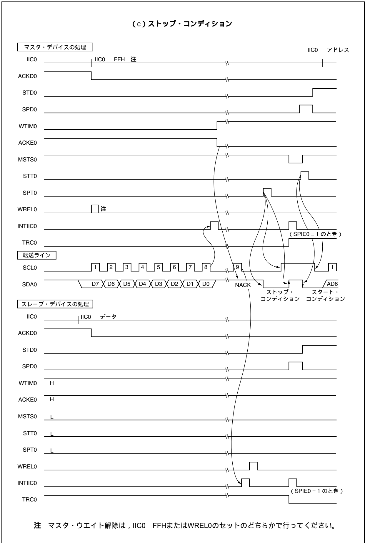
図18-21 スレーブ マスタ通信例 (マスタ: 8 クロック, スレーブ: 9クロックでウェイト選択時) (3/3)
