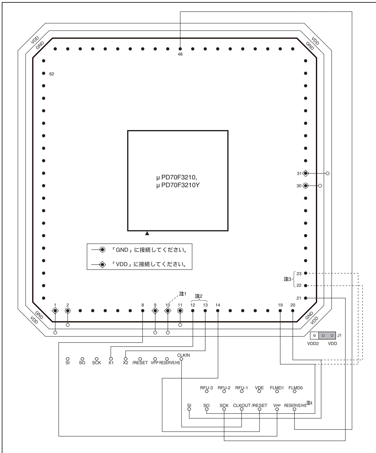
図26 - 1 V850ES/KF1フラッシュ書き込み用アダプタ (FA-80GC-8BT-A, FA-80GK-9EU-A) の配線例 (1/2)
