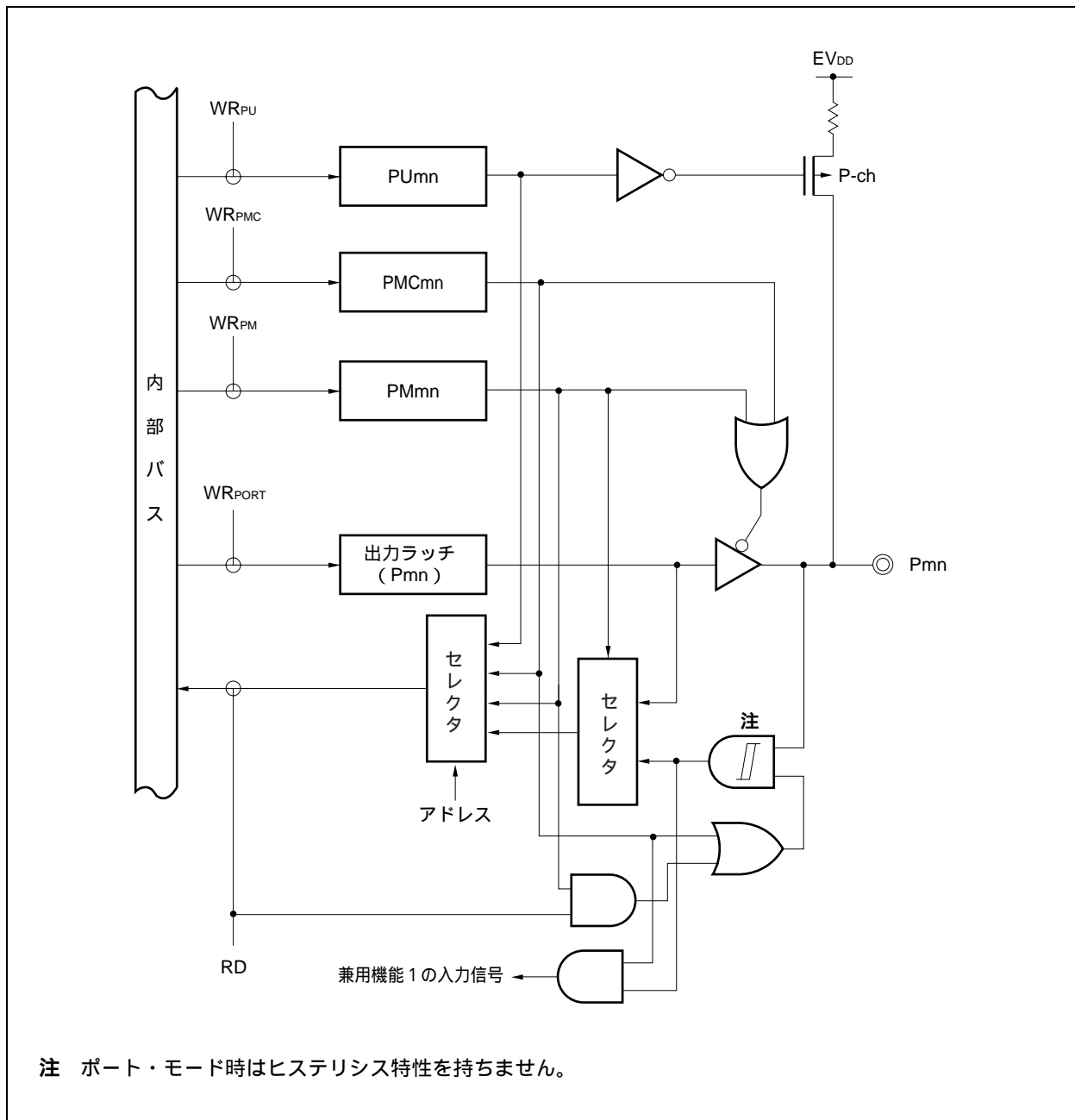
図4-8 タイプD-1-2のブロック図
