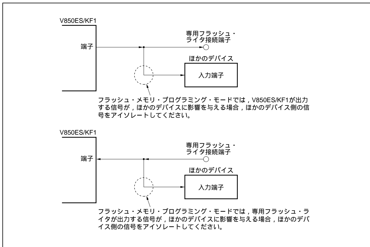
図25 - 13 ほかのデバイスの異常動作
