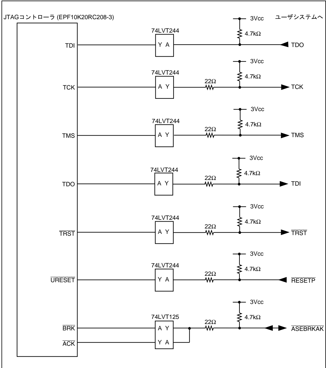
図 6.7 E10A エミュレータ内ユーザシステムインタフェース回路 (HS7660KCI01H) ( Model 名 : HS0005KCI03H )
