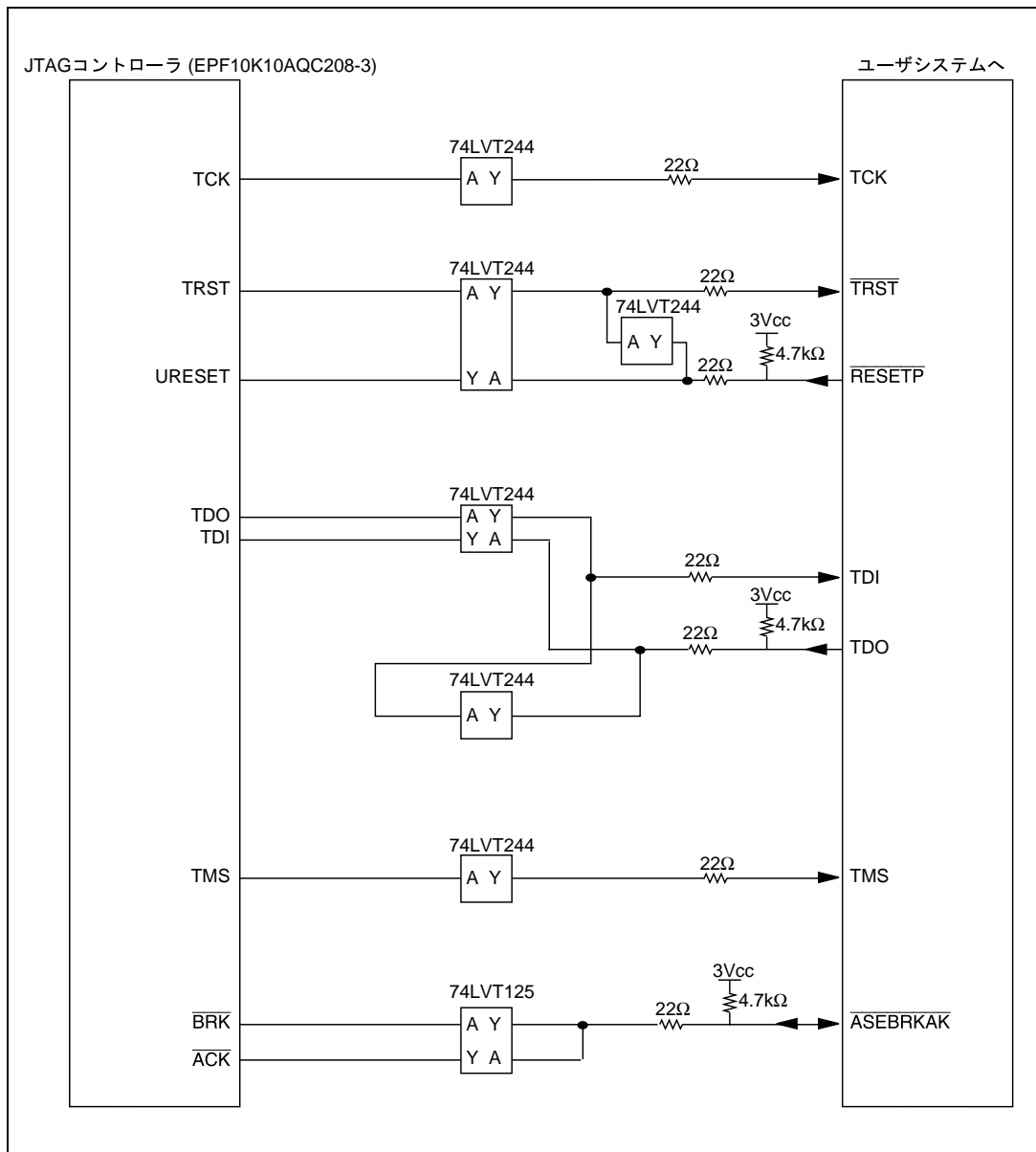
図 6.8 H-UDI 端子部分の E10A エミュレータ内ユーザシステムインタフェース回路 (HS7660KCI02H) (Model 名 : HS0005KCI04H)
