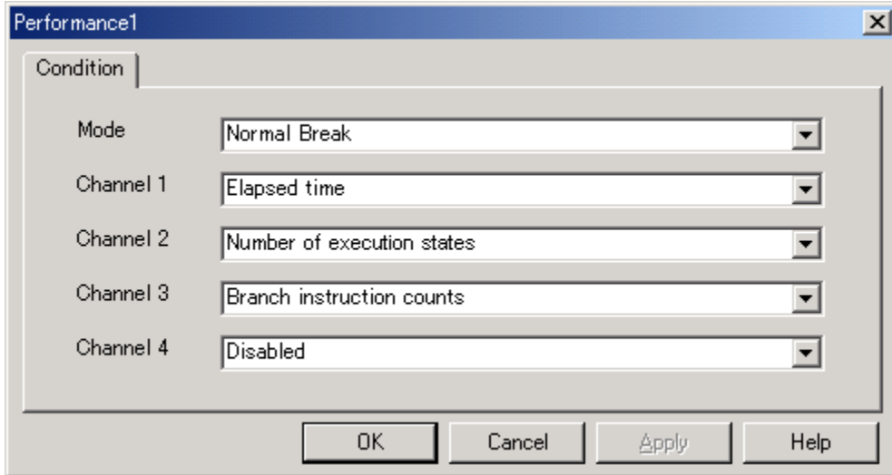
図 6.15 [Performance1]ダイアログボックス
