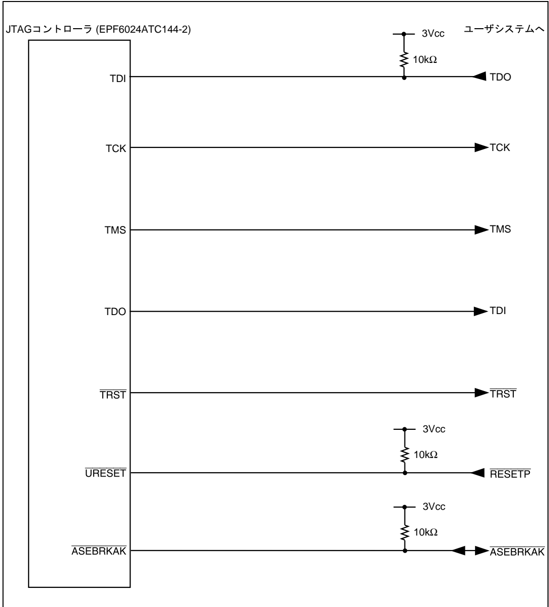
図 6.5 H-UDI 端子部分の E10A エミュレータ内ユーザシステムインタフェース回路 (HS7660KCM02H) (Model 名 : HS0005KCM04H)
