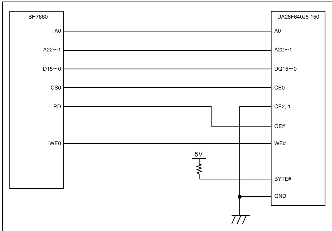
図 6.17 フラッシュメモリの結線図
