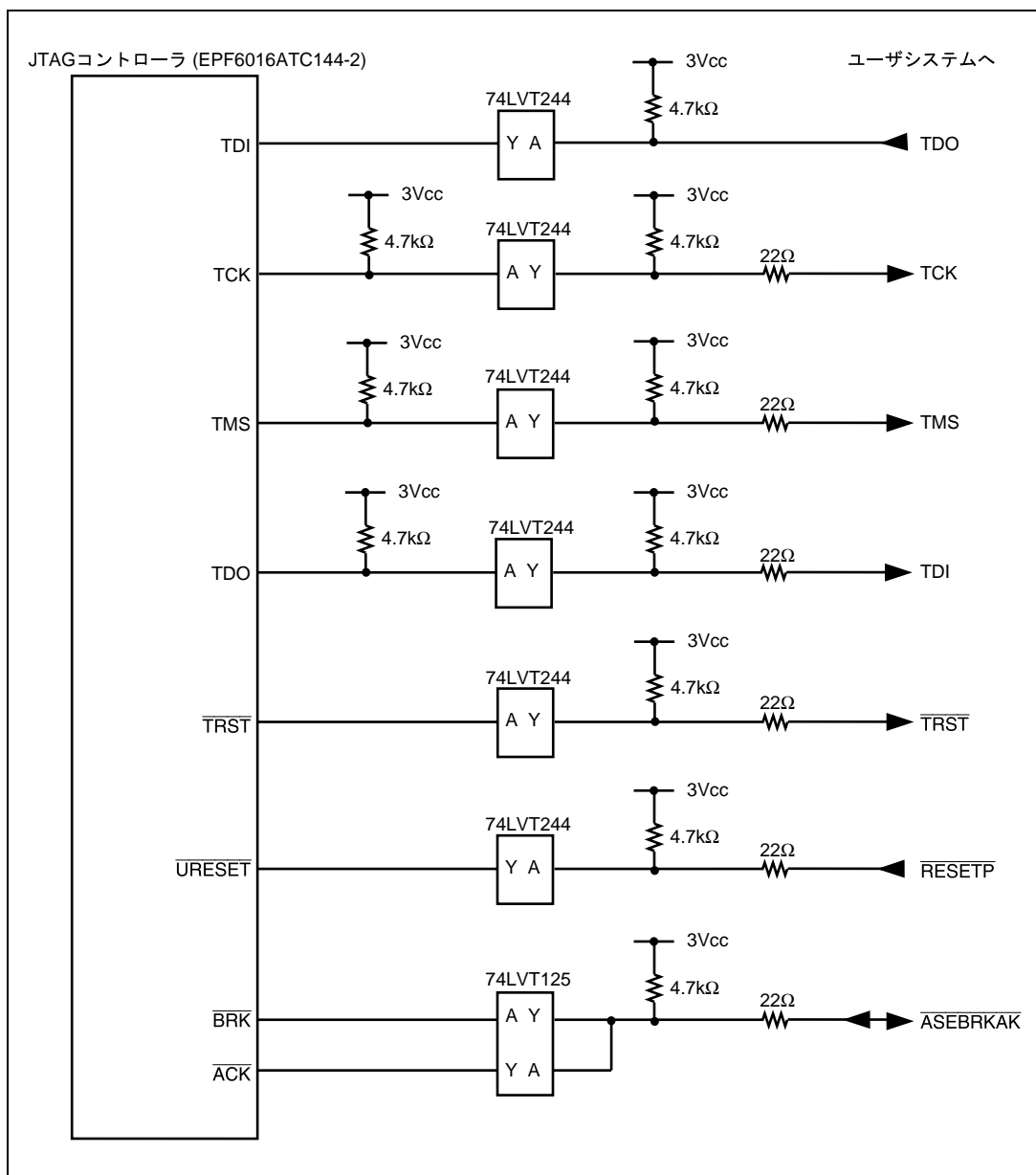
図 6.4 E10A エミュレータ内ユーザシステムインタフェース回路 (HS7660KCM01H) ( Model 名 : HS0005KCM03H )
