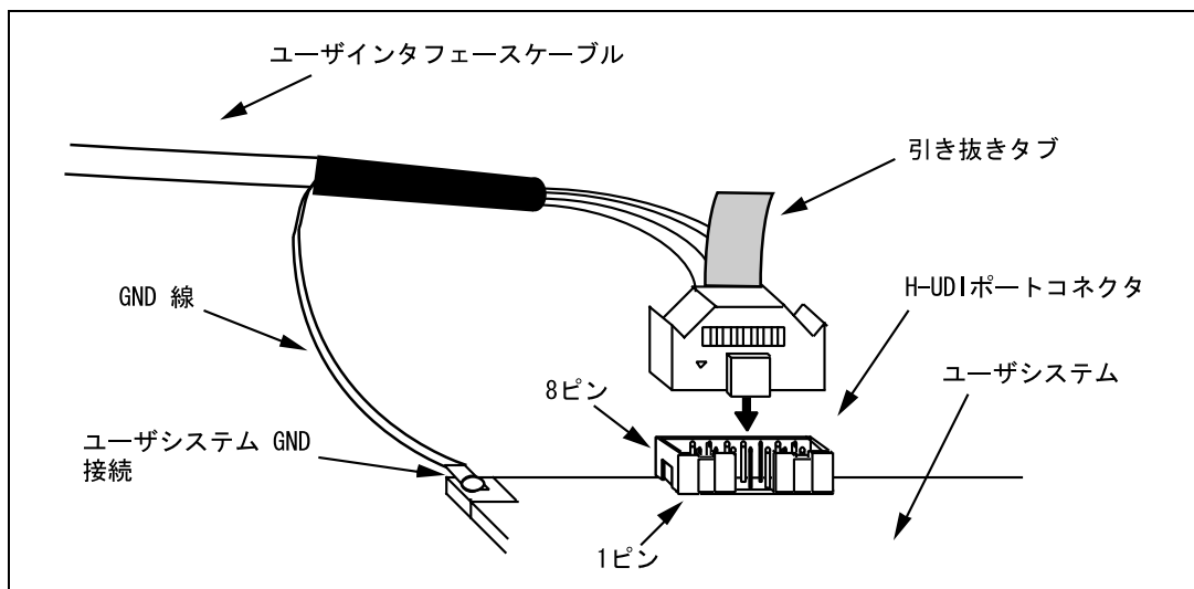
図 2.4 14 ピンストレートタイプコネクタ使用時のユーザシステム側のユーザインタフェースケーブル接続方法
