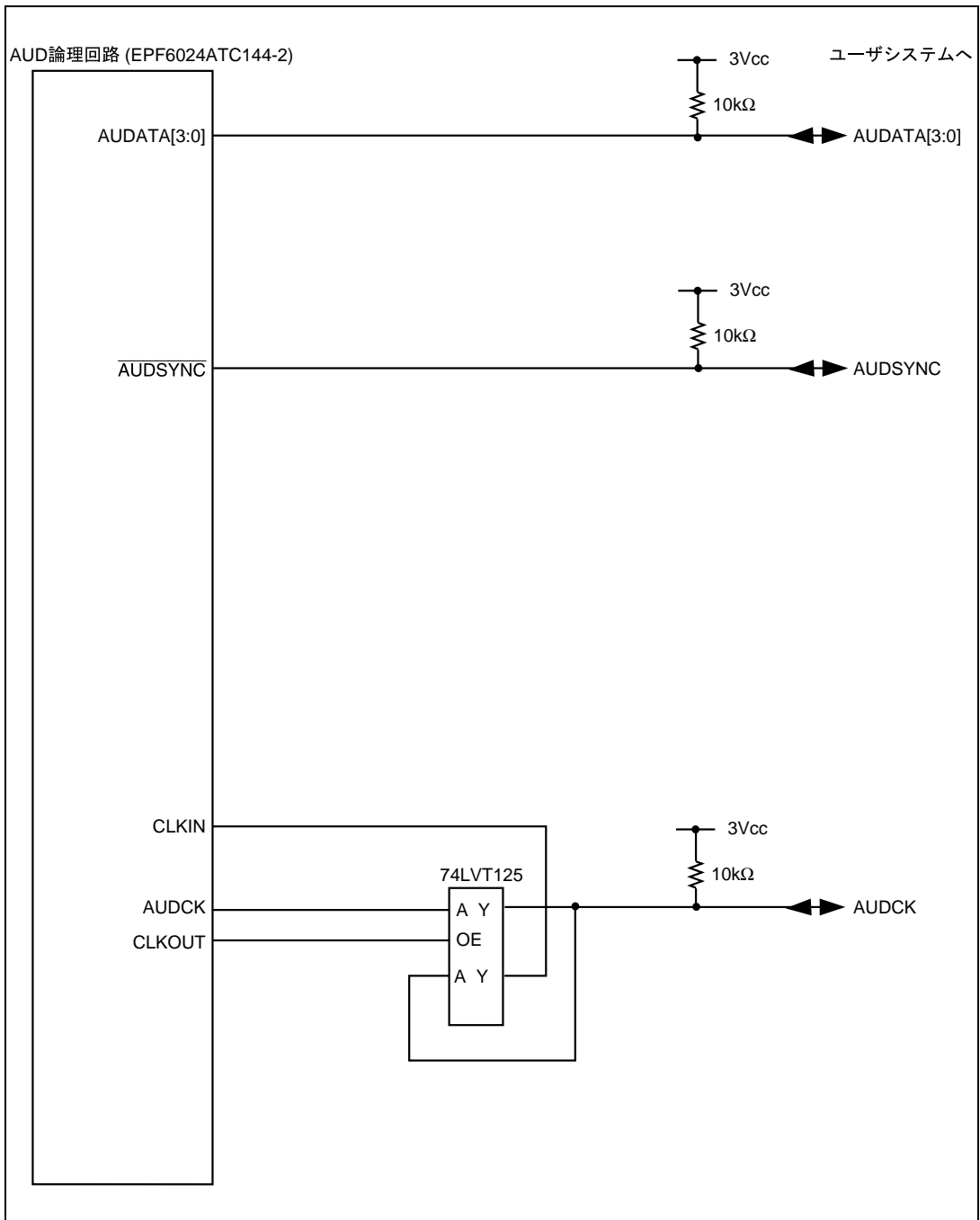
図 6.6 AUD 端子部分の E10A エミュレータ内ユーザーシステムインタフェース回路 (HS7660KCM02H) (Model 名 : HS0005KCM04H)
