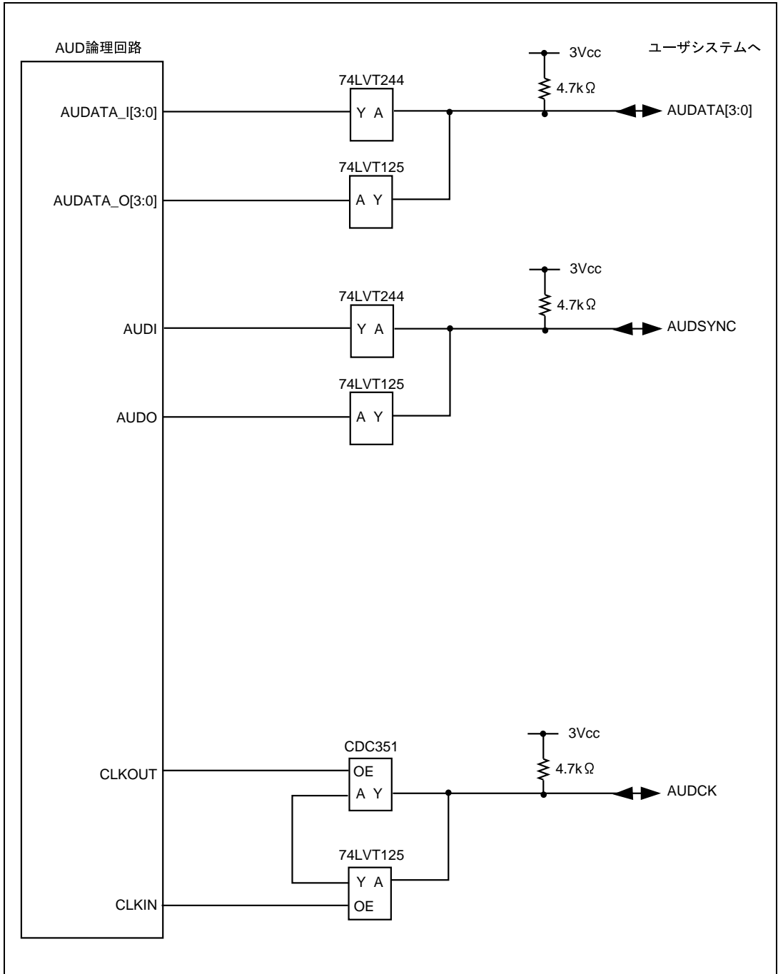
図 6.9 AUD 端子部分の E10A エミュレータ内ユーザーシステムインタフェース回路 (HS7660KCI02H) (Model 名 : HS0005KCI04H)
