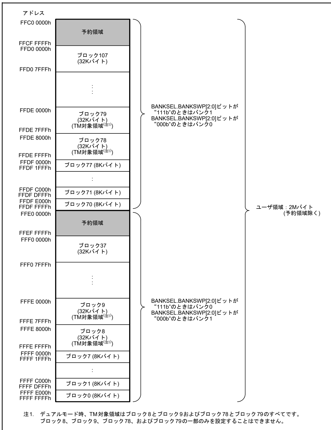
図 60.4 デュアルモード時のコードフラッシュメモリマッピング (コードフラッシュメモリ容量が2Mバイトの製品)
