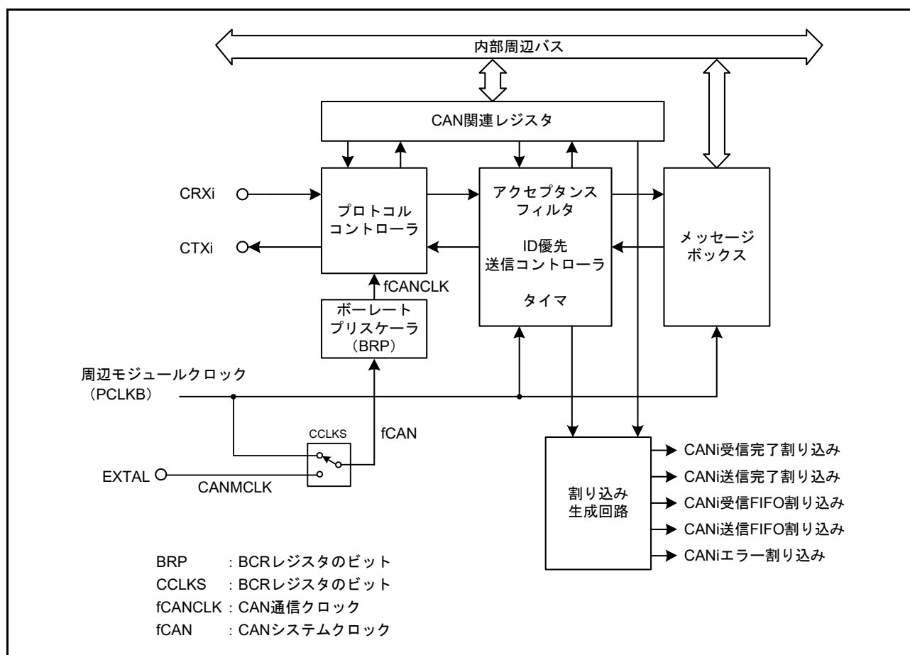
図 42.1 CAN モジュールブロック図 (i = 0 ~ 2)
