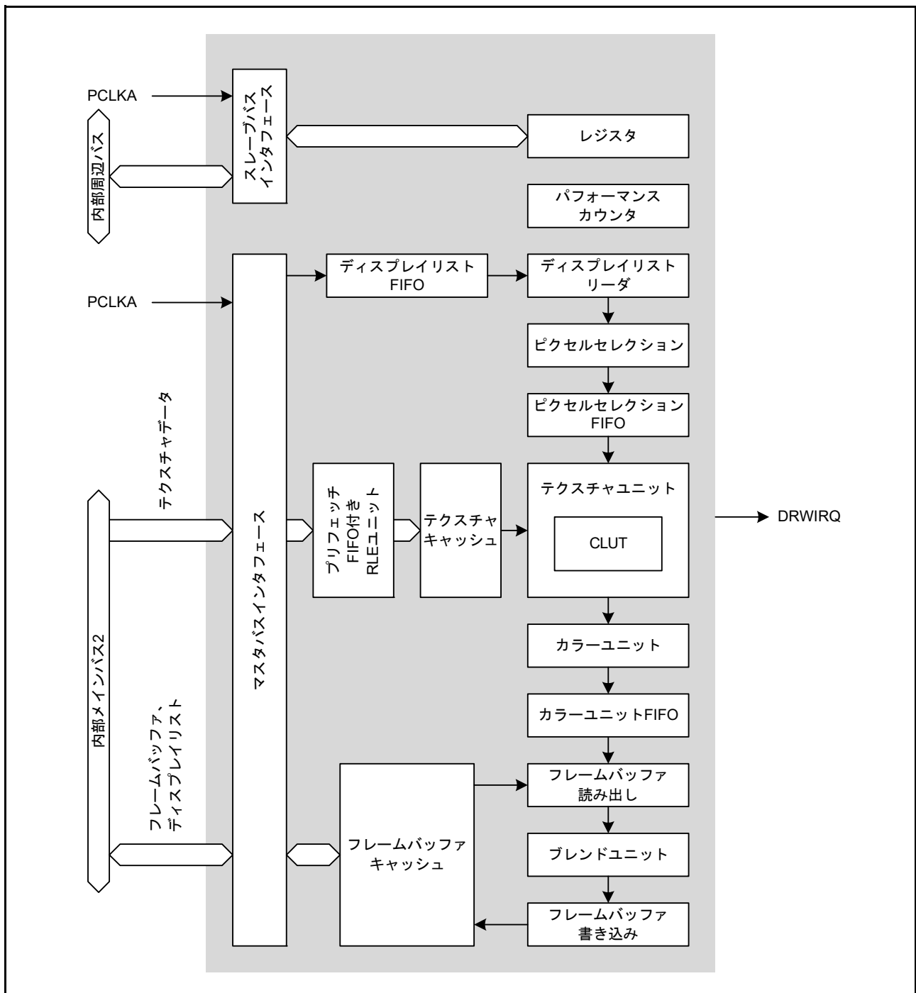
図 51.2 DRW2D のブロック図
