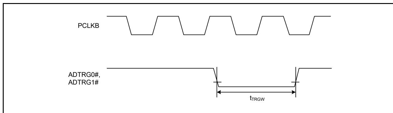
図 61.97 A/Dコンバータトリガ入力タイミング
