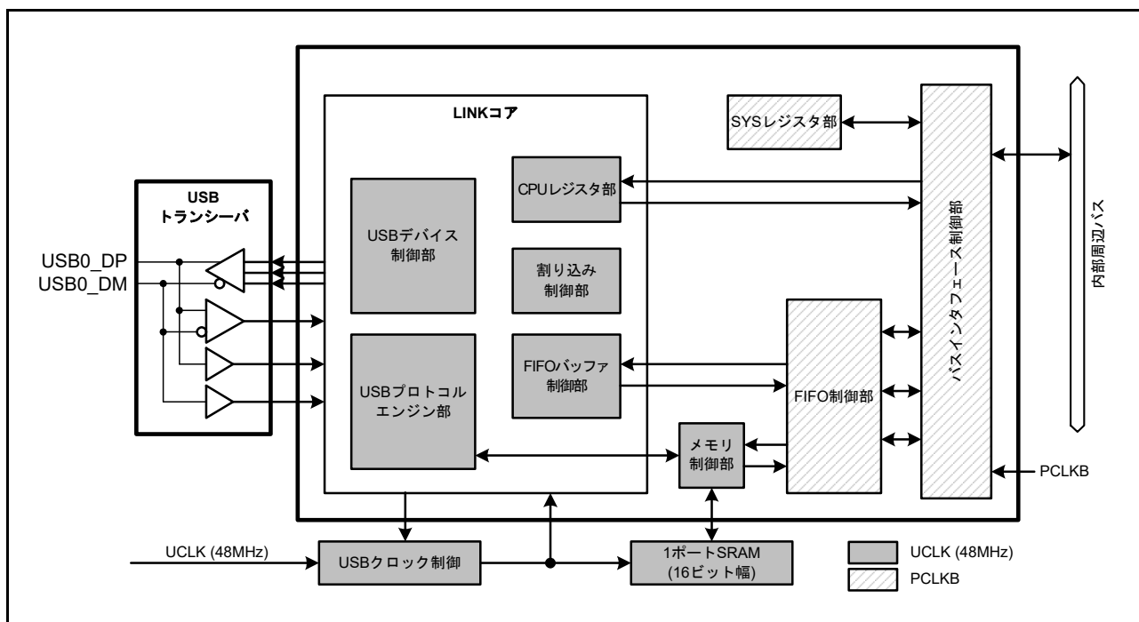
図 39.1 USB のブロック図
