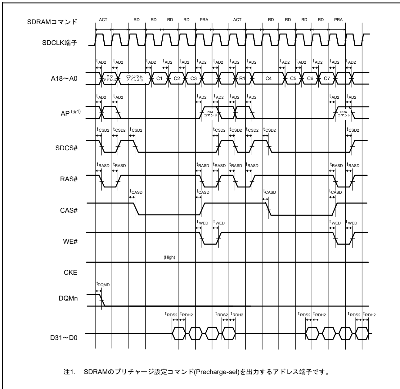
図 61.29 SDRAM 空間複数リード行またぎバスタイミング
