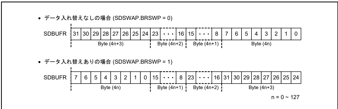
図 47.5 SDBUFRレジスタ読み出し時のデータ配置
