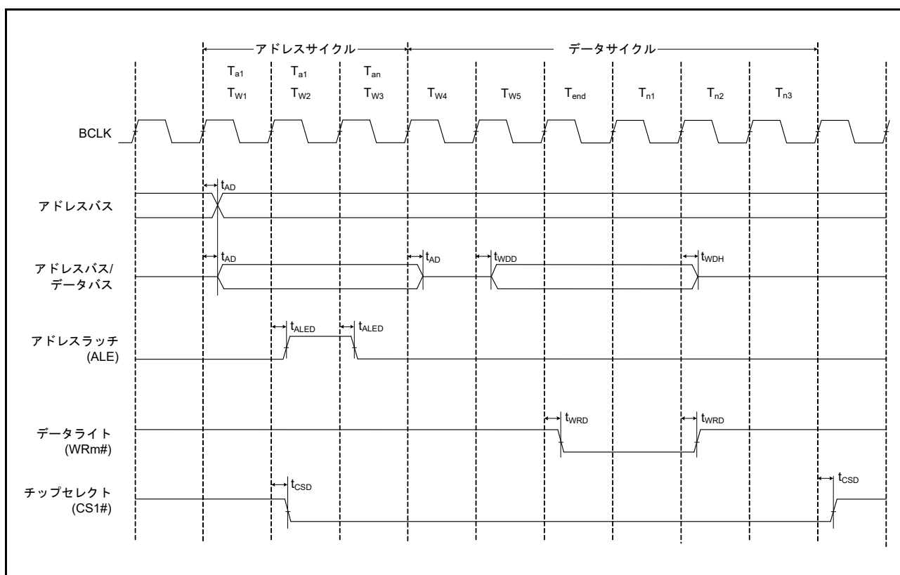
図 61.19 アドレス/データマルチプレクスバスのライトアクセスタイミング
