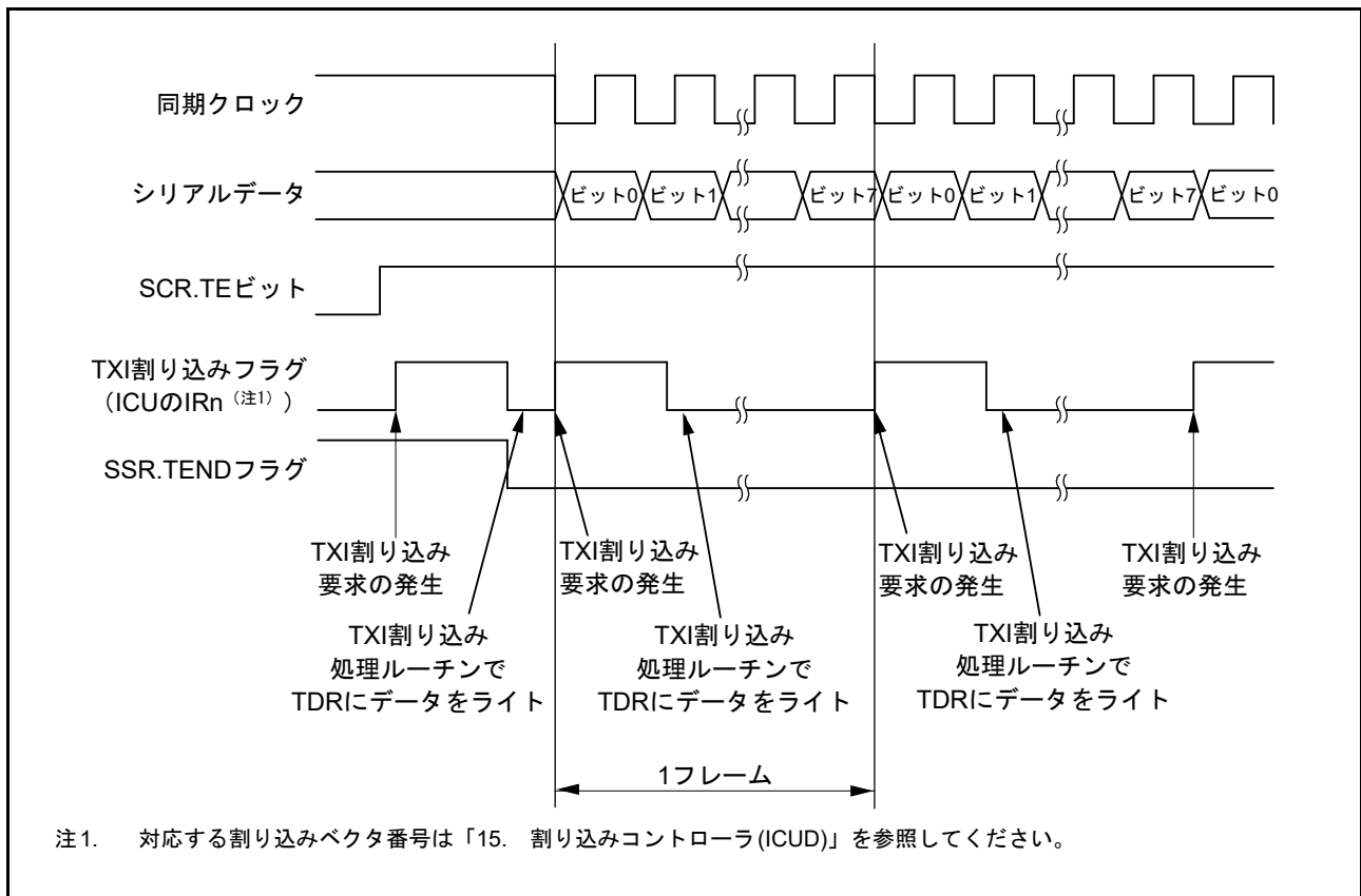
図 40.29 クロック同期式モードのシリアル送信の動作例 (1) (送信開始・CTS 機能使用しない)
