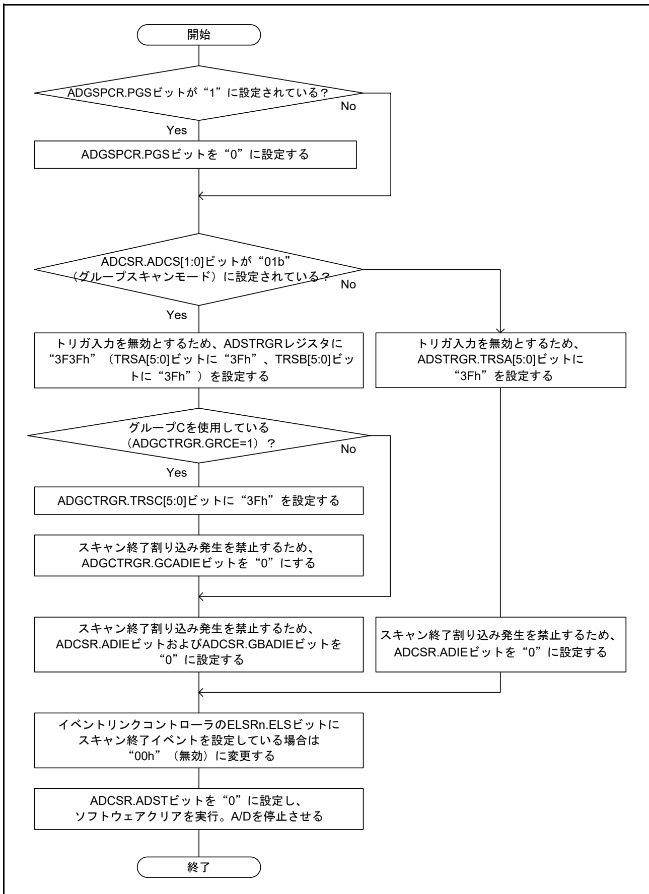
図 54.46 ADCSR.ADST ビットによるソフトウェアクリア実行の設定フロー
