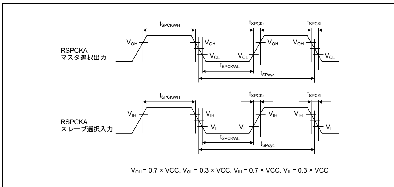
図 61.63 RSPCKA クロックタイミング
