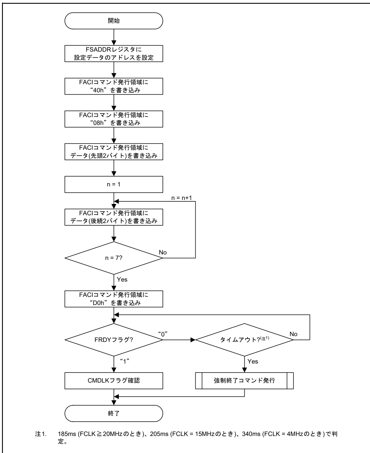
図 60.25 コンフィギュレーション設定コマンドの使用法
