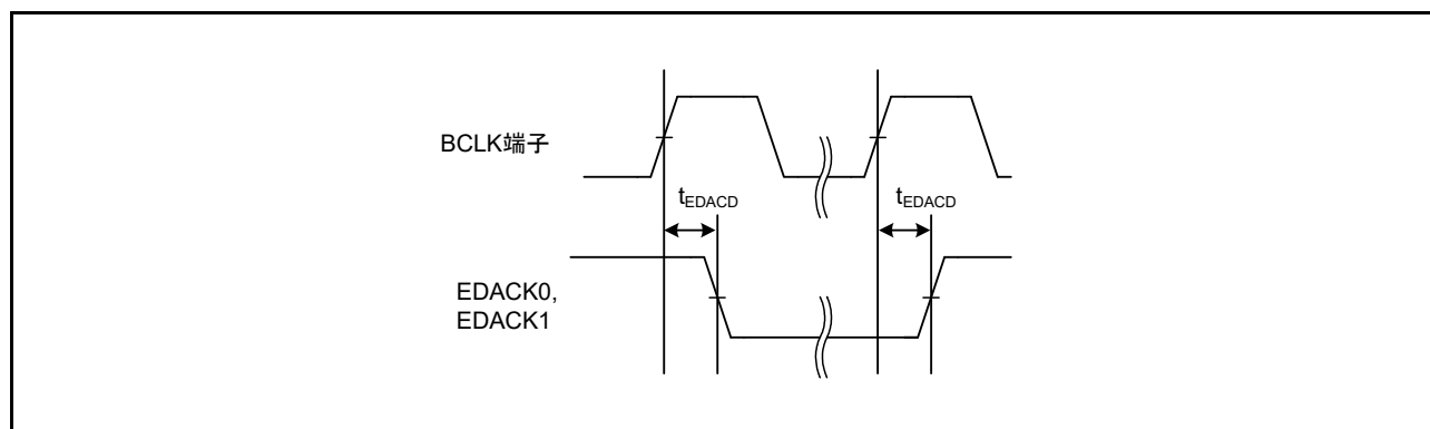
図 61.34 EDACK0、EDACK1 シングルアドレス転送タイミング (SDRAM 領域)
