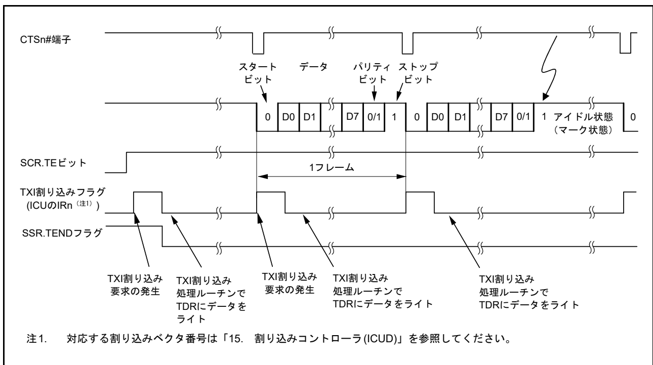
図 40.15 調歩同期式モードのシリアル送信の動作例 (2) (8ビットデータ / パリティあり / 1ストップビット / CTS 機能使用する / 送信開始時)
