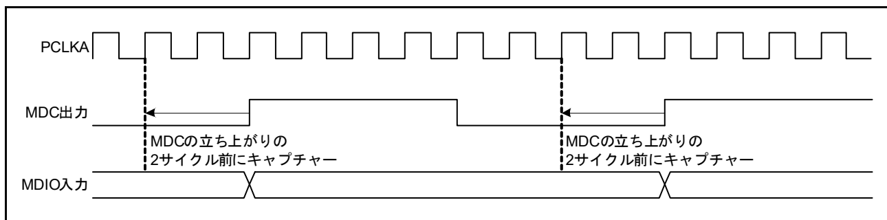
図 38.10 PCLKA の 2 サイクル前にキャプチャー時のタイミング
