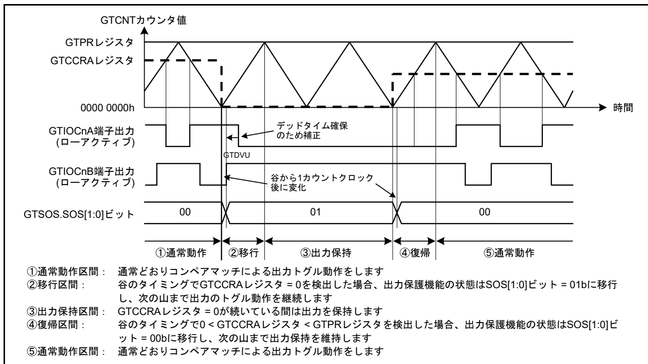
図 26.127 谷のバッファ転送で GTCCRA レジスタが “0000 0000h” である場合の出力保護機能の動作例 (谷のバッファ転送で 0 < \text{GTCCRA} < \text{GTPR} レジスタに復帰、アクティブレベルは Low の場合) (n = 0 ~ 3)
