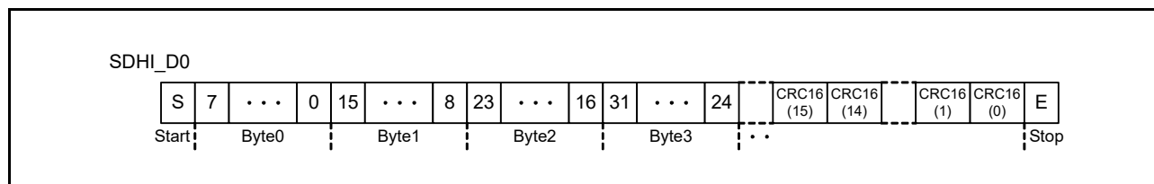
図 47.2 デフォルトバスモードの転送フォーマット (SDOPT.WIDTH ビットが“1”のとき)
