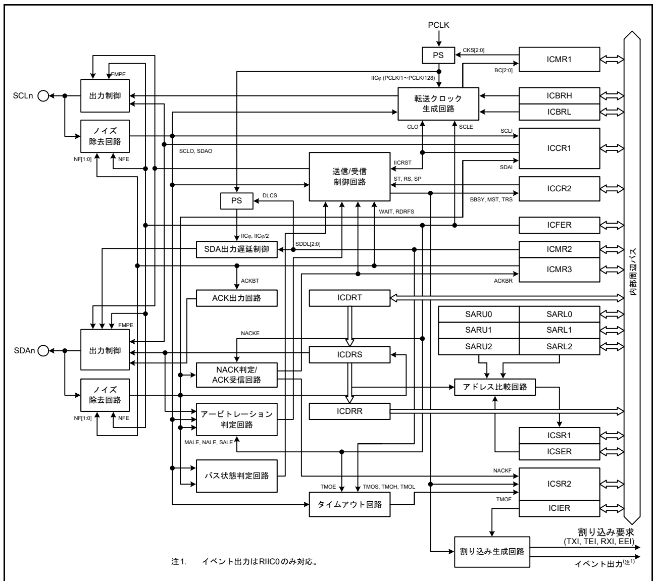
図 41.1 RIIC のブロック図 (n = 0 ~ 2)
