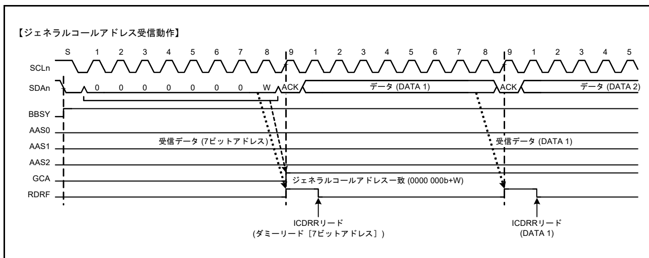
図 41.26 ジェネラルコールアドレス受信時に GCA フラグが“1”になるタイミング
