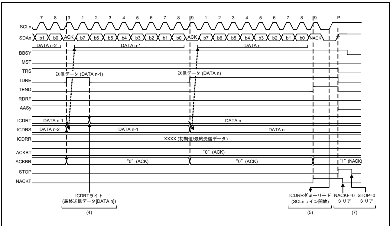
図 41.16 スレーブ送信の動作タイミング (2)
