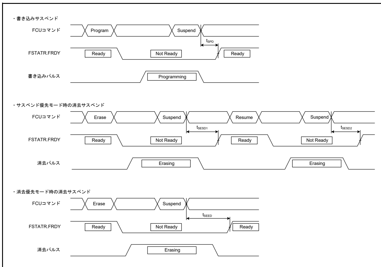
図 61.108 フラッシュメモリプログラム/イレーズサスペンドタイミング
