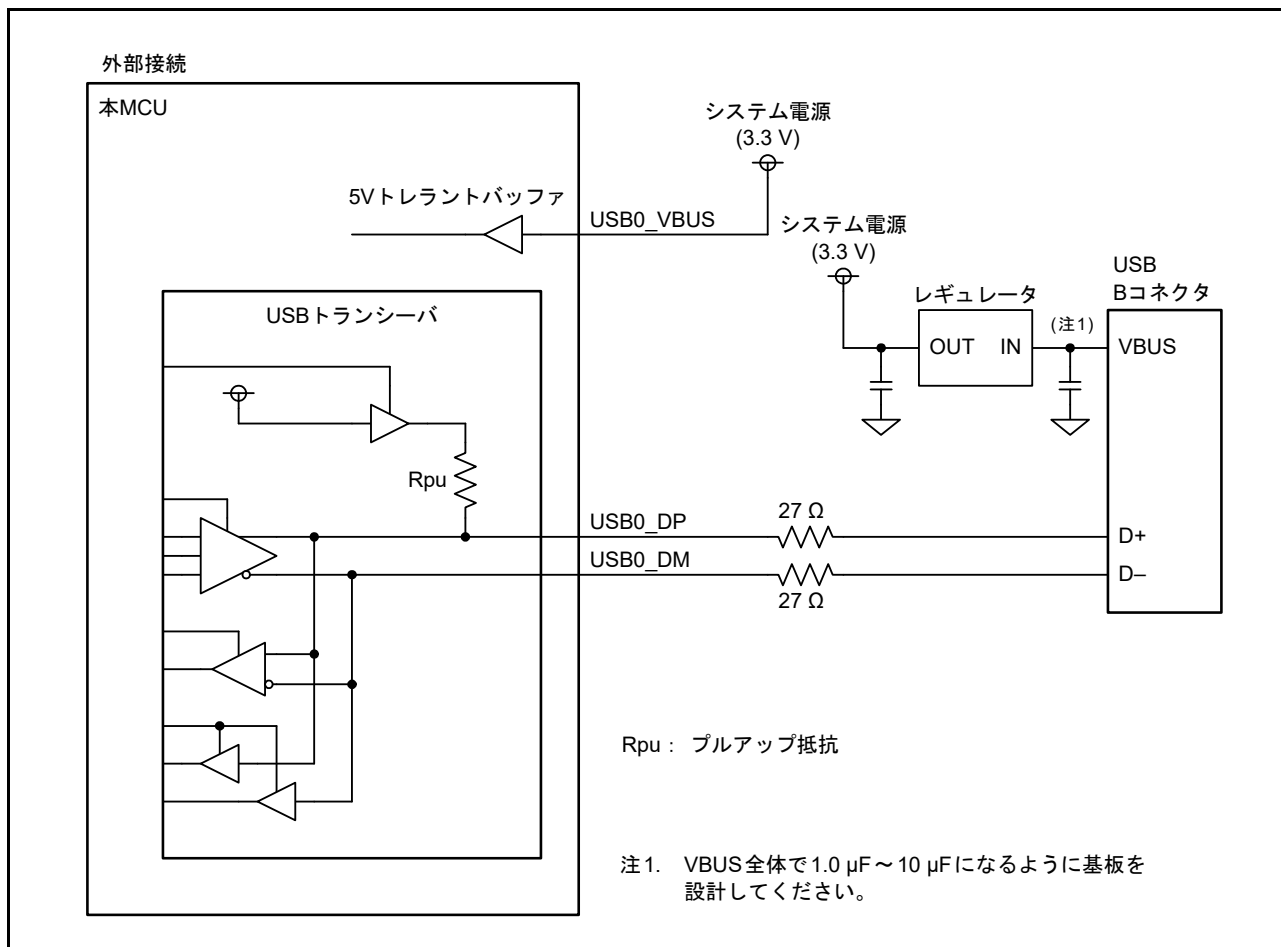
図 39.5 バスパワー時のファンクションコントローラと USB コネクタとの接続例
