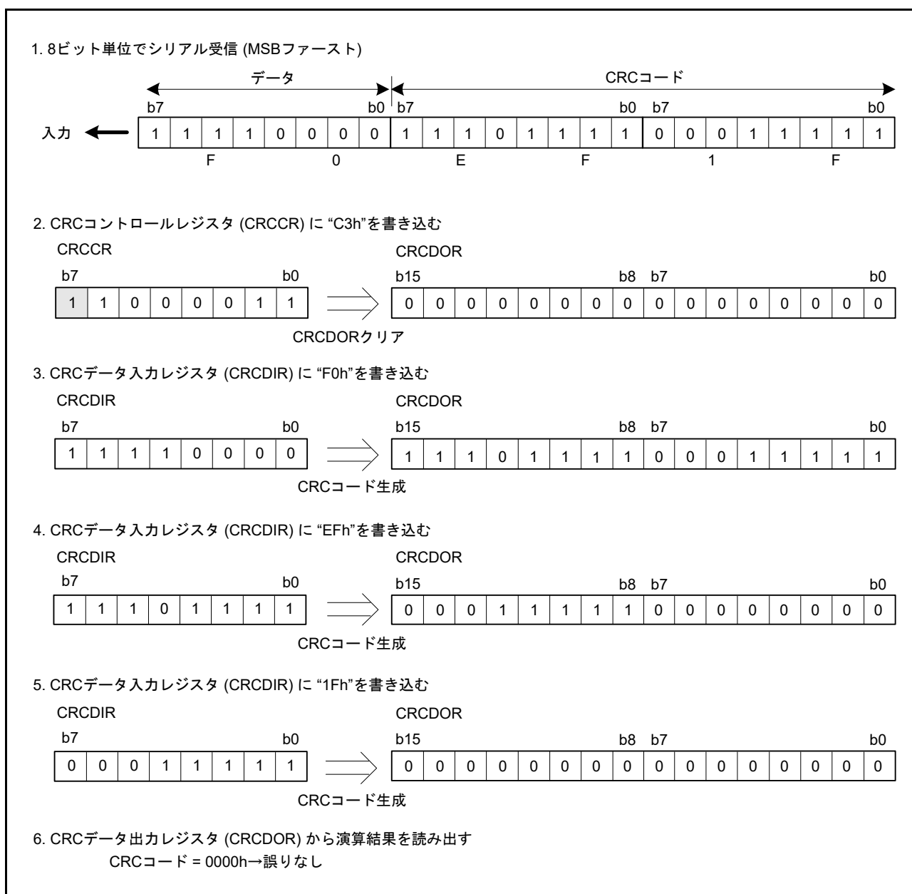
図 45.5 MSB ファーストでのデータ受信
