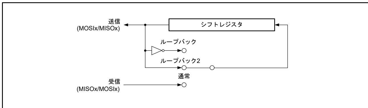
図 43.50 ループバックモード時のシフトレジスタ入出力構成 (マスターモード)
