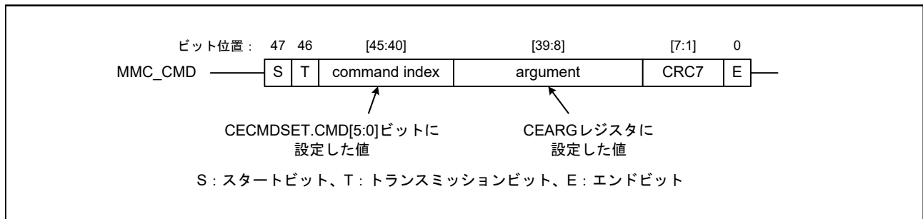
図 48.2 コマンドのフォーマット
