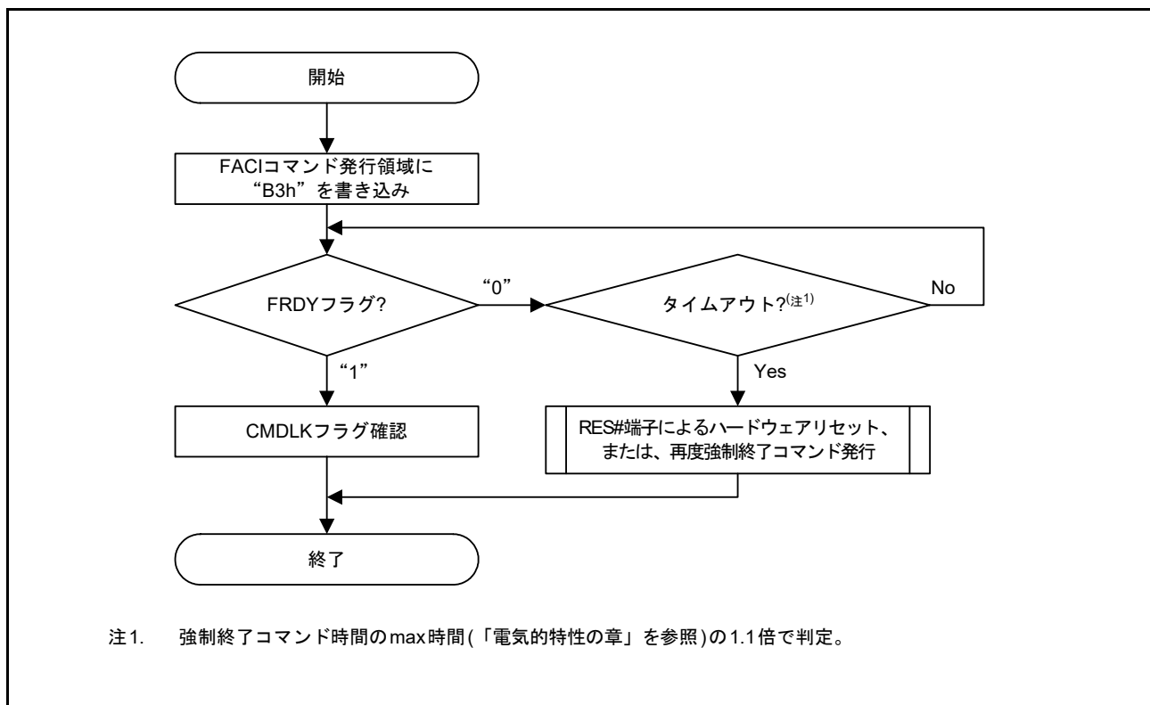
図 60.23 強制終了コマンドの使用方法
