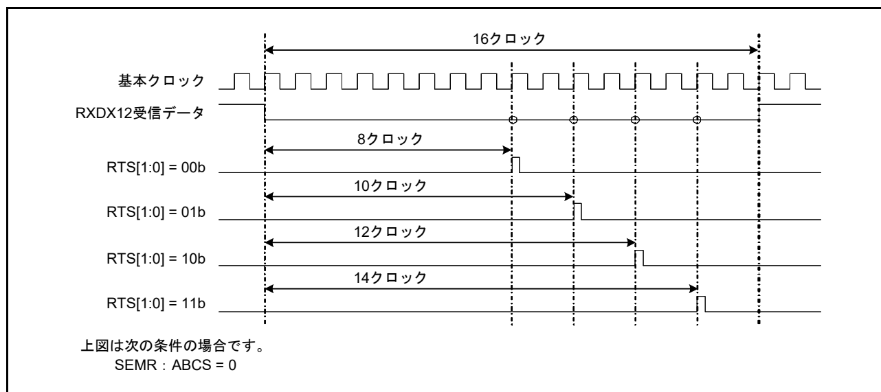
図 40.76 RXDX12 受信データサンプリングタイミング
