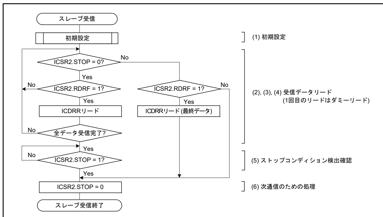
図 41.17 スレーブ受信のフローチャート例
