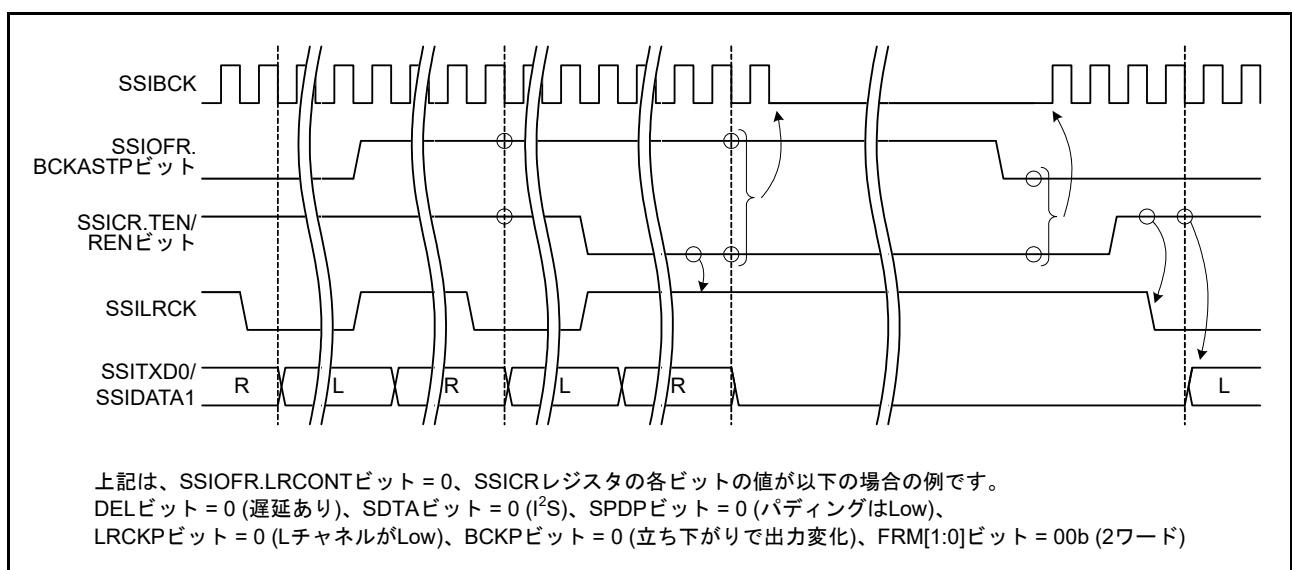
図 46.19 BCK 連続出力停止機能の動作例
