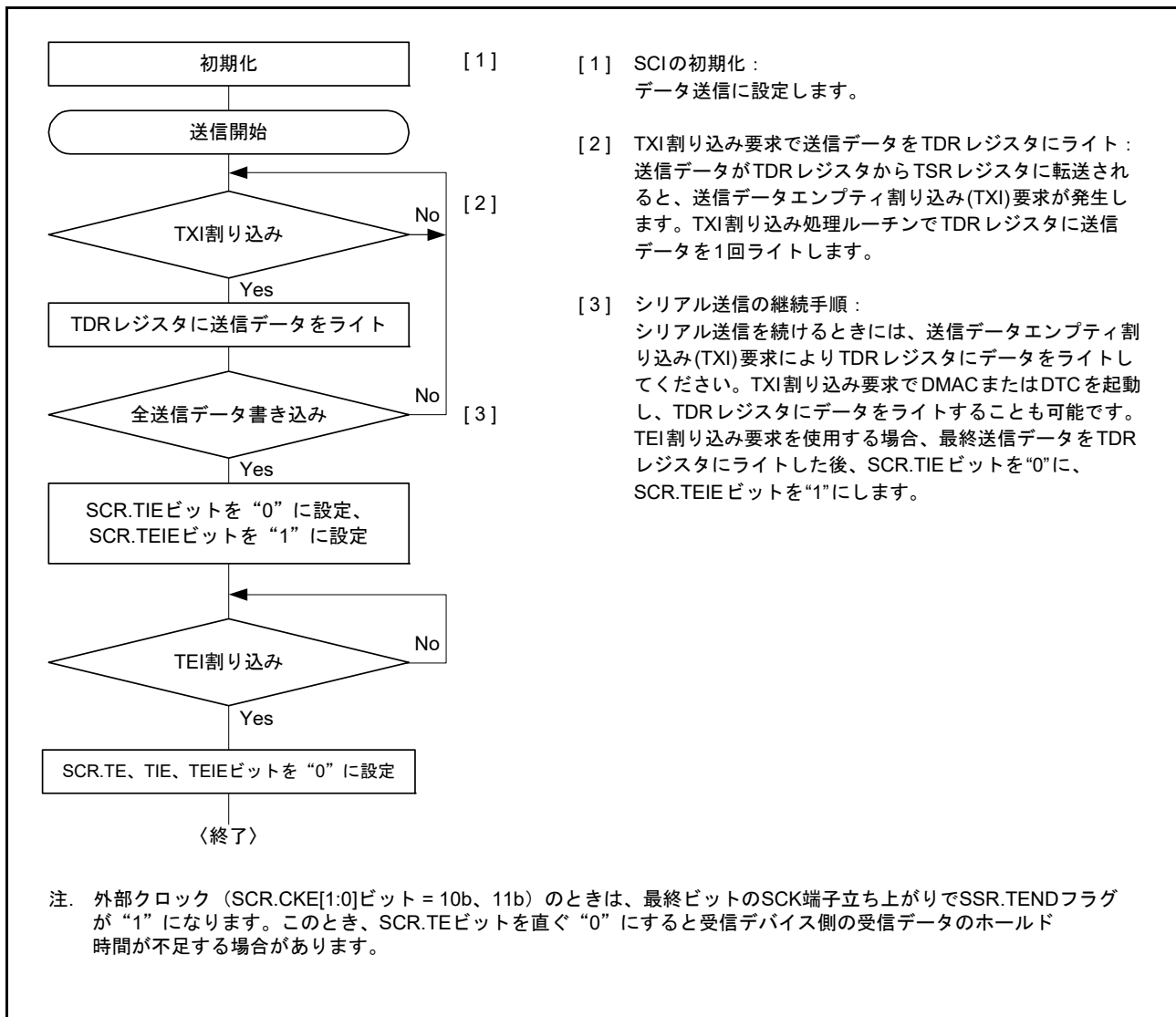
図 40.32 クロック同期式モードのシリアル送信のフローチャート例
