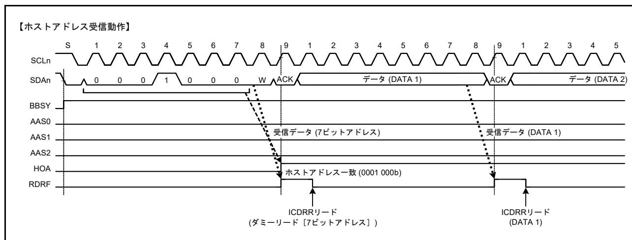
図 41.28 ホストアドレス受信時に HOA フラグが “1” になるタイミング
