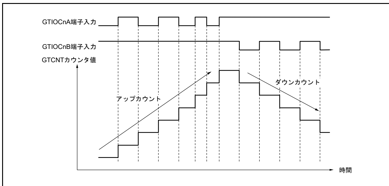
図 26.93 位相計数モード3の動作例 (n = 0 ~ 3)
