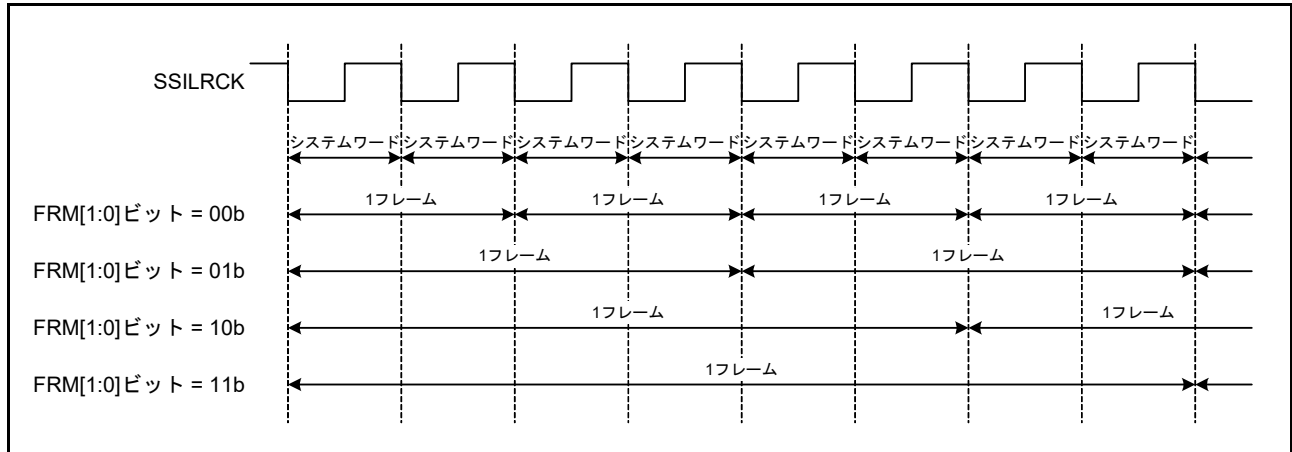
図 46.5 フレームワード長
