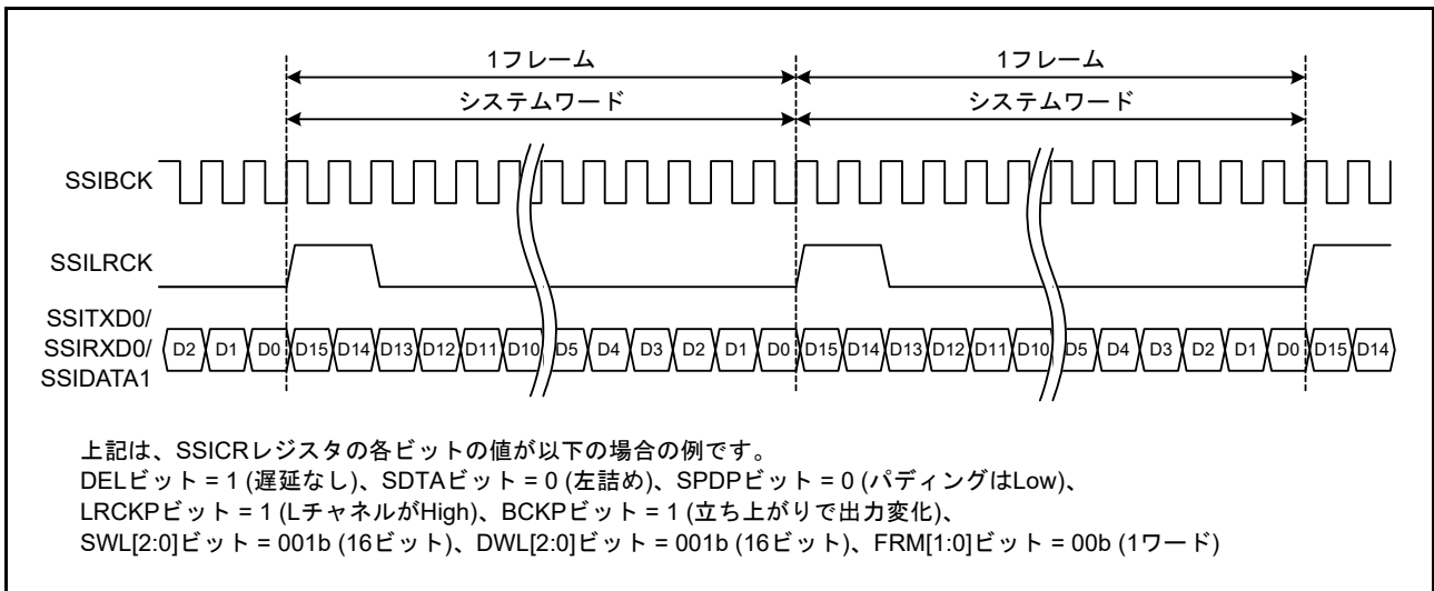
図 46.14 モノラルフォーマットの例 (3) (SSICR.DEL ビット = 1、パディングなし)
