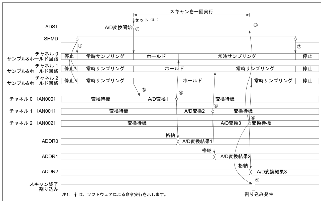
図 54.8 シングルスキャンモードの動作例 (チャンネル専用サンプル & ホールド回路使用 : AN000 ~ AN002 選択、常時サンプリング有効)
