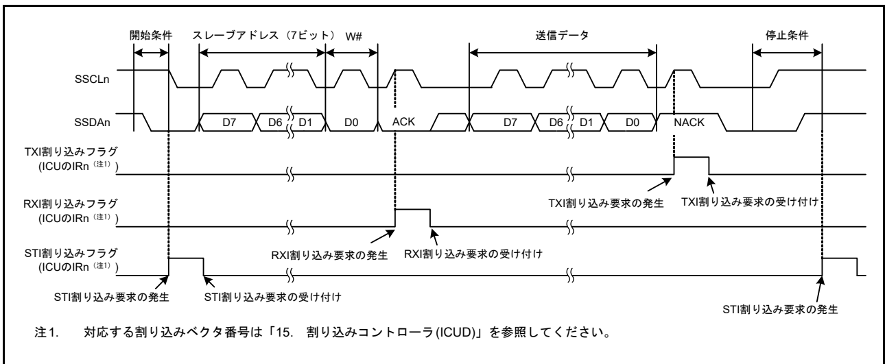
図 40.57 簡易 I 2 C バスモードのマスタ送信の動作例 2 (7 ビットスレーブアドレス、ACK 割り込み、NACK 割り込み使用時)
