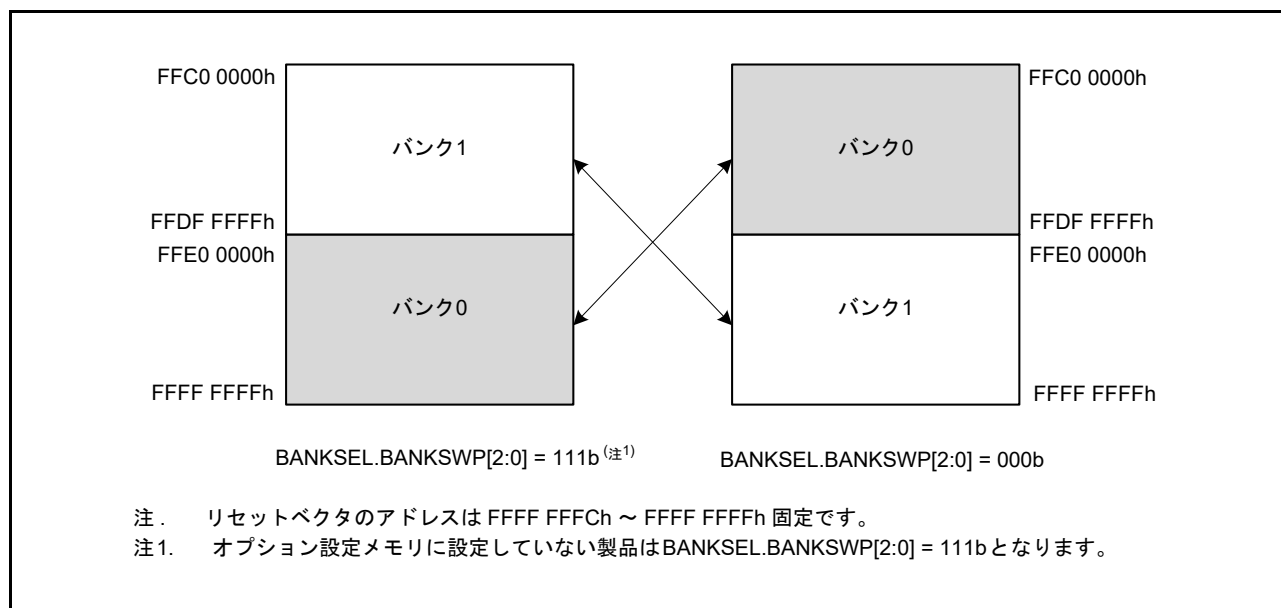
図 60.32 起動バンク選択例 (コードフラッシュメモリ容量が 4M バイトの製品の例)
