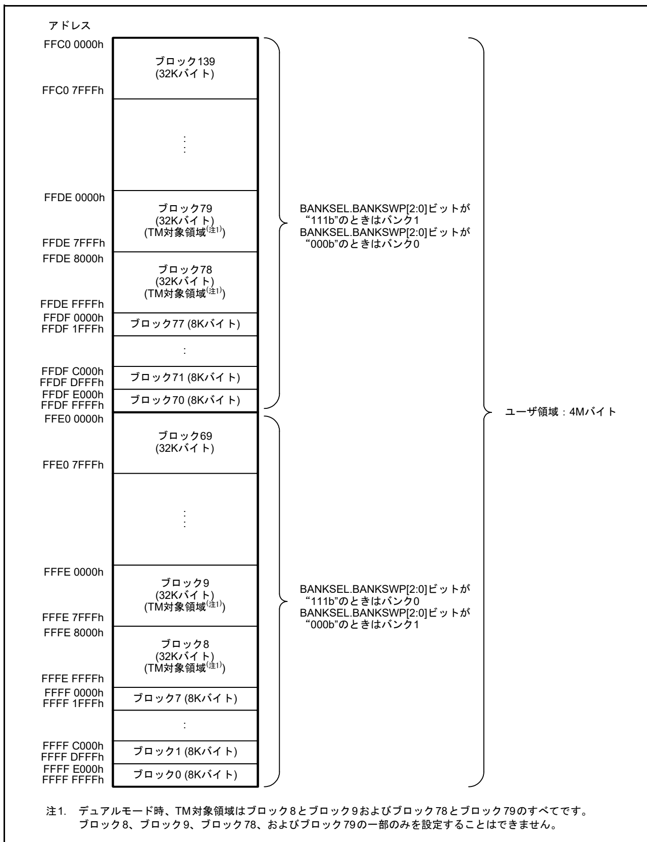
図 60.3 デュアルモード時のコードフラッシュメモリマッピング (コードフラッシュメモリ容量が4Mバイトの製品)
