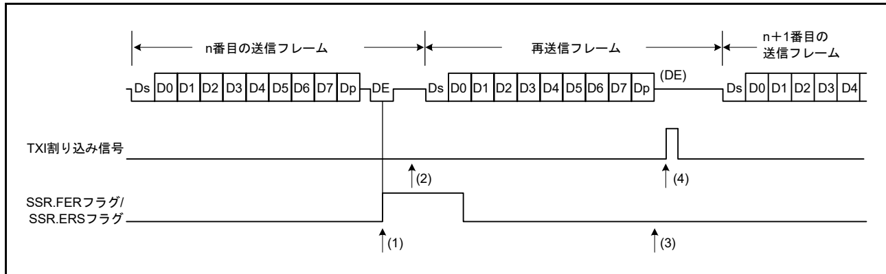
図 40.44 SCI 送信モードの場合の再送信動作 (送信時の再送信動作)
