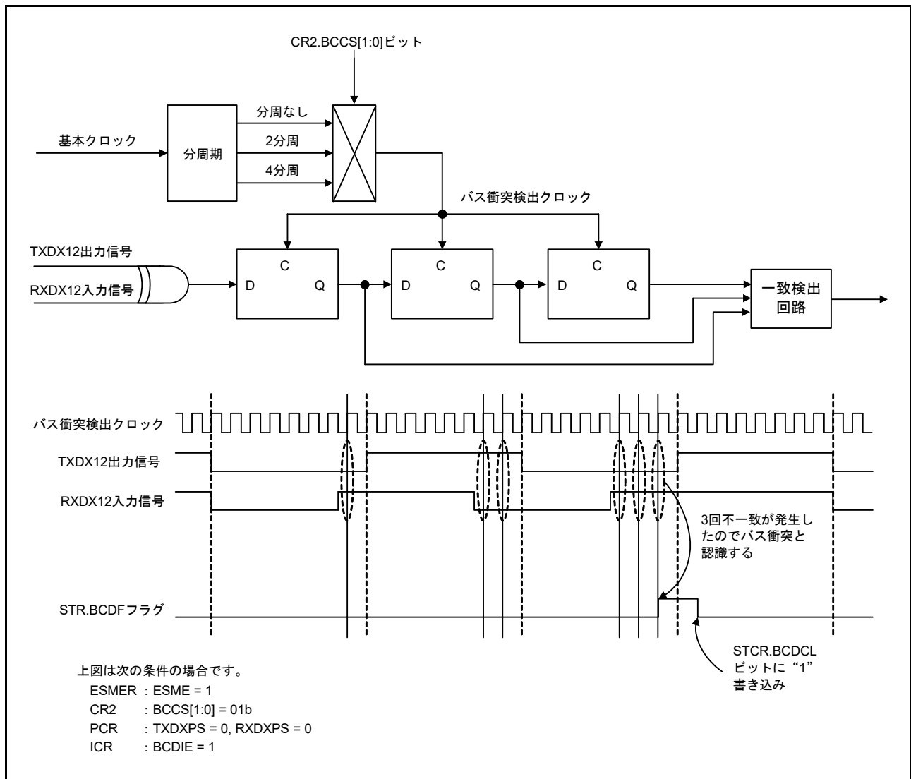
図 40.73 バス衝突検出機能の動作例
