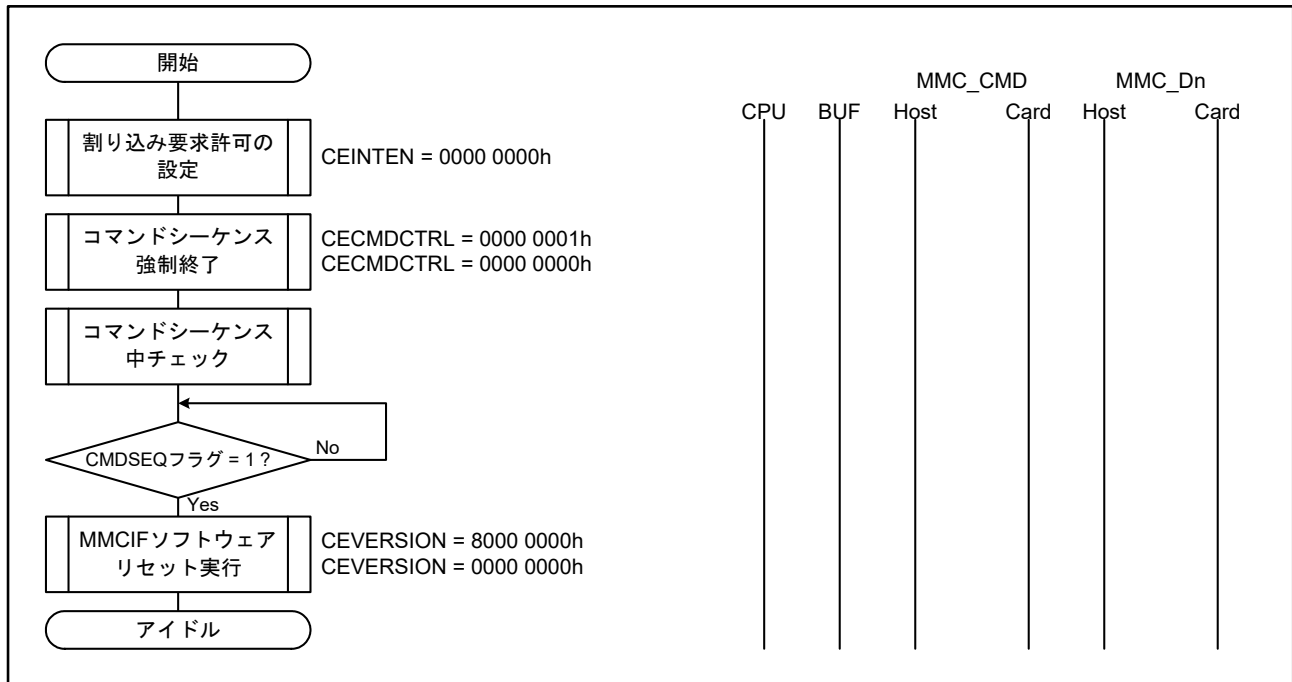
図 48.22 コマンドシーケンス強制終了例
