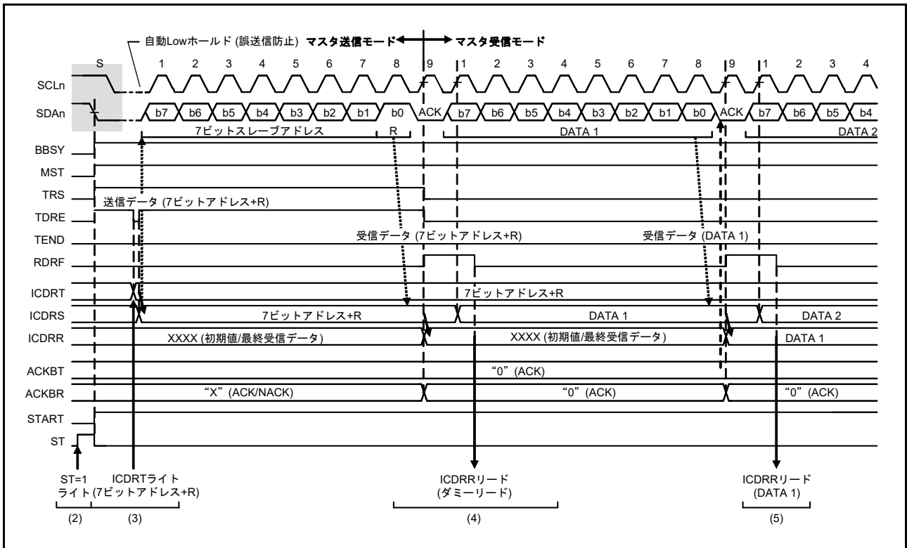
図 41.11 マスタ受信の動作タイミング (1) (7 ビットアドレスフォーマット、RDRFS ビット = 0 のとき)
