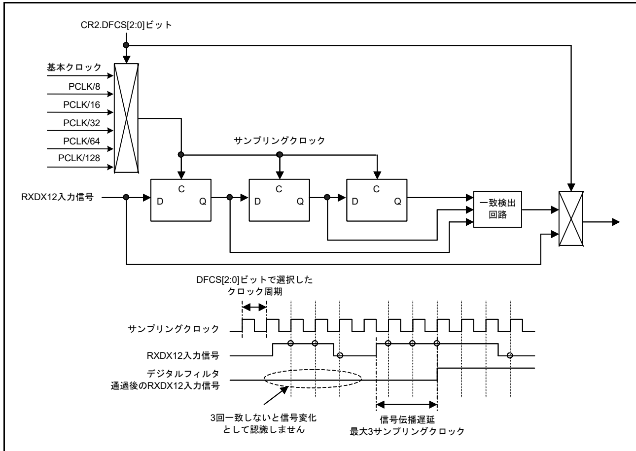
図 40.74 デジタルフィルタ機能の動作例
