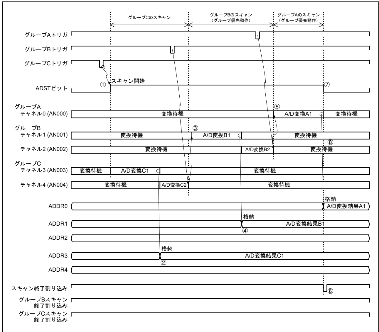
図 54.33 グループ優先動作の例 4 「低優先グループスキャン中の優先グループトリガ入力」再スキャンなし (ADGSPCR.GBRSCN = 0, ADGSPCR.GBRP = 0, ADGSPCR.LGRRS = 1 設定時)
