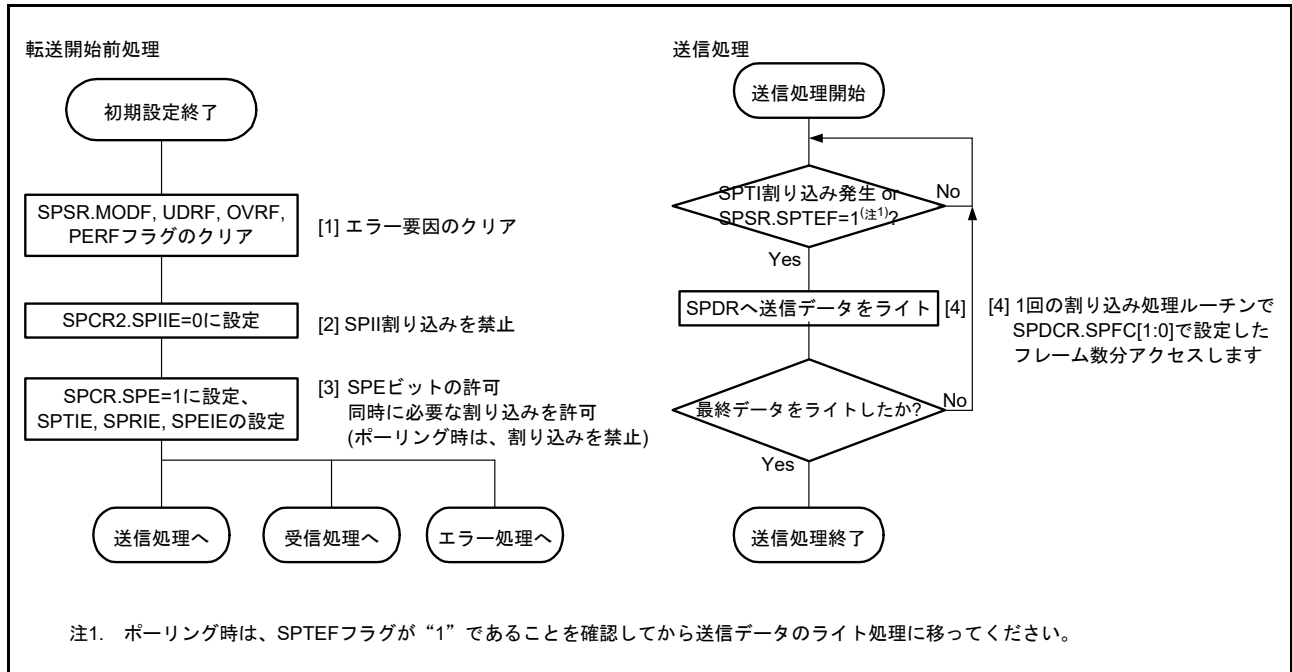
図 43.42 スレーブモード時のフローチャート (送信)
