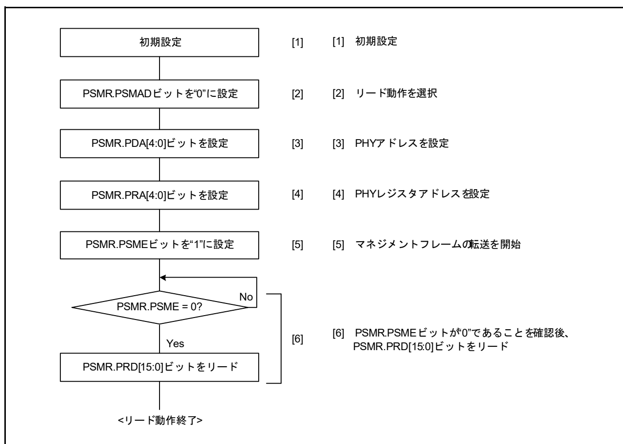
図 38.5 PHYレジスタリードのフローチャート例
