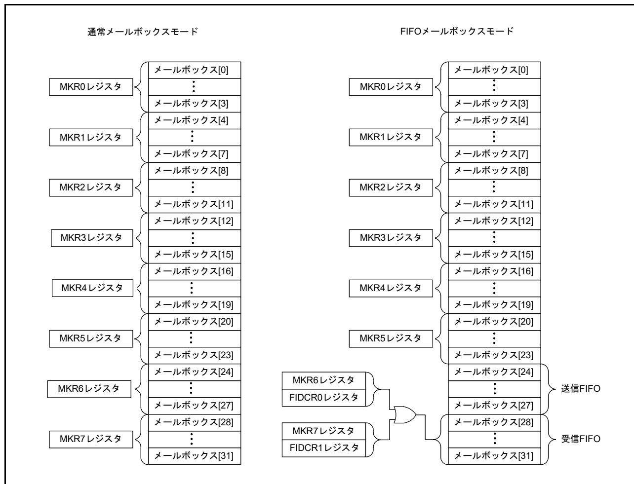
図 42.16 マスクレジスタとメールボックスの対応
