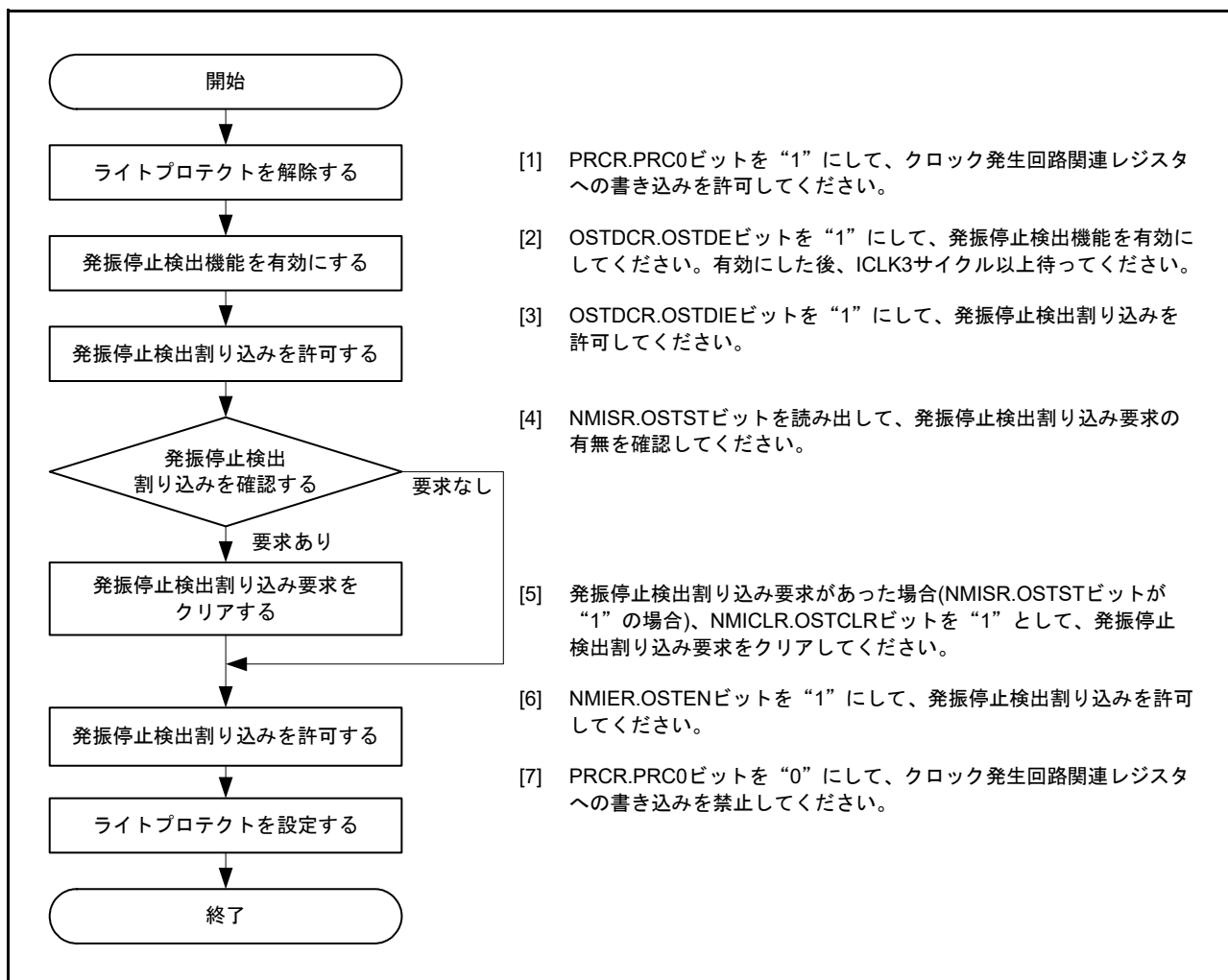
図 9.8 発振停止検出機能の初期化手順のフローチャート例
