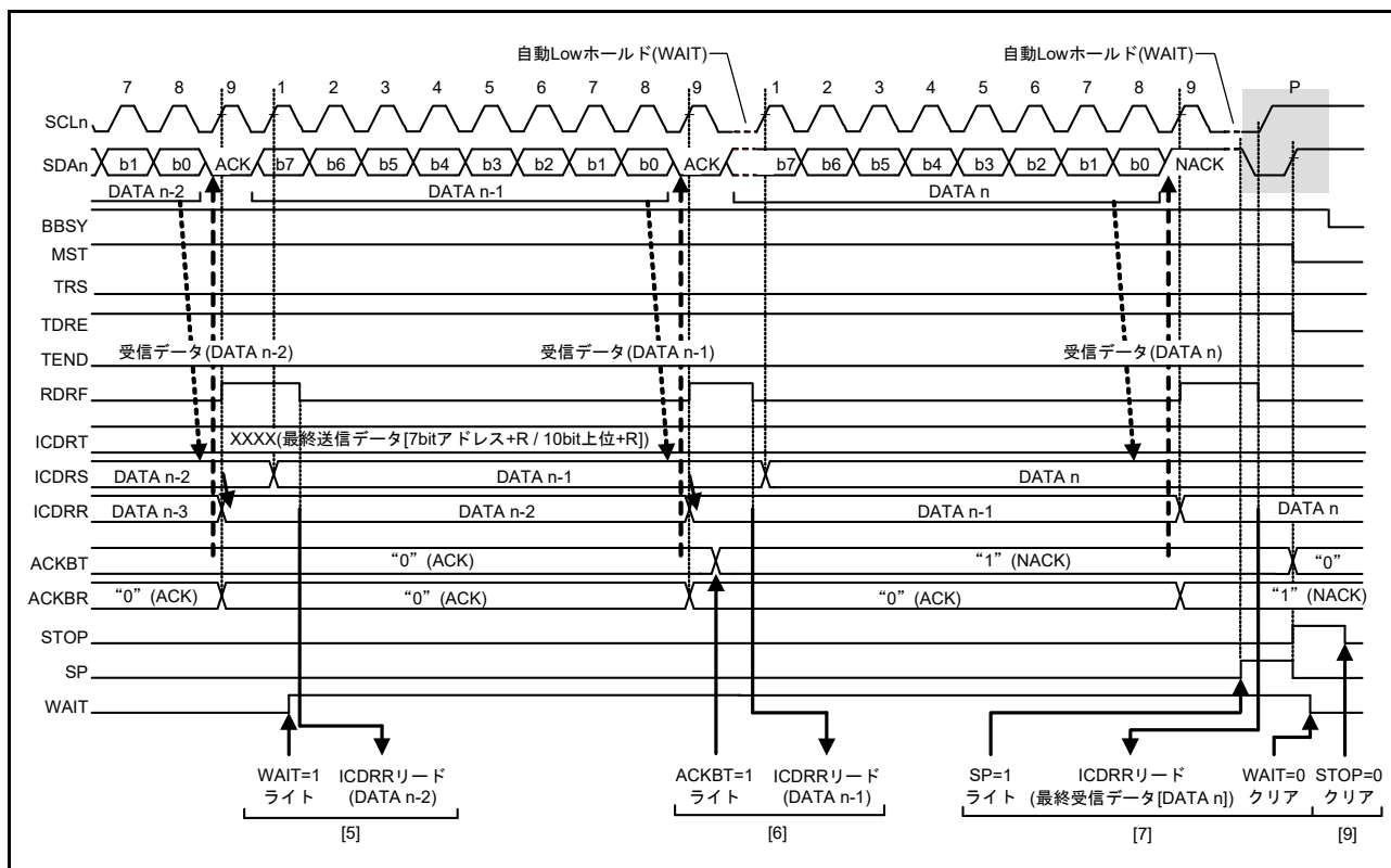
図 41.13 マスタ受信の動作タイミング (3) (RDRFS ビット = 0 のとき)
