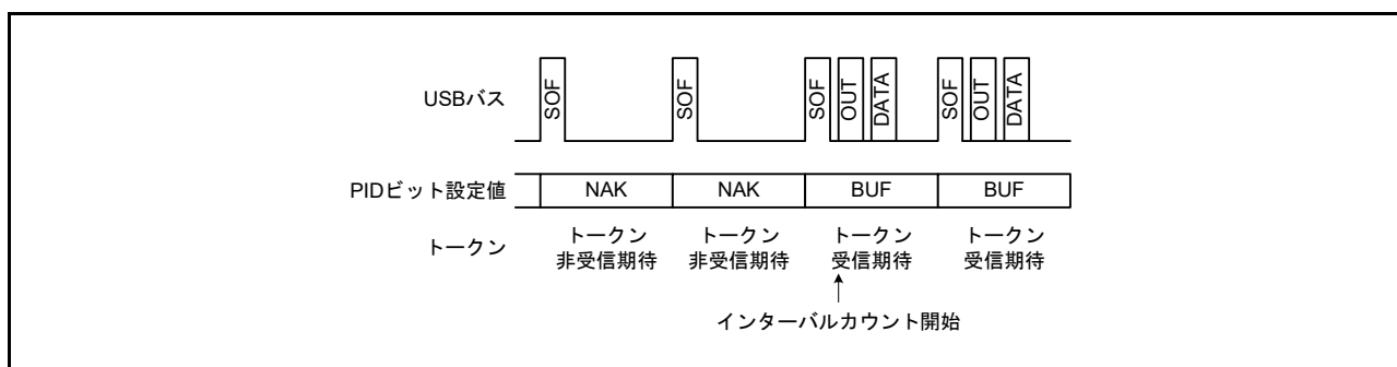
図 39.18 IITV[2:0] = 000b の場合のフレームとトークン受信期待有無の関係
