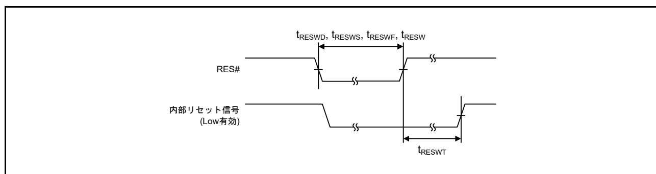
図 61.2 リセット入力タイミング
