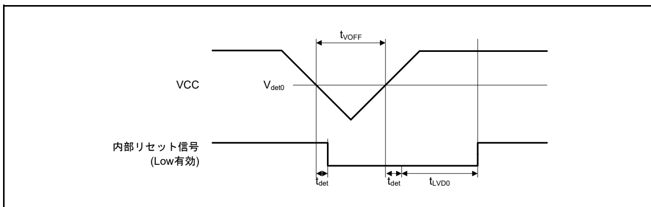
図 61.103 電圧検出回路タイミング (V det0 )
