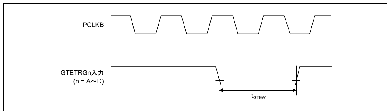
図 61.53 GPTW 外部トリガ入力タイミング
