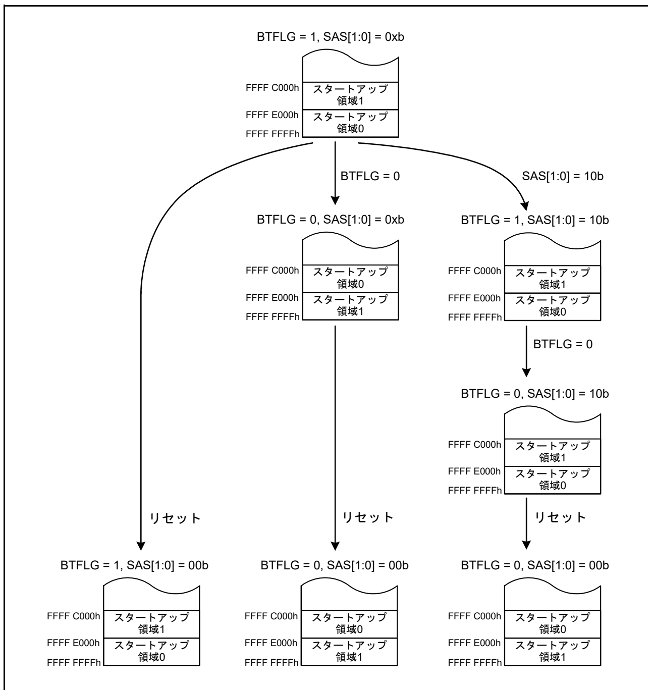
図 60.27 スタートアッププログラム保護機能の設定遷移例 1
