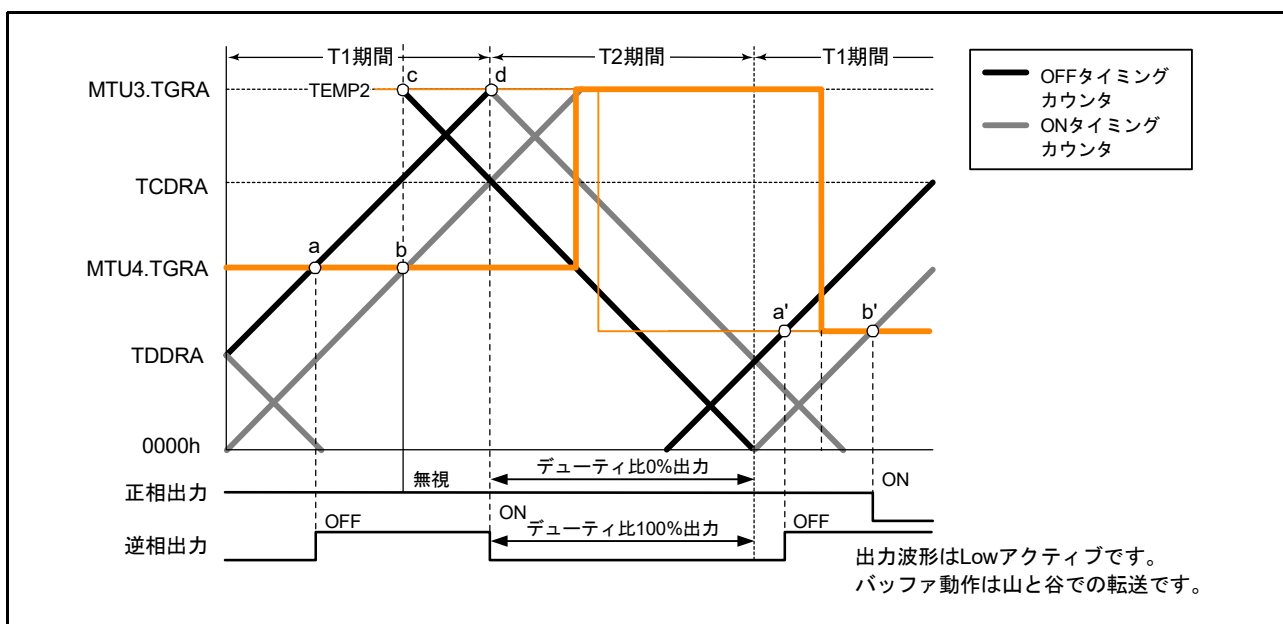
図 24.59 相補 PWM モード 0%、100% 波形出力例 (MTU3, MTU4) (1)
