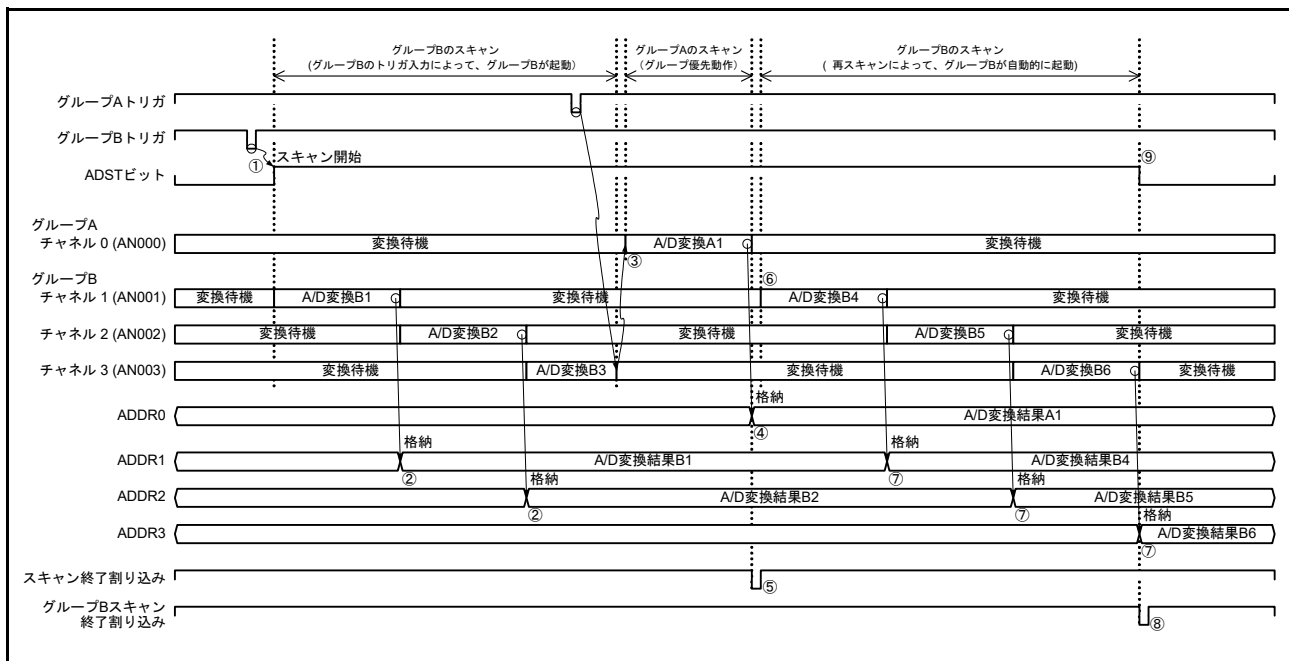
図 54.25 グループ優先動作の例 1 「グループ B スキャン中のグループ A トリガ入力」再スキャンあり (ADGSPCR.GBRSCN = 1, ADGSPCR.GBRP = 0, ADGSPCR.LGRRS = 0 設定時)
