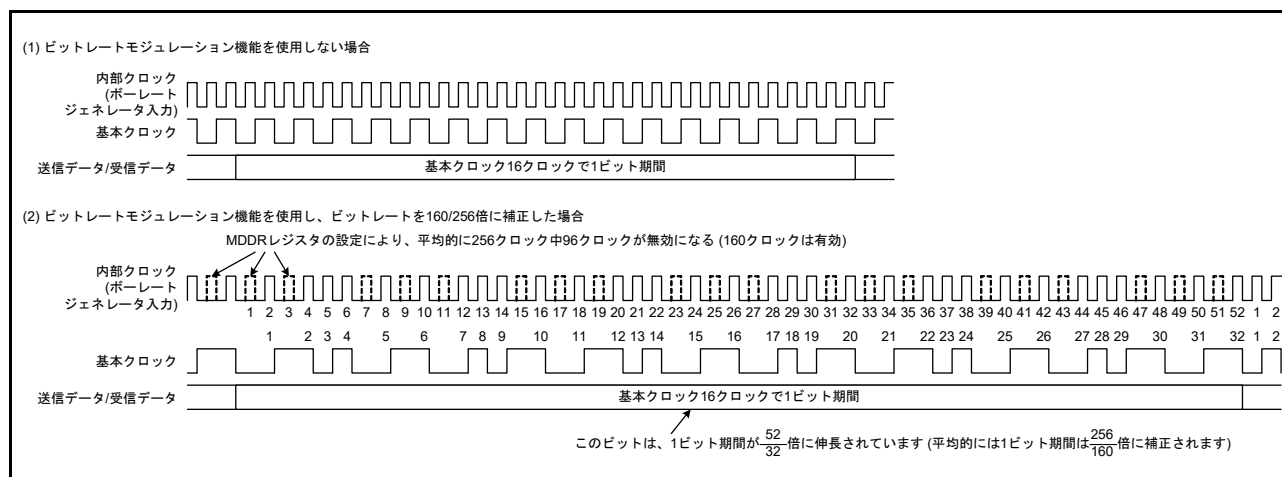
図 40.63 ビットレートモジュレーション機能使用時の基本クロックの例
