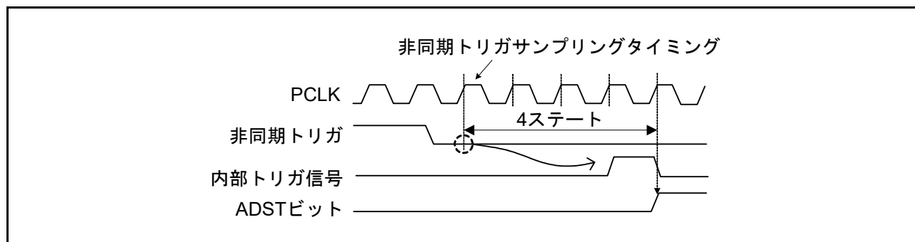
図 54.44 非同期トリガ入力タイミング
