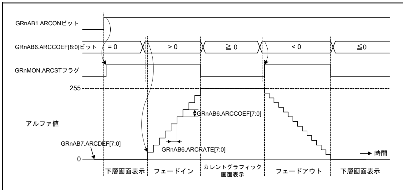
図 50.10 アルファ値の更新 (n = 1, 2)
