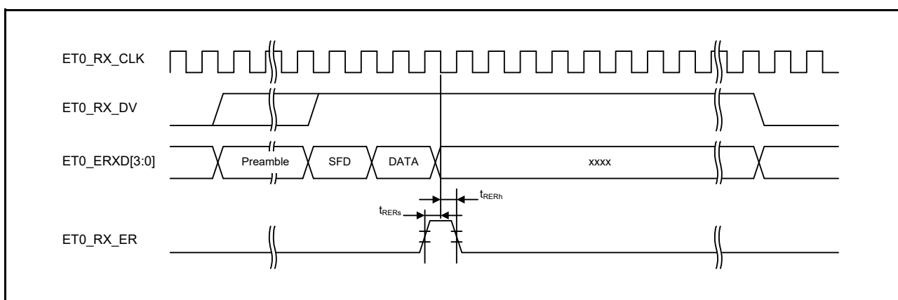
図 61.89 MII 受信タイミング (エラー発生ケース)
