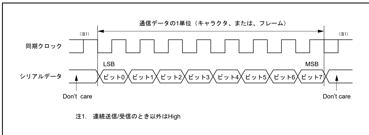
図 40.27 クロック同期式シリアル通信のデータフォーマット (LSB ファーストの場合)
