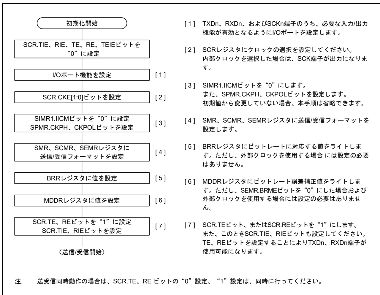
図 40.28 SCIの初期化フローチャートの例(クロック同期式モード)
