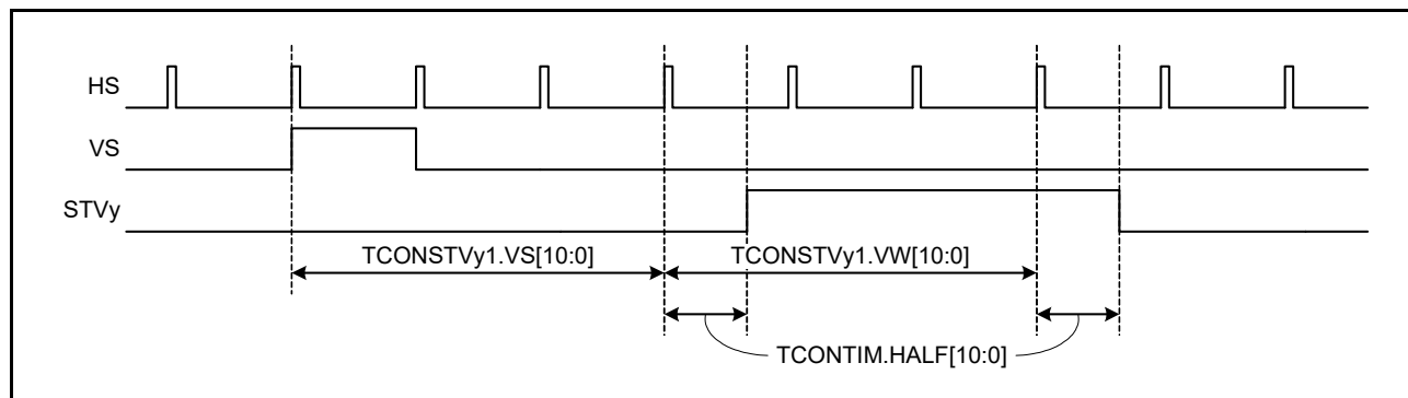
図 50.17 STVy 信号の生成 (y = A, B)
