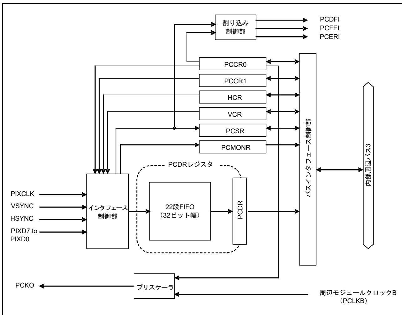
図 49.1 PDC のブロック図
