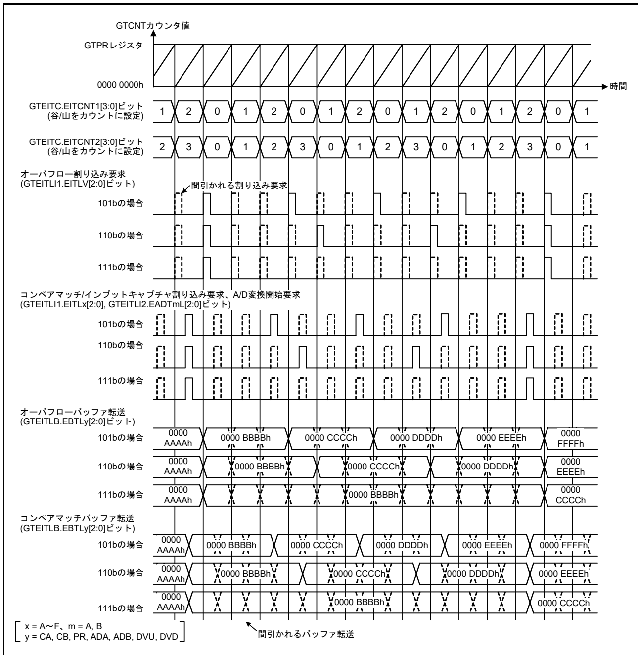
図 26.112 拡張割り込み間引き機能の動作例
