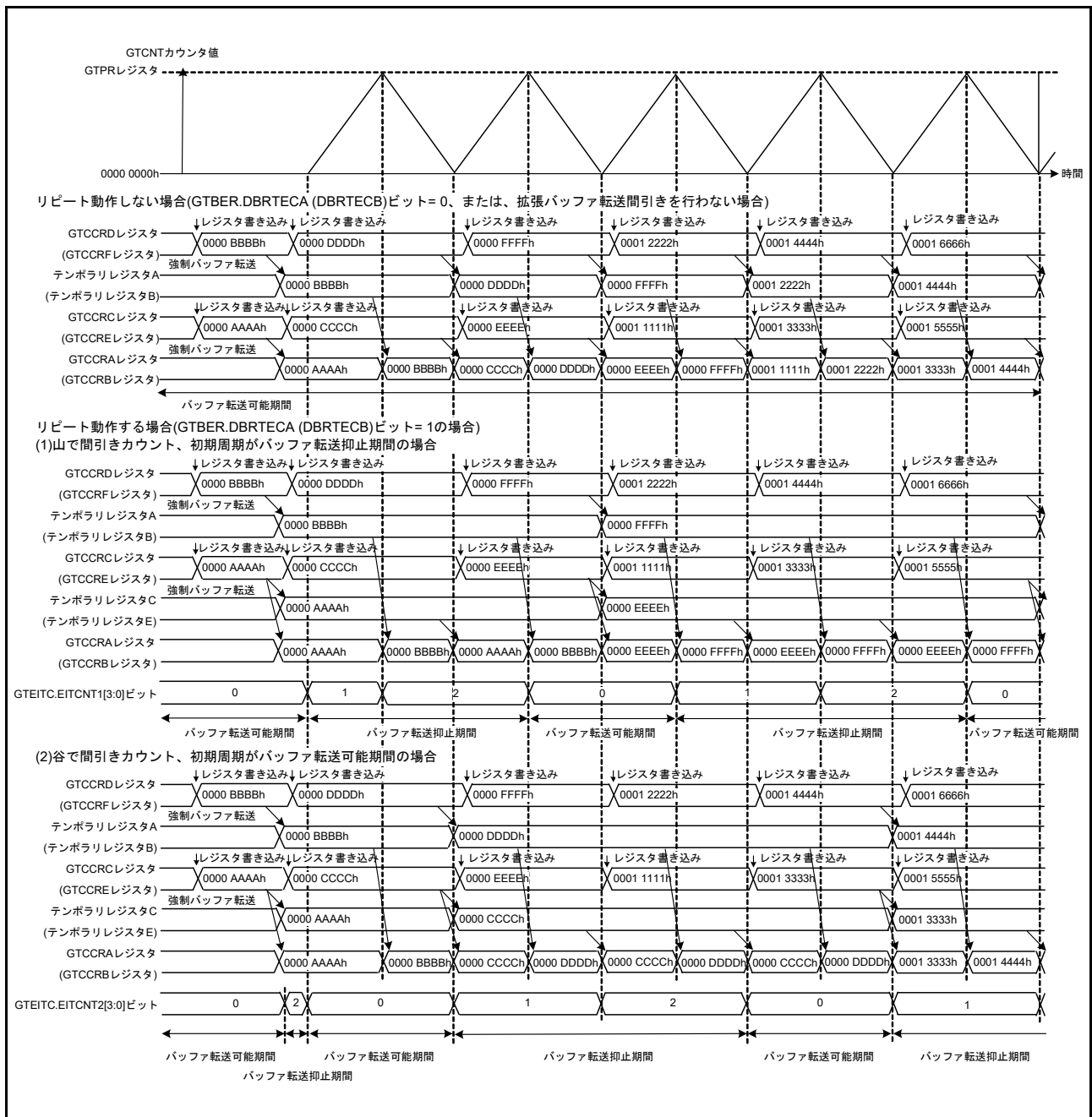
図 26.123 GTCCR バッファ転送抑止時ダブルバッファリピート動作例 (三角波 PWM モード 3、拡張バッファ転送間引き使用、GTBER.BD[0] ビットは常時 "0" の場合)
