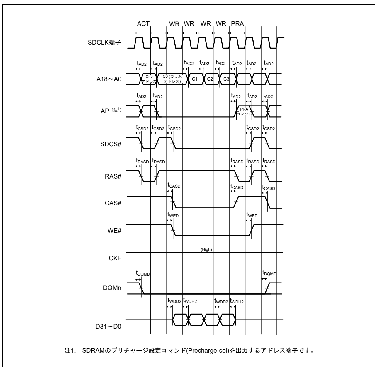
図 61.28 SDRAM 空間複数ライトバスタイミング
