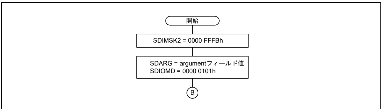
図 47.19 IO_RW_EXTENDED コマンド (CMD53) のシーケンス中に SDIO abort (CMD52) を送信する例
