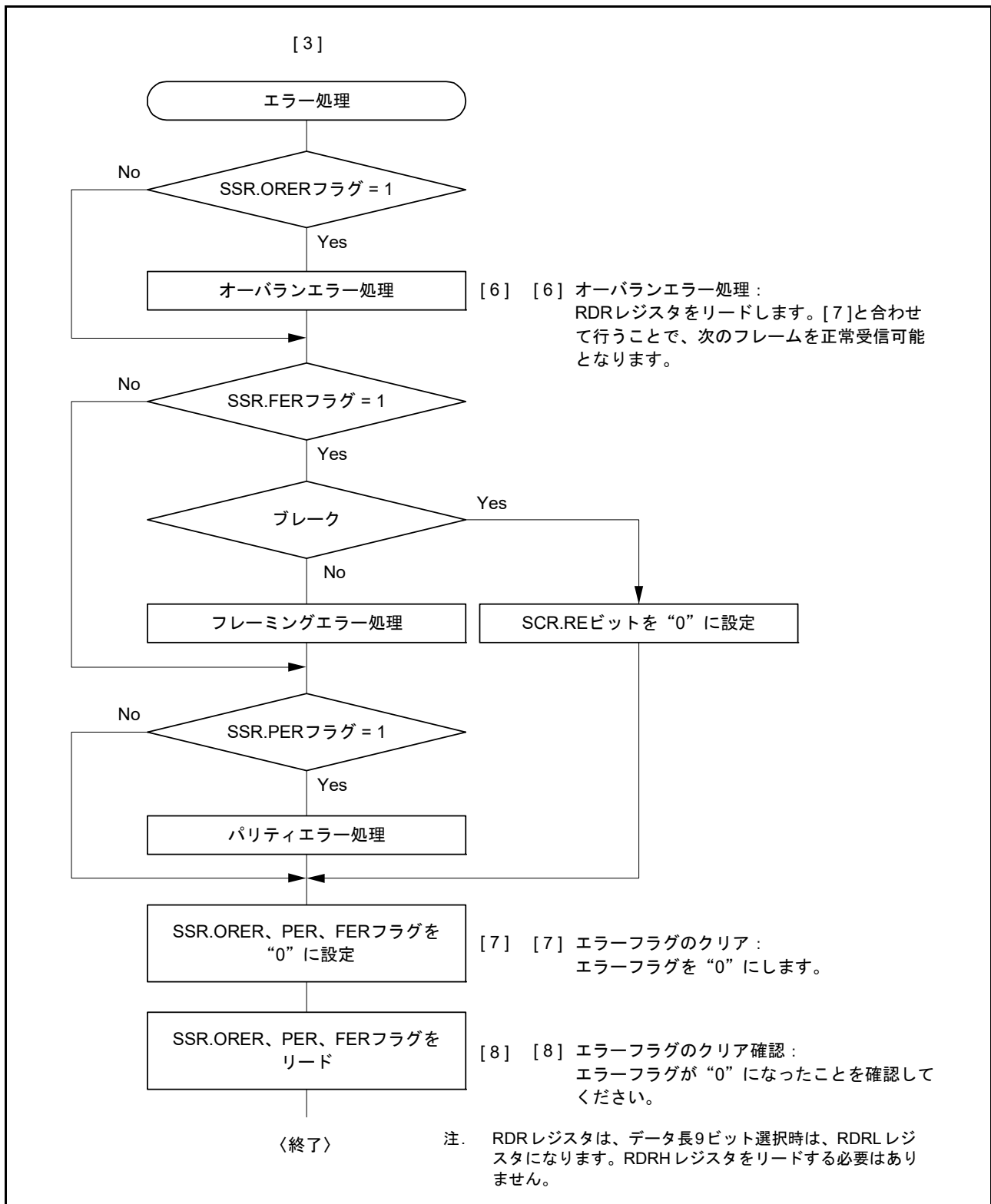
図 40.21 調歩同期式モードのシリアル受信のフローチャート例 (2)
