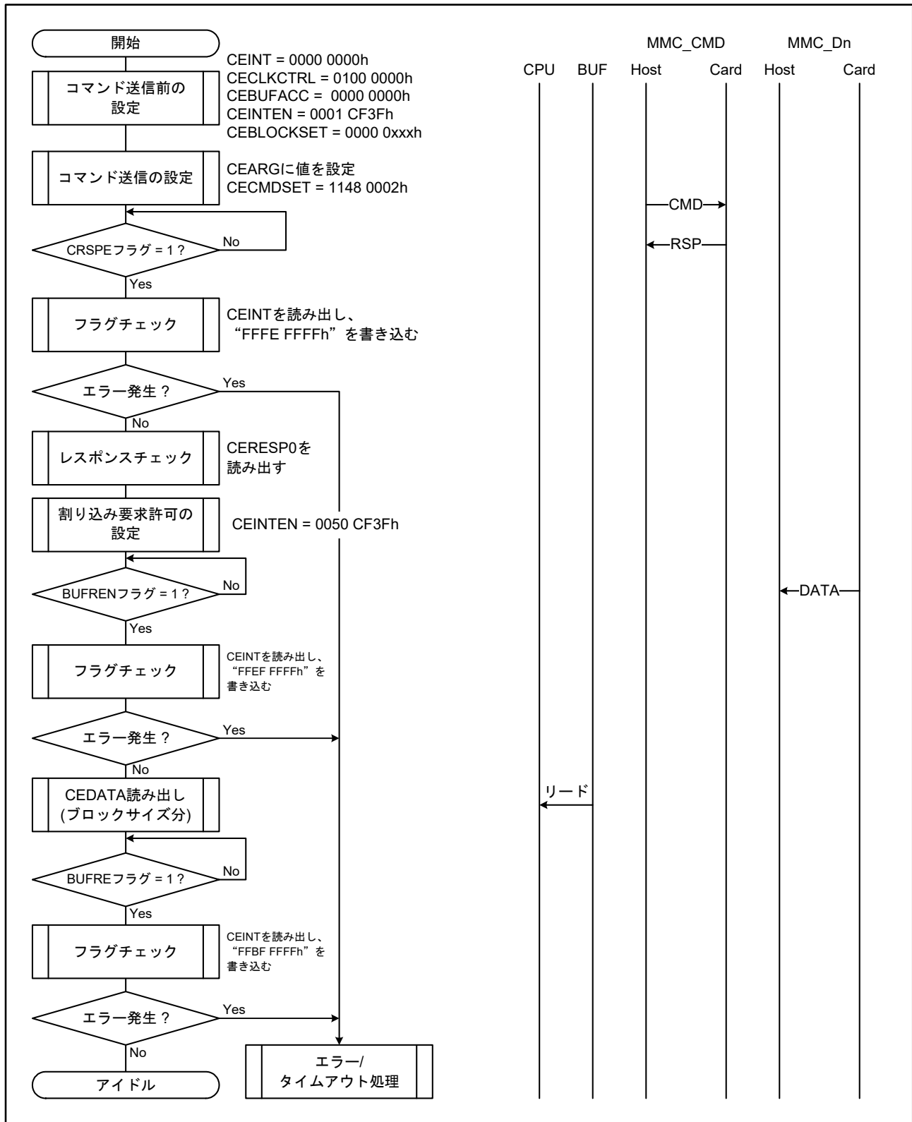
図 48.15 シングルブロックリードコマンドの送信例 (CMD17)
