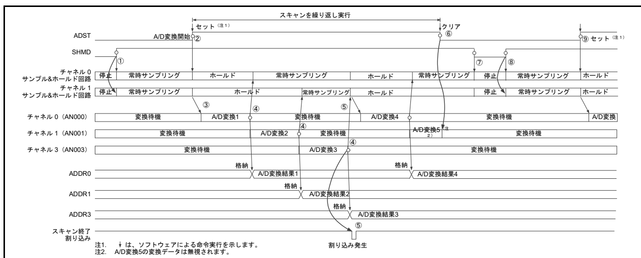
図 54.17 連続スキャンモードの動作例 (チャンネル専用サンプル & ホールド回路使用 : AN000, AN001, AN003 選択、常時サンプリング有効)
