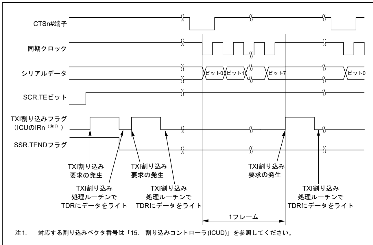
図 40.30 クロック同期式モードのシリアル送信の動作例 (2) (送信開始・CTS 機能使用する)
