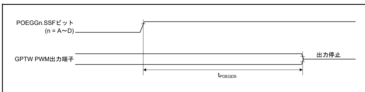
図 61.50 POEG 出力ディセーブル時間 (レジスタ設定)
