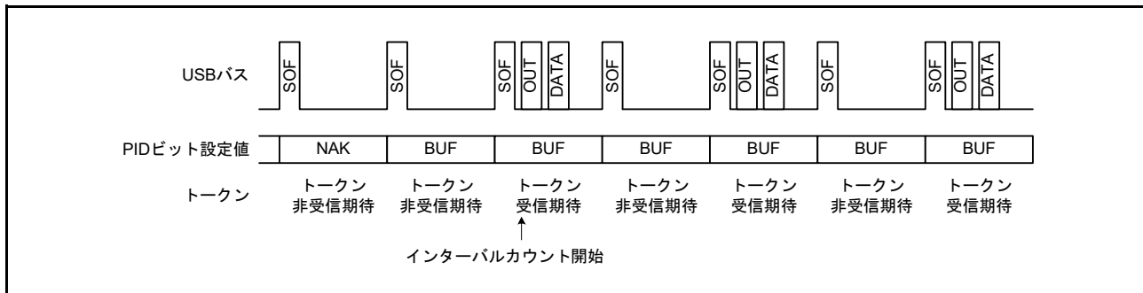
図 39.19 IITV[2:0] = 000b 以外の場合のフレームとトークン受信期待有無の関係
