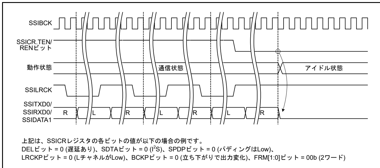
図 46.21 通信状態とアイドル状態への遷移
