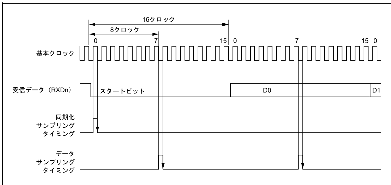
図 40.7 調歩同期式モードの受信データサンプリングタイミング
