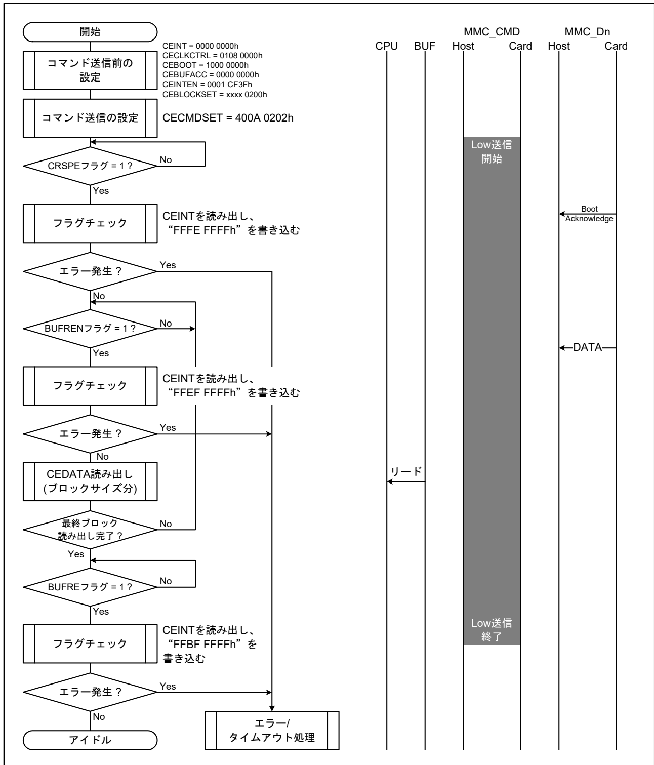
図 48.21 Boot Operation 例 (Boot Acknowledge あり)
