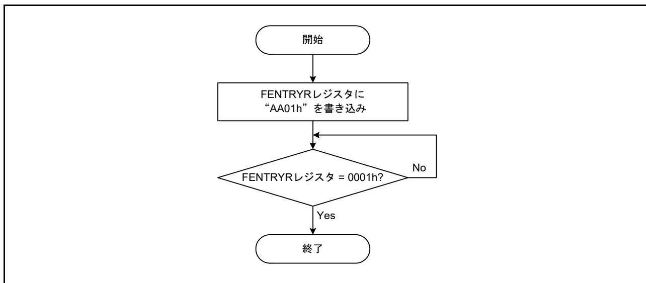
図 60.9 コードフラッシュメモリ P/E モード移行フロー
