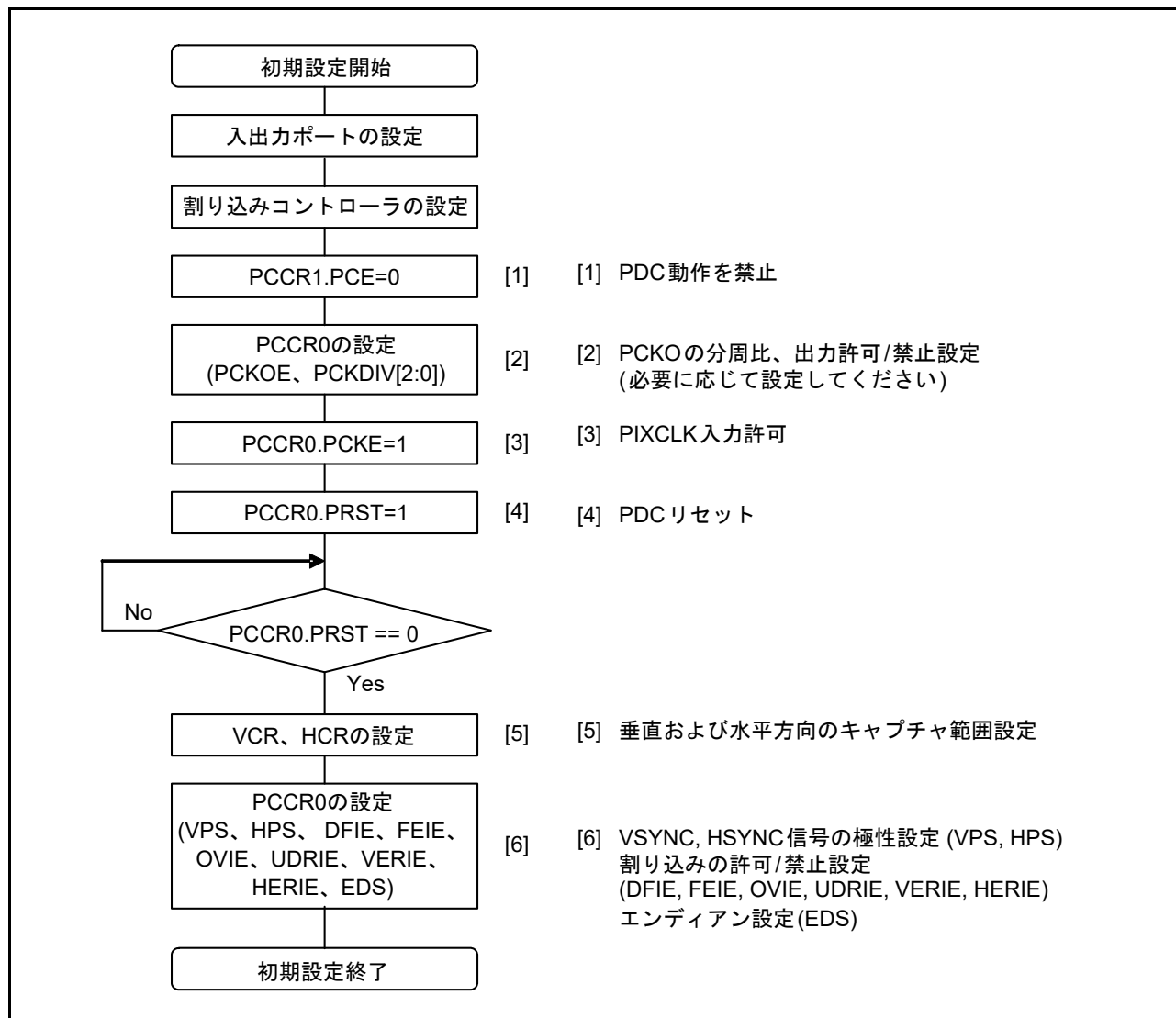
図 49.18 PDC の初期化フロー例
