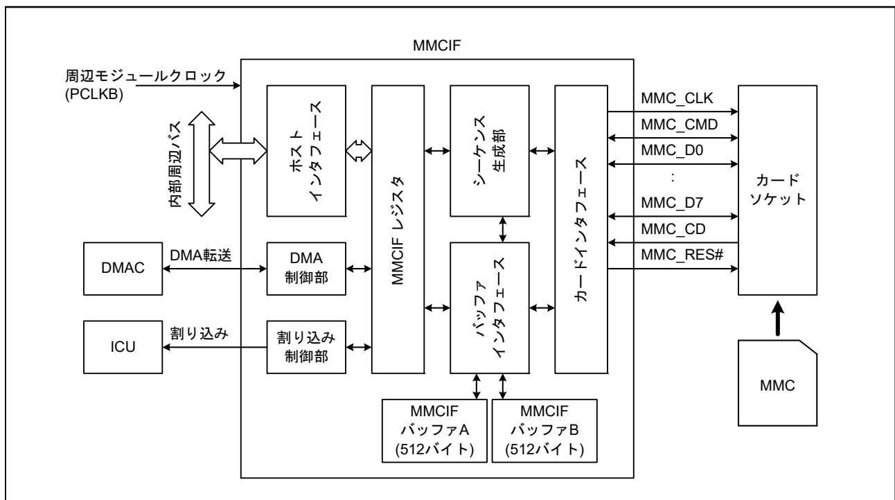
図 48.1 MMCIF のブロック図
