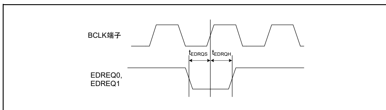
図 61.32 EDREQ0、EDREQ1 入力タイミング
