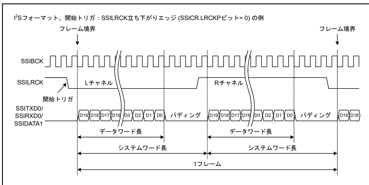
図 46.1 データフォーマットに関する用語の定義
