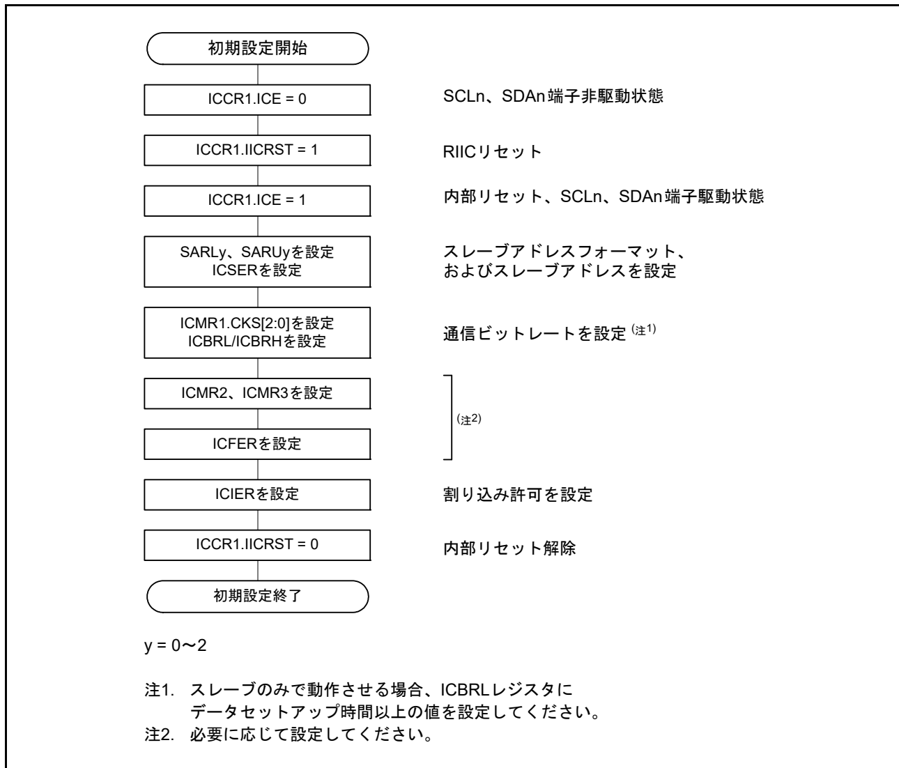
図 41.4 RIIC の初期化フローチャート例
