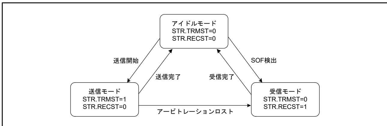
図 42.10 CAN オペレーションモードのサブモード
