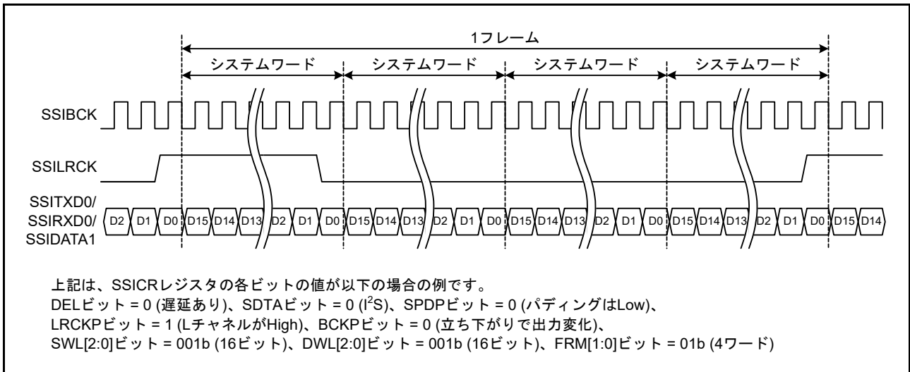
図 46.15 TDM フォーマットの例 (1) (SSICR.DEL ビット = 0、パディングなし)
