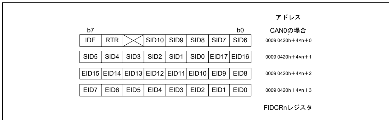
図 42.15 FIDCRn レジスタの構成 (n = 0, 1)
