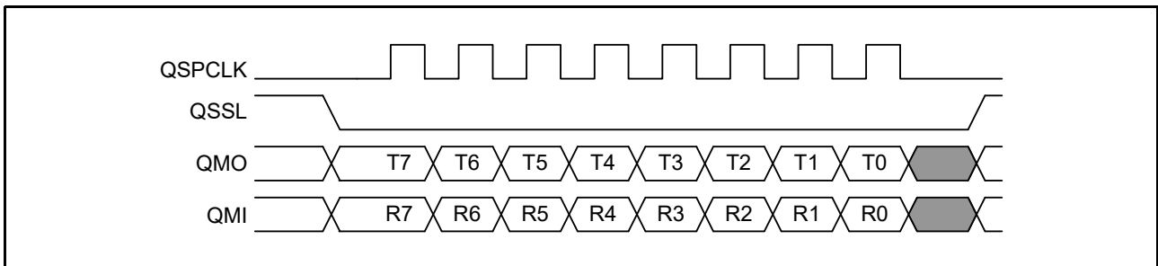
図 44.3 Single-SPI モード転送フォーマット
