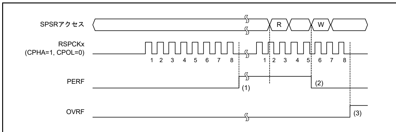
図 43.32 PERF フラグの動作例
