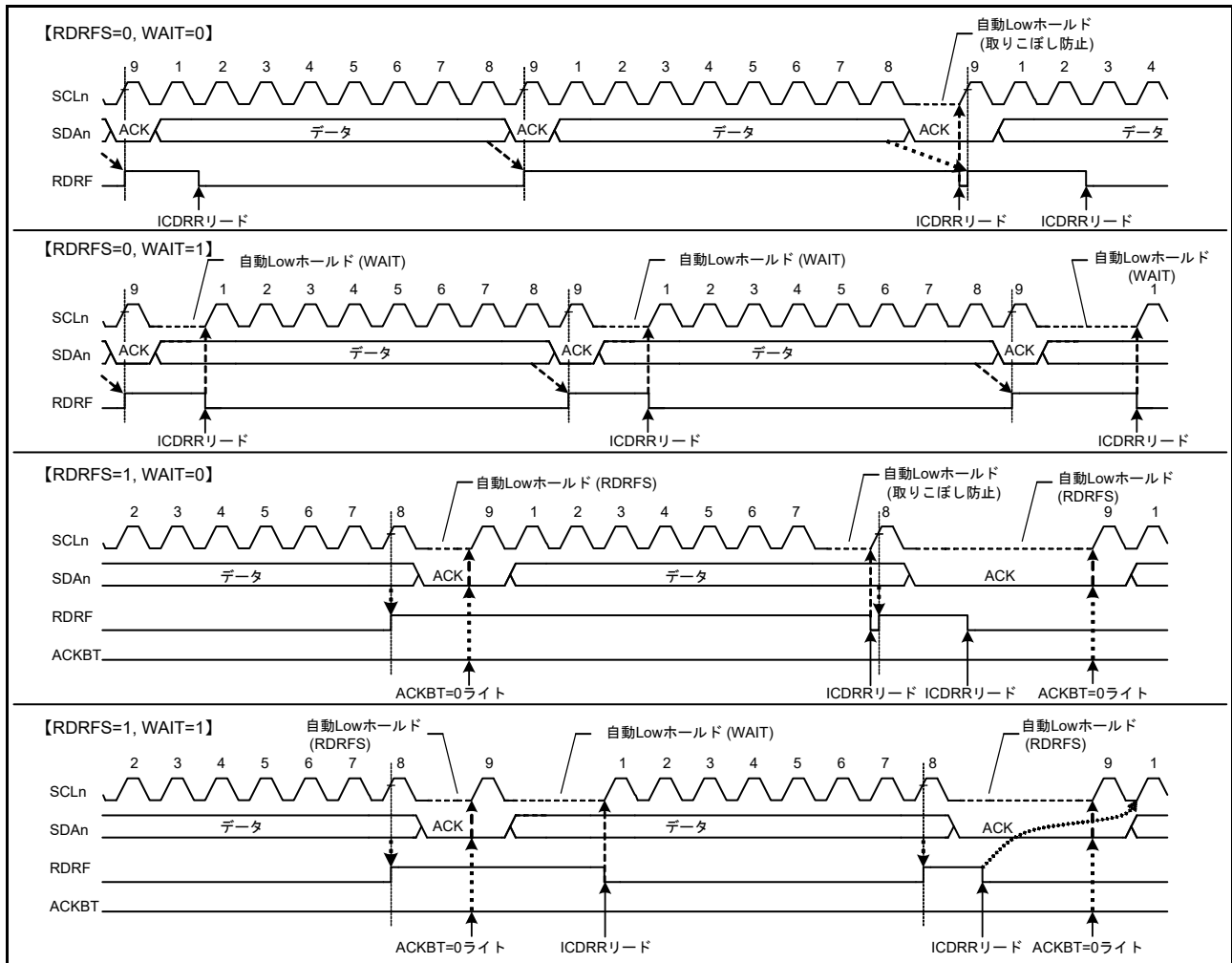
図 41.31 受信モードの自動 Low ホールド動作 (RDRFS、WAIT ビット)
