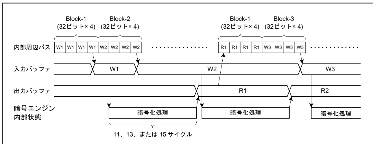
図 53.6 AES 暗号 / 復号処理タイミング図
