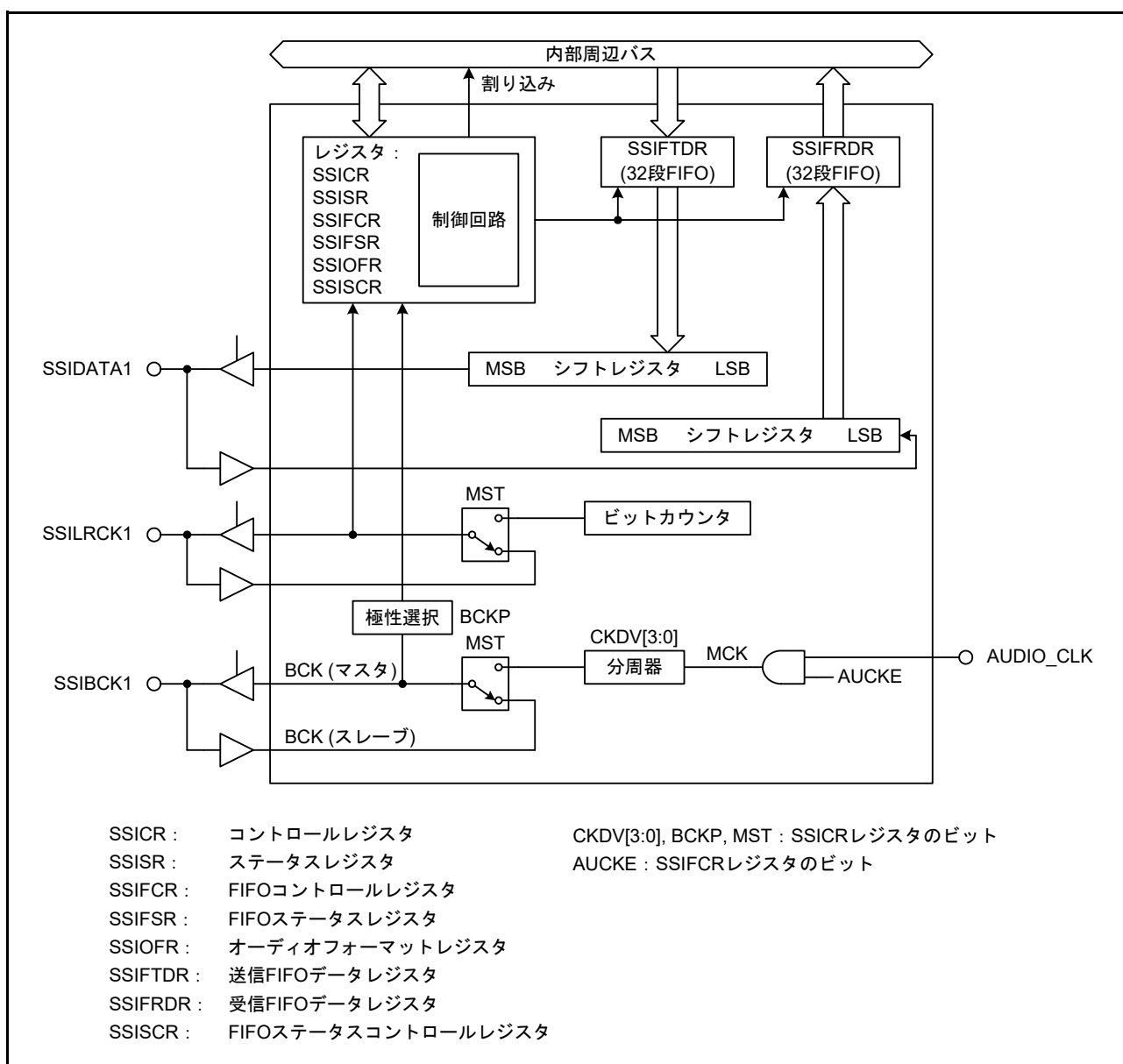
図 46.3 SSIE1 ブロック図
