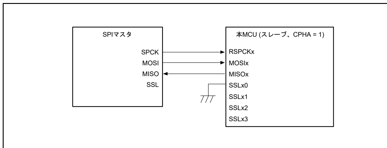
図 43.7 シングルマスタ / シングルスレーブの構成例 (本 MCU = スレーブ、CPHA = 1)
