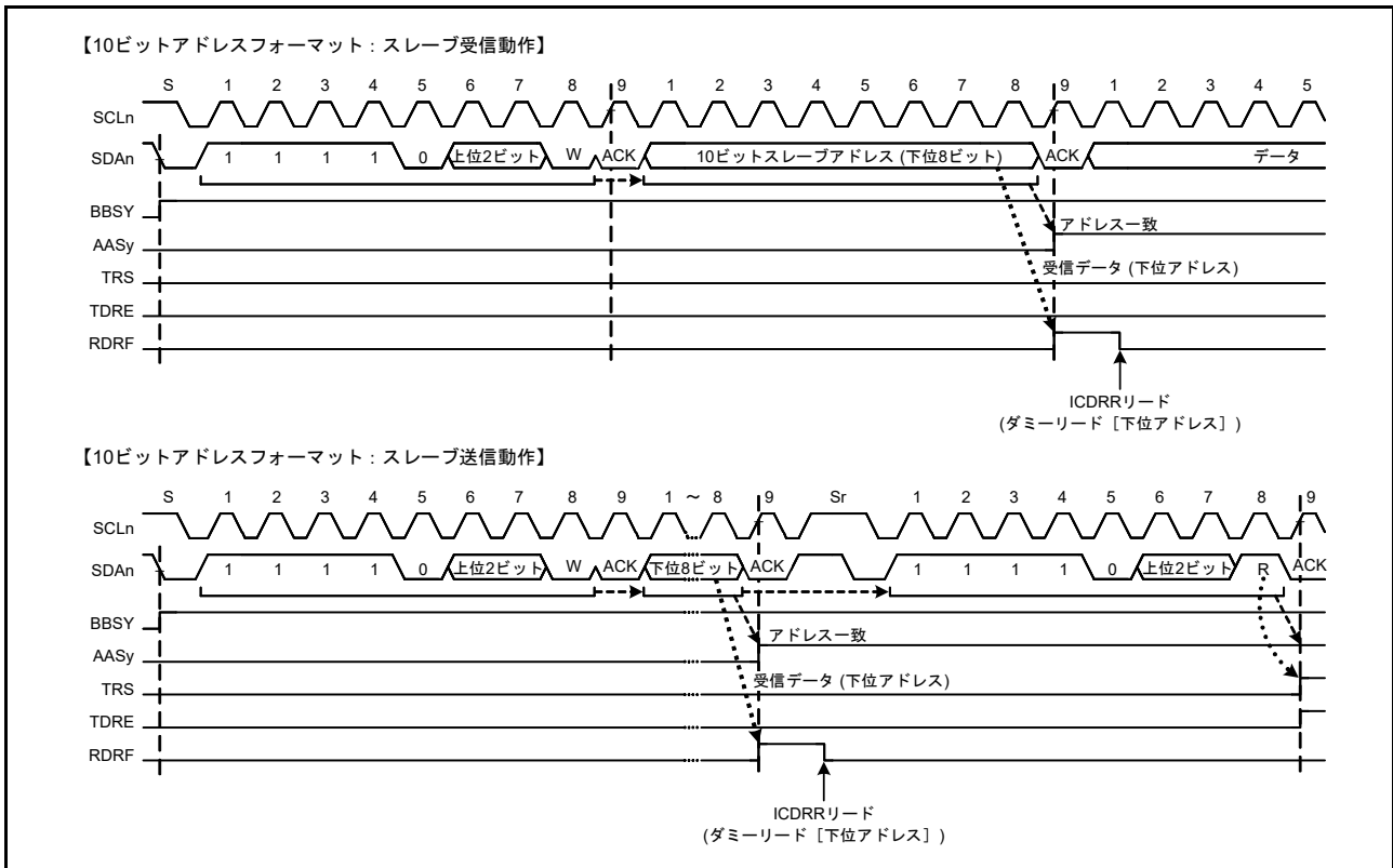
図 41.24 10 ビットアドレスフォーマット選択時に AASy フラグが“1”になるタイミング
