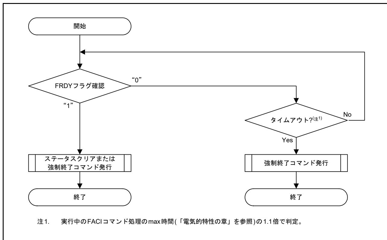
図 60.13 コマンドロック状態からの復帰方法
