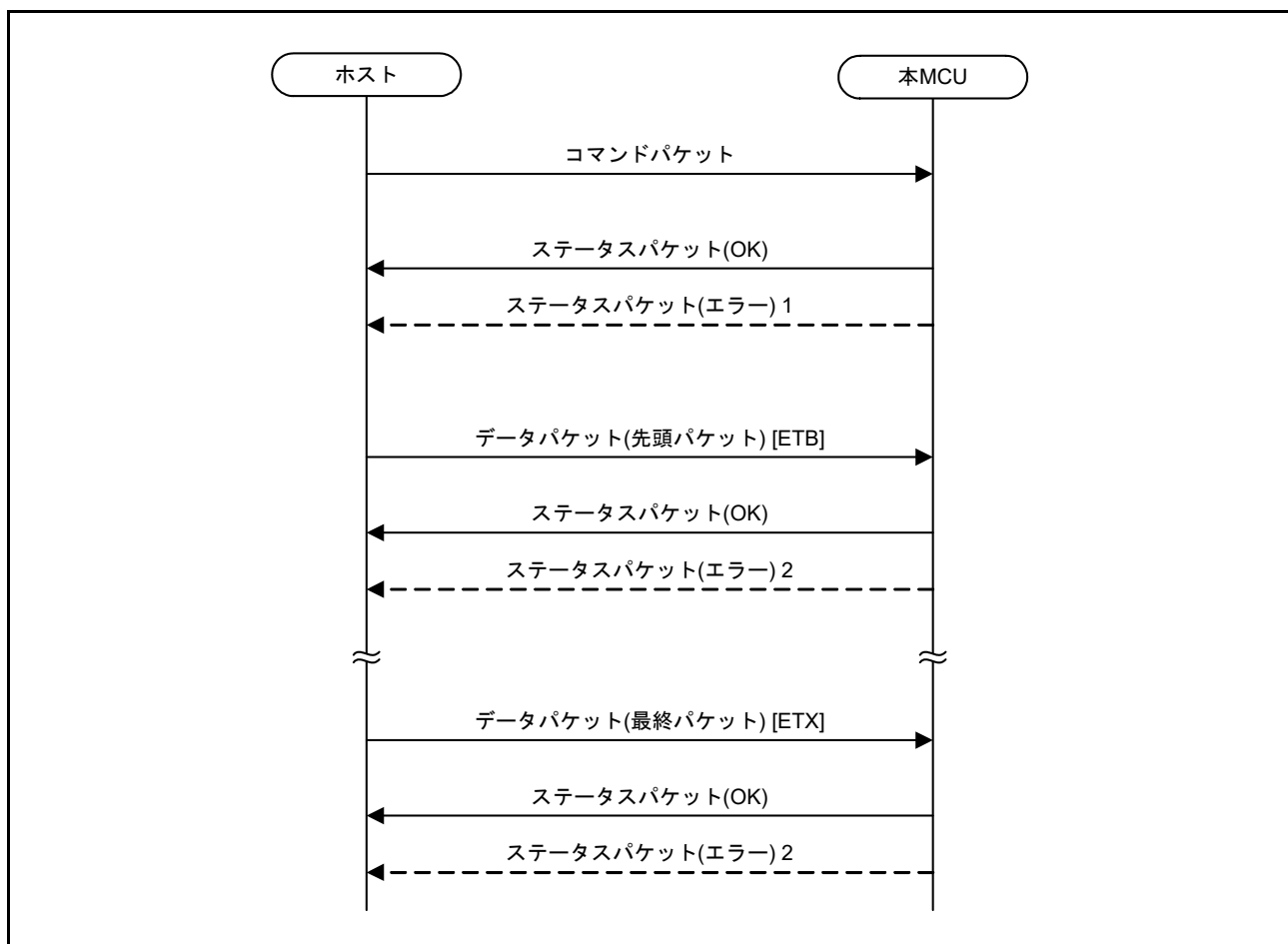
図 60.48 プログラムコマンドの通信シーケンス
