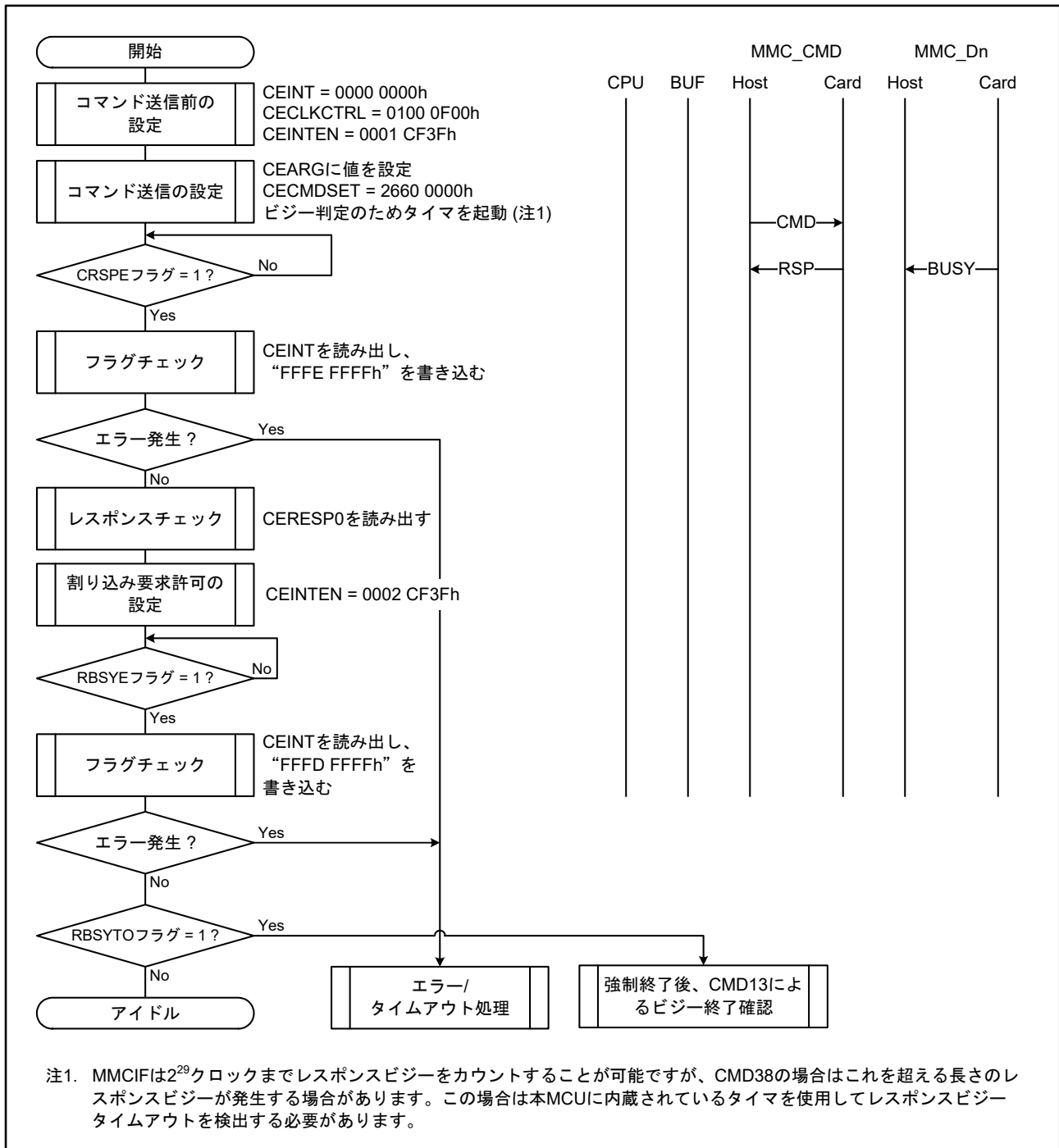
図 48.14 データ転送を行わないコマンド ( レスポンスビジーあり ) の送信例 (CMD38)
