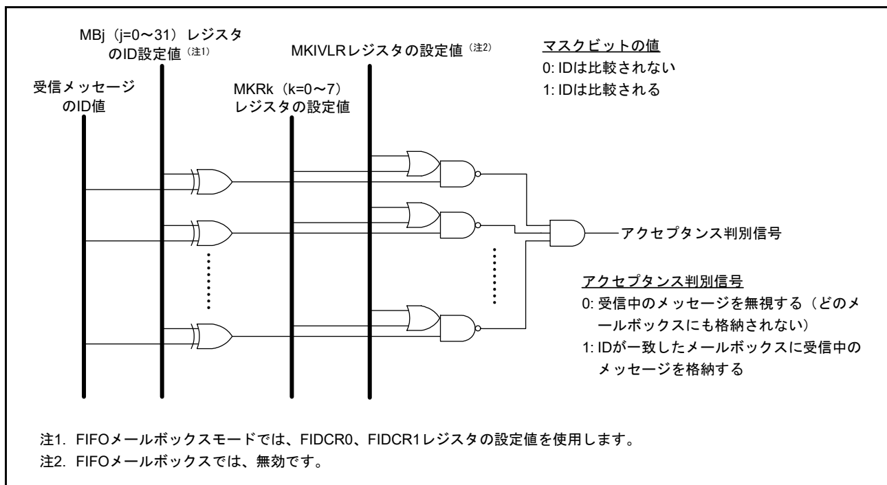
図 42.17 アクセプタンスフィルタ処理
