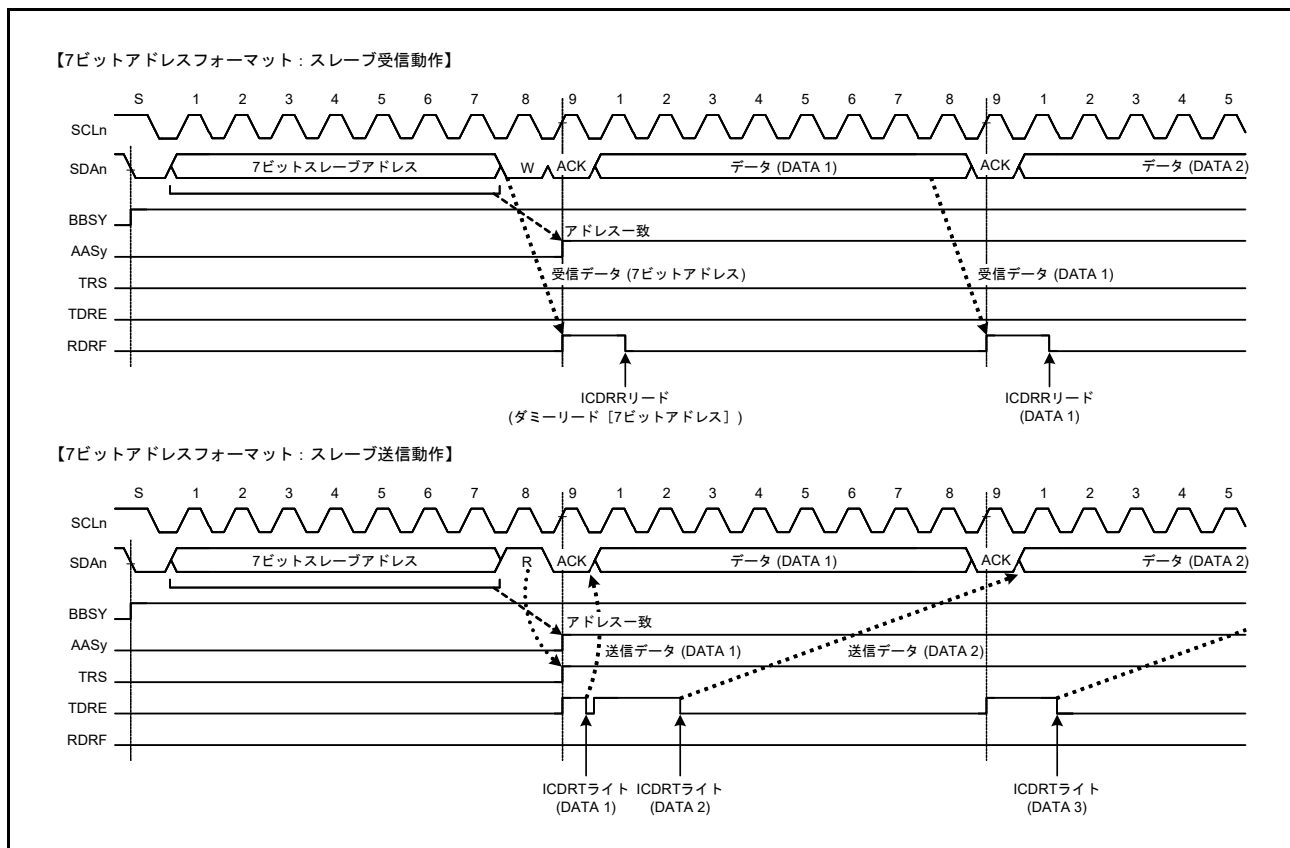
図 41.23 7 ビットアドレスフォーマット選択時に AASy フラグが“1”になるタイミング
