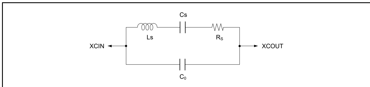
図 9.6 水晶振動子の等価回路
