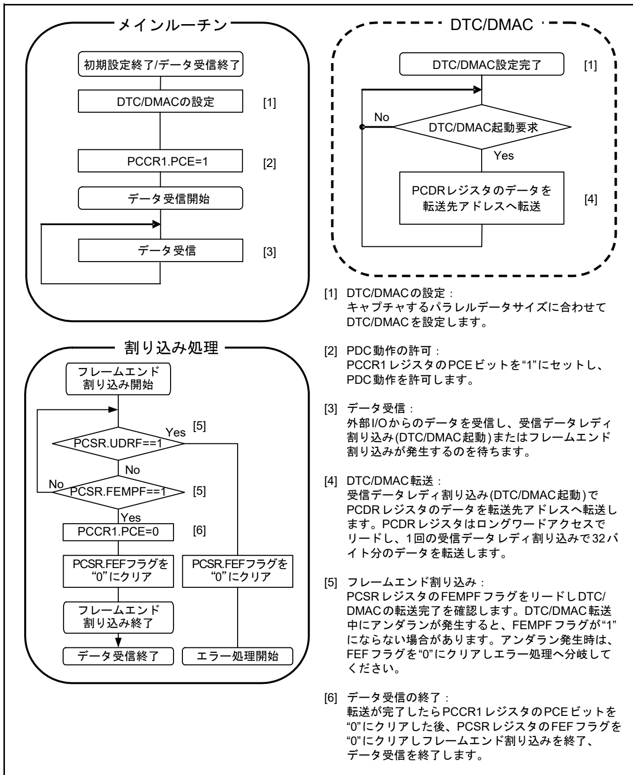
図 49.19 動作フロー例
