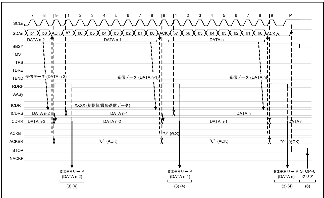
図 41.19 スレーブ受信の動作タイミング (2) (RDRFS ビット = 0 のとき)
