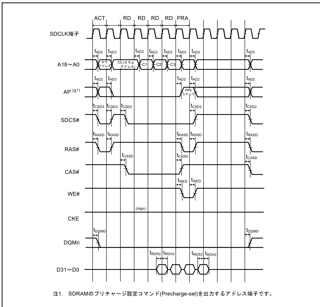
図 61.27 SDRAM 空間複数リードバスタイミング
