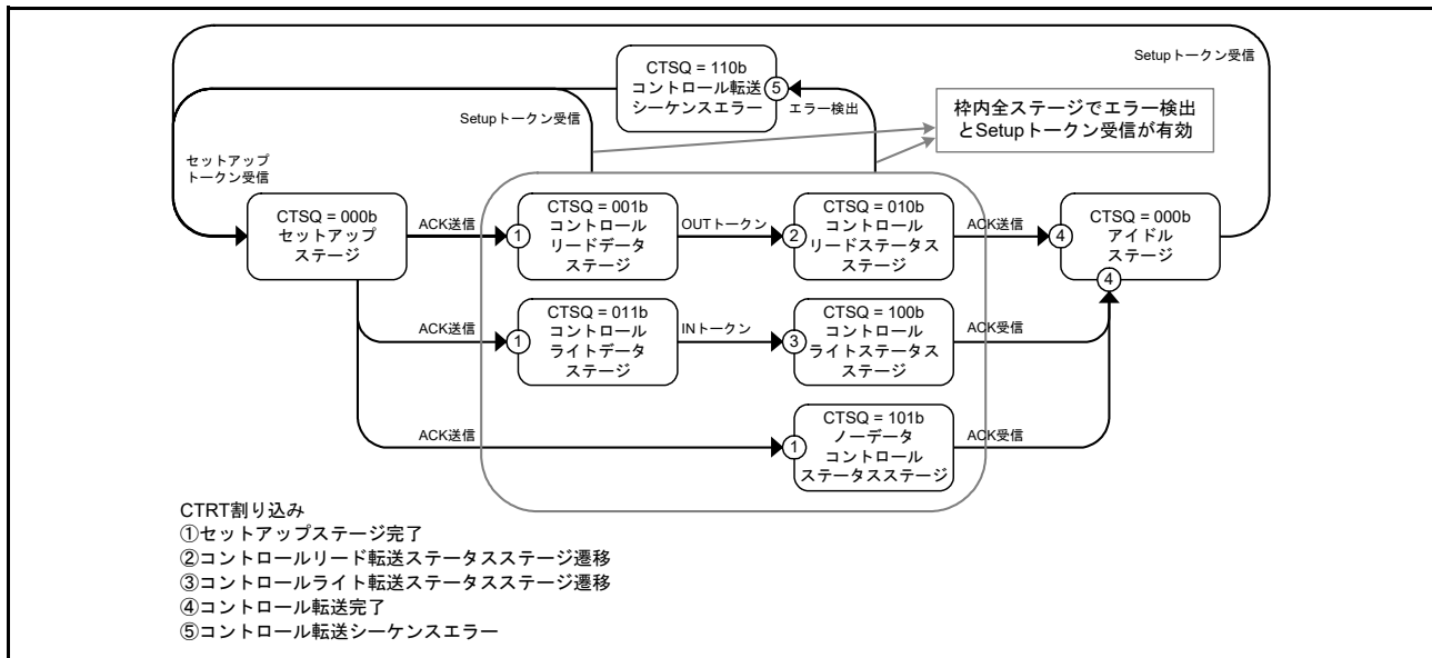
図 39.15 コントロール転送ステージ遷移図
