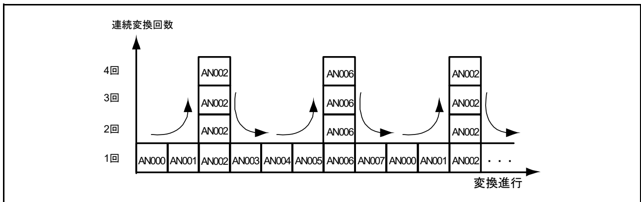
図 54.3 S12AD.ADADC.ADC[2:0] = 011b, S12AD.ADADC.AVEE = 0, S12AD.ADADS0.ADS002 = 1, S12AD.ADADS0.ADS006 = 1 選択時のスキャン変換シーケンス
