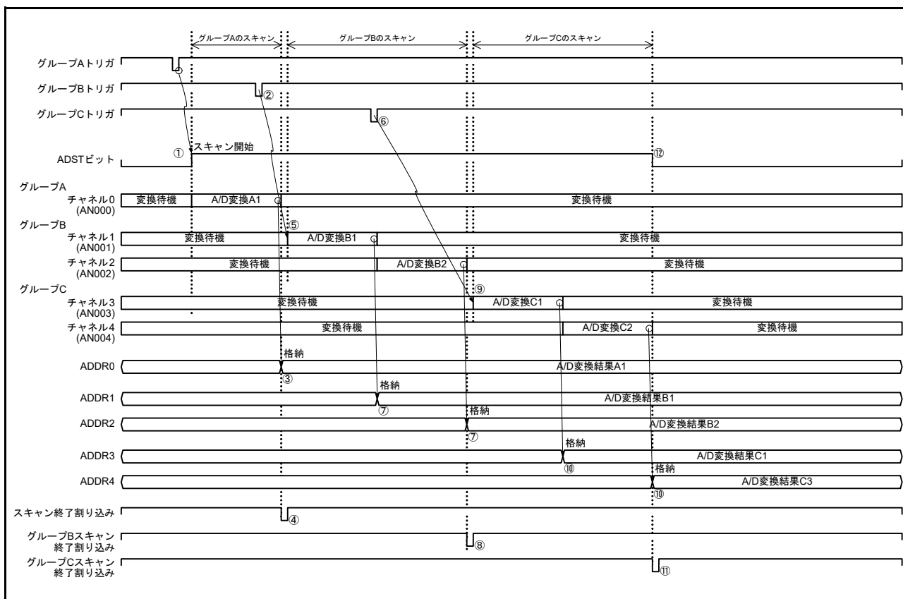
図 54.32 グループ優先動作の例 3 「優先グループスキャン中の低優先グループトリガ入力」再スキャンあり (ADGSPCR.GBRSCN = 1, ADGSPCR.GBRP = 0, ADGSPCR.LGRRS = 1, ADGCTRGR.GRCE = 1 時の動作)
