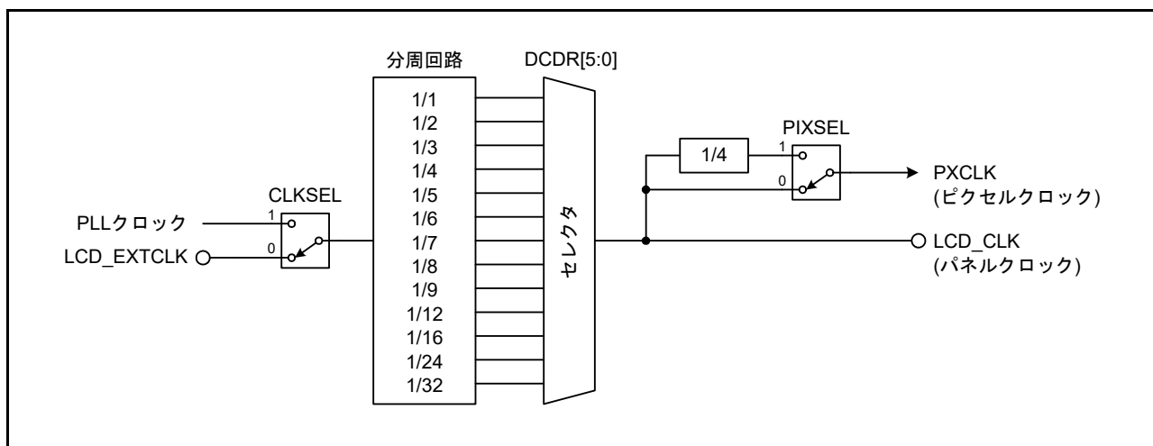
図 50.19 クロック生成部の構成
