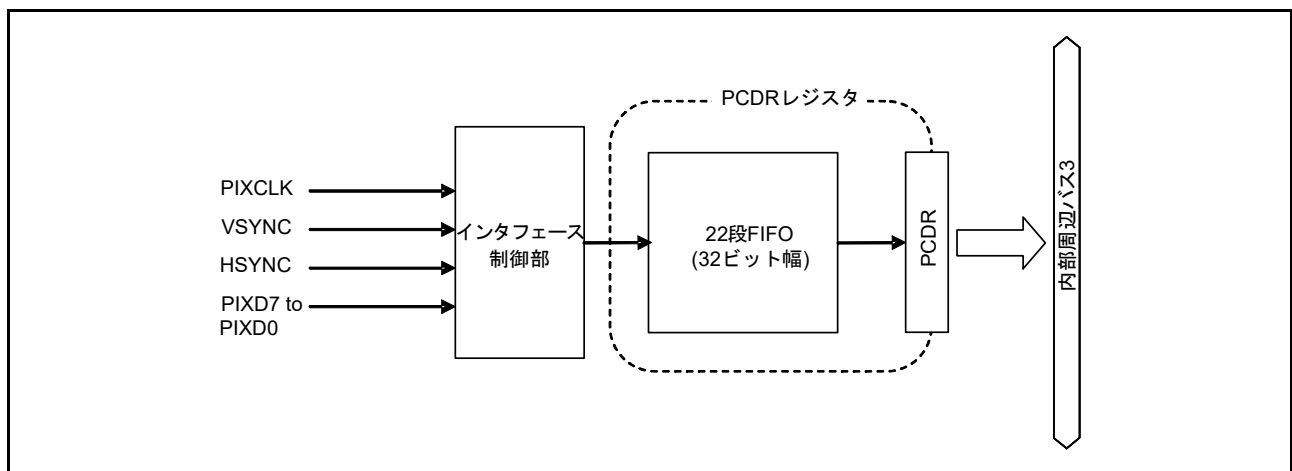
図 49.2 PCDR レジスタの構造図
