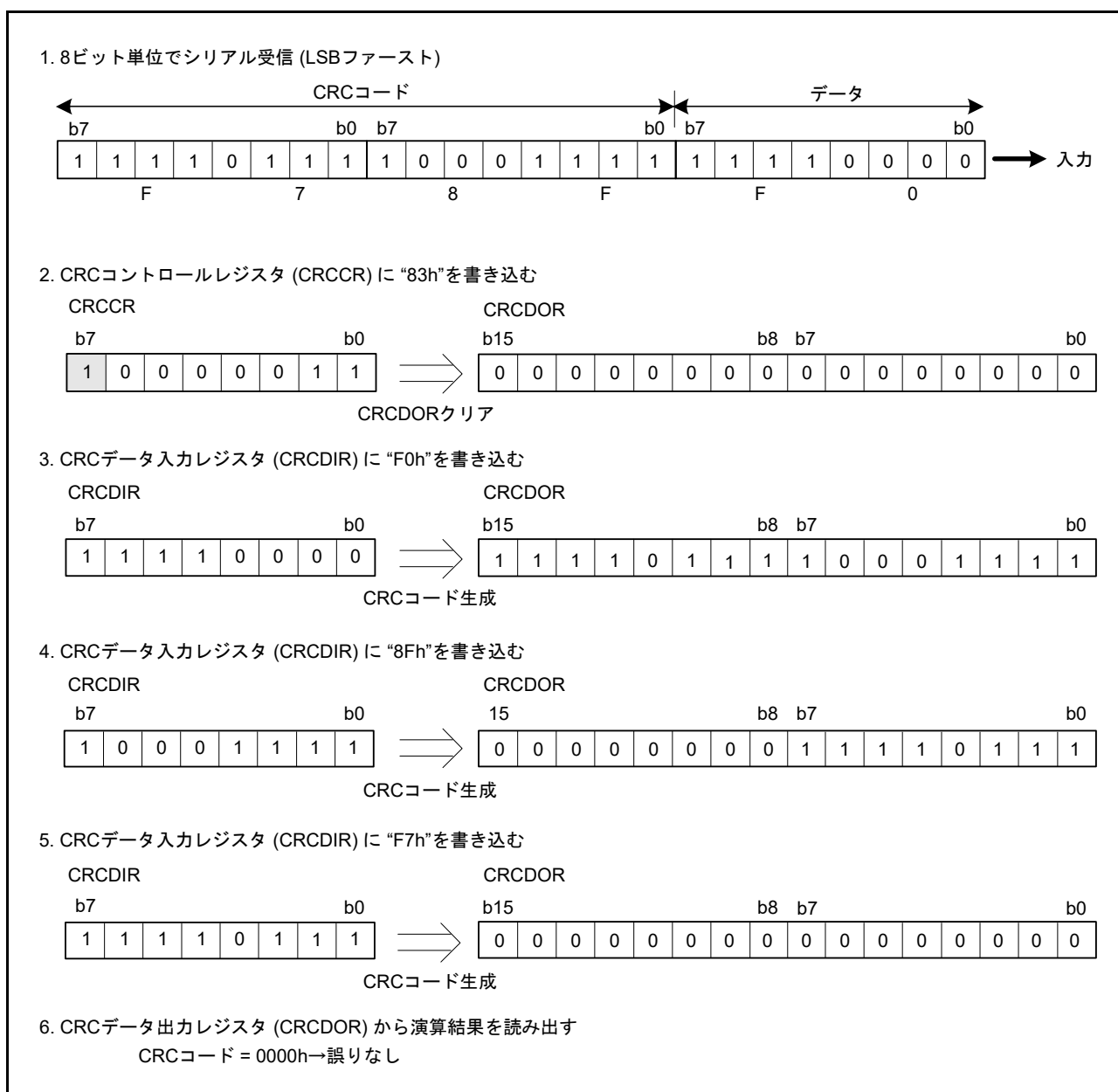
図 45.4 LSBファーストでのデータ受信
