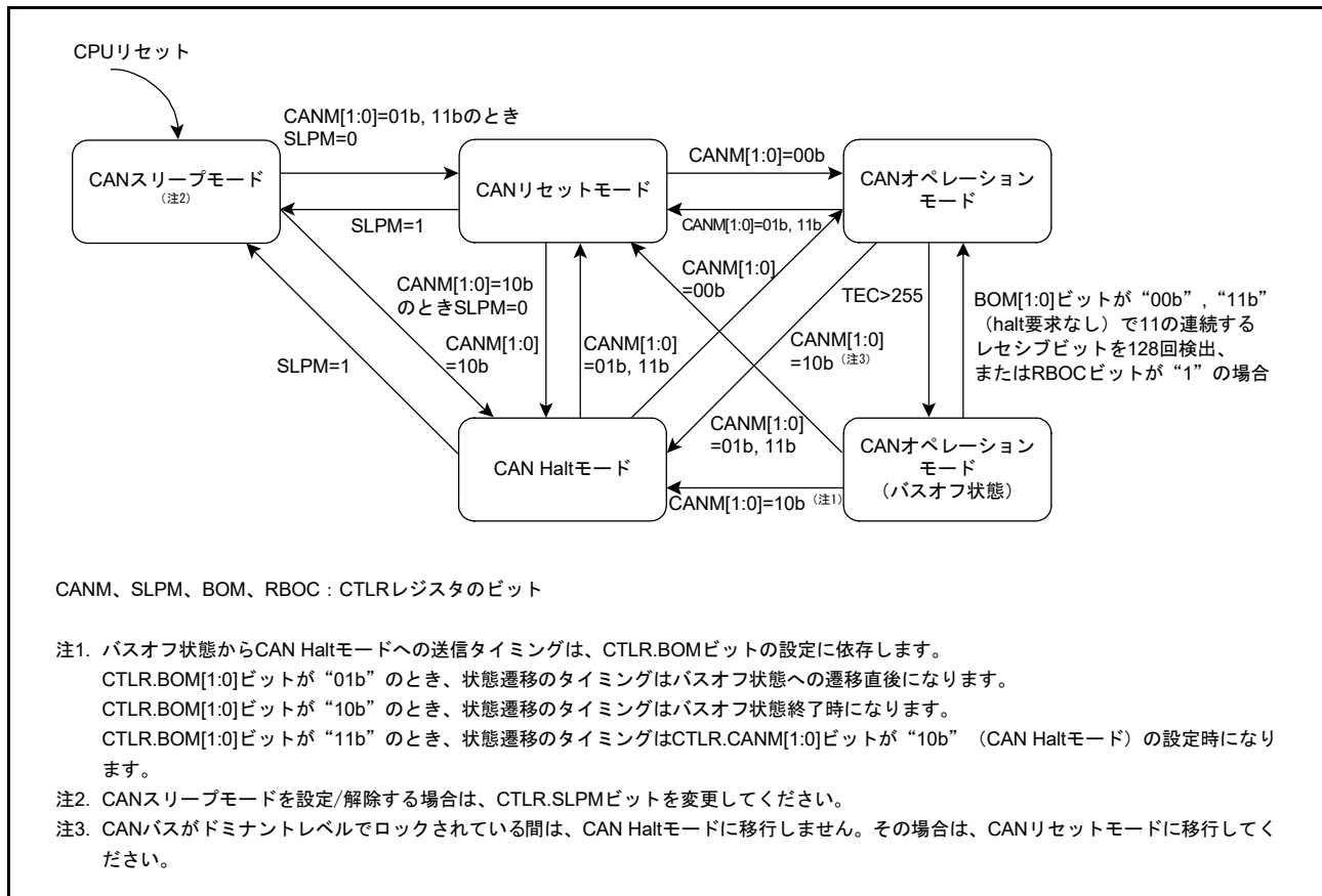
図 42.9 CAN 動作モード間の移行
