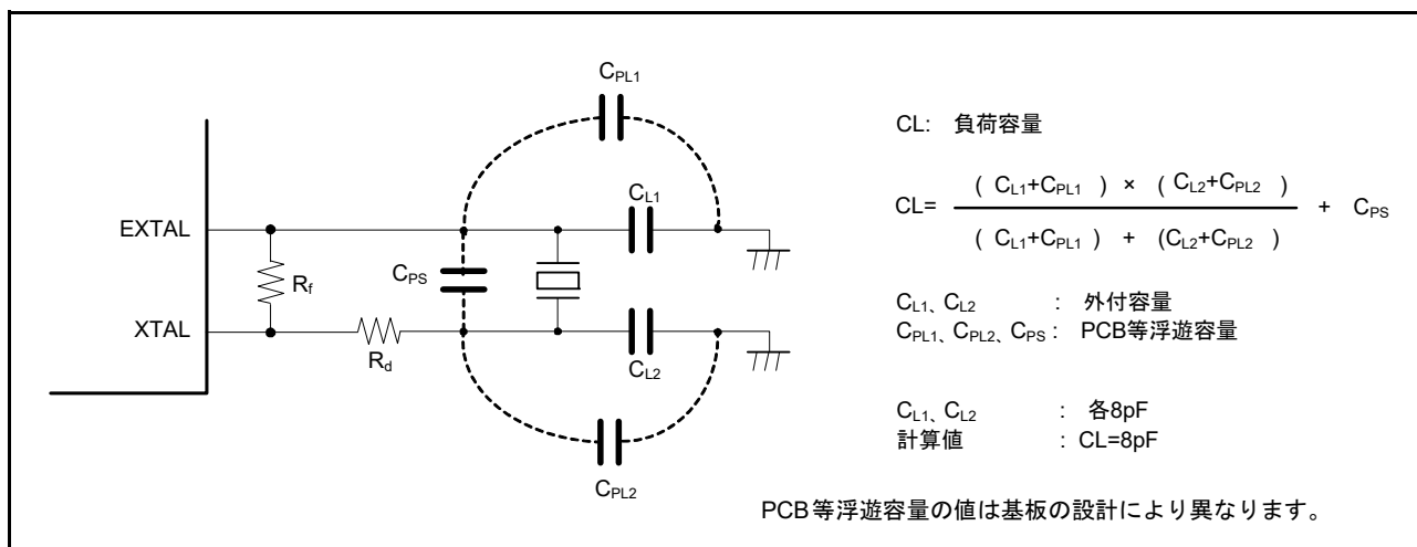
図 9.2 水晶振動子の接続例
