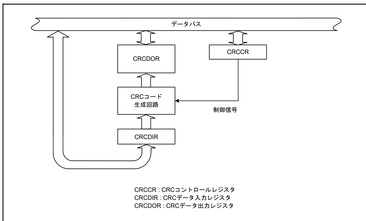
図 45.1 CRC 演算器のブロック図
