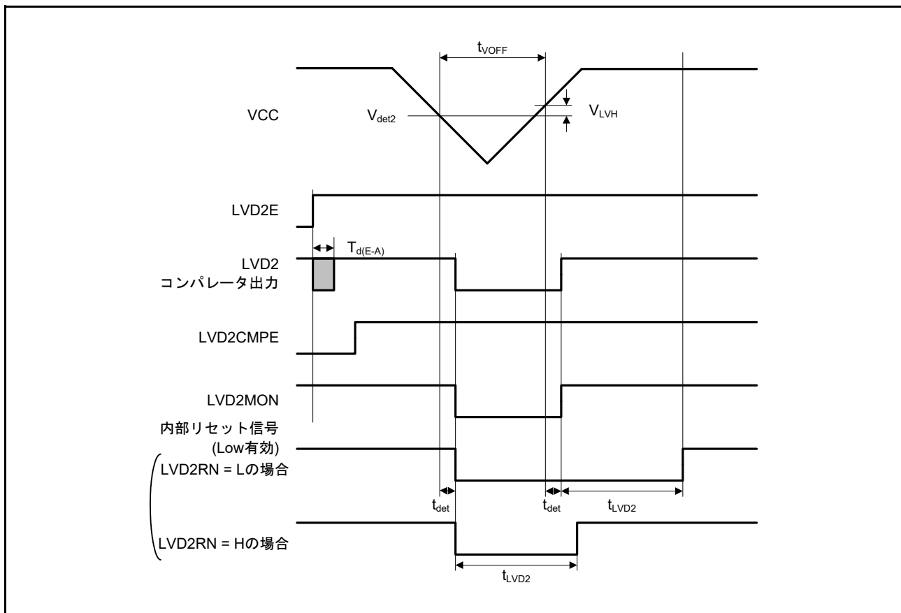
図 61.105 電圧検出回路タイミング ( V_{det2} )
