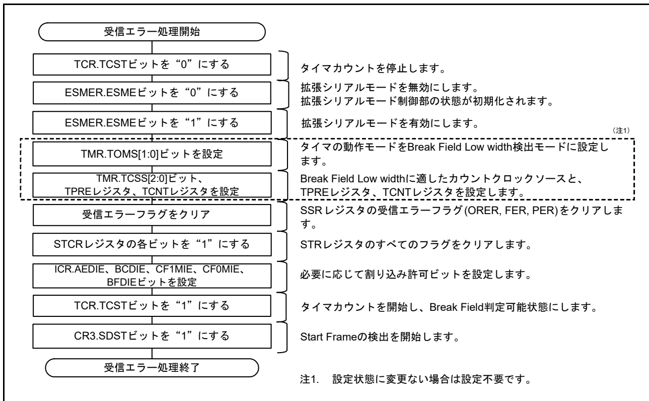
図 40.86 受信エラー処理のフローチャートの例 (Start Frame 受信中)
