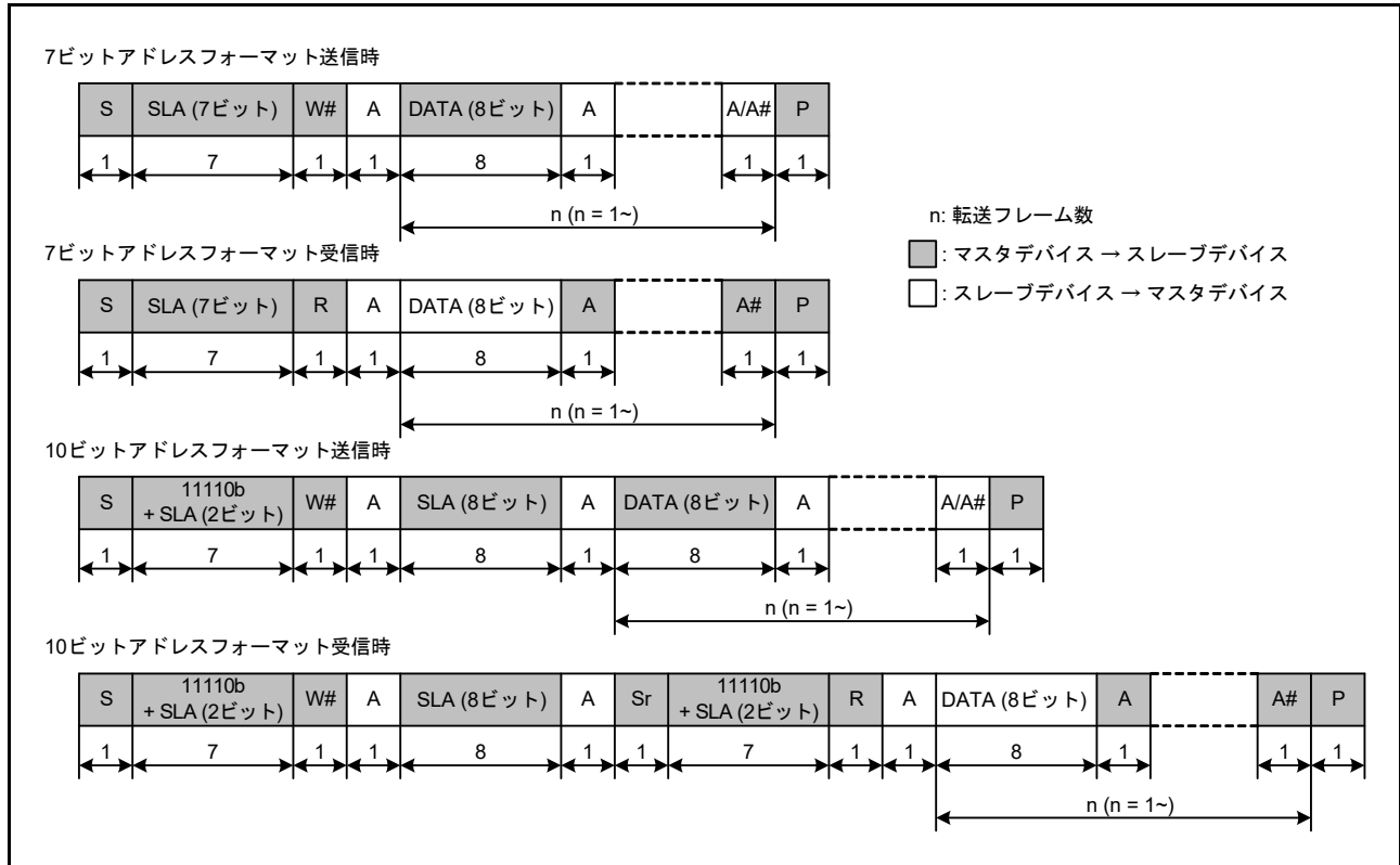
図 40.50 I 2 C バスフォーマット
