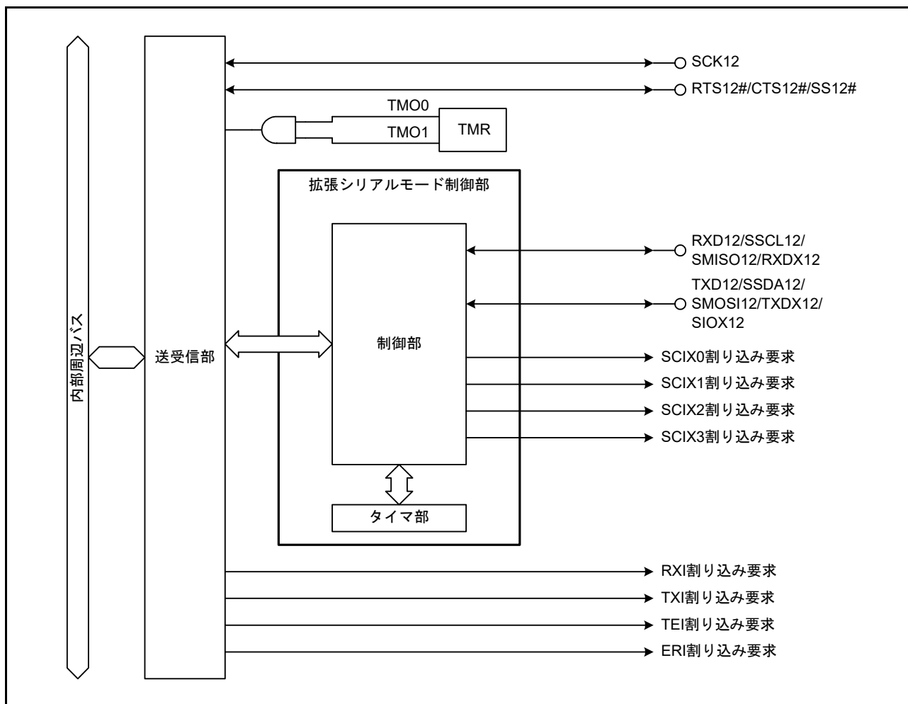
図 40.4 SClh (SCI12) のブロック図
