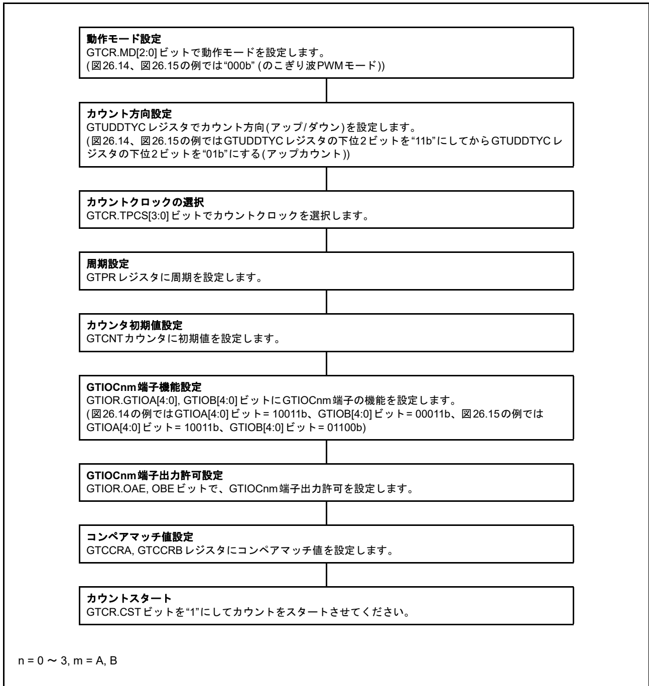
図 26.16 トグル出力動作設定例
