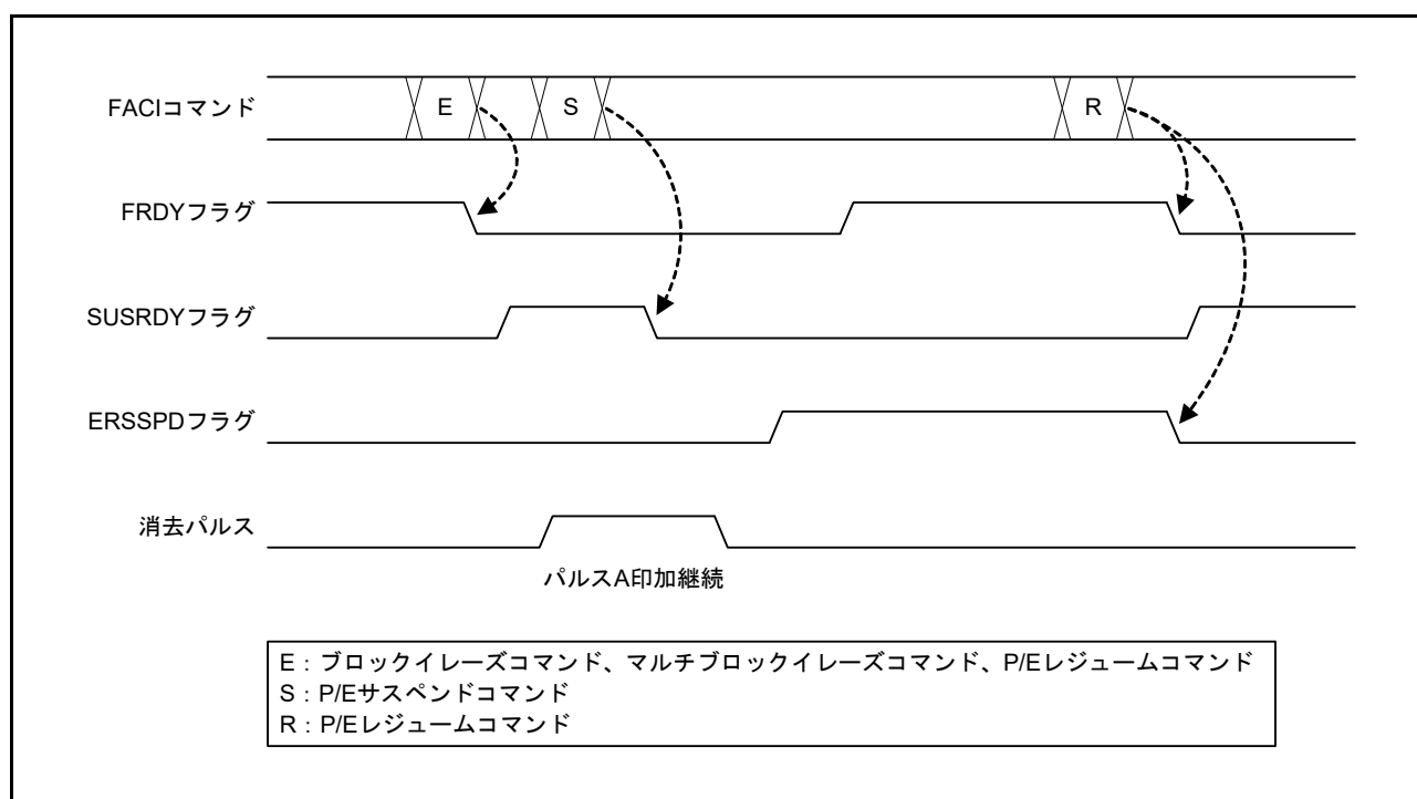
図 60.20 イレーズ処理の中断動作 (イレーズ優先モード)
