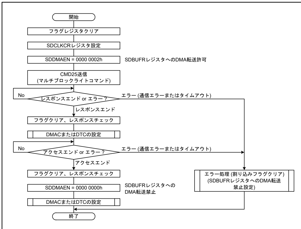
図 47.22 マルチブロックライトコマンド (CMD25) を送信した後、DMA 転送で SDBUFR レジスタへ転送する例
