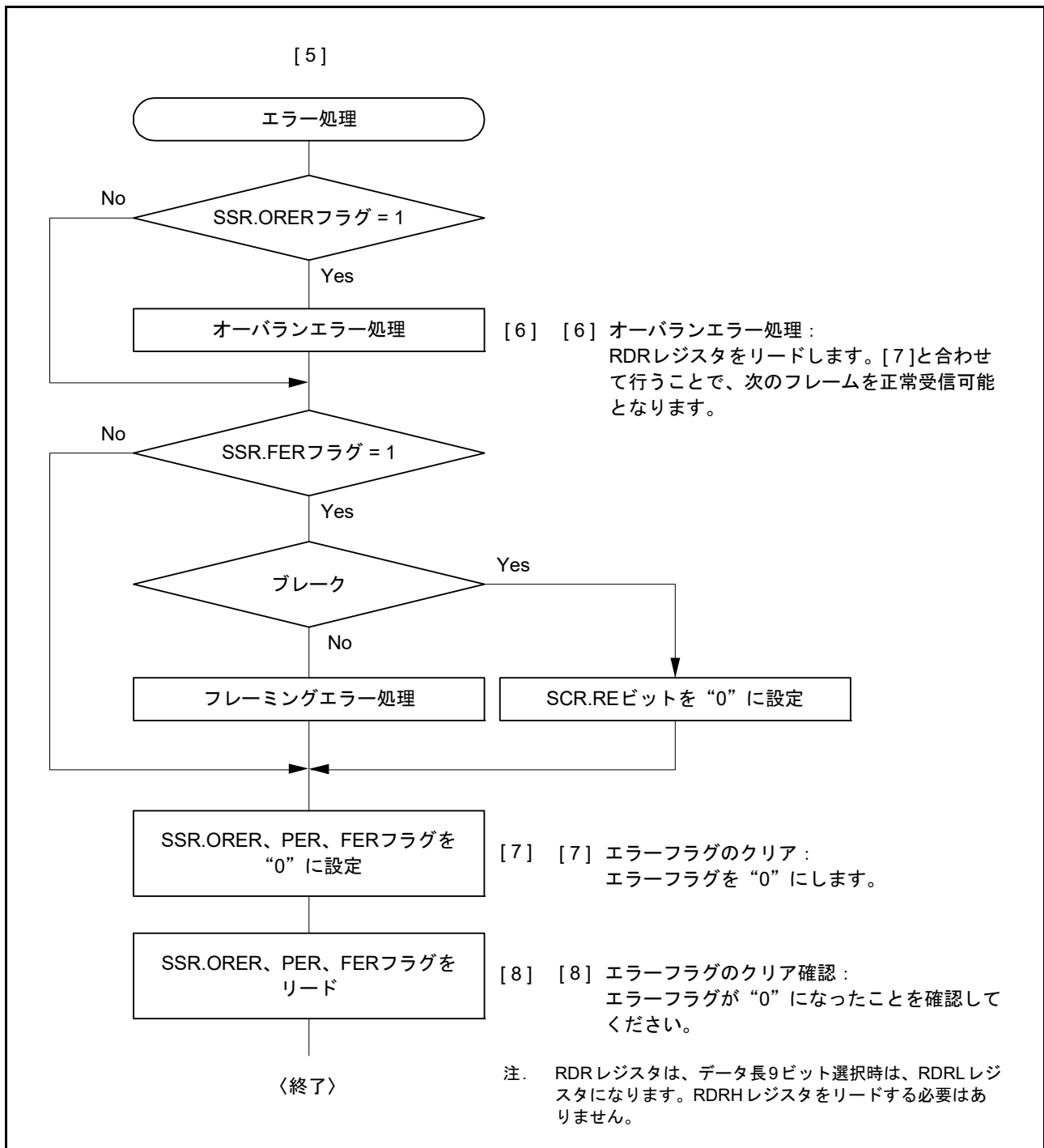
図 40.26 マルチプロセッサシリアル受信のフローチャートの例 (2)
