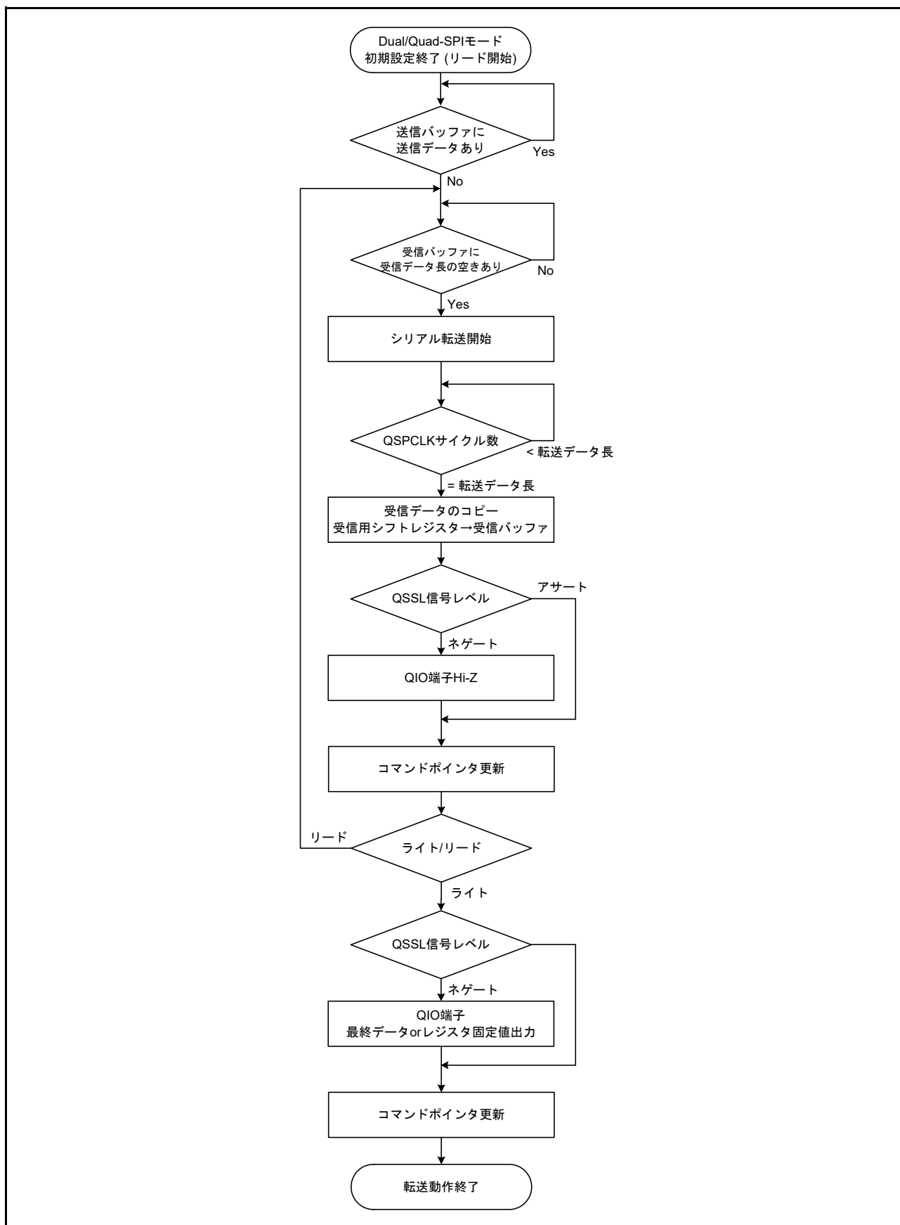
図 44.25 Dual/Quad-SPI モードの動作フロー (シーケンスを Dual/Quad のリードのみで構成)
