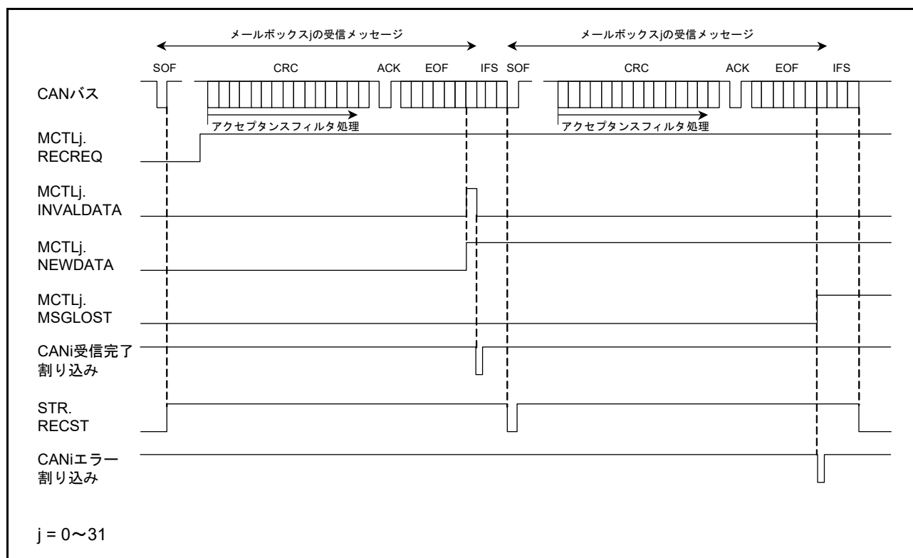
図 42.19 データフレーム受信時の動作例（オーバランモードの場合）
