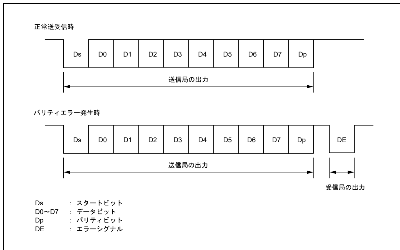
図 40.38 スマートカードインタフェースモードのデータフォーマット
