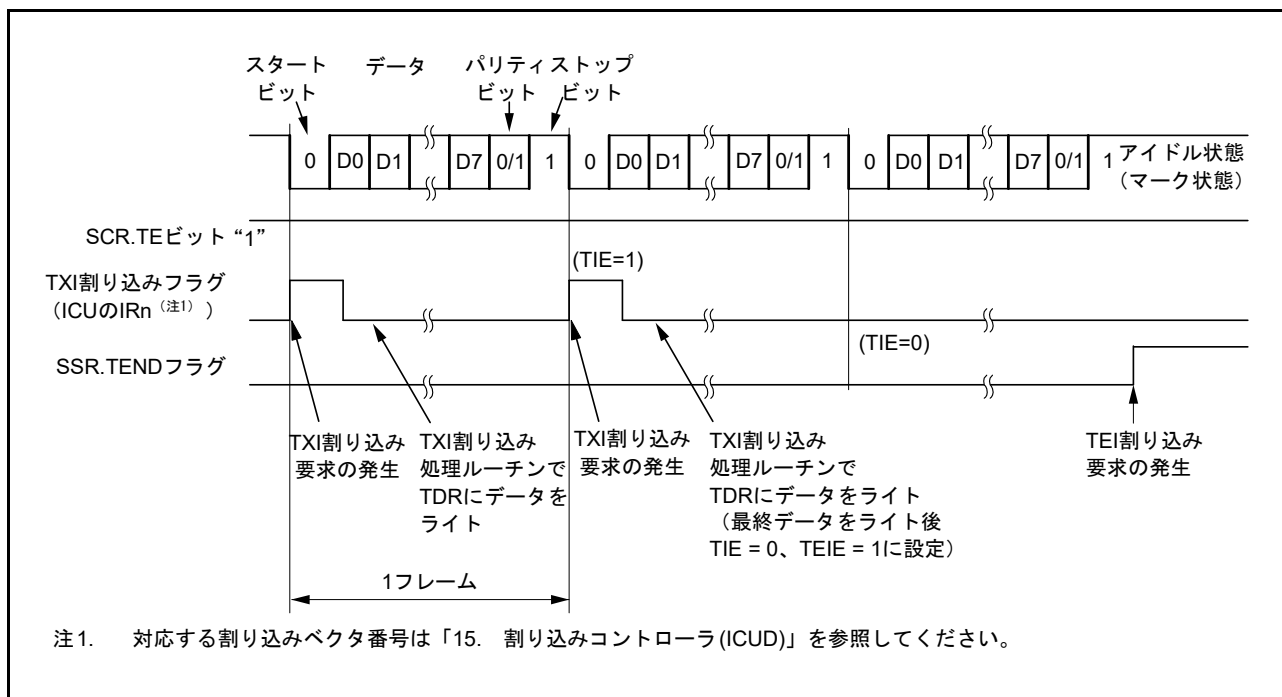
図 40.16 調歩同期式モードのシリアル送信の動作例 (3) (8ビットデータ / パリティあり / 1ストップビット / CTS機能使用しない / 送信中～送信終了時)
