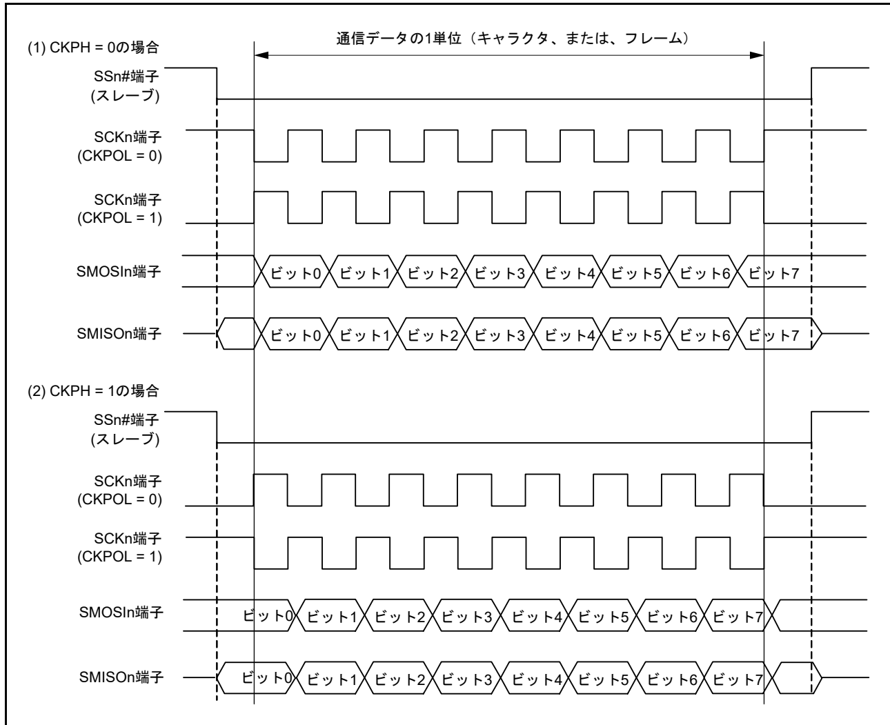
図 40.62 簡易 SPI モードのクロックと送受信データの関係
