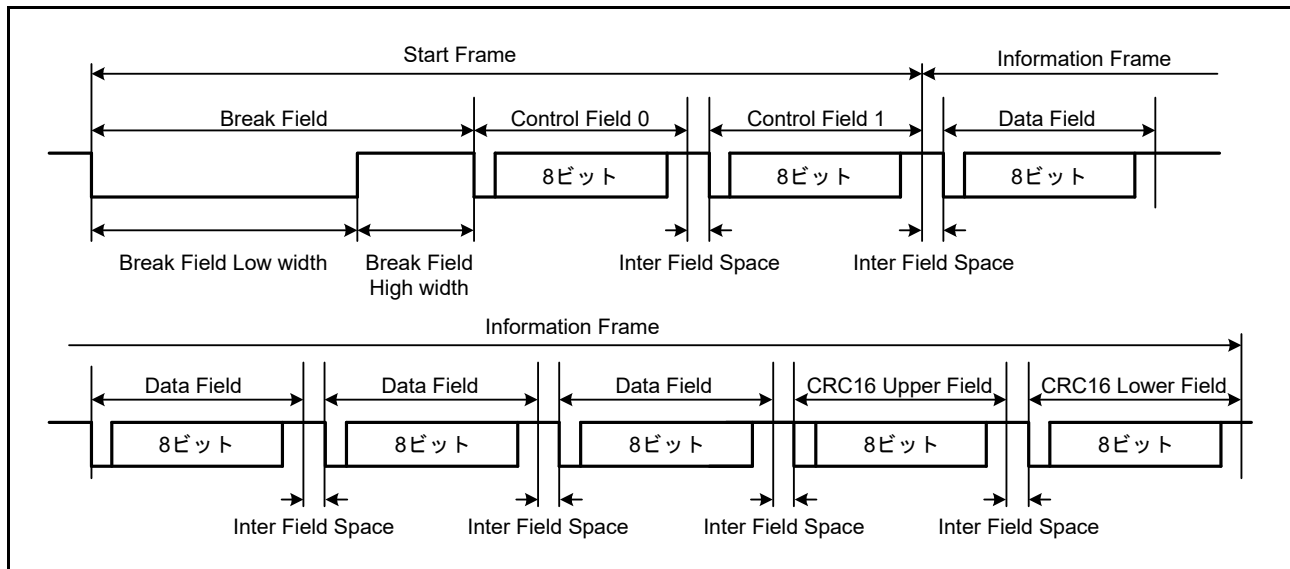
図 40.64 拡張シリアルモード制御部シリアル通信プロトコル
