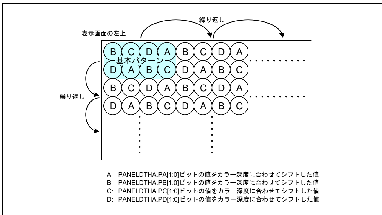
図 50.13 2×2 パターンディザの加算値選択方法
