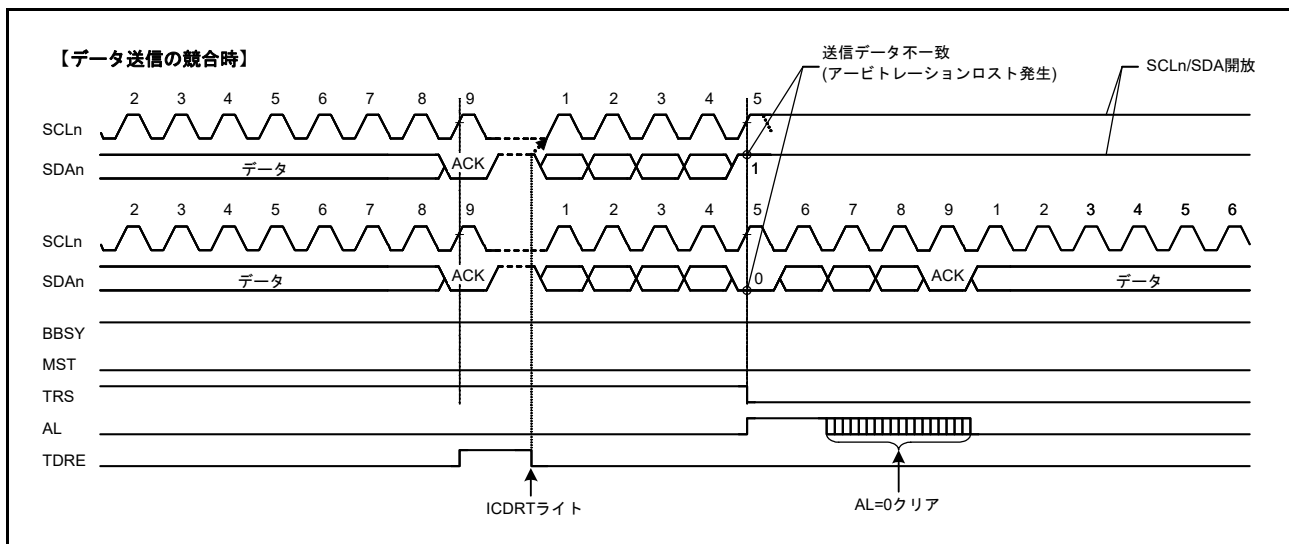
図 41.35 スレーブアービトレーションロスト検出動作例 (SALE ビット = 1 のとき)
