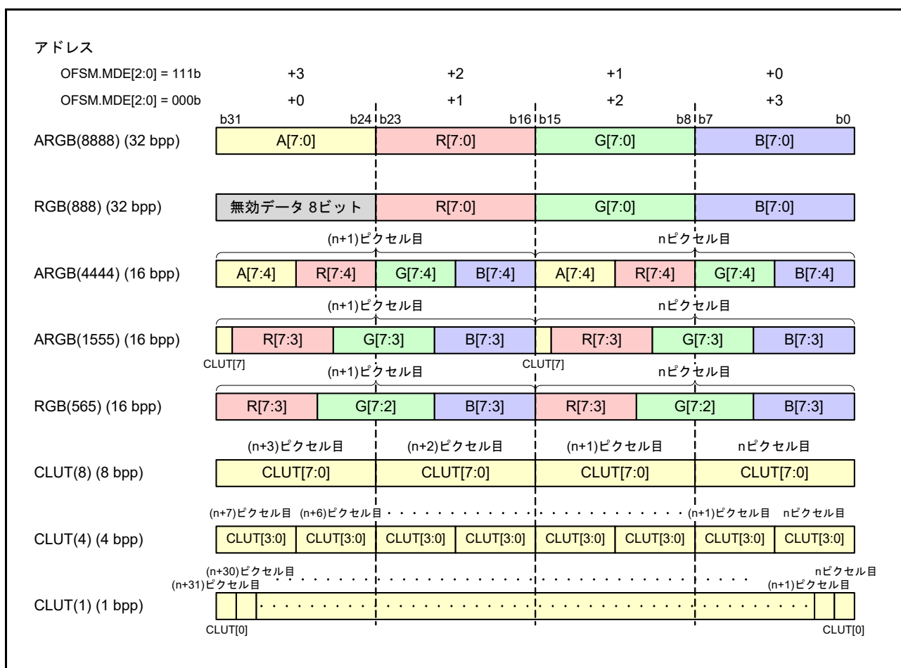
図 50.6 フレームデータのカラーフォーマット
