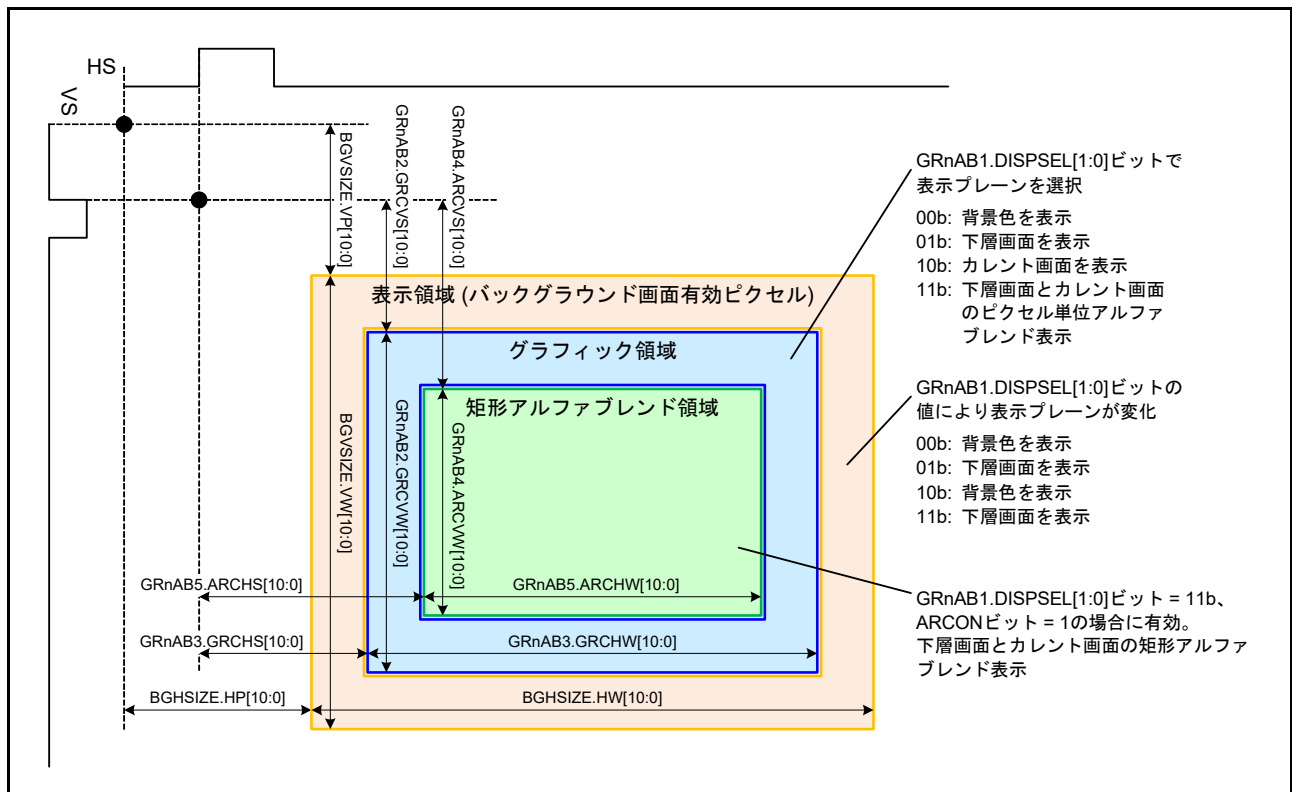
図 50.9 グラフィック表示画面選択 (n = 1, 2)
