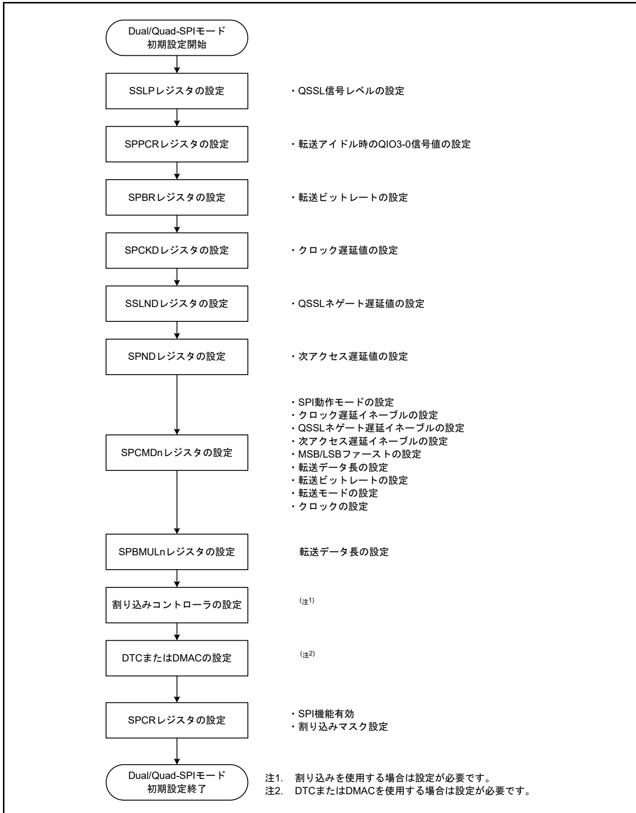
図 44.23 Dual/Quad-SPI モードの初期設定フロー例 (n = 0 ~ 3)
