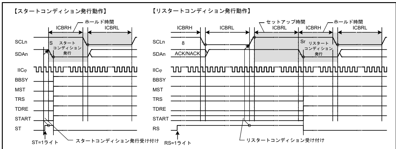
図 41.36 スタートコンディション/リスタートコンディション発行動作タイミング (ST、RS ビット)
