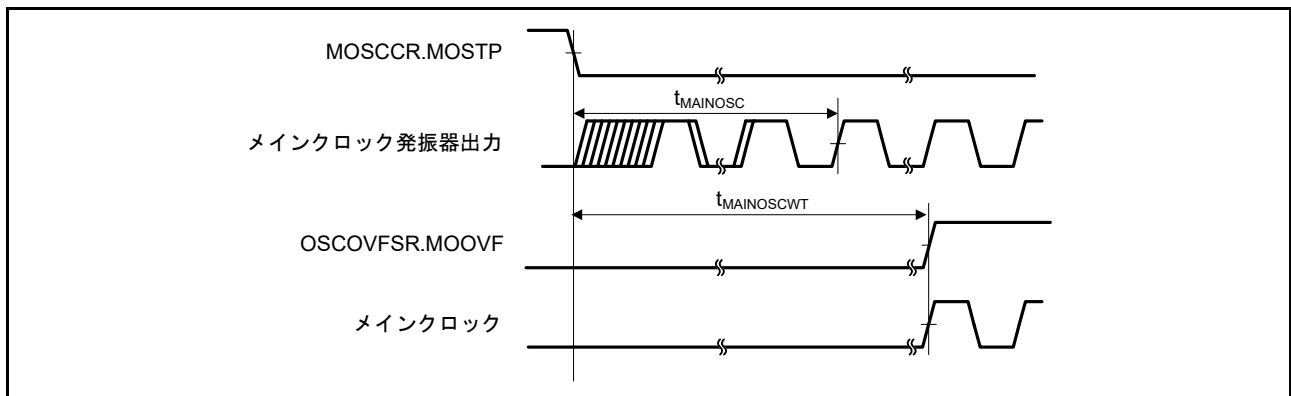
図 61.5 メインクロック発振開始タイミング
