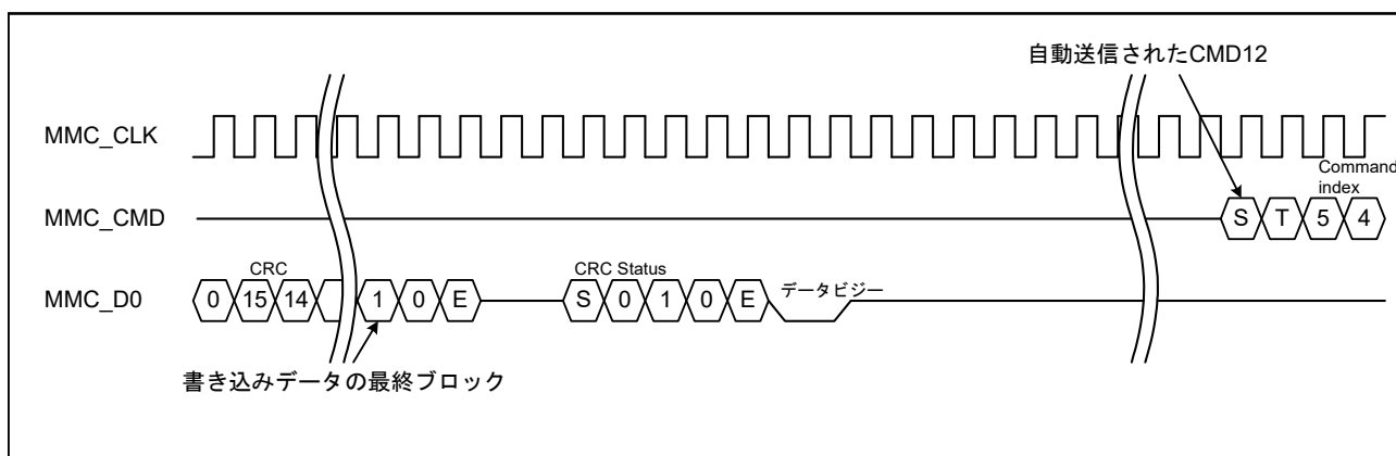
図 48.9 マルチブロックライト時の CMD12 自動送信タイミング (1 ビットモード時)
