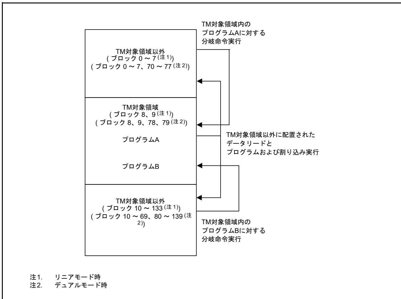
図 60.55 TM 機能有効時、TM 対象領域で CPU が動作可能なケース
