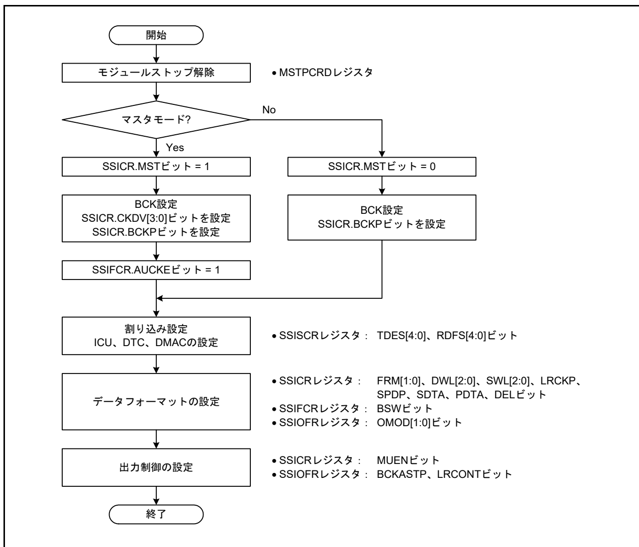
図 46.22 初期設定フロー例
