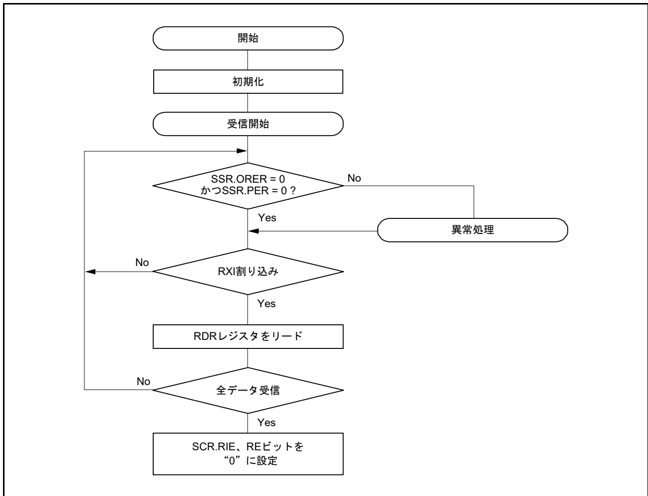
図 40.48 スマートカードインタフェース受信のフローチャート例
