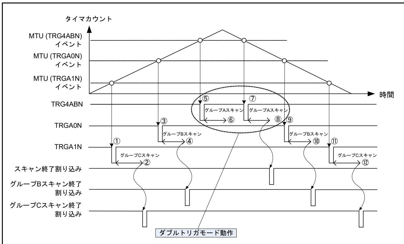
図 54.23 グループスキャンモードでダブルトリガモード選択時の動作例 (MTU からの同期トリガ発生による基本動作)
