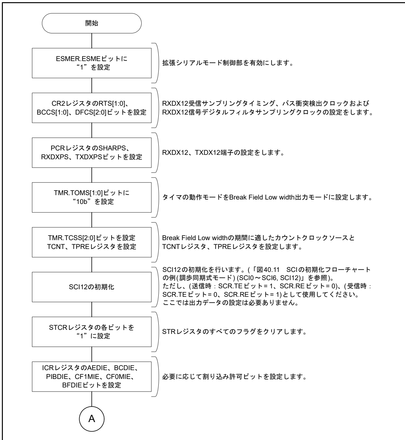
図 40.66 Start Frame 送信フローチャート例 (1)
