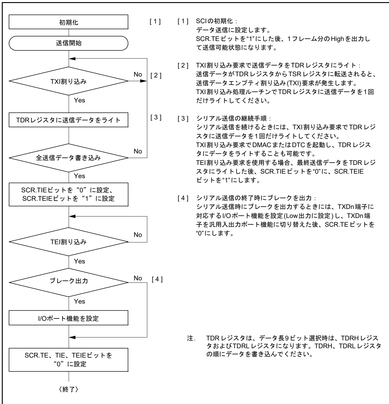
図 40.17 調歩同期式モードのシリアル送信のフローチャート例
