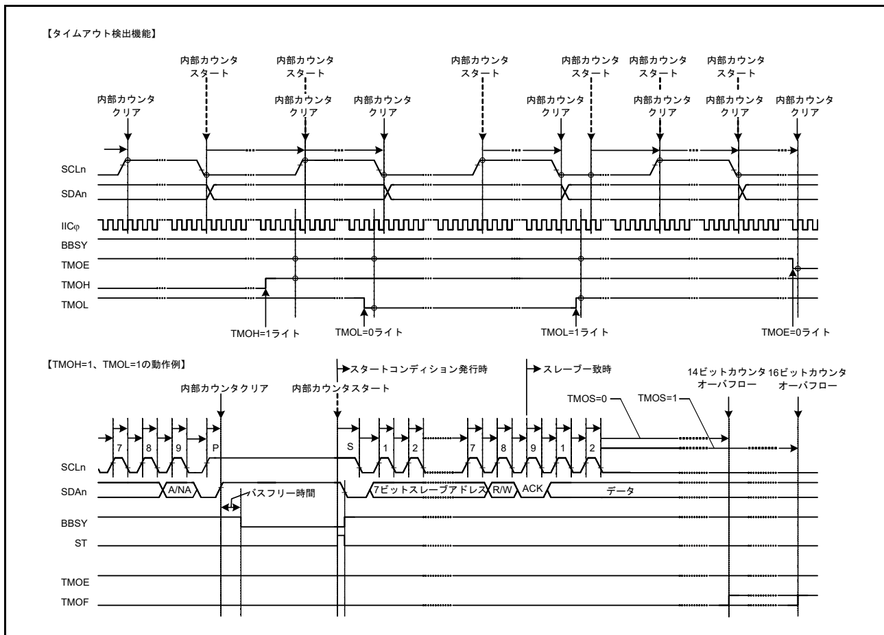
図 41.38 タイムアウト検出機能
