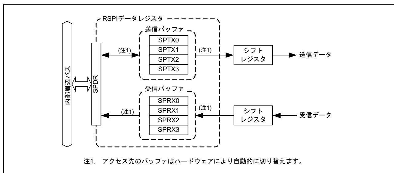
図 43.2 SPDR レジスタの構造図
