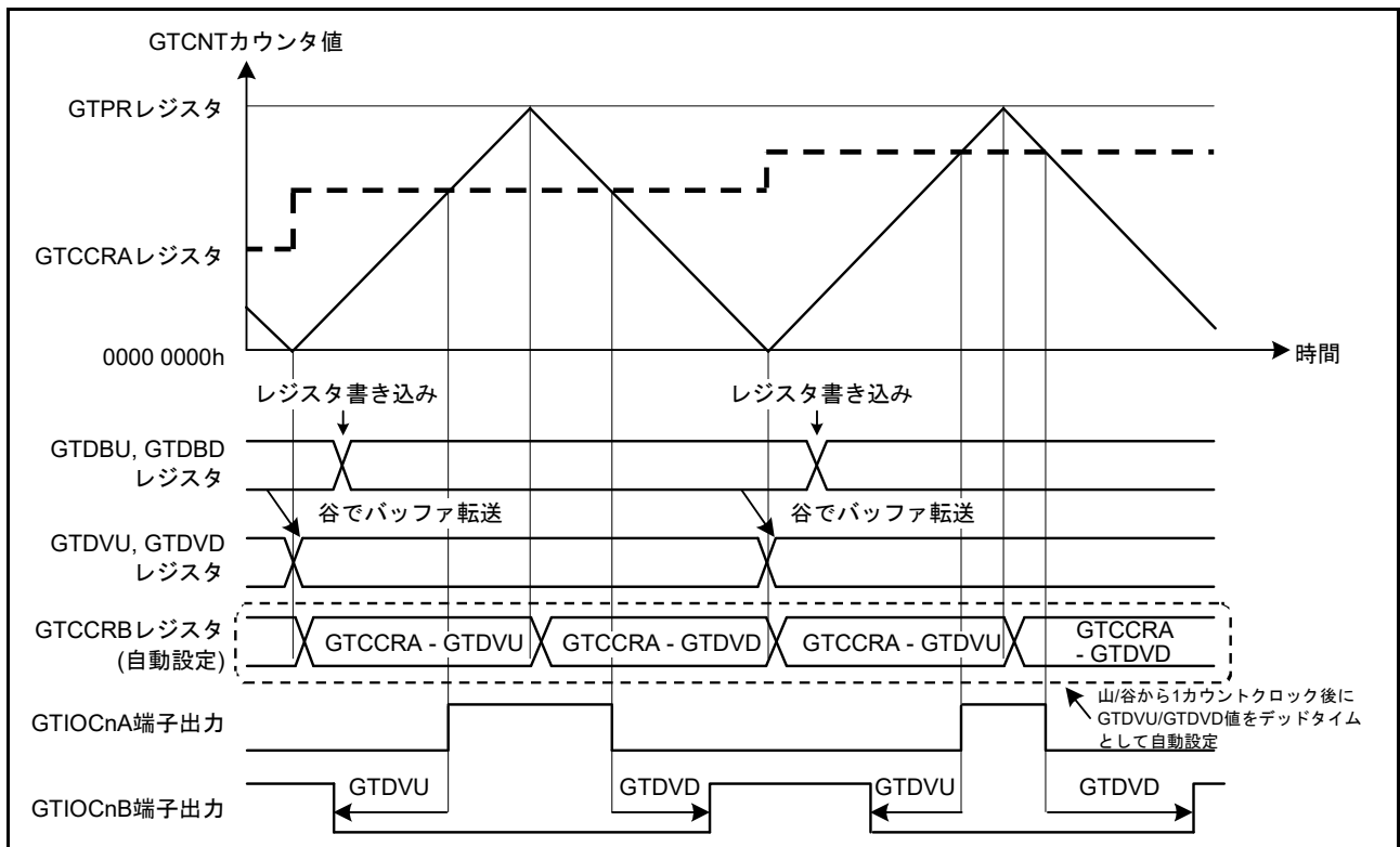
図 26.49 デッドタイム付きコンペアマッチ値の自動設定機能の動作例 (三角波 PWM モード 1、GTDVU/GTDVD レジスタはバッファ動作、アクティブレベルは High の場合) (n = 0 ~ 3)
