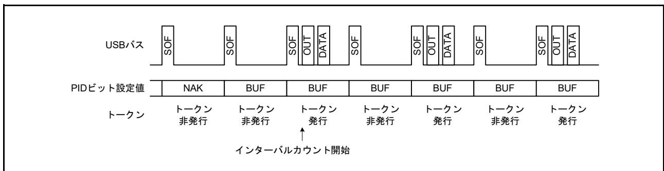
図 39.17 IITV[2:0] = 001b の場合のトークン発行有無
