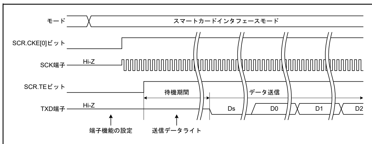
図 40.43 スマートカードインタフェースモード時のデータ送信タイミング例
