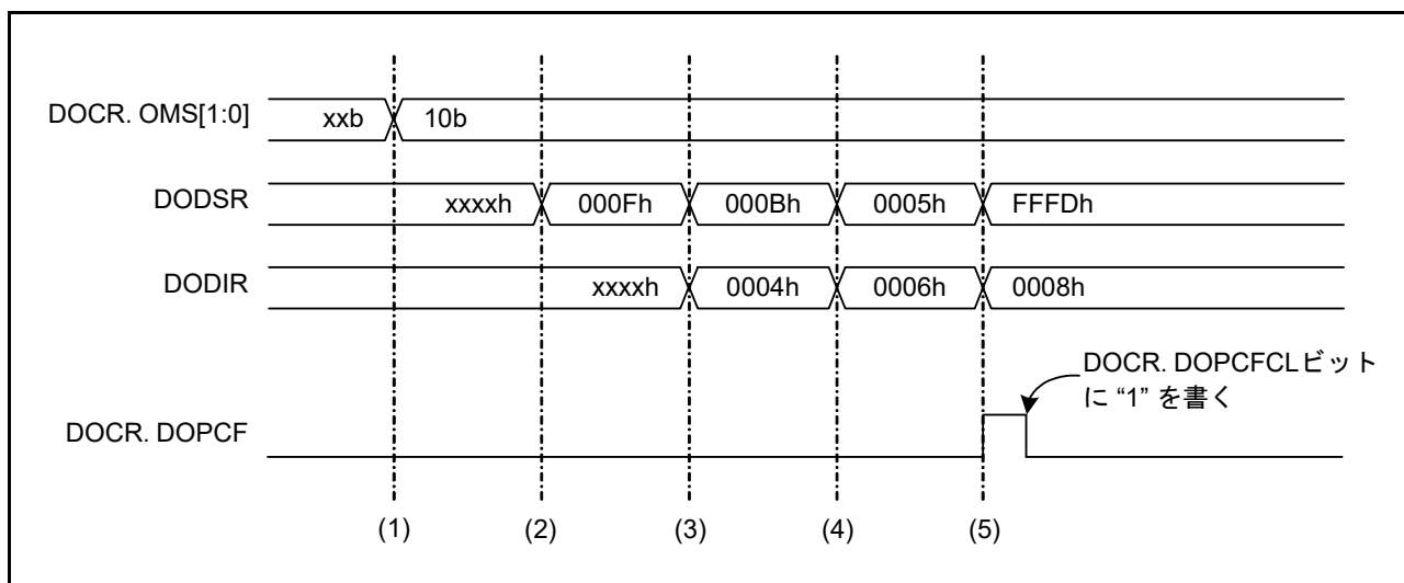
図 57.4 データ減算モードの動作例
