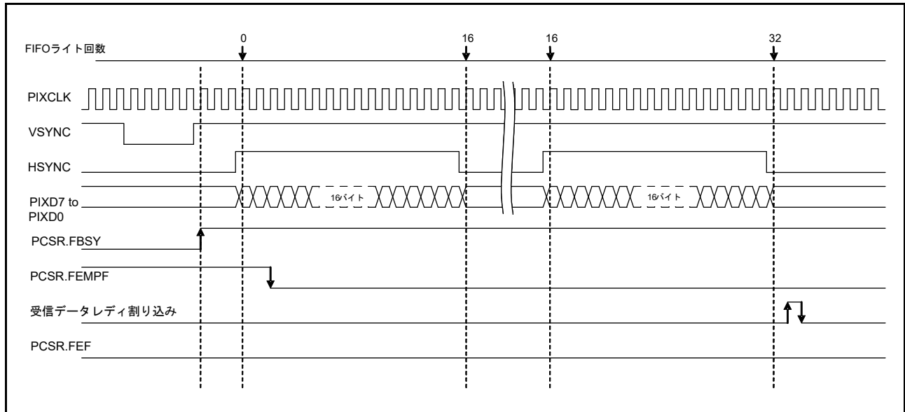
図 49.12 水平ブランキング期間中の動作例
