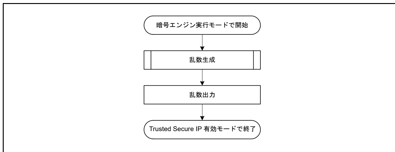
図 53.10 乱数生成フロー
