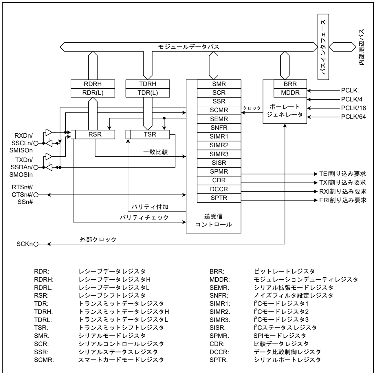
図 40.1 SCIj (SCI0 ~ SCI4) のブロック図
