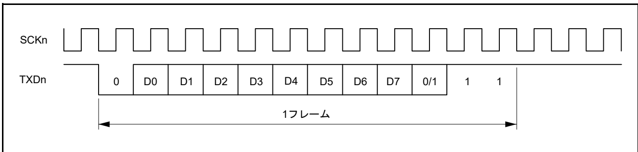
図 40.8 出カクロックと送信データの位相関係 (調歩同期式モード: SMR.CHR = 0、PE = 1、MP = 0、STOP = 1)
