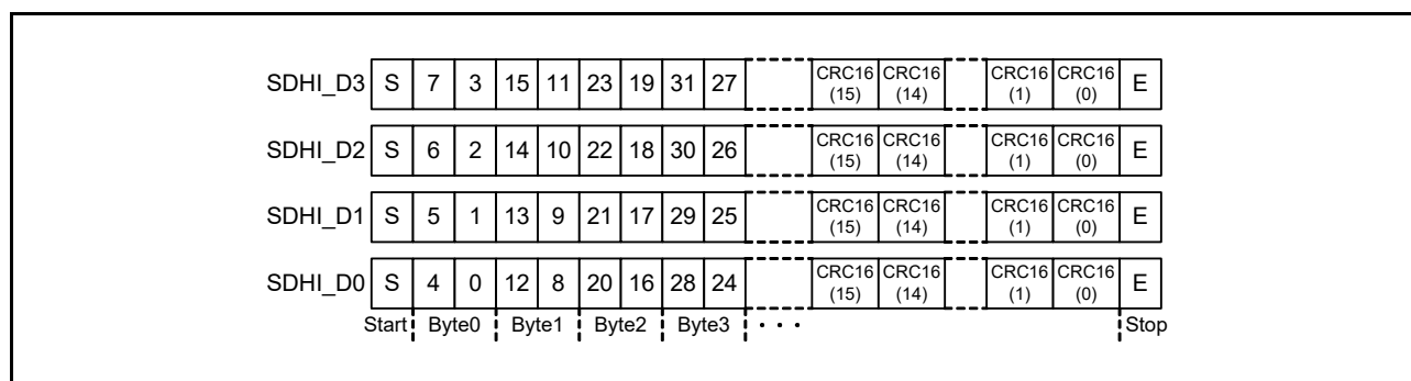
図 47.3 ワイドバスモードの転送フォーマット (SDOPT.WIDTH ビットが“0”のとき)
