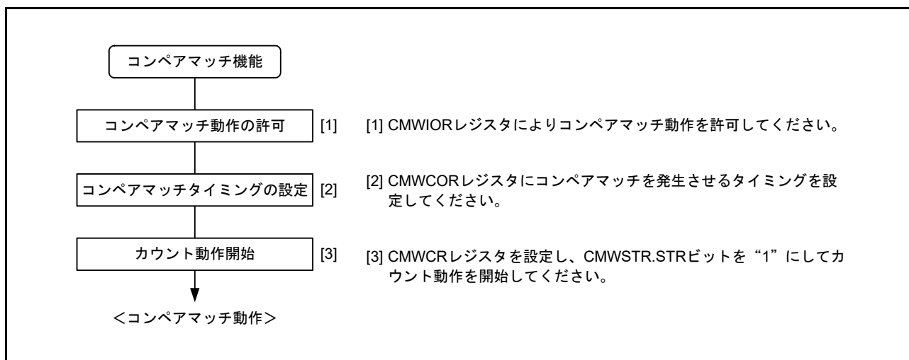
図 32.3 コンペアマッチ動作の設定手順例
