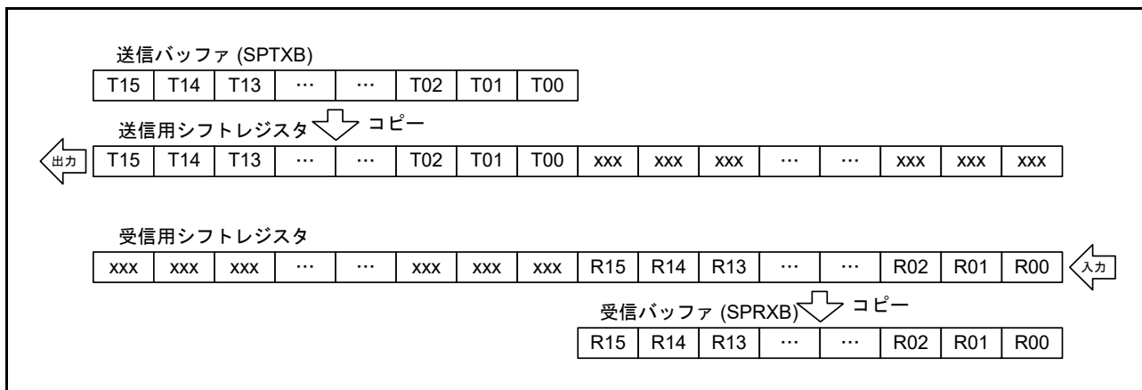
図 44.7 MSB ファースト転送 (16 ビットデータ)
