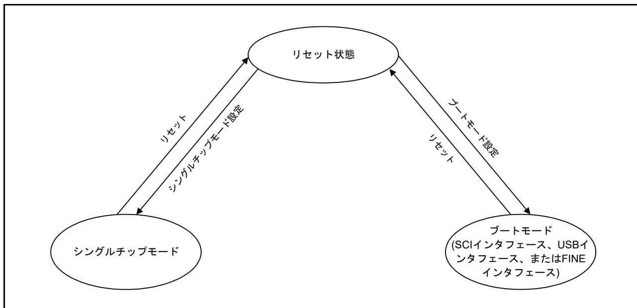
図 60.6 フラッシュメモリに関するモード遷移図
