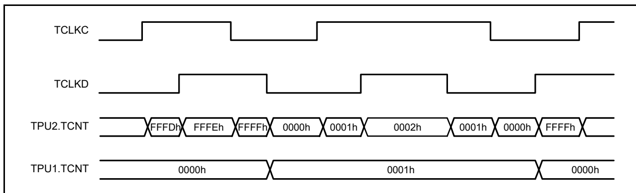
図 28.19 カスケード接続動作例 (2)
