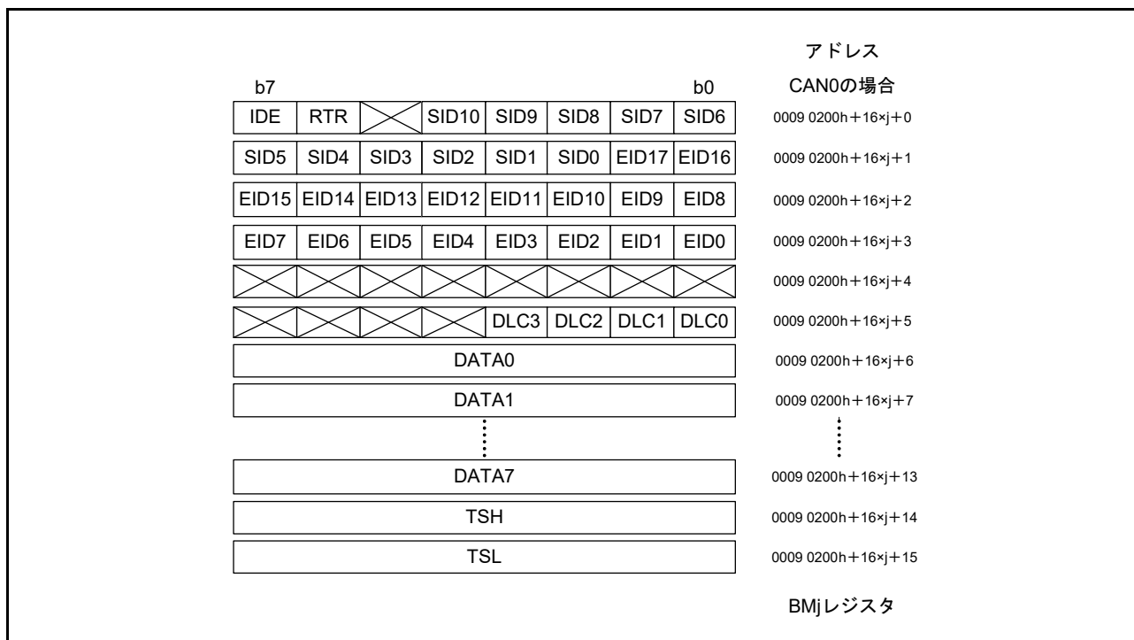
図 42.13 MBj レジスタの構成 (j = 0 ~ 31)
