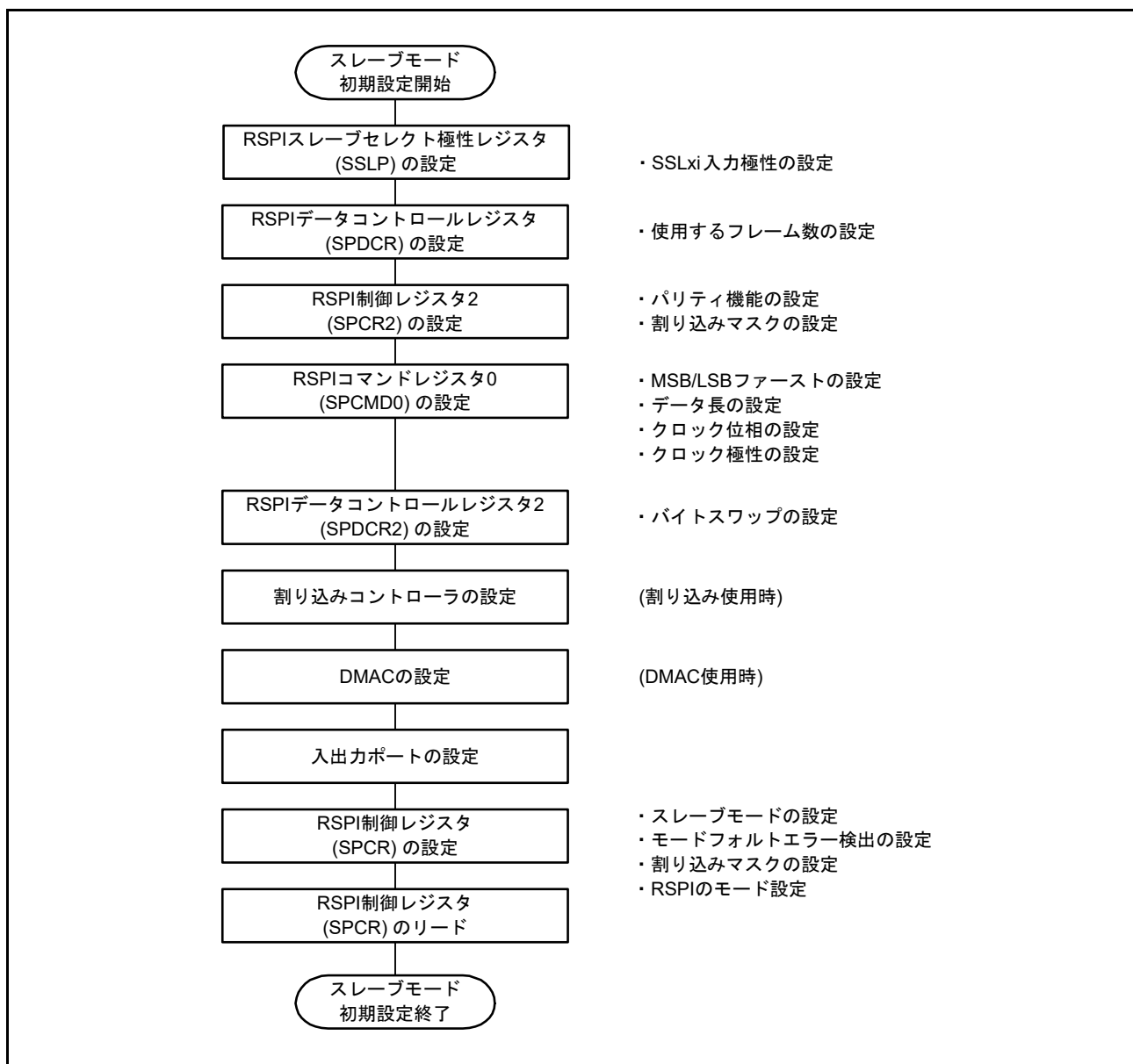
図 43.41 スレーブモード時の初期化フロー例 (SPI 動作)
