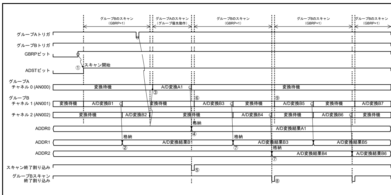
図 54.29 グループ優先動作の例 5「グループ B のシングルスキャン連続動作」 (ADGSPCR.GBRP = 1, ADGSPCR.LGRRS = 1, ADGCTRGR.GRCE = 0 設定時)
