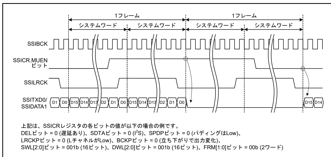
図 46.17 ミュート機能の動作例
