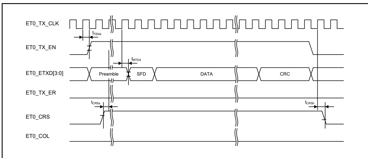
図 61.86 MII 送信タイミング (正常動作時)
