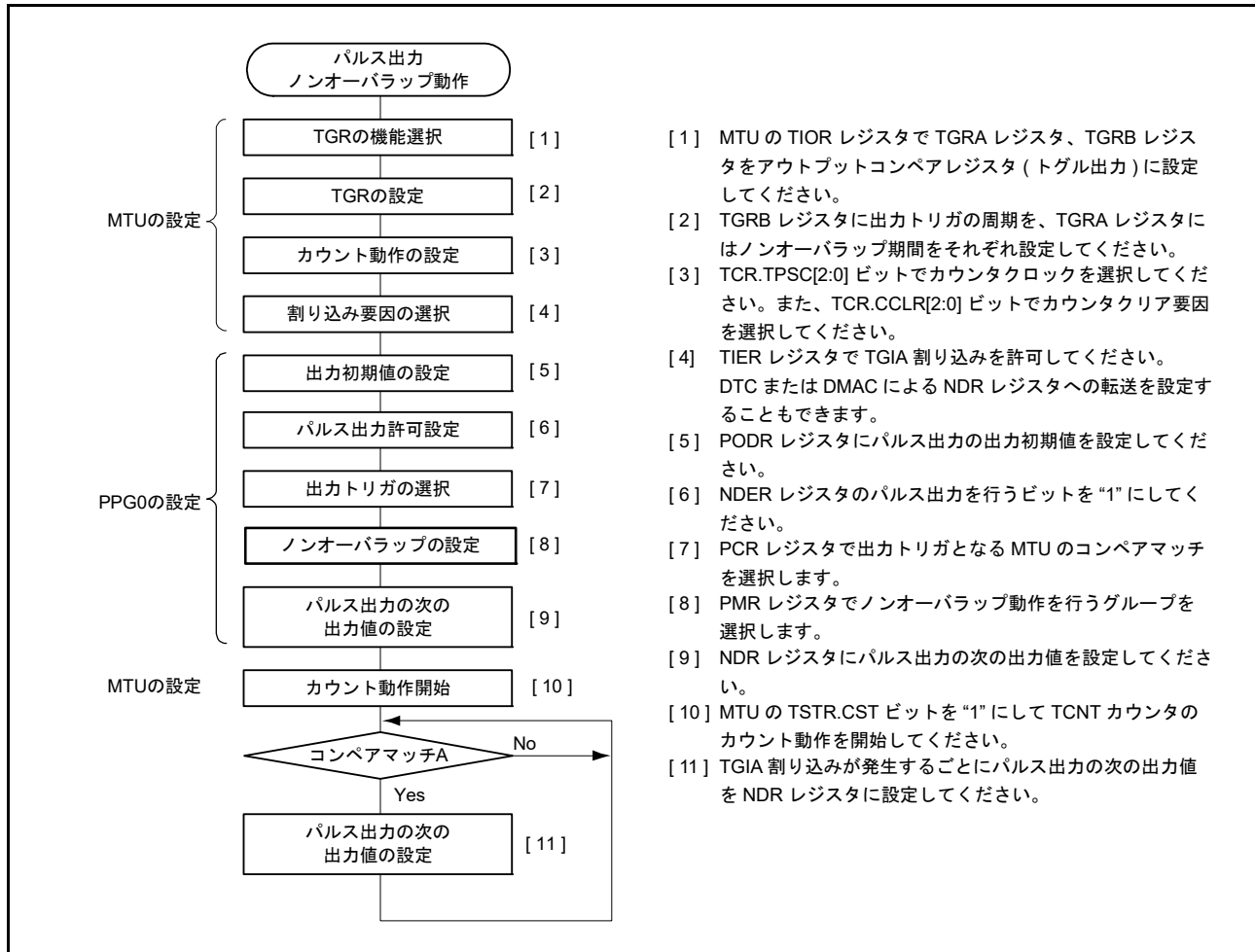
図 29.11 パルス出力ノンオーバーラップ動作の設定手順例 (PPG0 の設定)
