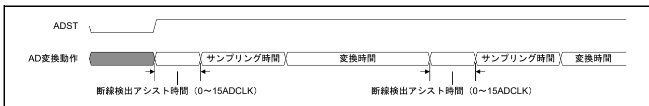
図 54.41 断線検出アシスト機能を使用した場合の A/D 変換動作図
