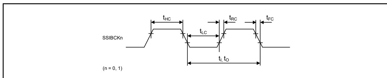
図 61.74 SSIE クロック入出力タイミング
