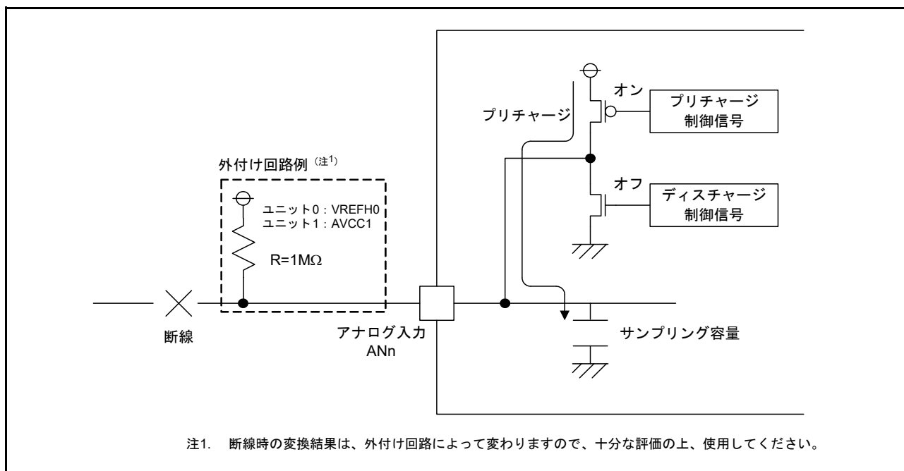
図 54.42 プリチャージを選択した場合の断線検出例
