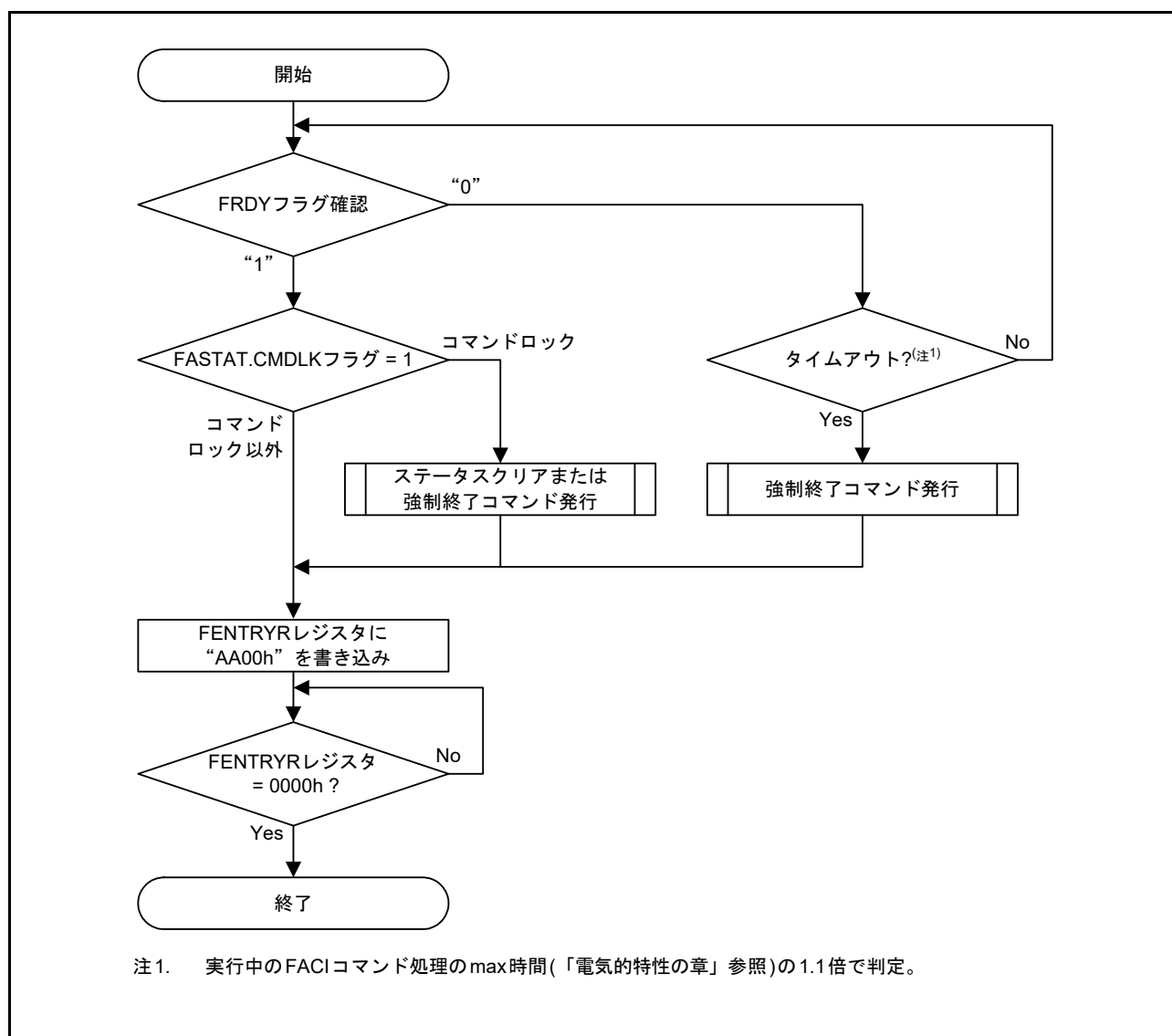
図 60.11 リードモード移行フロー
