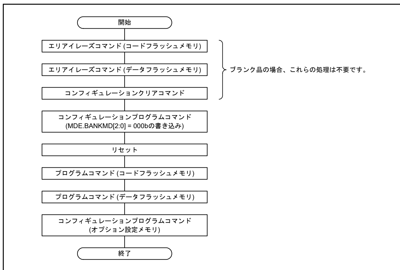
図 60.50 デュアルモードに切り替えてからフラッシュメモリを書き換える例
