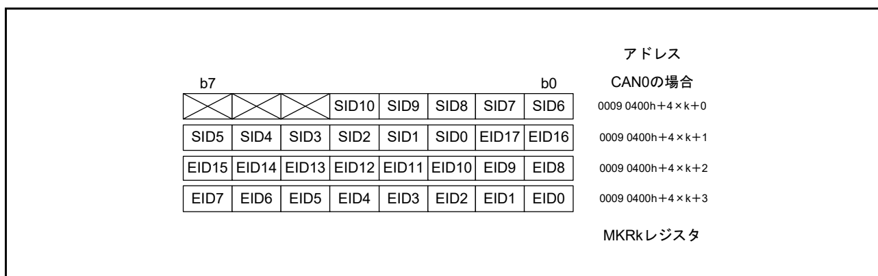
図 42.14 MKRk レジスタの構成 (k = 0 ~ 7)
