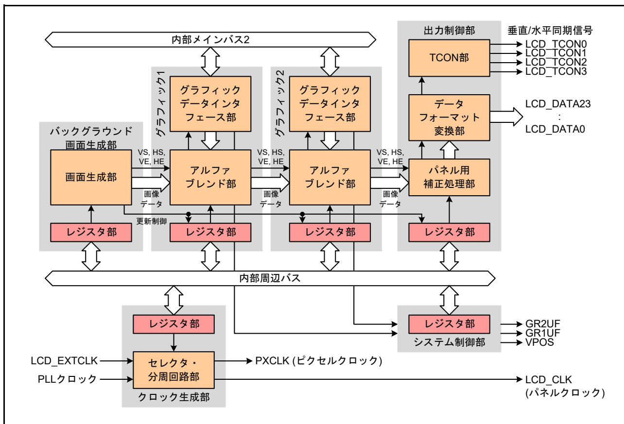
図 50.1 GLCDC のブロック図
