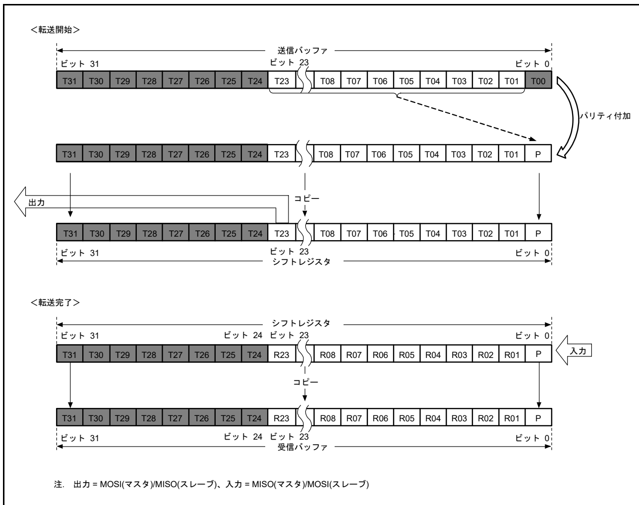
図 43.19 MSB ファースト転送 (24 ビットデータ / パリティ機能有効)
