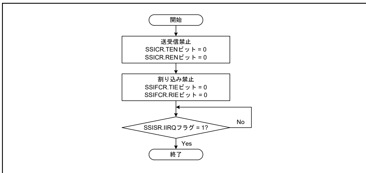
図 46.25 通信停止フロー例
