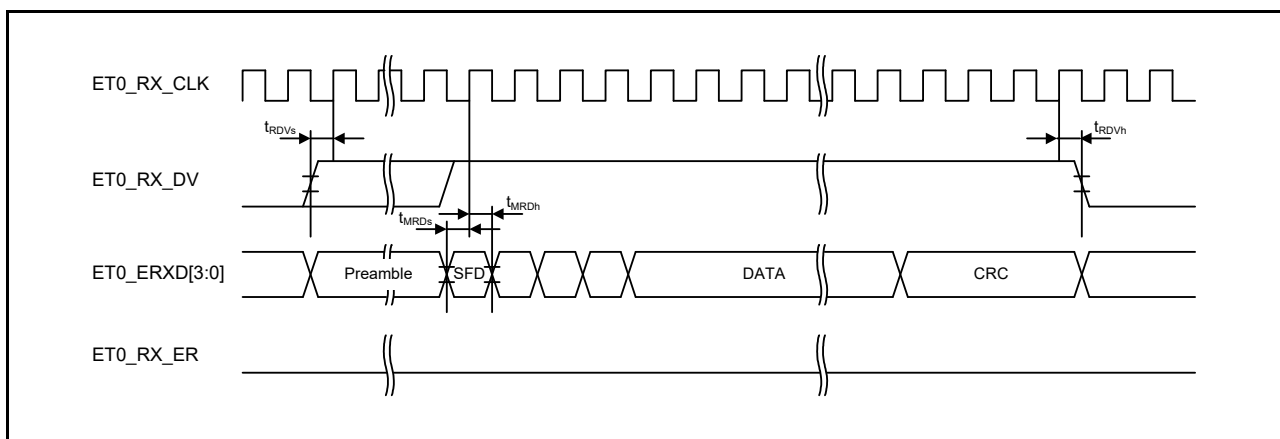
図 61.88 MII 受信タイミング (正常動作時)
