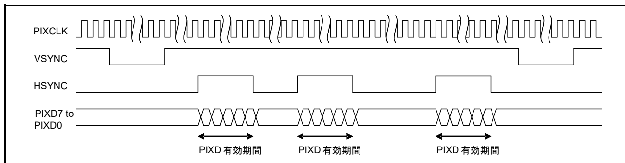
図 49.4 PDC 通信フォーマット (VPS = 0, HPS = 0)
