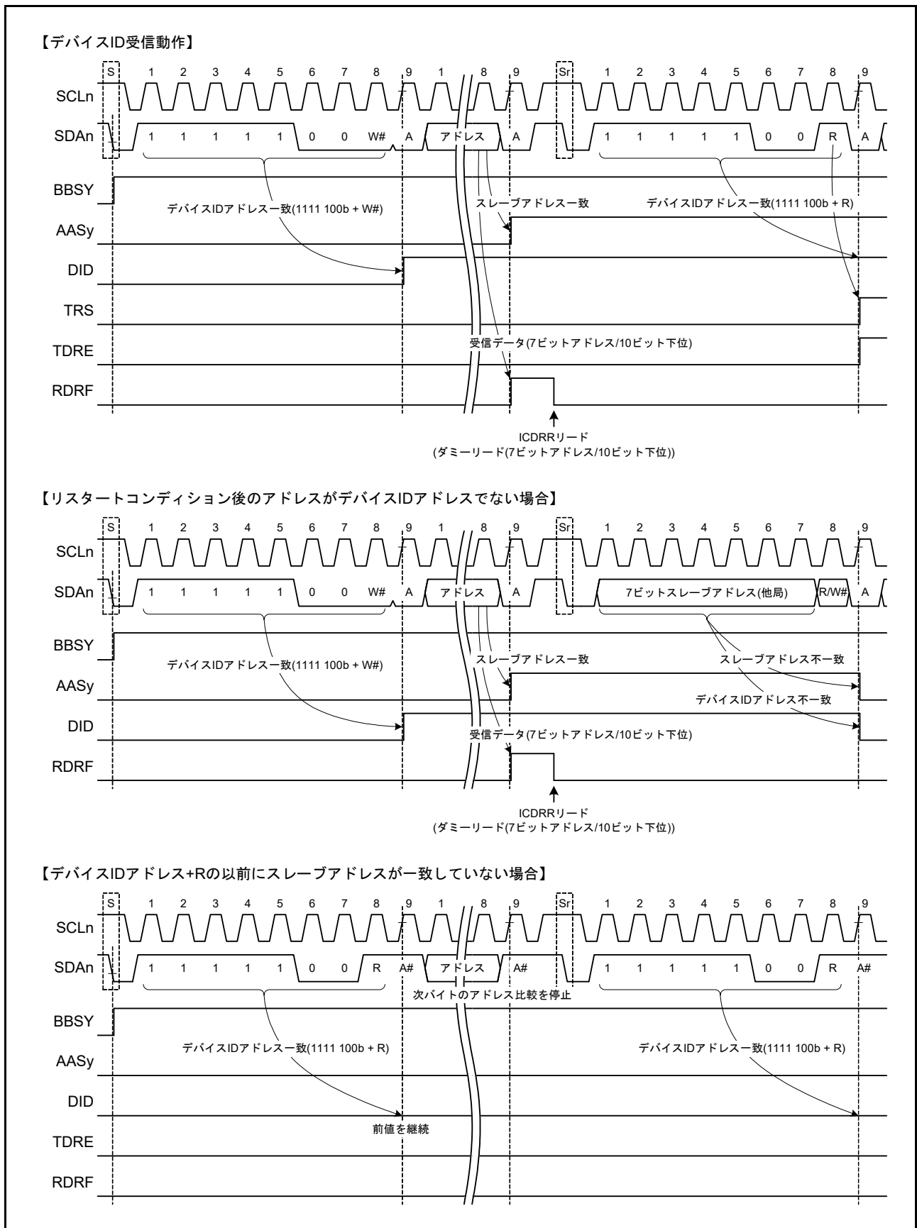
図 41.27 デバイス ID アドレス受信時の AASy、DID フラグセット / クリアタイミング
