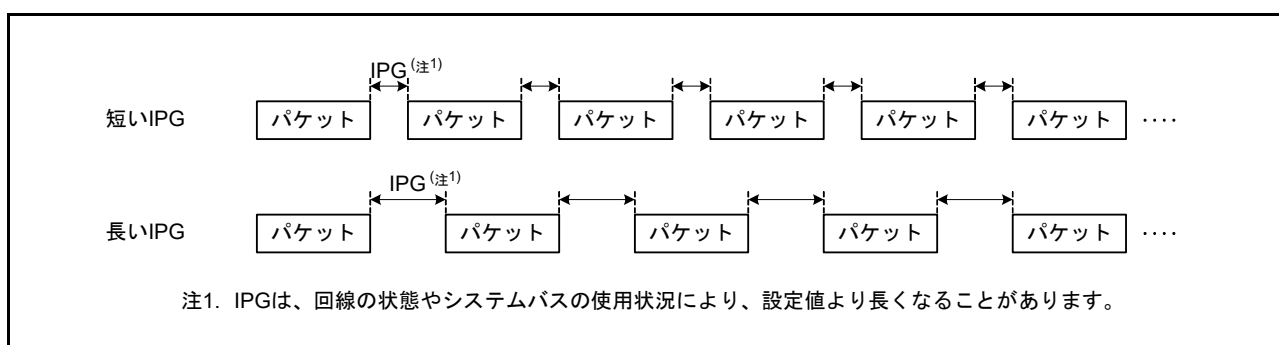
図 36.18 IPG の変更による伝送効率の違い
