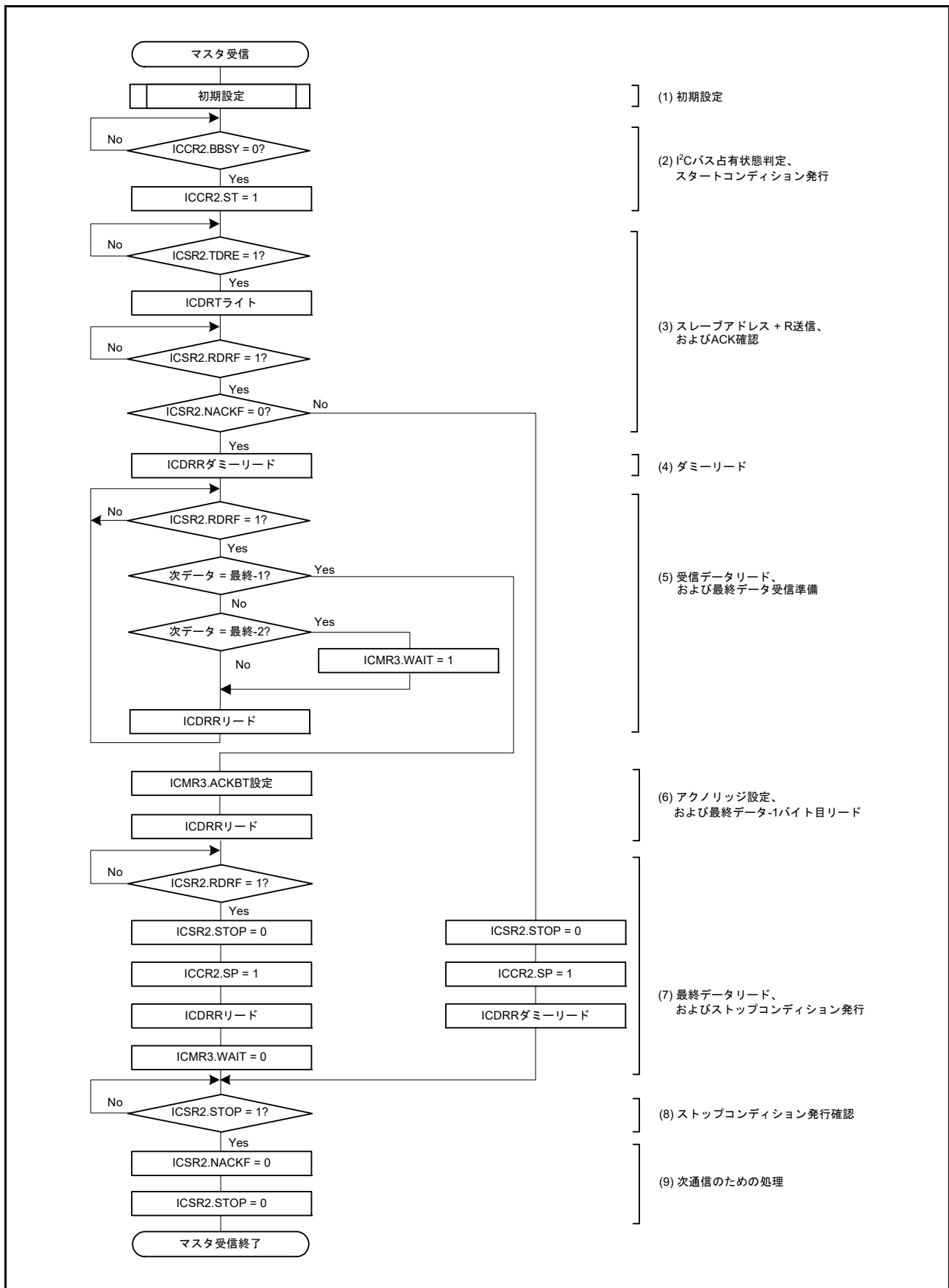
図 41.10 マスタ受信のフローチャート例 (7 ビットアドレスフォーマット、3 バイト以上の場合)
