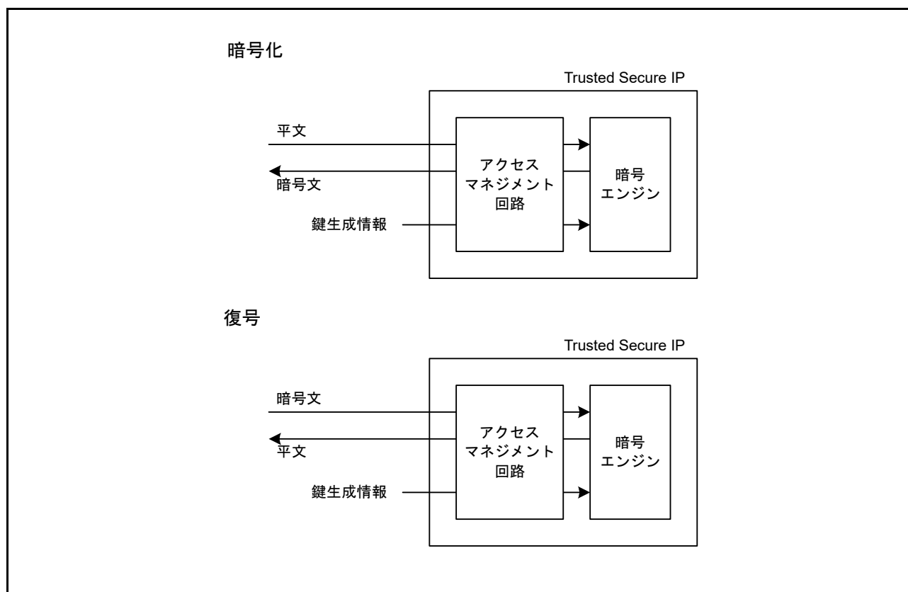
図 53.3 暗号エンジン概念図
