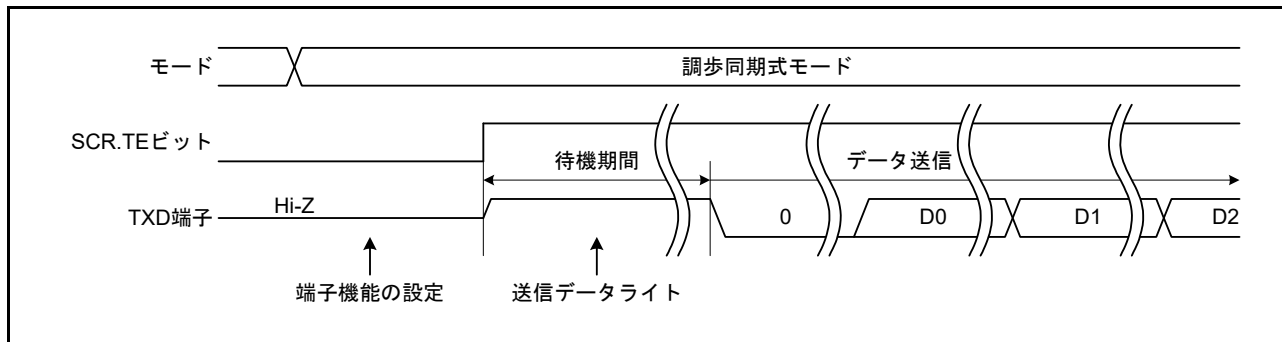
図 40.13 調歩同期式モード時のデータ送信タイミング例
