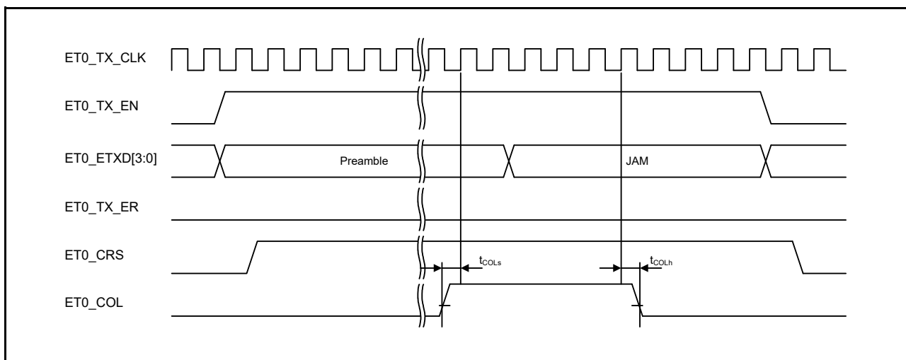
図 61.87 MII 送信タイミング (衝突発生ケース)
