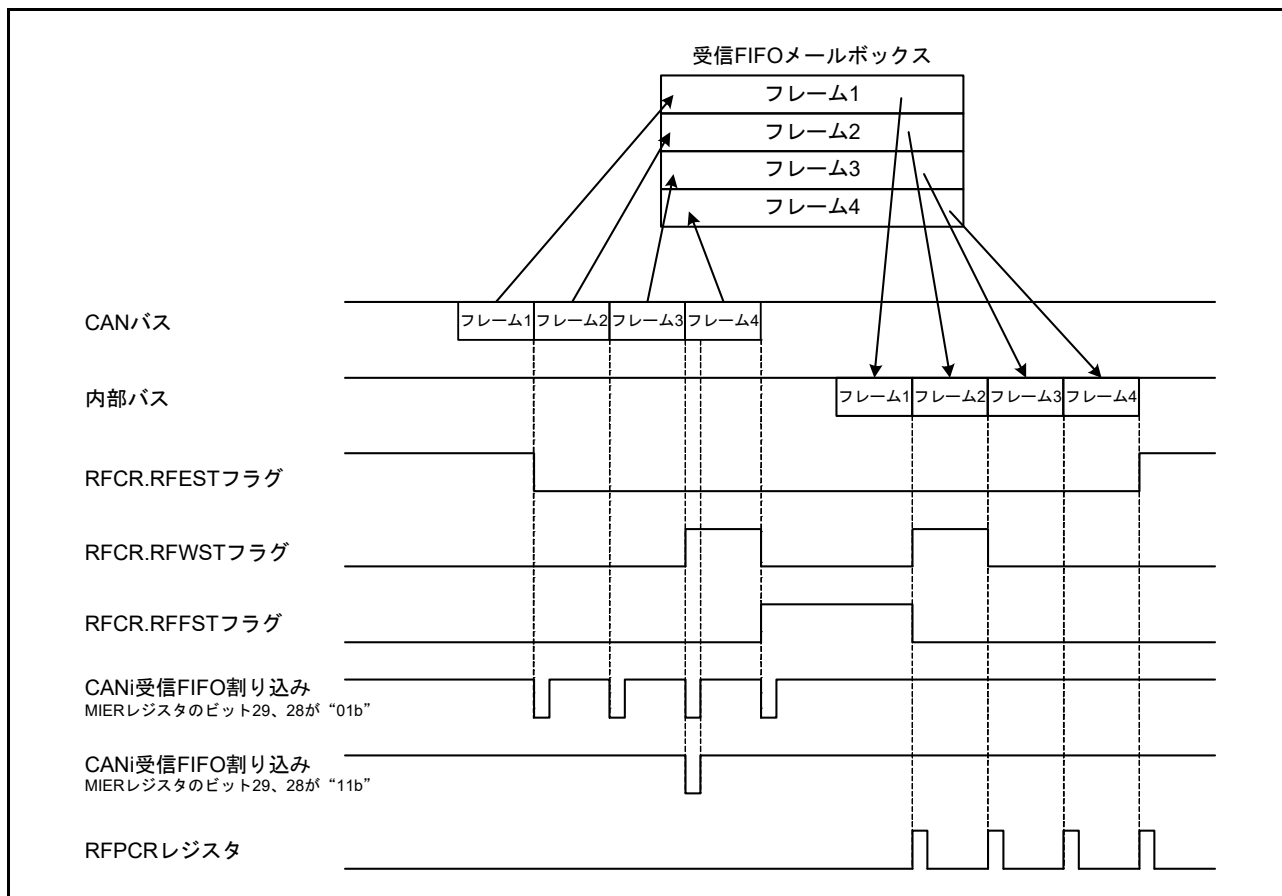
図 42.2 受信 FIFO メールボックスの動作 (MIER レジスタのビット 29、28 が "01b" または "11b")
