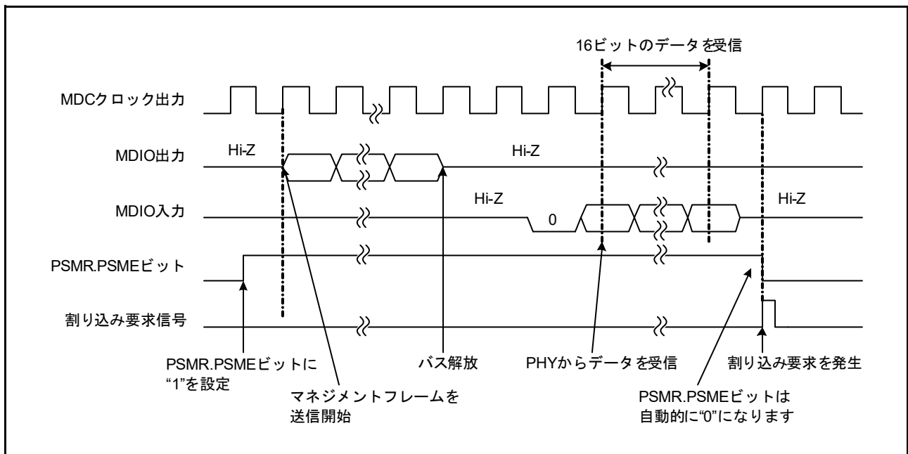
図 38.6 PHYレジスタリードの動作例
