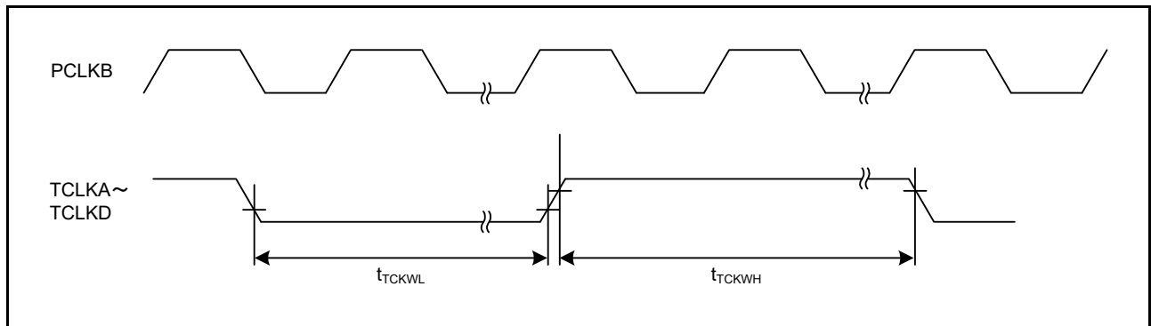
図 61.37 TPU クロック入力タイミング
