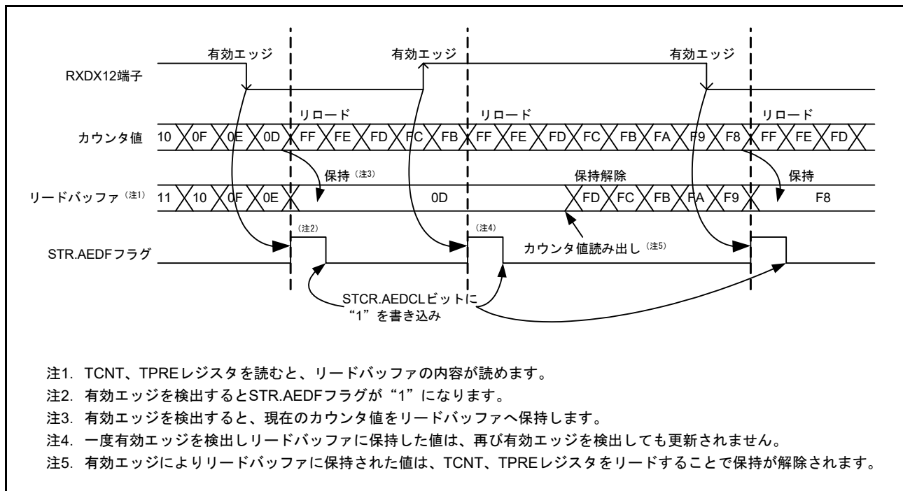
図 40.75 ビットレート測定機能動作例
