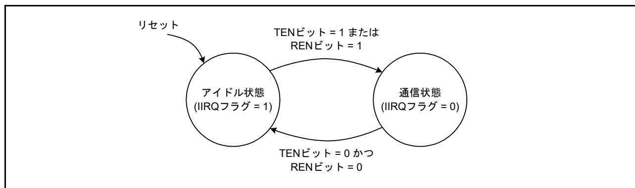
図 46.20 SSIE の状態遷移
