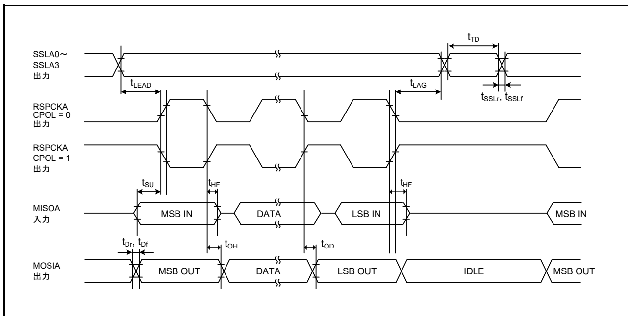
図 61.65 RSPi タイミング ( マスタ、CPHA = 0 ) ( ビットレート : PCLKA を 2 分周に設定 )
