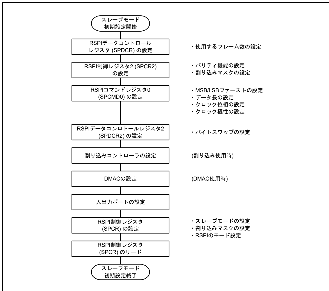
図 43.49 スレーブモード時の初期化フロー例 (クロック同期式動作)
