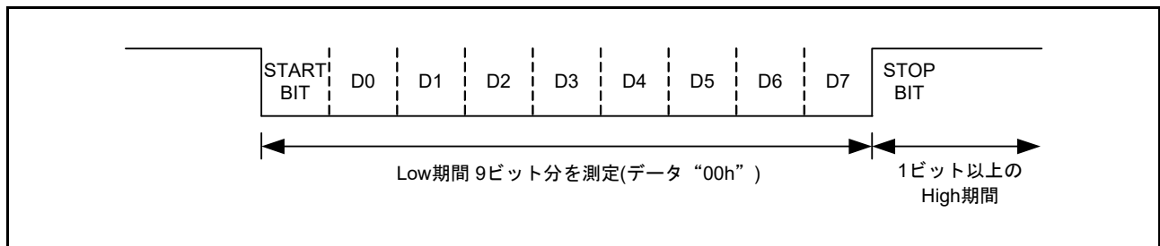
図 60.41 ビットレート自動調整時の SCI 送受信フォーマット
