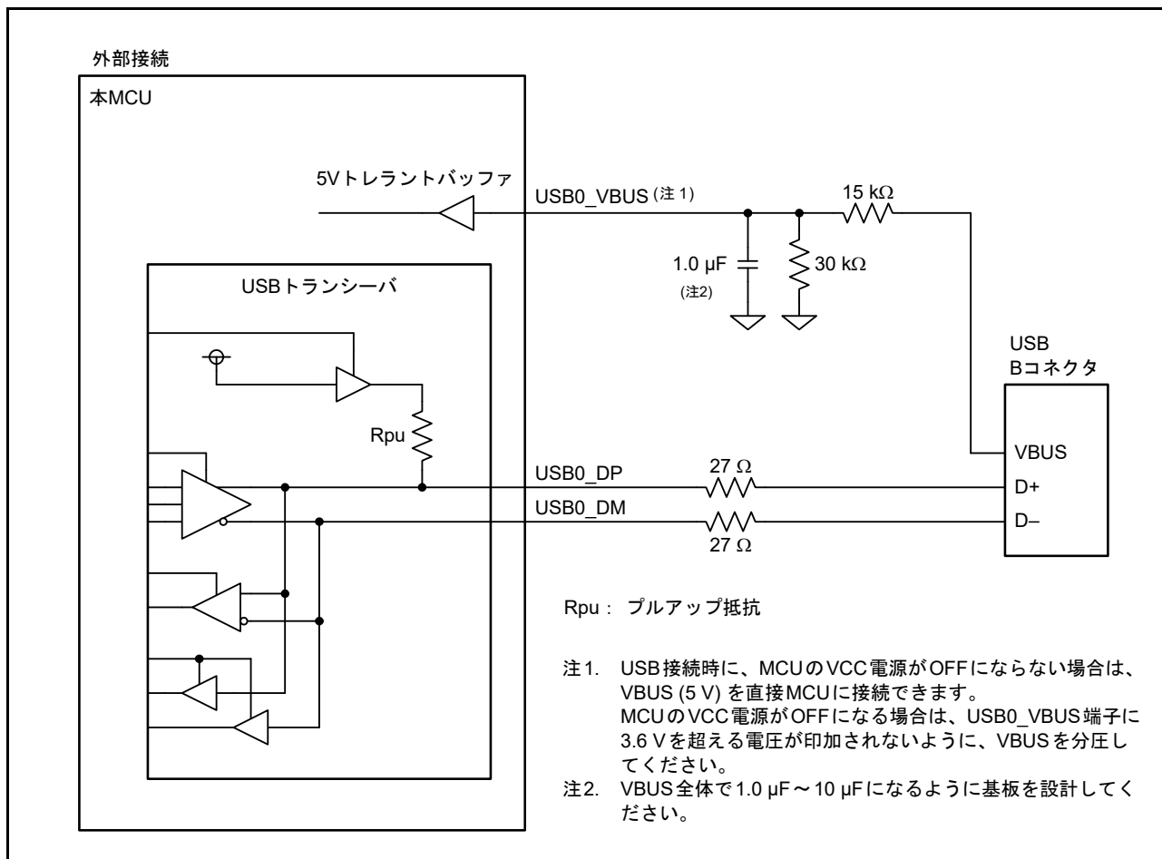
図 39.3 セルフパワー時のファンクションコントローラと USB コネクタとの接続例
