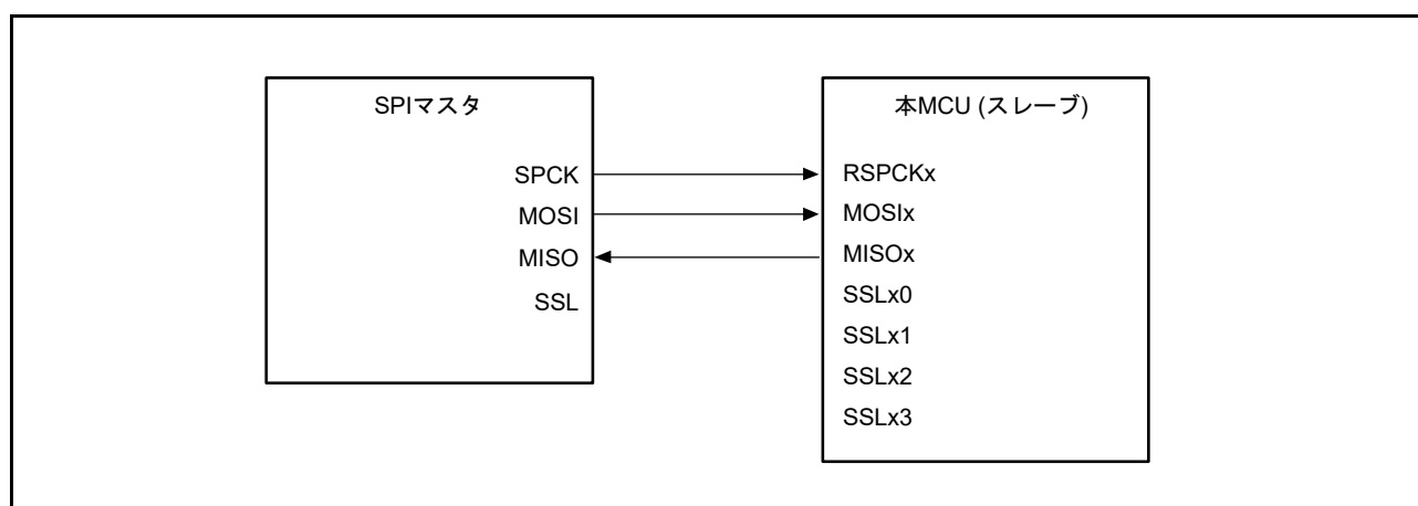
図 43.12 マスタ (クロック同期式動作) / スレーブ (クロック同期式動作) の構成例 (本 MCU = スレーブ、CPHA = 1)
