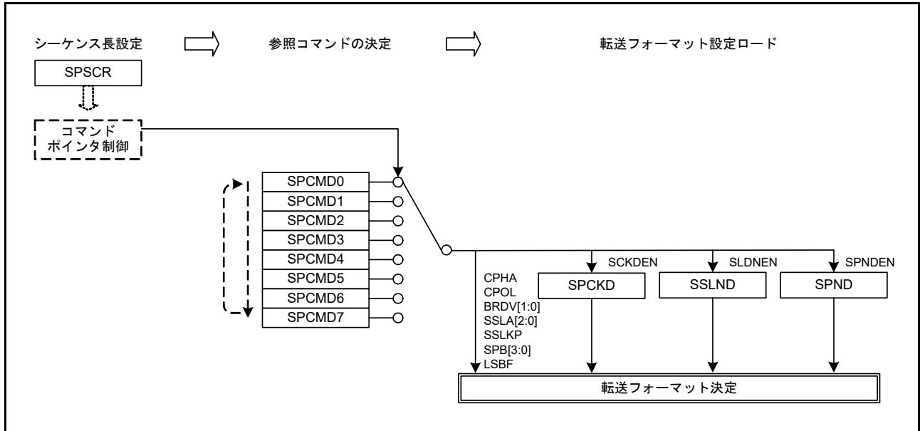
図 43.45 マスタモードでのシリアル転送方式の決定方法
