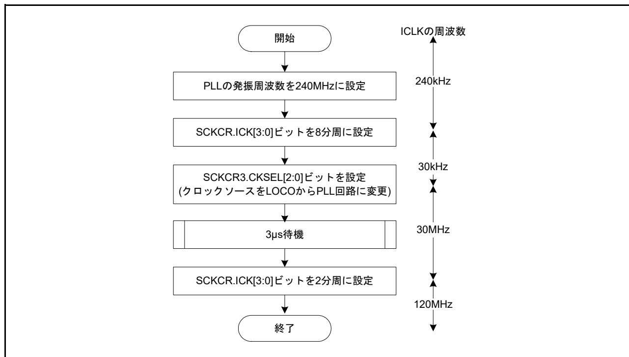
図 9.14 ICLK を LOCO クロック (240kHz) から PLL クロック (240MHz) の 2 分周設定で 120MHz に変更する変更手順例
