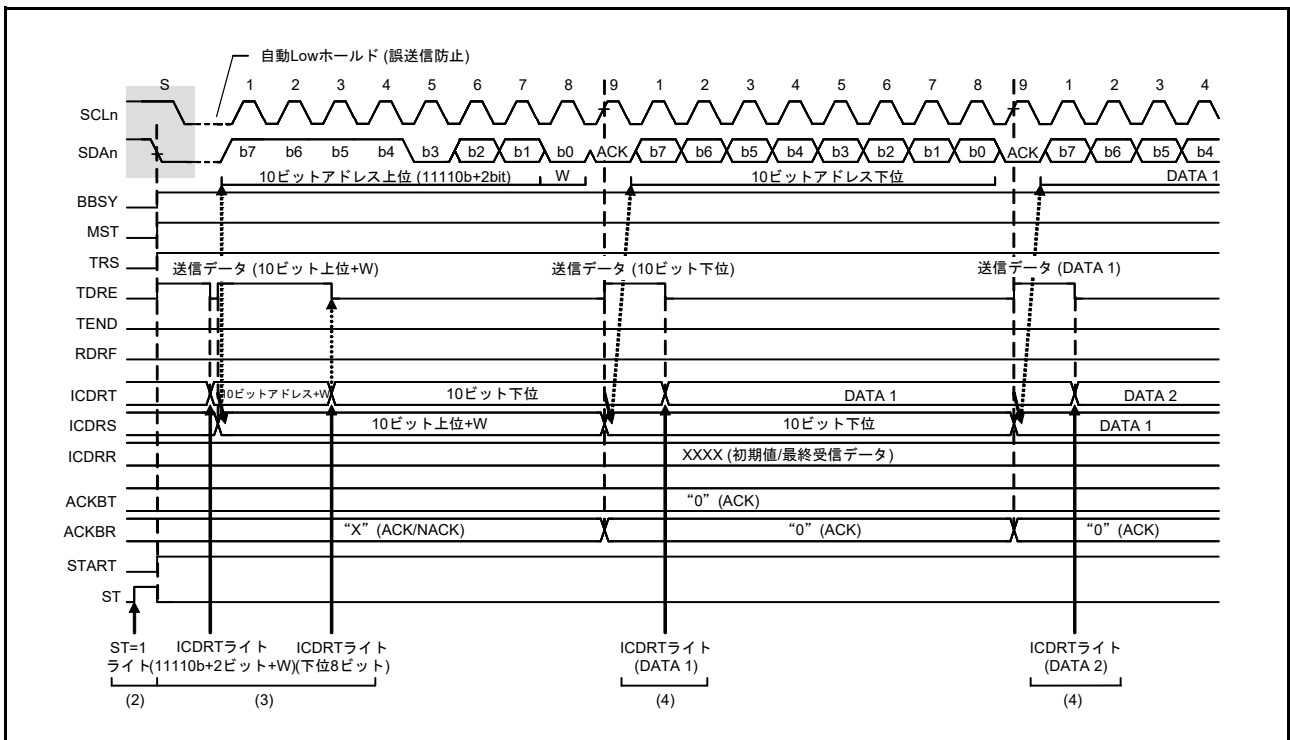
図 41.7 マスタ送信の動作タイミング (2) (10 ビットアドレスフォーマットのとき)
