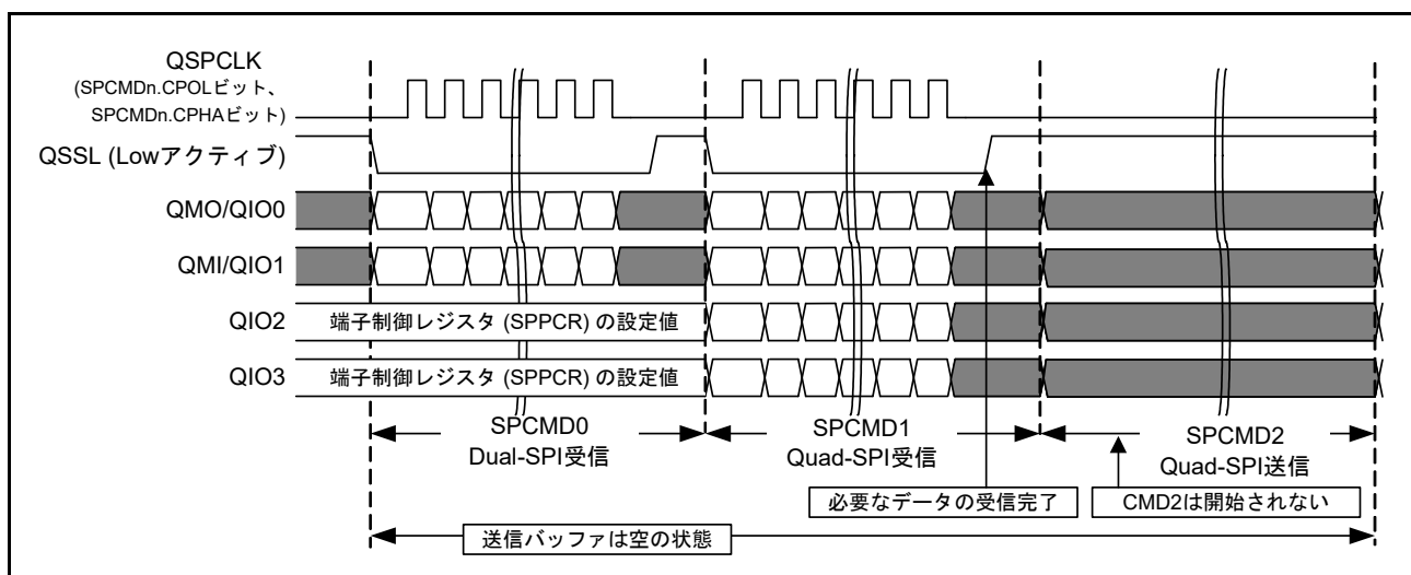
図 44.20 転送モードを切り替えたシーケンス構成の例 (n = 0 ~ 3) (シーケンスを構成するコマンドがすべて Dual/Quad-SPI リード動作である場合の終了方法 (b))
