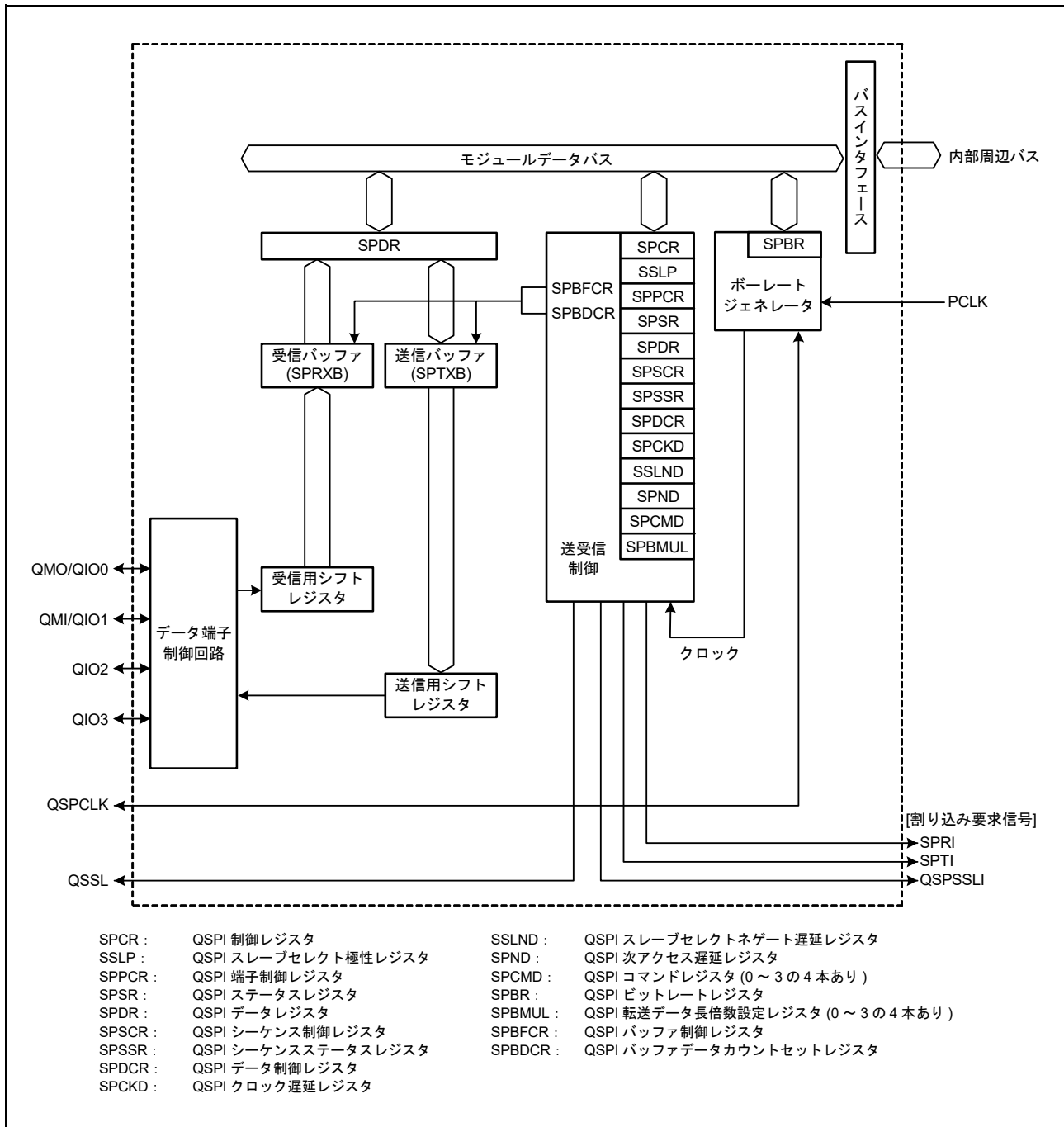
図 44.1 QSPI のブロック図
