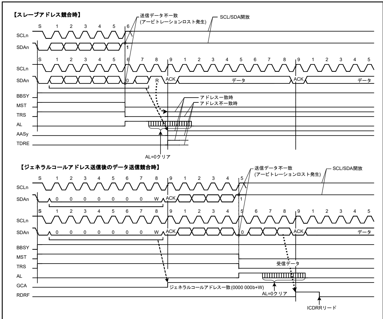
図 41.32 マスターアービトレーションロスト検出動作例 (MALE ビット = 1 のとき)
