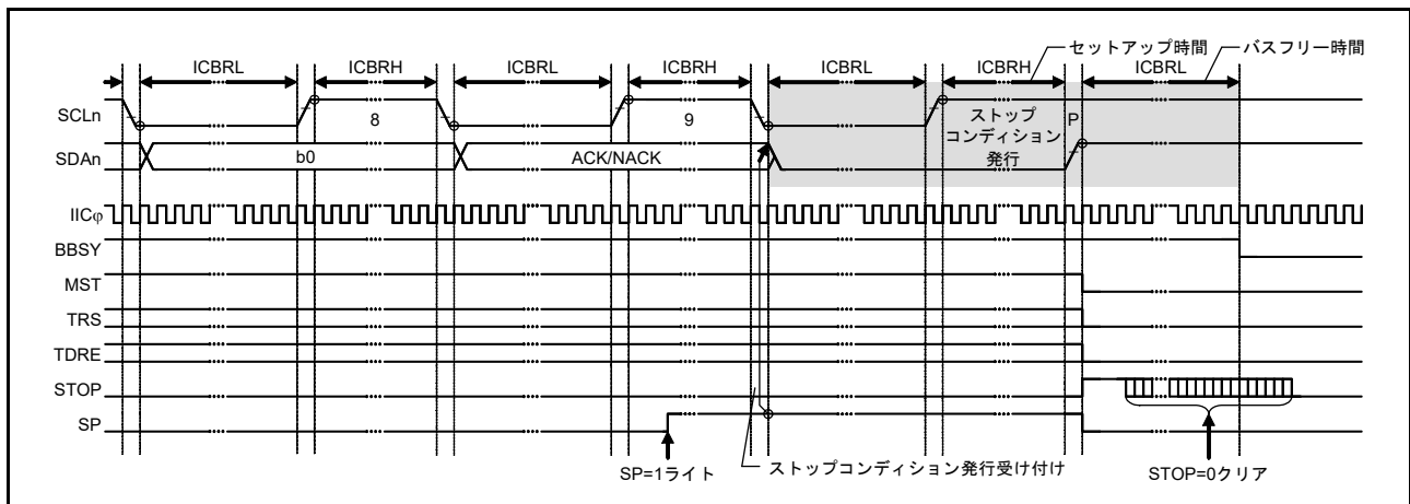
図 41.37 ストップコンディション発行動作タイミング (SP ビット)
