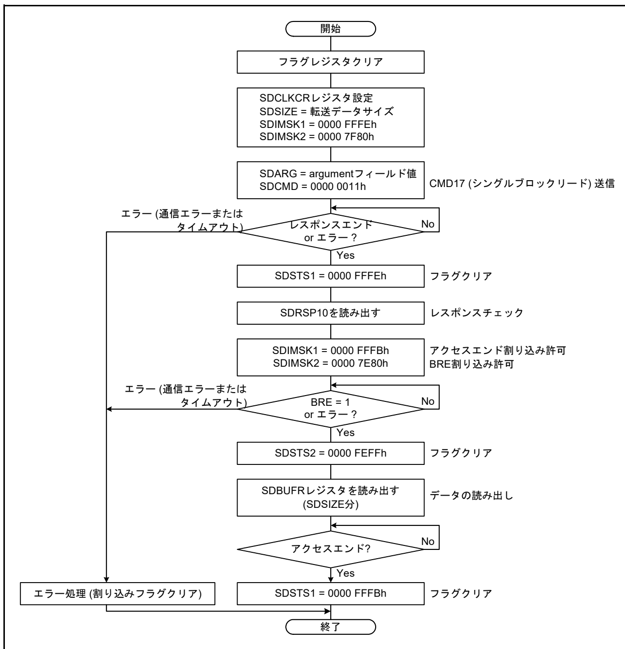
図 47.10 シングルブロックリードコマンドの送信例
