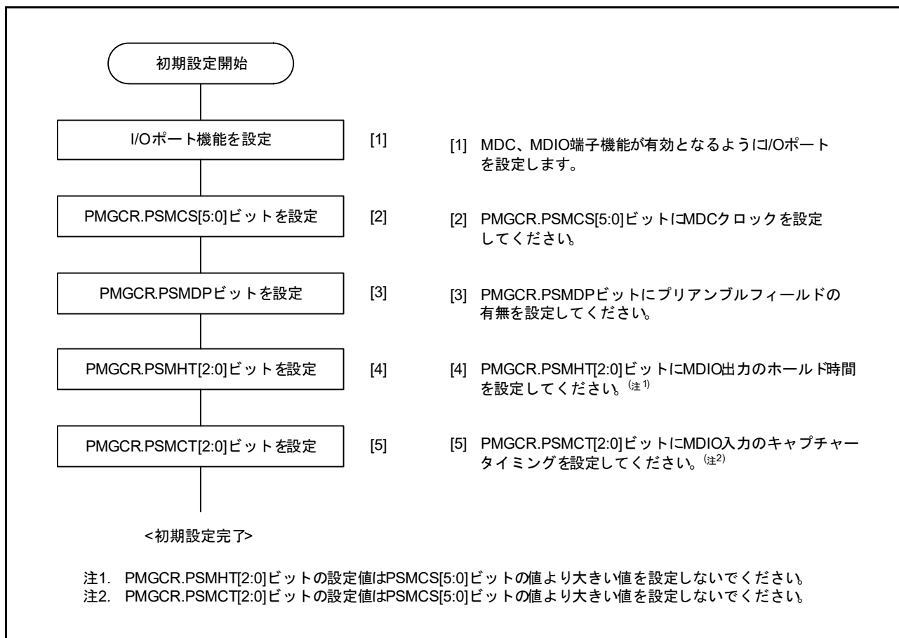
図 38.4 PMGI の初期設定フローチャートの例
