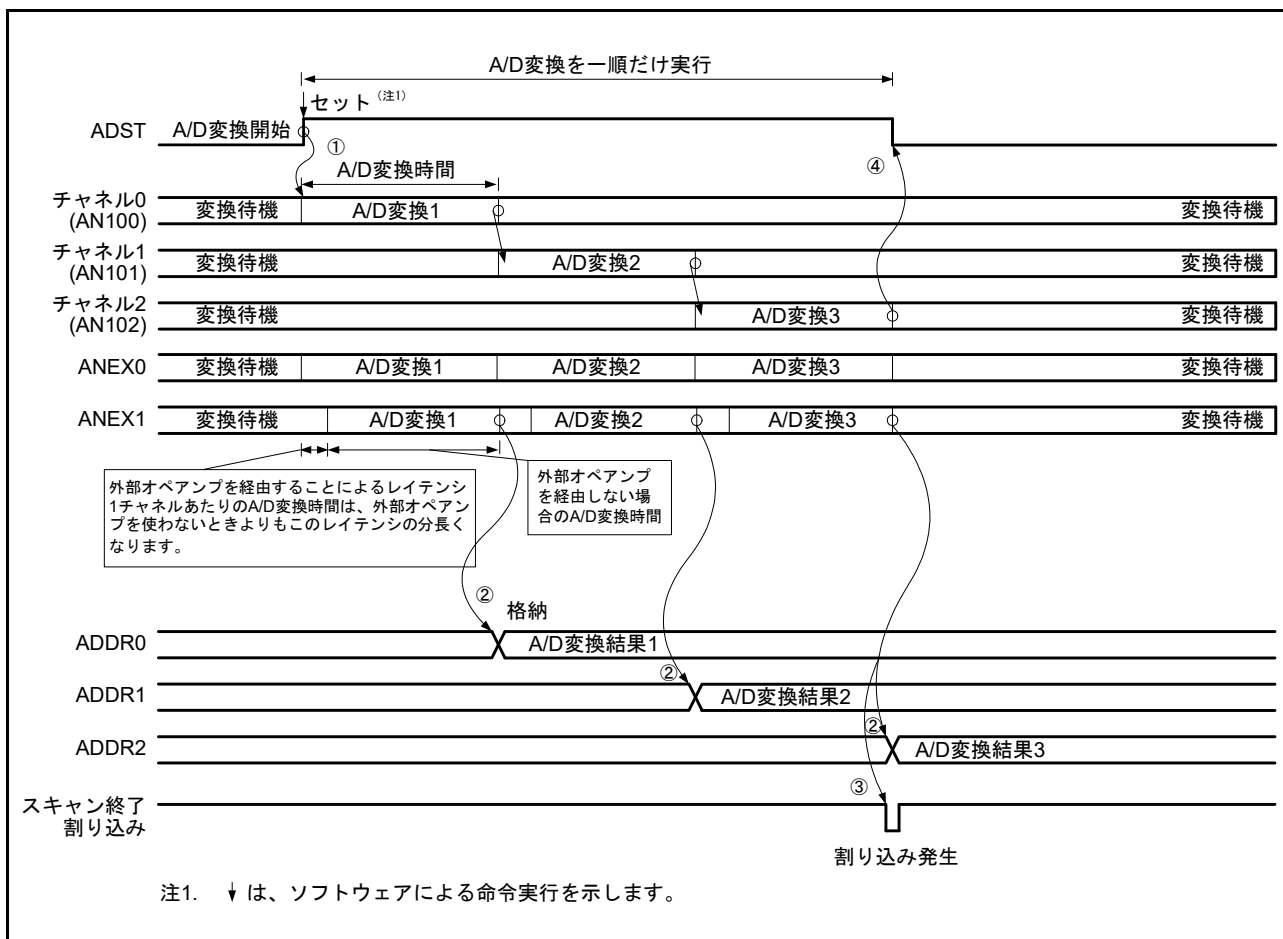
図 54.36 ANEX1 入力の動作例 (シングルスキャンモード)
