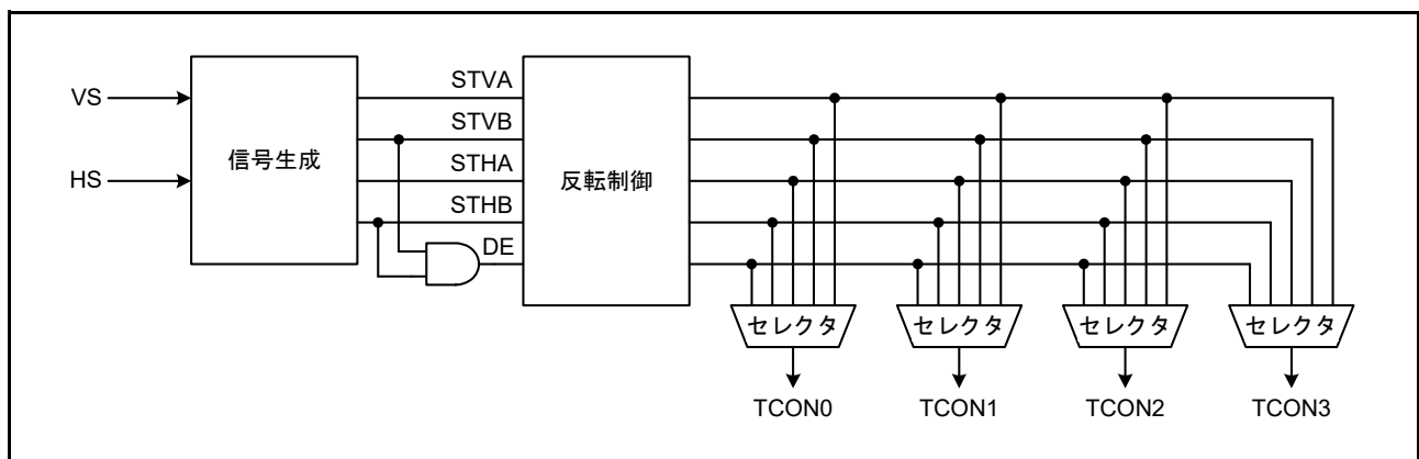
図 50.18 反転制御と出力信号選択部の構成
