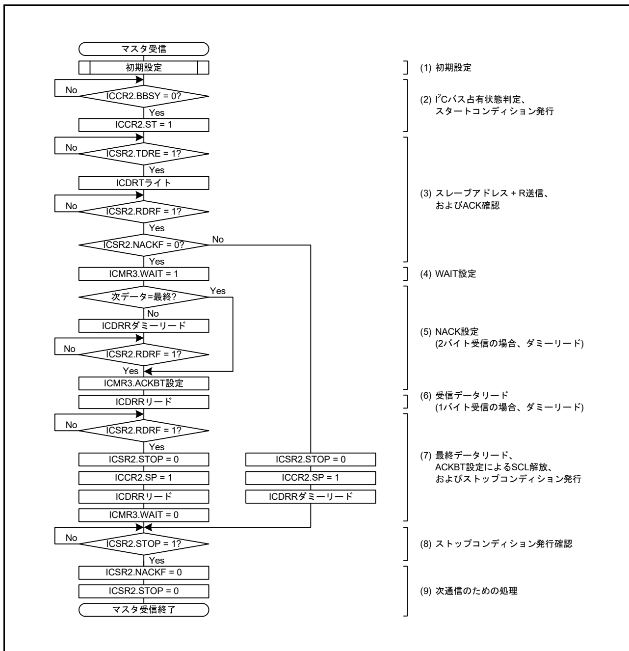
図 41.9 マスタ受信のフローチャート例 (7 ビットアドレスフォーマットの場合、2 バイト以下の場合)
