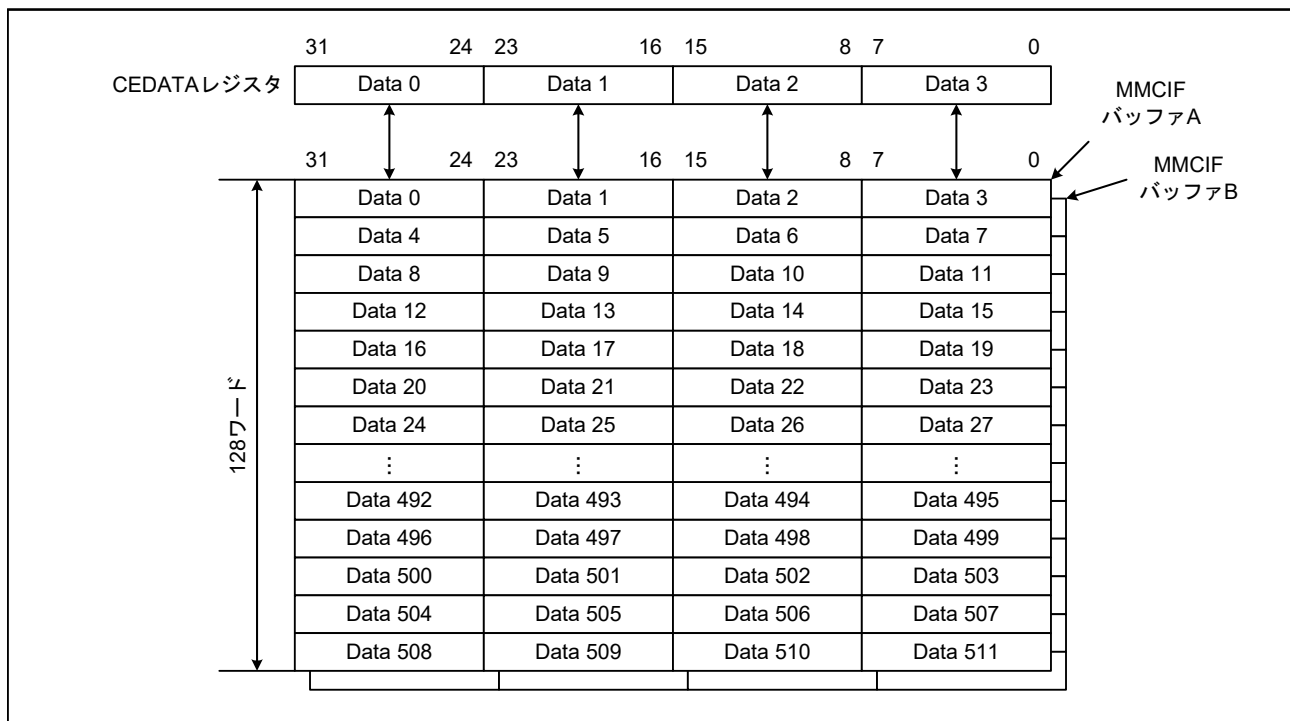
図 48.6 MMCIF バッファの構成 (32 ビットアクセス)
