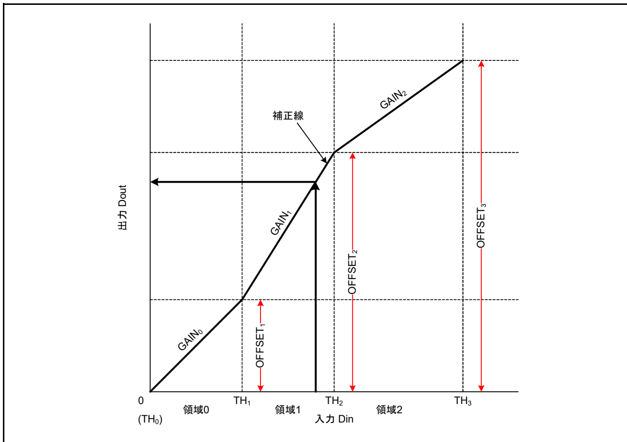
図 50.11 ガンマ補正値の計算
