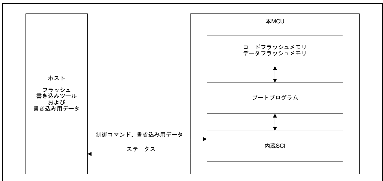
図 60.34 ブートモード (SCI インタフェース) 時のシステム構成
