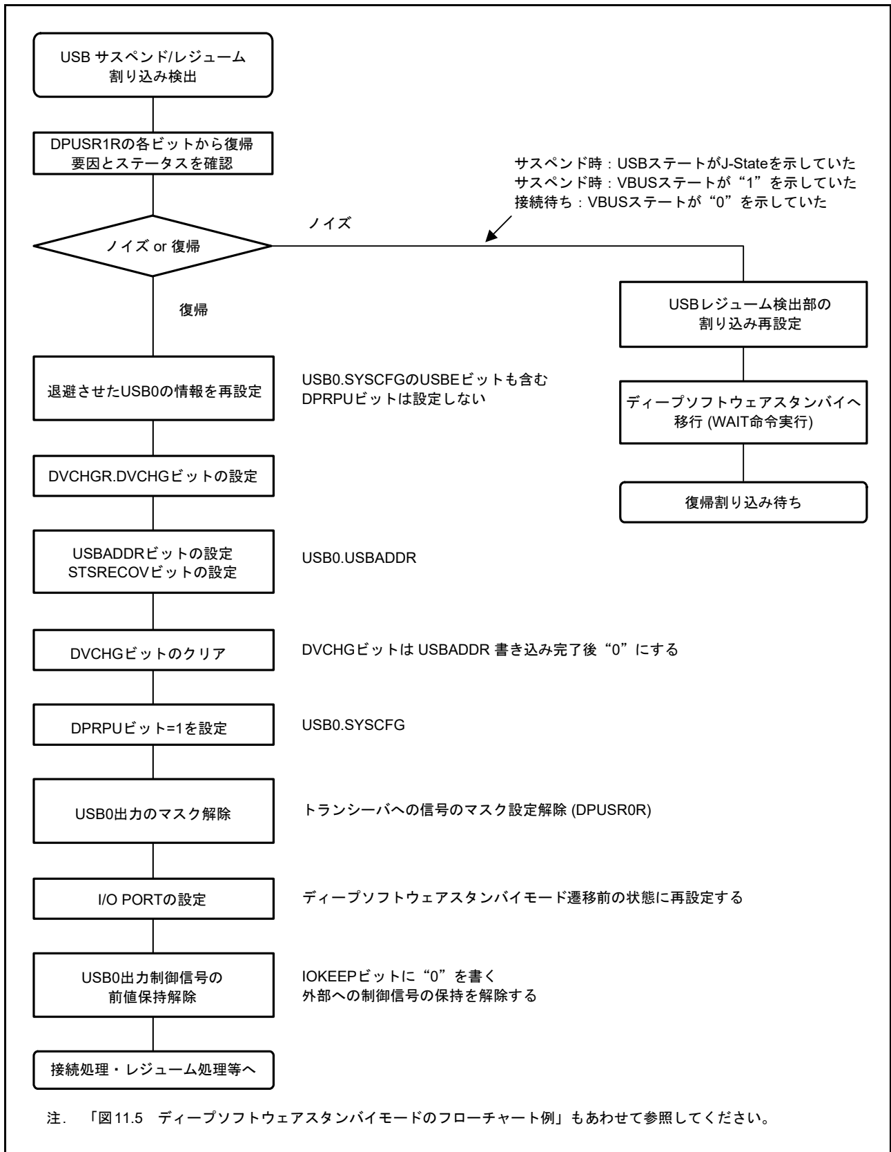
図 39.9 ファンクション時のディープソフトウェアスタンバイ解除時の USB 設定フロー
