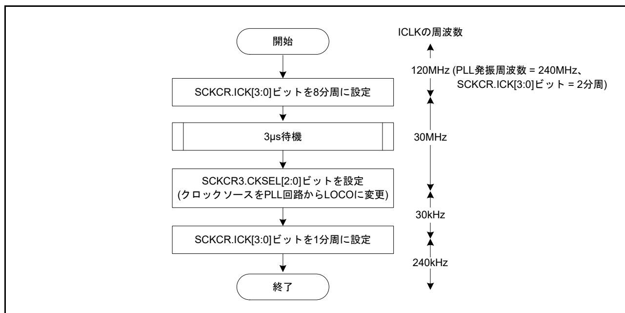
図 9.15 ICLK を PLL クロック (240MHz) の 2 分周設定で 120MHz から LOCO クロック (240kHz) に変更する変更手順例
