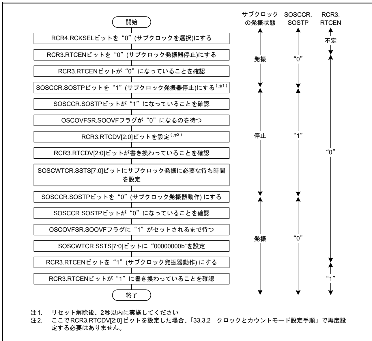
図 9.11 サブクロックをリアルタイムクロックのカウンタソースに使用する場合の初期化フローチャート例
