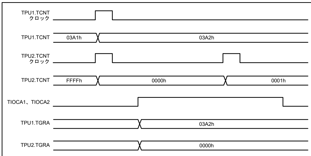
図 28.18 カスケード接続動作例 (1)
