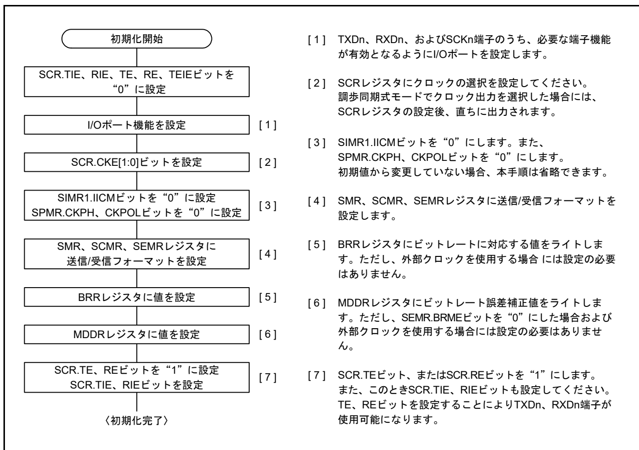
図 40.11 SCIの初期化フローチャートの例 (調歩同期式モード) (SCI0 ~ SCI6, SCI12)
