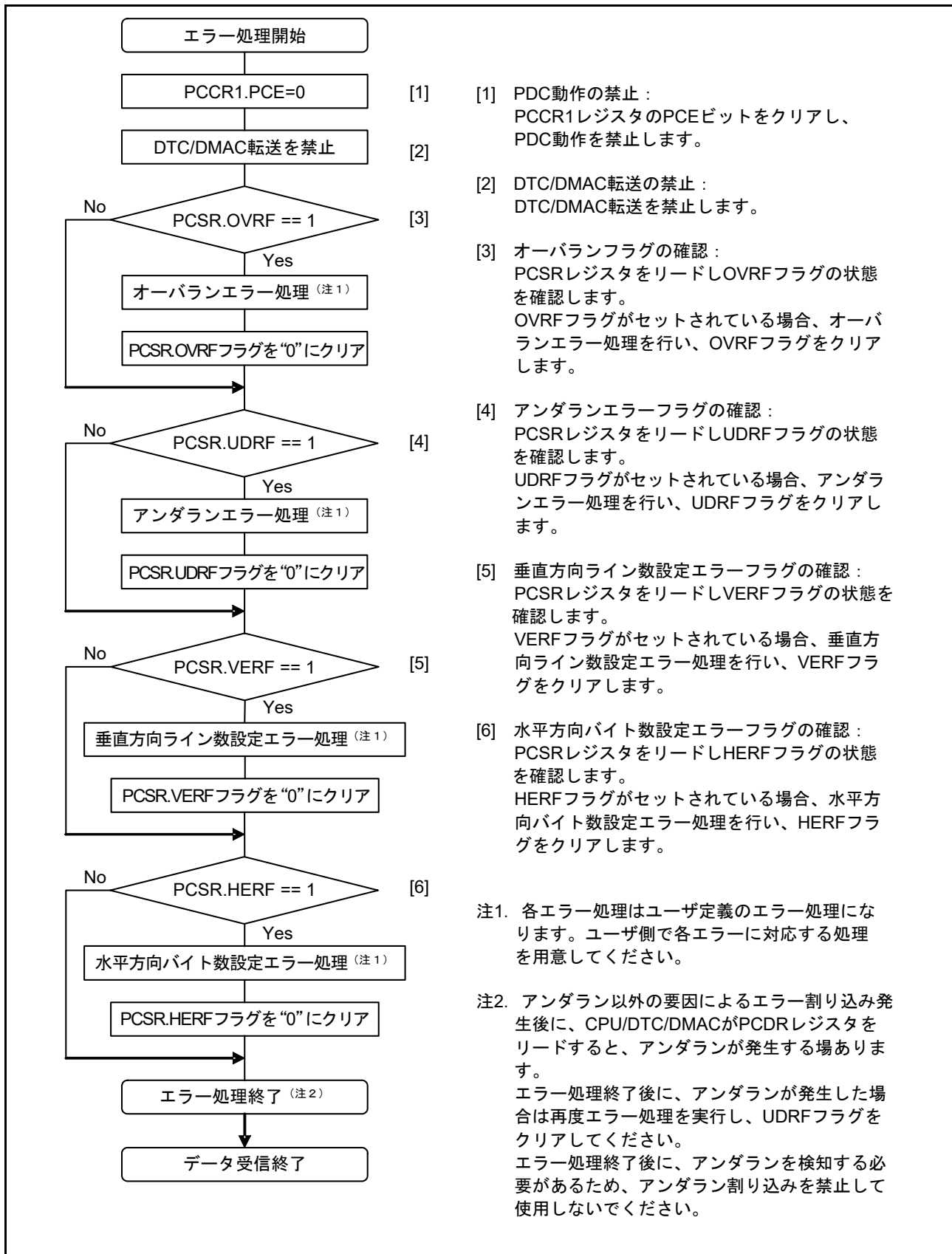
図 49.20 エラー処理フロー例
