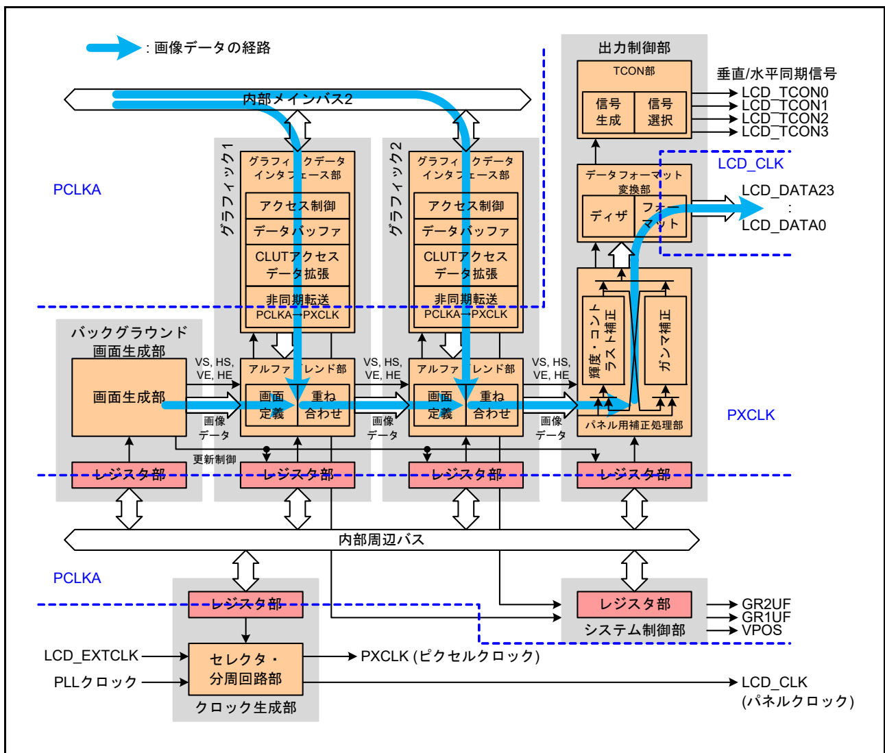
図 50.20 GLCDC の構成
