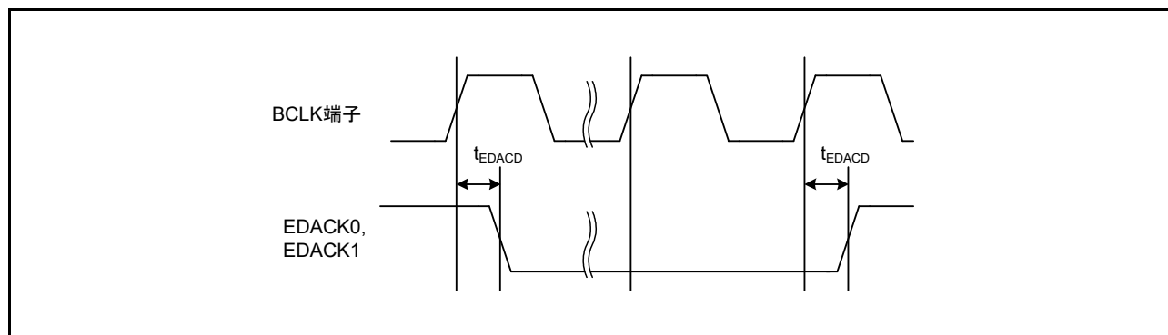
図 61.33 EDACK0、EDACK1 シングルアドレス転送タイミング (CS 領域)
