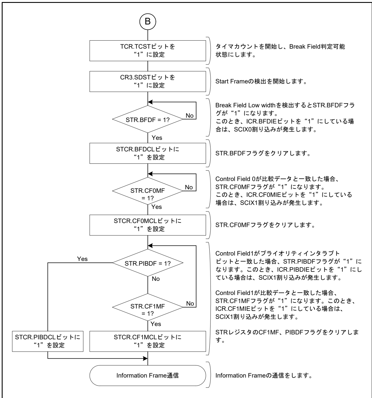
図 40.70 Start Frame 受信フローチャート例 (2)
