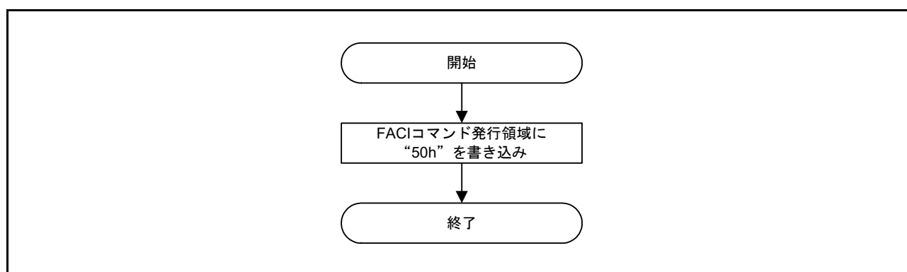
図 60.22 ステータスクリアコマンドの使用方法
