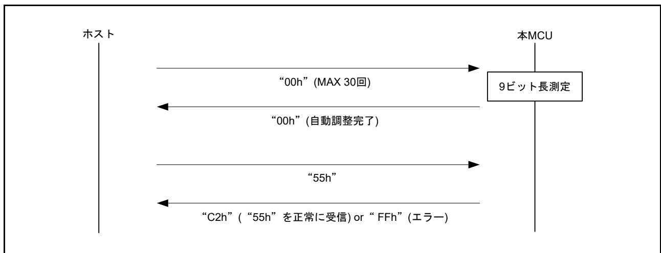
図 60.42 ホストと本 MCU 間の通信シーケンス
