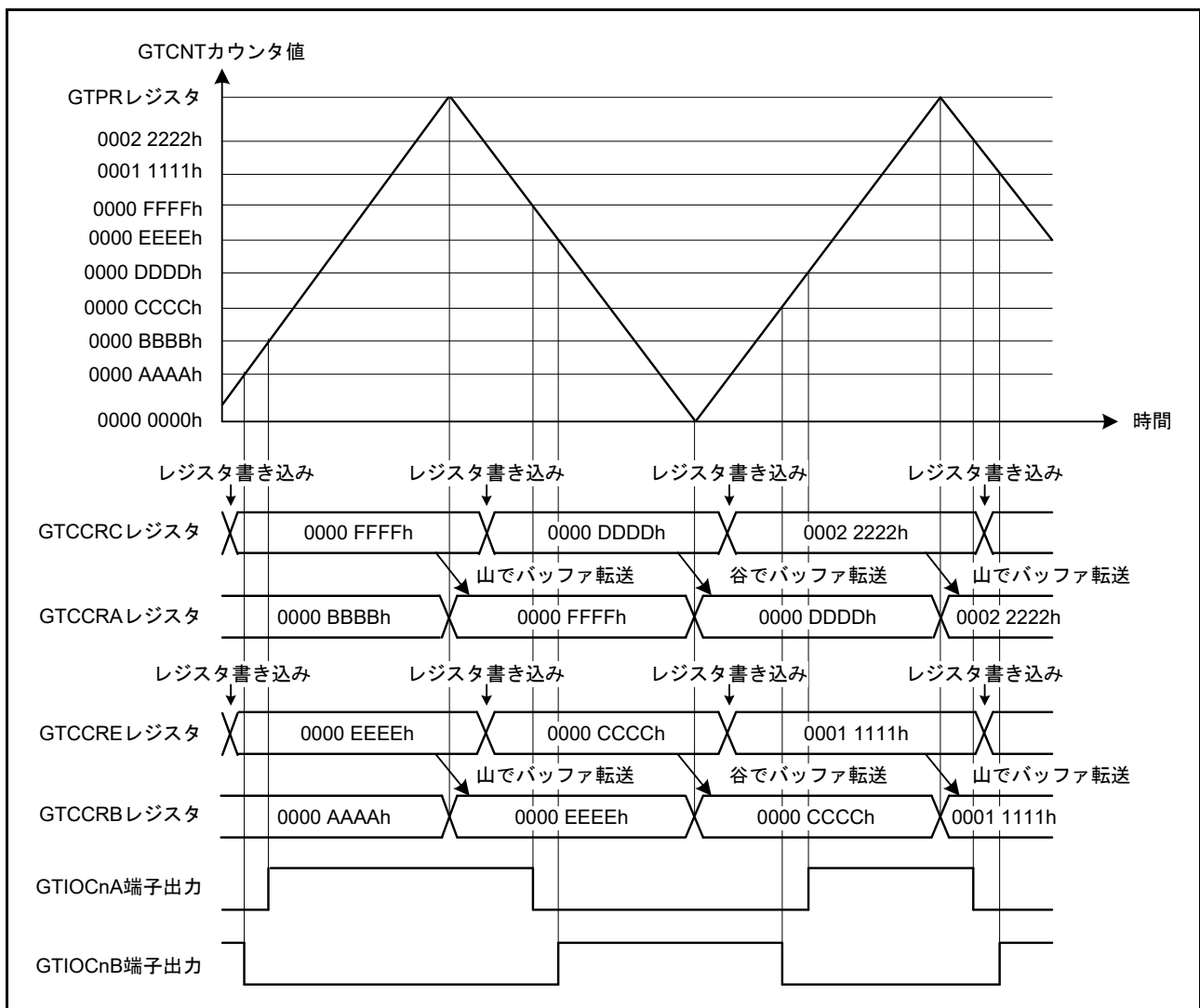
図 26.43 三角波 PWM モード 2 動作例 (バッファ動作、初期出力で GTIOCnA 端子 = Low 出力 / GTIOCnB 端子 = High 出力、GTCCRA/GTCRB レジスタのコンペアマッチでトグル出力、周期の終わりで出力保持の場合) (n = 0 ~ 3)
