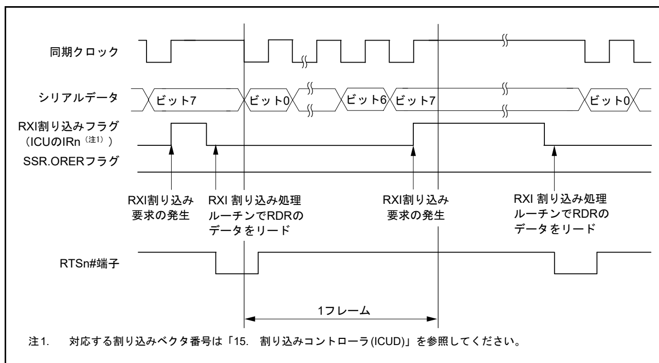
図 40.34 クロック同期式モードのシリアル受信時の動作例 (2) (RTS 機能使用時)
