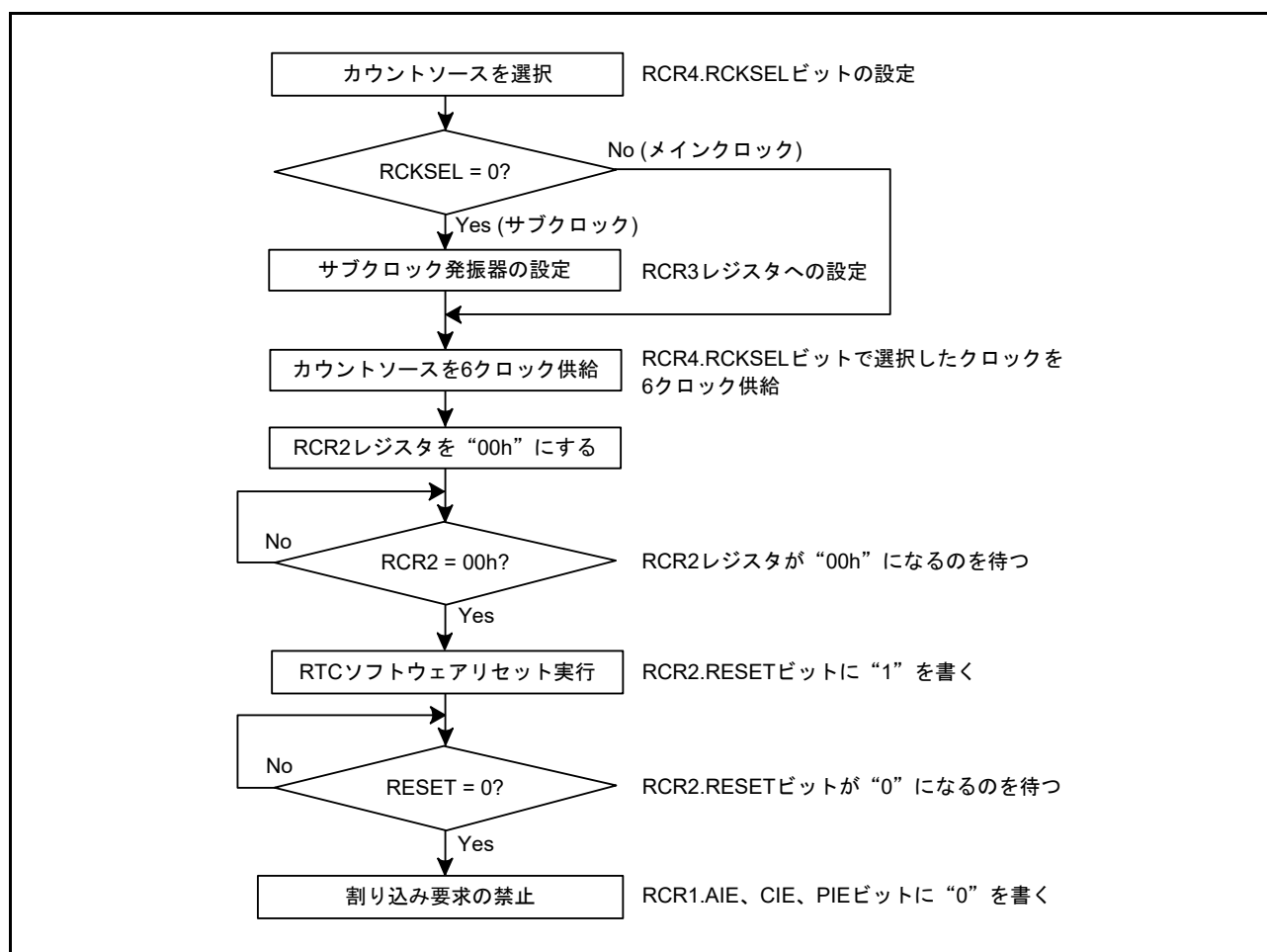
図 33.14 初期化手順
