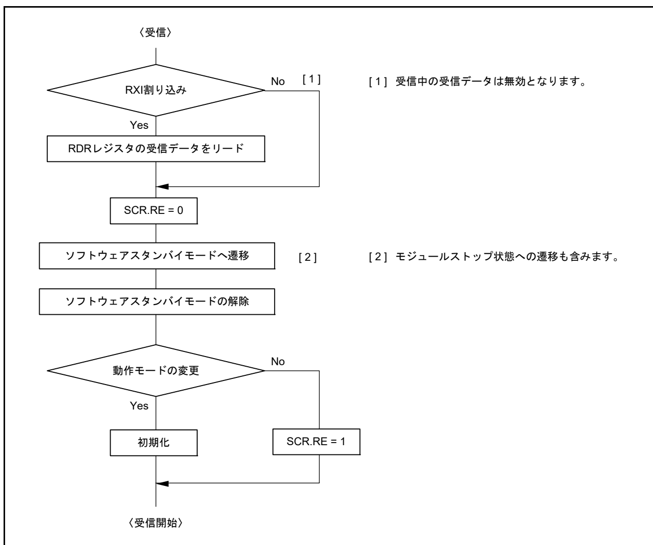
図 40.84 受信時のソフトウェアスタンバイモード遷移フローチャートの例
