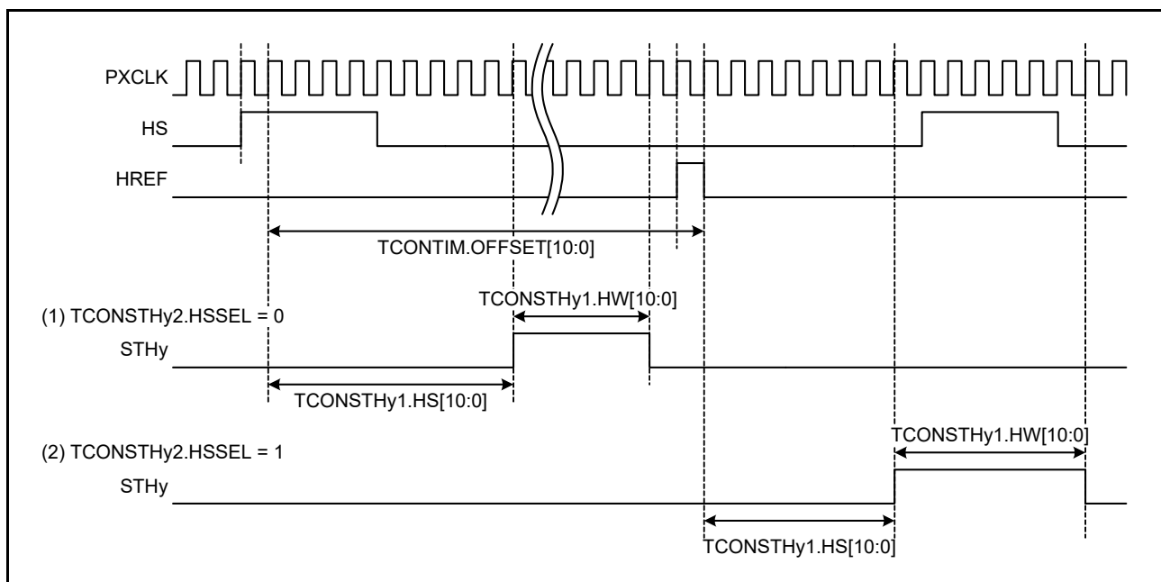
図 50.14 TCON 部における水平同期信号生成タイミング (y = A, B)
