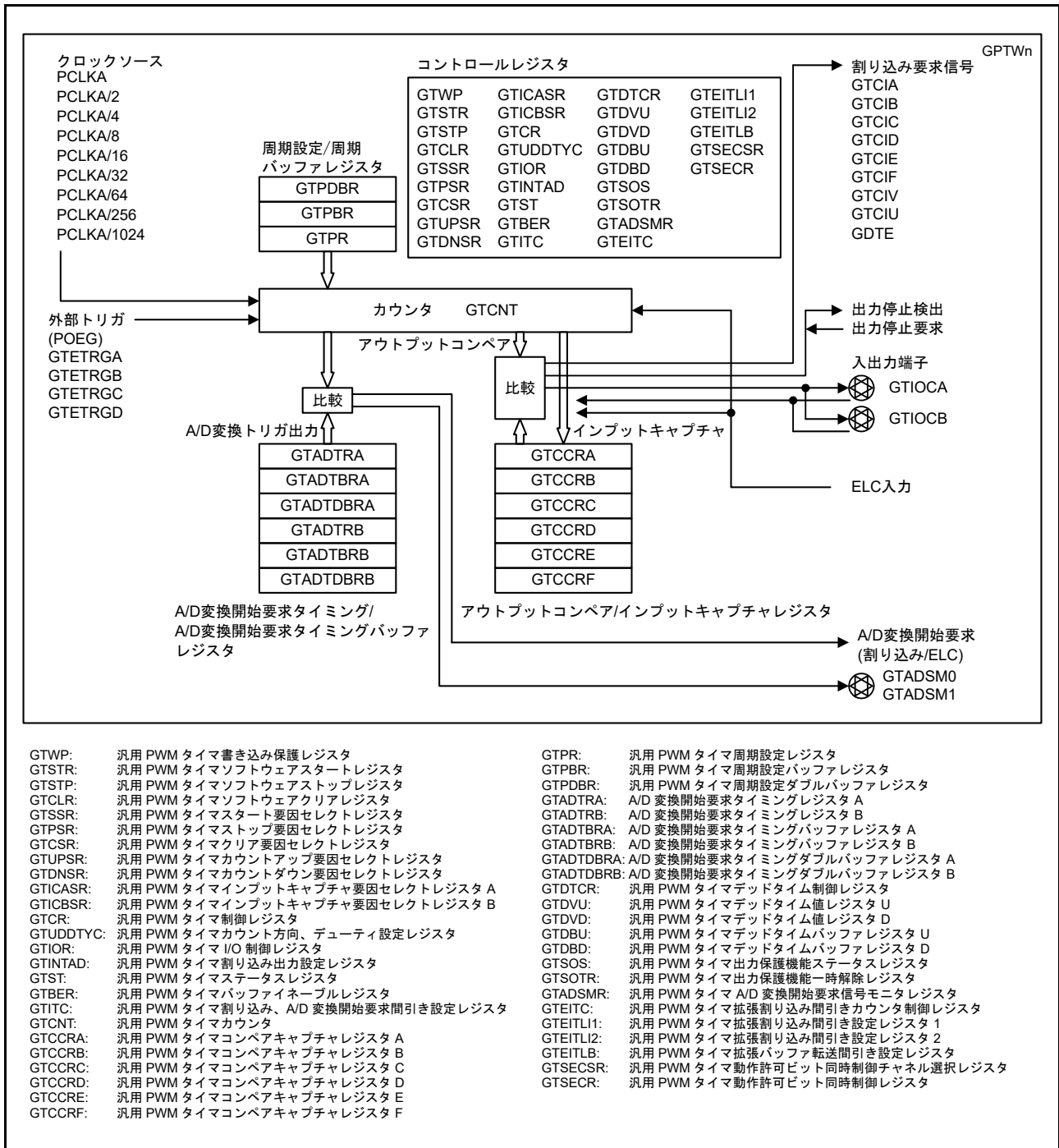
図 26.1 GPTW のブロック図 (n = 0 ~ 3)
