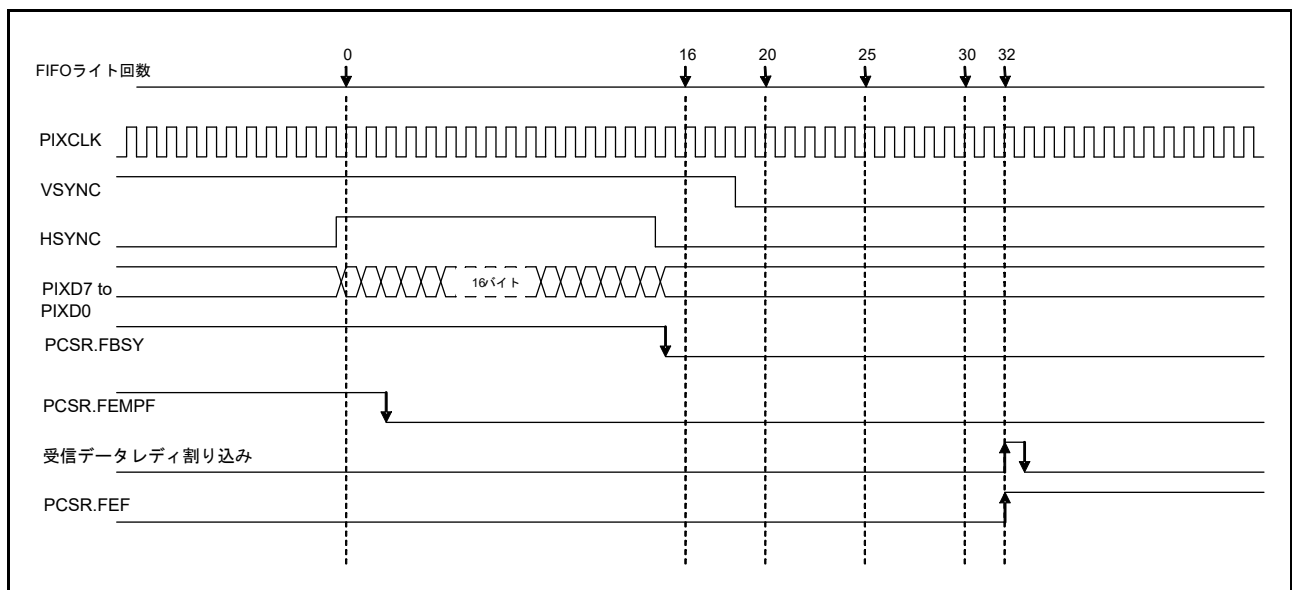
図 49.13 フレームエンド時の継続受信動作例
