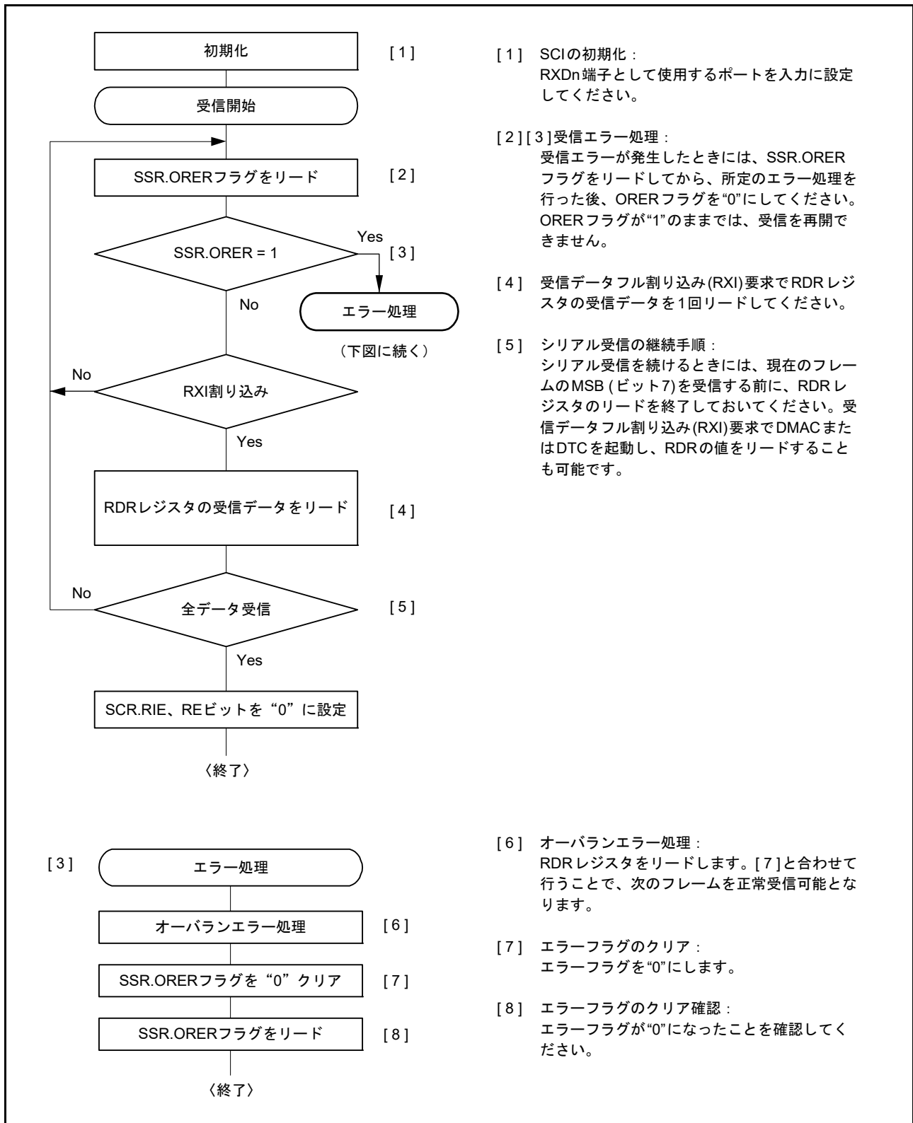
図 40.35 クロック同期式モードのシリアル受信のフローチャート例
