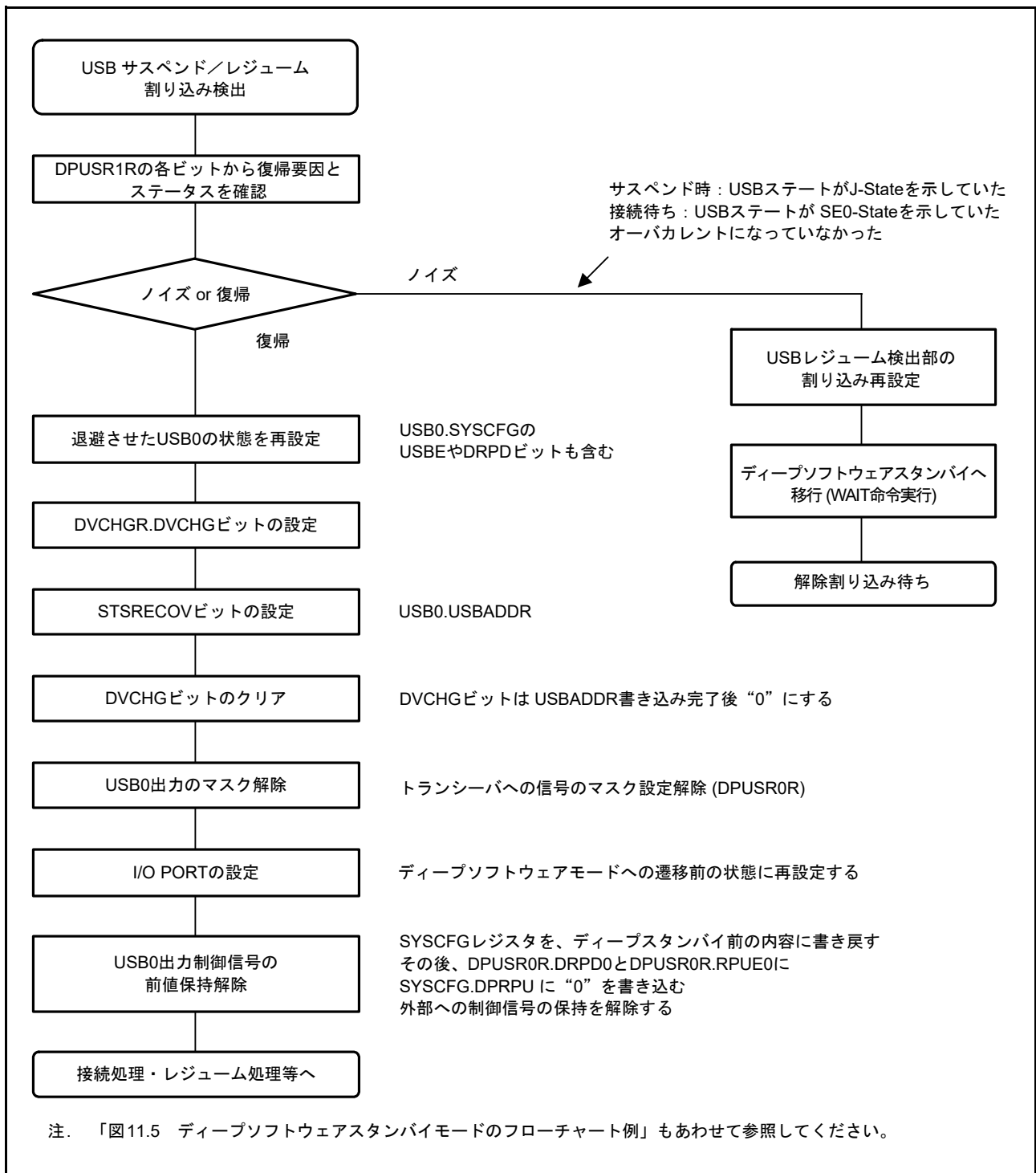
図 39.8 ホスト時のディープソフトウェアスタンバイ解除時の USB 設定フロー
