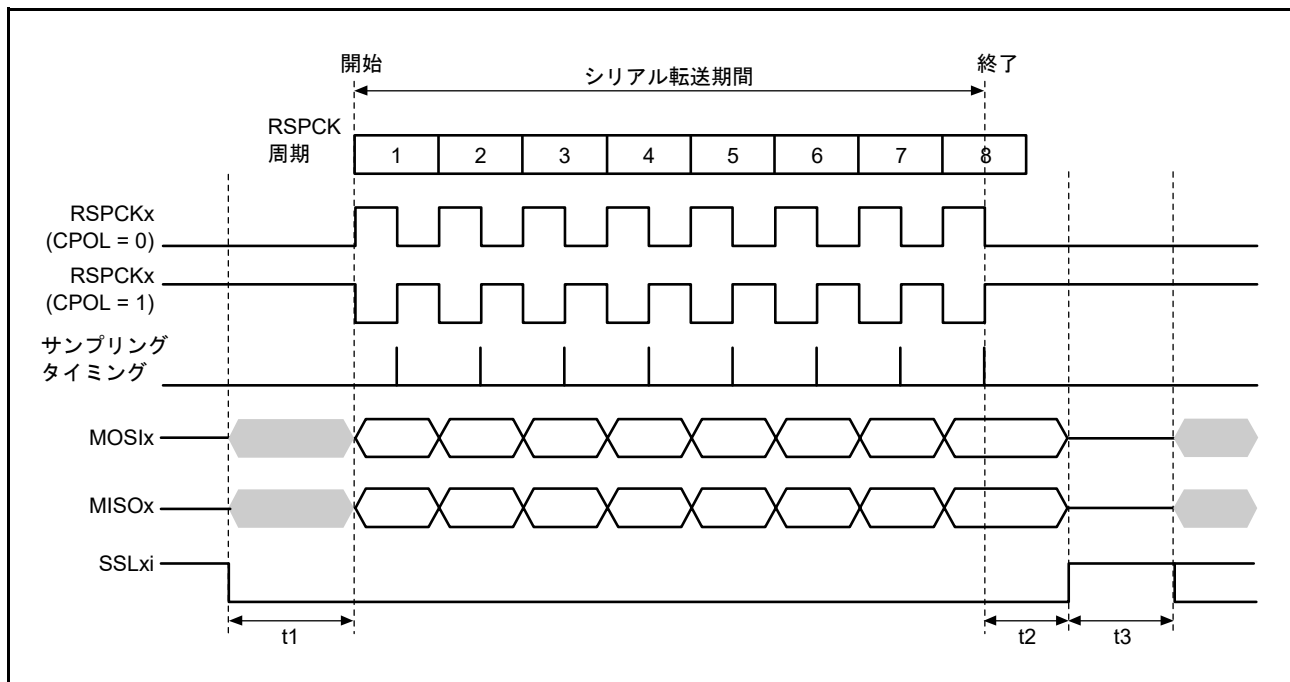
図 43.25 RSPI 転送フォーマット (CPHA ビット = 1)
