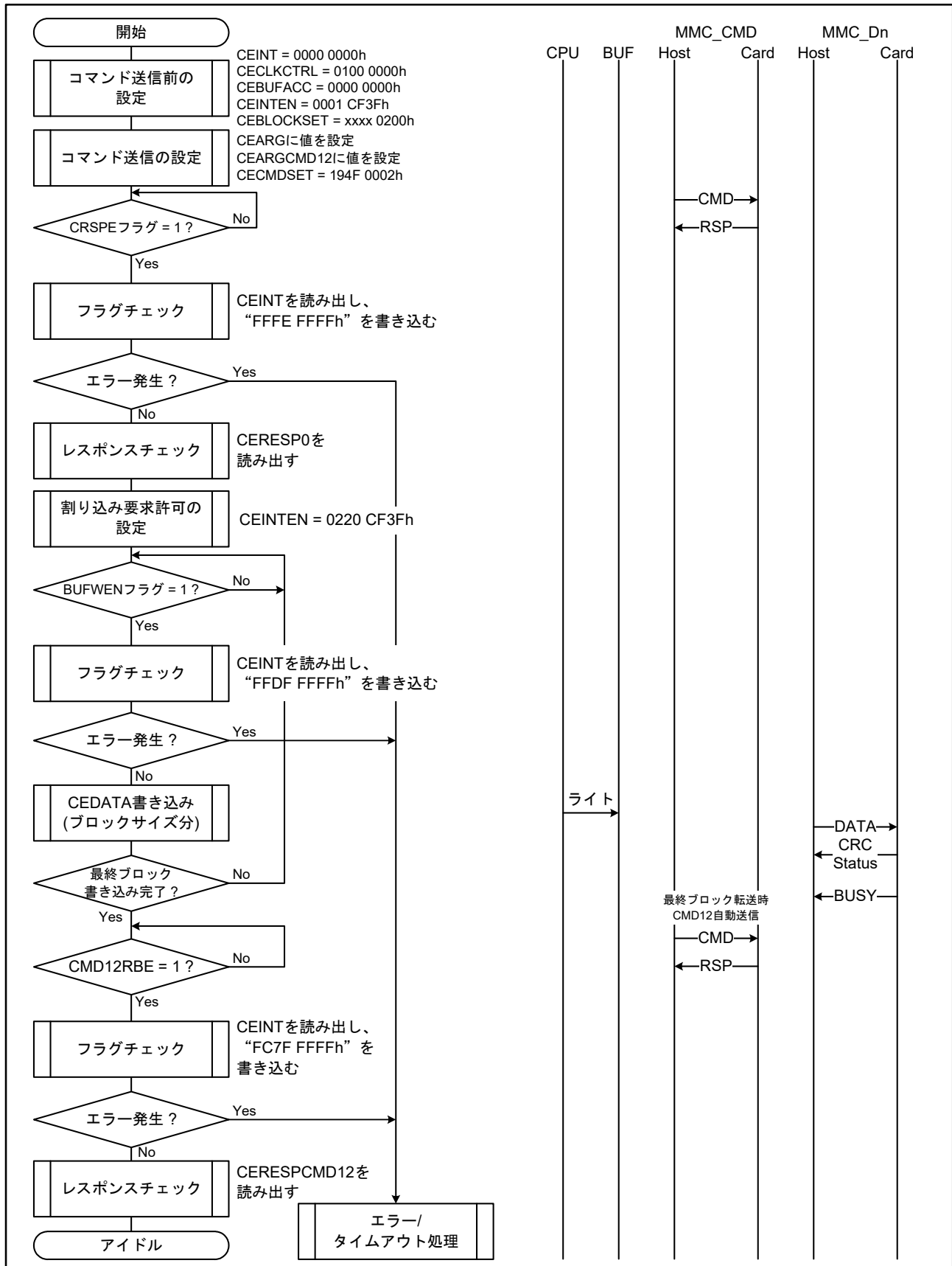
図 48.20 マルチブロックライトの送信例 (CMD25 Open-ended)
