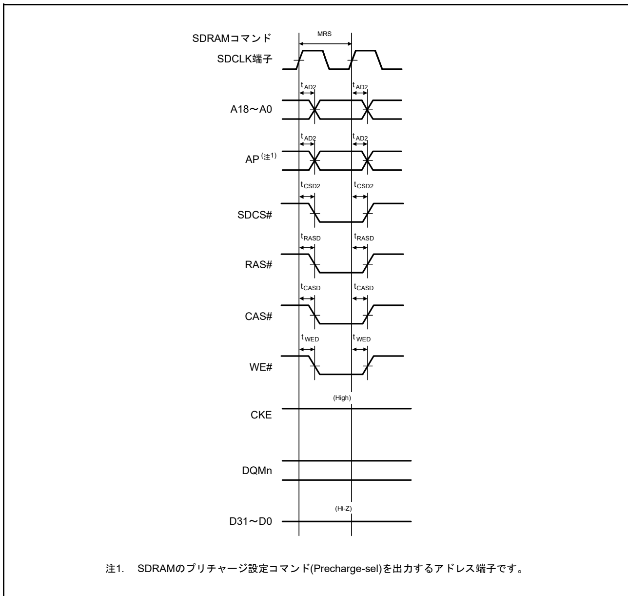
図 61.30 SDRAM 空間モードレジスタセットバスタイミング
