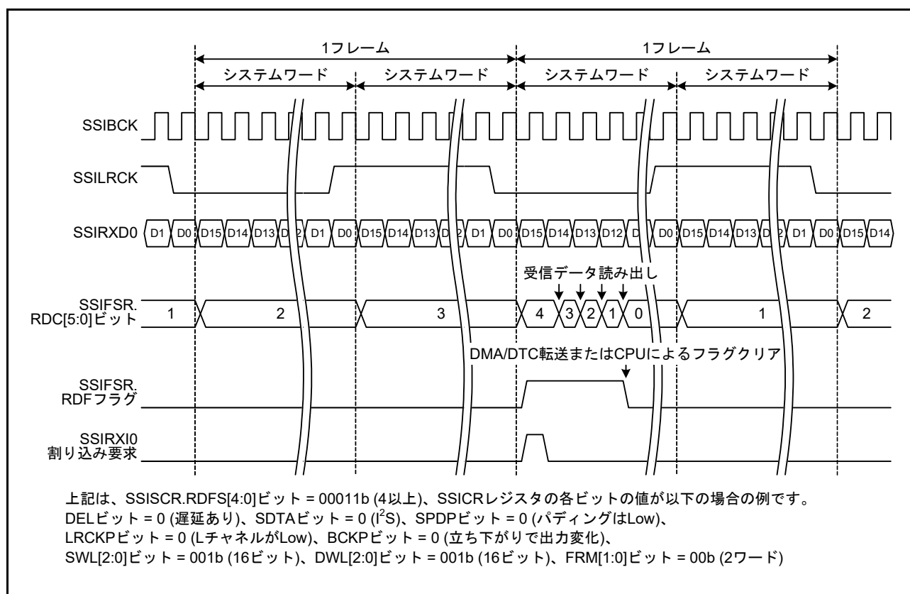
図 46.28 SSIRXIO 割り込みのタイミング図
