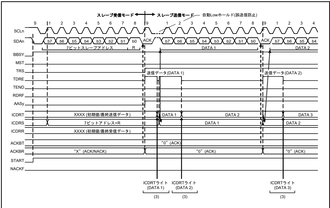
図 41.15 スレーブ送信の動作タイミング (1) (7 ビットアドレスフォーマットの時)
