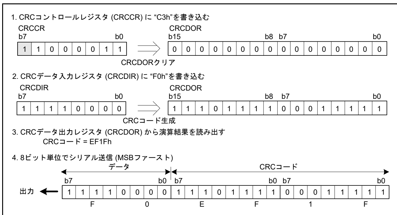
図 45.3 MSB ファーストでのデータ送信
