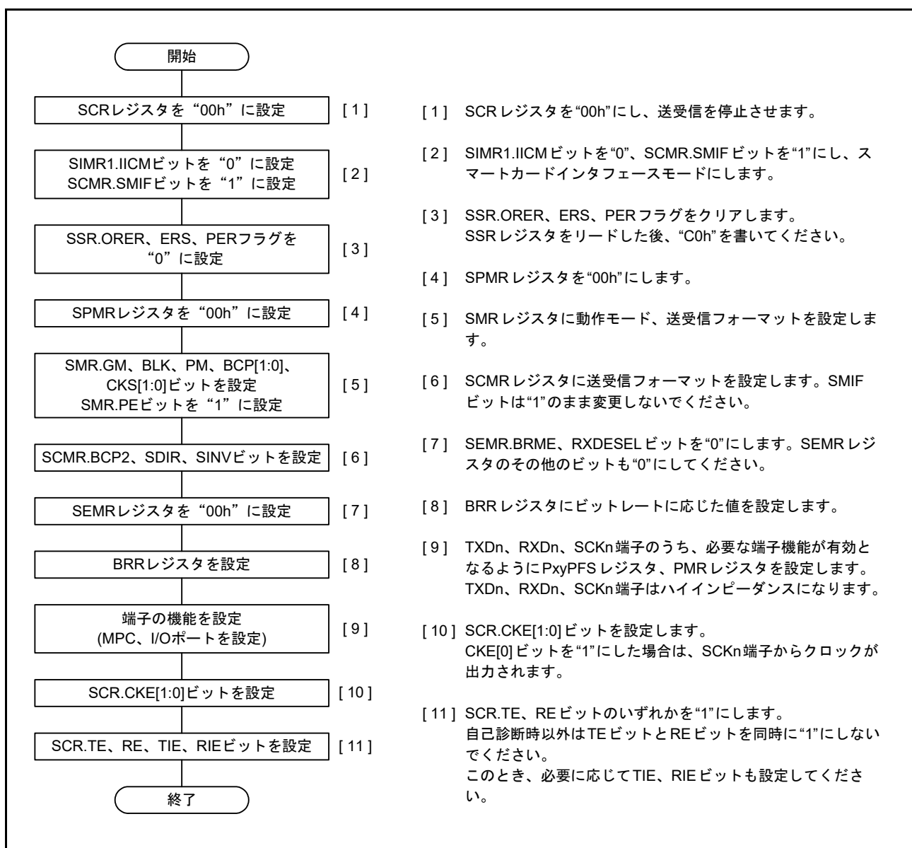
図 40.42 SCIの初期化フローチャートの例 (スマートカードインタフェースモード)
