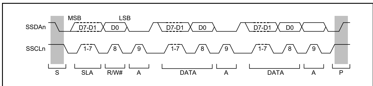
図 40.51 I 2 C バスタイミング (SLA = 7 ビットの場合)
