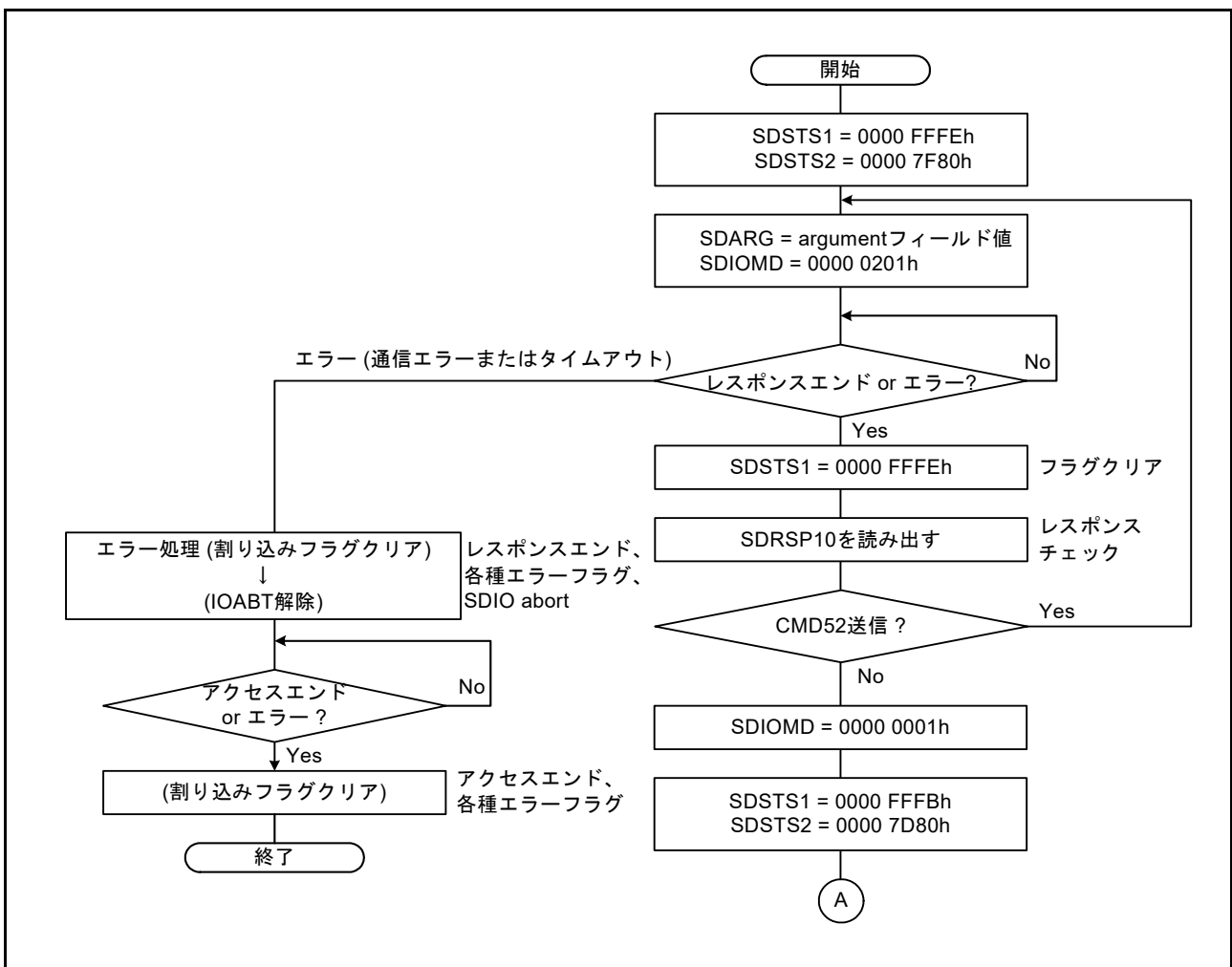
図 47.20 IO_RW_EXTENDED コマンド (CMD53/ マルチブロックライト) のシーケンス中に SDIO none abort (CMD52) を送信する例
