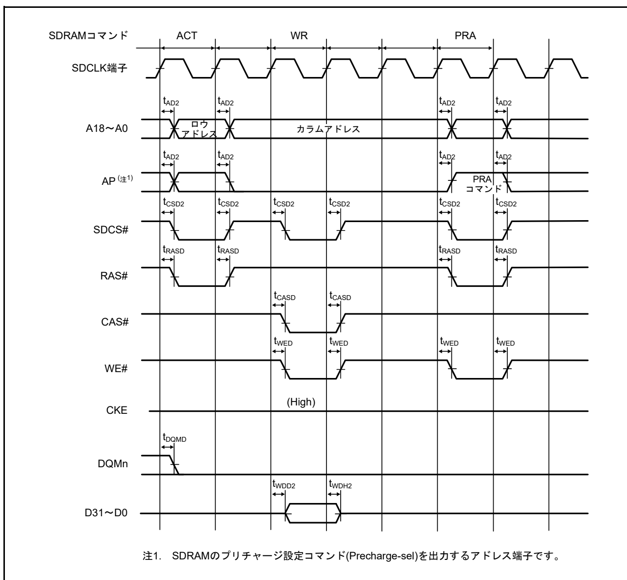
図 61.26 SDRAM 空間シングルライトバスタイミング
