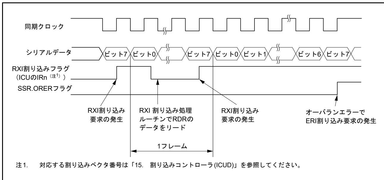
図 40.33 クロック同期式モードのシリアル受信時の動作例 (1) (RTS 機能未使用時)
