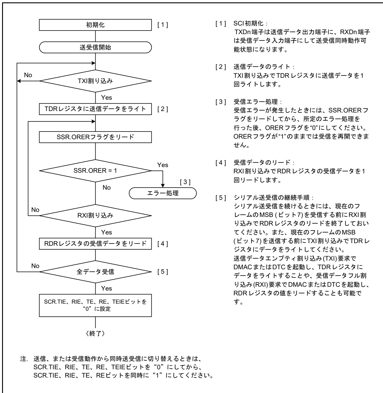
図 40.36 クロック同期式モードのシリアル送受信同時動作のフローチャート例
