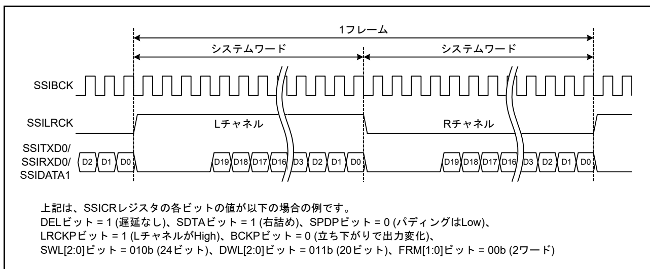
図 46.11 右詰めフォーマットの例
