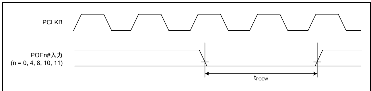
図 61.42 POE# 端子入力タイミング
