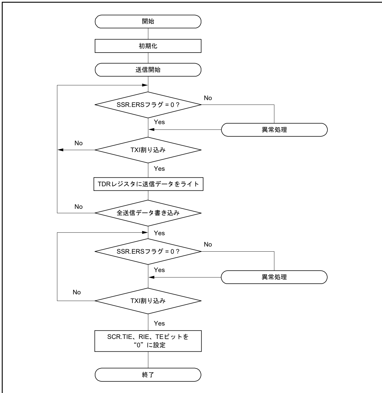
図 40.45 スマートカードインタフェース送信のフローチャート例
