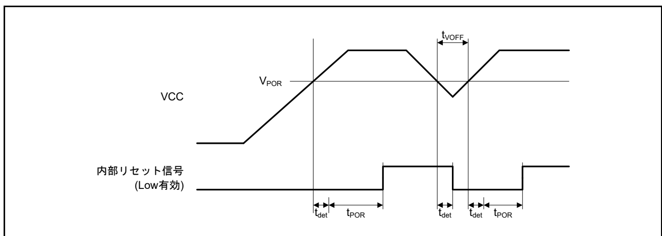
図 61.102 パワーオンリセットタイミング
