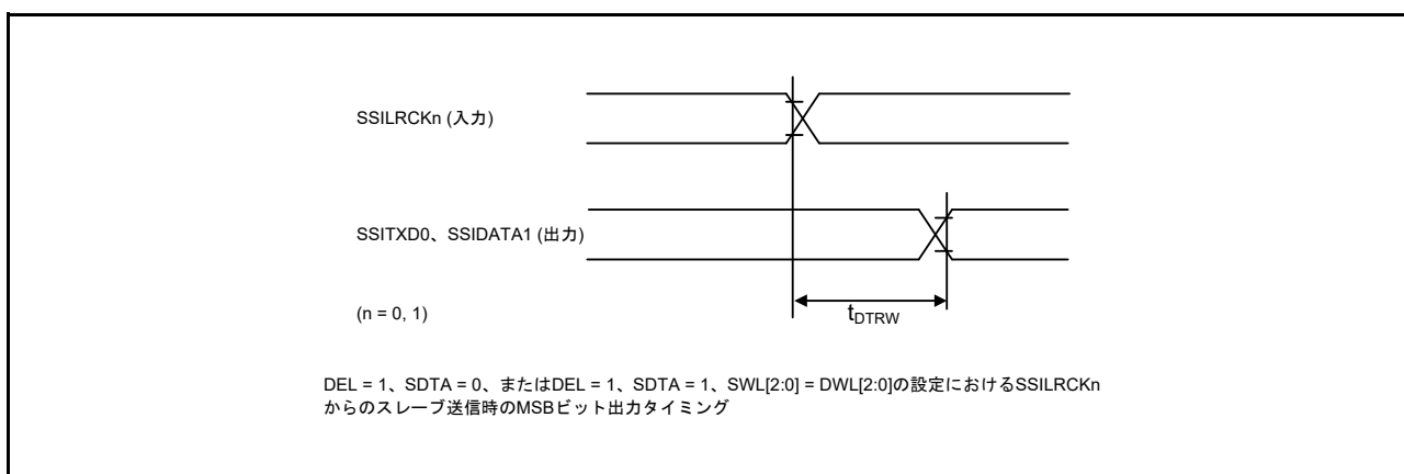
図 61.77 SSILRCKn 変化時からの SSIE データ出力遅延
