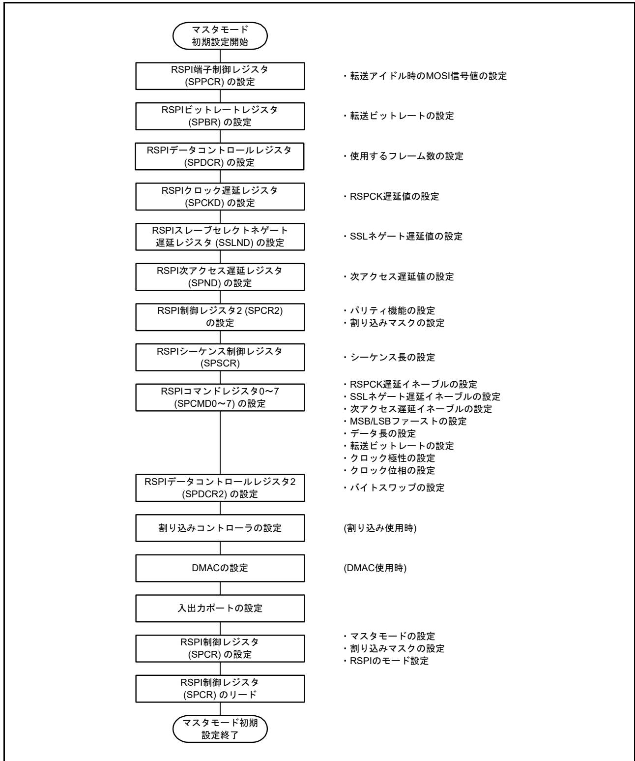
図 43.48 マスタモード時の初期化フロー例 (クロック同期式動作)
