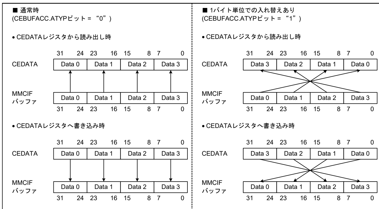
図 48.7 1バイト単位でのデータ入れ替えの概念 (32 ビットアクセス)
