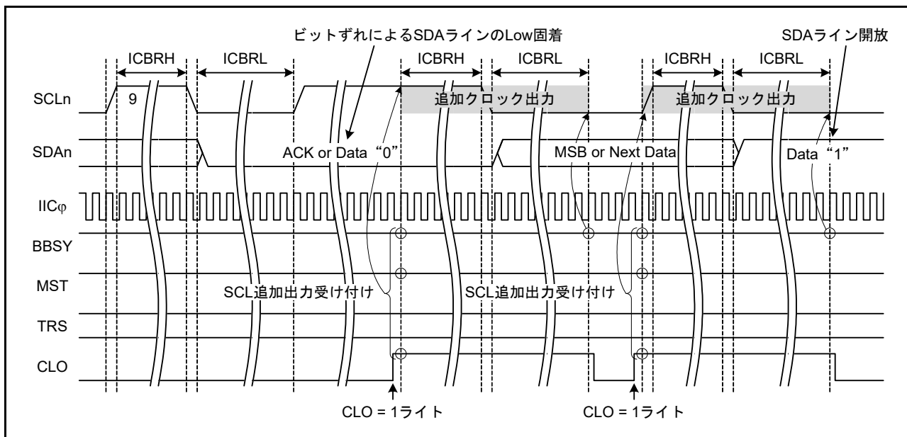
図 41.39 SCL 追加出力機能 (CLO ビット)
