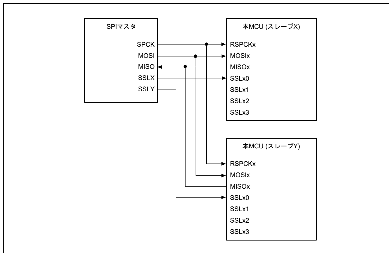
図 43.9 シングルマスタ / マルチスレーブの構成例 (本 MCU = スレーブ)
