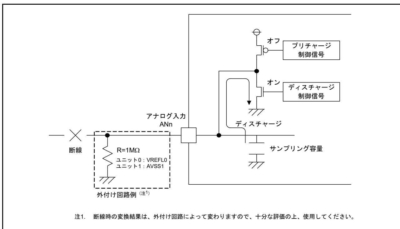
図 54.43 ディスチャージを選択した場合の断線検出例
