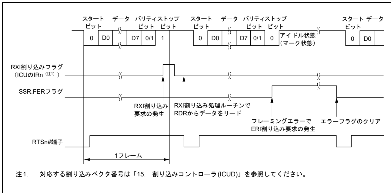
図 40.19 調歩同期式モードのシリアル受信時の動作例 (2) (RTS 機能使用時) (8ビットデータ/パリティあり/1ストップビットの例)
