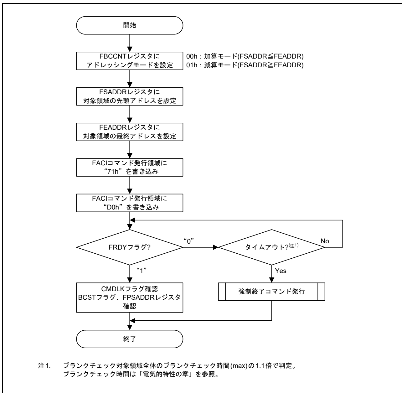
図 60.24 ブランクチェックコマンドの使用方法
