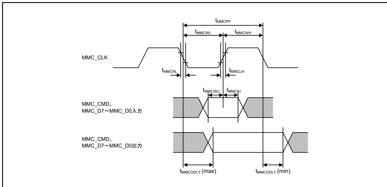
図 61.79 MMC インタフェース
