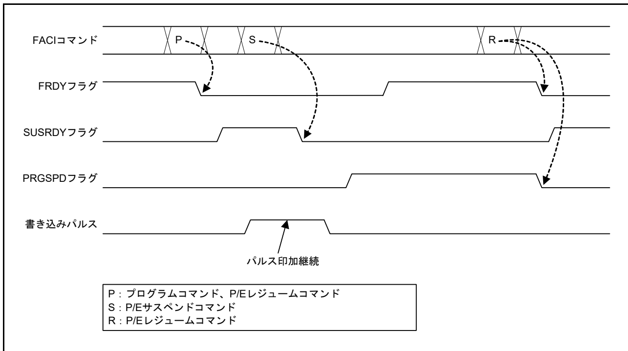
図 60.18 プログラム処理の中断動作
