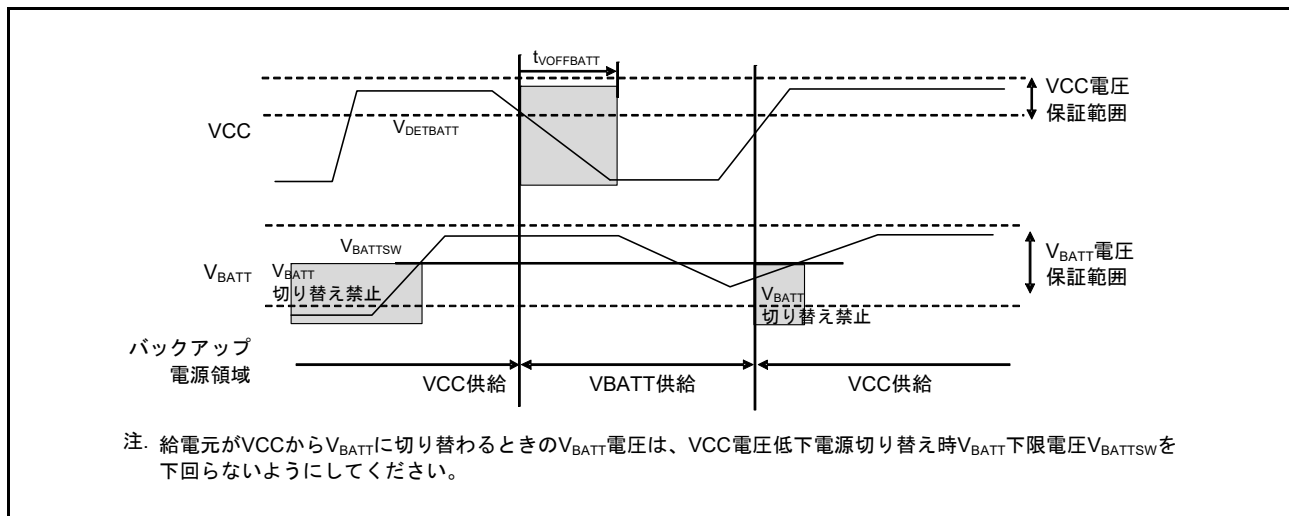
図 61.107 バッテリバックアップ機能特性
