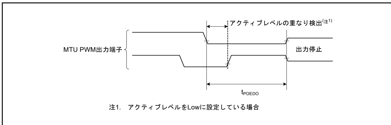
図 61.44 POE 出力ディセーブル時間 (出力端子の短絡)
