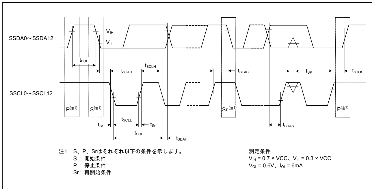
図 61.56 簡易 IIC バスインタフェース入出力タイミング
