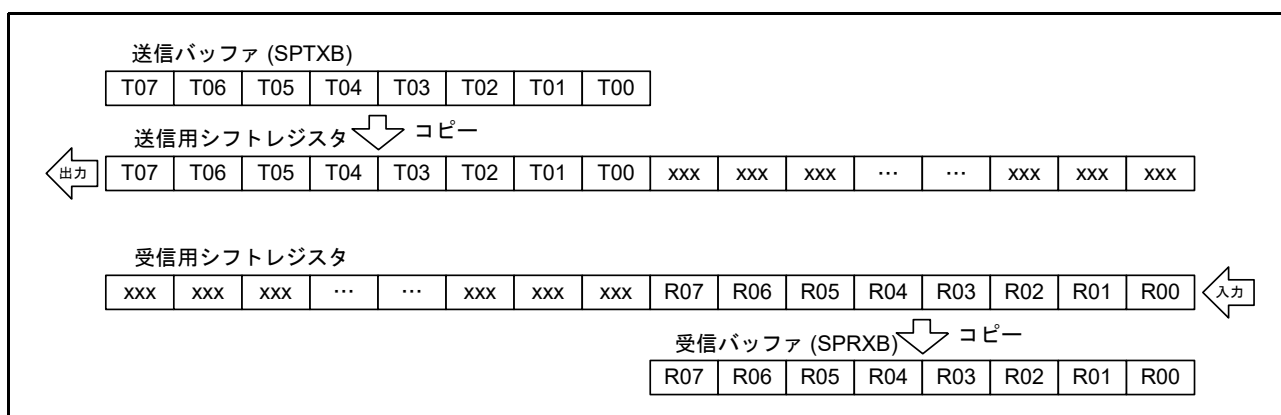
図 44.8 MSB ファースト転送 (8 ビットデータ)
