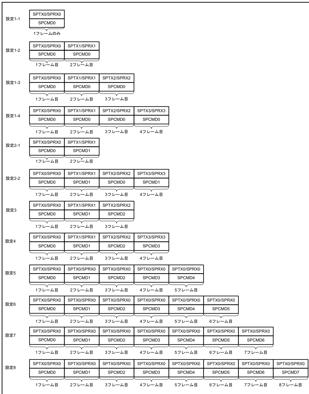
図 43.35 シーケンス動作時の RSPI コマンドレジスタと送受信バッファの対応
