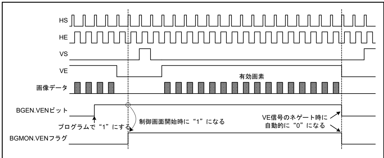
図 50.22 内部動作へのレジスタ値反映制御信号
