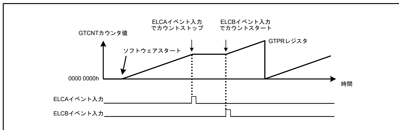
図 26.60 ハードウェア要因によるカウントストップ動作例 (ソフトウェアでスタート、ELCA イベント入力でストップ、ELCB イベント入力で再スタート時)
