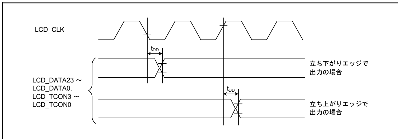
図 61.96 LCD 出力データタイミング
