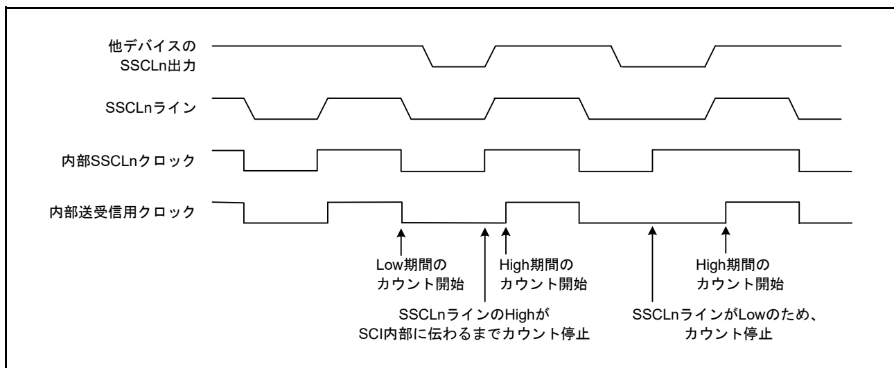
図 40.53 クロック同期化の動作例
