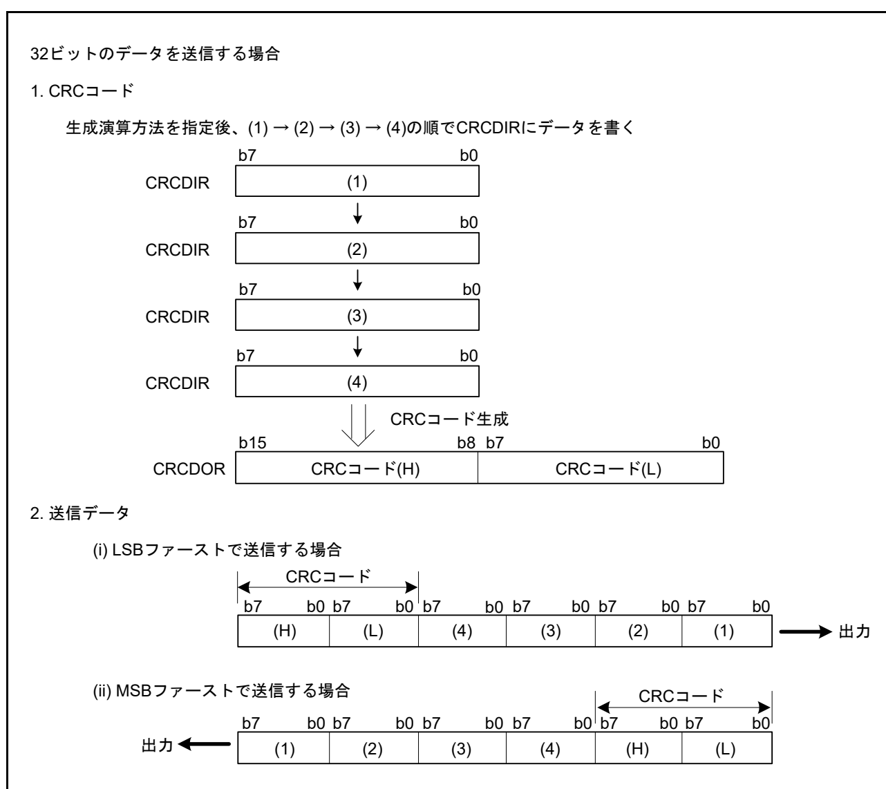
図 45.6 LSB ファーストと MSB ファーストの送信データ
