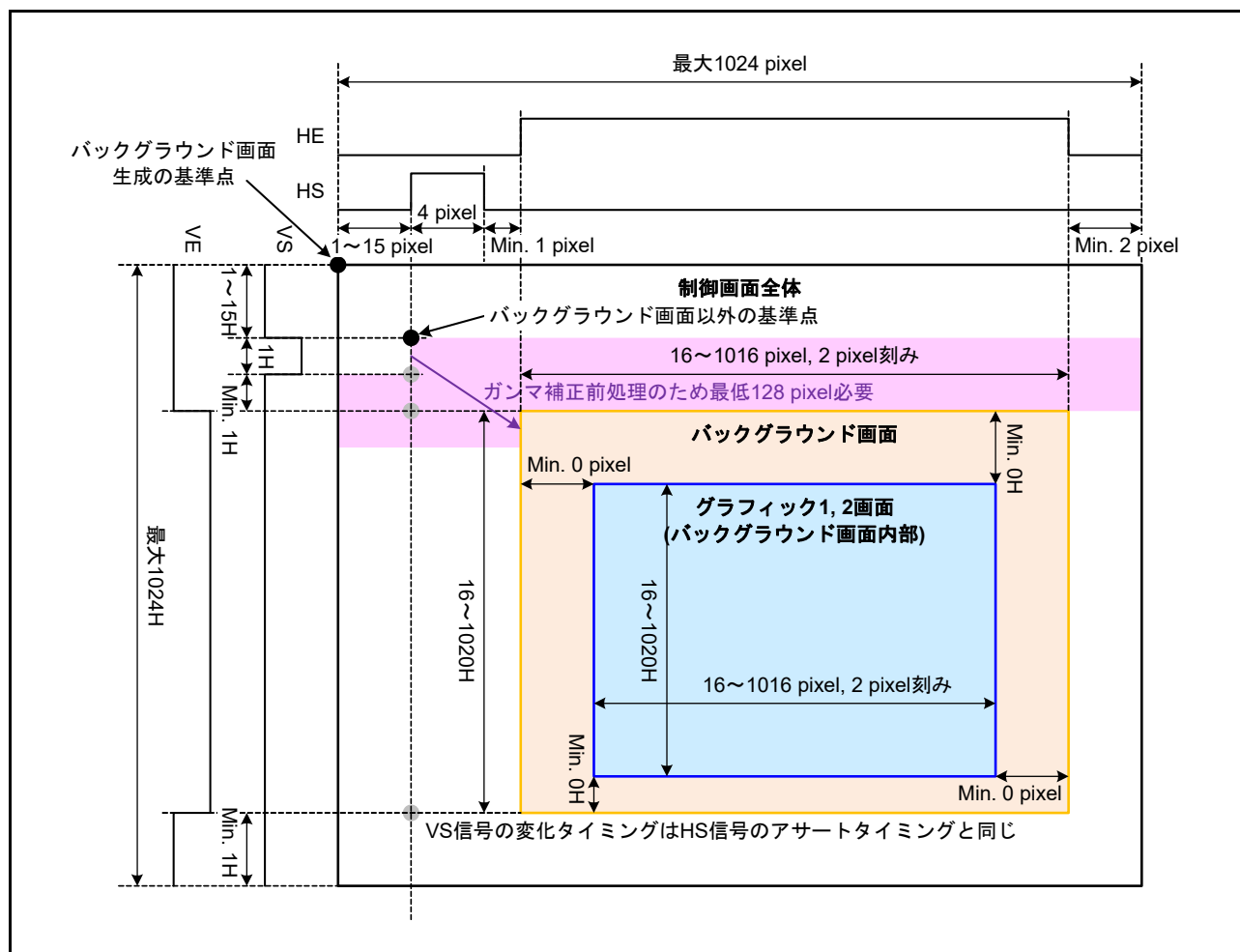
図 50.3 画面フォーマット
