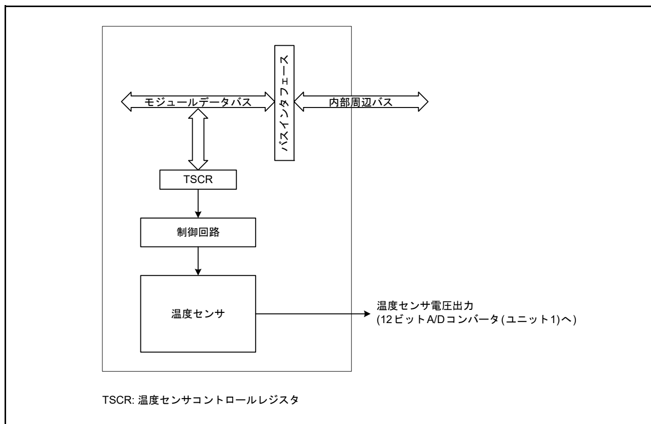
図 56.1 温度センサのブロック図
