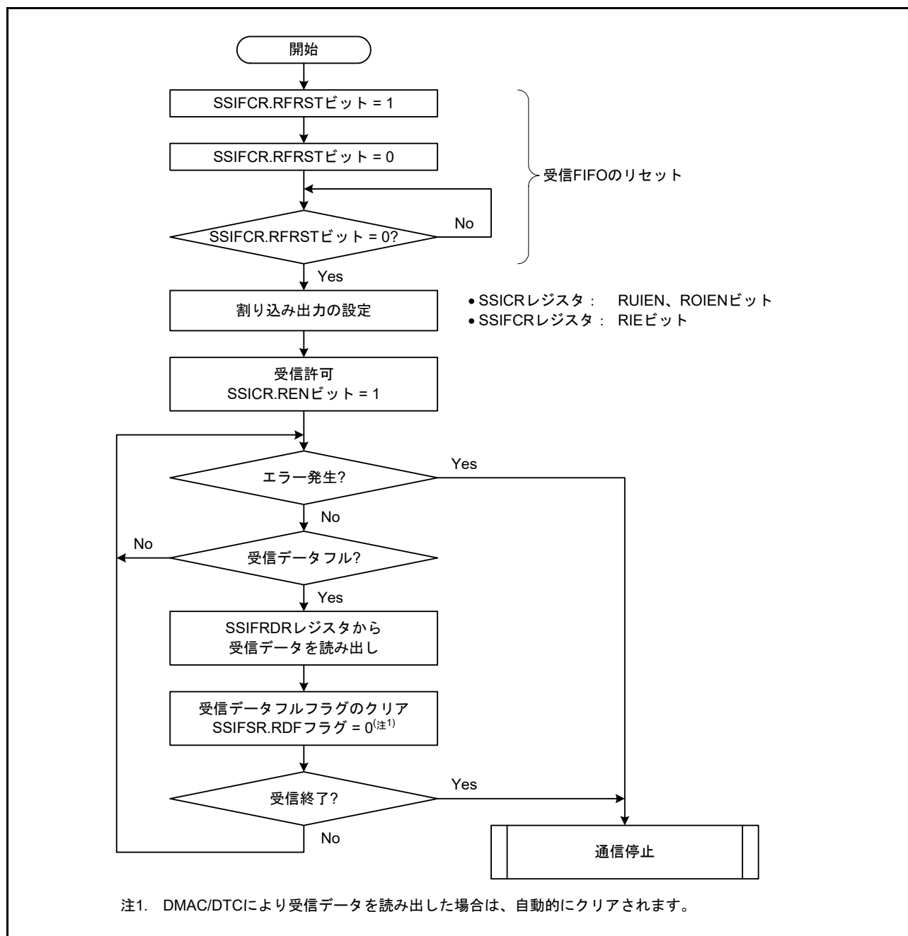
図 46.24 受信フロー例
