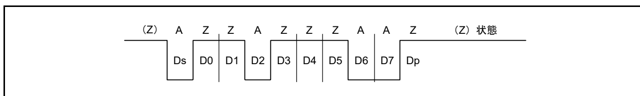
図 40.39 ダイレクトコンベンション (SCMR.SDIR ビット = 0、SCMR.SINV ビット = 0、SMR.PM ビット = 0)
