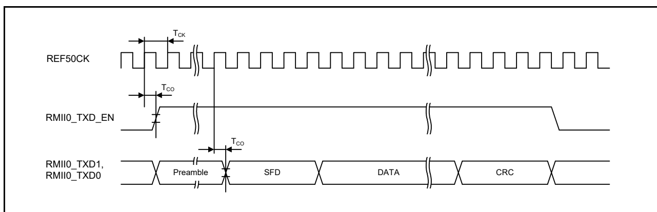
図 61.82 RMII 送信タイミング
