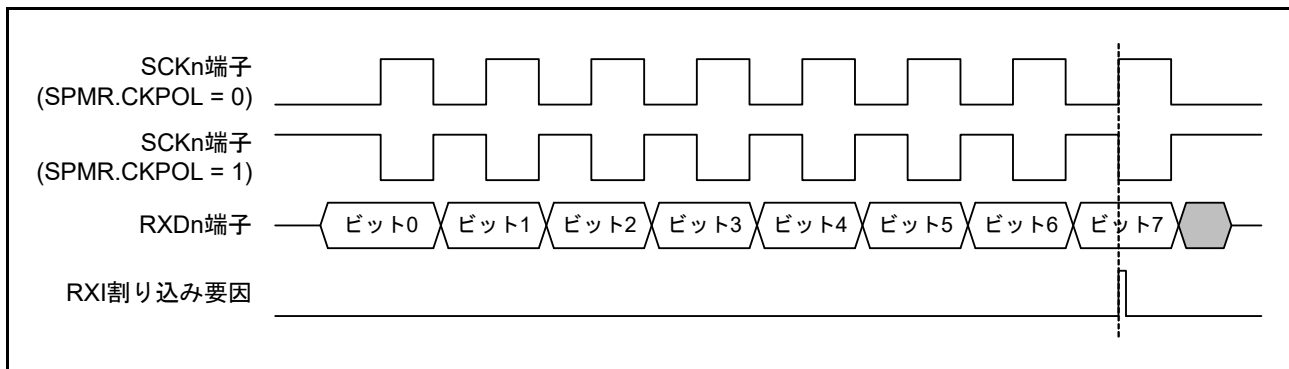
図 40.85 簡易 SPI モード (クロック遅れあり) RXI 割り込み発生タイミング
