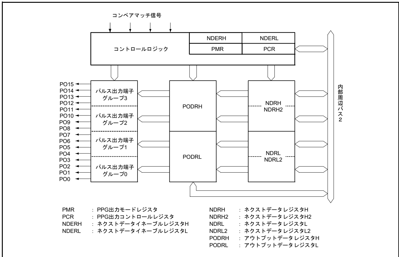
図 29.1 PPG0 のブロック図
