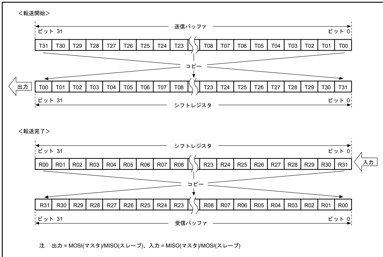
図 43.16 LSB ファースト転送 (32 ビットデータ / パリティ機能無効)
