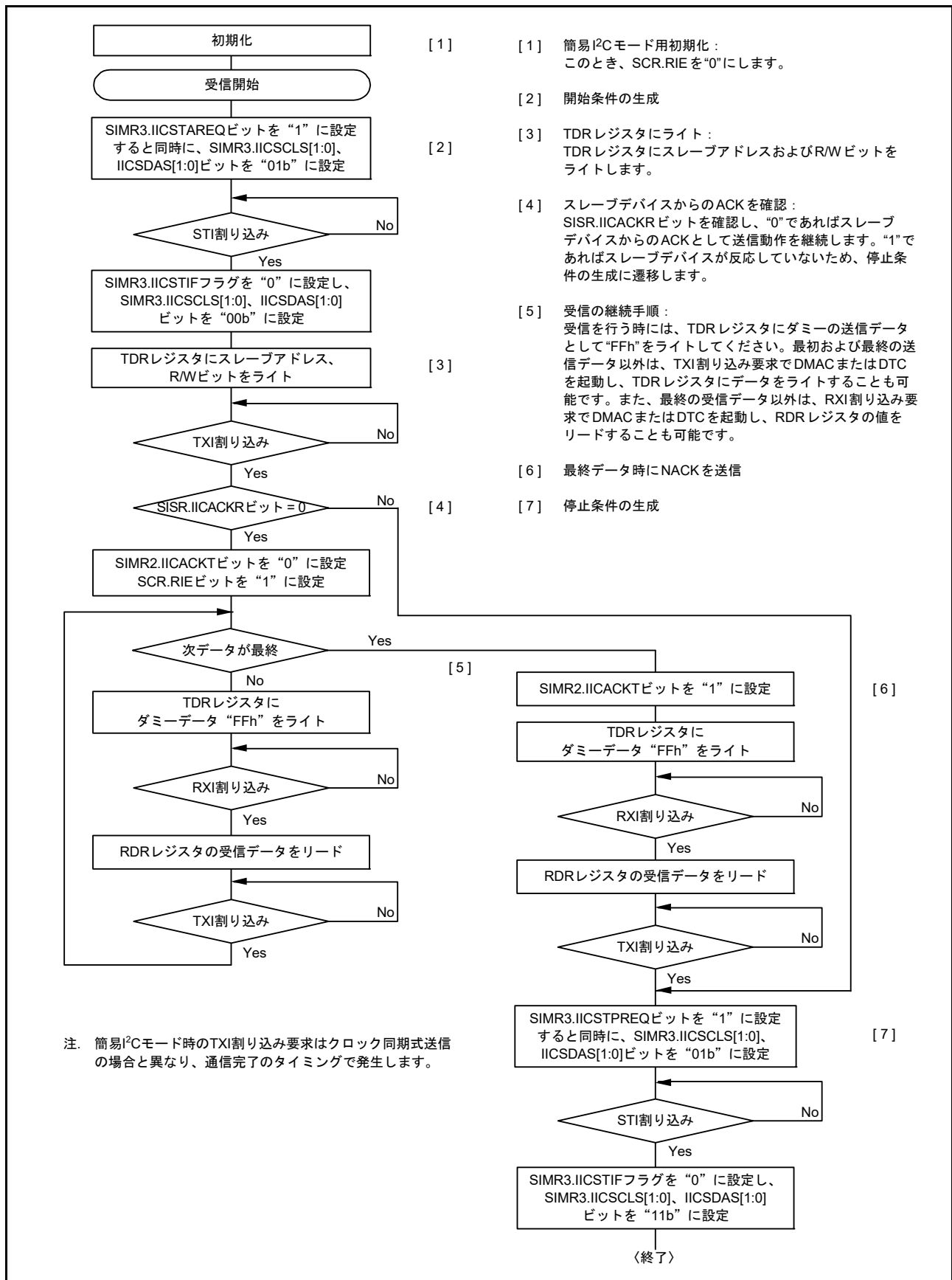
図 40.60 簡易 I 2 C モードのマスタ受信動作のフローチャート例 (送信割り込み、受信割り込み使用時)
