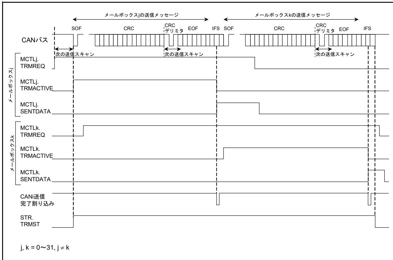
図 42.20 データフレーム送信時の動作例
