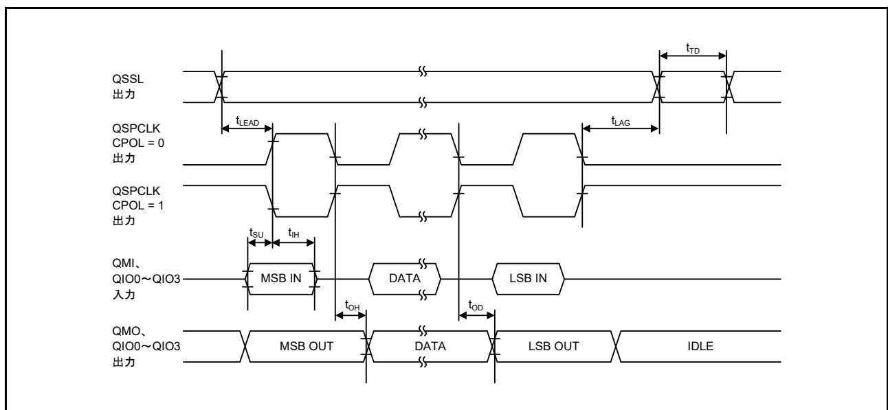
図 61.71 送受信タイミング (CPHA = 0)
