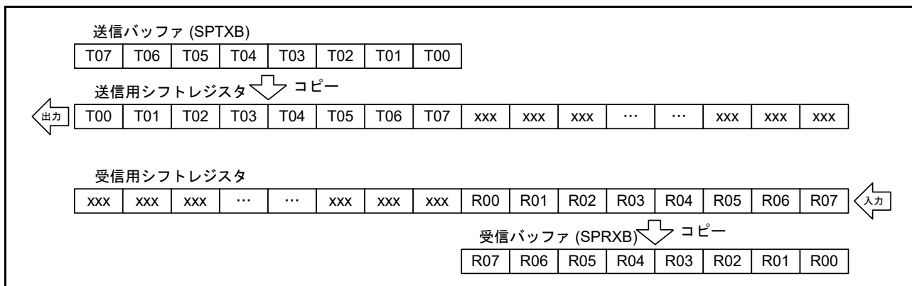
図 44.11 LSB ファースト転送 (8 ビットデータ)
