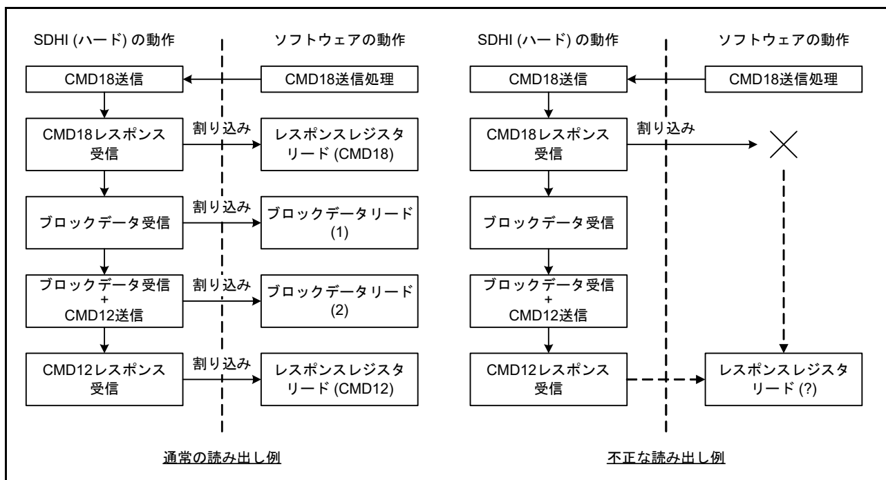
図 47.23 マルチブロックリード処理例 (2 ブロック)
