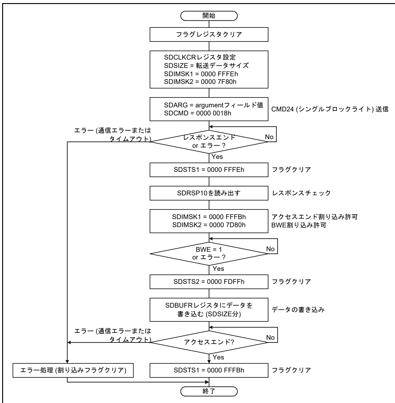
図 47.11 シングルブロックライトコマンドの送信例
