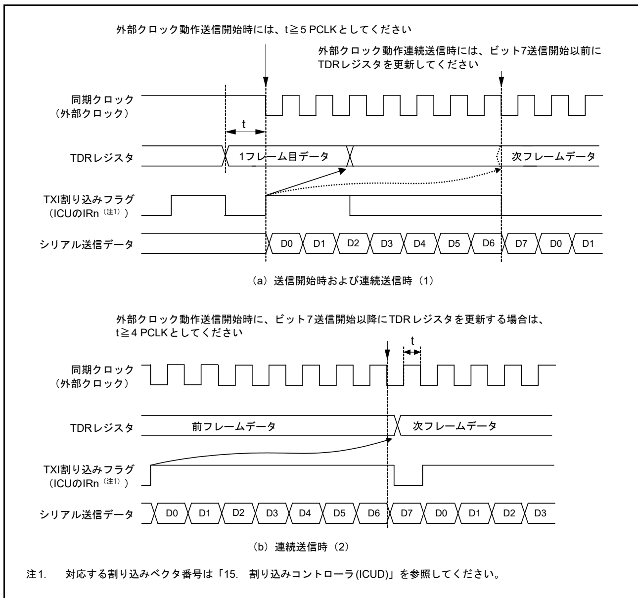
図 40.80 クロック同期式モード送信での外部クロック使用の制約事項
