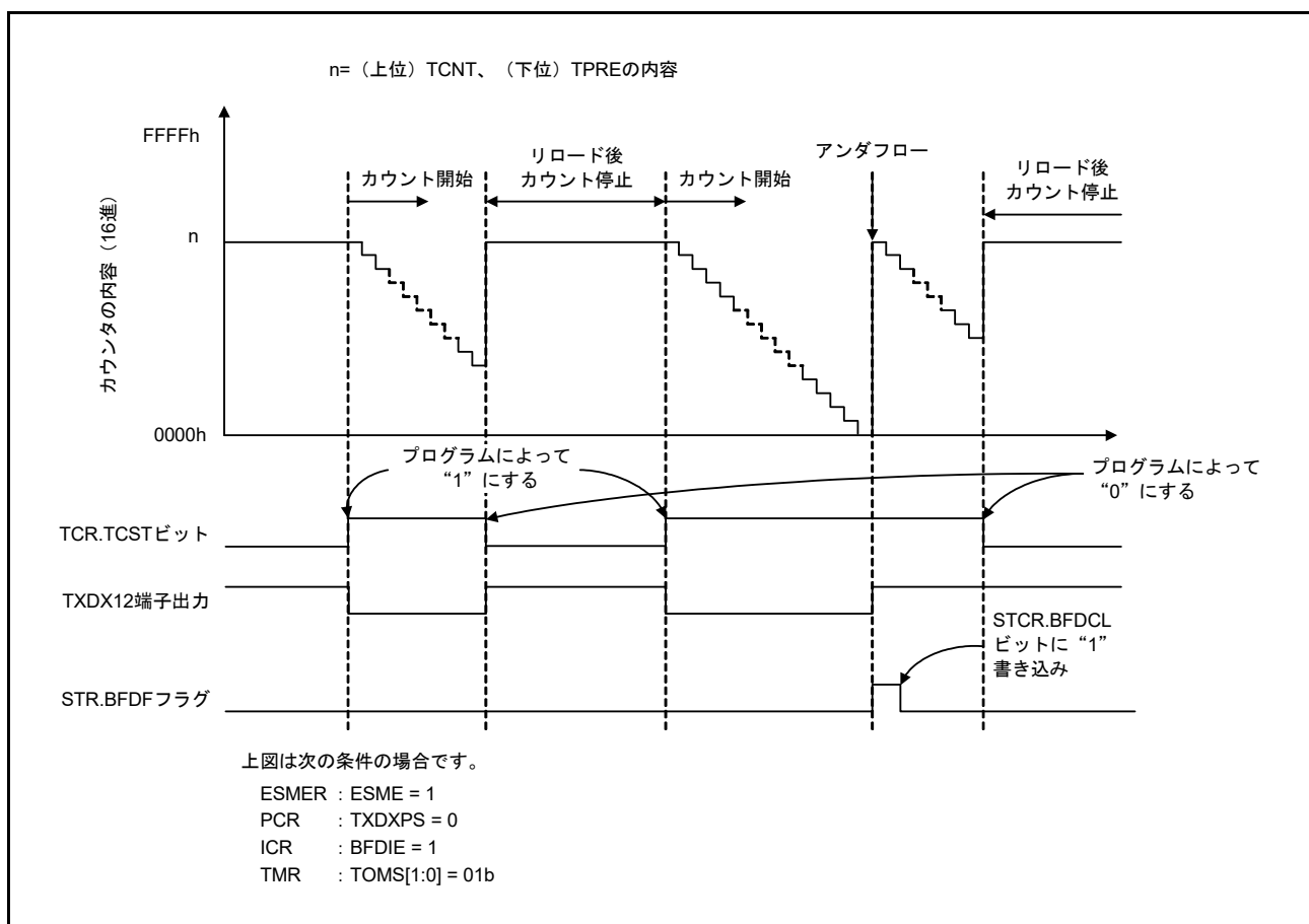
図 40.77 Break Field Low width 出力モードの動作例
