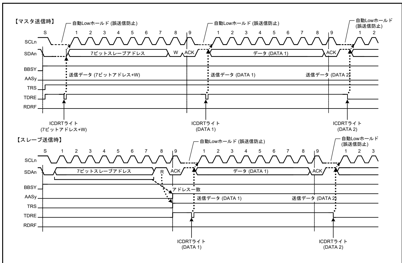
図 41.29 送信モードの自動 Low ホールド動作
