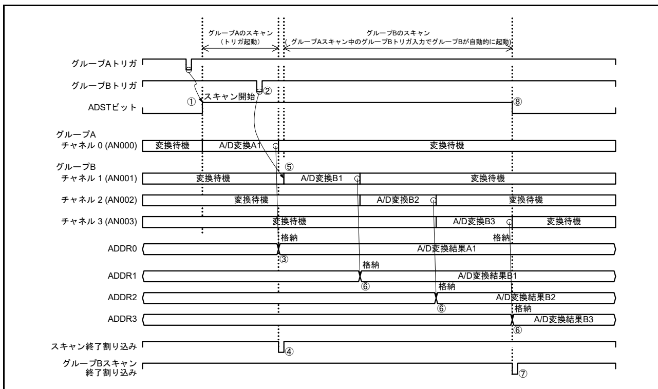
図 54.27 グループ優先動作の例3 「グループA スキャン中のグループB トリガ入力」再スキャンあり (ADGSPCR.GBRSCN = 1, ADGSPCR.GBRP = 0, ADGSPCR.LGRRS = 0 設定時)
