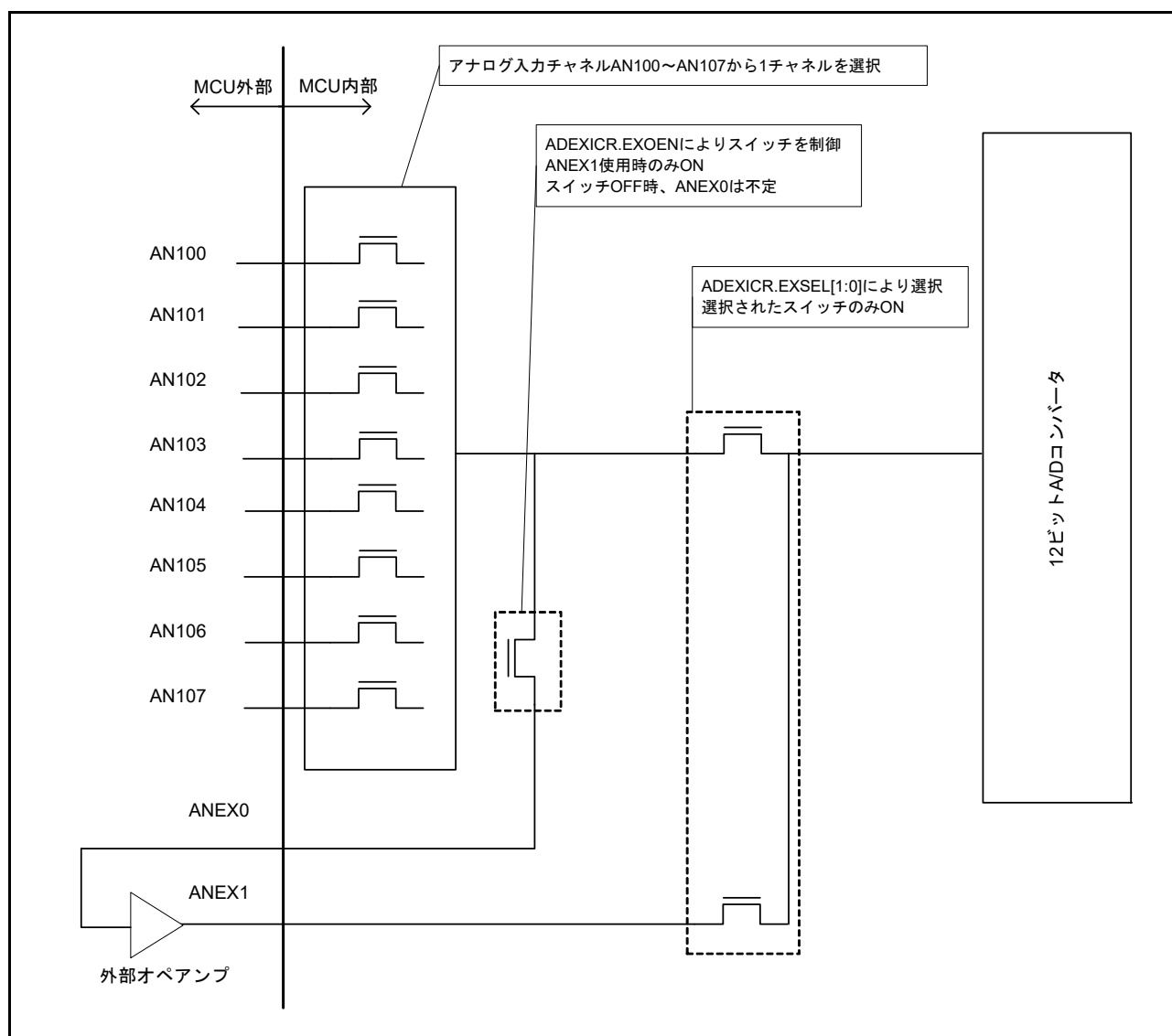
図 54.35 ANEX1 使用時の拡張アナログ入力構成例
