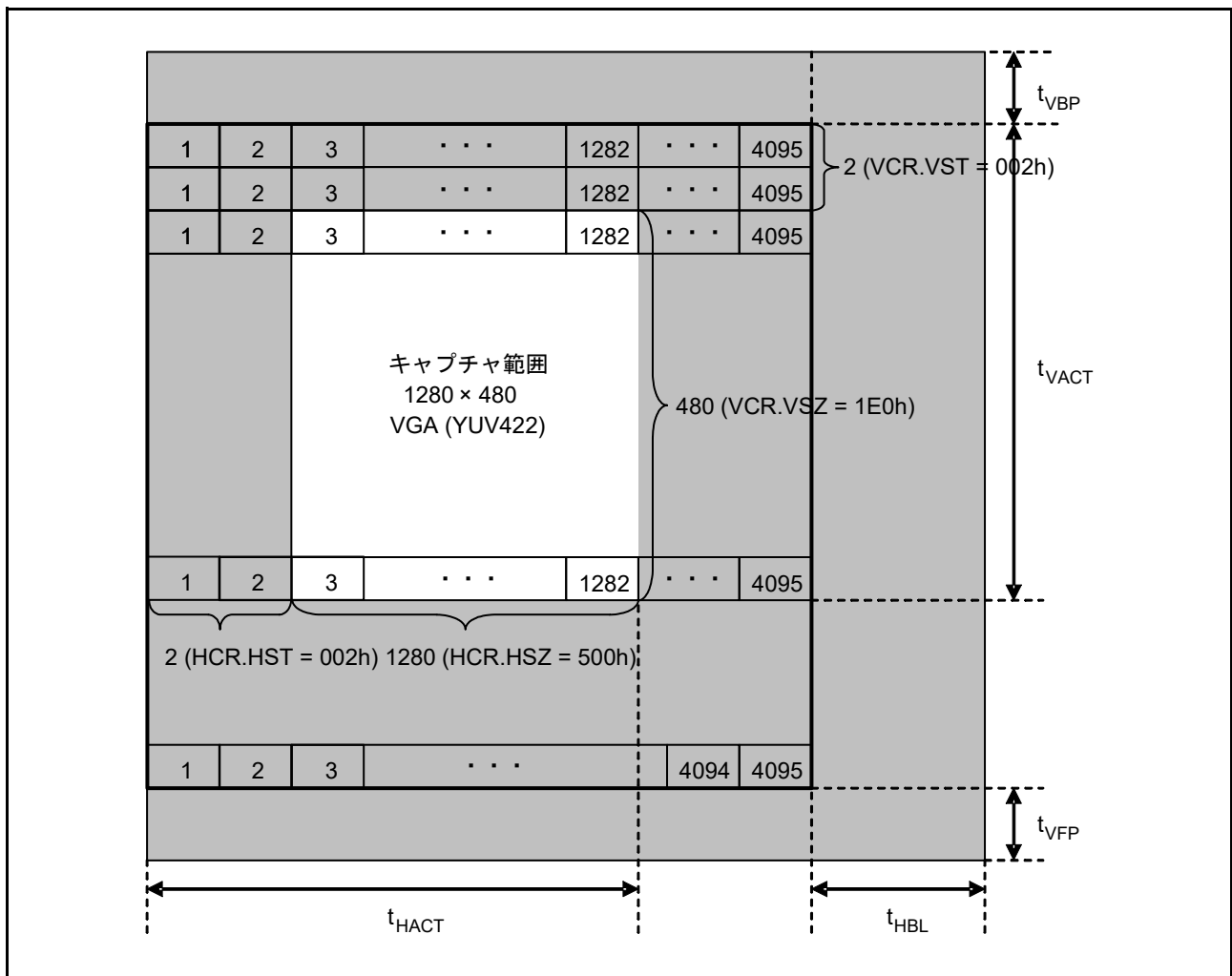
図 49.10 VCR レジスタ、HCR レジスタ設定とキャプチャ範囲 (VCR = 01E0 0002h, HCR = 0500 0002h)
