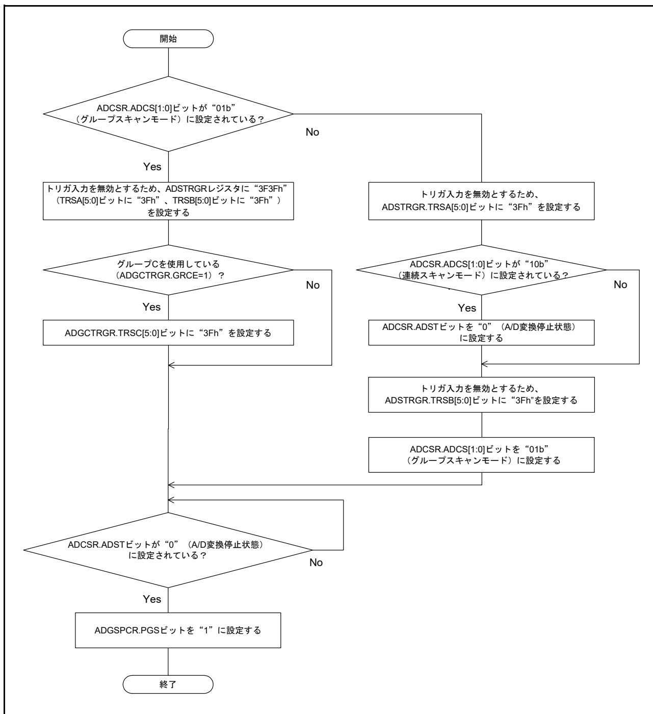
図 54.24 ADGSPCR.PGS ビット設定時のフローチャート
