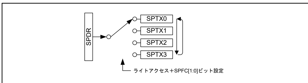
図 43.3 SPDR レジスタの構成図 (ライト時)
