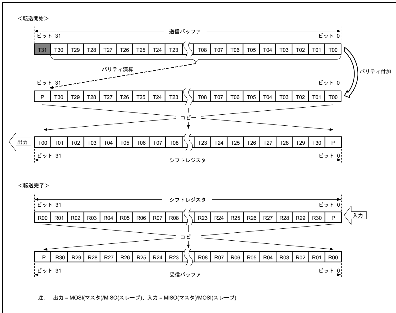
図 43.20 LSB ファースト転送 (32 ビットデータ / パリティ機能有効)
