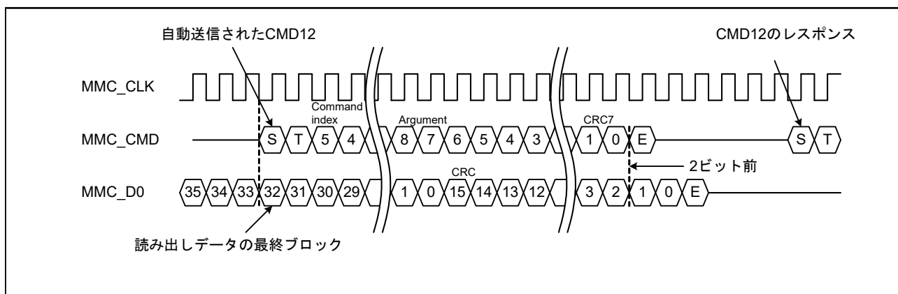
図 48.8 マルチブロックリード時の CMD12 自動送信タイミング (1 ビットモード時)
