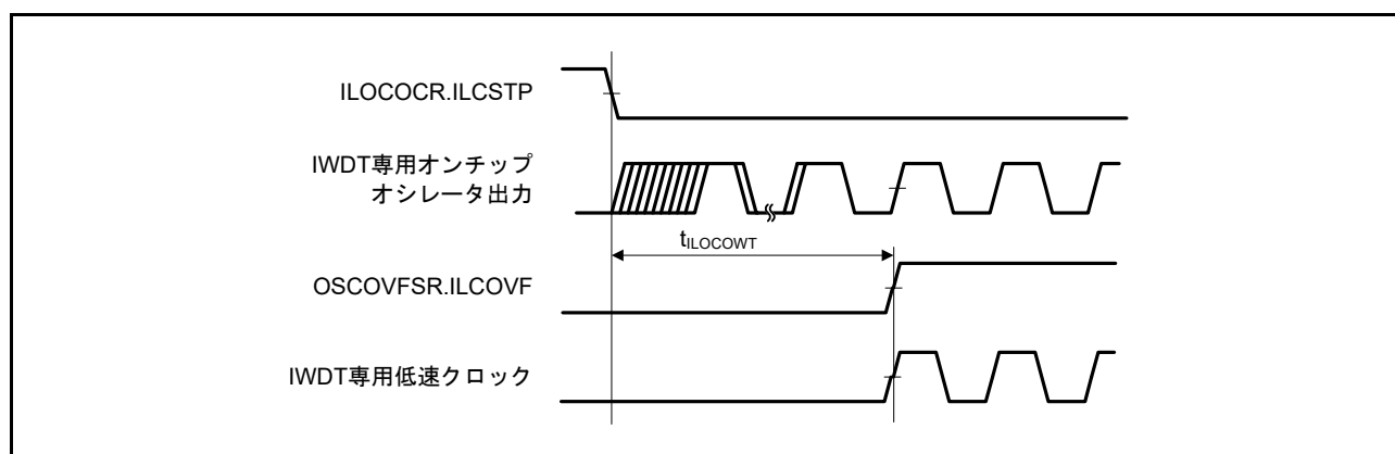
図 61.7 IWDT 専用低速クロック発振開始タイミング
