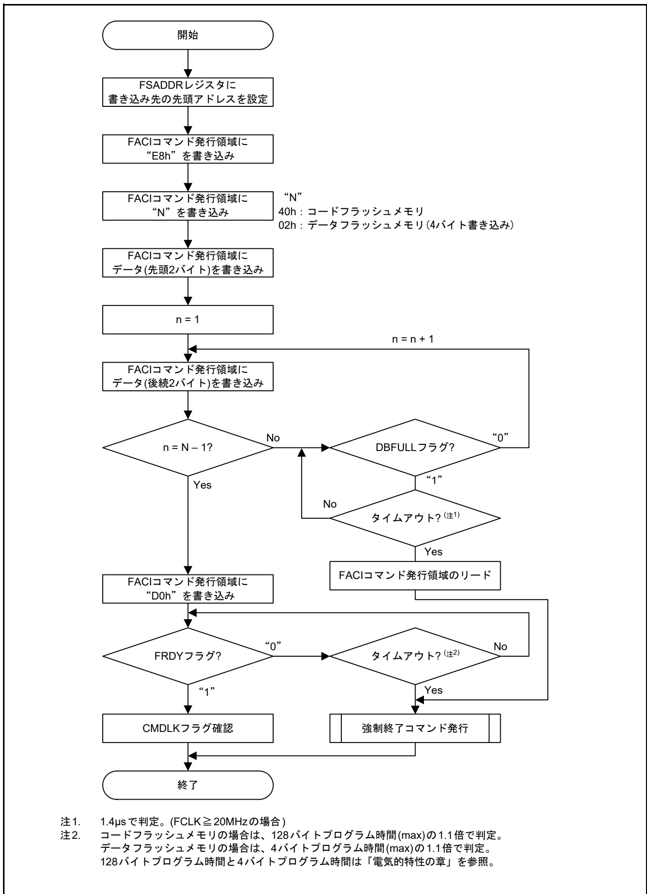
図 60.14 プログラムコマンドの使用方法
