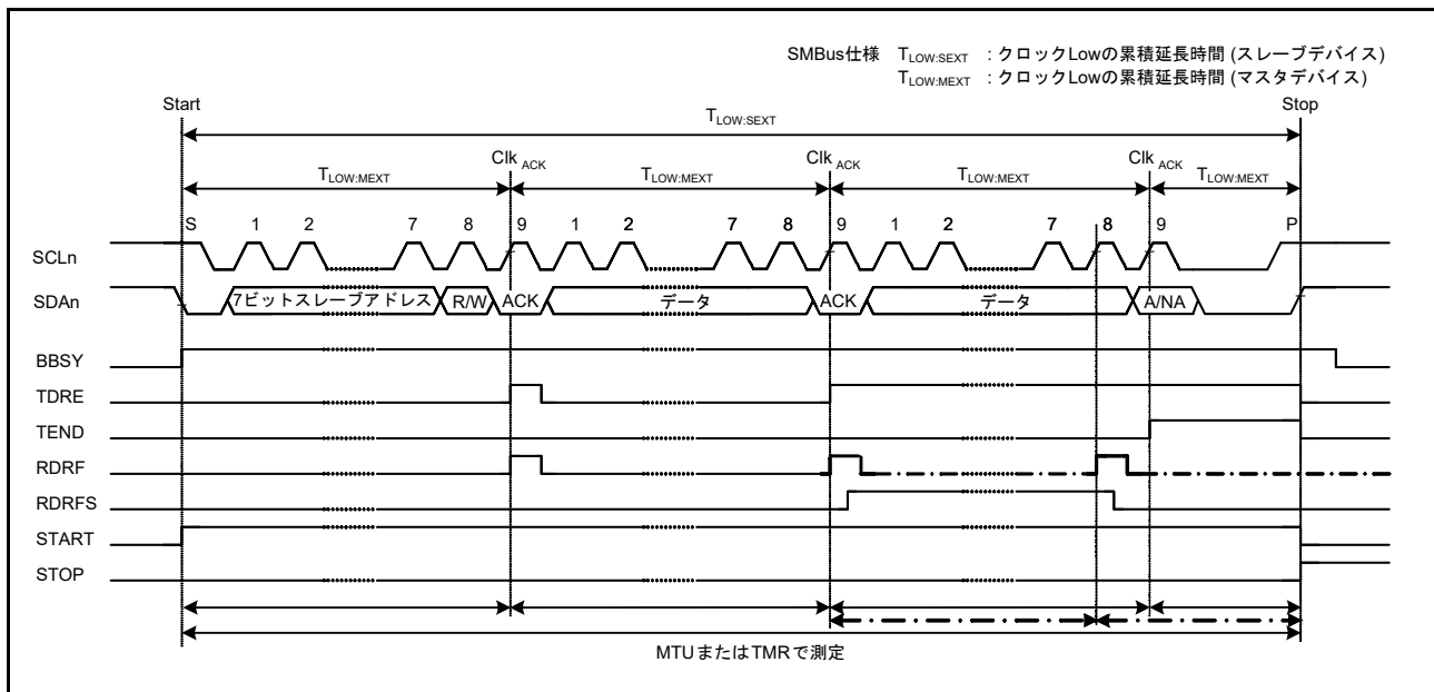
図 41.40 SMBus タイムアウト測定
