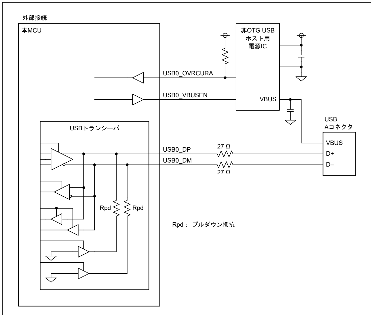
図 39.4 ホストコントローラと USB コネクタとの接続例
