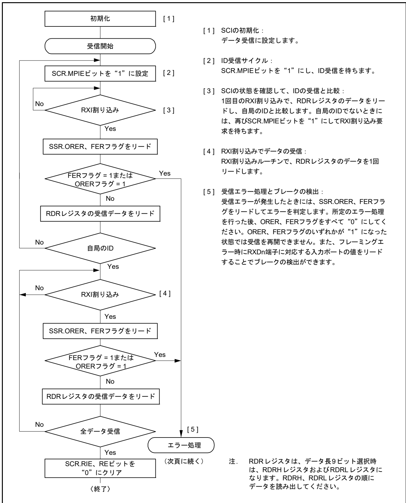
図 40.25 マルチプロセッサシリアル受信のフローチャートの例 (1)
