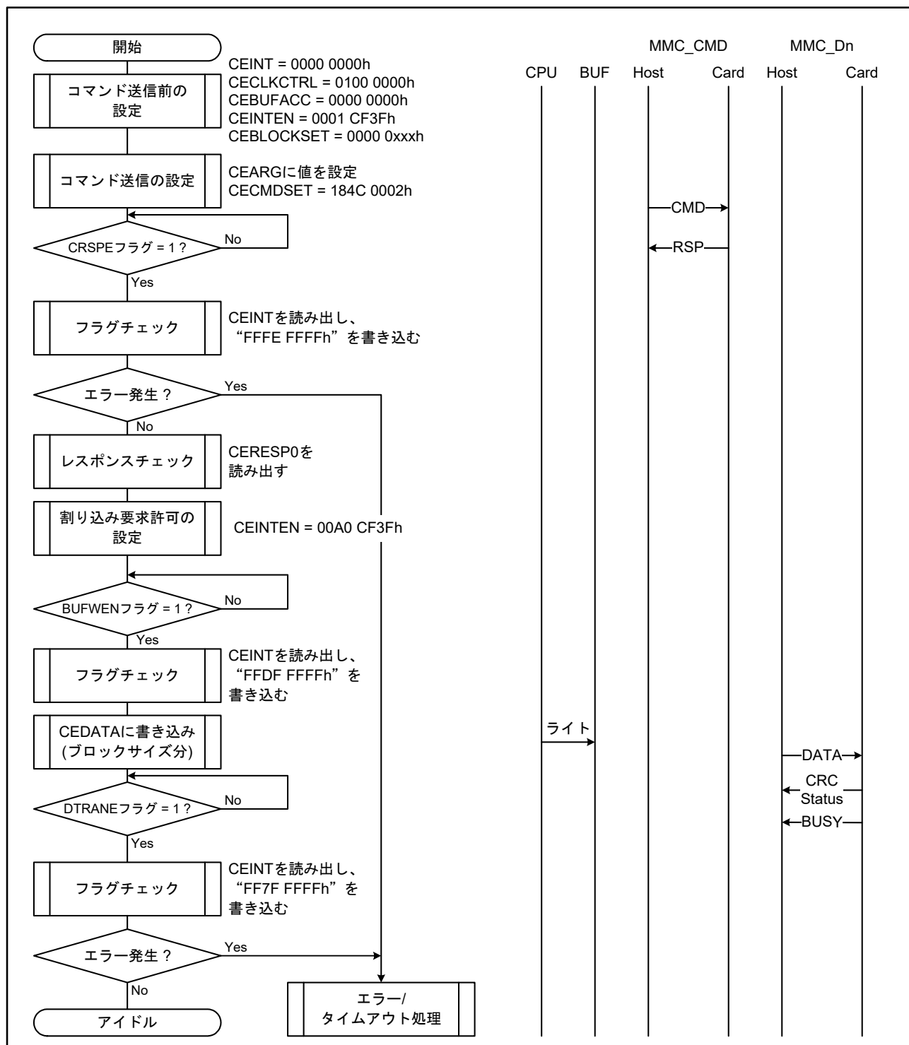
図 48.18 シングルブロックライトコマンドの送信例 (CMD24)
