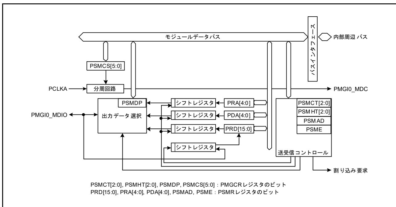
図 38.1 PMGI のブロック図
