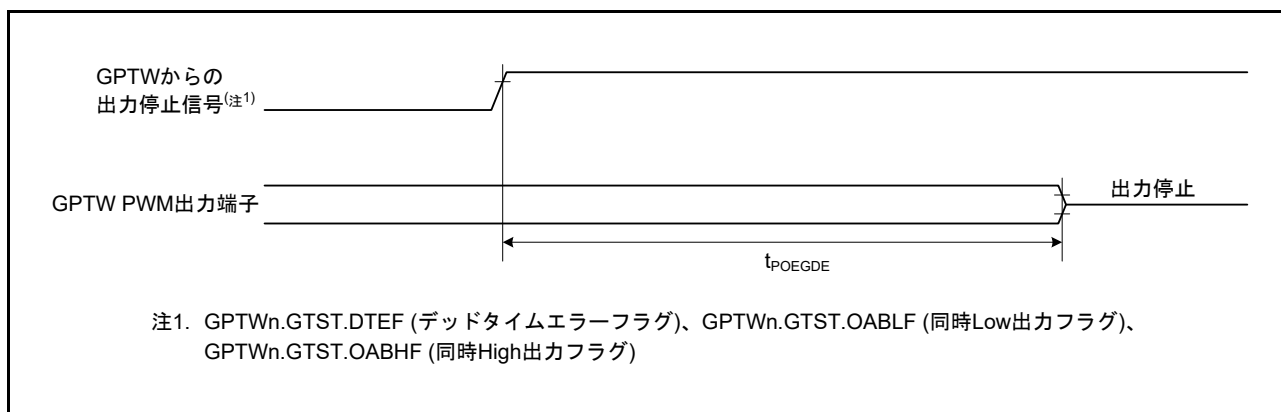
図 61.49 POEG 出力ディセーブル時間 (GPTW からの出力停止信号検出)
