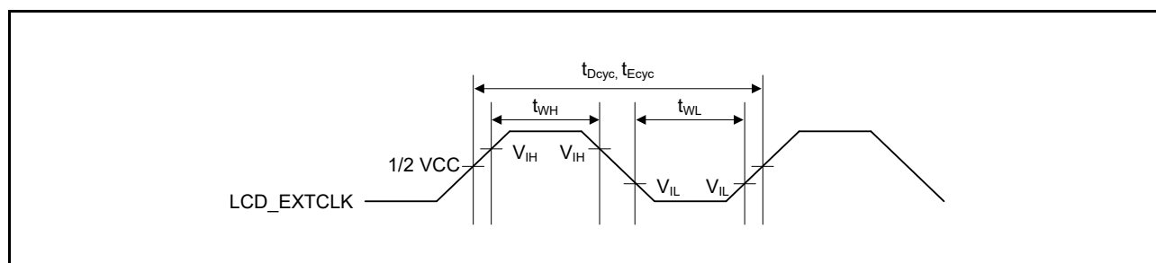
図 61.94 LCD_EXTCLK クロック入カタイミング
