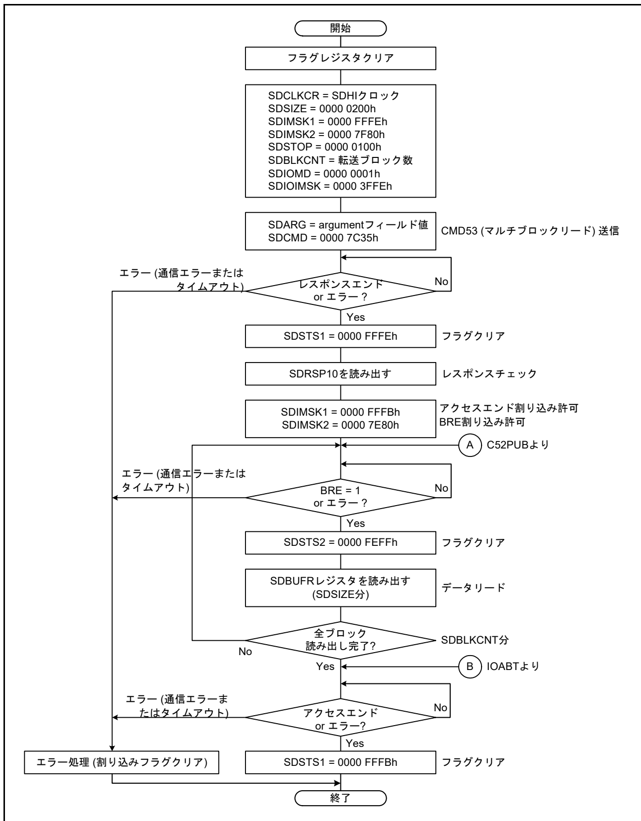
図 47.15 IO_RW_EXTENDED コマンド (CMD53/ マルチブロックリード) の送信例
