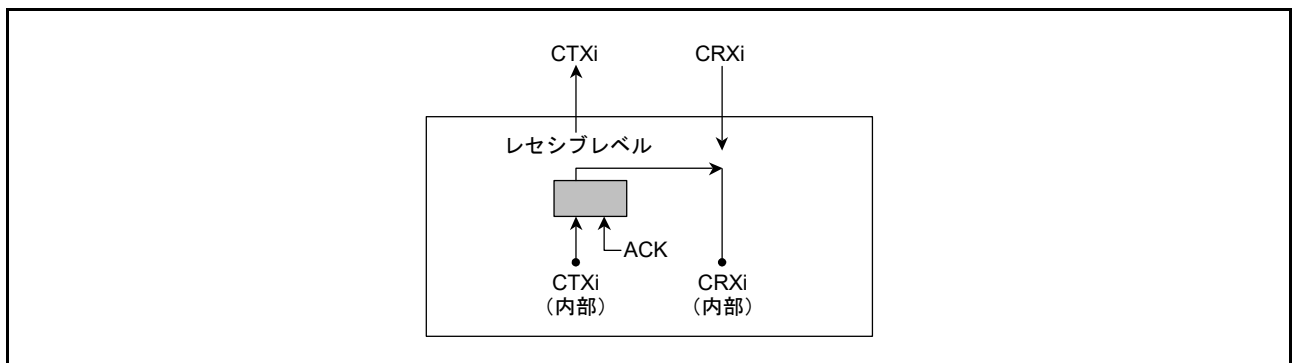
図42.8 セルフテストモード1選択時の接続 (i=0~2)
