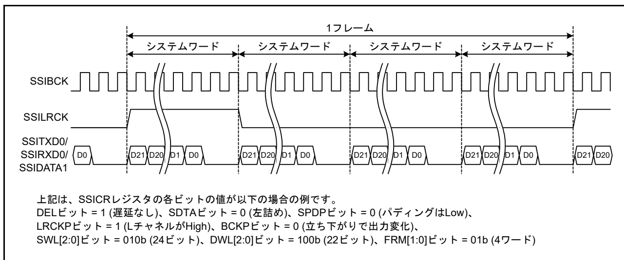
図 46.16 TDM フォーマット (2) (SSICR.DEL ビット = 1、パディングあり)
