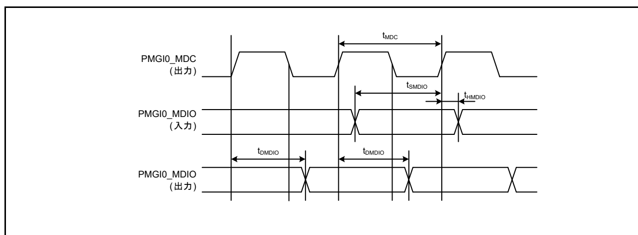
図 61.78 シリアルマネージメントアクセスタイミング
