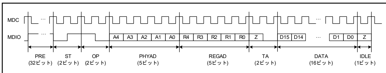
図 38.2 リードアクセスのデータフォーマット
