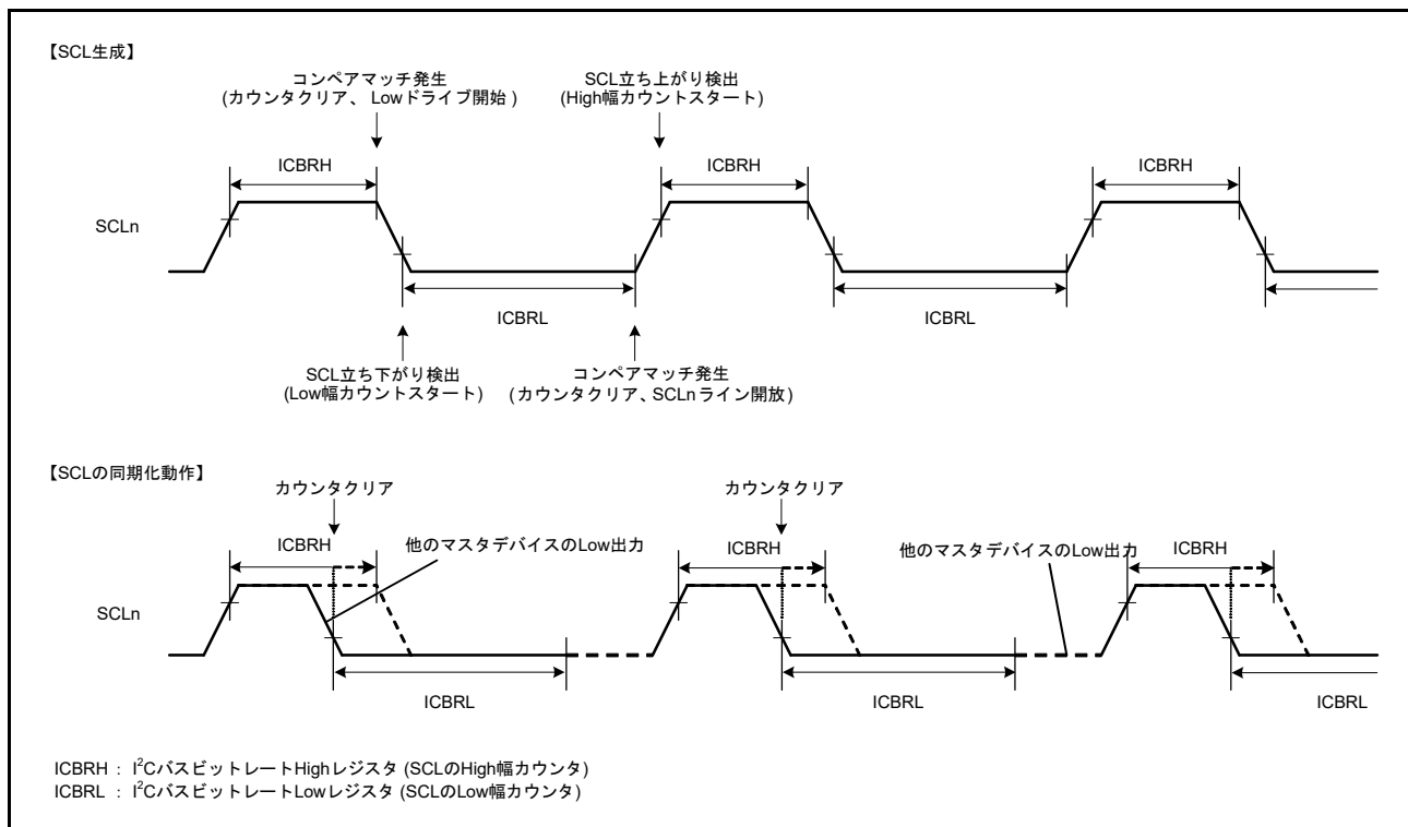
図 41.20 RIIC の SCL 生成および SCL 同期化動作
