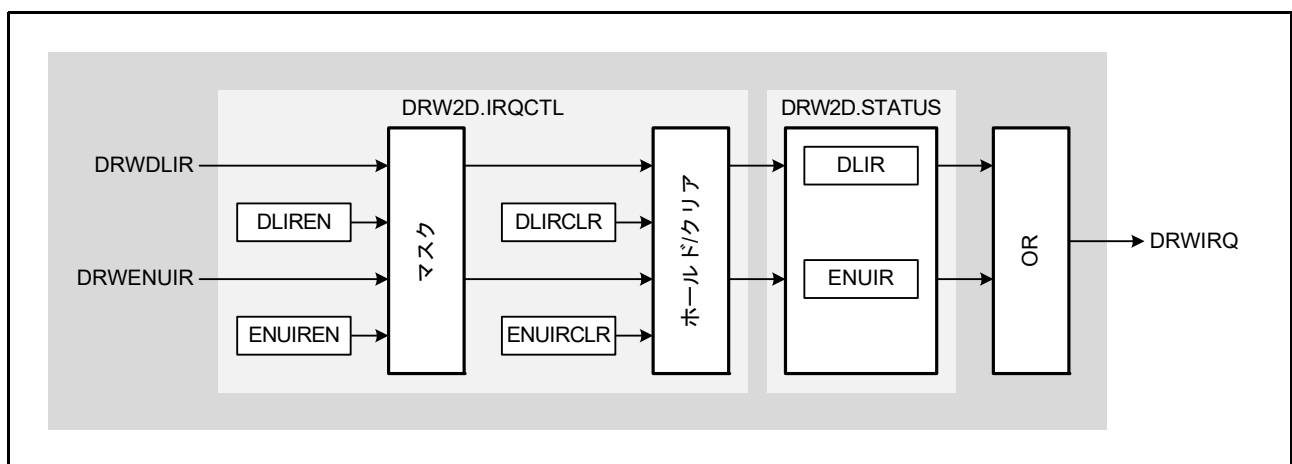
図 51.3 割り込みコントローラユニット
