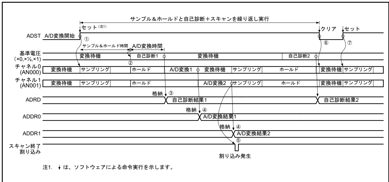
図 54.19 連続スキャンモードの動作例 (チャンネル専用サンプル & ホールド回路使用 : AN000, AN001 選択 + 自己診断)
