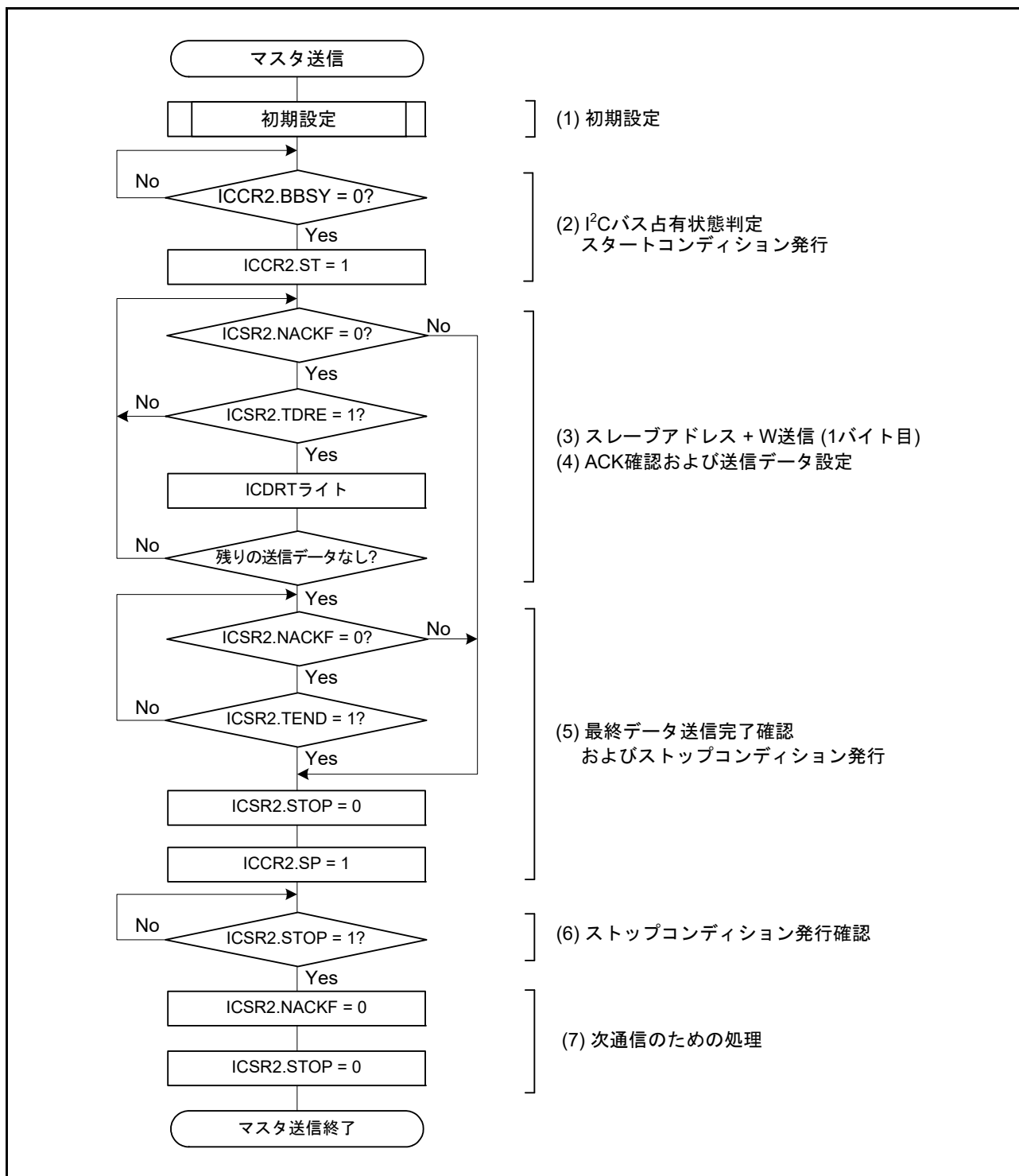
図 41.5 マスタ送信のフローチャート例
