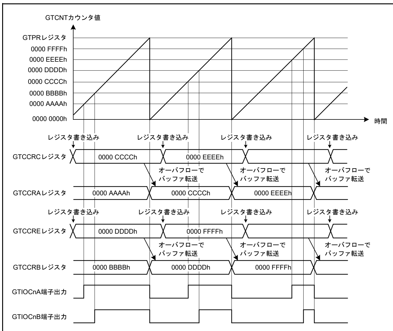
図 26.37 のこぎり波 PWM モード動作例 (アップカウント、バッファ動作、GTCCRA/GTCCRB レジスタのコンペアマッチで High 出力、周期の終わりで Low 出力の場合) (n = 0 ~ 3)
