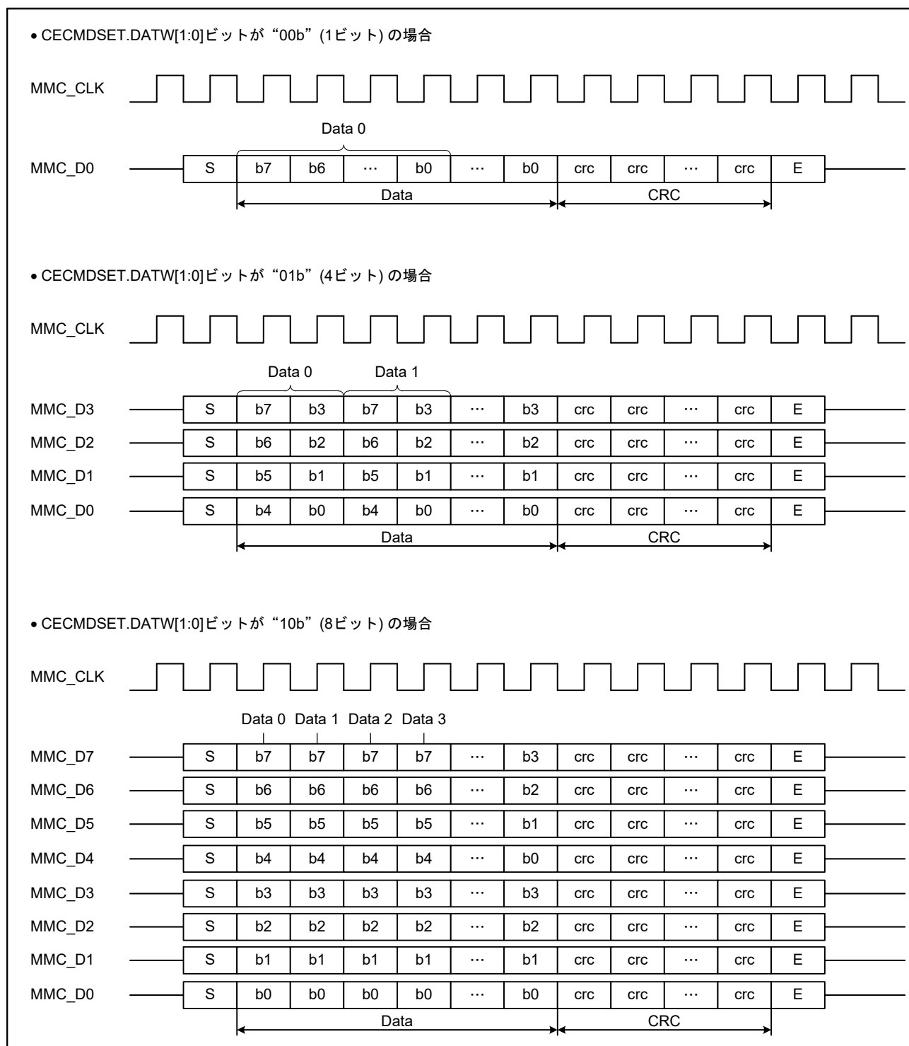
図 48.5 データブロックのフォーマット
