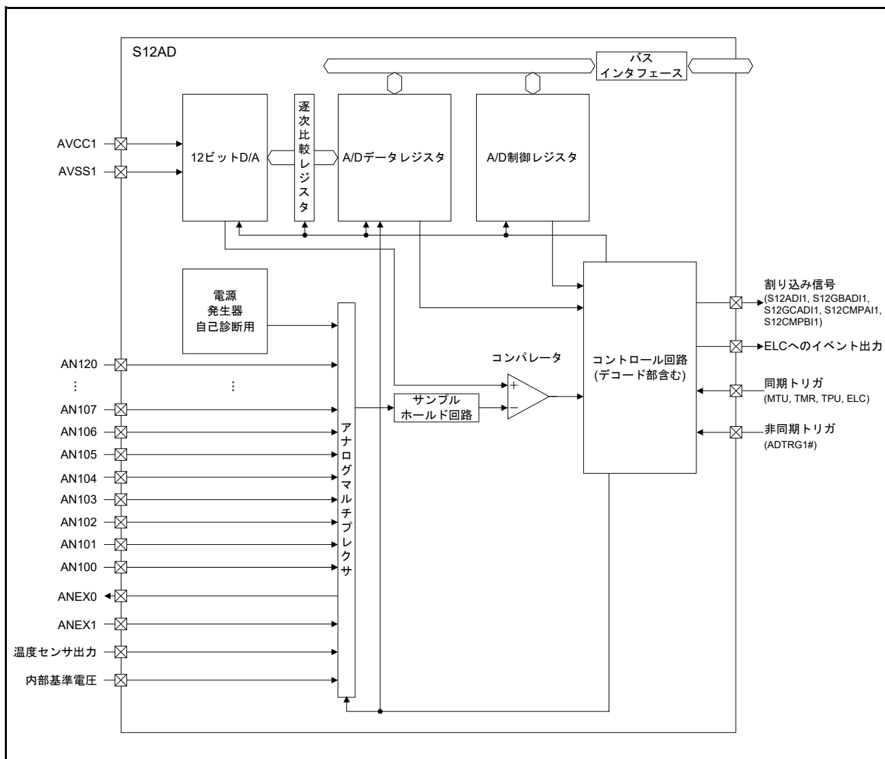
図 54.2 12ビットA/Dコンバータのブロック図 (ユニット1)
