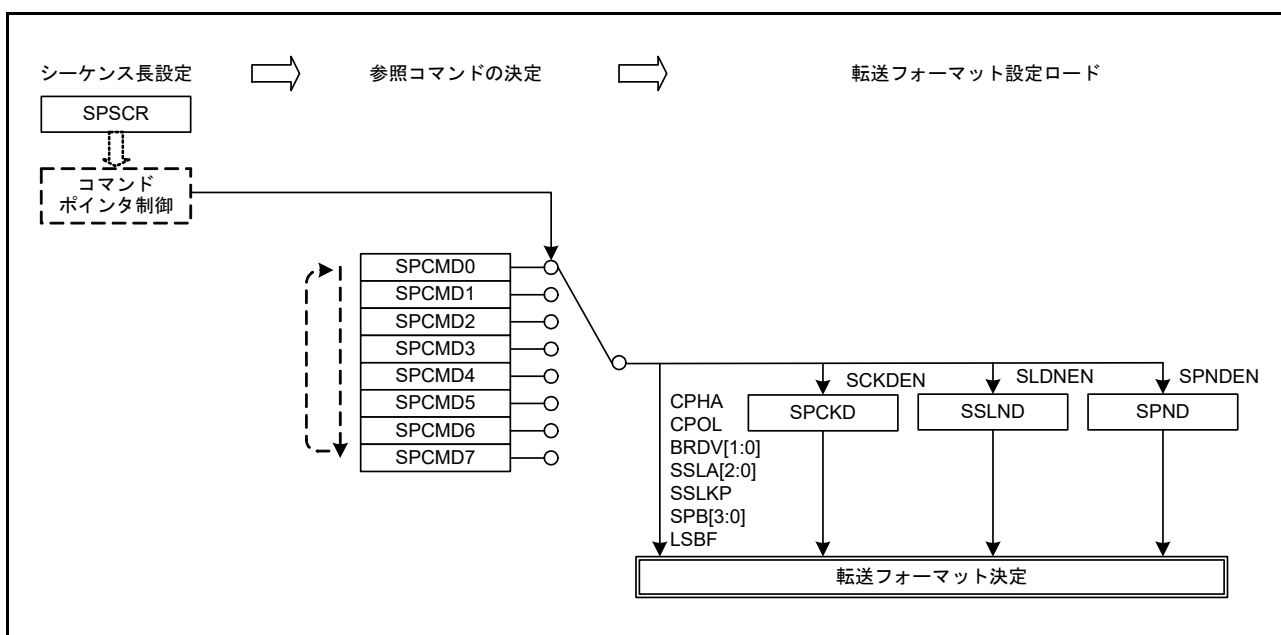
図 43.33 マスタモードでのシリアル転送方式の決定方法
