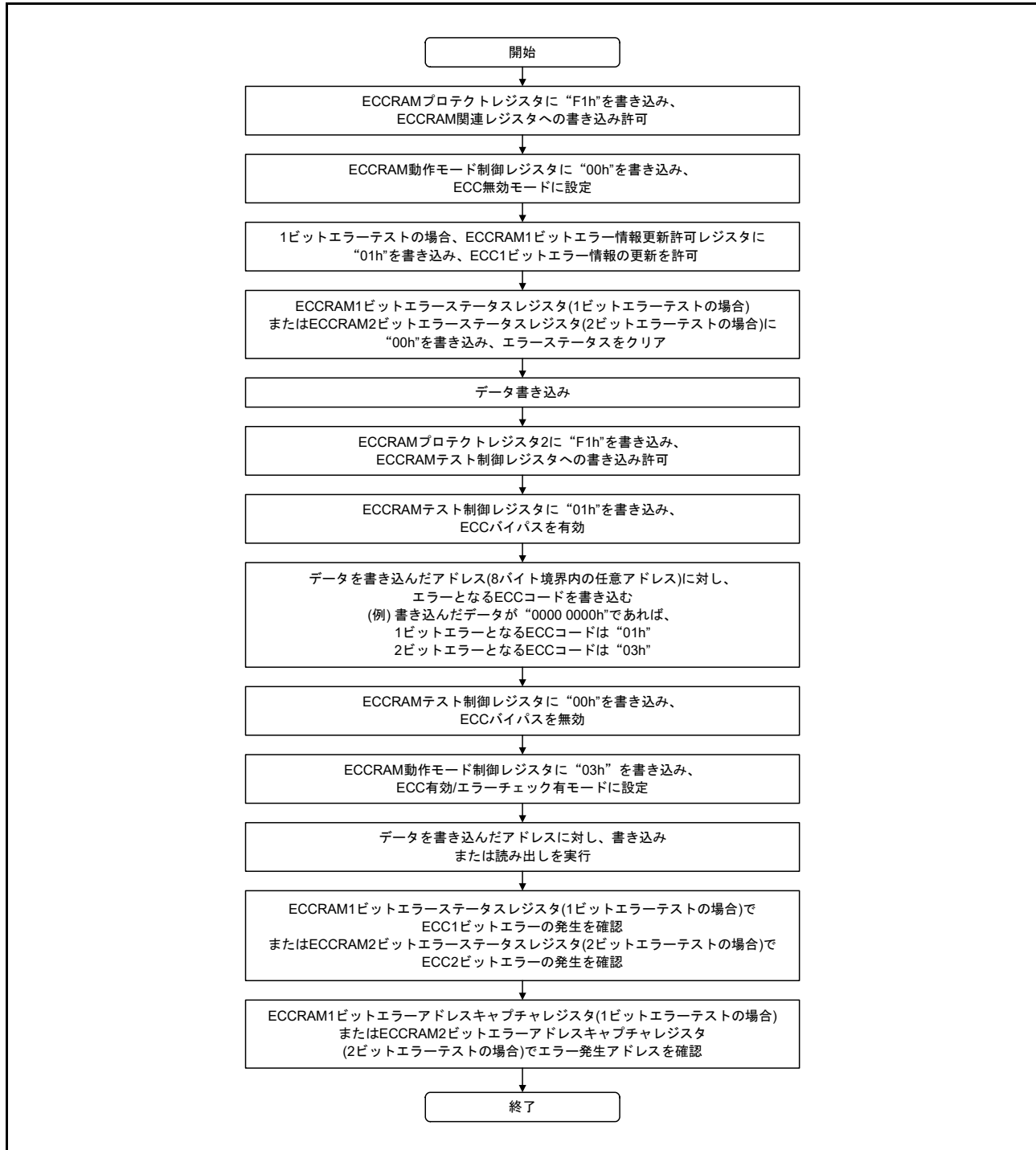
図 58.1 ECC コード制御回路テストフロー
