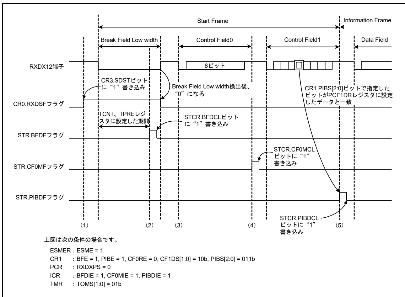
図 40.72 Start Frame の受信時の動作例 (プライオリティインタラプトビット使用時)
