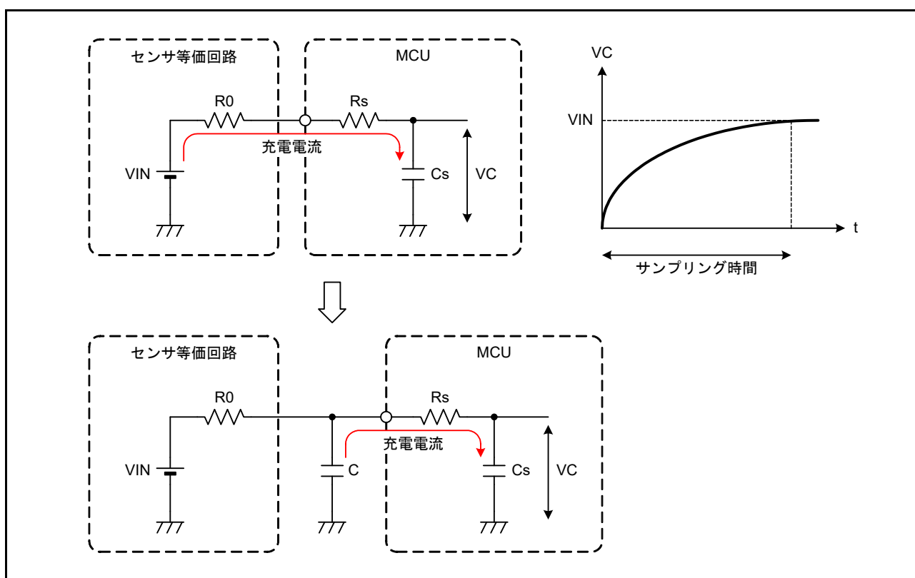
図 54.45 アナログ入力端子と外部センサの等価回路
