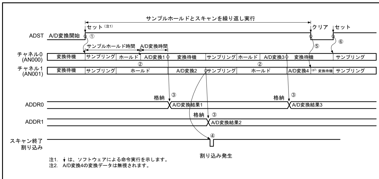
図 54.16 連続スキャンモードの動作例 (チャンネル専用サンプル & ホールド回路使用 : AN000, AN001 選択、常時サンプリング無効)
