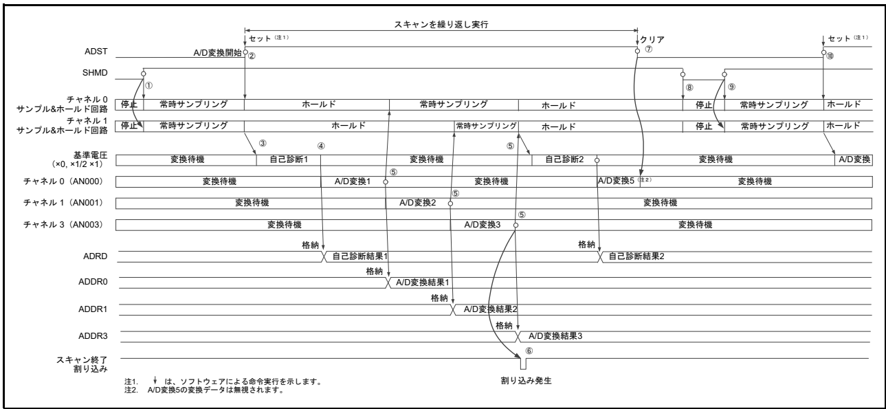
図 54.20 連続スキャンモードの動作例 (チャンネル専用サンプル & ホールド回路使用 : AN000, AN001, AN003 選択 + 自己診断、常時サンプリング有効)
