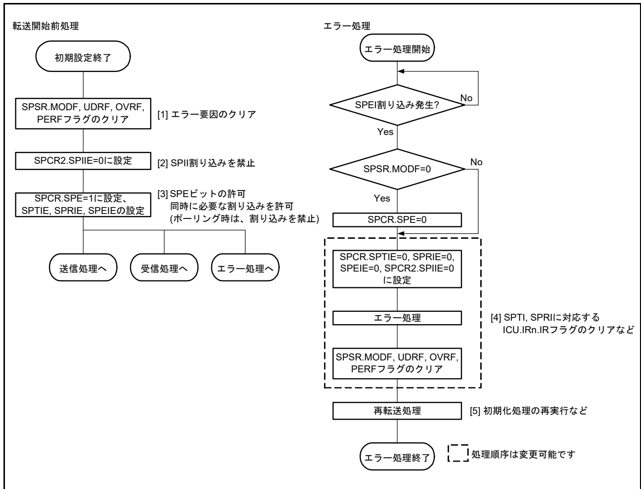
図 43.44 スレーブモード時のフローチャート (エラー処理)
