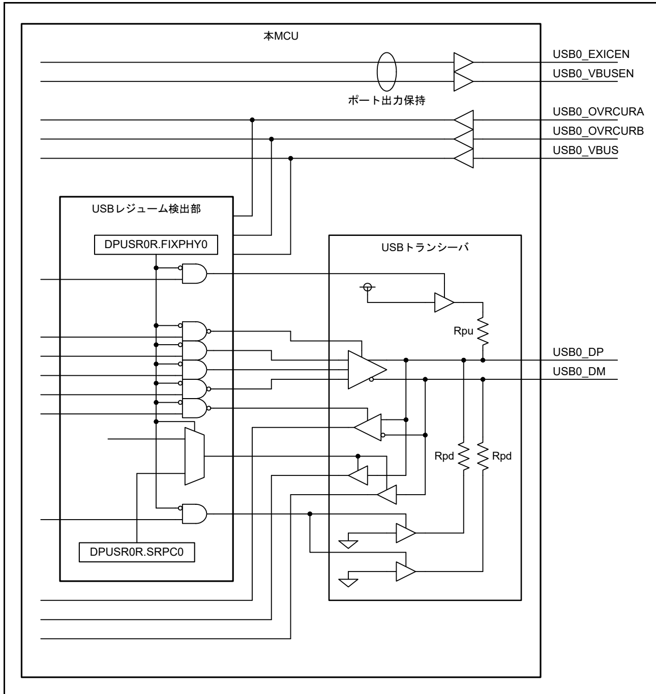
図 39.6 USB レジューム検出部と USB0 用入出力端子の接続概略図
