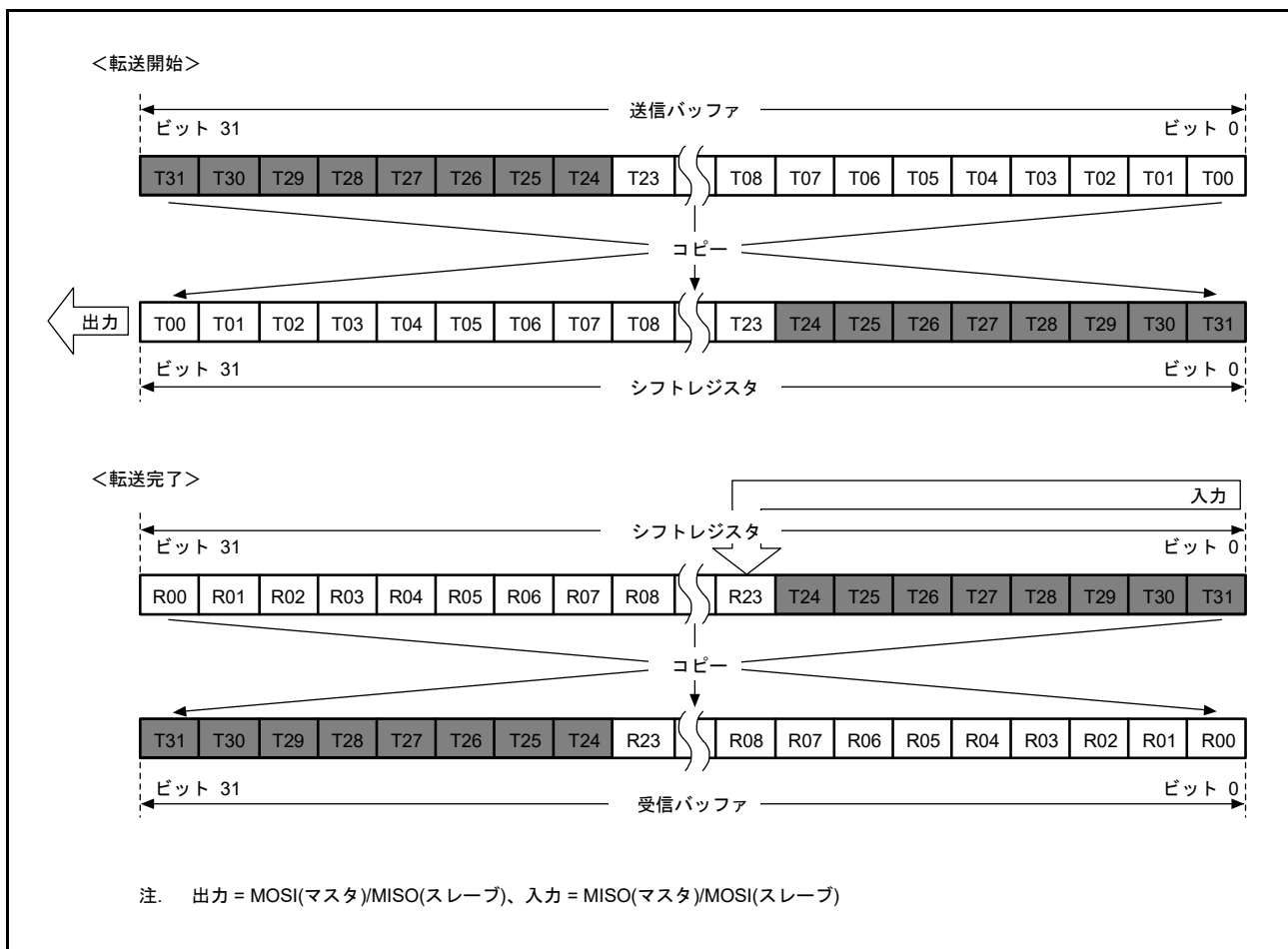
図 43.17 LSB ファースト (24 ビットデータ / パリティ機能無効)
