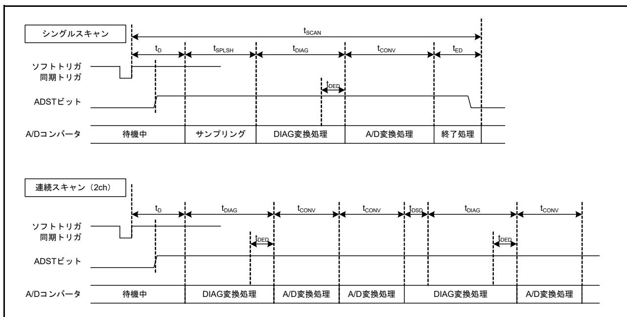
図 54.38 スキャン変換のタイミング (ソフトウェア起動、同期トリガ起動の場合)
