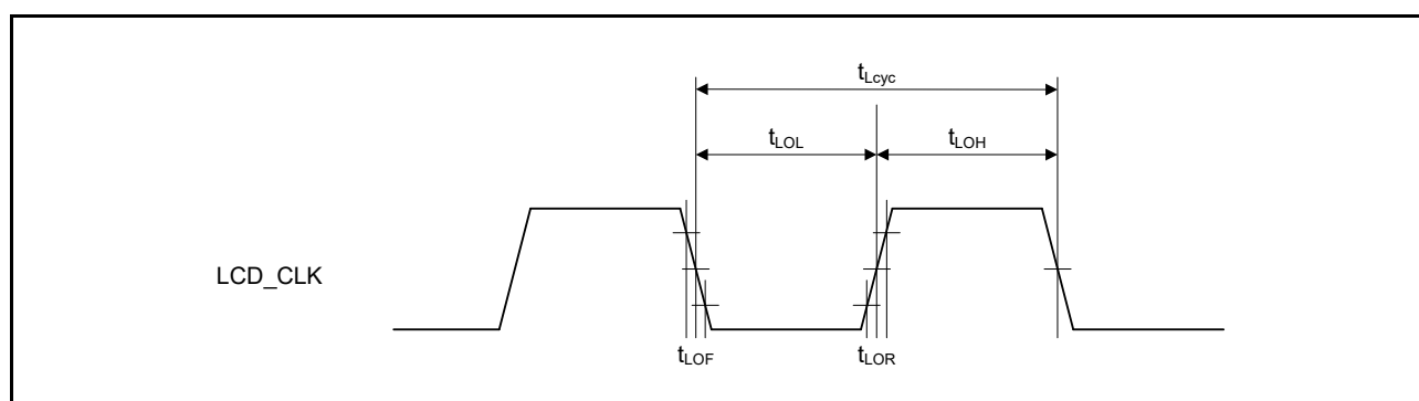
図 61.95 LCD_CLK クロック出カタイミング
