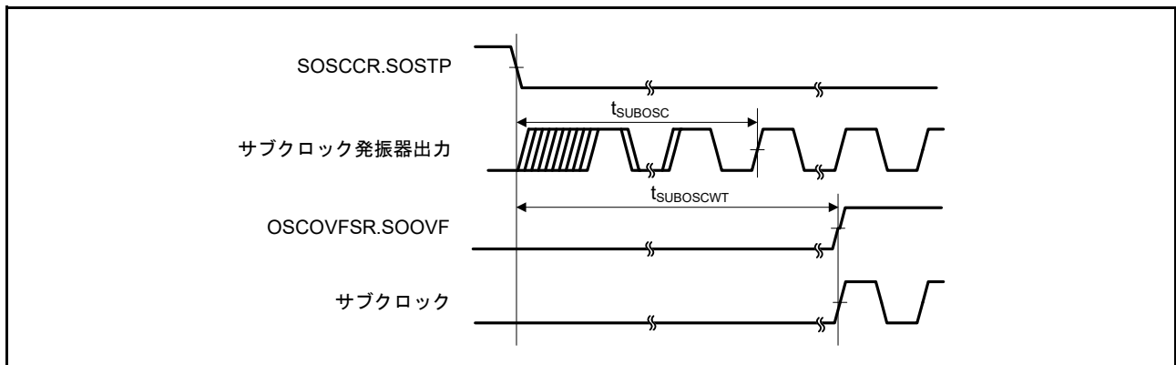
図 61.11 サブクロック発振開始タイミング
