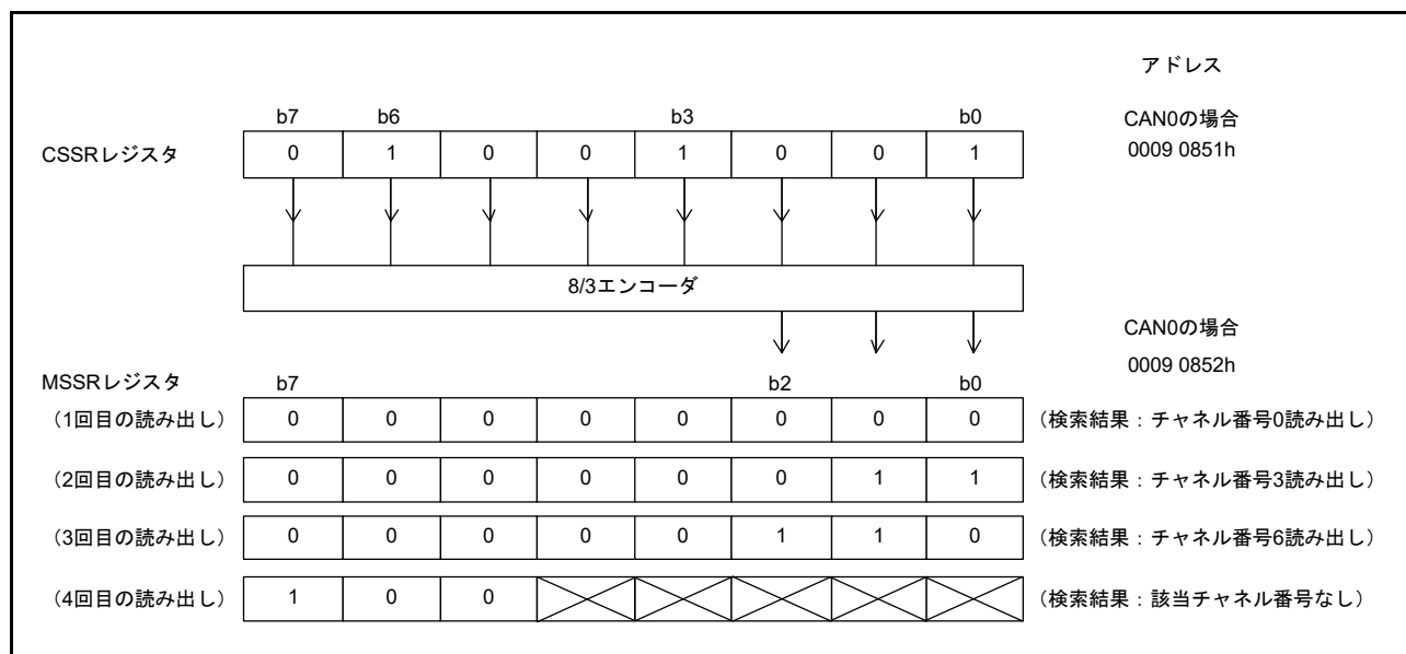
図 42.4 CSSR、MSSR レジスタの書き込みと読み出し
