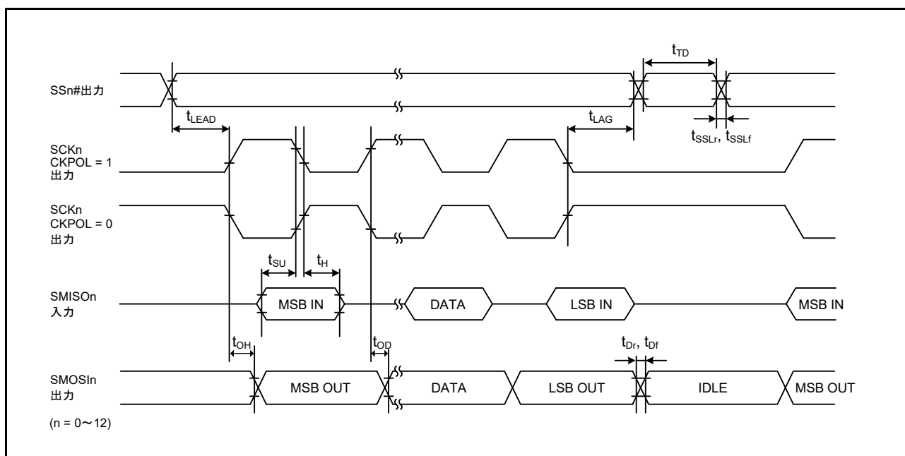
図 61.59 簡易 SPI タイミング (マスタ、CKPH = 0)
