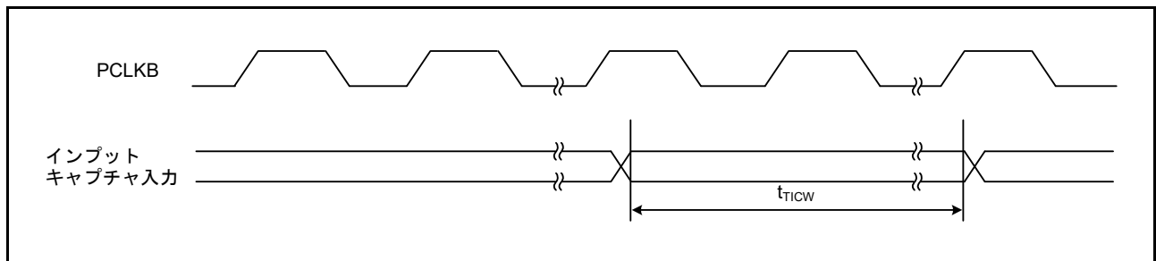
図 61.36 TPU インプットキャプチャ入力タイミング
