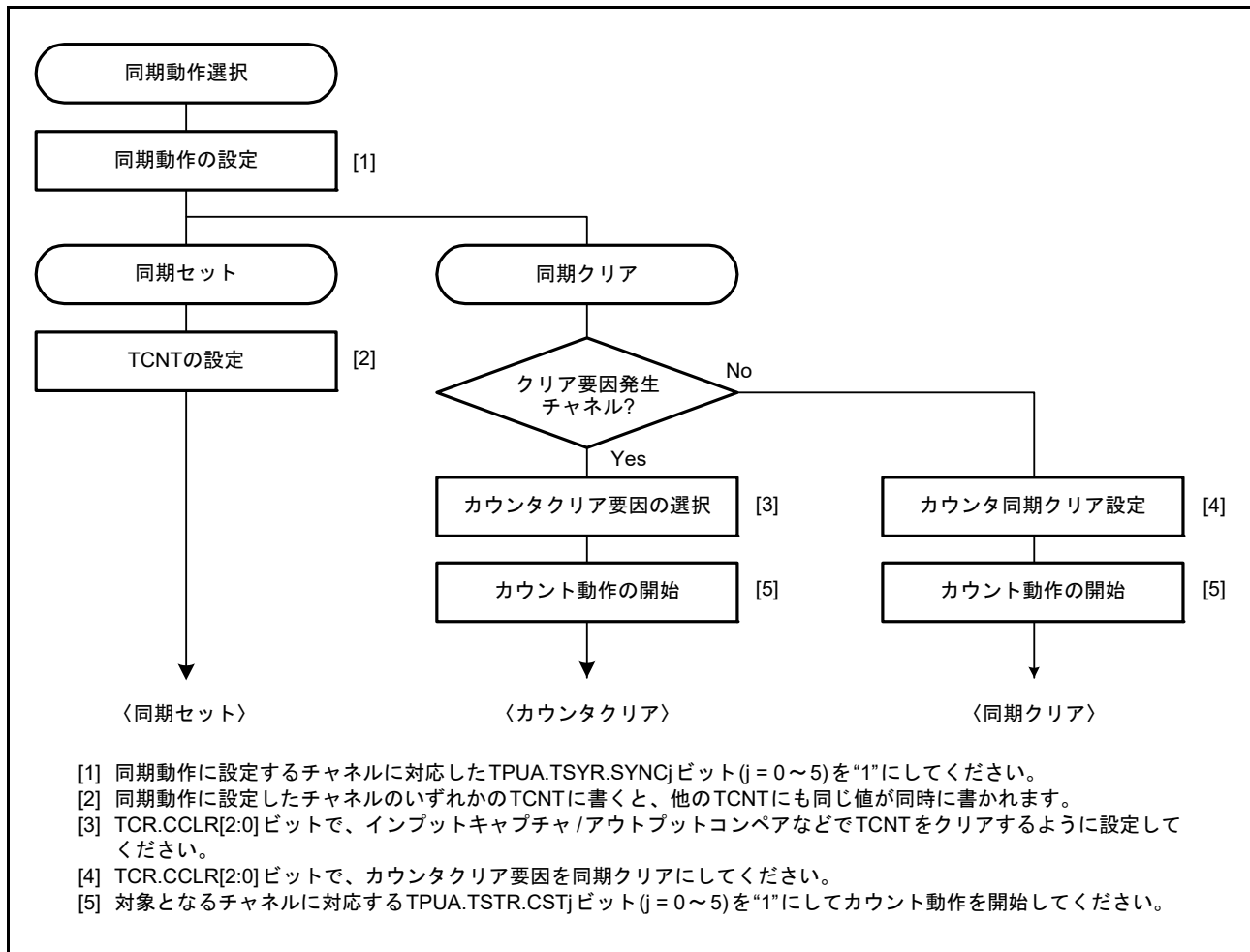
図 28.10 同期動作の設定手順例
