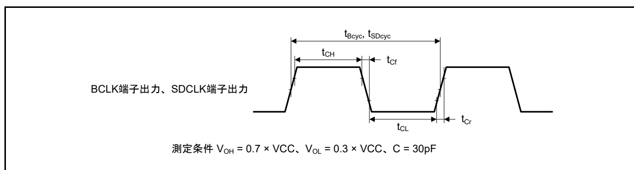
図 61.3 BCLK 端子出力、SDCLK 端子出力タイミング
