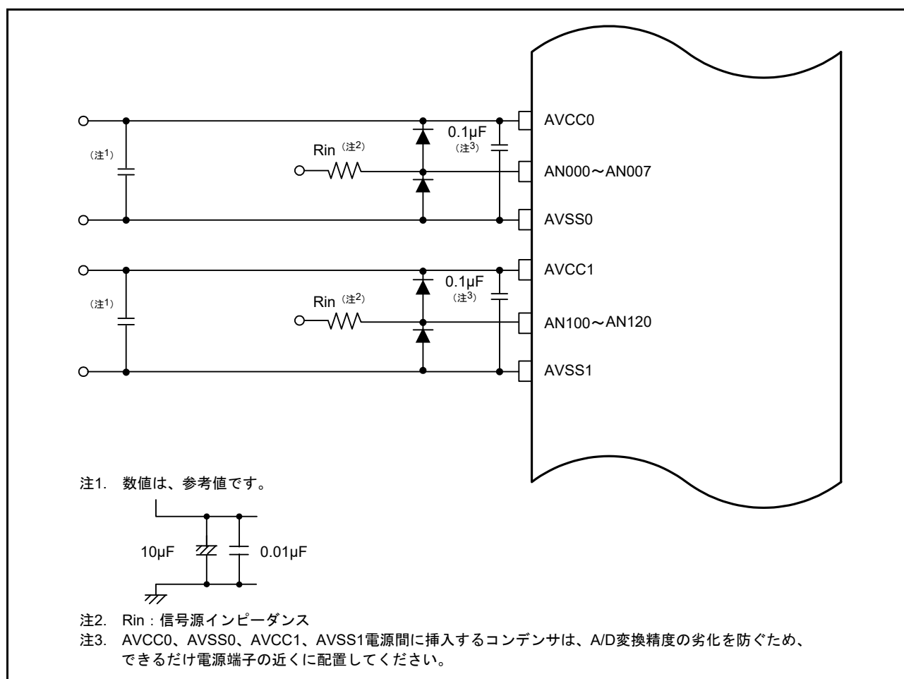
図 54.48 アナログ入力保護回路の例
