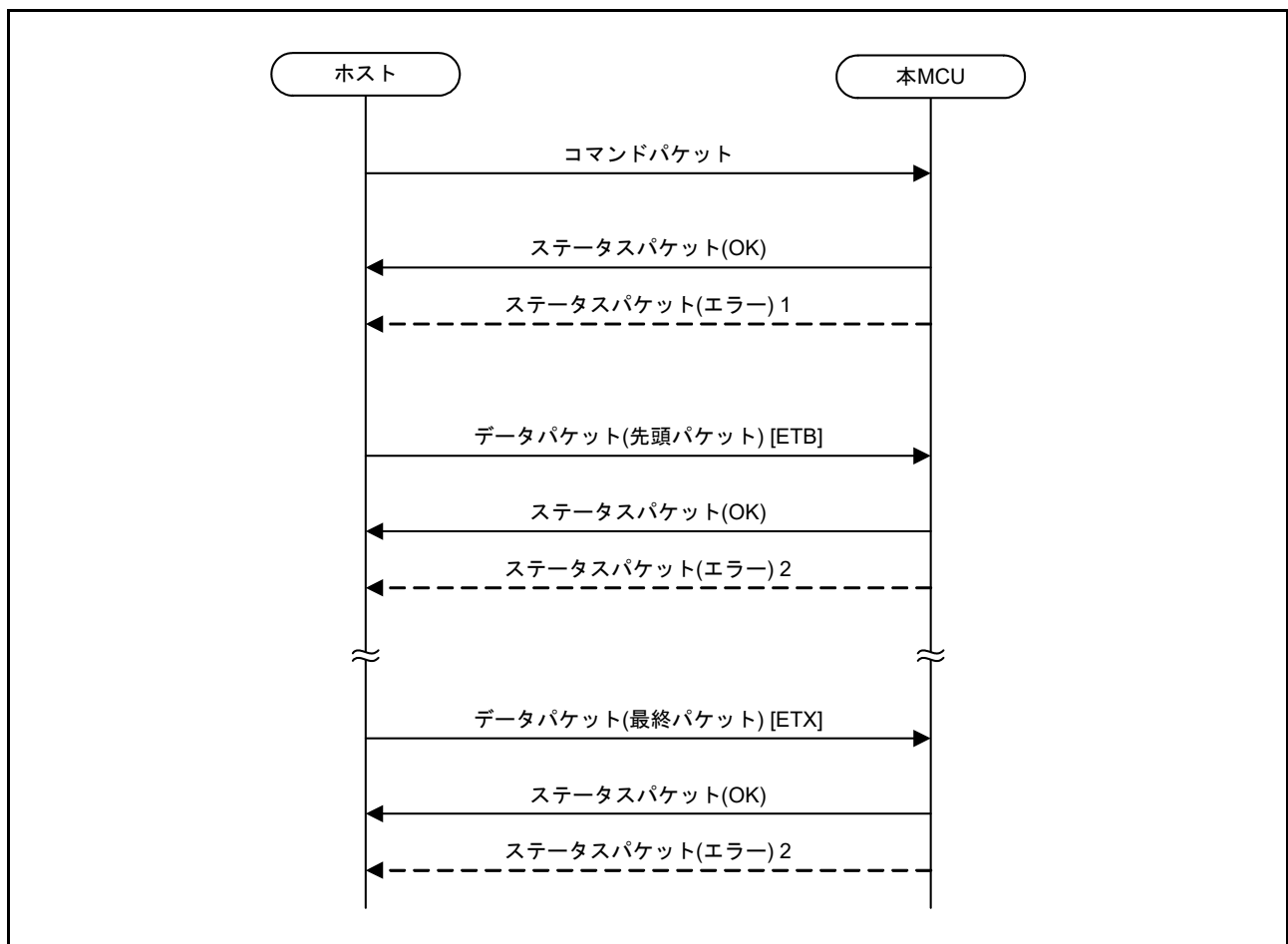
図 60.46 プログラムコマンドの通信シーケンス
