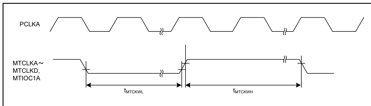
図 61.41 MTU クロック入力タイミング
