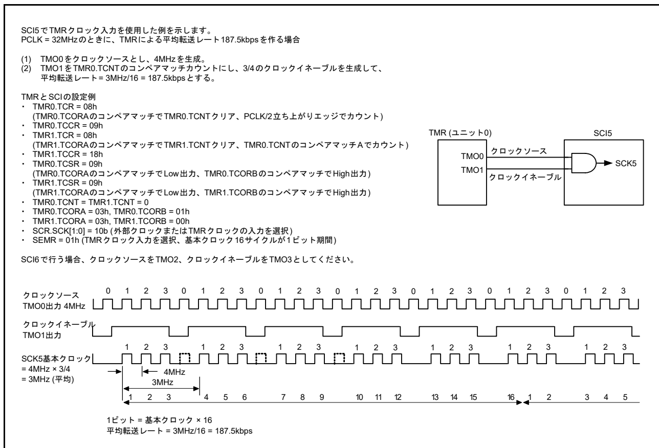
図 40.5 TMR クロック入力時の平均転送レート設定例
