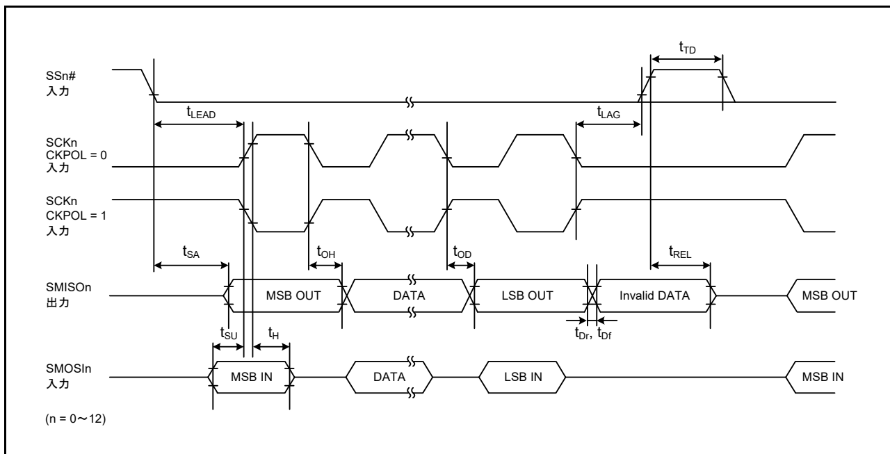
図 61.60 簡易 SPI タイミング (スレーブ、CKPH = 1)
