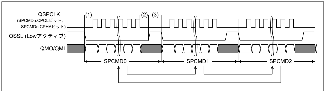
図 44.12 シーケンス制御動作例 (n = 0 ~ 3)
