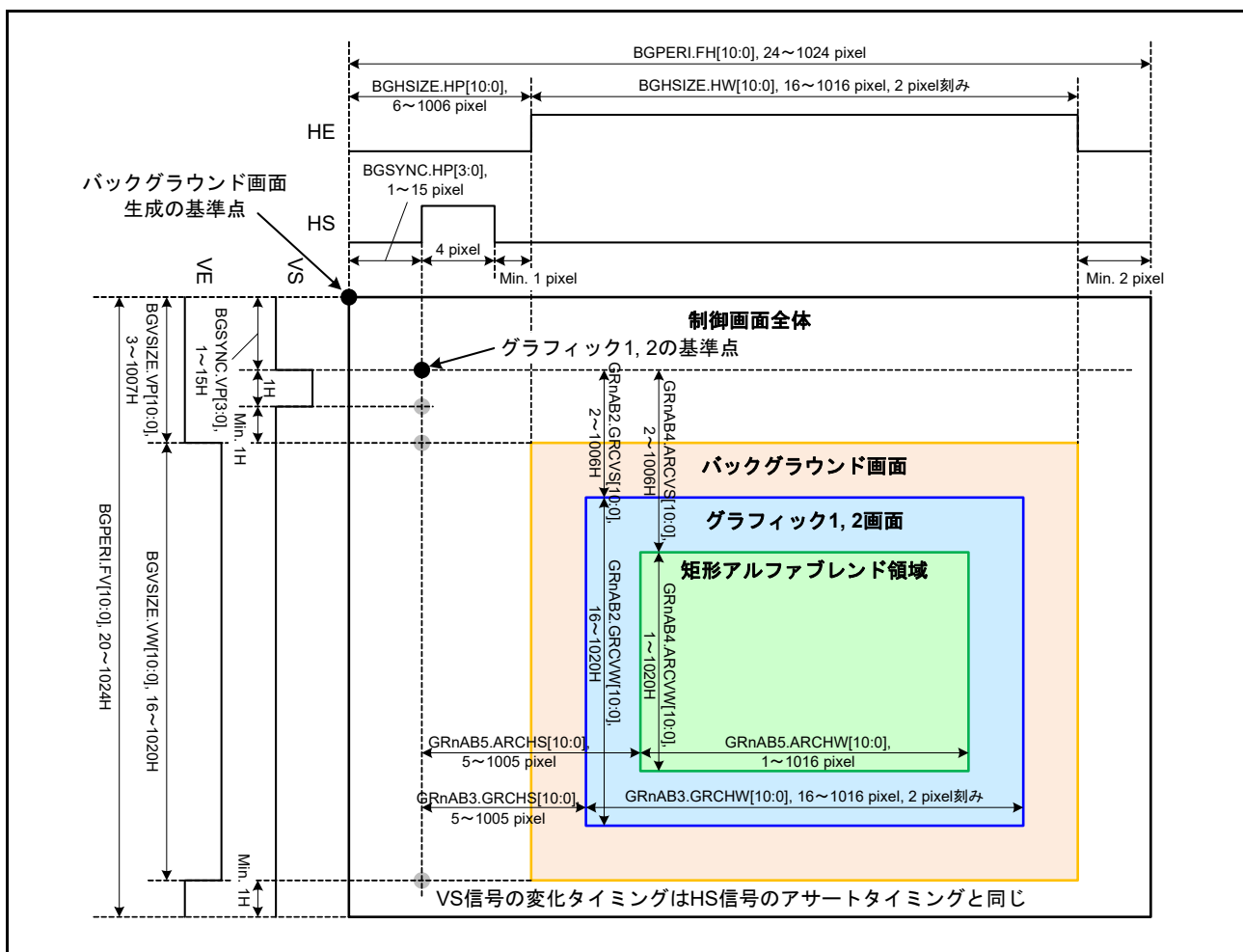
図 50.24 画面の定義
