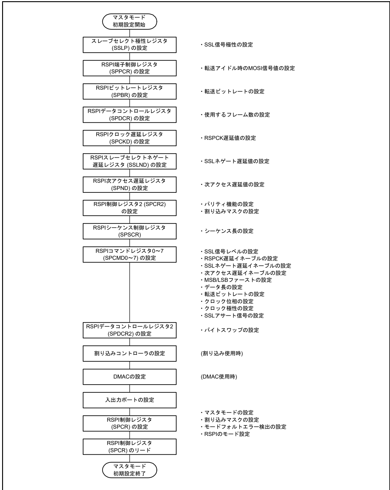
図 43.37 マスタモード時の初期化フロー例 (SPI 動作)
