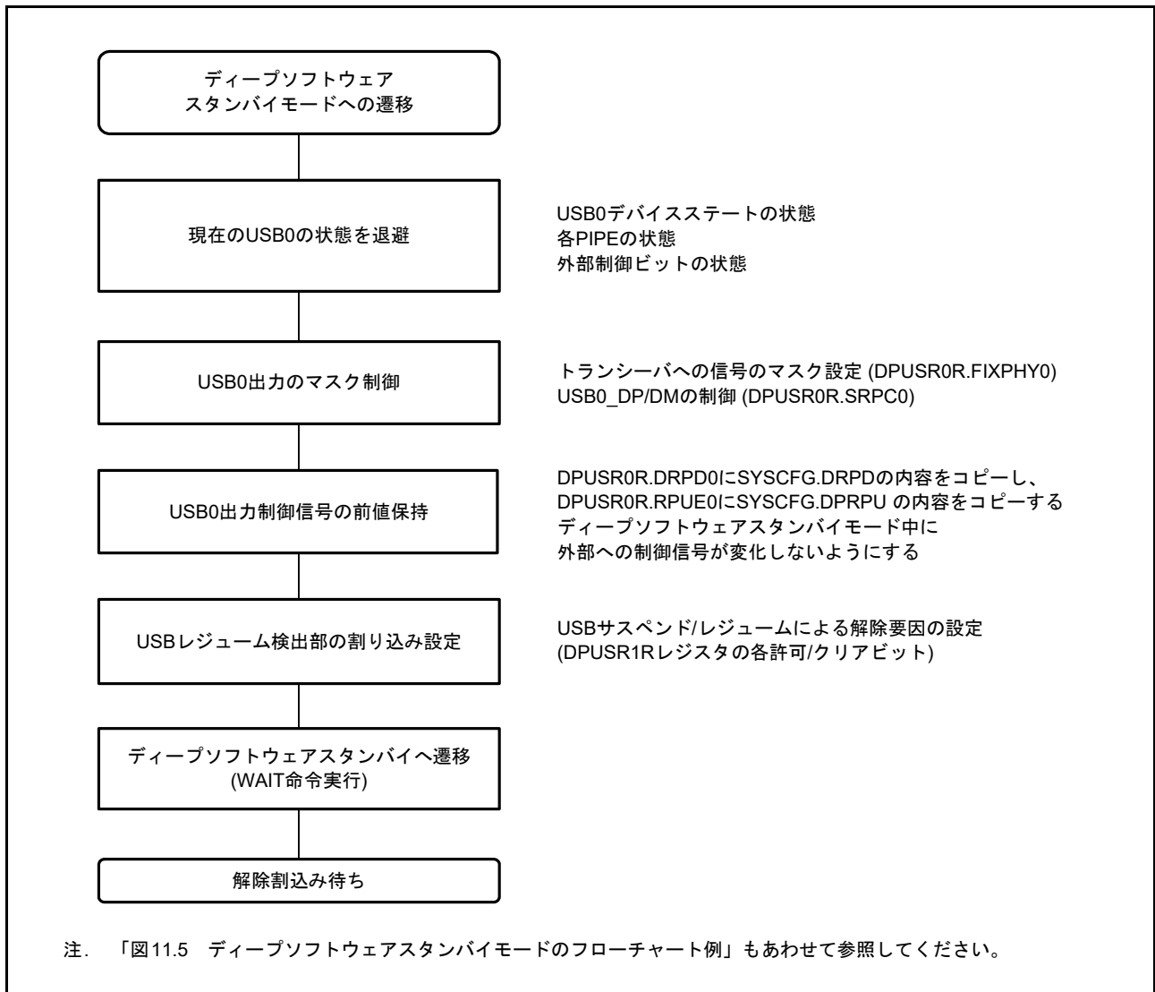
図 39.7 ホスト時またはファンクション時のディープソフトウェアスタンバイ遷移時の USB 設定フロー
