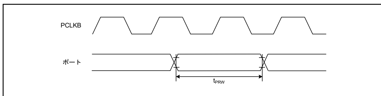
図 61.35 I/Oポート入力タイミング
