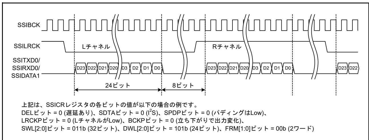
図 46.8 パディングビットの挿入例 (I 2 S フォーマット、システムワード長 > データワード長)
