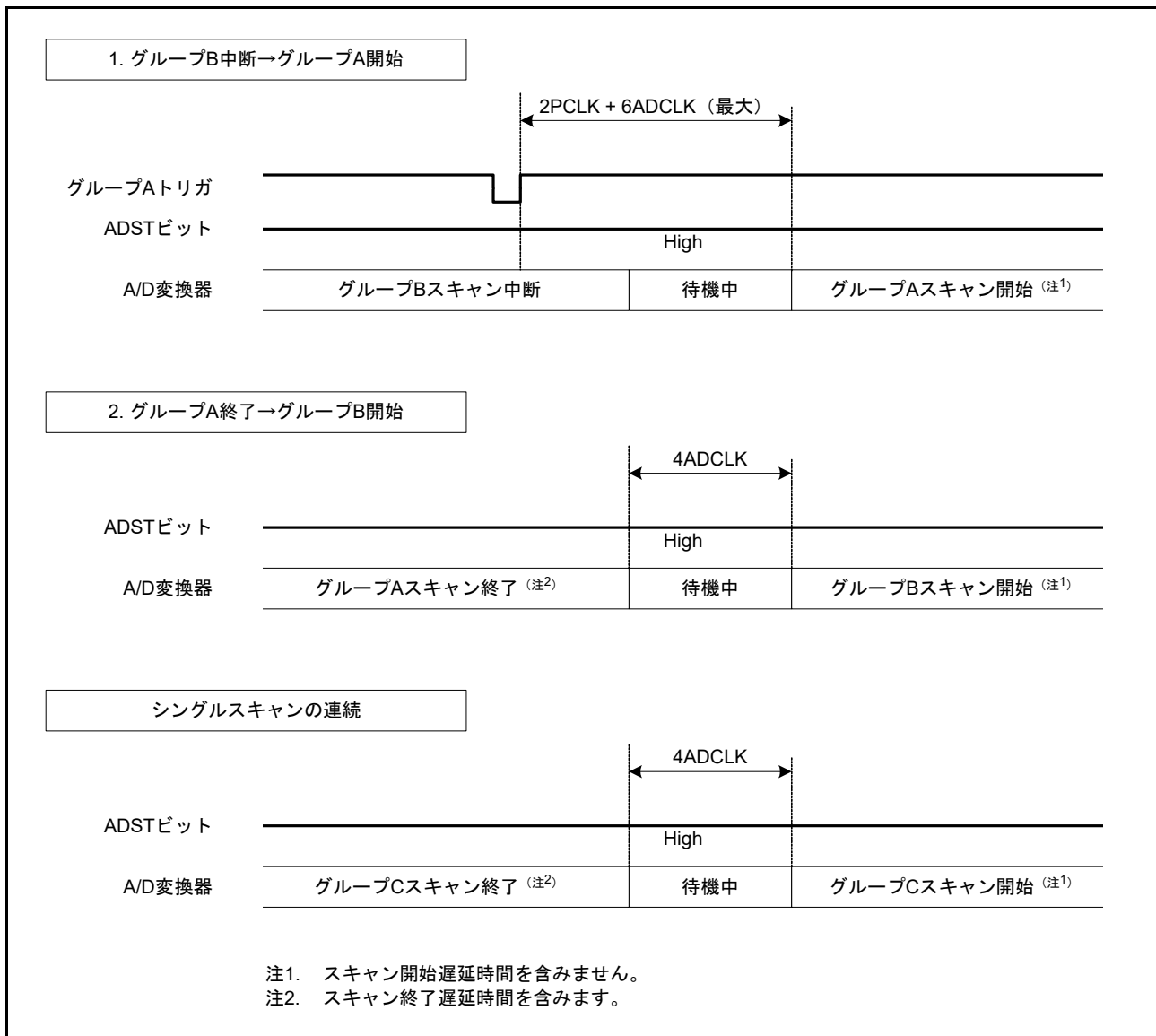
図 54.40 グループ優先でのスキャン停止 / 起動タイミング
