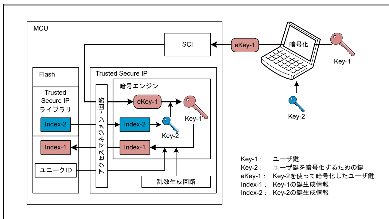
図 53.4 鍵インストール概念図
