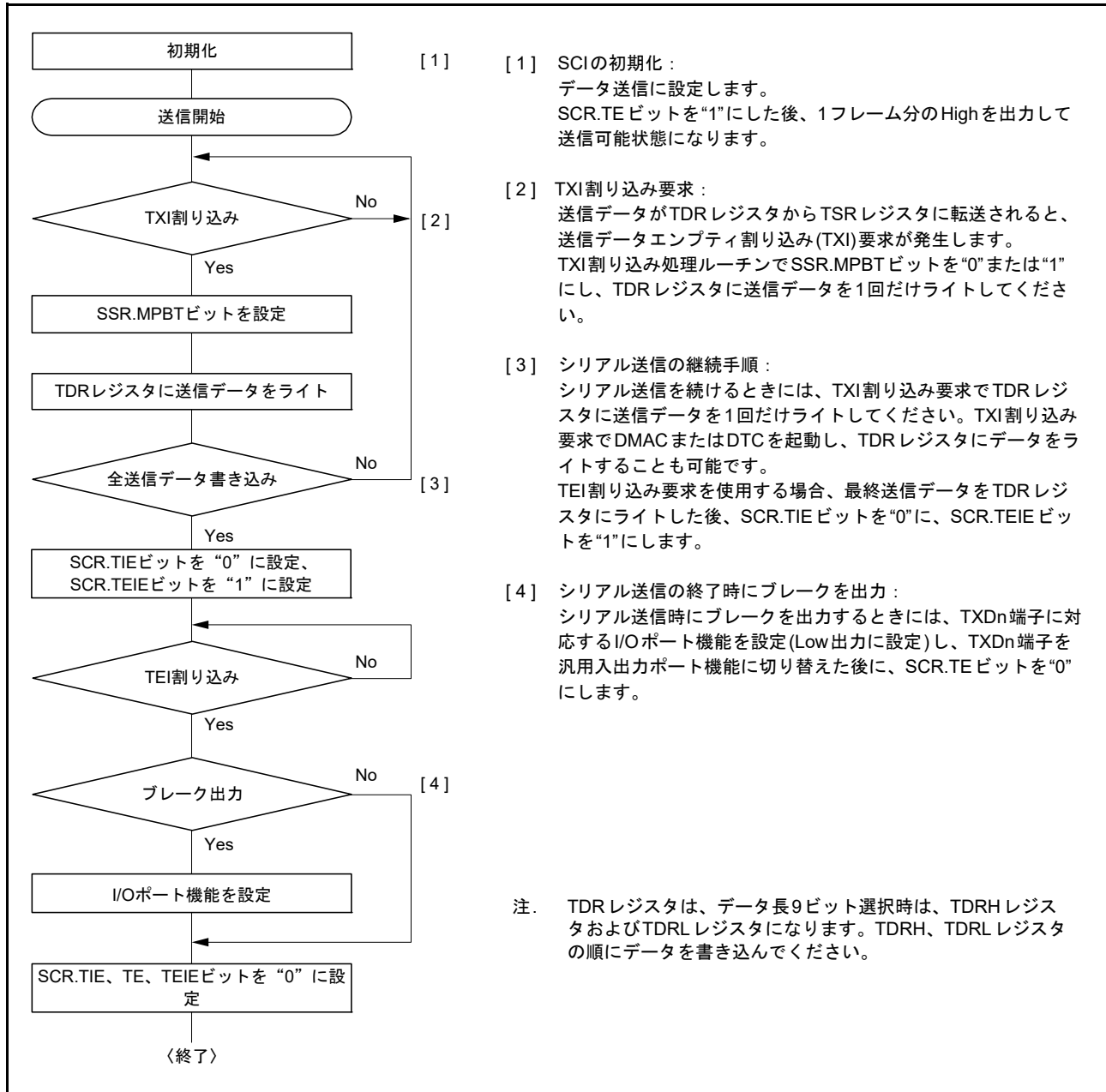
図 40.23 マルチプロセッサシリアル送信のフローチャートの例
