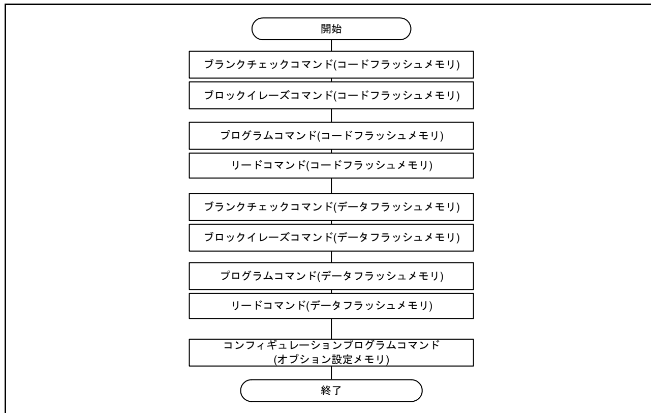
図 60.49 書き換え方法の例
