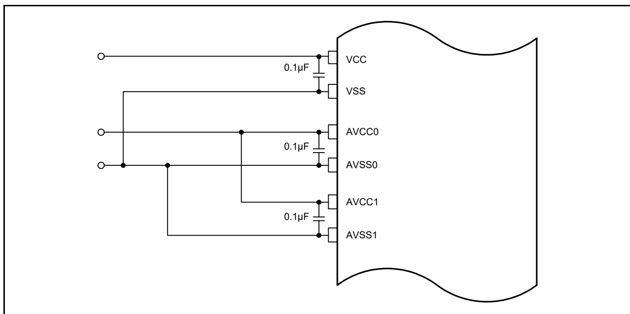
図 54.47 各電源端子の接続例
