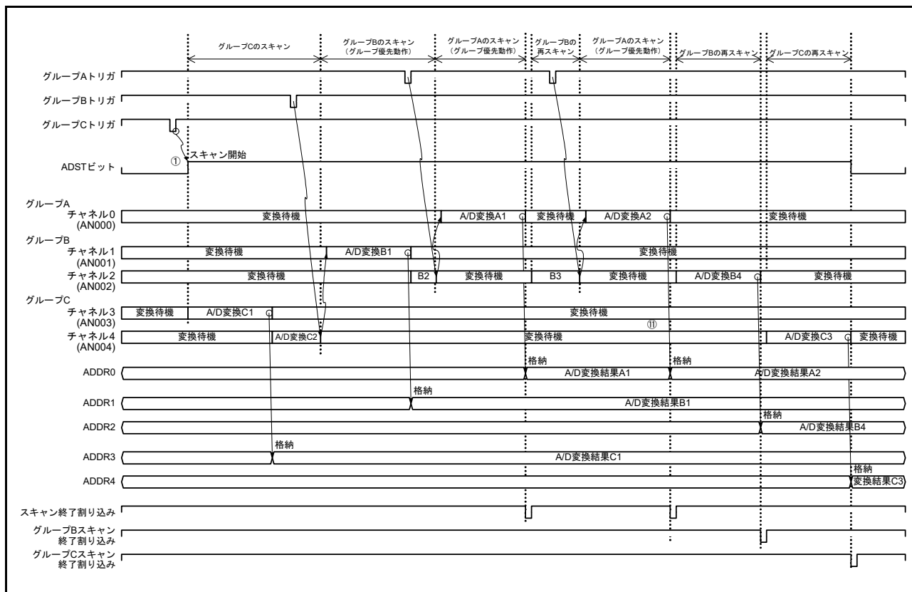
図 54.31 グループ優先動作の例 2 「低優先グループ再スキャン中の優先グループトリガ入力」再スキャンあり (ADGSPCR.GBRSCN = 1, ADGSPCR.GBRP = 0, ADGSPCR.LGRRS = 1 設定時)
