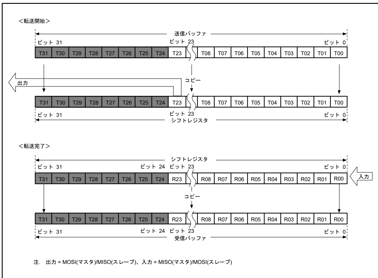
図 43.15 MSB ファースト転送 (24 ビットデータ / パリティ機能無効)
