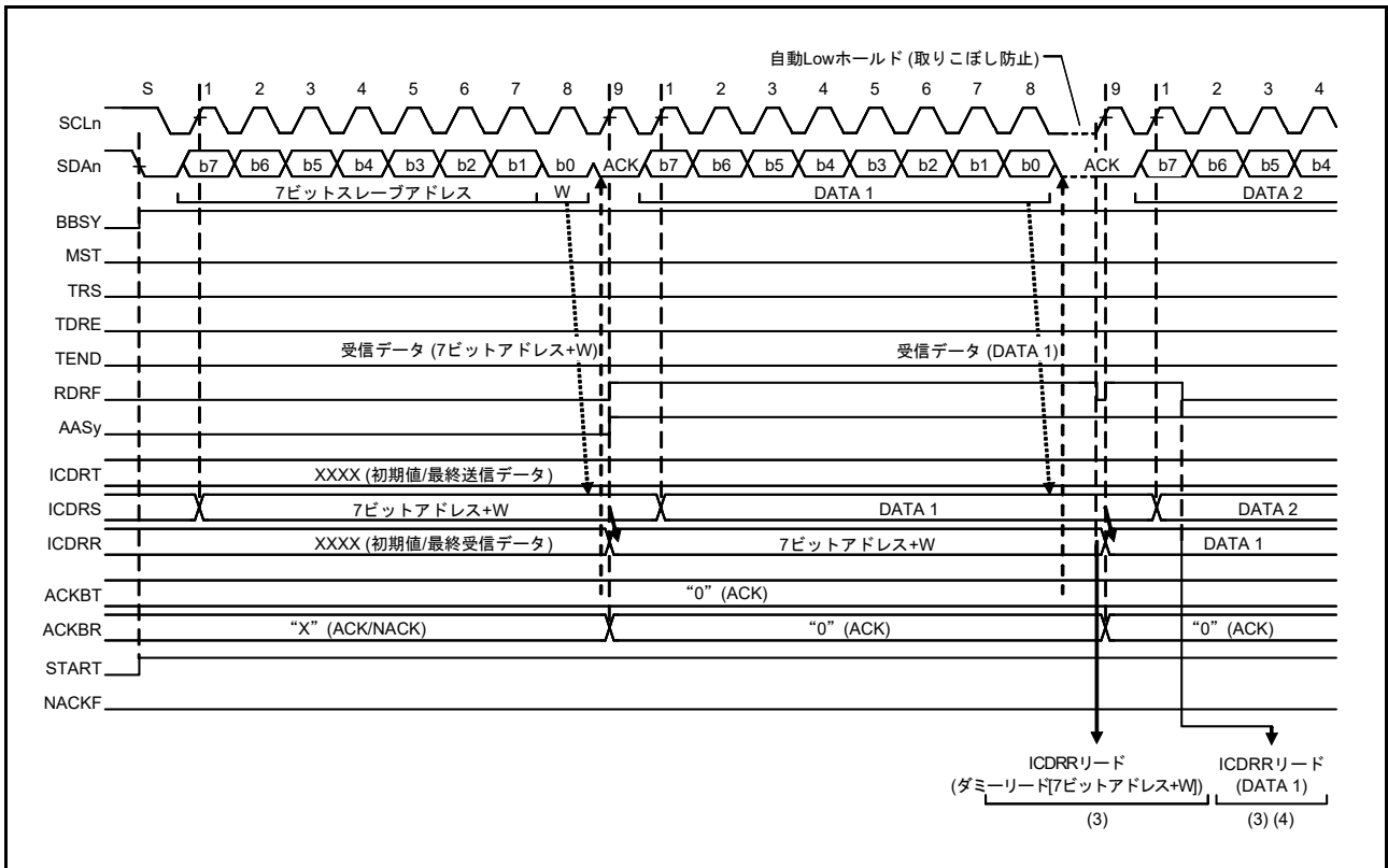
図 41.18 スレーブ受信の動作タイミング (1) (7 ビットアドレスフォーマット、RDRFS ビット = 0 のとき)
