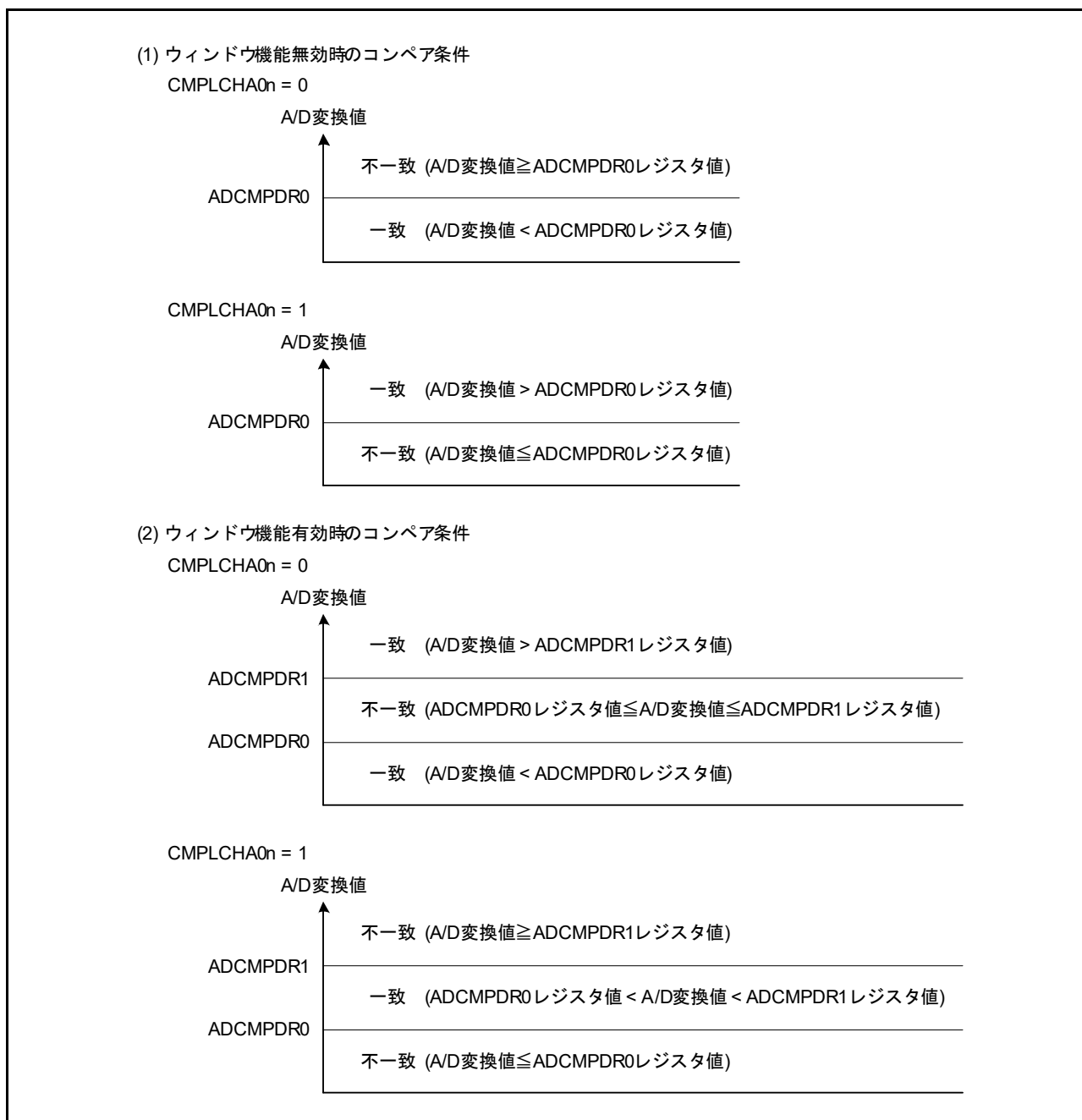
図 54.4 コンペア機能ウィンドウ A コンペア条件説明
