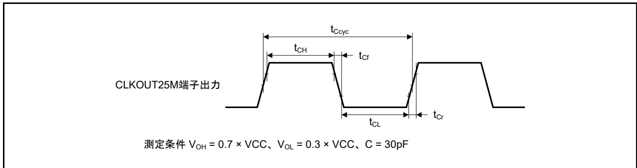
図 61.13 CLKOUT25M 端子出カタイミング
