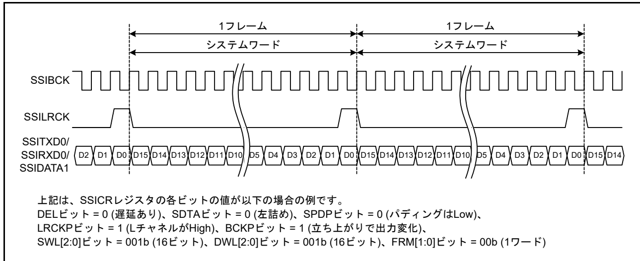
図 46.12 モノラルフォーマットの例 (1) (SSICR.DEL ビット = 0、パディングなし)
