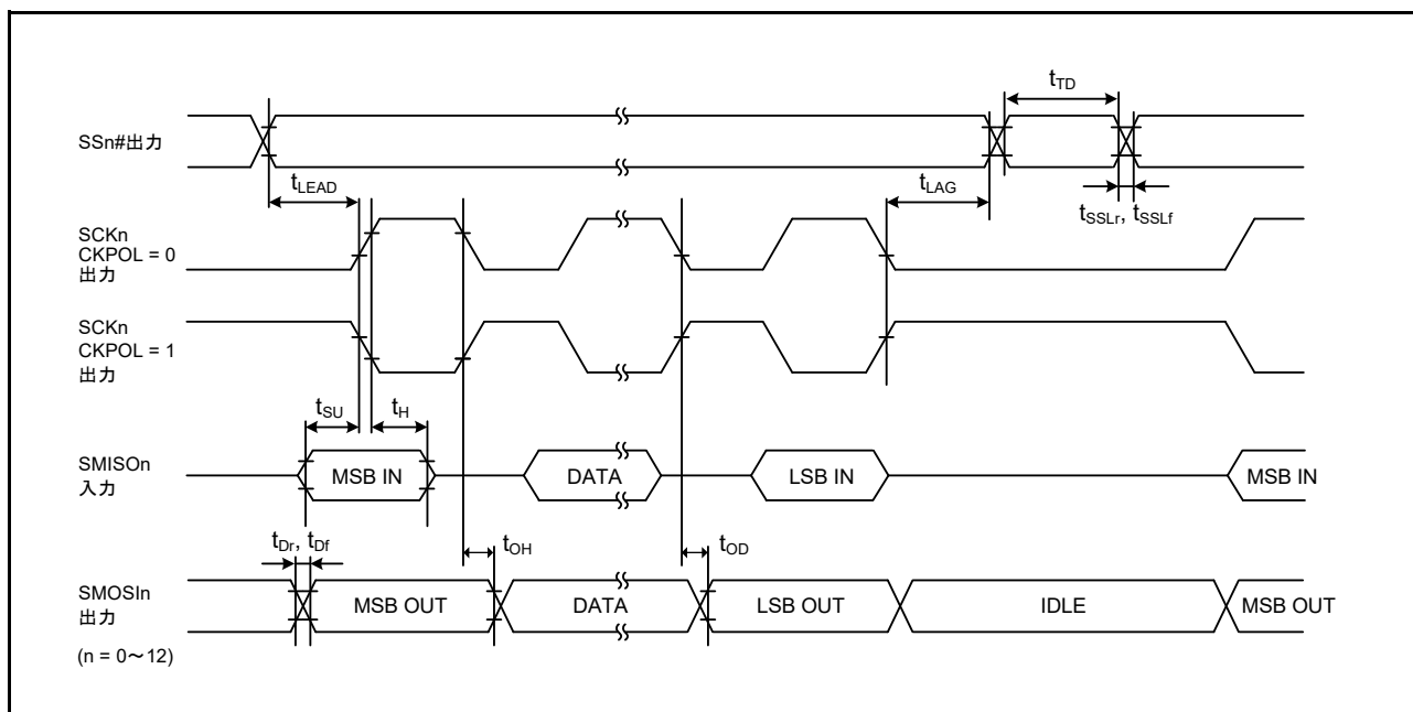
図 61.58 簡易 SPI タイミング (マスタ、CKPH = 1)
