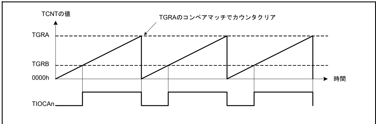
図 28.21 PWM モードの動作例 (1) (n = 0 ~ 5)
