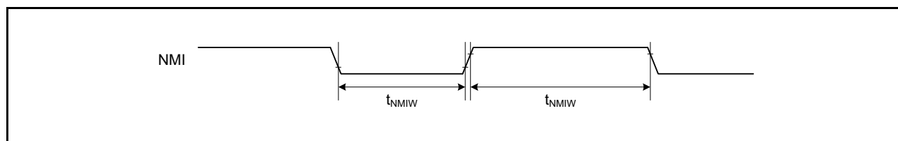
図 61.16 NMI 割り込み入カタイミング
