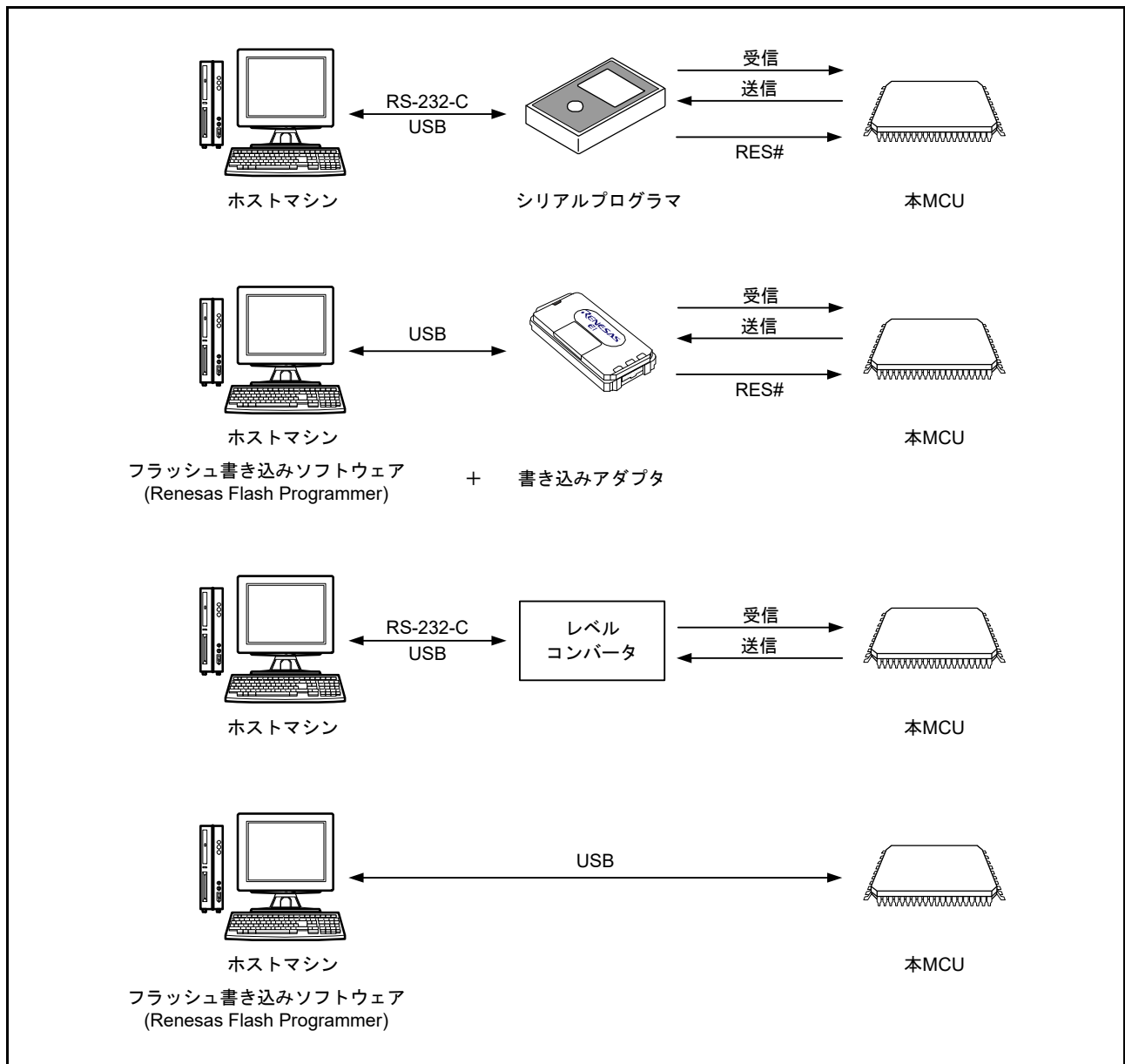
図 60.53 フラッシュメモリを書き換えるための環境
