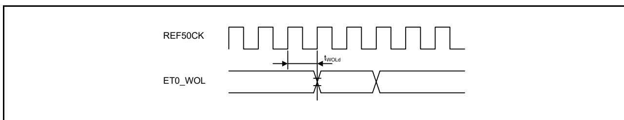
図 61.85 WOL 出カタイミング (RMII)
