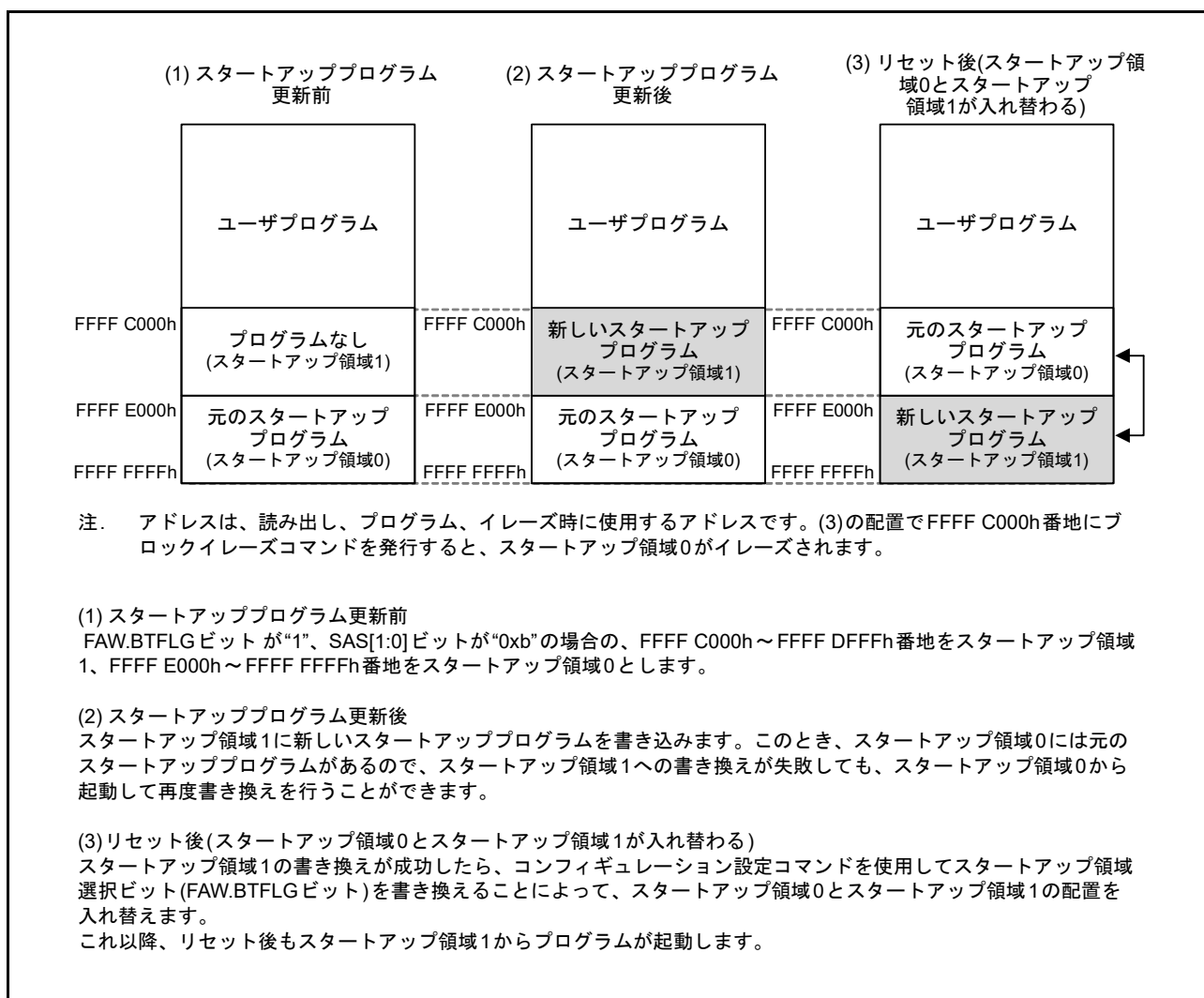
図 60.26 スタートアッププログラム保護機能の概念
