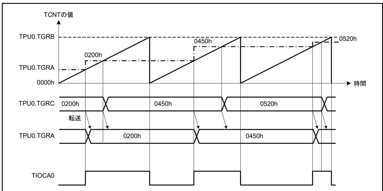
図 28.15 バッファ動作例 (1)
