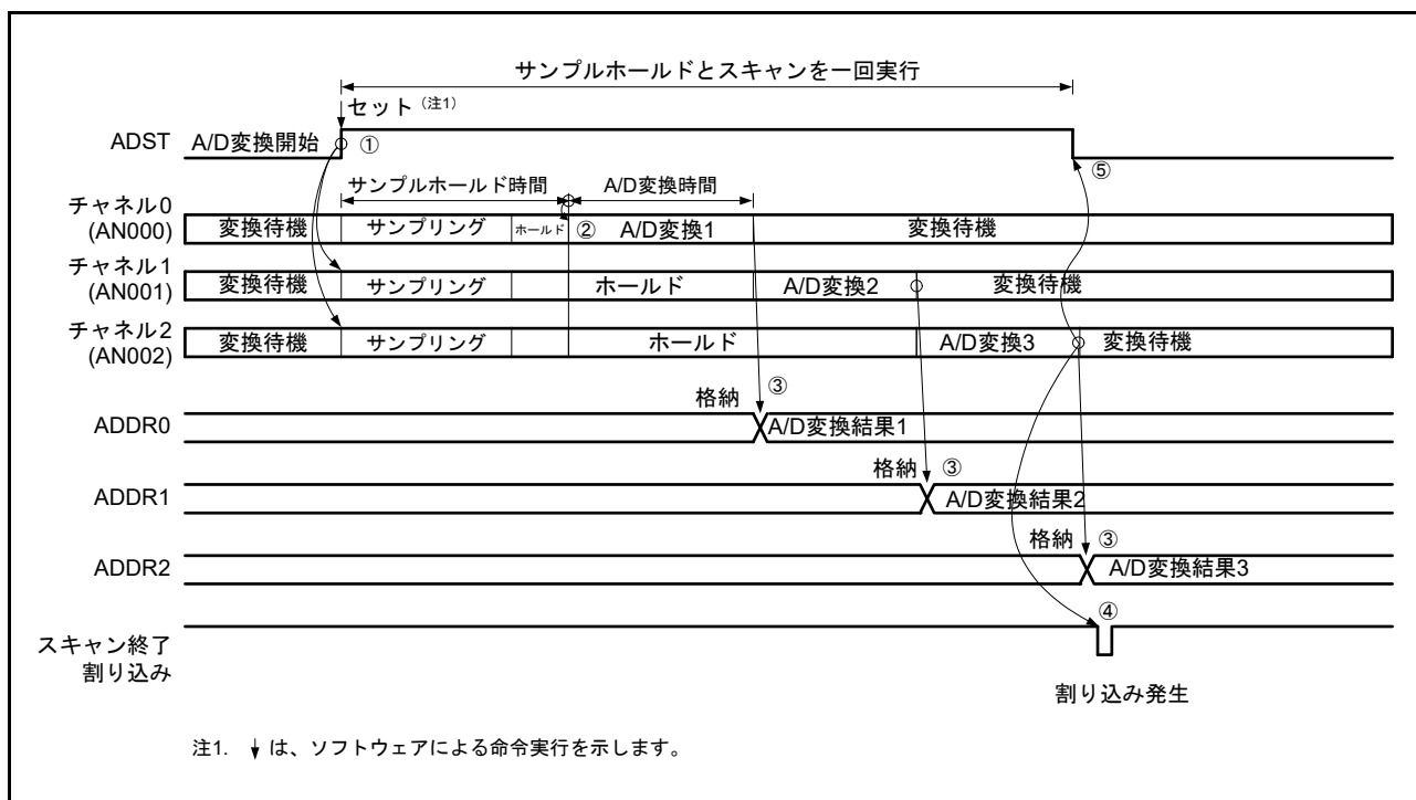
図 54.7 シングルスキャンモードの動作例 (チャンネル専用サンプル & ホールド回路使用チャンネル AN000, AN001, AN002 選択、常時サンプリング無効)
