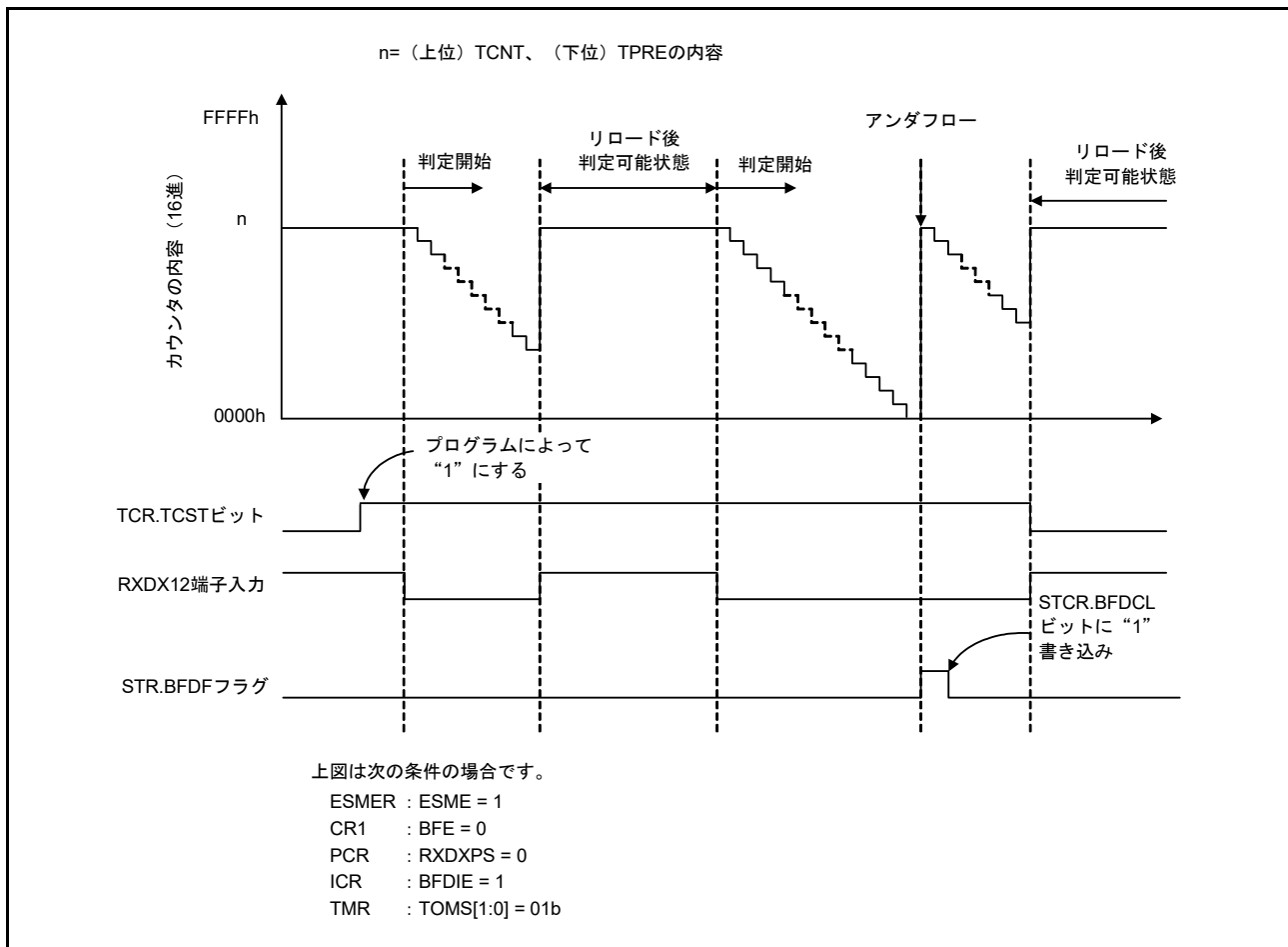
図 40.78 Break Field Low width 判定モードの動作例
