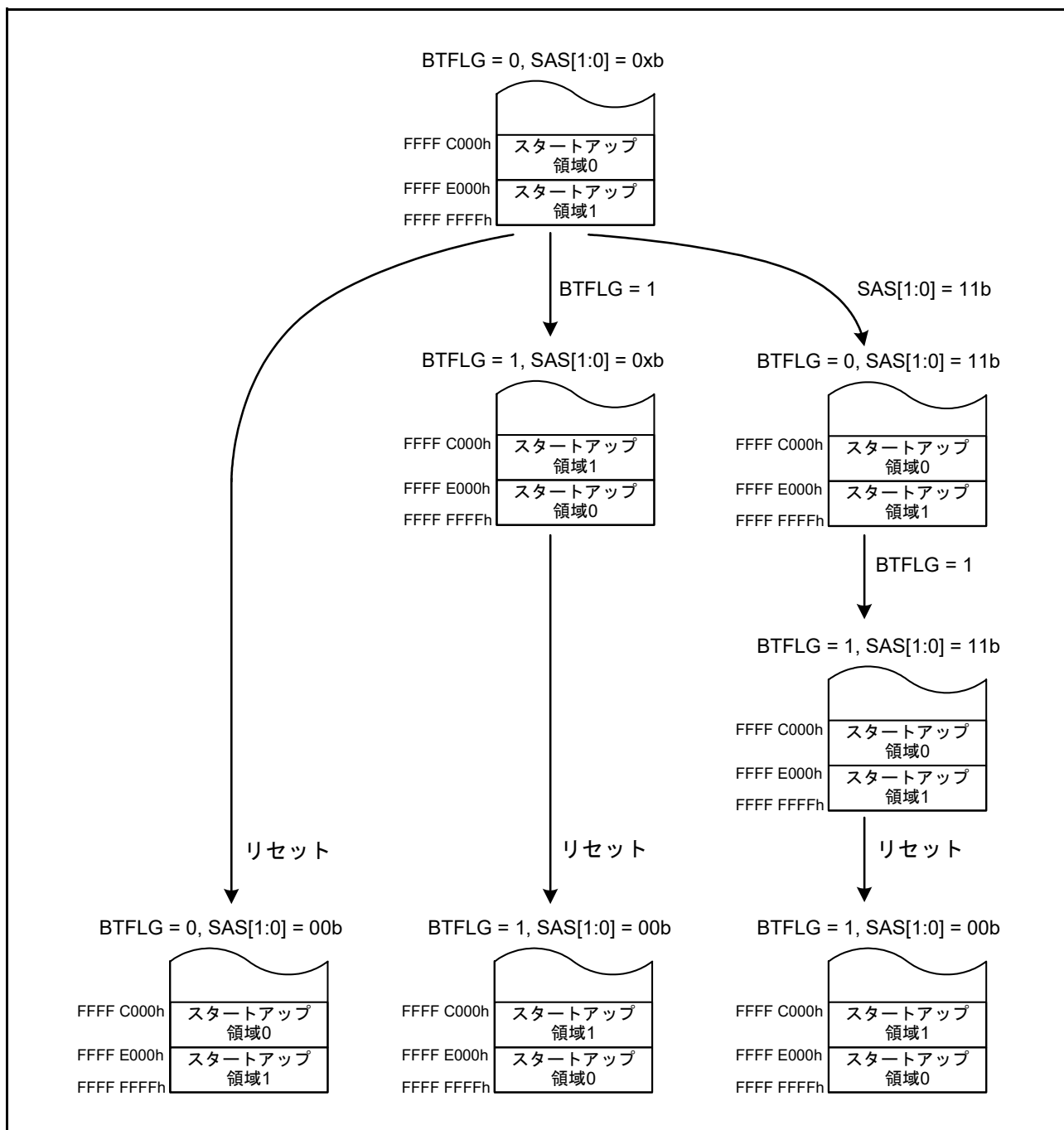
図 60.28 スタートアッププログラム保護機能の設定遷移例 2
