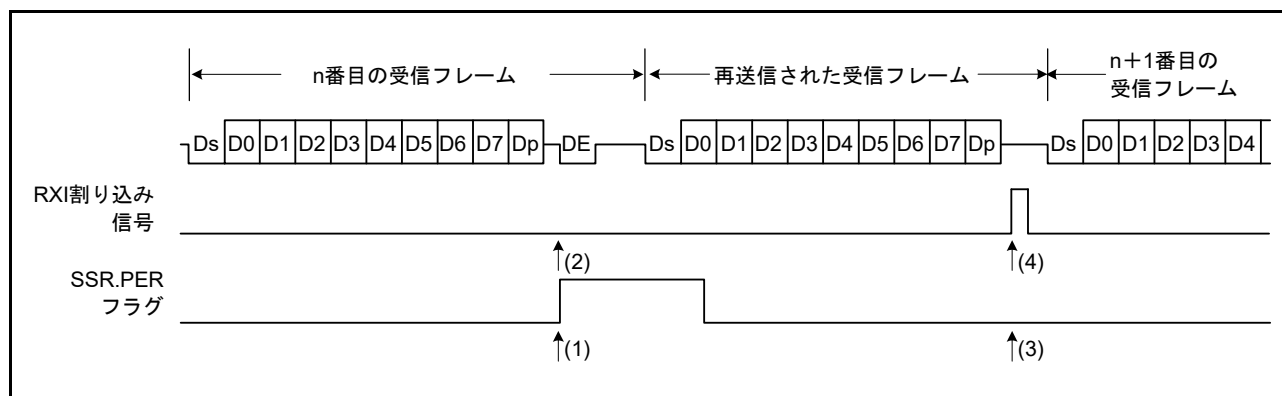
図 40.47 SCI 受信モードの場合の再送信動作 (受信時の再送信動作)
