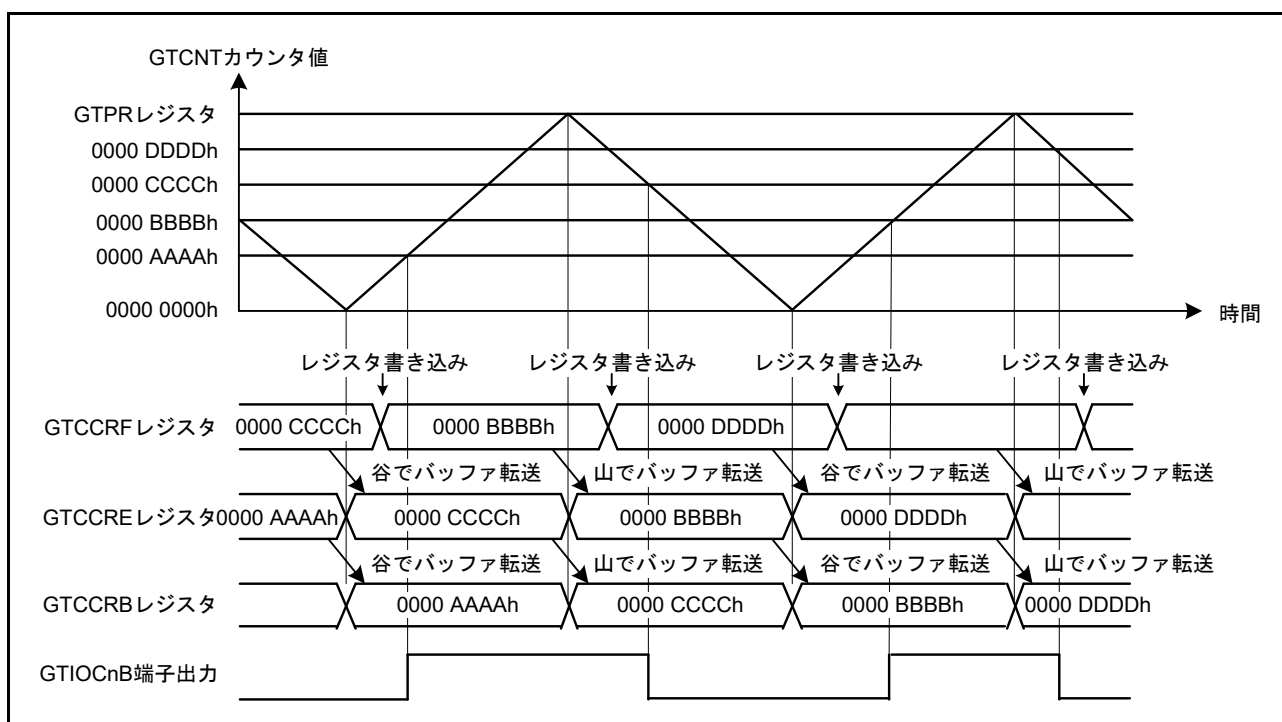
図 26.28 GTCCRA, GTCCRB レジスタのダブルバッファ動作例 ( アウトプットコンペア、三角波、谷 / 山両方でバッファ転送、GTCCRB レジスタコンペアマッチでトグル出力、周期の終わりで出力保持の場合 ) (n = 0 ~ 3)
