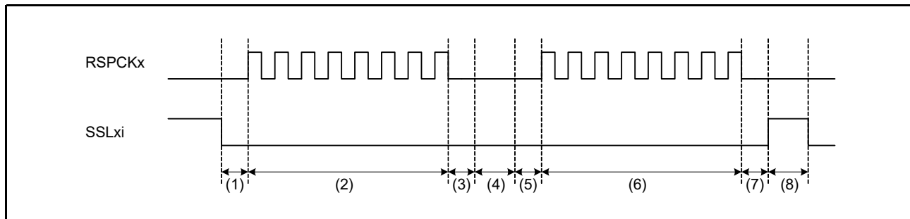
図 43.36 SSLKP ビットを利用したバースト転送動作の例 (CPHA = 1, CPOL = 0)
