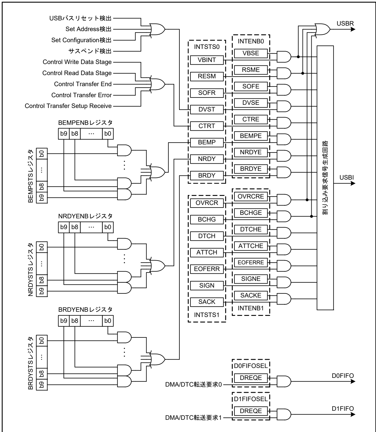
図 39.10 USB 割り込みの関連図
