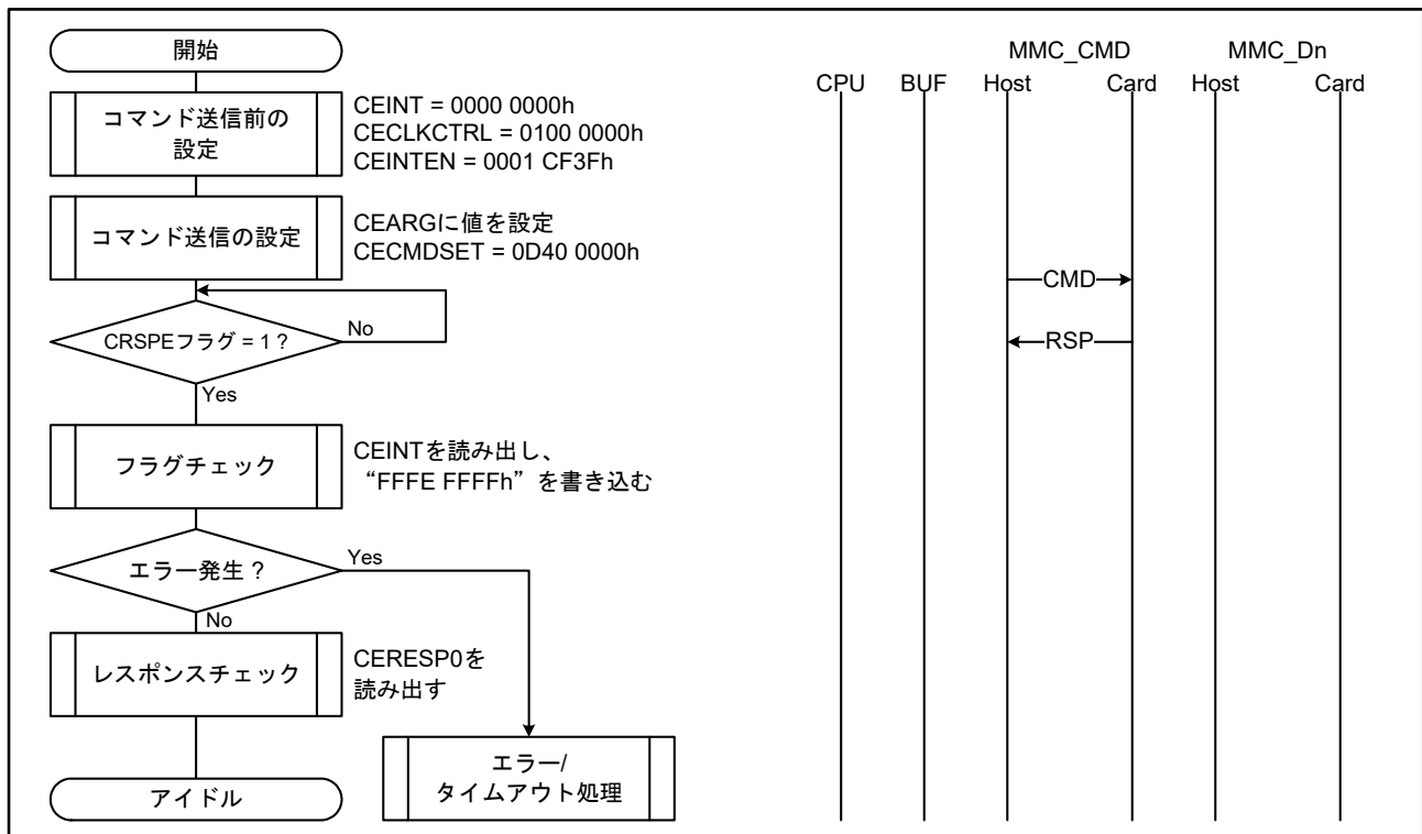
図 48.12 データ転送を行わないコマンドの送信例 (CMD13)
