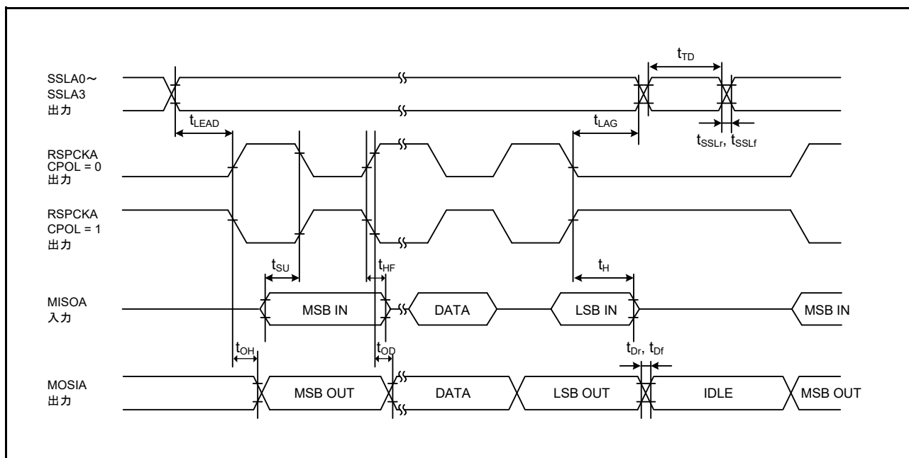
図 61.67 RSPi タイミング (マスタ、CPHA = 1) (ビットレート : PCLKA を 2 分周に設定)
