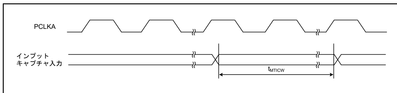
図 61.40 MTU インプットキャプチャ入力タイミング
