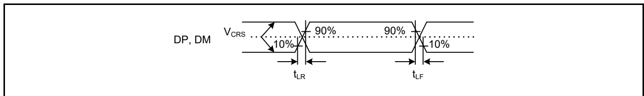
図 61.98 DP, DM 出力タイミング (ロースピード時)
