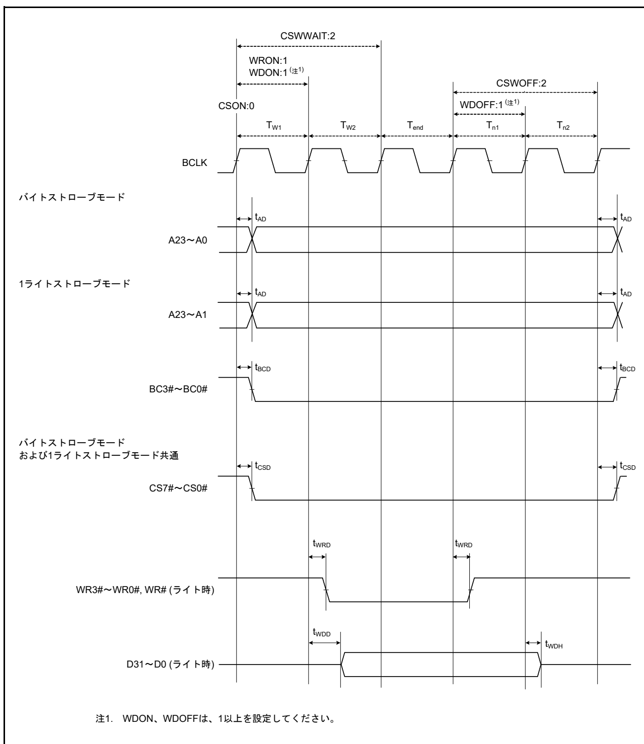
図 61.21 外部バスタイミング / ノーマルライトサイクル (バスクロック同期)
