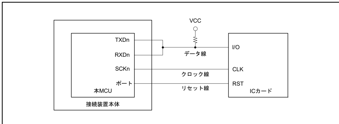
図 40.37 スマートカード (IC カード) との接続例
