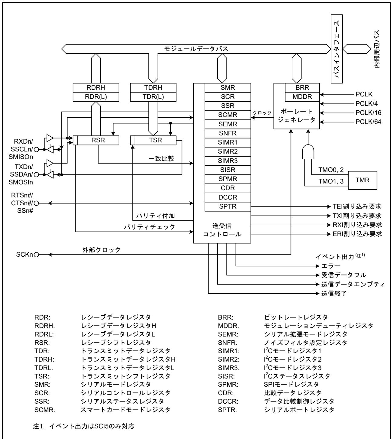
図 40.2 SCIj (SCI5, SCI6) のブロック図
