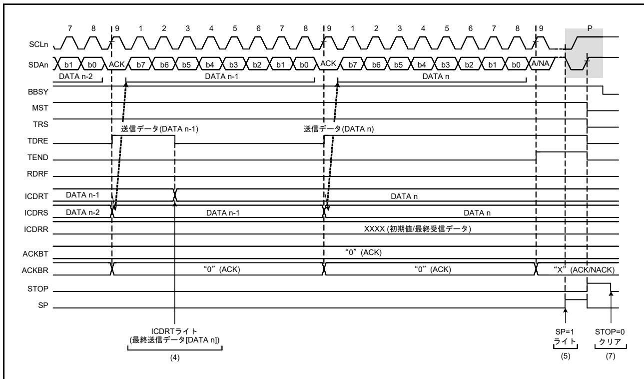
図 41.8 マスタ送信の動作タイミング (3)
