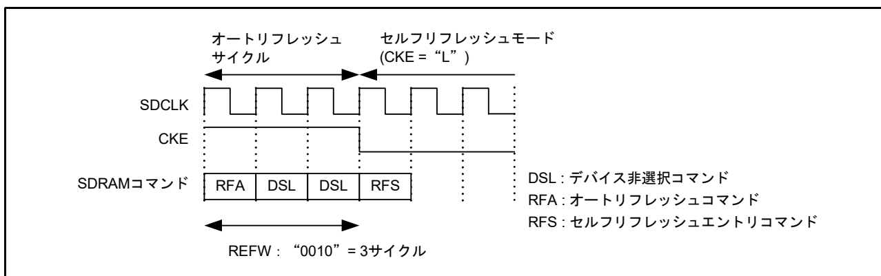
図 16.51 セルフリフレッシュモード移行タイミング例 (SDRFCR.REFW[3:0] ビット = "0010b" : 3 サイクルの場合)
