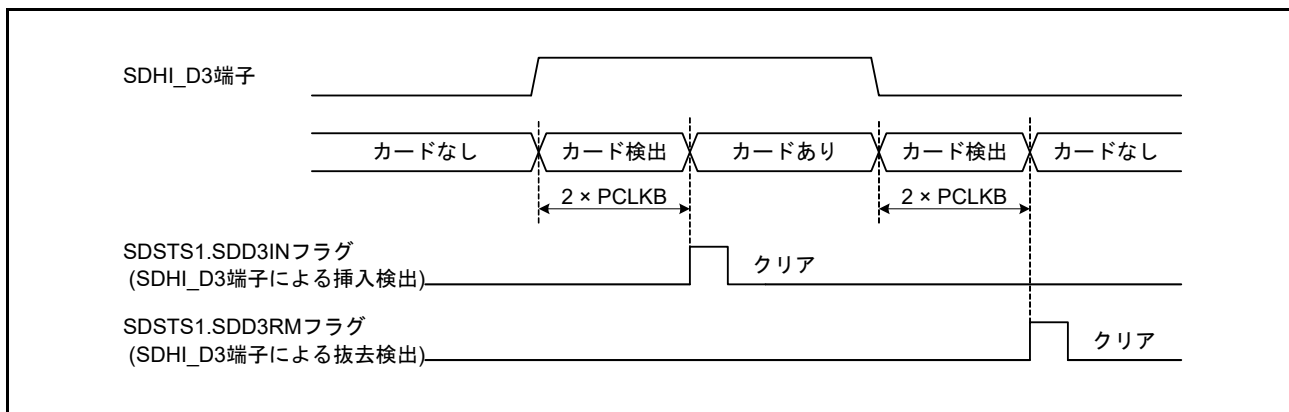
図 47.7 SDHI_D3 端子による SD カード検出
