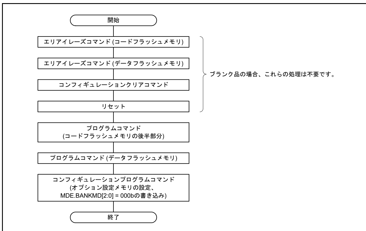
図 60.51 リニアモードのままフラッシュメモリを書き換える例
