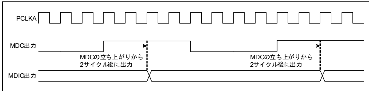
図 38.9 PCLKA の 2 サイクル遅延時のホールド時間調整タイミング
