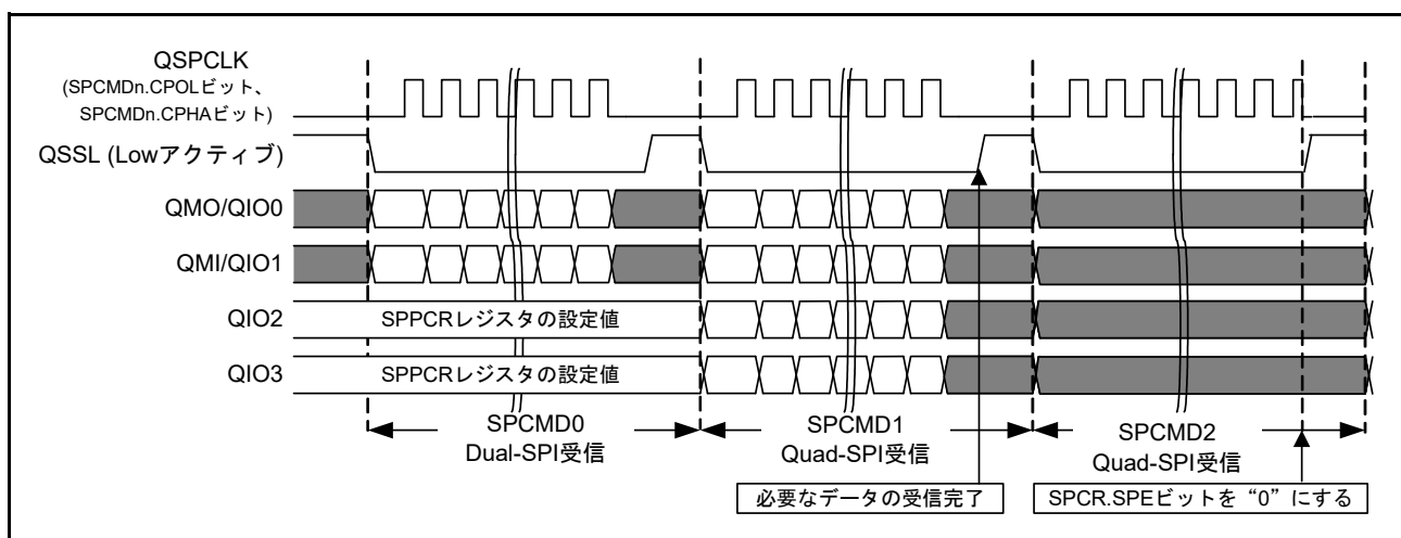
図 44.19 転送モードを切り替えたシーケンス構成の例 (n = 0 ~ 3) (シーケンスを構成するコマンドがすべて Dual/Quad-SPI リード動作である場合の終了方法 (a))
