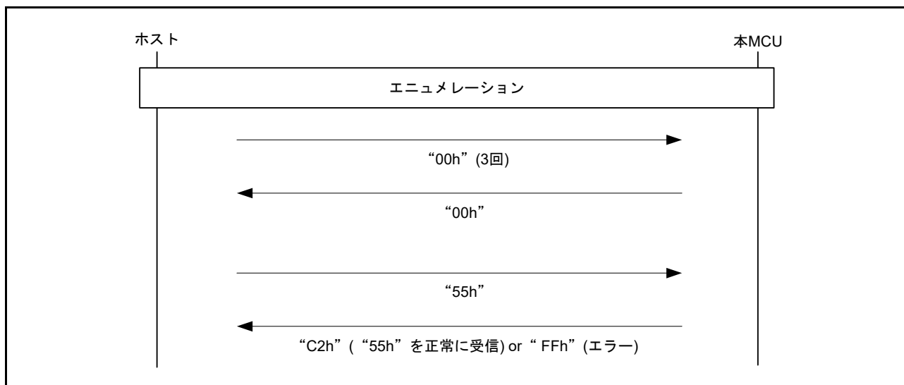
図 60.40 ホストと本 MCU 間の初期通信
