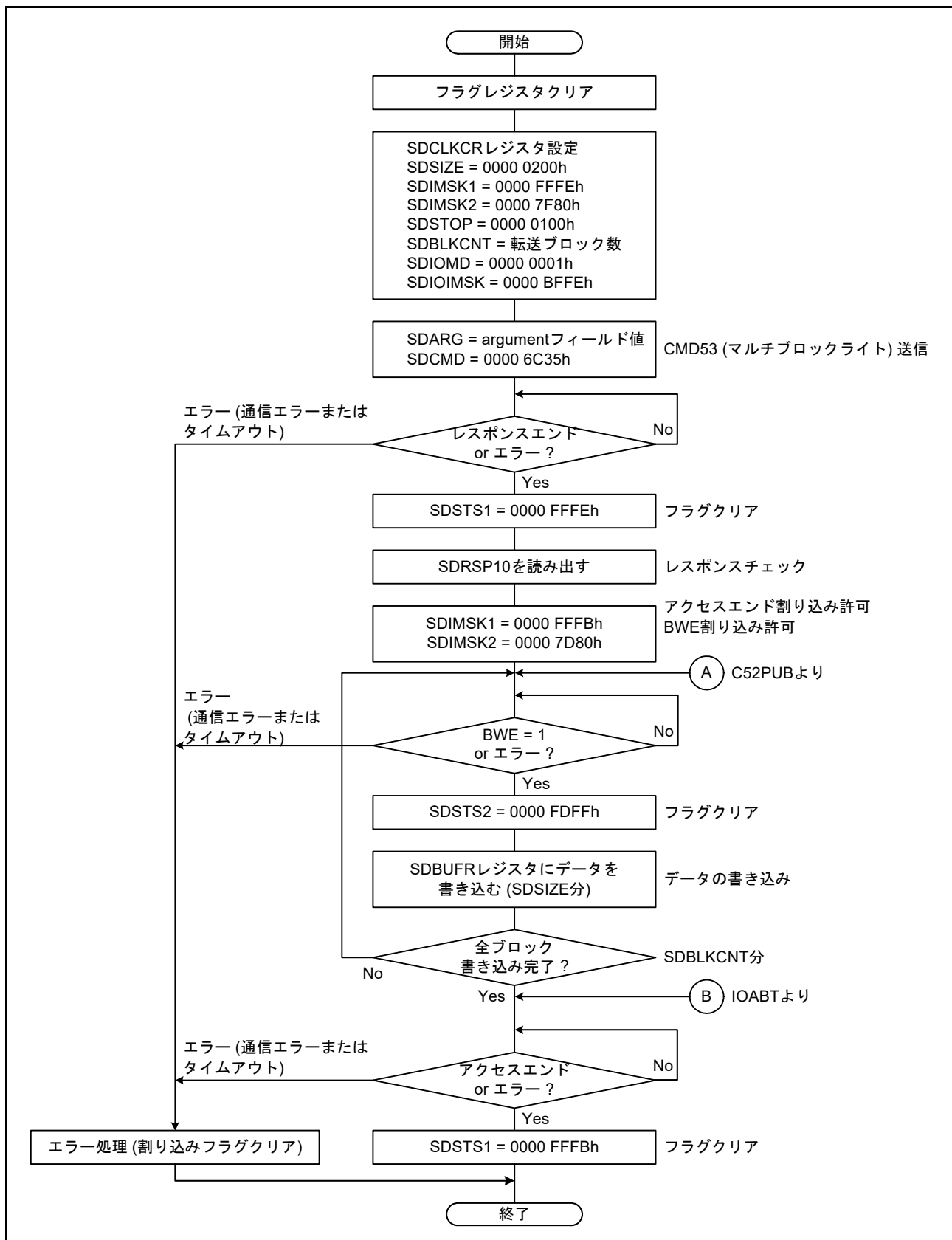
図 47.18 IO_RW_EXTENDED コマンド (CMD53/ マルチブロックライト) の送信例
