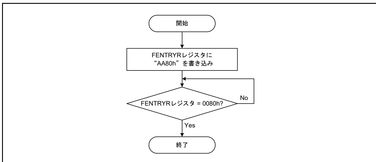
図 60.10 データフラッシュメモリ P/E モード移行フロー
