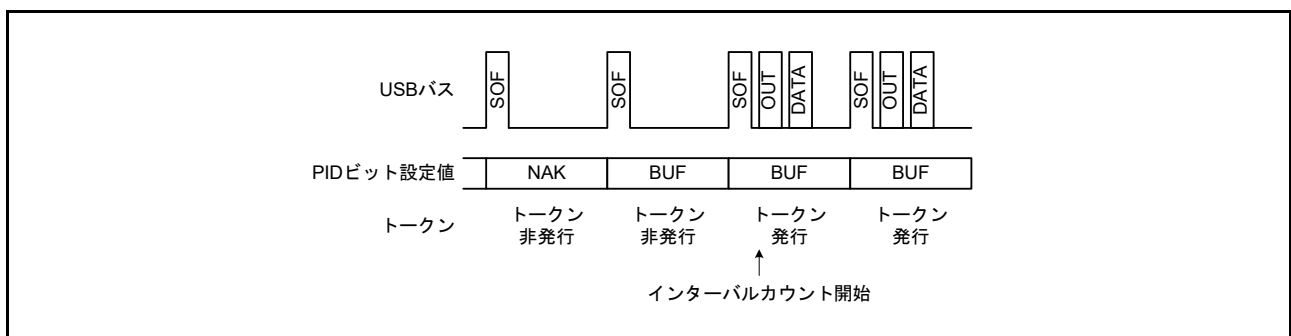
図 39.16 IITV[2:0] = 000b の場合のトークン発行有無
