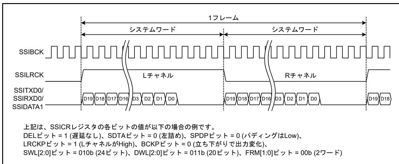
図 46.10 左詰めフォーマットの例
