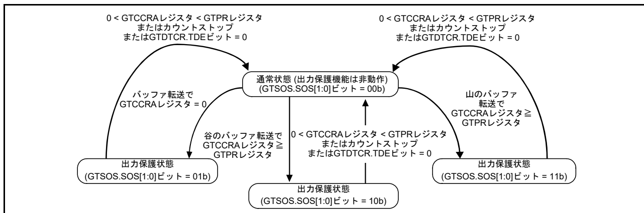
図 26.126 出力保護機能
