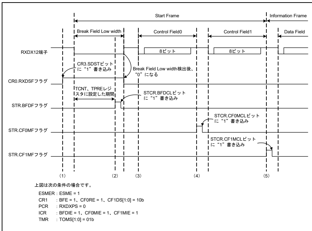
図 40.68 Start Frame 受信時の動作例
