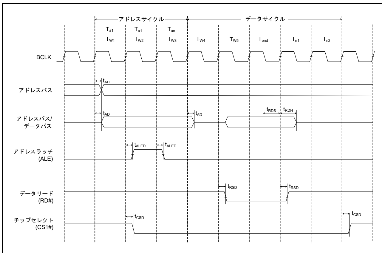
図 61.18 アドレス/データマルチプレクスバスのリードアクセスタイミング
