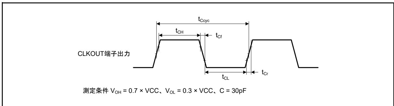
図 61.12 CLKOUT 端子出カタイミング
