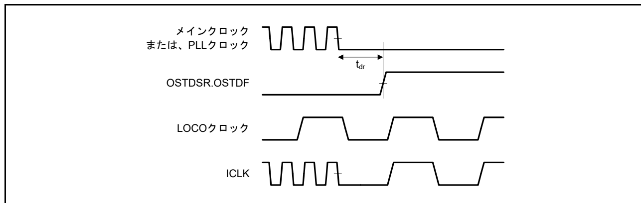
図 61.106 発振停止検出タイミング
