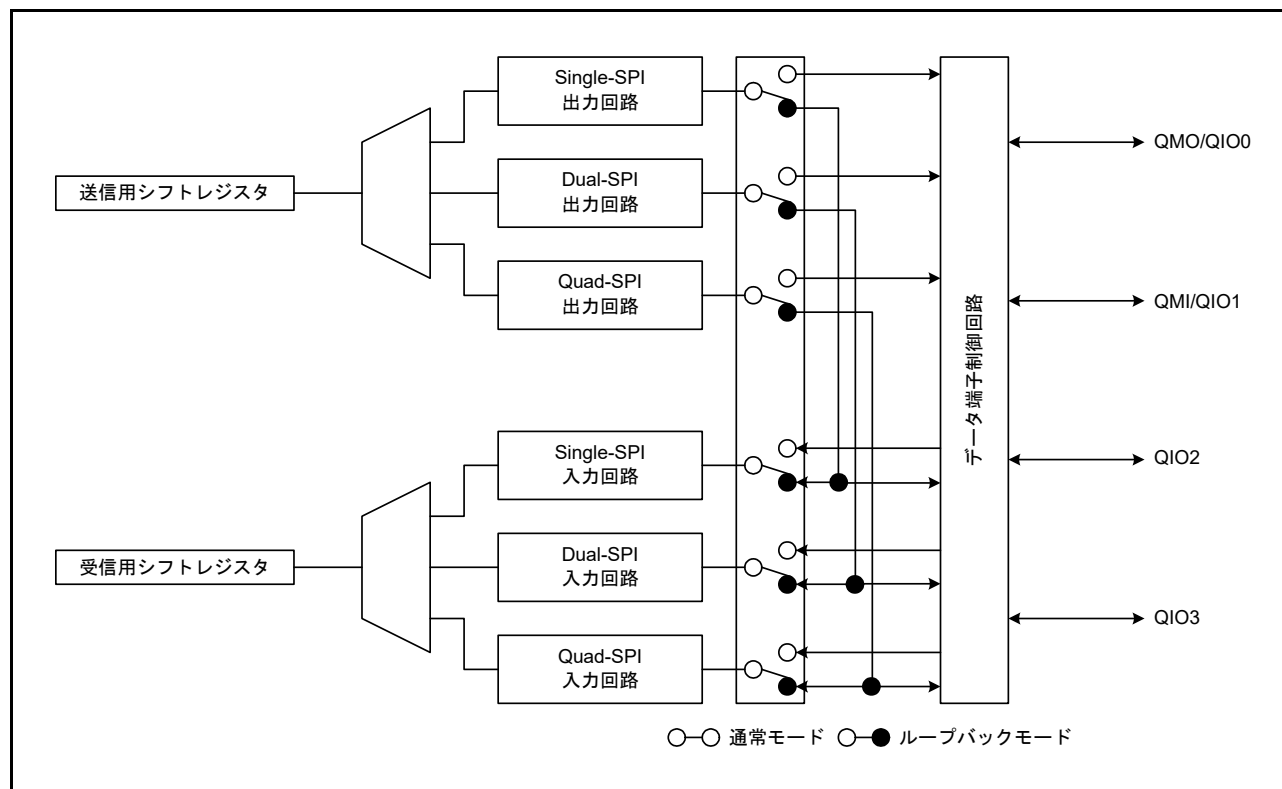
図 44.26 ループバックモードの内部結線概略図
