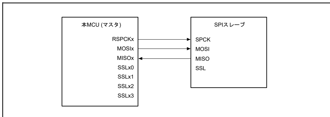
図 43.11 マスタ (クロック同期式動作) / スレーブ (クロック同期式動作) の構成例 (本 MCU = マスタ)
