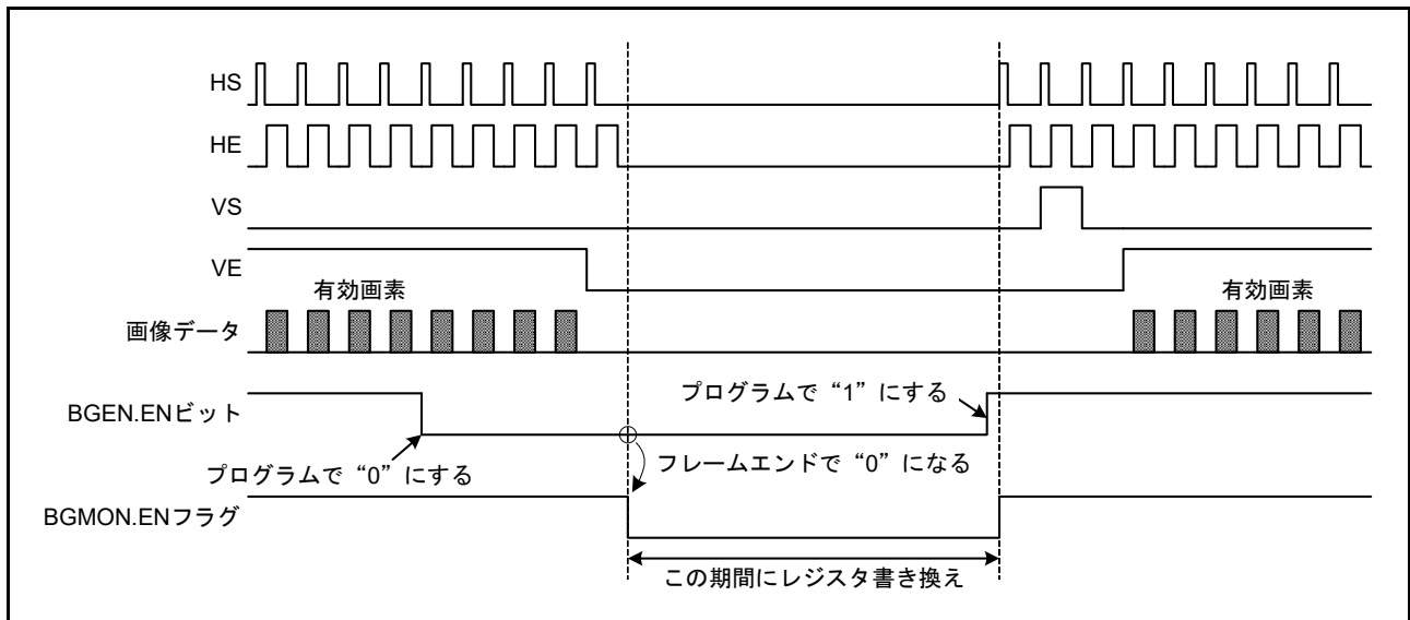
図 50.23 正常動作時の停止と再開
