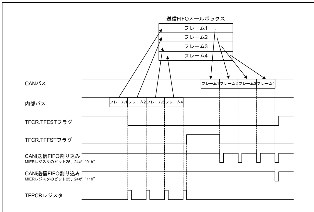
図 42.3 送信 FIFO メールボックスの動作 (MIER レジスタのビット 25、24 が "01b" または "11b")
