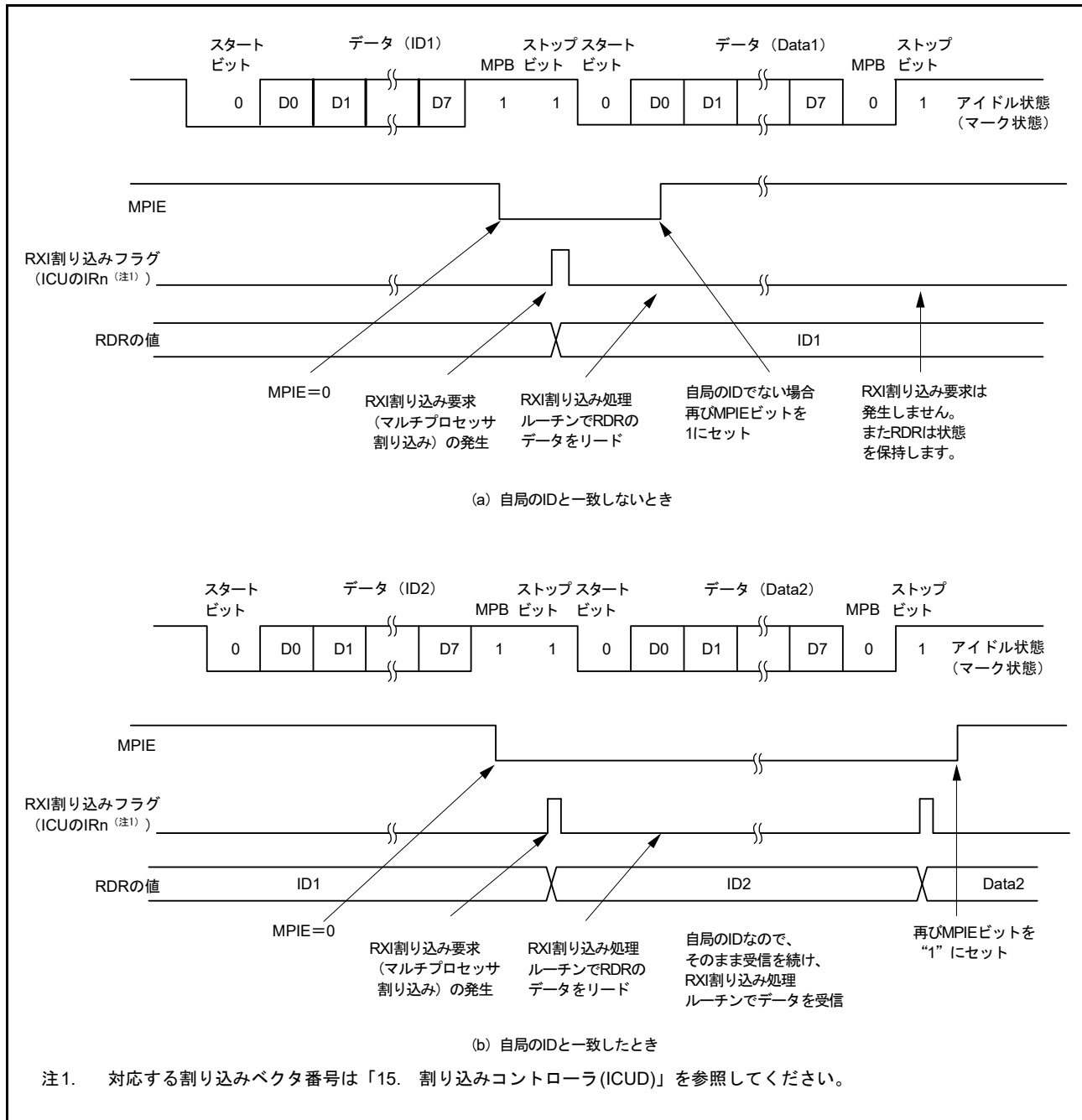
図 40.24 SCI の受信時の動作例 (8 ビットデータ / マルチプロセッサビットあり / 1 ストップビットの例)
