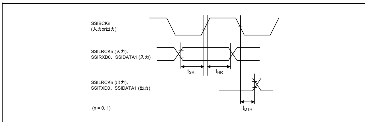
図 61.75 SSICR.BCKP = 0 の場合の SSIE データ送受信タイミング
