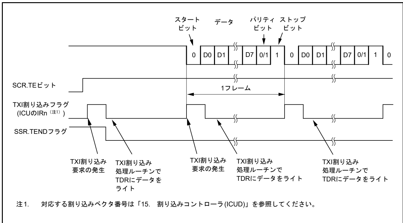
図 40.14 調歩同期式モードのシリアル送信の動作例 (1) (8ビットデータ / パリティあり / 1ストップビット / CTS 機能使用しない / 送信開始時)
