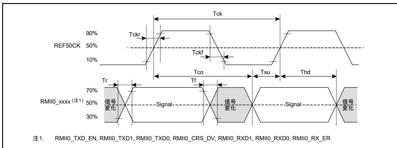
図 61.81 REF50CK と RMII 信号とのタイミング
