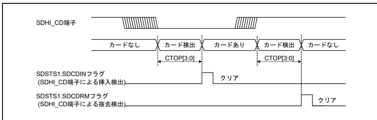
図47.6 SDHI_CD端子によるカード検出例
