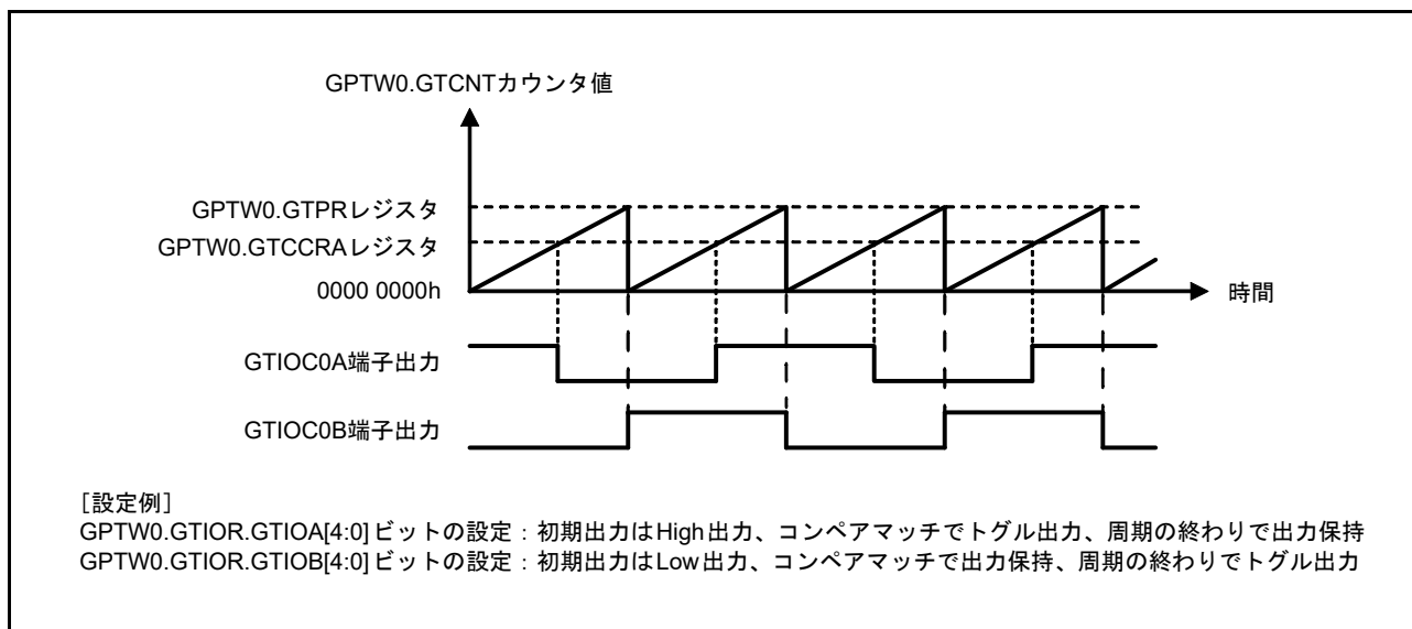
図 26.15 トグル出力動作例 (2)
