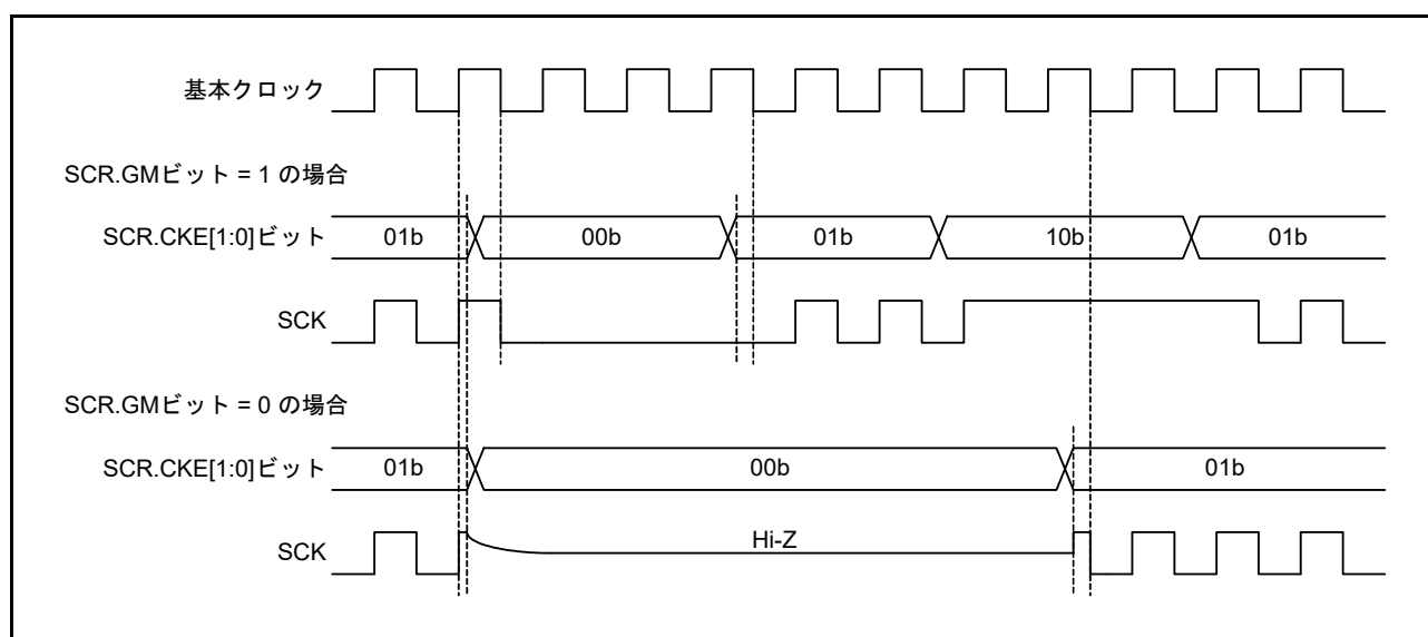
図 40.49 クロック出力制御
