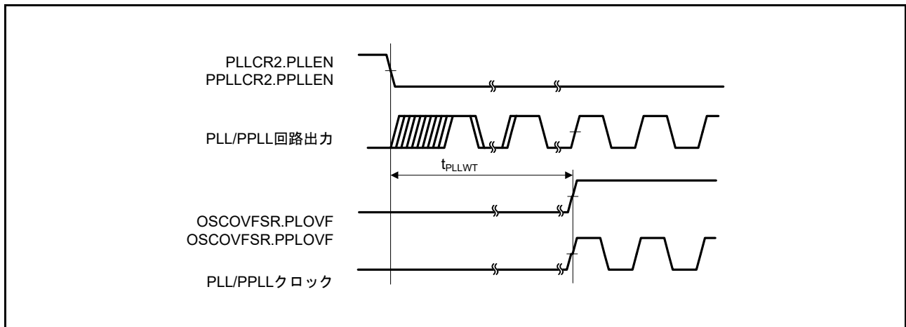
図 61.10 PLL/PPLL クロック発振開始タイミング
