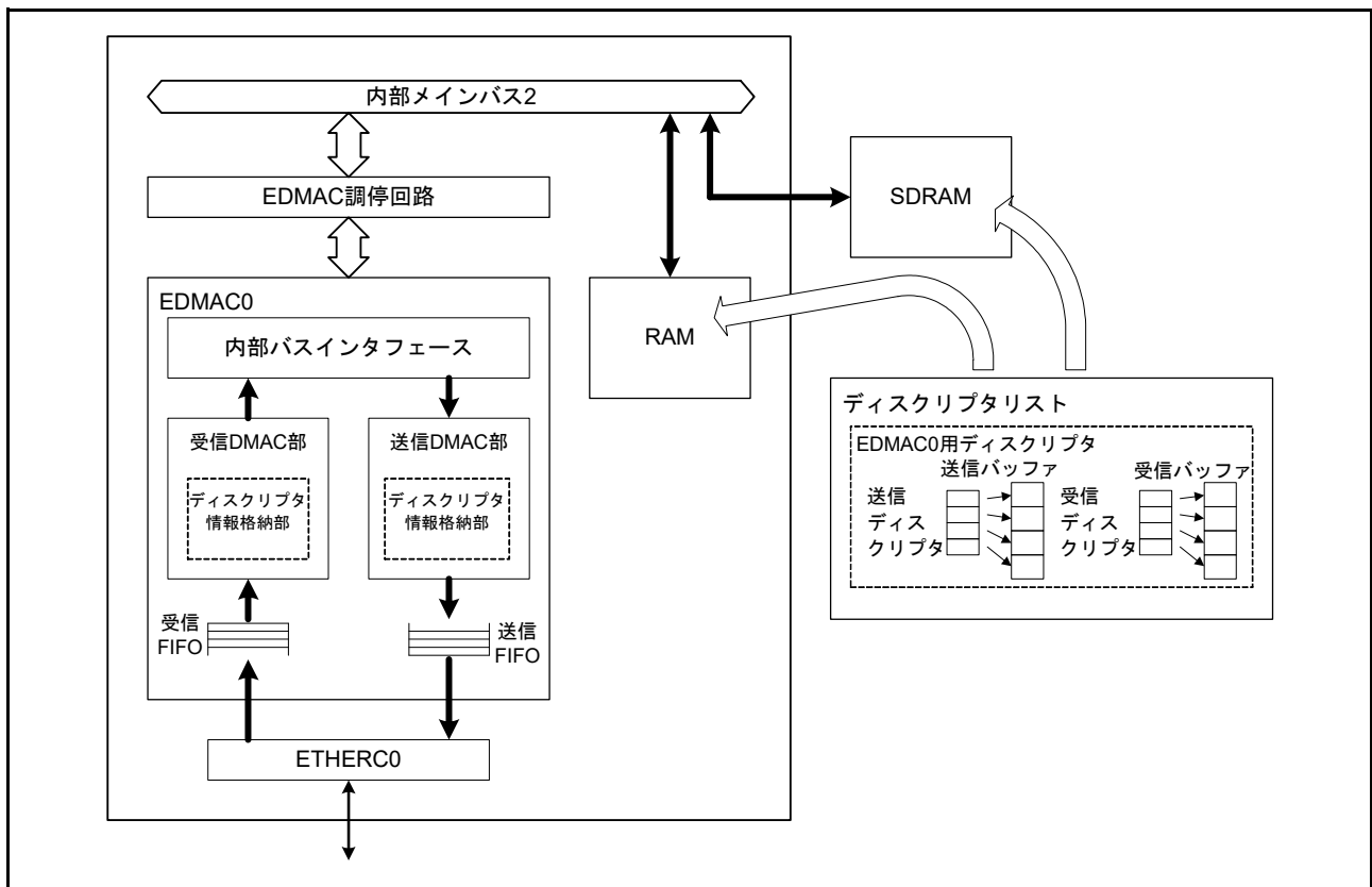
図 37.2 EDMAC とメモリ上のディスクリプタおよび送受信バッファの構成
