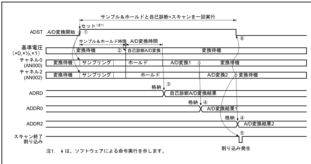
図 54.10 シングルスキャンモードの動作例 (チャンネル専用サンプル & ホールド回路使用チャンネル AN000, AN002 選択 + 自己診断、常時サンプリング無効)
