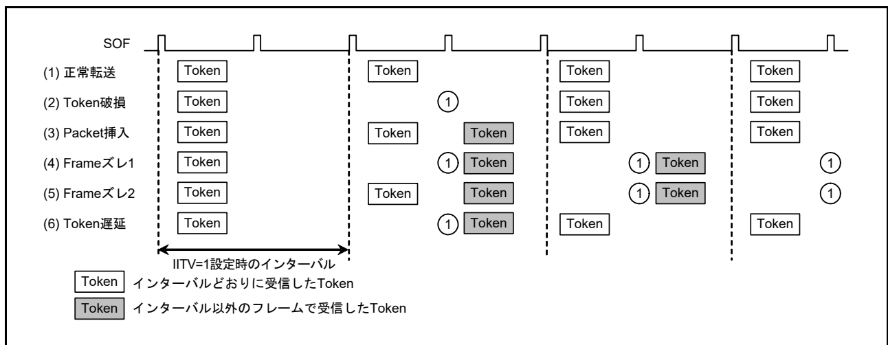
図 39.22 IITV[2:0] = 001b のときのインターバルエラー発生例
