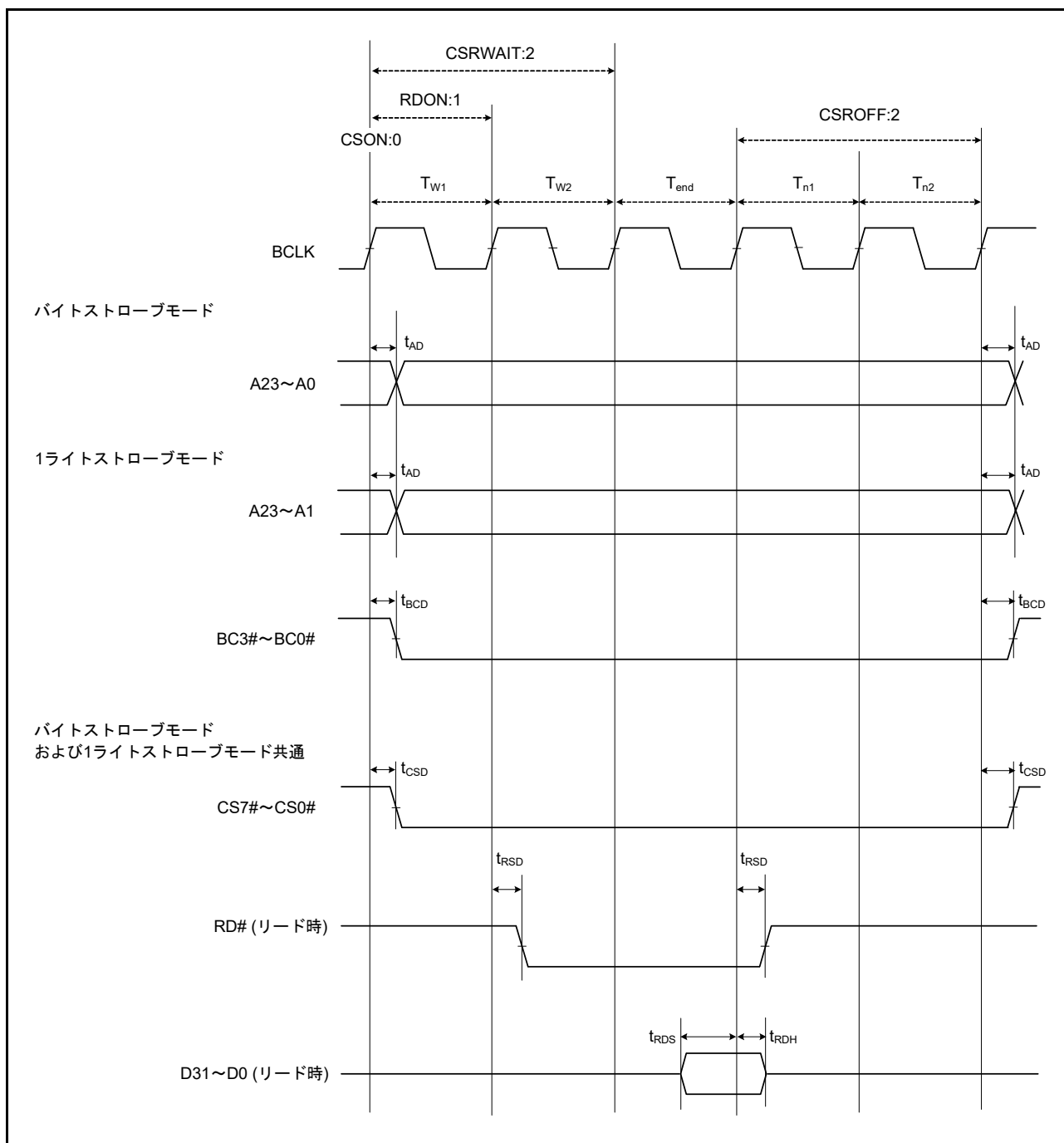
図 61.20 外部バスタイミング / ノーマルリードサイクル (バスクロック同期)
