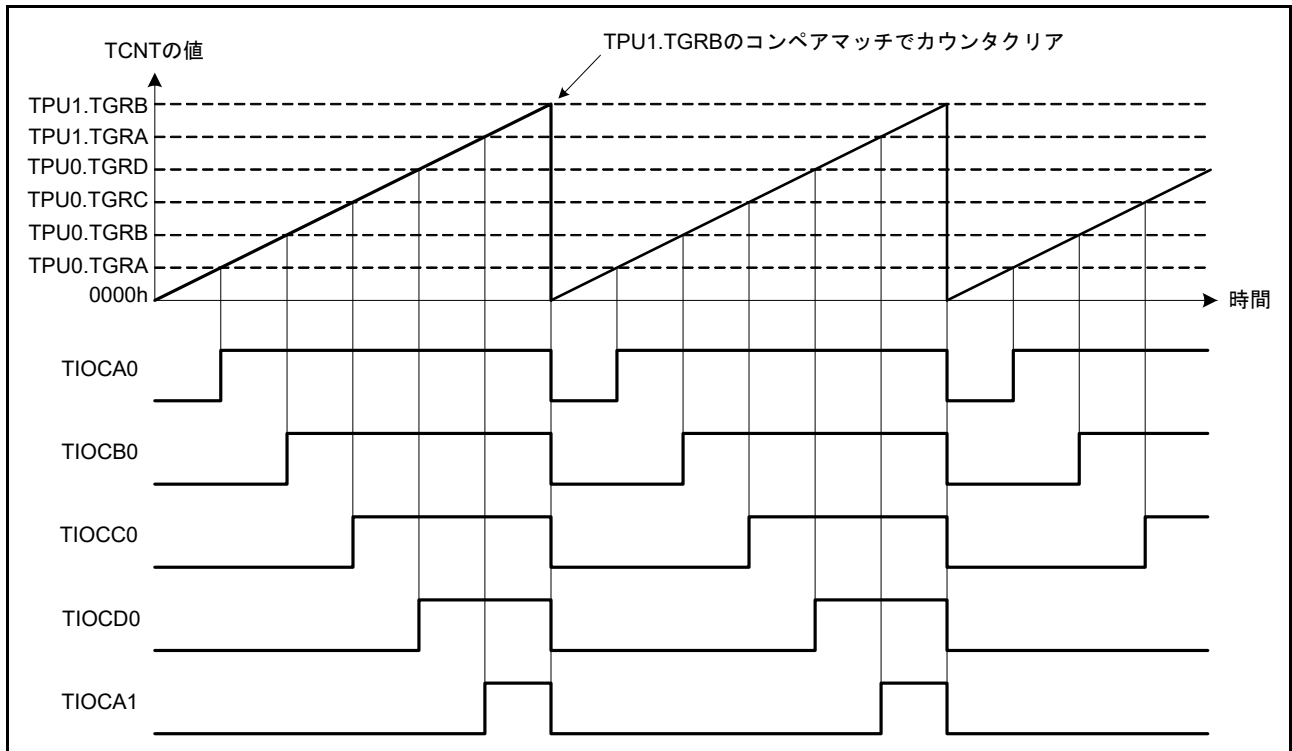
図 28.22 PWM モードの動作例 (2)
