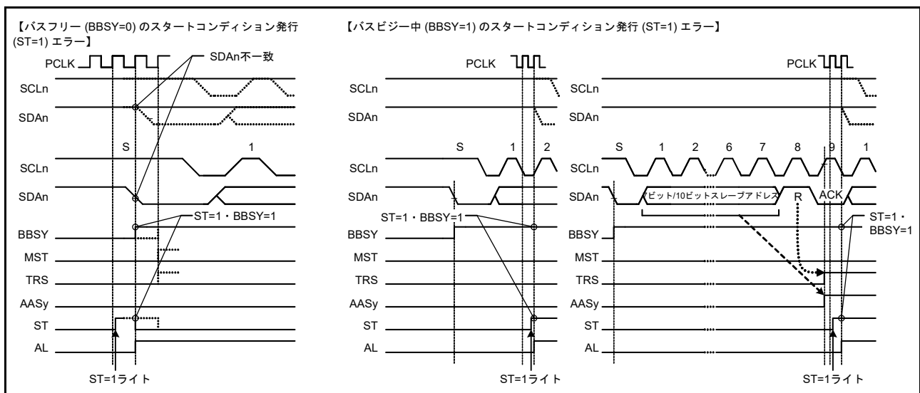
図 41.33 スタートコンディション発行時のアービトレーションロスト (MALE ビット = 1 のとき)
