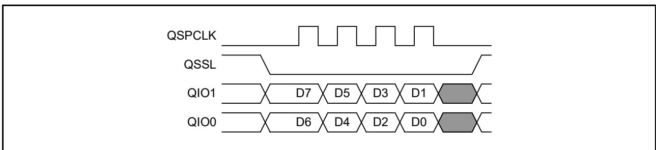
図 44.4 Dual-SPI モード転送フォーマット
