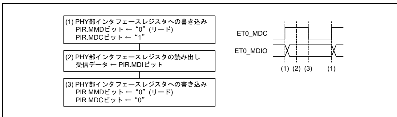
図 36.16 1 ビットデータのリードフロー
