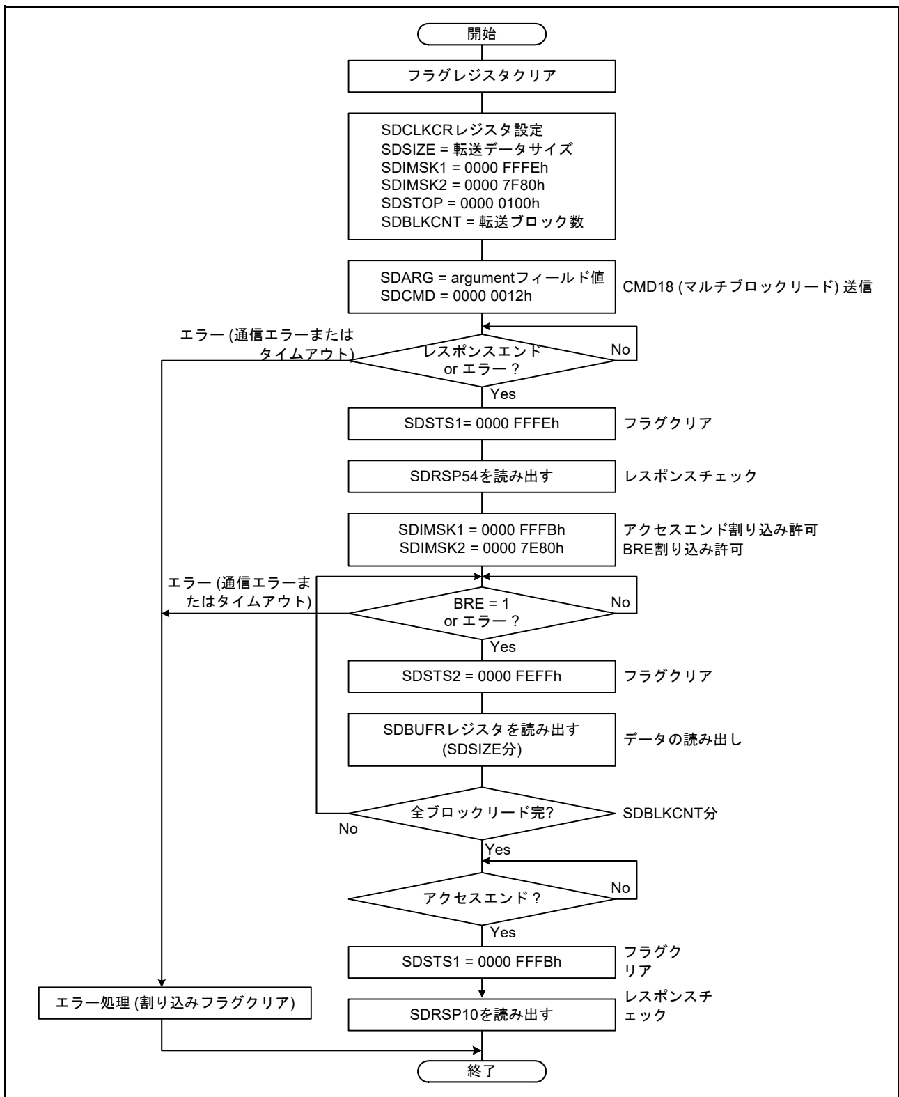
図 47.12 マルチブロックリードコマンドの送信例
