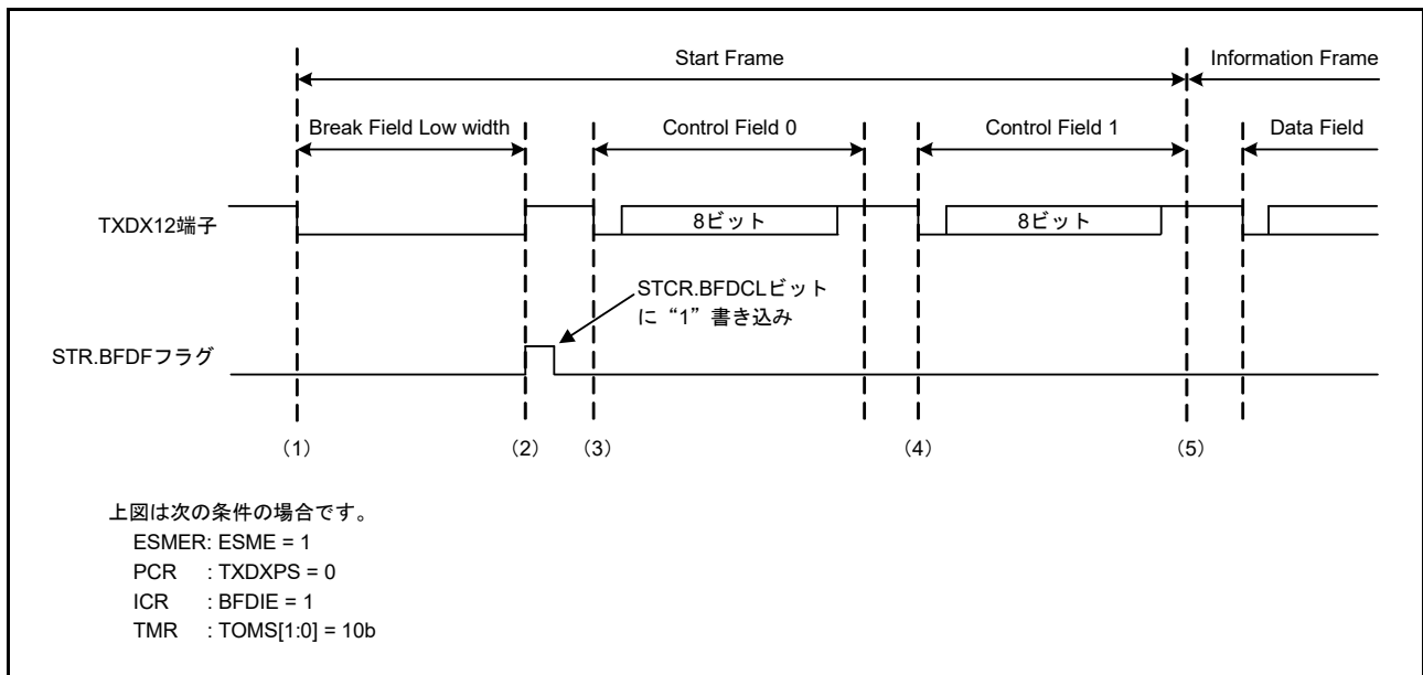
図 40.65 Start Frame 送信時の動作例
