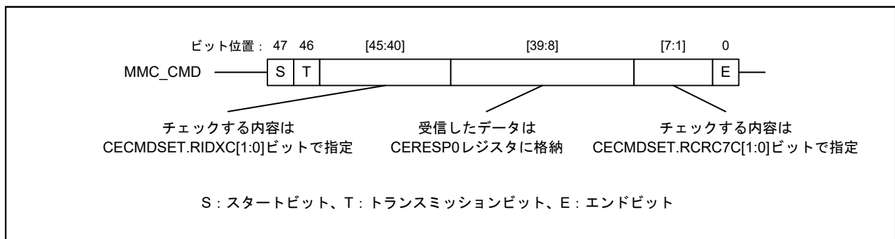
図 48.3 6 バイトのレスポンス (R2 レスポンス以外) のフォーマット
