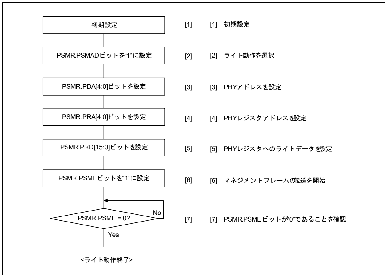
図 38.7 PHY レジスタライトのフローチャート例
