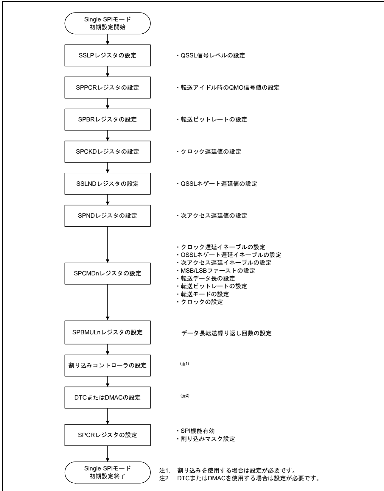
図 44.15 Single-SPIモードの初期設定フロー例 (n = 0 ~ 3)
