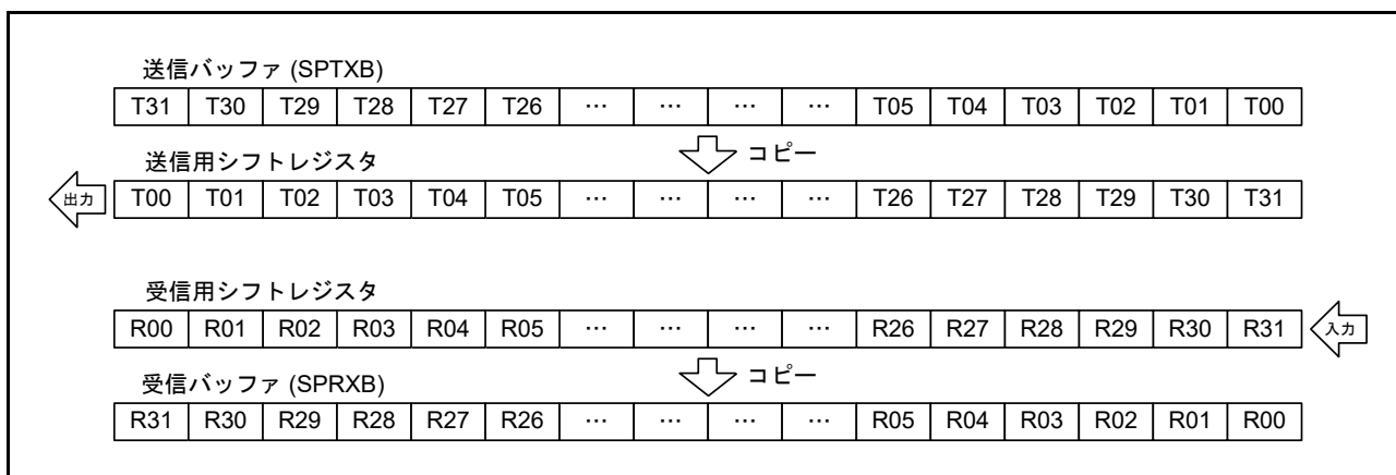
図 44.9 LSB ファースト転送 (32 ビットデータ)
