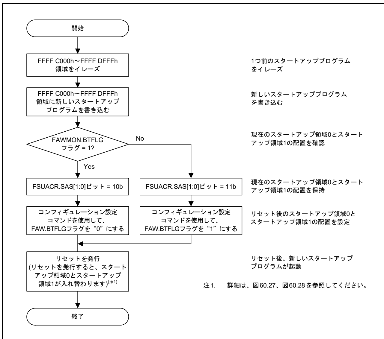
図 60.29 スタートアップ領域選択フロー例
