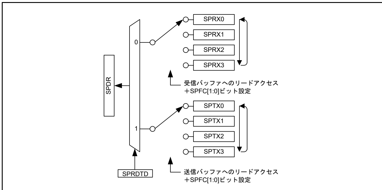
図 43.4 SPDR レジスタの構成図 (リード時)
