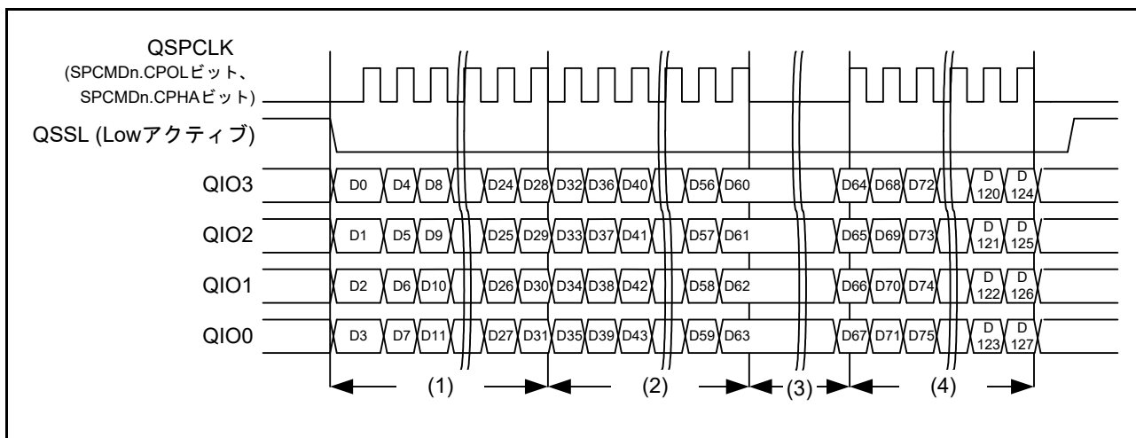
図 44.21 転送データ長を 128 ビットに設定したバースト転送の例 (Quad-SPI モード) (n = 0 ~ 3)
