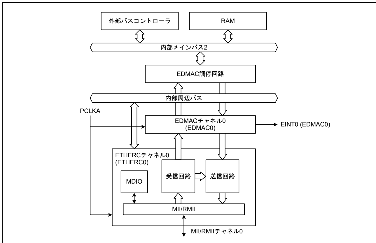
図 36.1 ETHERC の構成
