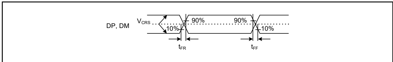
図 61.100 DP, DM 出カタイミング (フルスピード時)
