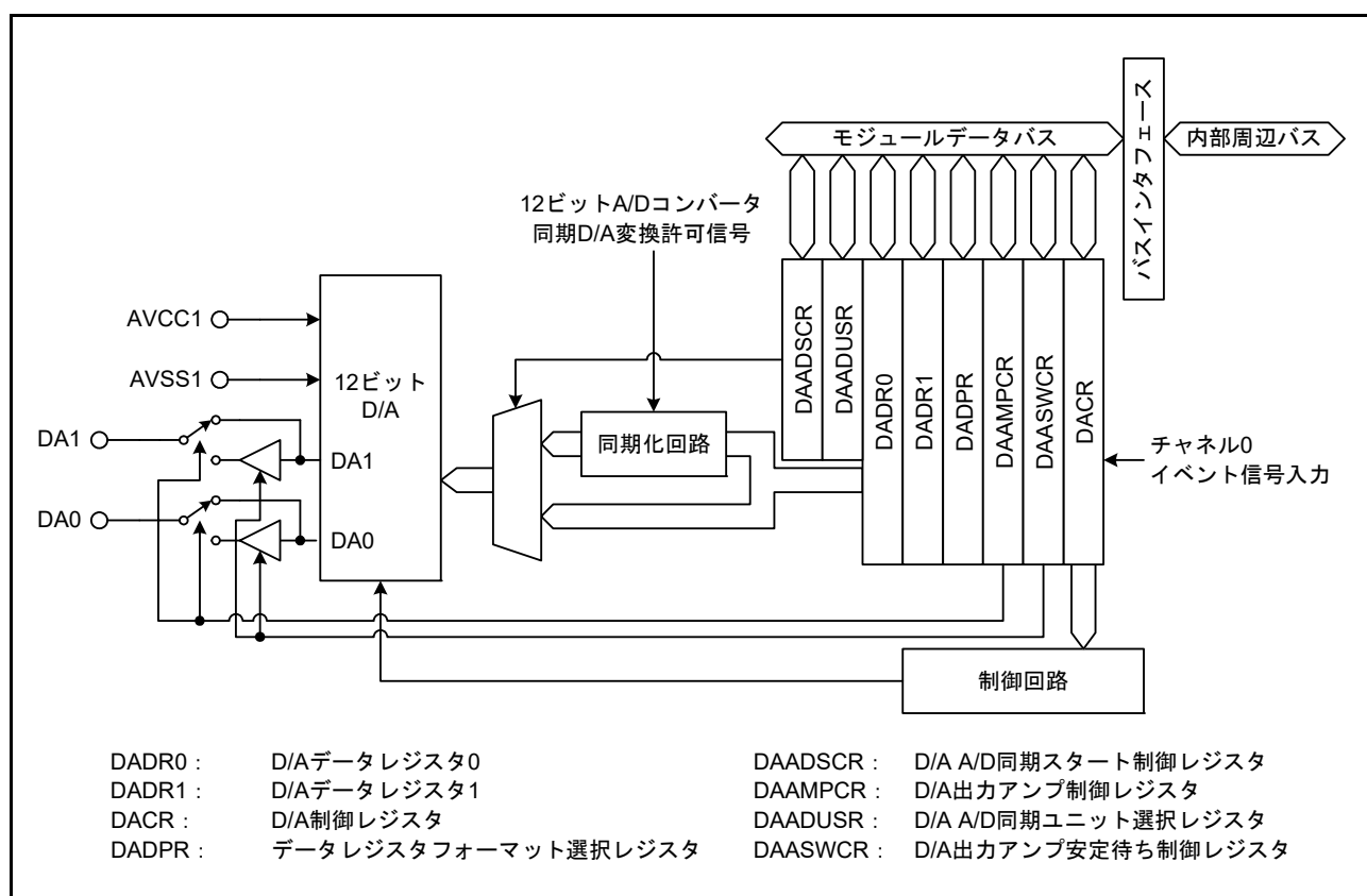
図55.1 12ビットD/Aコンバータのブロック図
