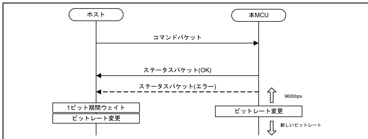
図 60.45 ビットレート設定コマンドの通信シーケンス
