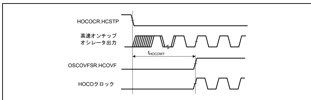
図 61.8 HOCO クロック発振開始タイミング (HOCOCR.HCSTP 設定による発振開始)
