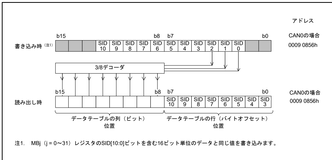
図 42.5 AFSR レジスタの書き込み、読み出し
