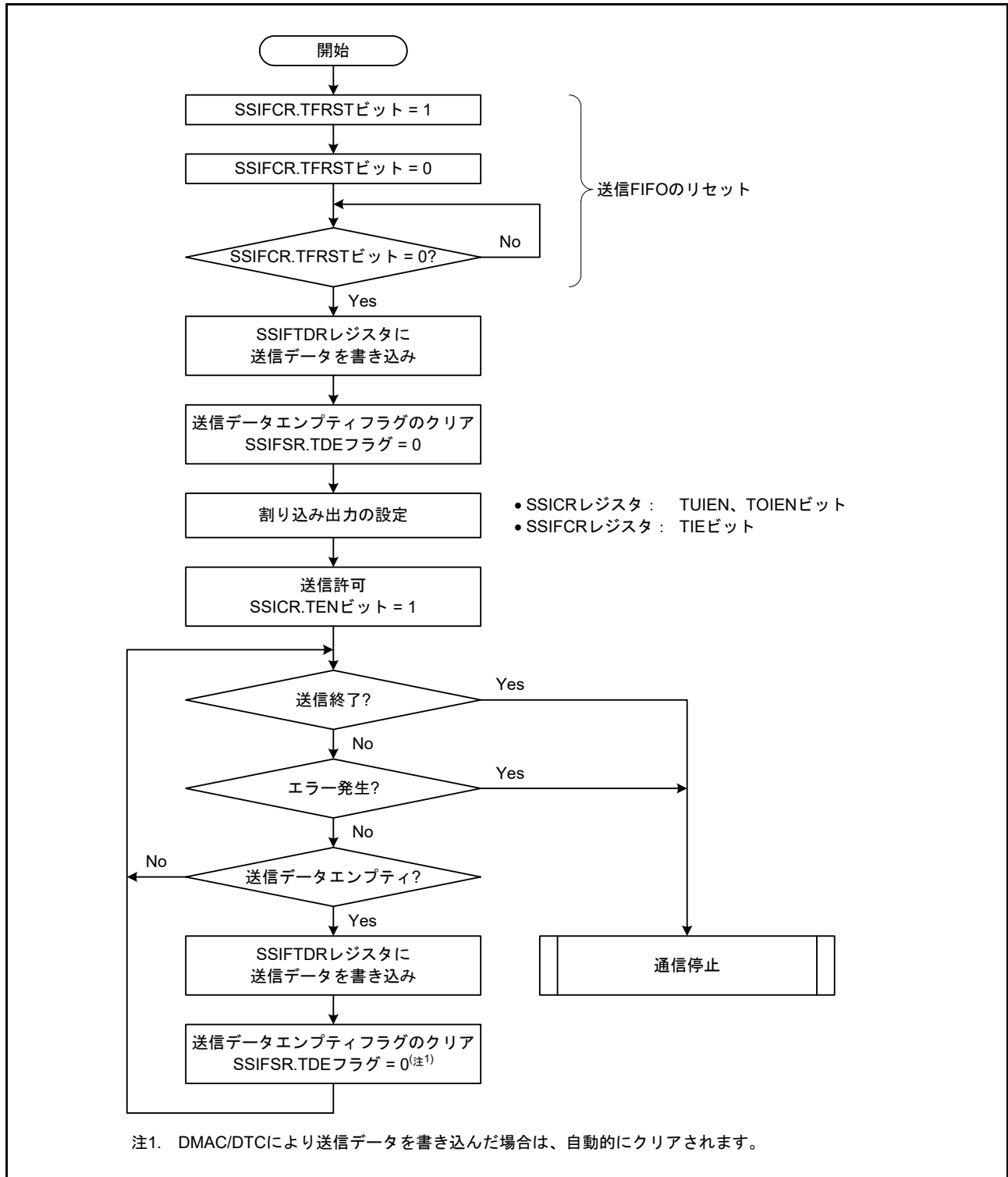
図 46.23 送信フロー例
