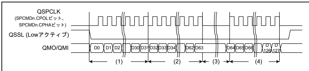
図 44.13 転送データ長を 128 ビットに設定したバースト転送の例 (Single-SPI モード) ( n = 0 \sim 3 )
