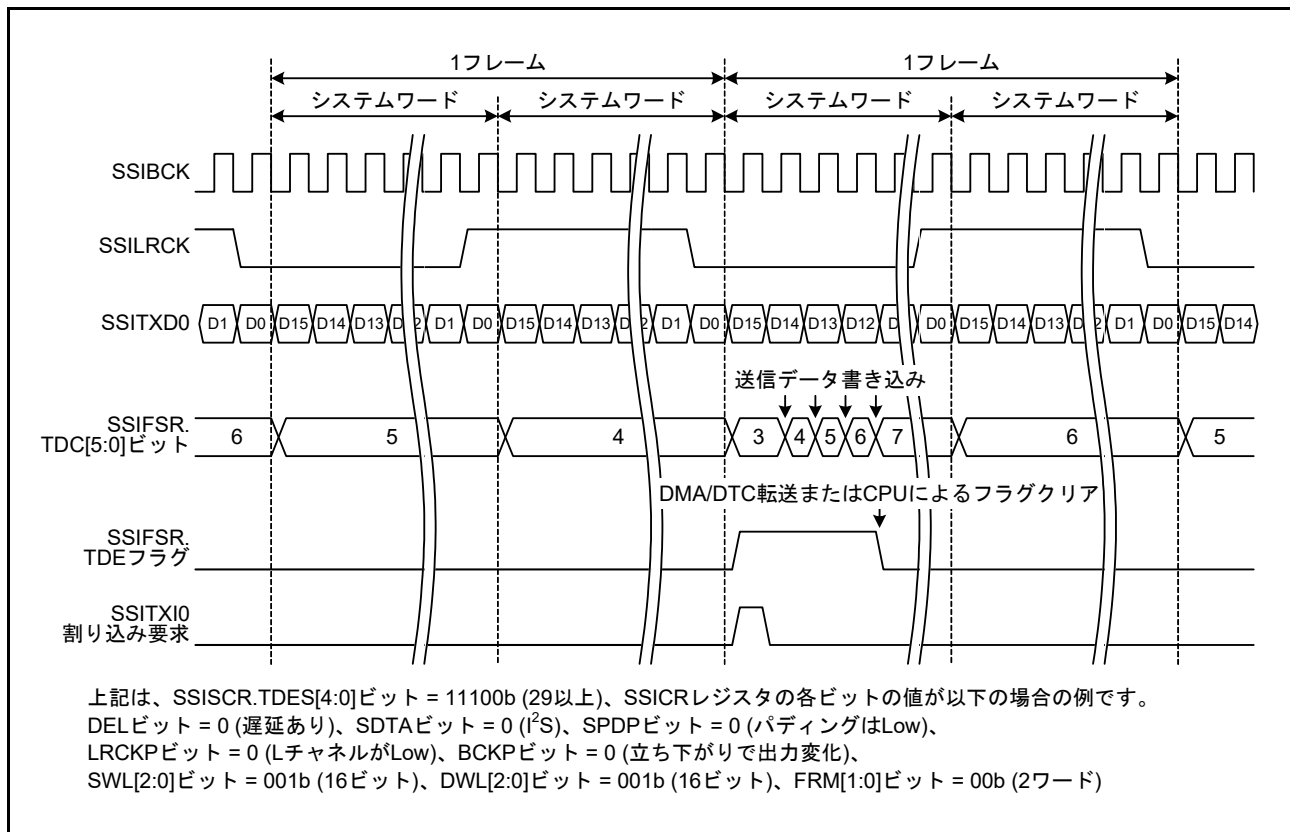
図 46.27 SSITXIO 割り込みのタイミング図
