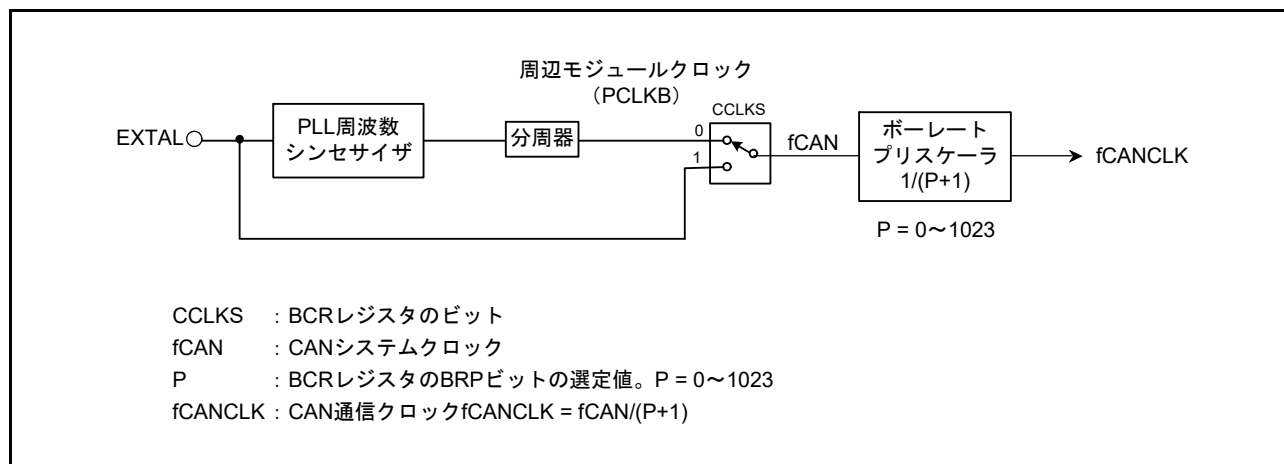
図 42.11 CAN クロック発生回路のブロック図
