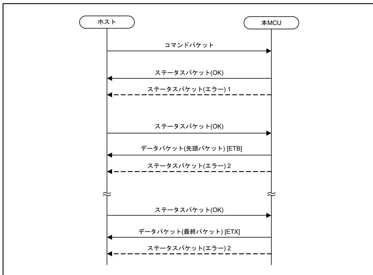
図 60.47 リードコマンドの通信シーケンス
