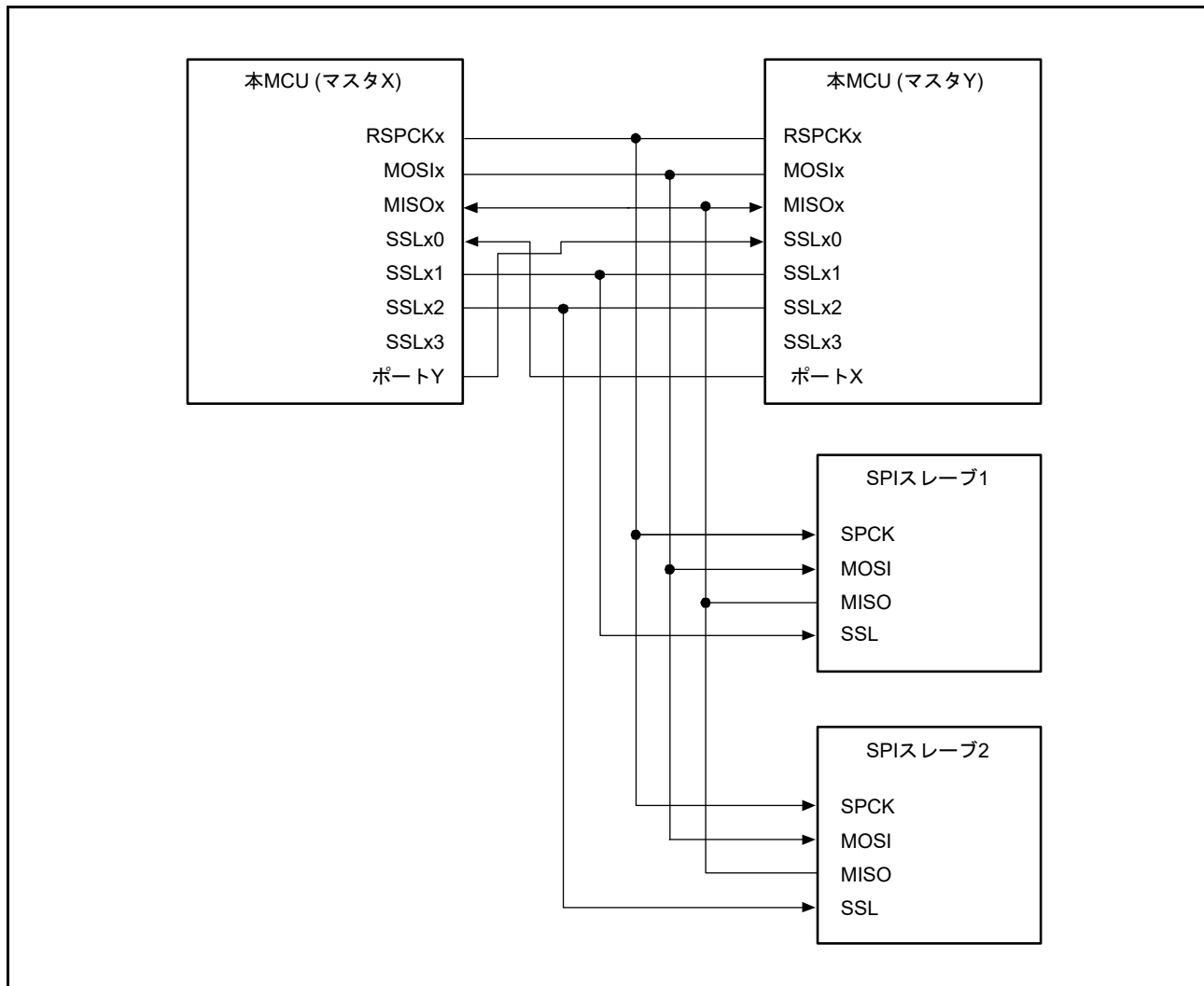
図 43.10 マルチマスタ / マルチスレーブの構成例 (本 MCU = マスタ)
