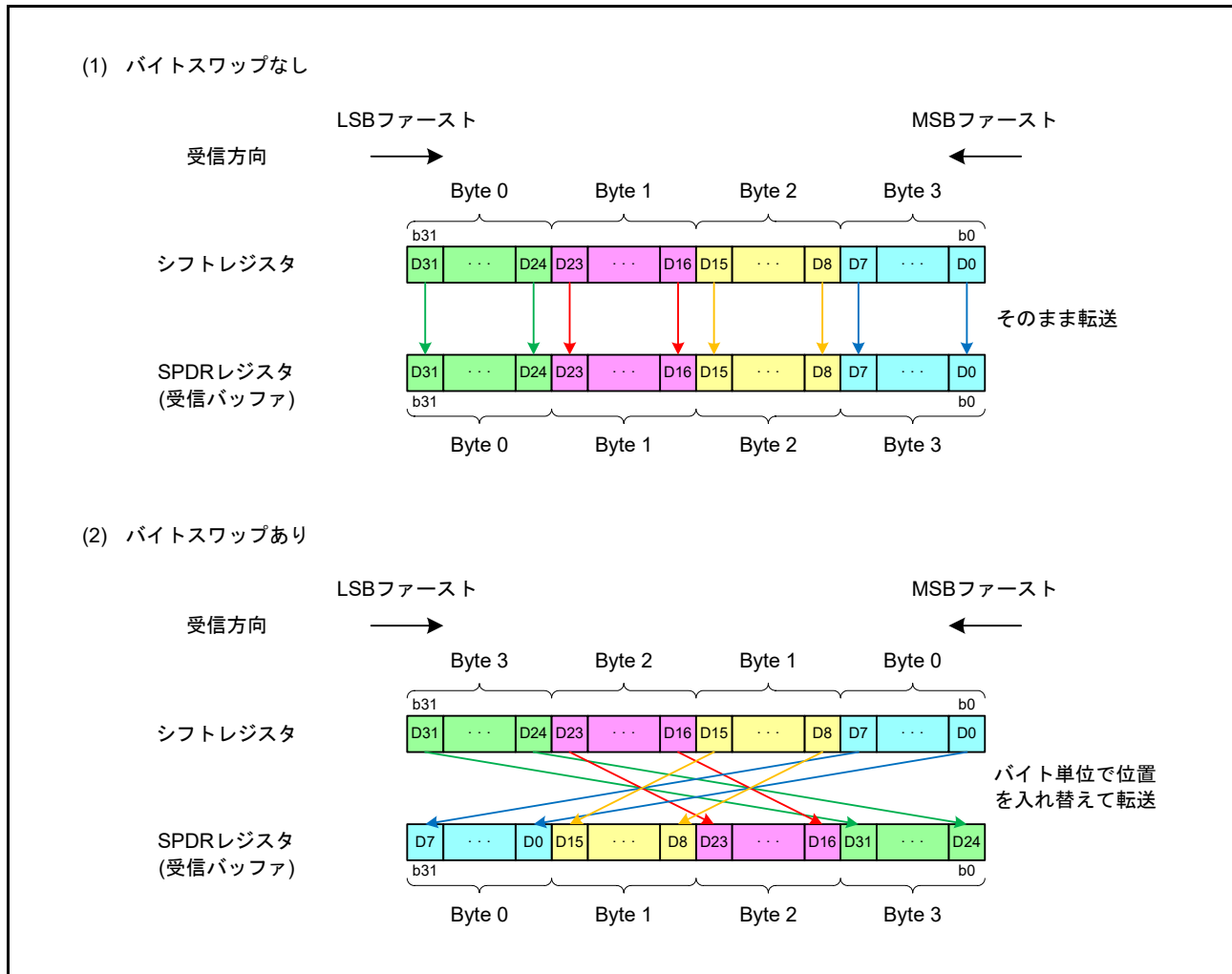
図 43.23 MSB/LSB ファーストとバイトスワップあり/なしの設定と受信データ変換
