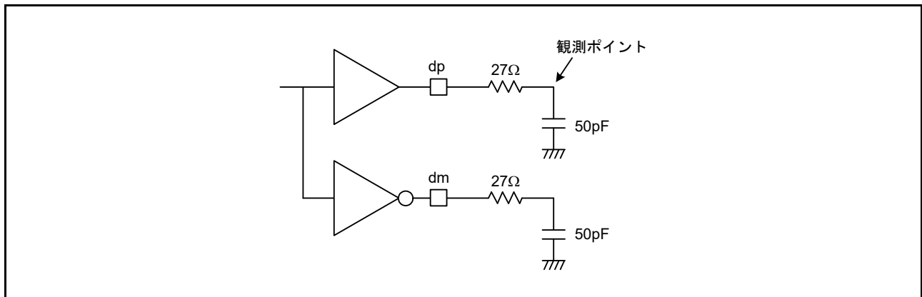
図 61.101 測定回路 (フルスピード時)
