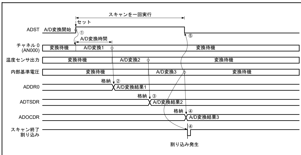
図 54.12 シングルスキャンモードの動作例 (基本動作 : AN000、温度センサ出力、内部基準電圧選択)
