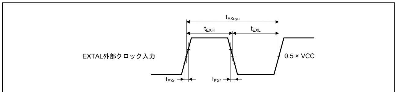
図 61.4 EXTAL 外部クロック入力タイミング
