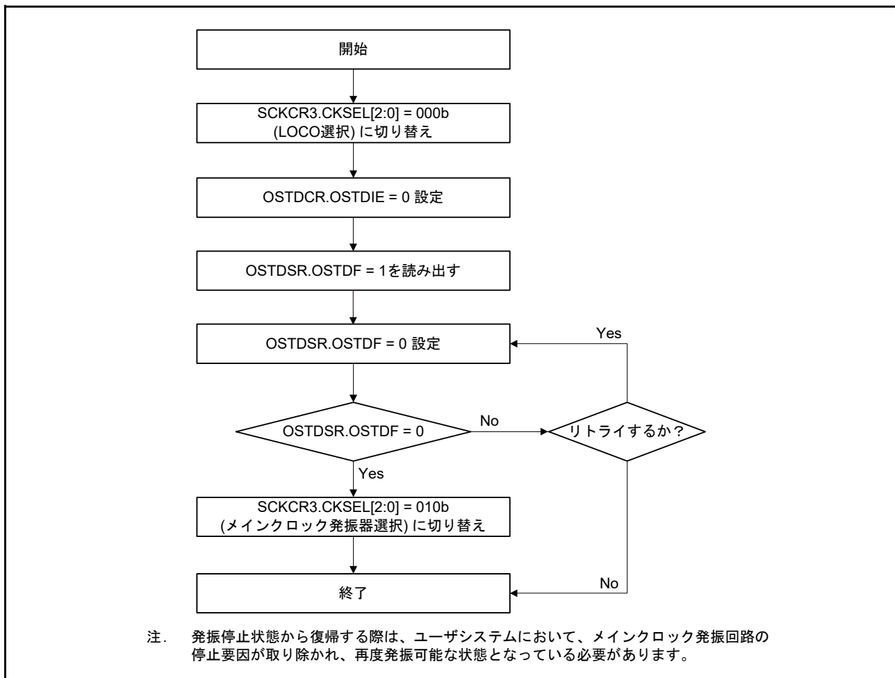
図 9.9 発振停止検出からの復帰のフローチャート例
