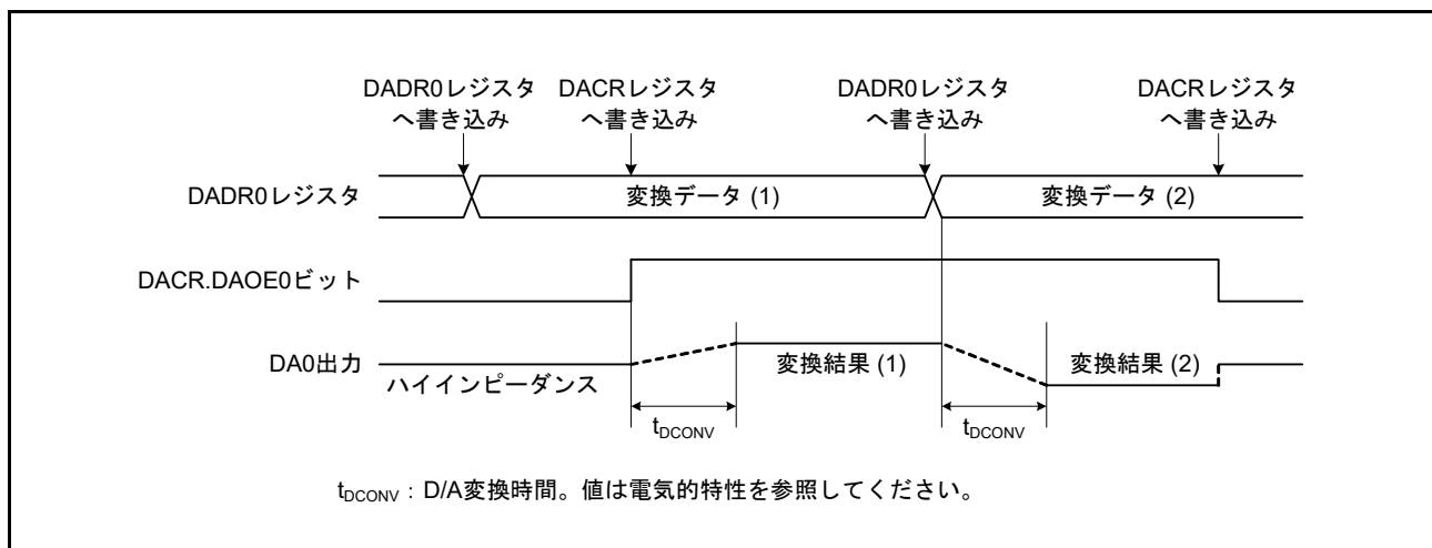
図 55.2 12ビットD/Aコンバータの動作例
