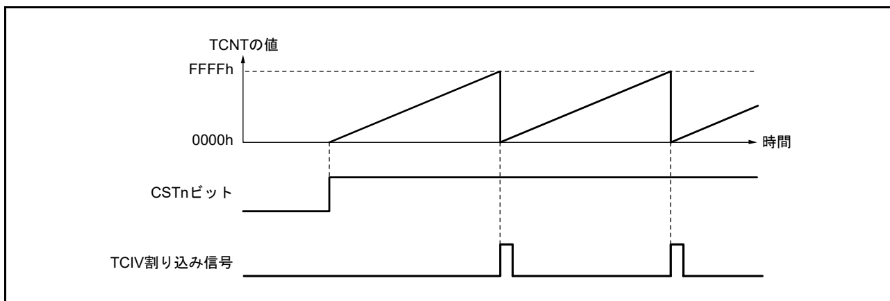
図 24.6 フリーランニングカウンタの動作
