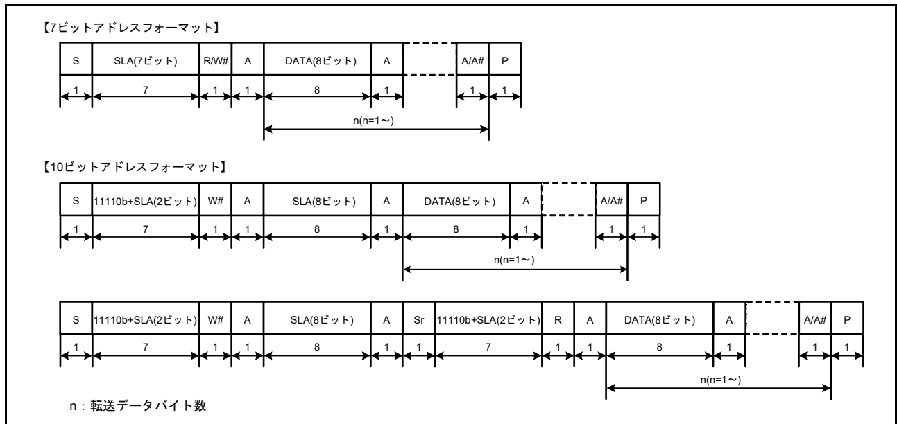
図 41.2 I 2 C バスフォーマット
