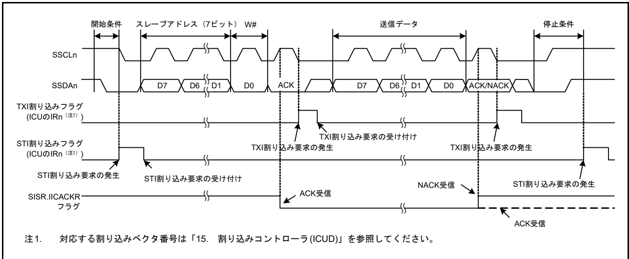
図 40.56 簡易 I 2 C バスモードのマスタ送信の動作例 1 (7 ビットスレーブアドレス、送信割り込み、受信割り込み使用時)
