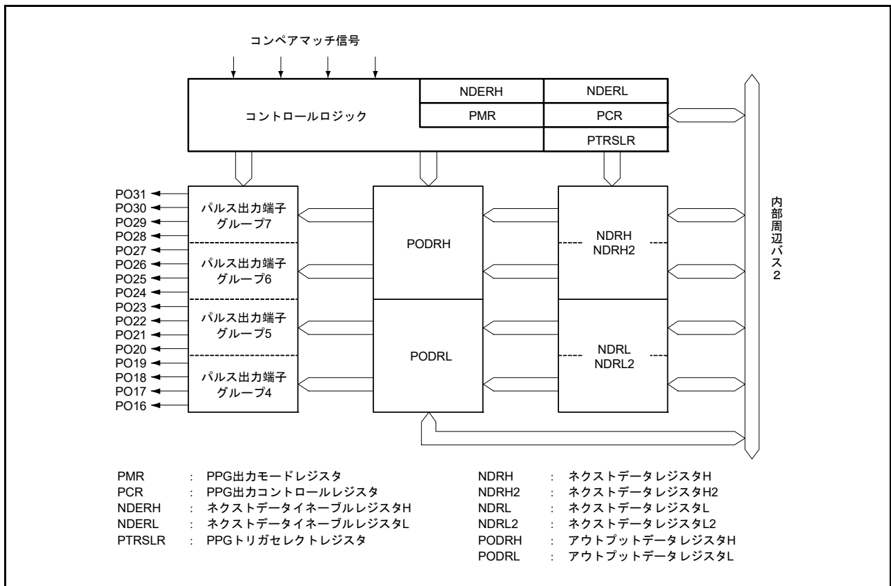
図 29.2 PPG1 のブロック図
