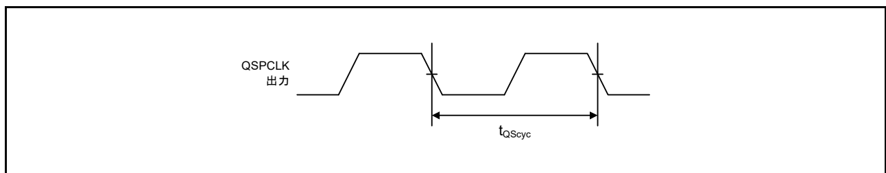
図 61.70 QSPI クロックタイミング
