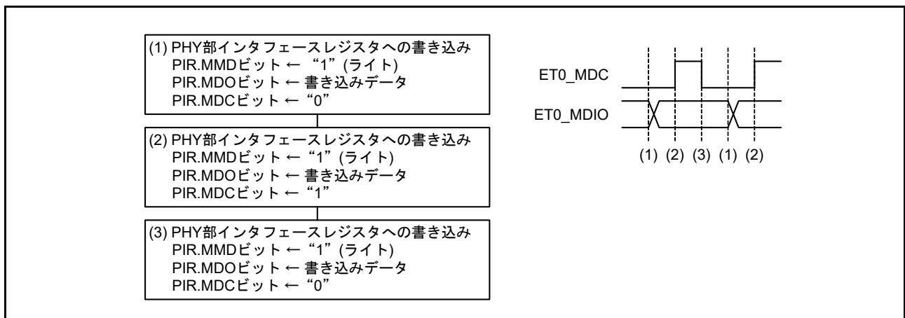
図 36.14 1 ビットデータのライトフロー
