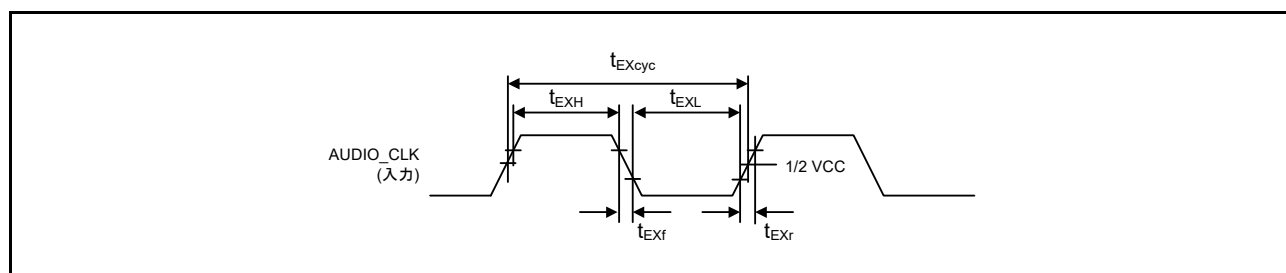
図 61.73 クロック入力タイミング
