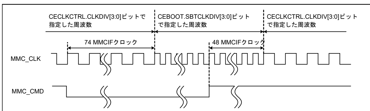
図 48.10 Boot Operation 時の MMCIF クロック周波数切り替え
