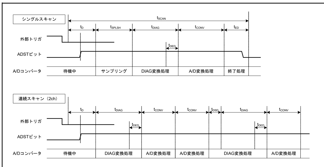
図 54.39 スキャン変換のタイミング (非同期トリガ起動の場合)
