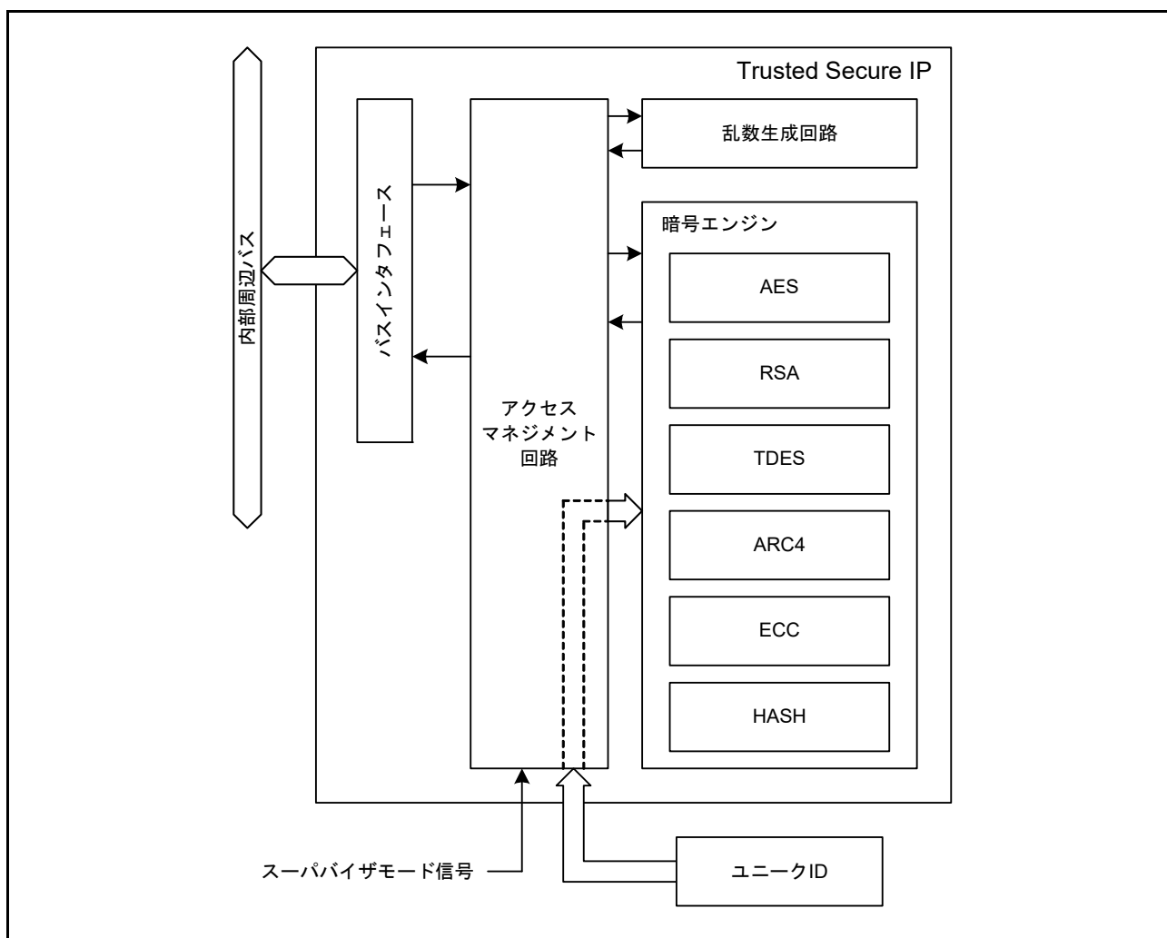
図 53.1 Trusted Secure IPのブロック図
