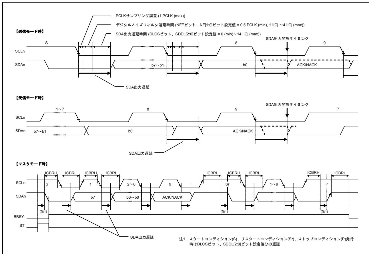
図 41.21 SDA 出力遅延タイミング
