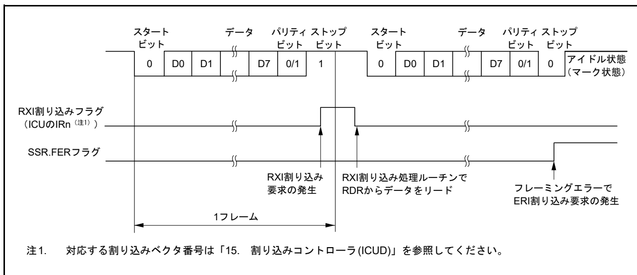
図 40.18 調歩同期式モードのシリアル受信時の動作例 (1) (RTS 機能未使用時) (8 ビットデータ / パリティあり / 1 ストップビットの例)
