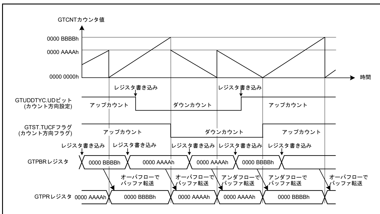
図 26.53 カウント方向切り替え機能の動作例 (バッファ動作時)
