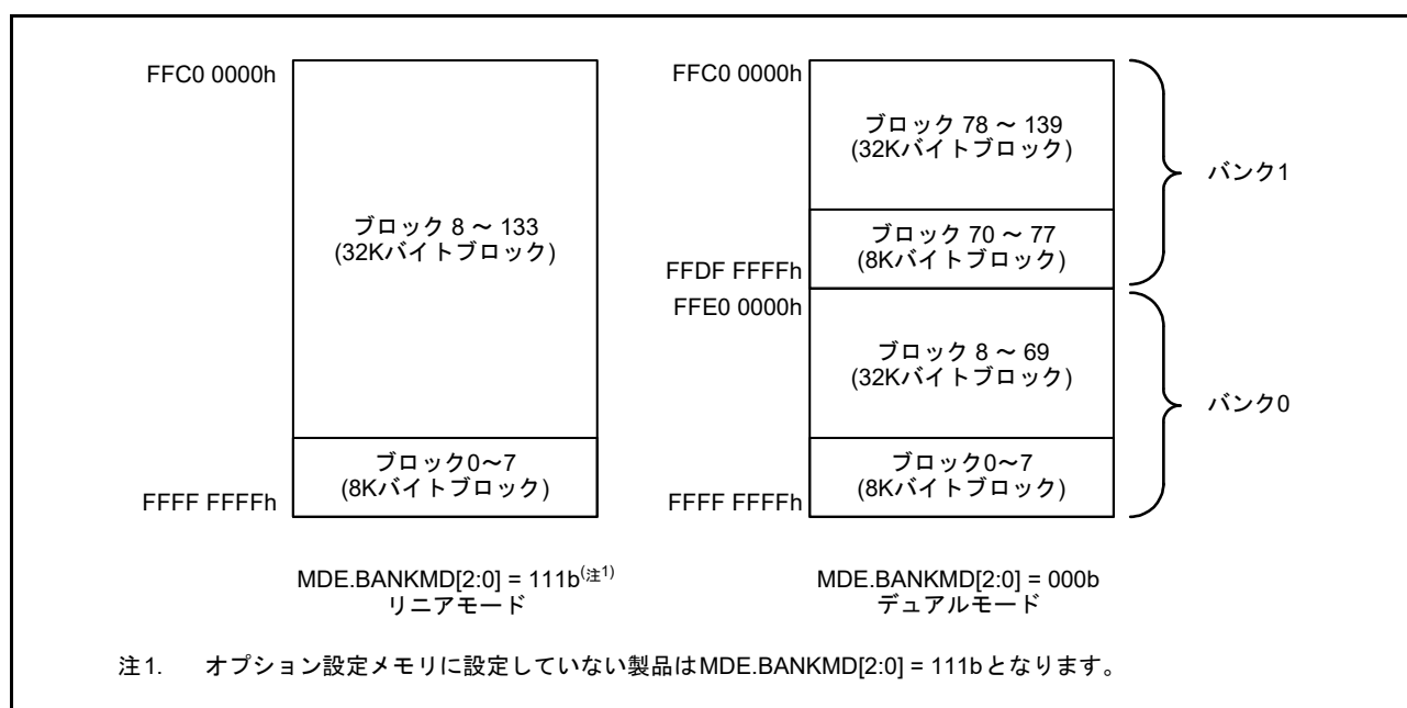
図 60.31 バンクモード切り替え例 (コードフラッシュメモリ容量が4Mバイトの製品の例)
