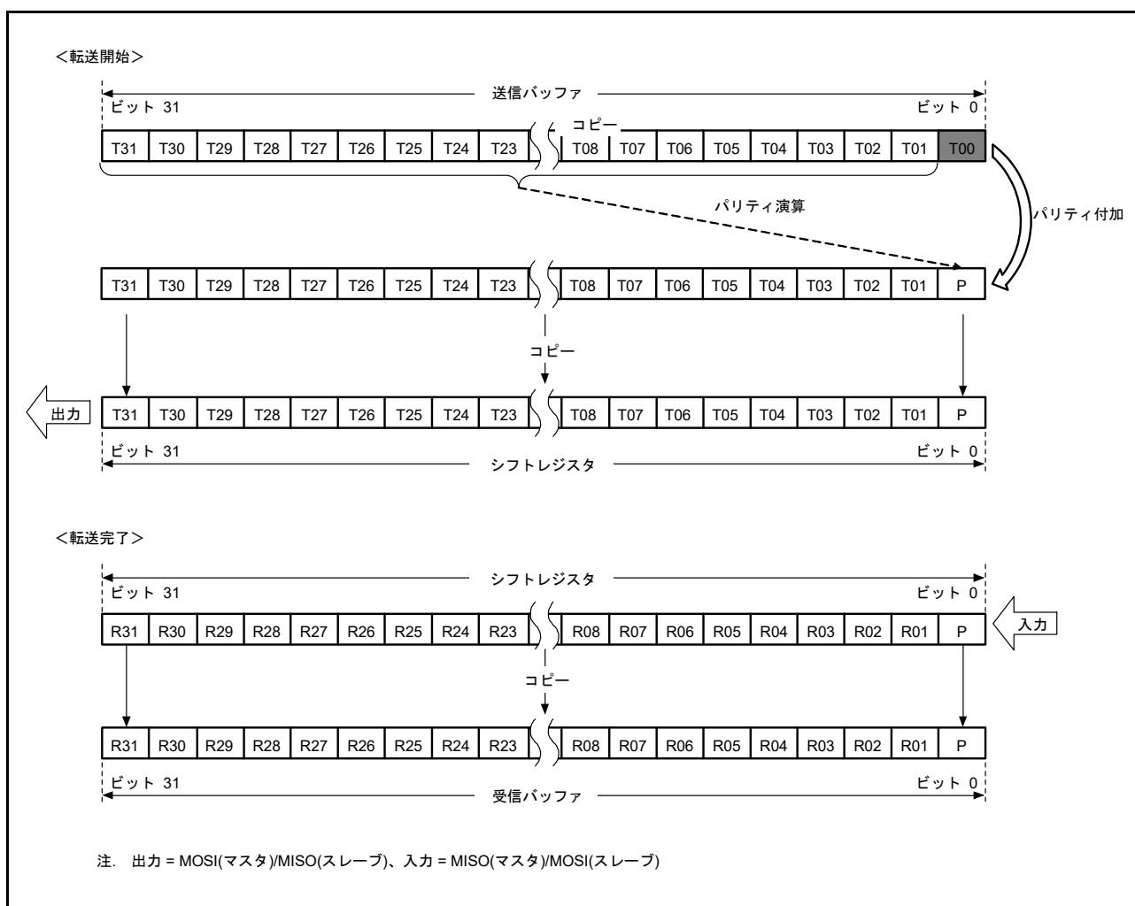
図 43.18 MSB ファースト転送 (32 ビットデータ / パリティ機能有効)
