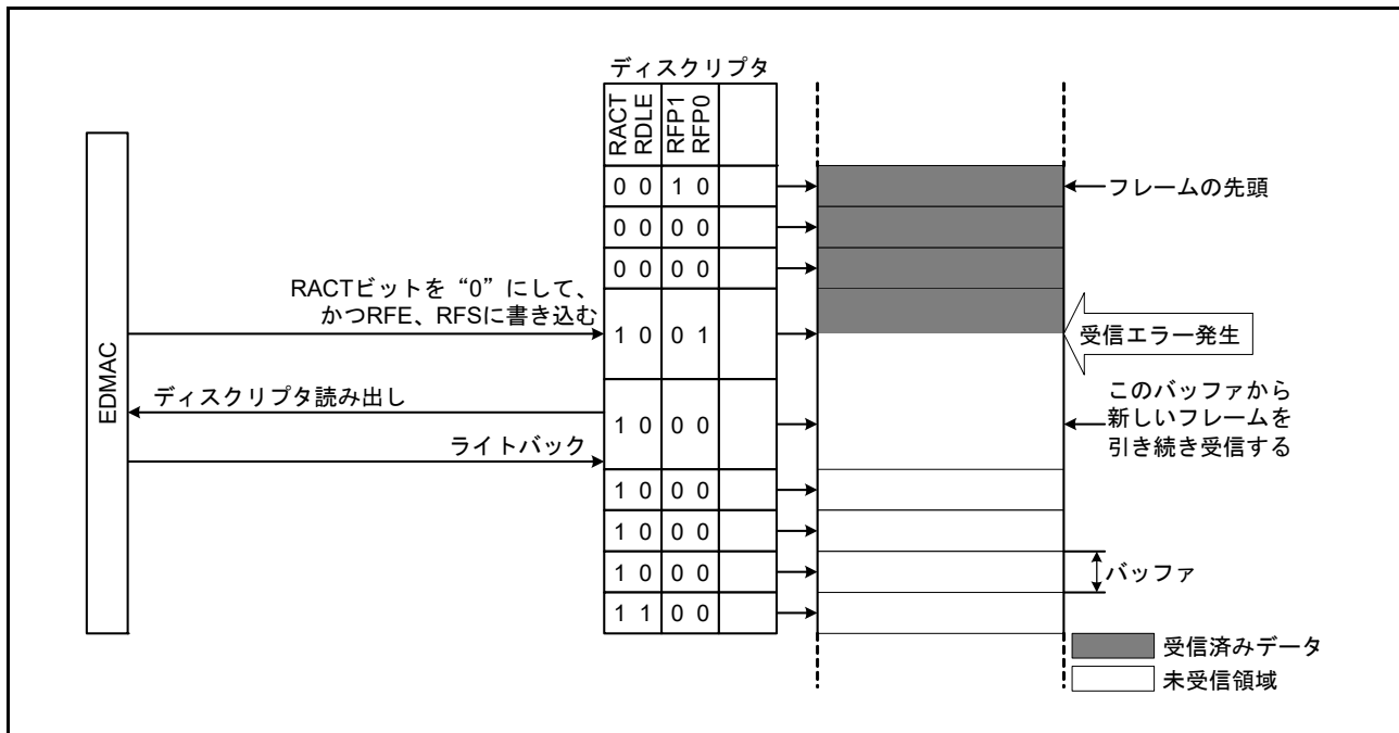
図 37.8 受信エラー発生後の EDMA 動作
