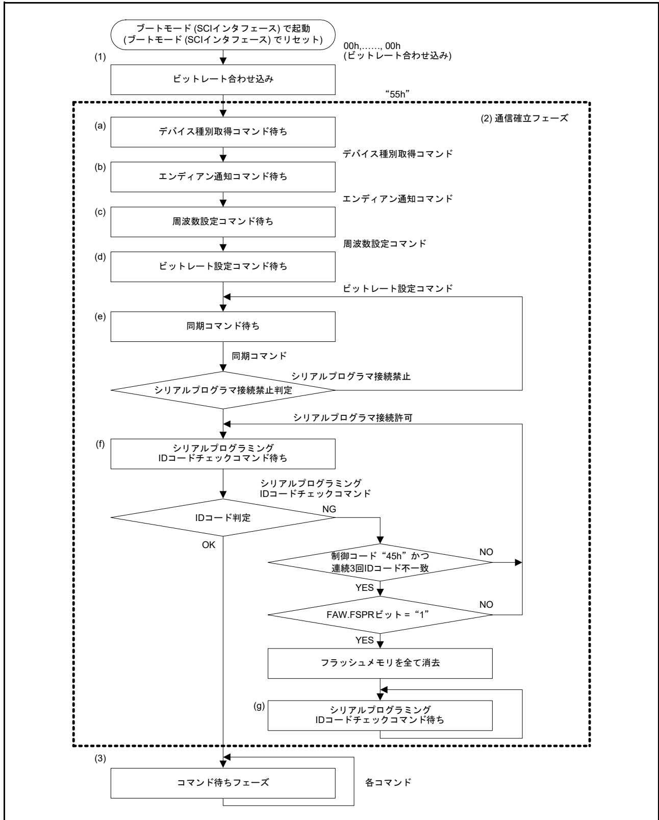
図 60.38 ブートモード (SCI インタフェース) の状態遷移フロー
