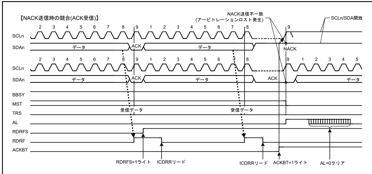
図 41.34 NACK 送信アービトレーションロスト検出動作例 (NALE ビット = 1 のとき)
