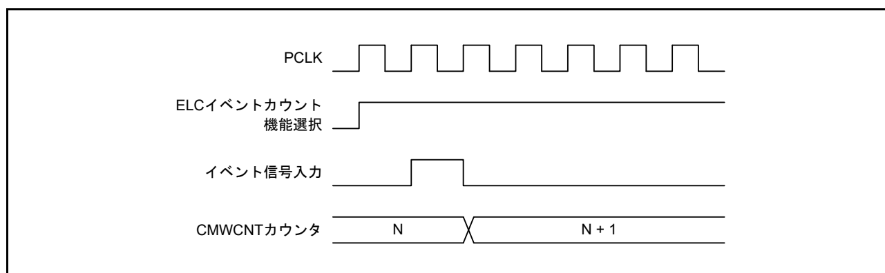
図 32.18 イベント受け付けによるイベントカウント動作
