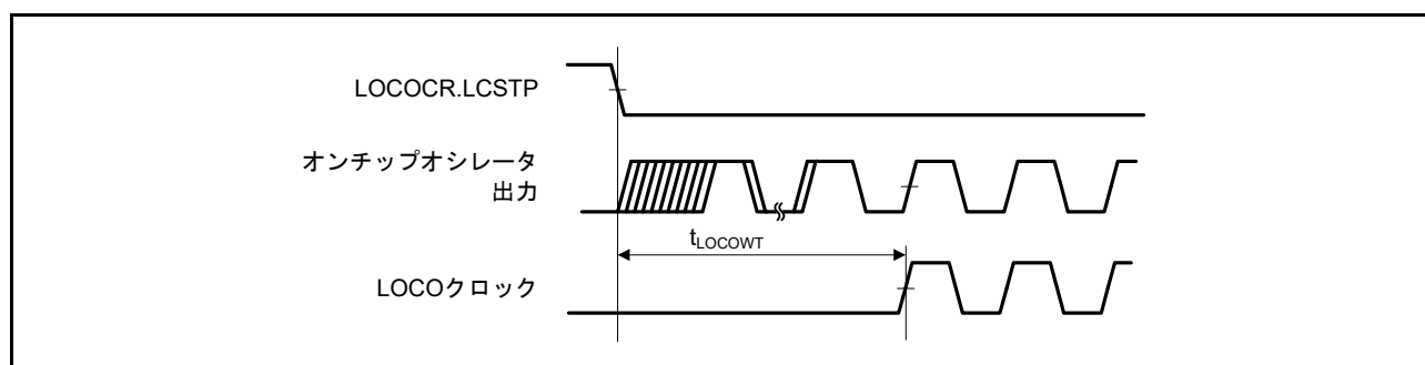
図 61.6 LOCO クロック発振開始タイミング
