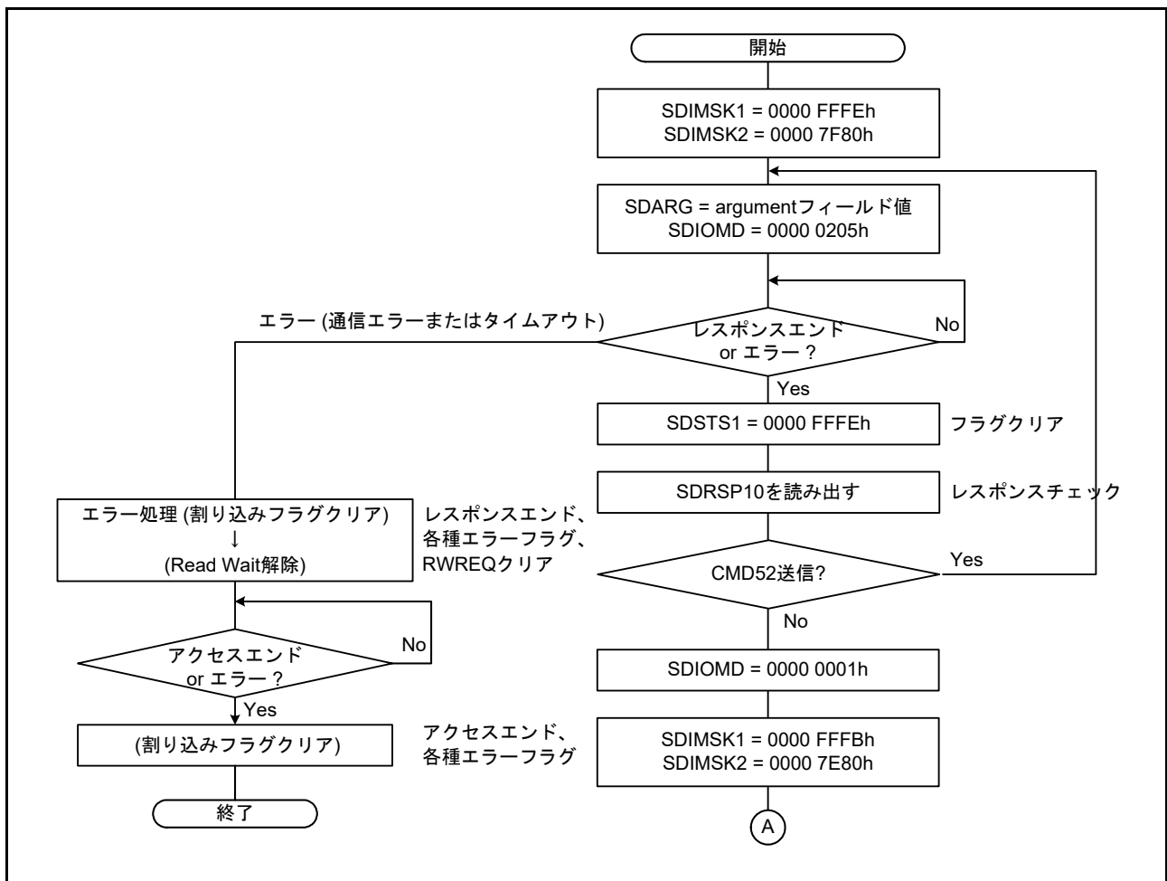
図 47.17 IO_RW_EXTENDED コマンド (CMD53/ マルチブロックリード) のシーケンス中に Read Wait 状態にした後、SDIO none abort コマンド (CMD52) を送信する例
