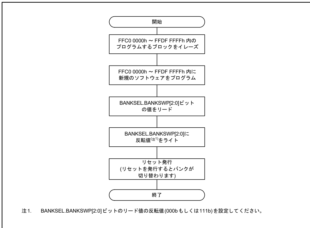
図 60.33 起動バンク選択フロー例 (コードフラッシュメモリ容量が4Mバイトの製品の例)
