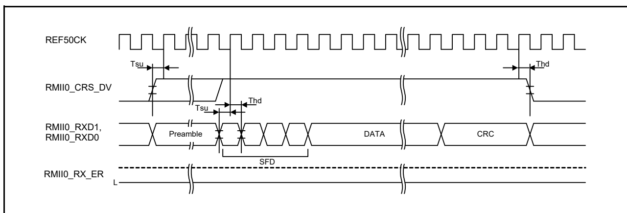
図 61.83 RMII 受信タイミング (正常動作時)
