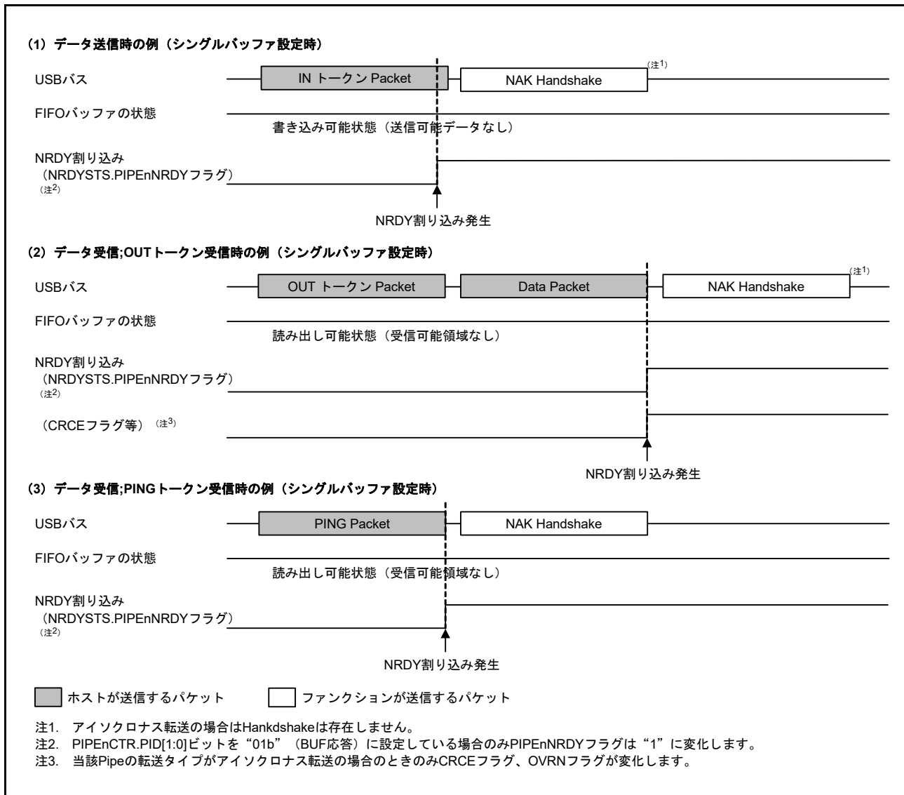
図 39.12 NRDY 割り込み発生タイミング図 (ファンクションコントローラ機能選択時)
