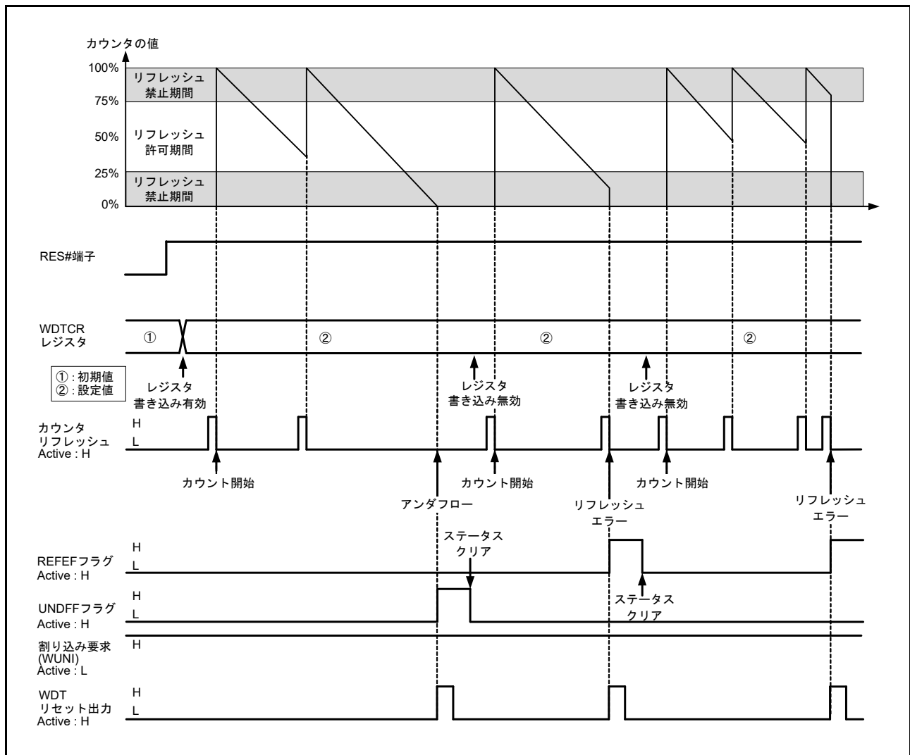
図 34.3 レジスタスタートモード動作例
