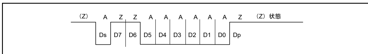
図 40.40 インバースコンベンション (SCMR.SDIR ビット = 1、SCMR.SINV ビット = 1、SMR.PM ビット = 1)
