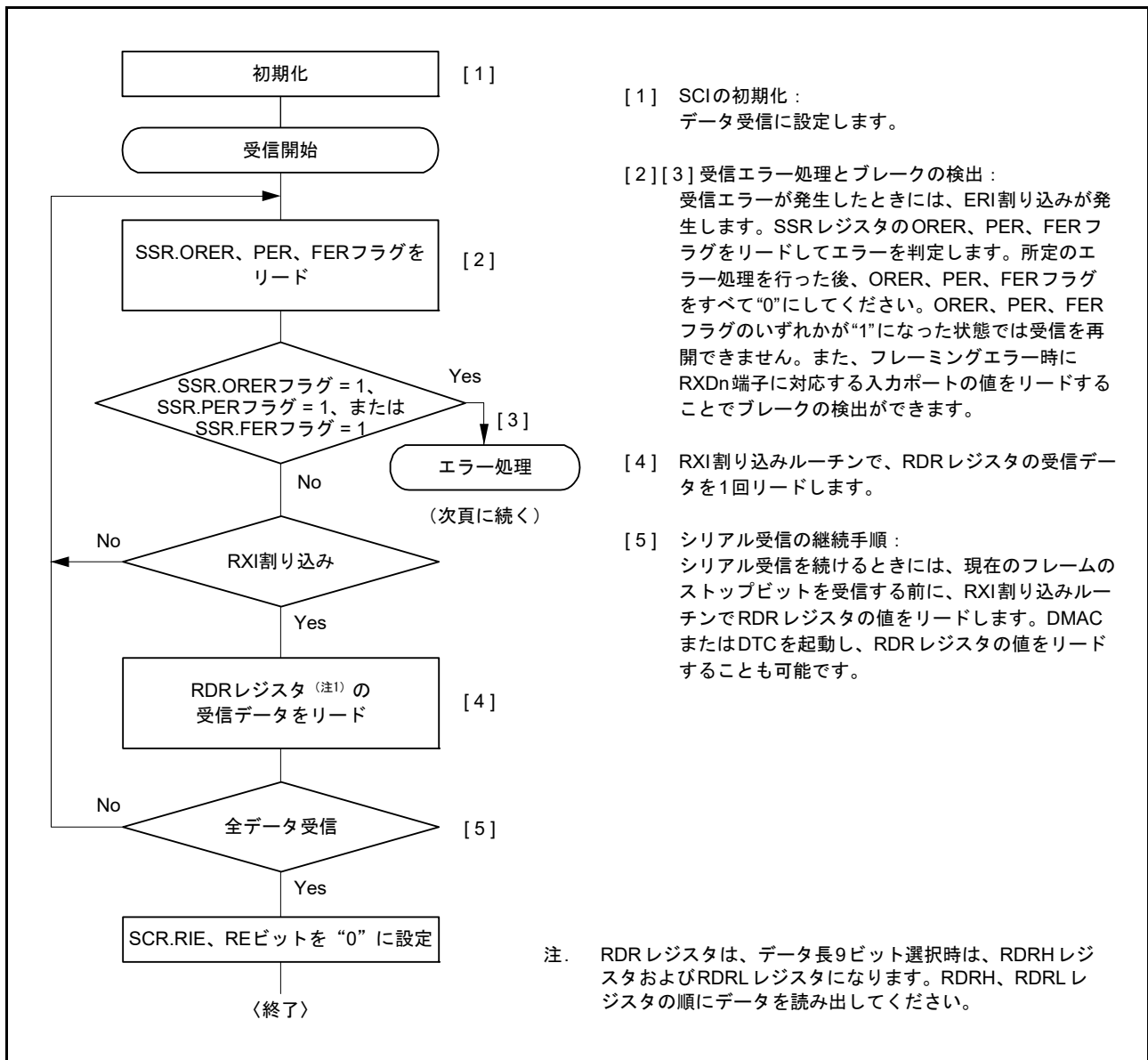
図 40.20 調歩同期式モードのシリアル受信のフローチャート例 (1)
