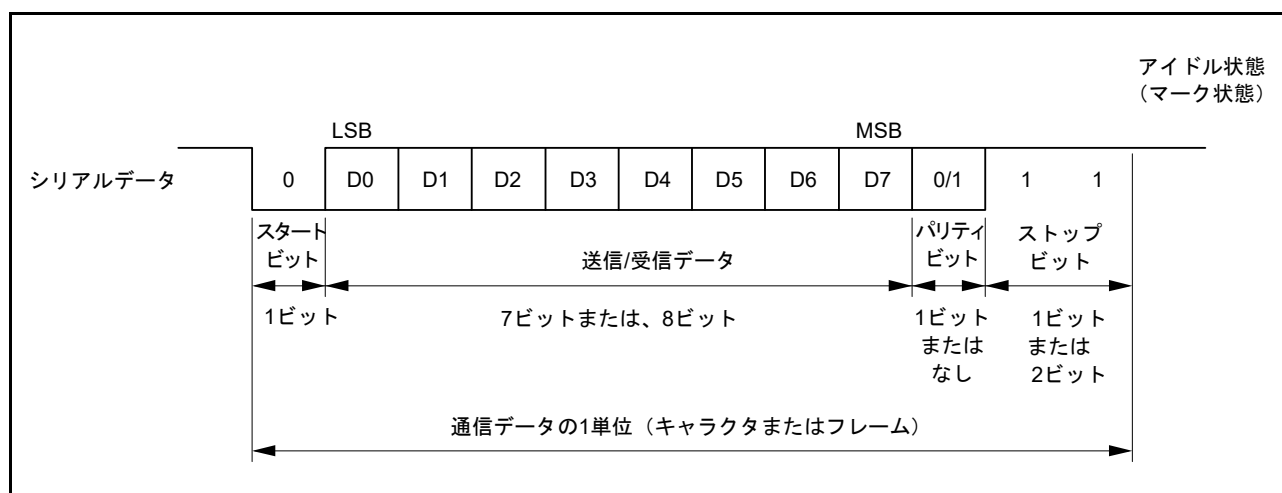
図 40.6 調歩同期式シリアル通信のデータフォーマット (8 ビットデータ / パリティあり / 2 ストップビットの例)
