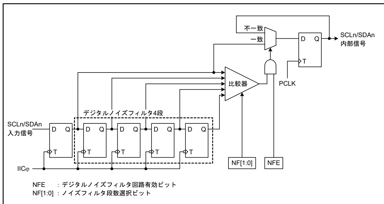
図 41.22 デジタルノイズフィルタ回路のブロック図
