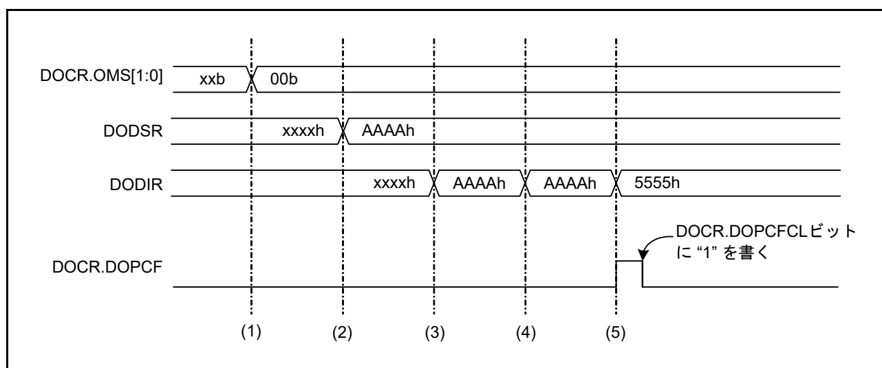
図 57.2 データ比較モードの動作例
