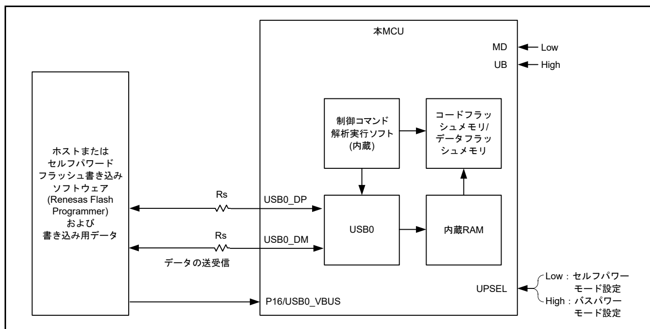
図 60.35 ブートモード (USB インタフェース) 時のシステム構成
