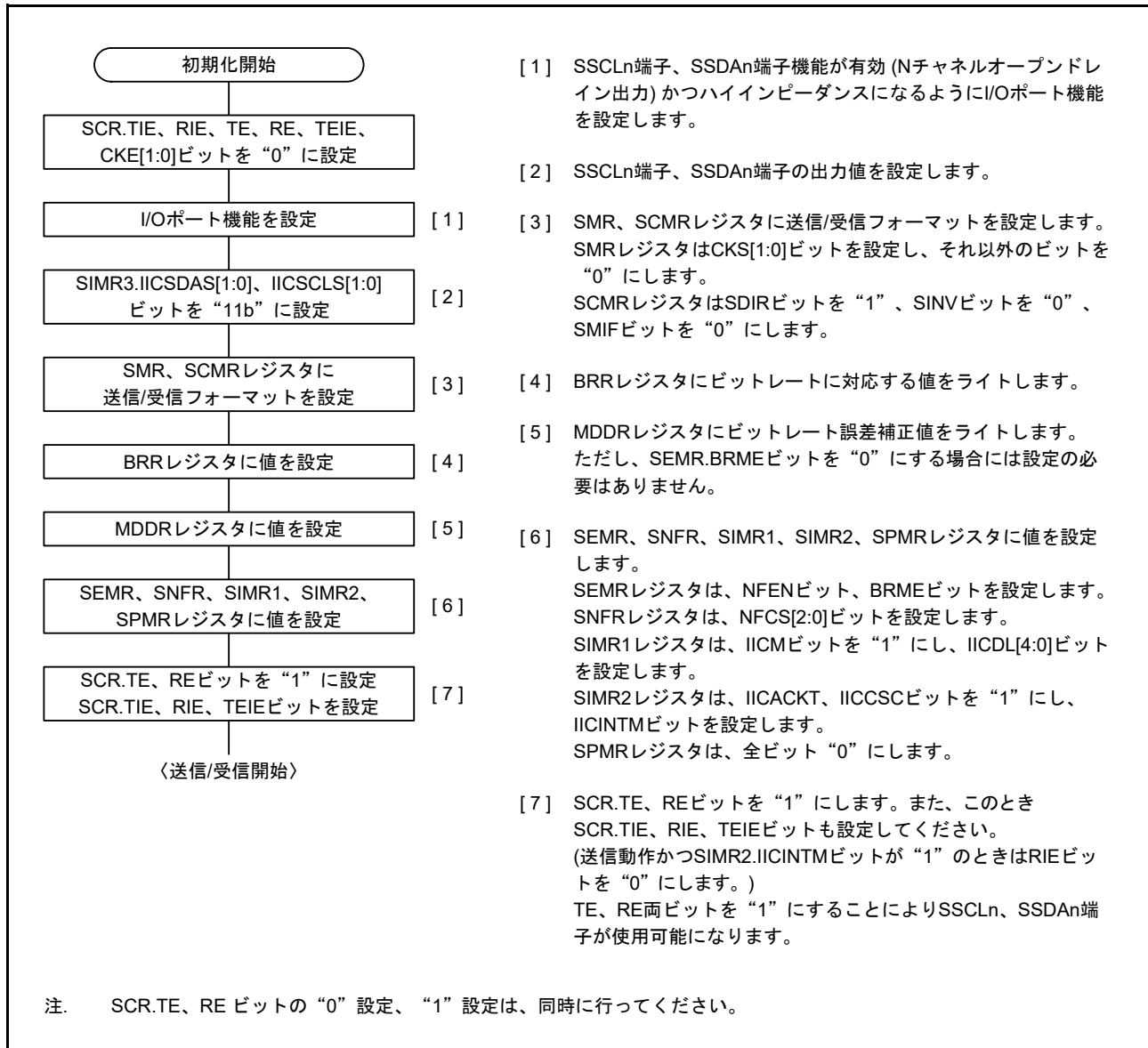
図 40.55 SCIの初期化フローチャート例 (簡易 I 2 C モード)
