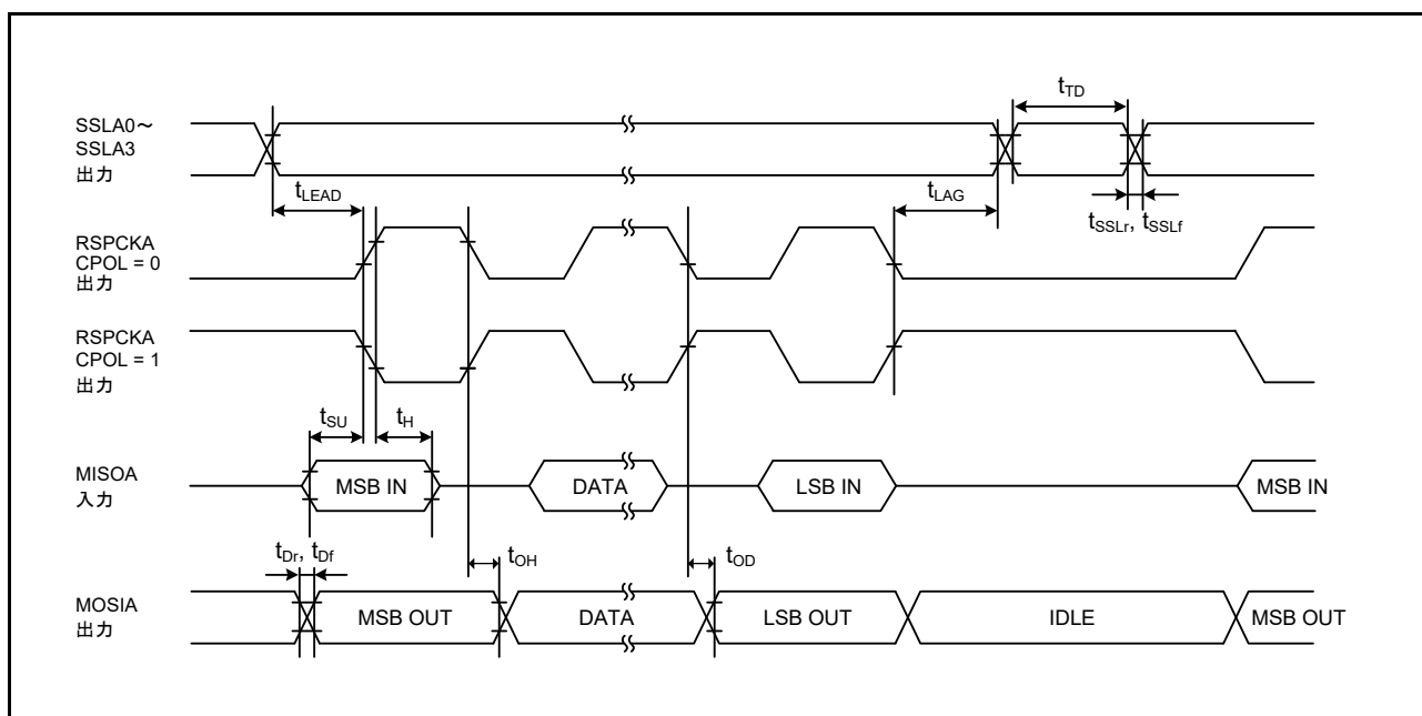
図 61.64 RSPCKA タイミング (マスタ、CPHA = 0) (ビットレート : PCLKA を 2 分周以外に設定)
