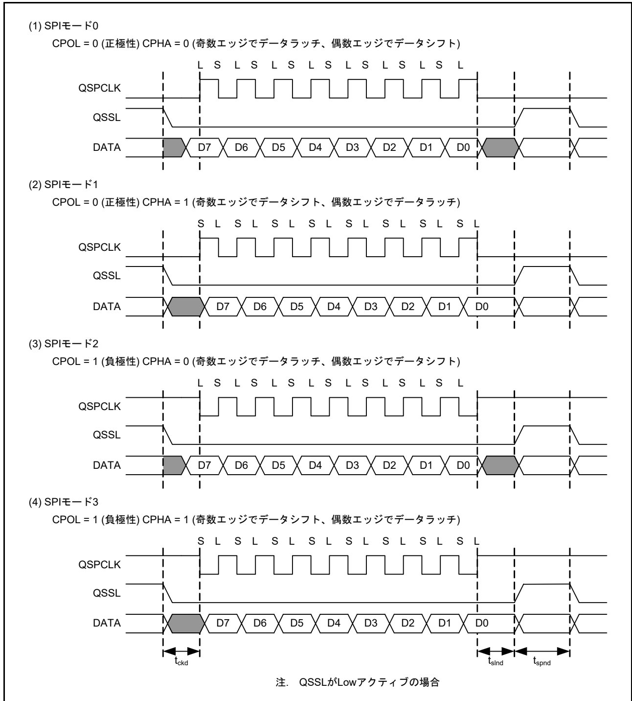
図 44.2 クロック設定と転送タイミング
