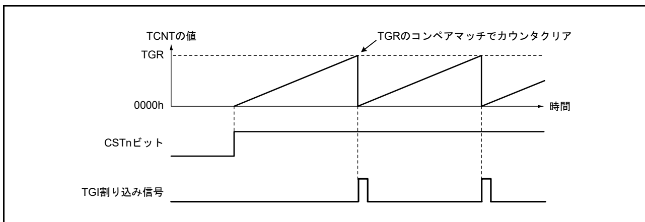
図 24.7 周期カウンタの動作
