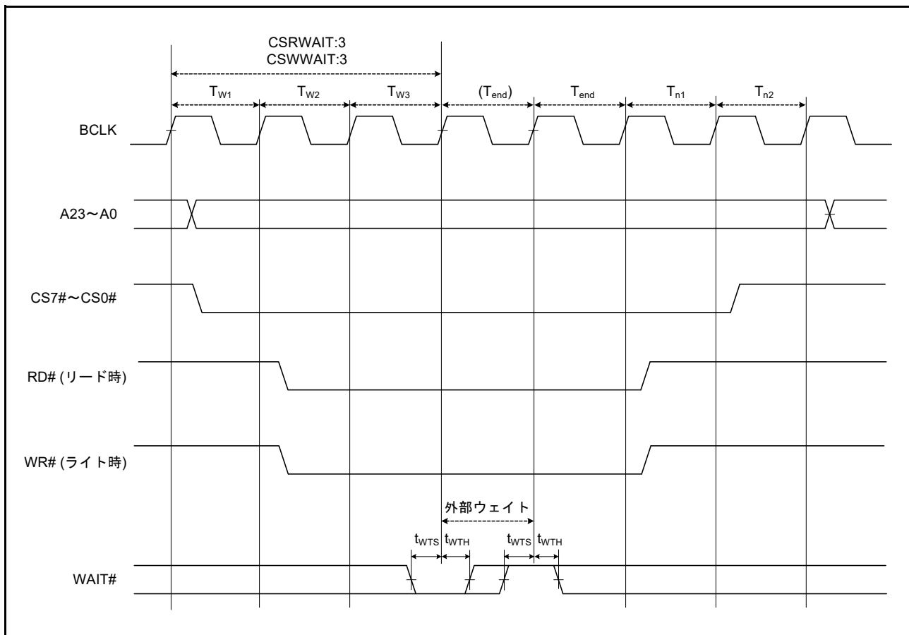
図 61.24 外部バスタイミング / 外部ウェイト制御
