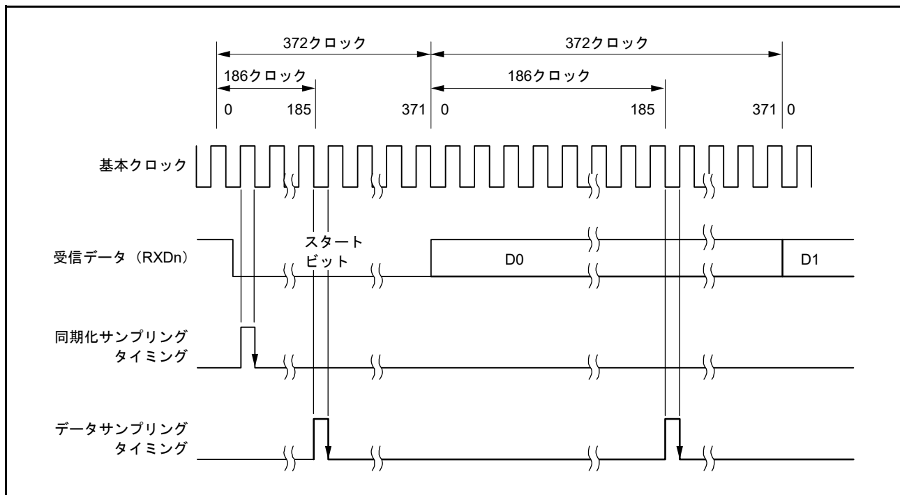
図 40.41 スマートカードインタフェースモード時の受信データサンプリングタイミング (372 倍のクロック使用時)
