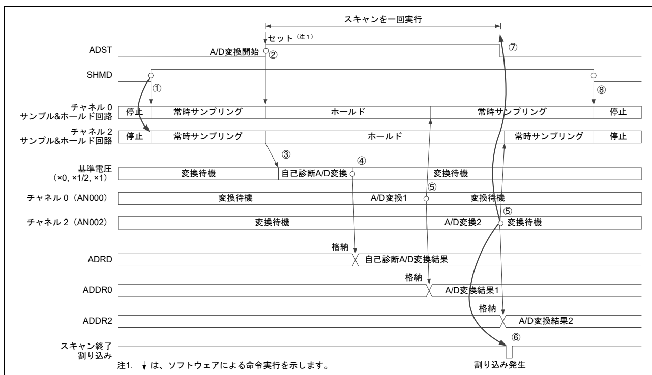
図 54.11 シングルスキャンモードの動作例 (チャンネル専用サンプル & ホールド回路使用 : AN000, AN002 選択 + 自己診断、常時サンプリング有効)
