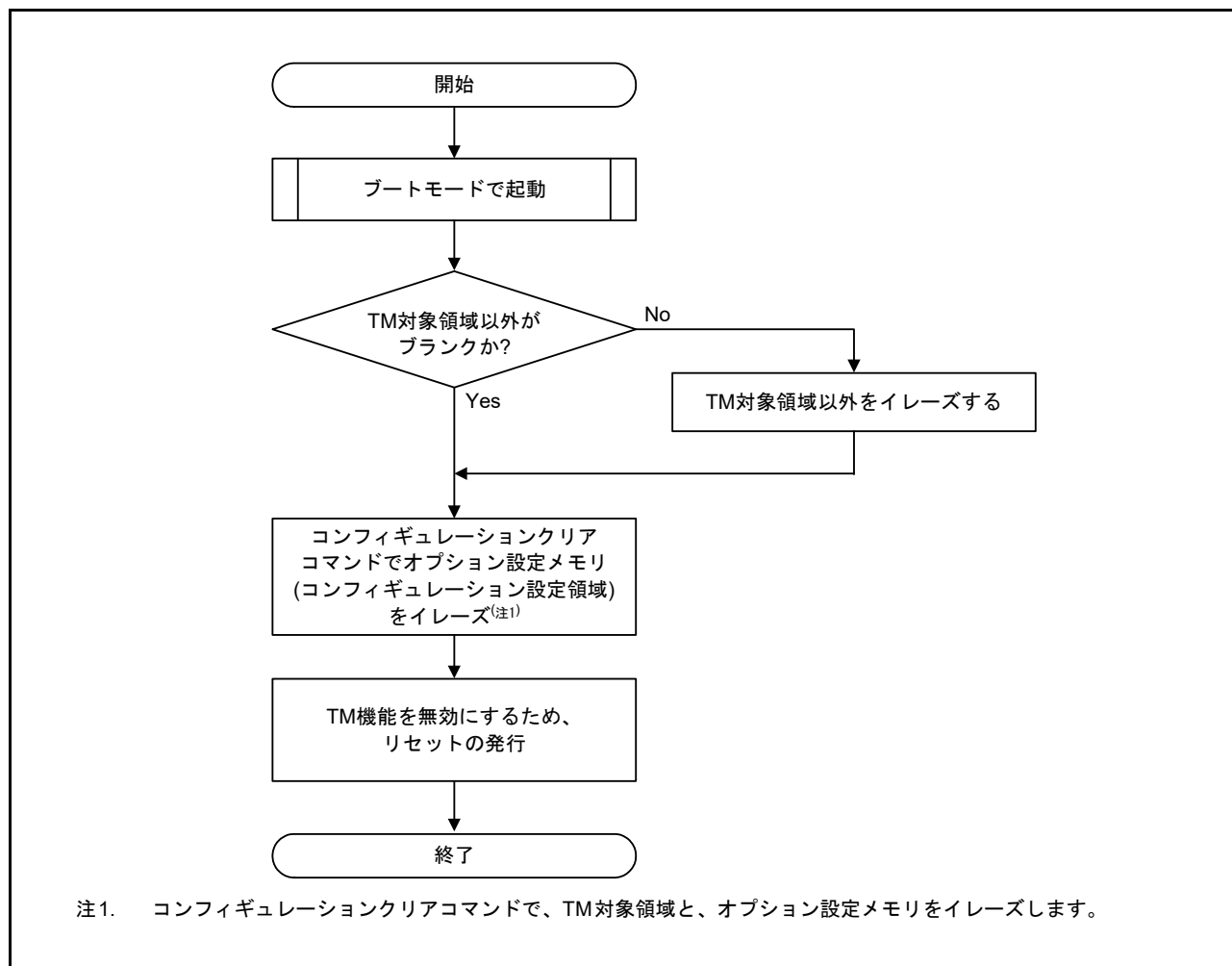
図 60.58 ブートモードで TM 機能を無効にするためのフロー
