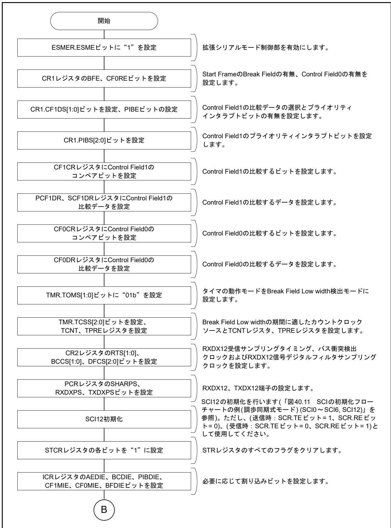
図 40.69 Start Frame 受信フローチャート例 (1)
