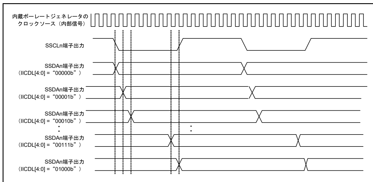
図 40.54 SSDA 出力遅延のタイミング
