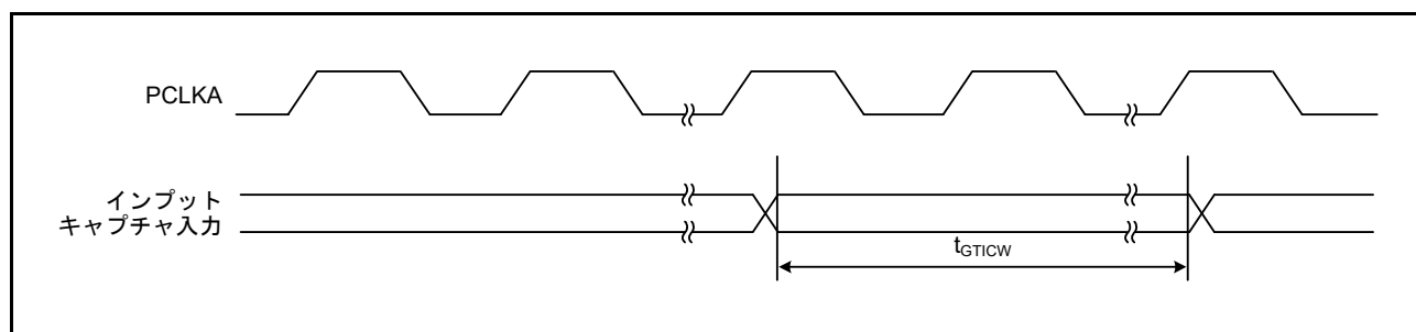
図 61.52 GPTW インプットキャプチャ入力タイミング
