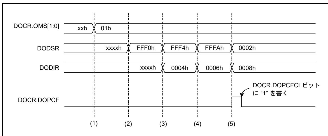
図 57.3 データ加算モードの動作例
