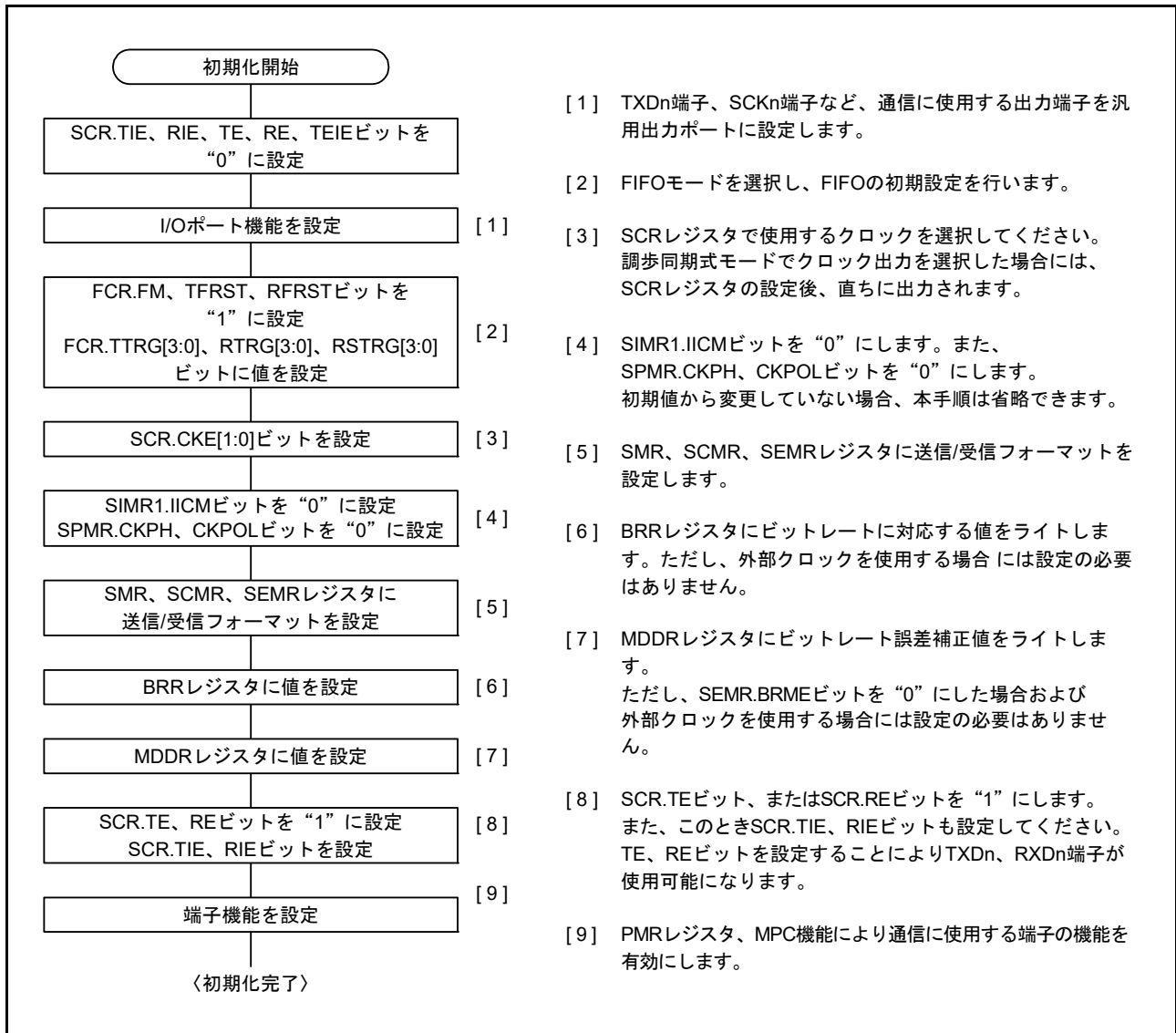
図 40.12 SCI の初期化フローチャートの例 ( 調歩同期式モード、FIFO 使用 ) (SCI7 ~ SCI11)
