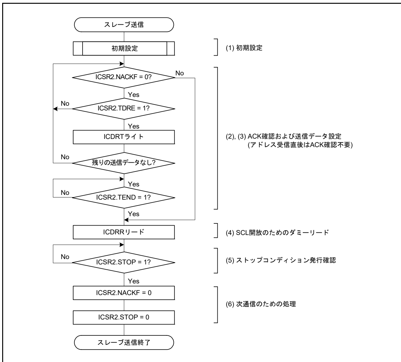
図 41.14 スレーブ送信のフローチャート例
