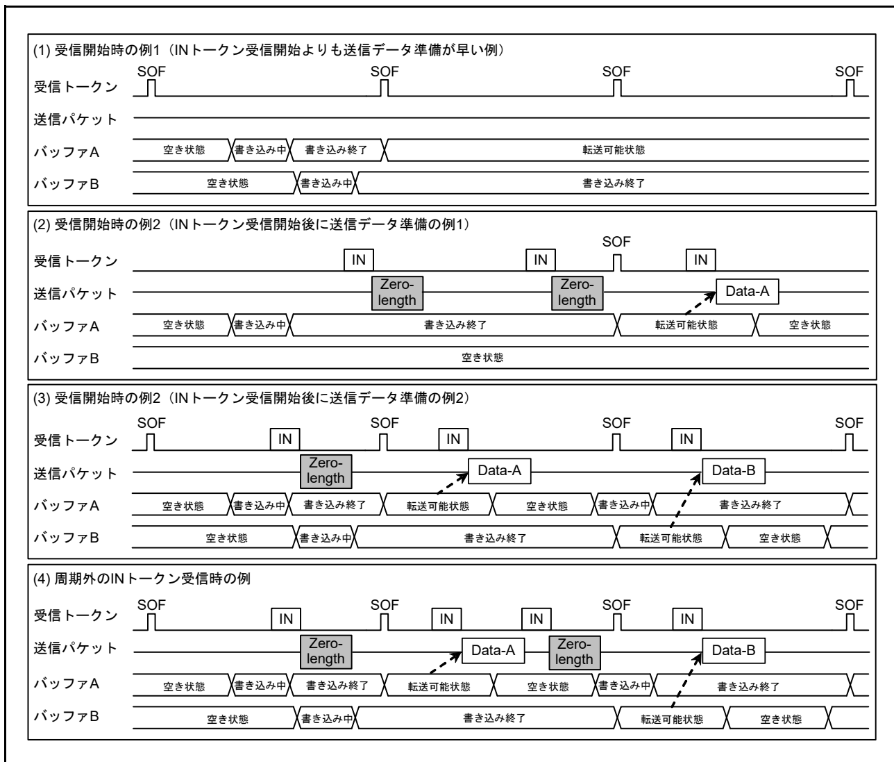
図 39.20 データセットアップ機能動作例
