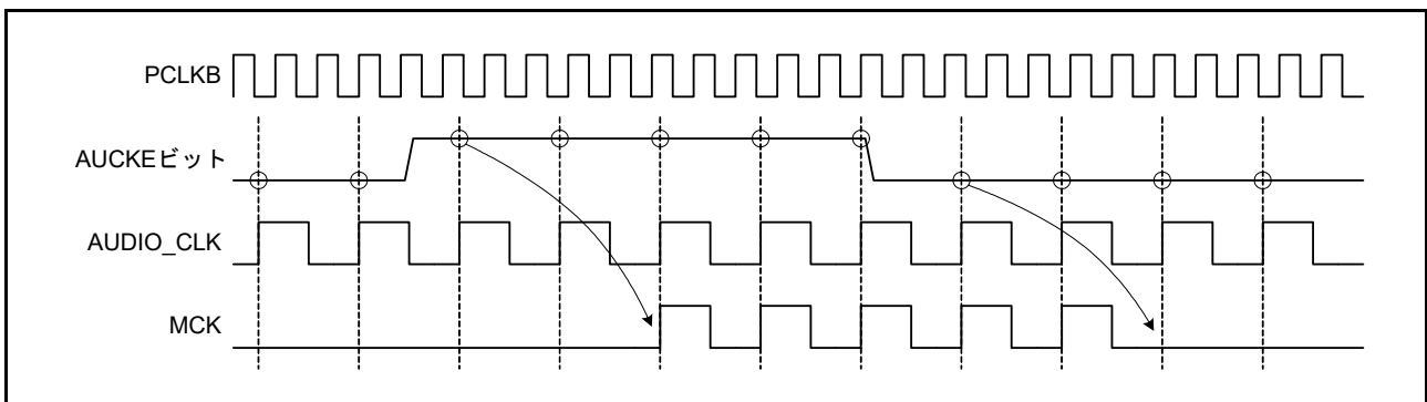
図 46.7 MCK の供給 / 停止
