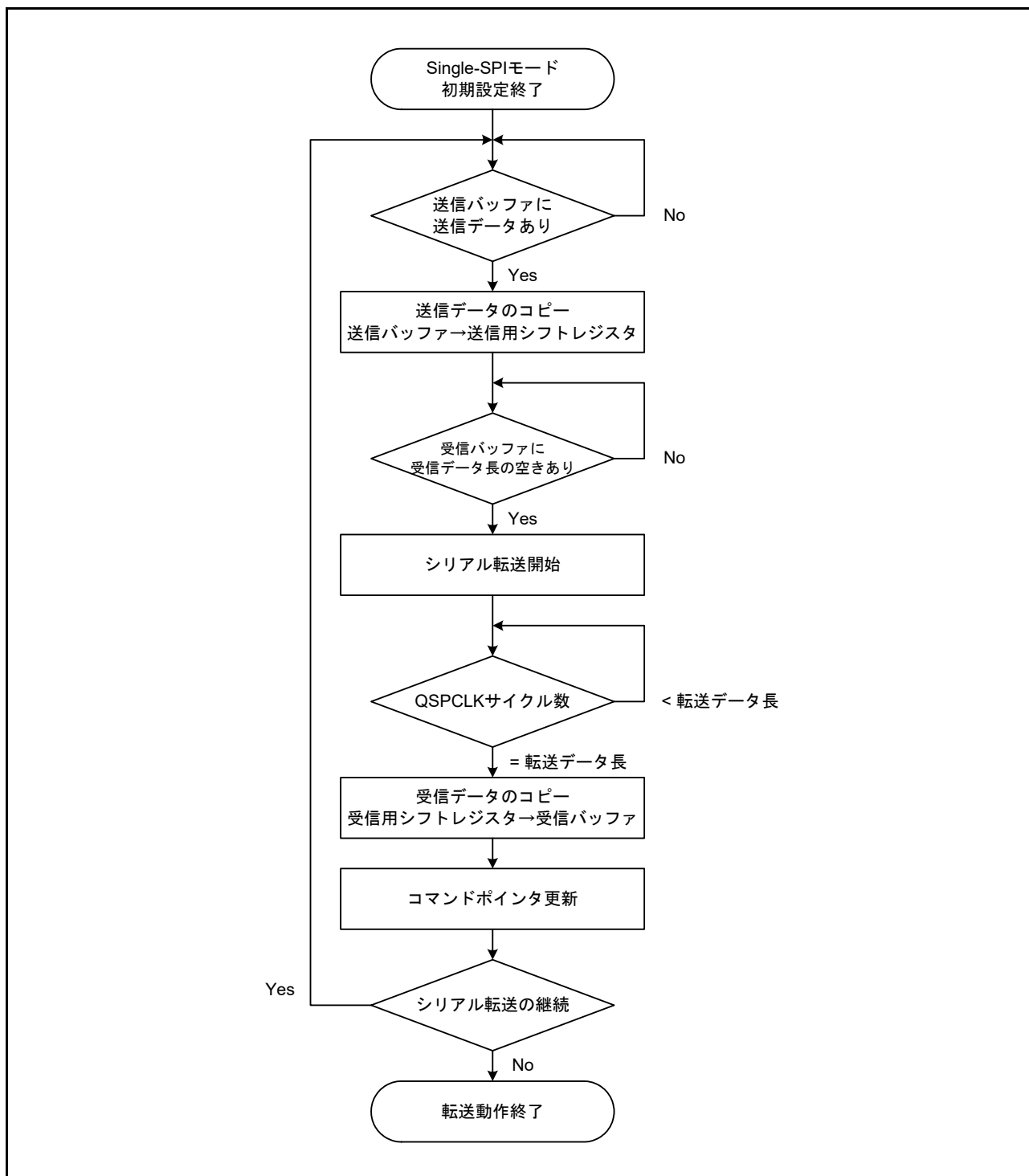
図 44.16 Single-SPIモードの動作フロー
