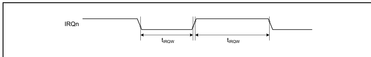
図 61.17 IRQ 割り込み入カタイミング
