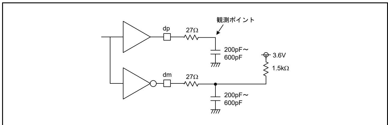
図 61.99 測定回路 (ロースピード時)
