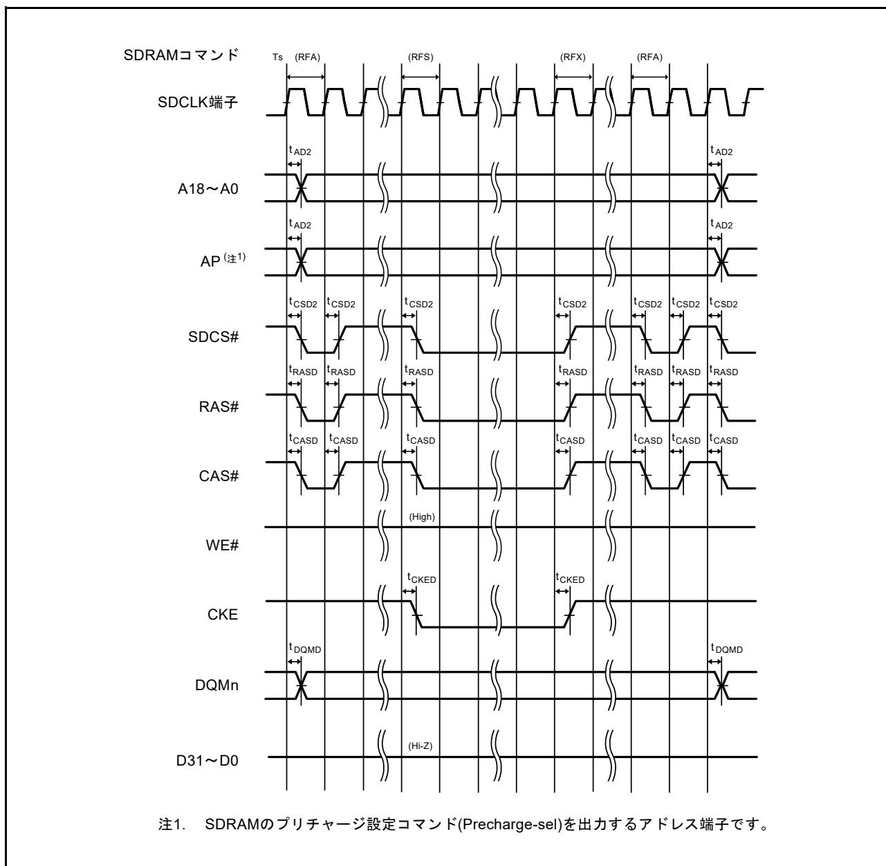
図 61.31 SDRAM 空間セルフリフレッシュバスタイミング
