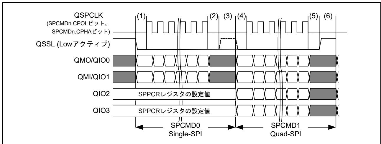
図 44.22 QSSL 信号レベル保持を利用したバースト転送の例 (Single-SPI、Quad-SPI 混合) (n = 0 ~ 3)
