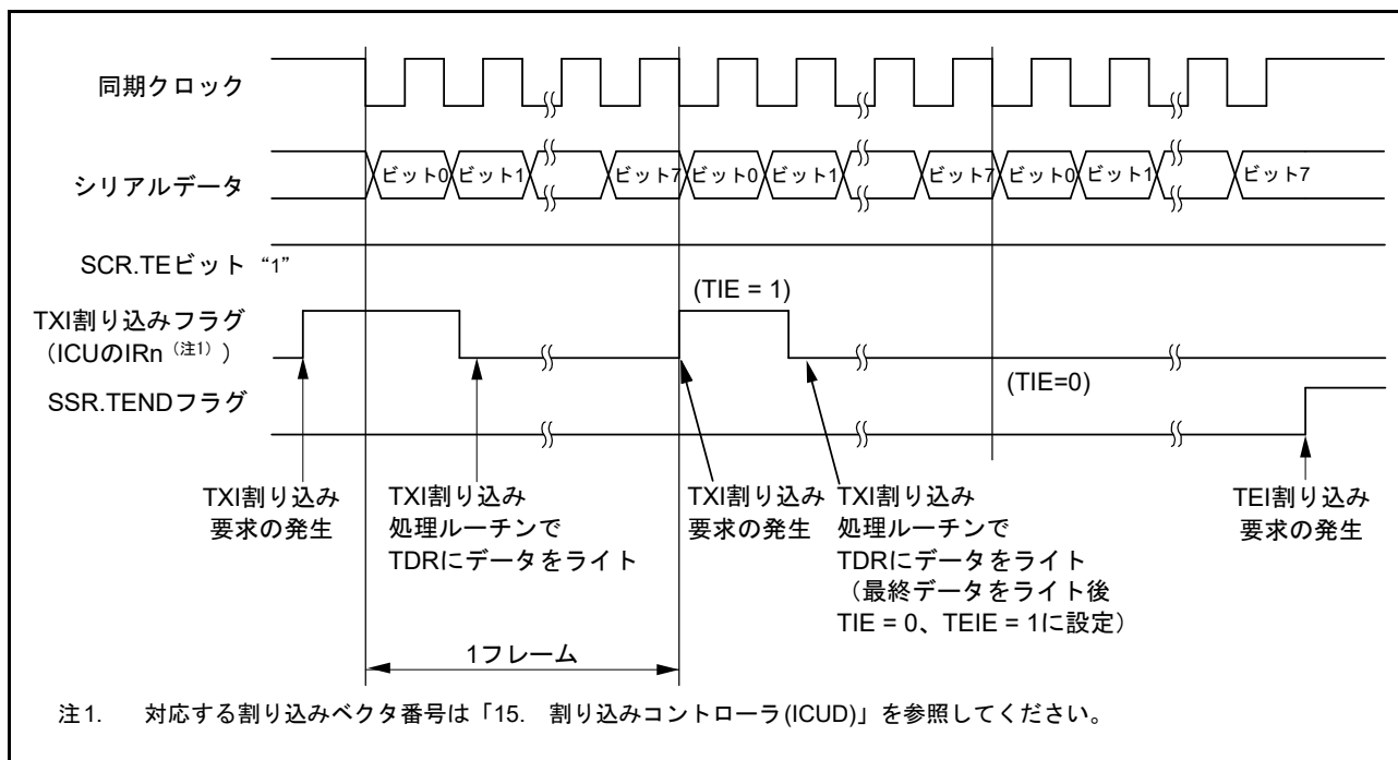
図 40.31 クロック同期式モードのシリアル送信の動作例 (3) (送信中～送信終了時)
