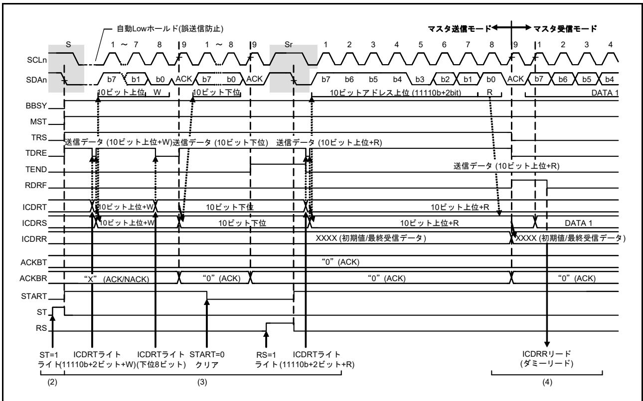
図 41.12 マスタ受信の動作タイミング (2) (10 ビットアドレスフォーマット、RDRFS ビット = 0 のとき)
