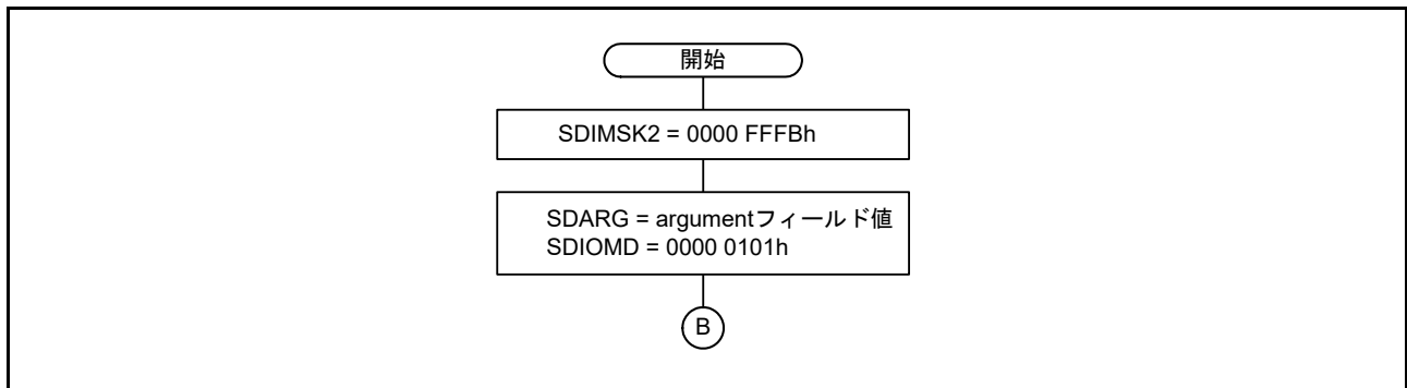
図 47.16 IO_RW_EXTENDED コマンド (CMD53/ マルチブロックリード) のシーケンス中に SDIO abort コマンド (CMD52) を送信する例
