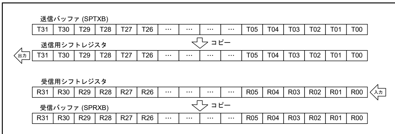
図 44.6 MSB ファースト転送 (32 ビットデータ)
