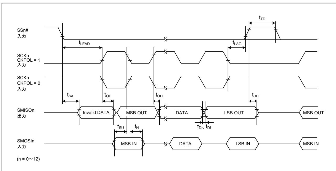
図 61.61 簡易 SPI タイミング (スレーブ、CKPH = 0)
