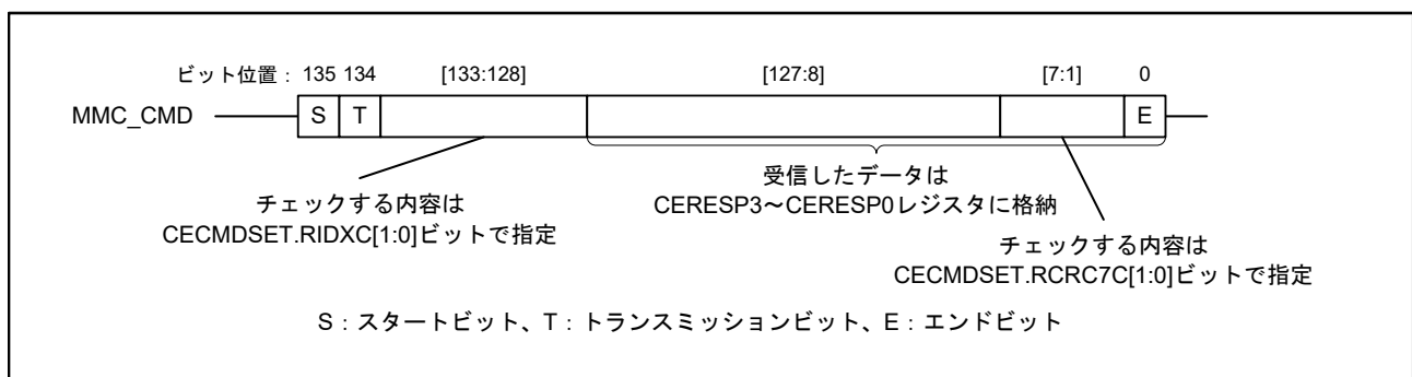
図 48.4 17 バイトのレスポンス (R2 レスポンス) のフォーマット
