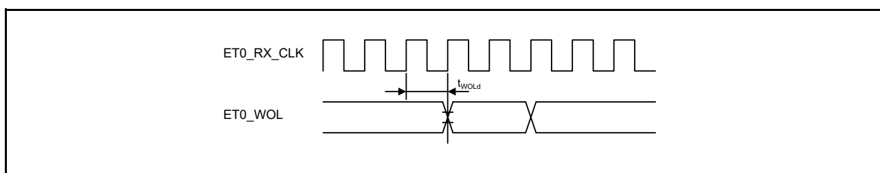
図 61.90 WOL 出カタイミング (MII)
