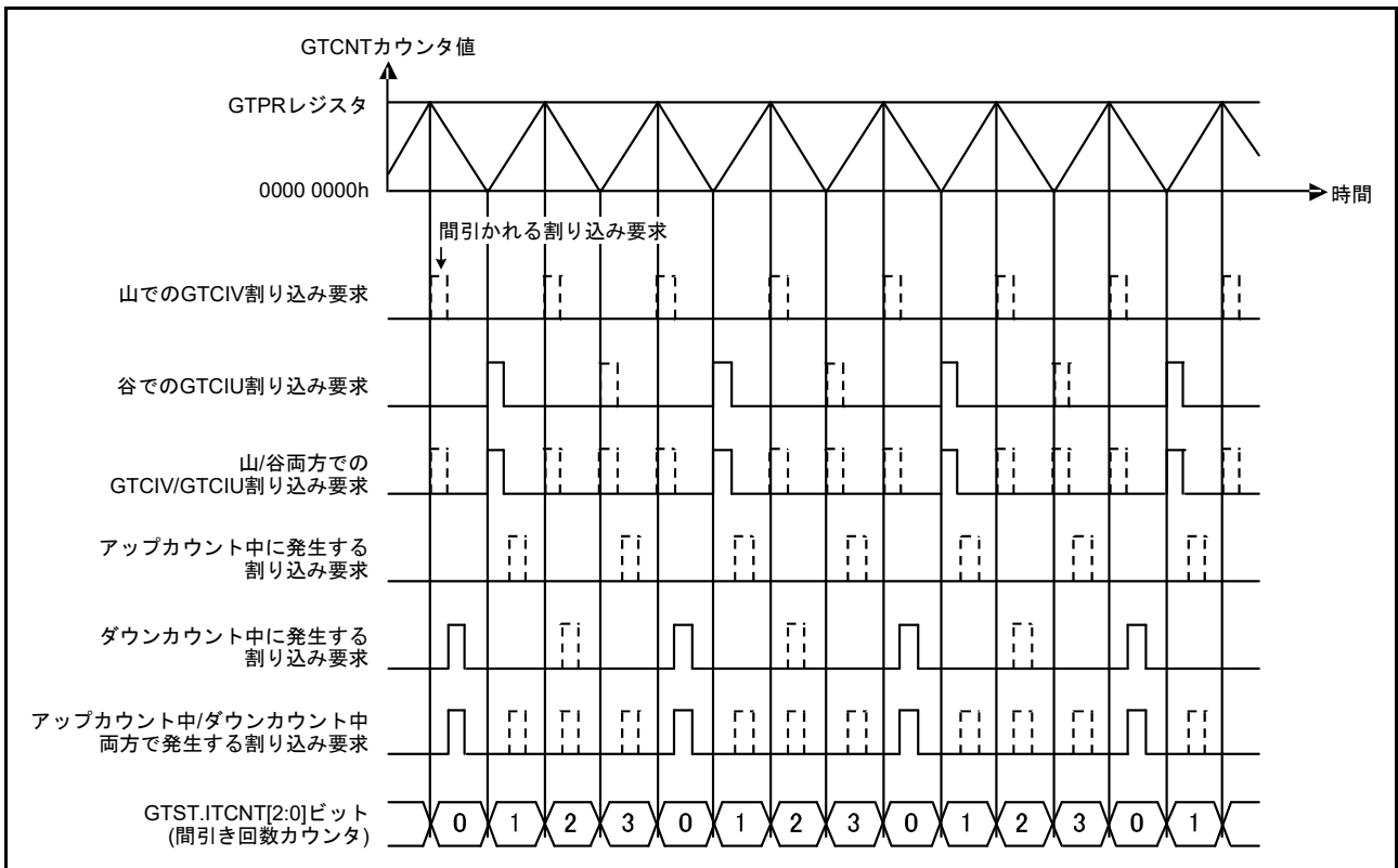
図 26.100 割り込み間引き機能の動作例 (三角波、谷 / 山両方をカウントして間引き、間引き回数 3、アップカウントで間引き開始の場合)
