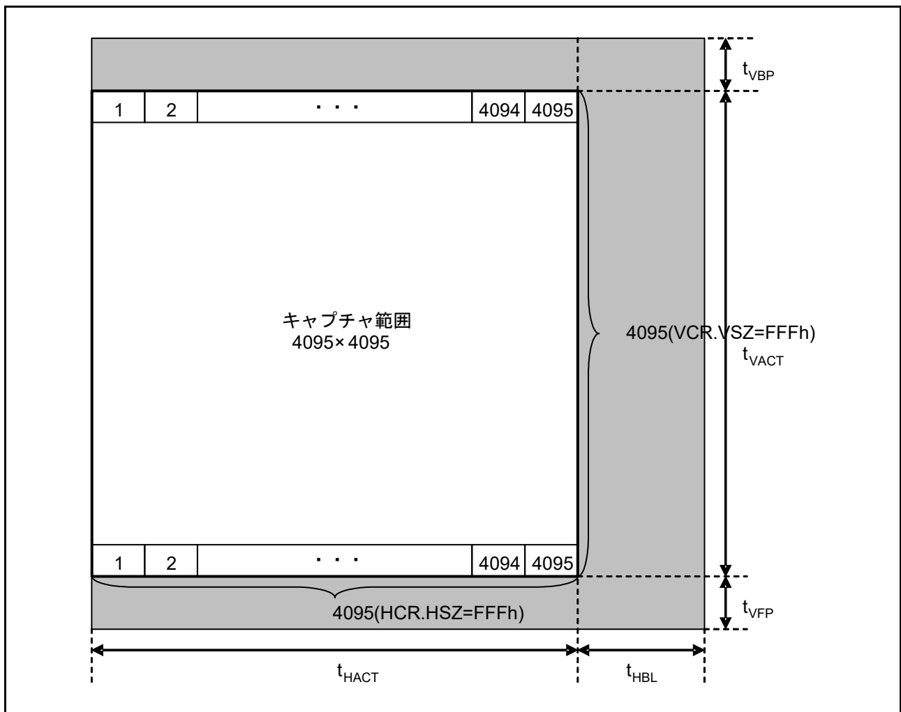
図 49.9 VCR レジスタ、HCR レジスタ設定とキャプチャ範囲 (VCR = 0FFF 0000h, HCR = 0FFF 0000h)
