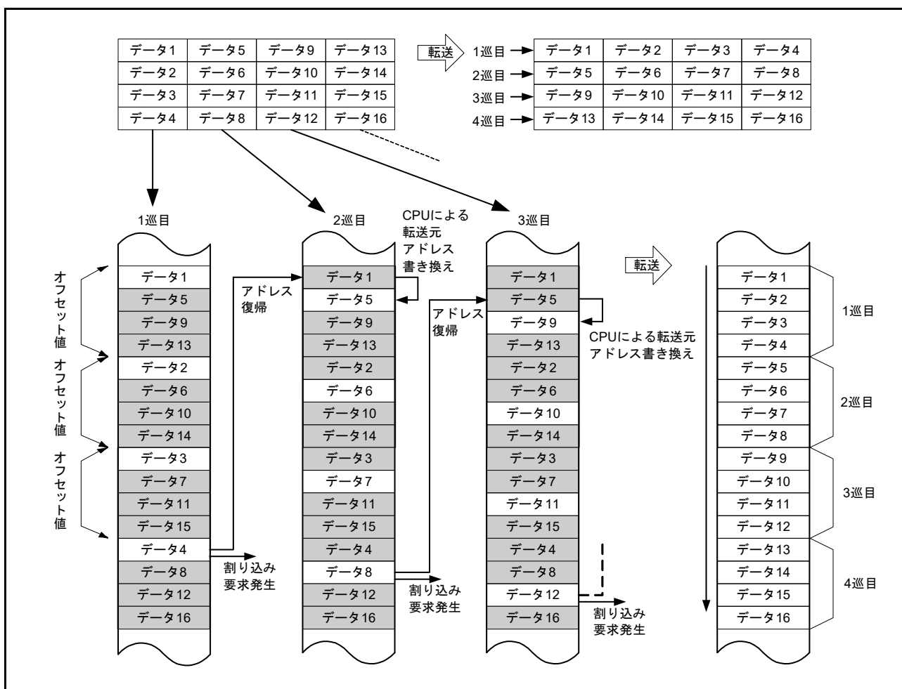
図 18.8 リピータ転送モード + オフセット加算による XY 変換のときの動作
