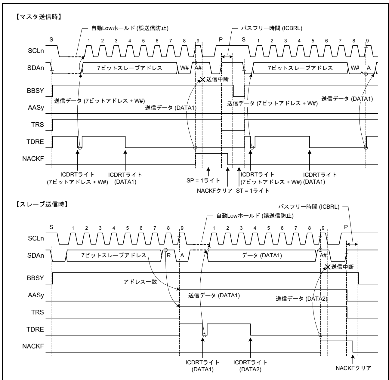
図 41.30 NACK 受信時の転送中断動作 (NACK ビット = 1 のとき)
