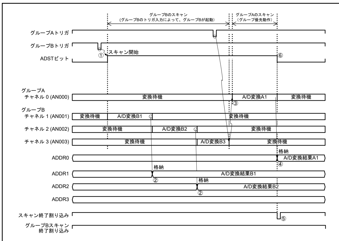
図 54.28 グループ優先動作の例 4 「グループ B スキャン中のグループ A トリガ入力」再スキャンなし (ADGSPCR.GBRSCN = 0, ADGSPCR.GBRP = 0, ADGSPCR.LGRRS = 0 設定時)
