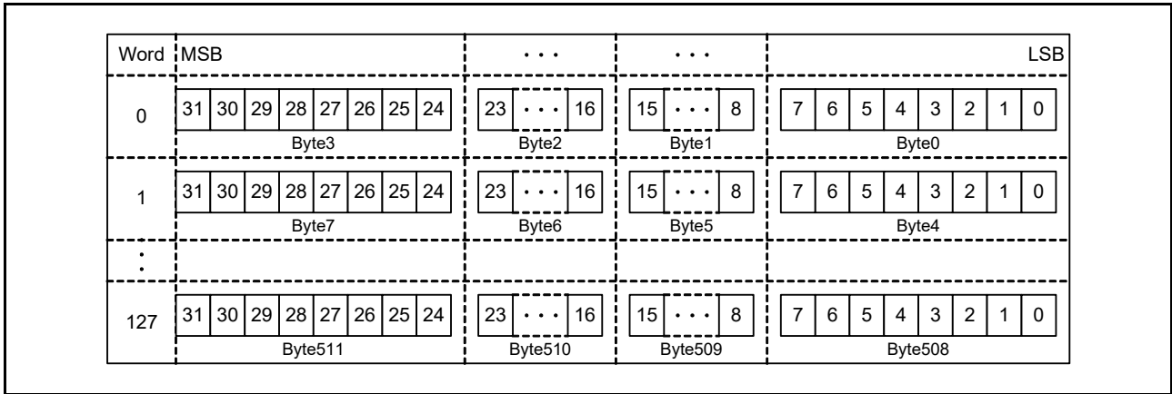
図 47.4 SDバッファのデータ構造 (ダブルバッファのうちのひとつ)
