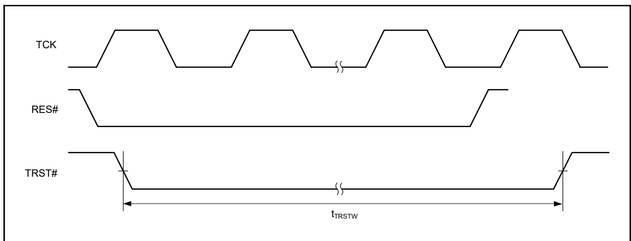
図 61.110 バウンダリスキャン TRST# タイミング
