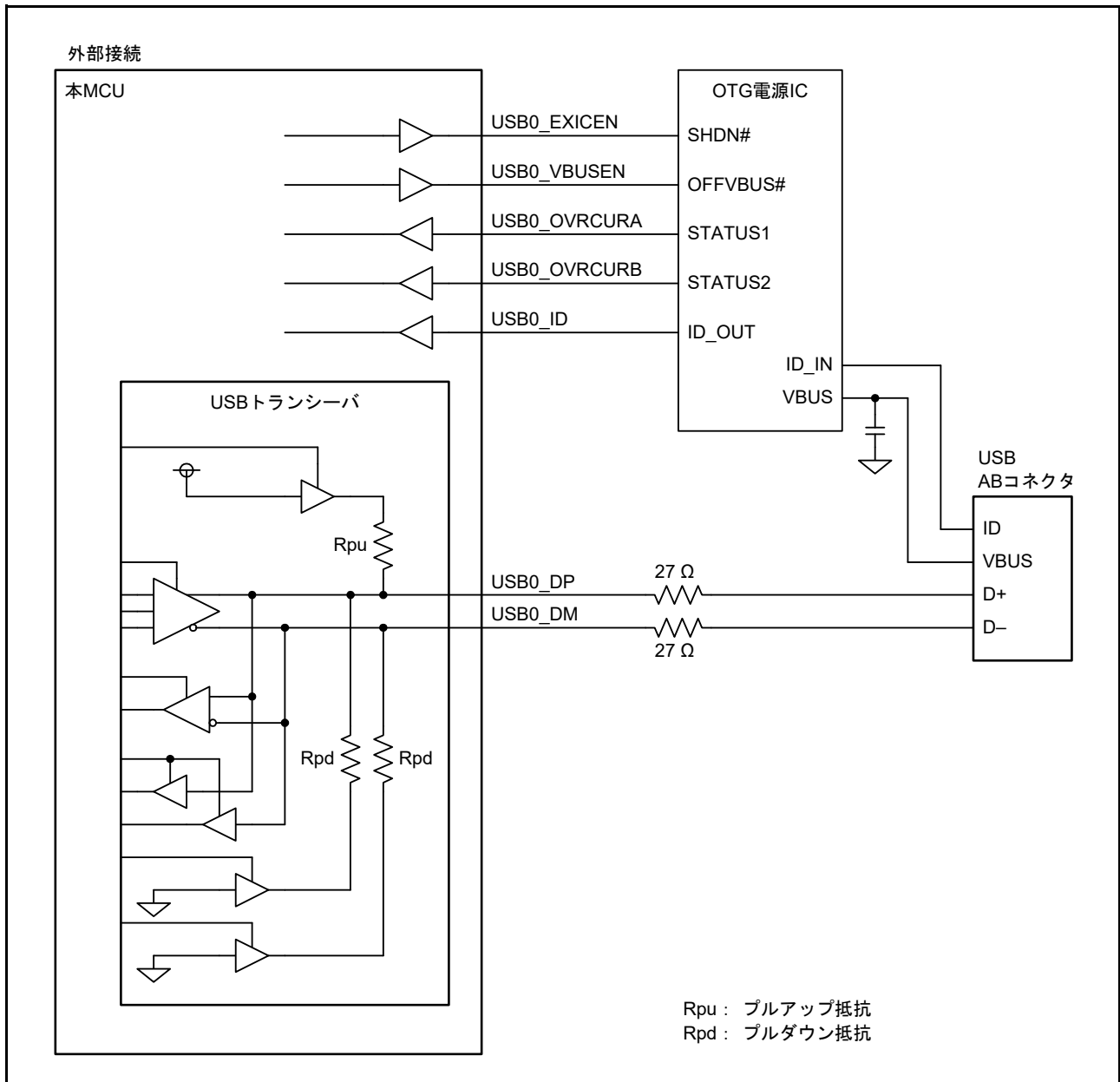
図 39.2 セルフパワー時の OTG デバイスと USB コネクタとの接続例
