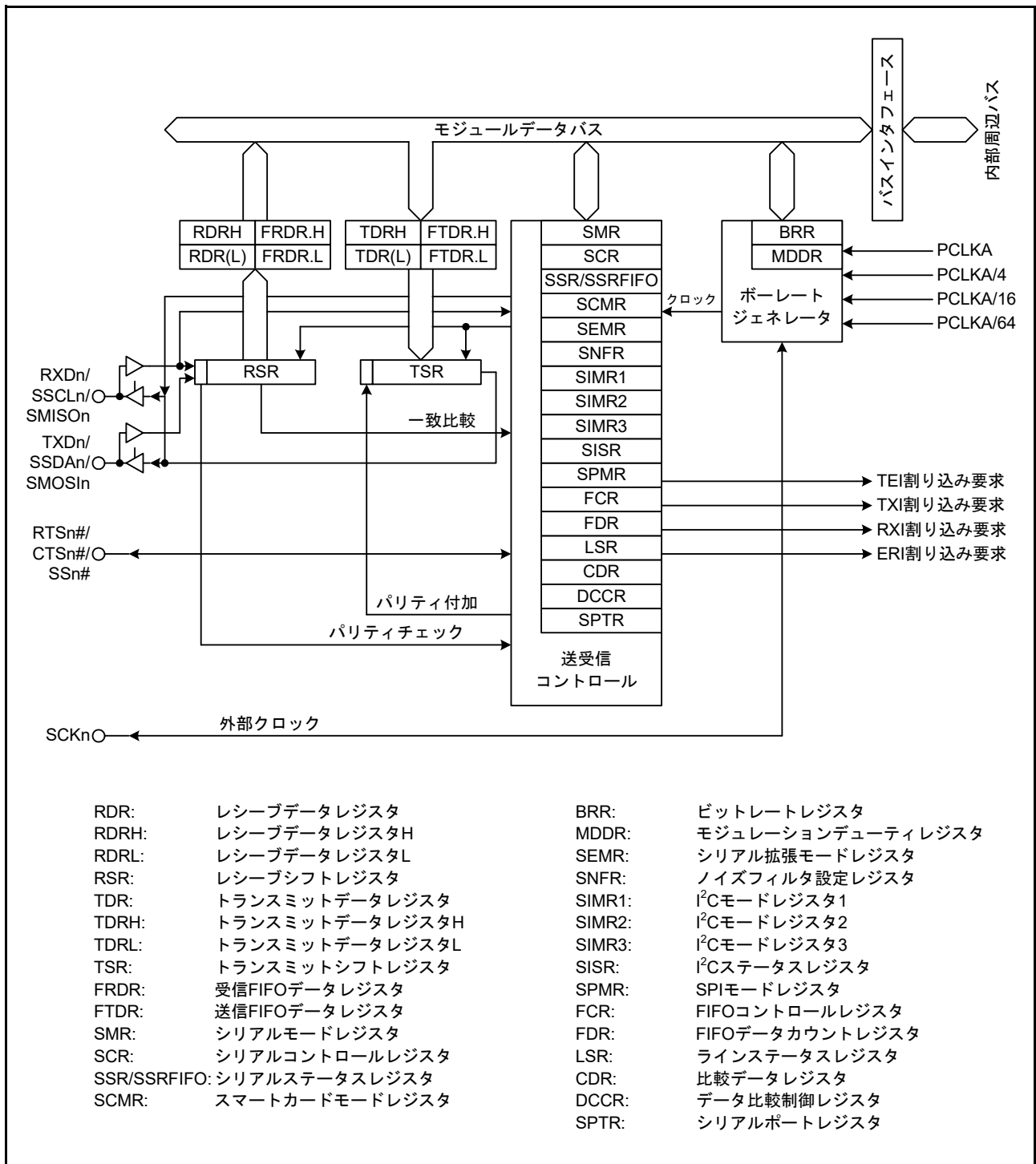
図 40.3 SCli (SCI7 ~ SCI11) のブロック図
