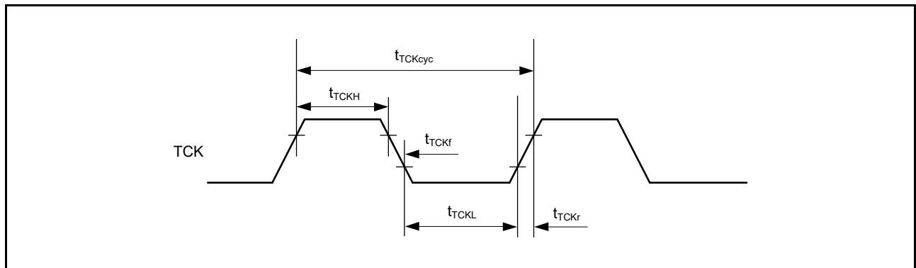
図 61.109 バウンダリスキャン TCK タイミング
