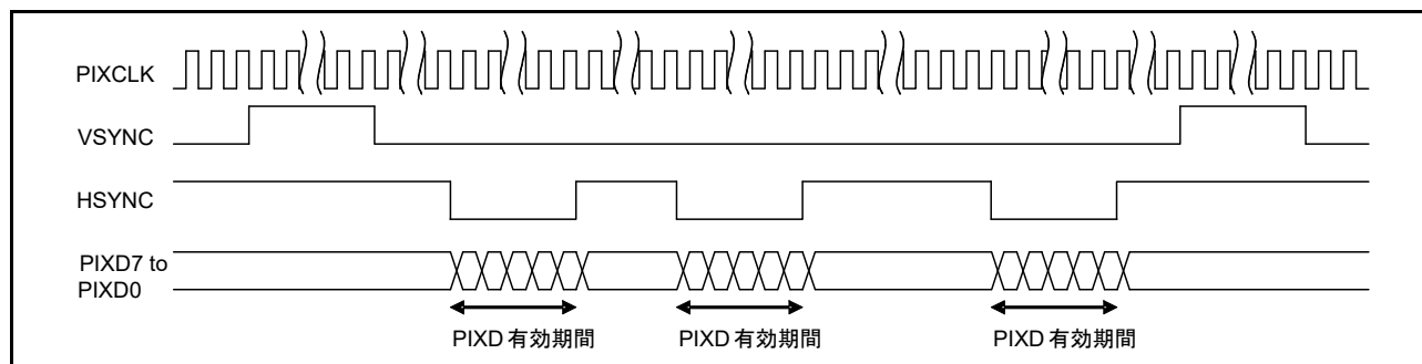
図 49.7 PDC 通信フォーマット (VPS = 1, HPS = 1)
