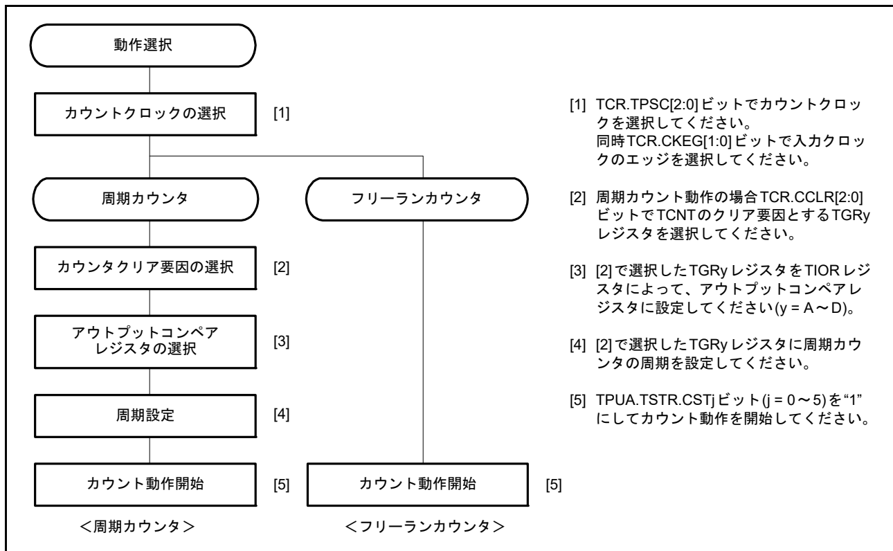
図 28.2 カウント動作設定手順例
