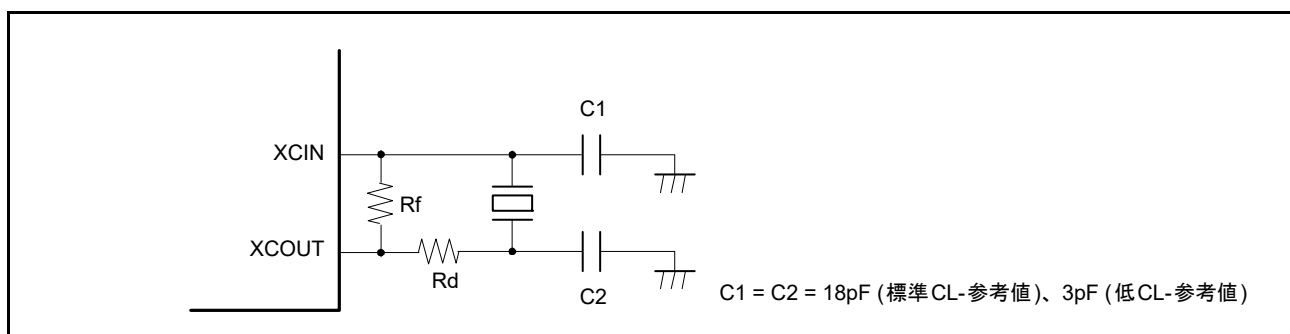
図 9.5 32.768kHz 水晶振動子の接続例
