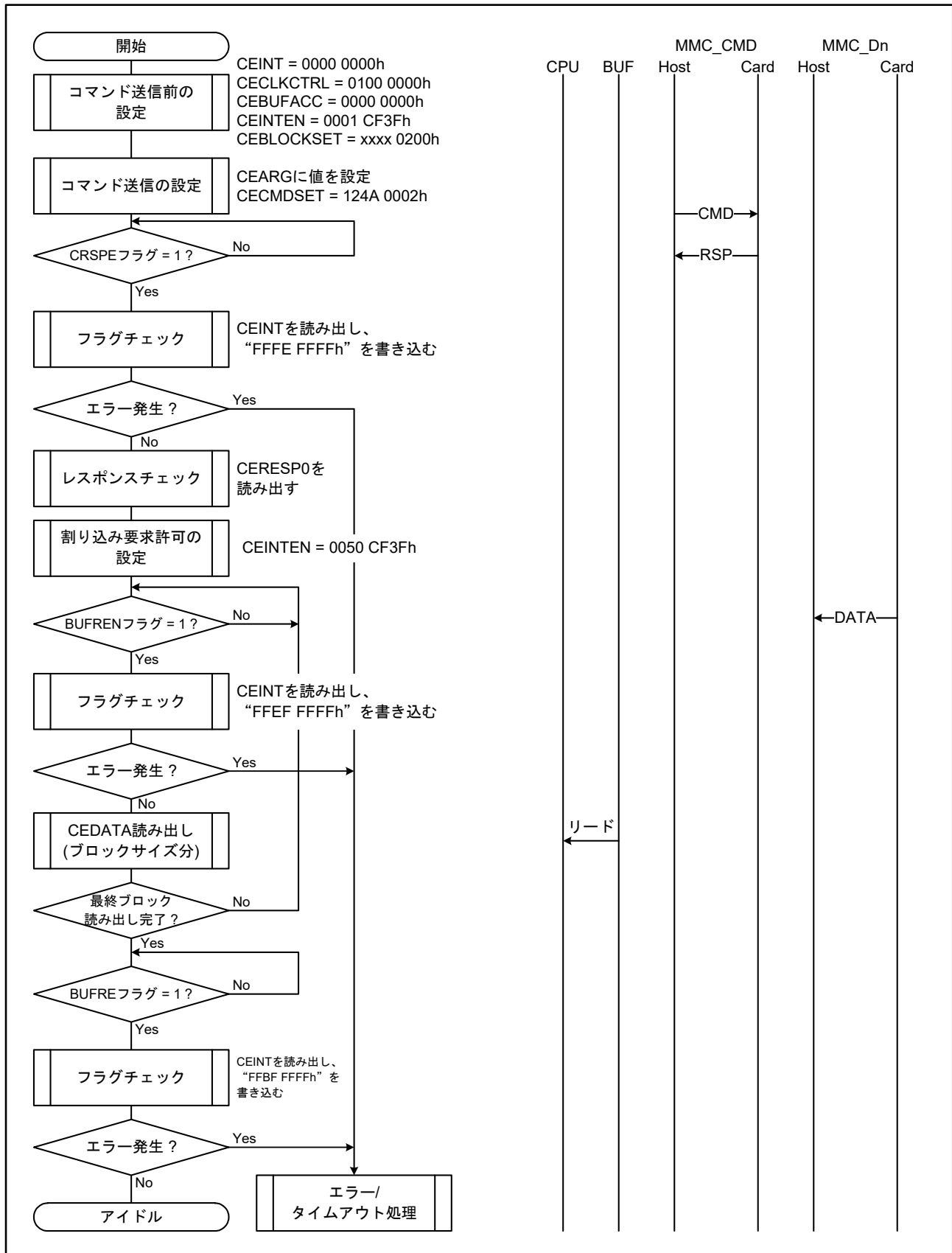
図 48.16 マルチブロックリードコマンドの送信例 (CMD18 Pre-defined)
