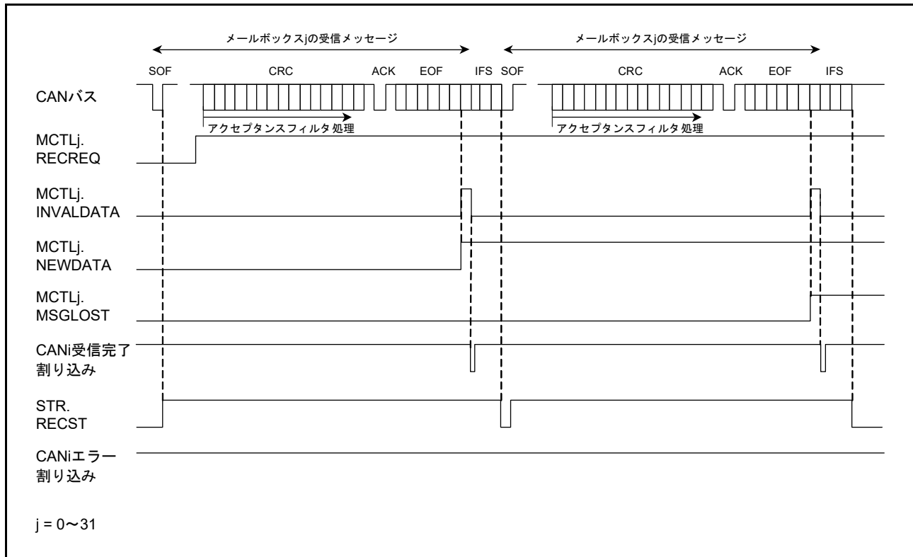
図 42.18 データフレーム受信時の動作例（オーバーライトモードの場合）
