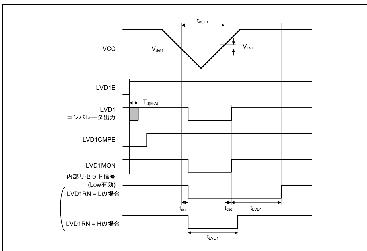
図 61.104 電圧検出回路タイミング (V det1 )
