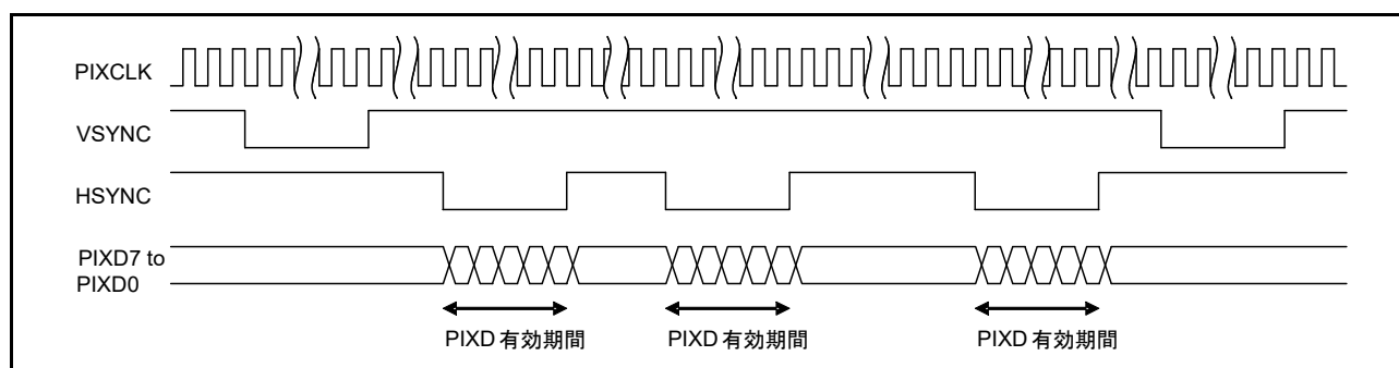
図 49.6 PDC 通信フォーマット (VPS = 0, HPS = 1)
