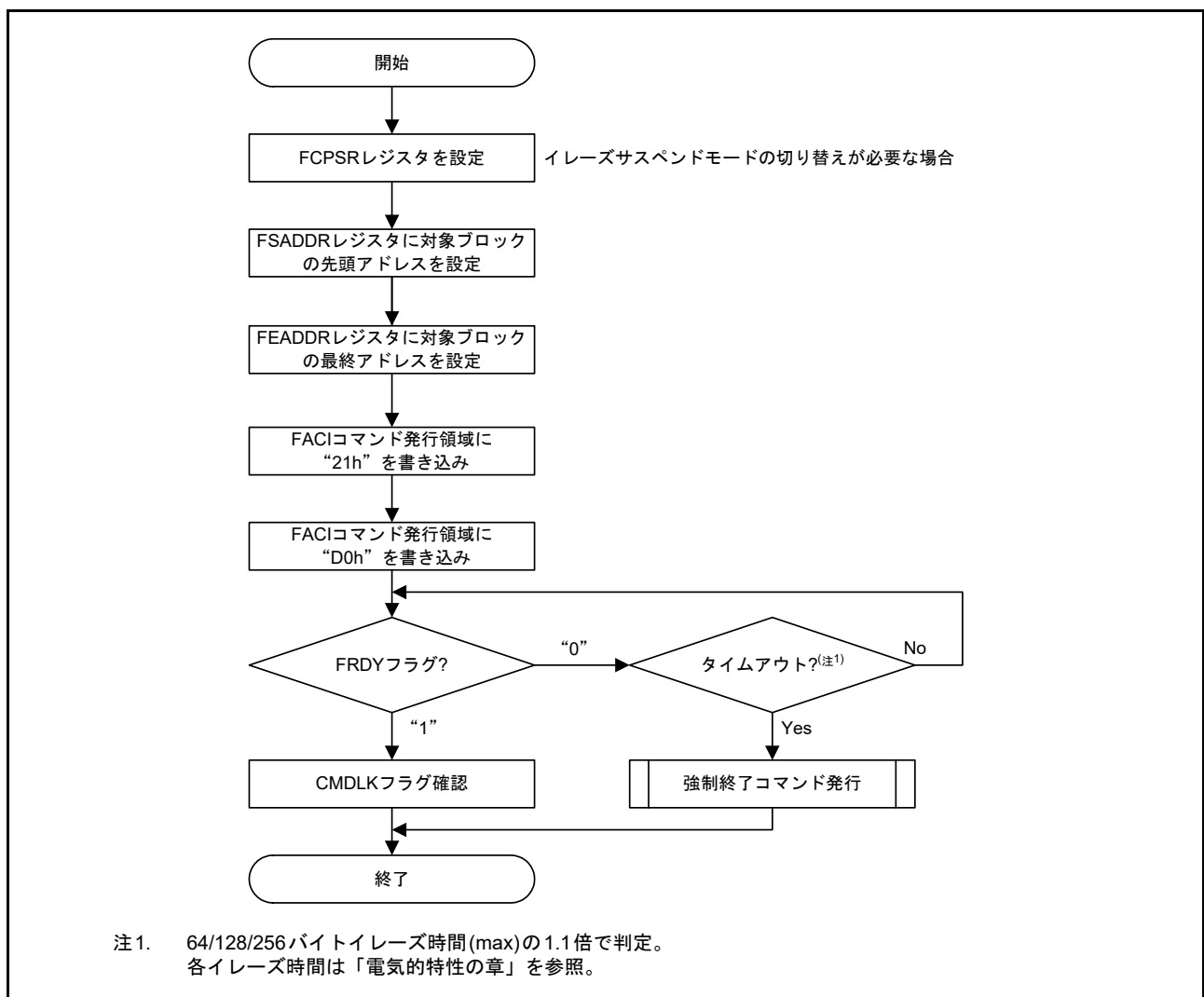
図 60.16 マルチブロックイレーズコマンドの使用法
