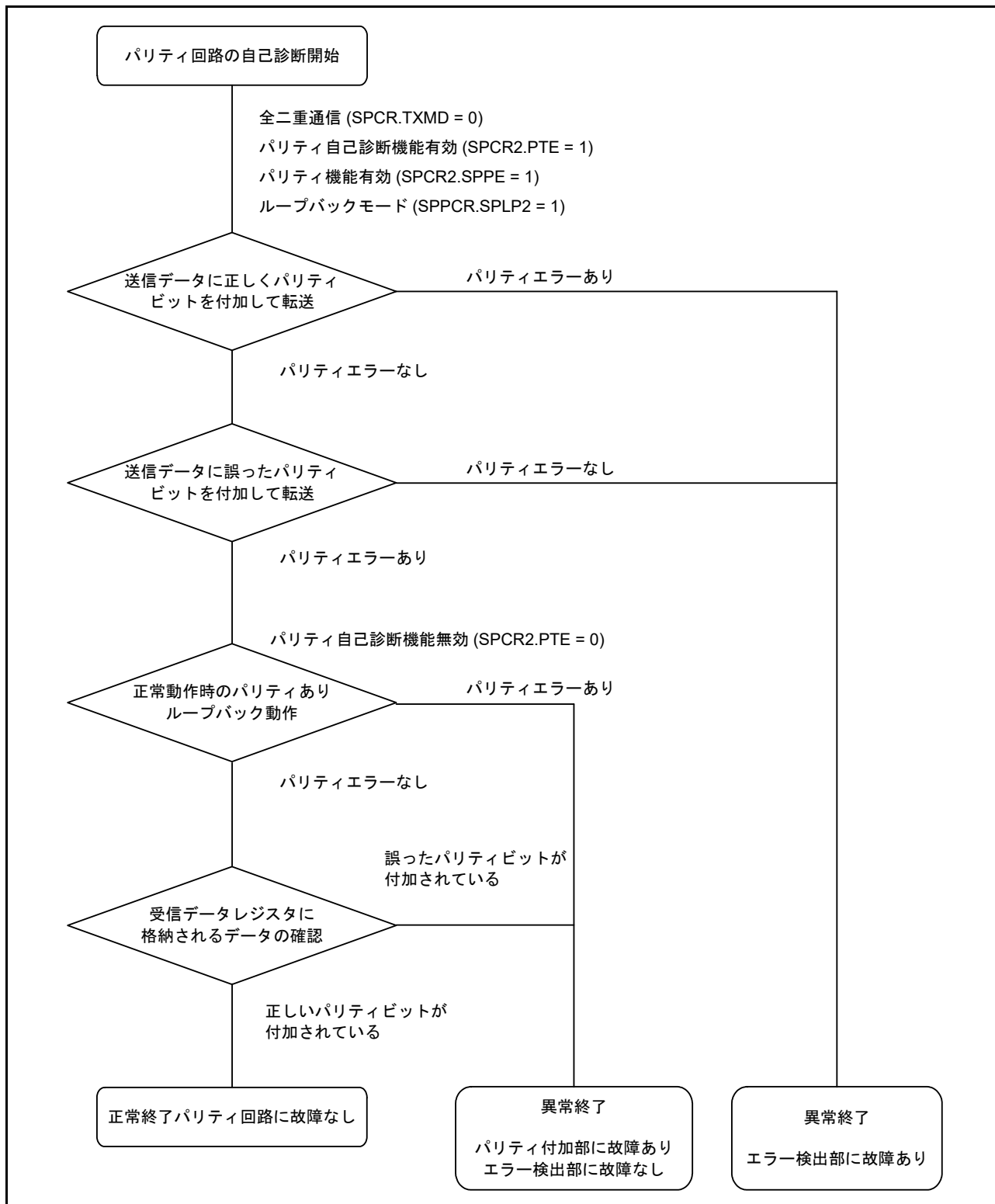
図 43.51 パリティ回路の自己判断フロー
