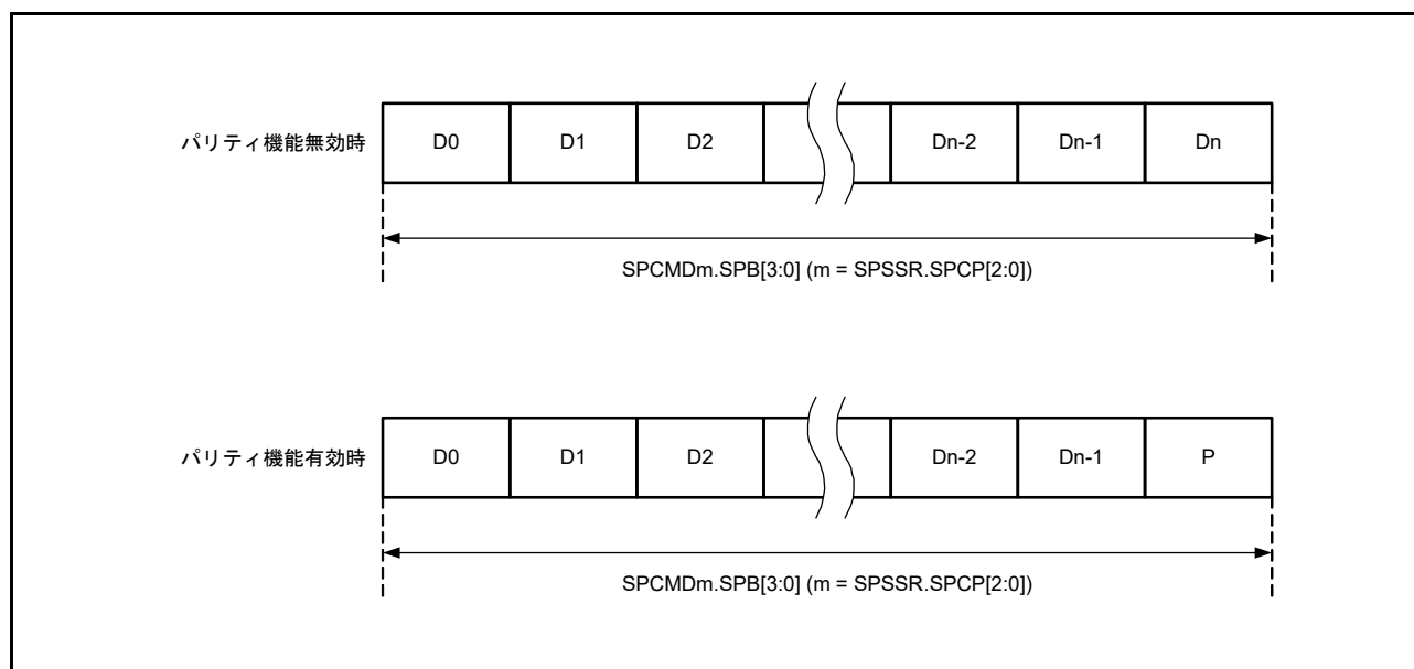
図 43.13 データフォーマット概要 (パリティ機能無効時 / 有効時)
