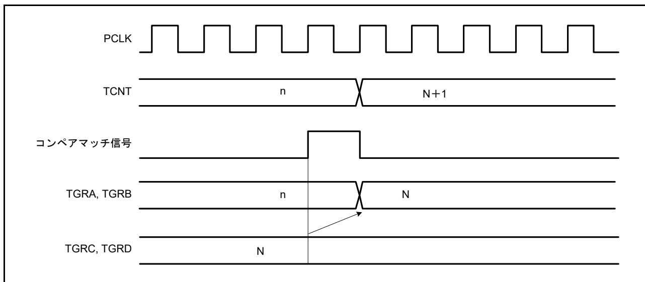
図 28.37 バッファ動作タイミング (コンペアマッチ)
