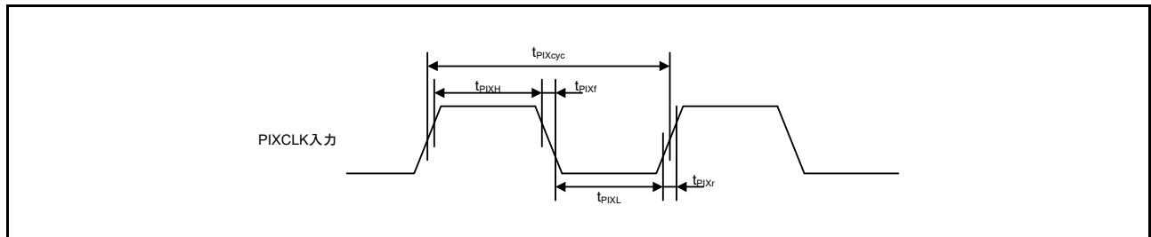
図 61.91 PDC 入力クロックタイミング
