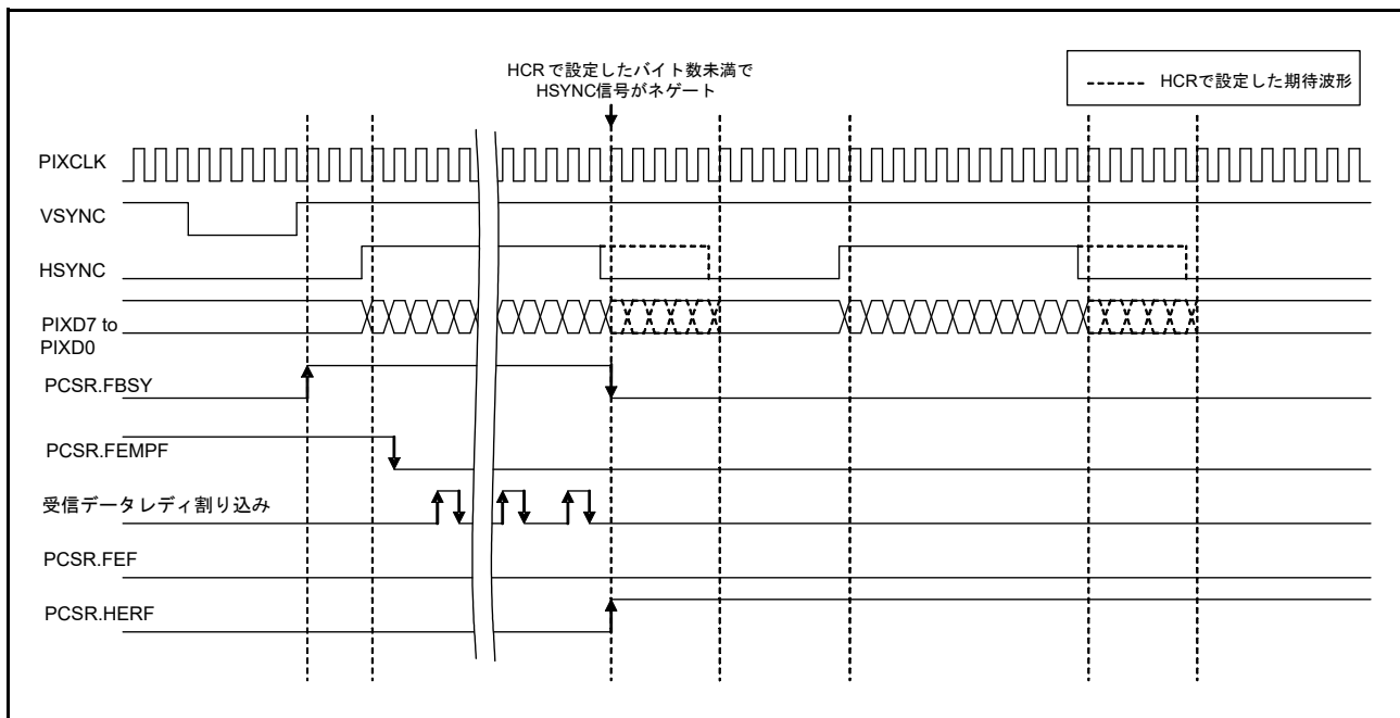
図 49.17 水平方向バイト数設定エラー検出
