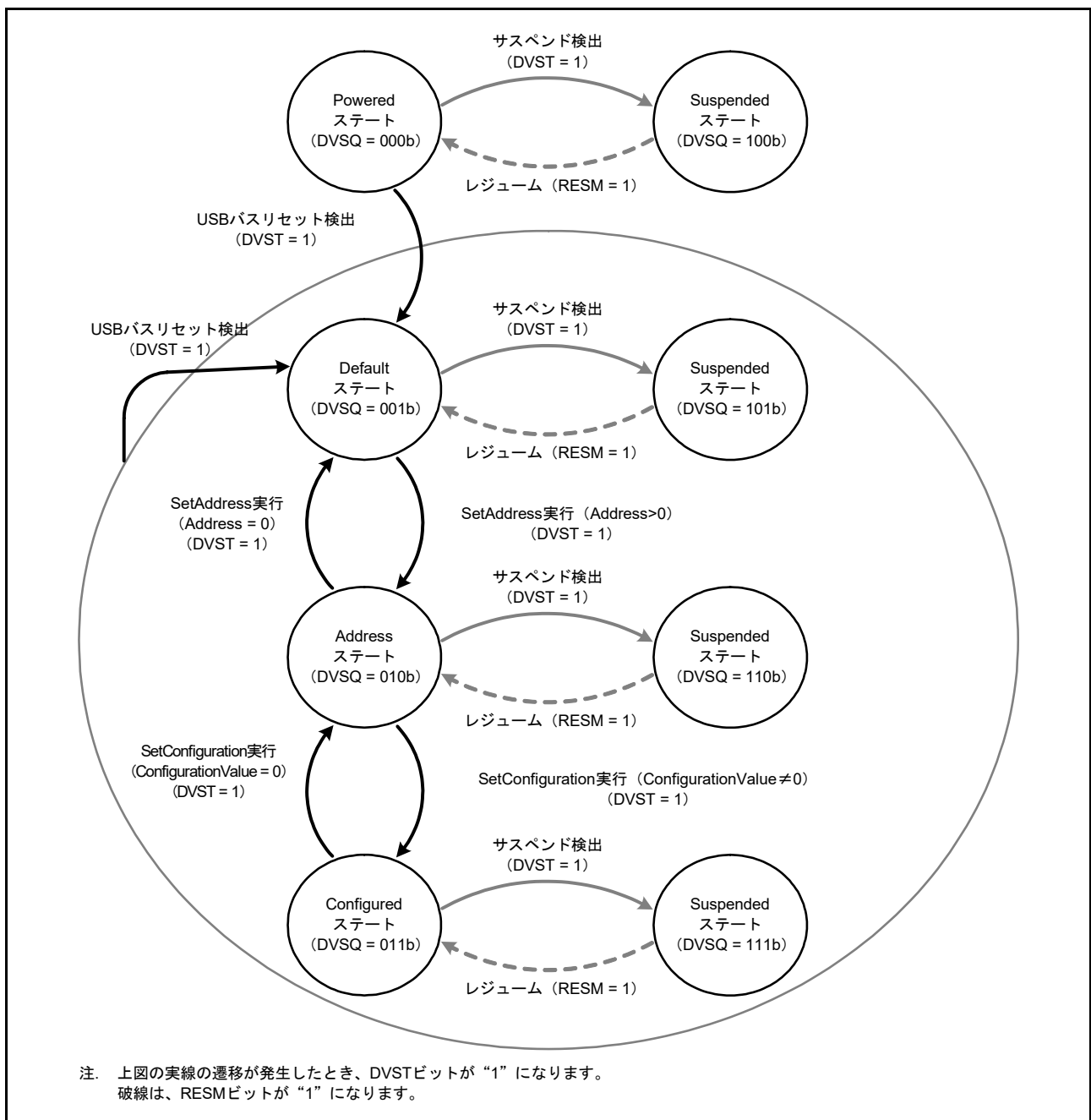
図 39.14 デバイスステート遷移図
