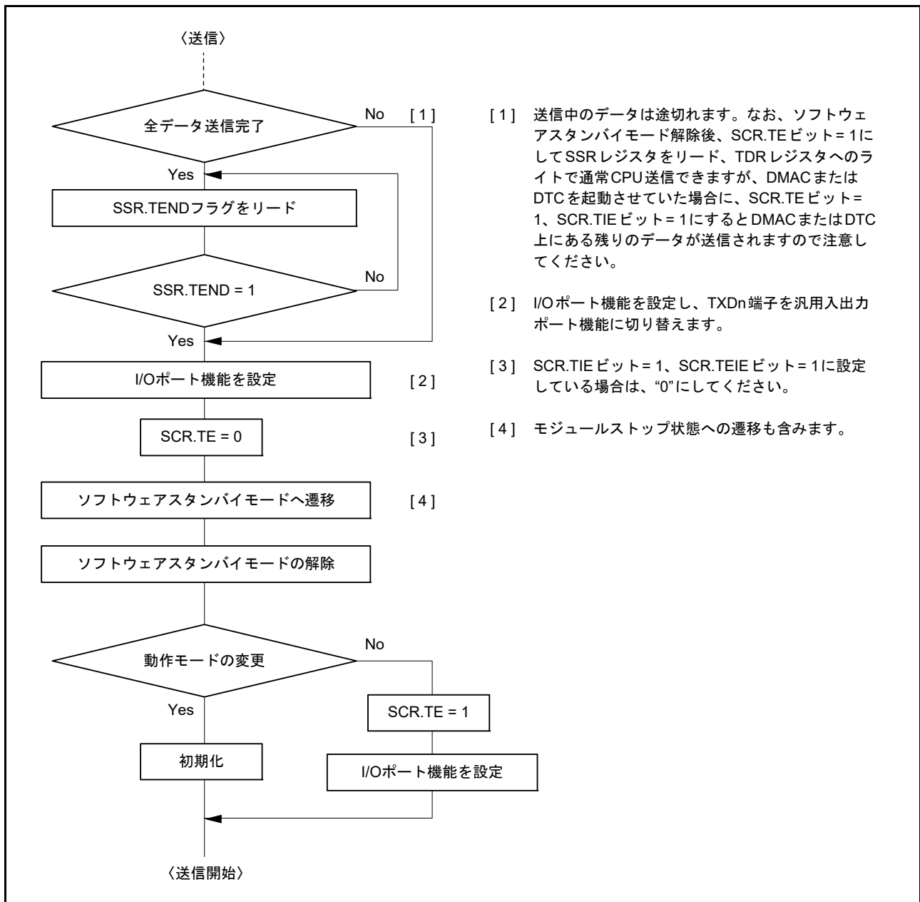
図 40.81 送信時のソフトウェアスタンバイモード遷移フローチャートの例
