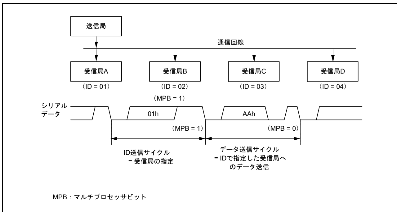
図 40.22 マルチプロセッサフォーマットを使用した通信例 (受信局 A へのデータ “AAh” の送信の例)
