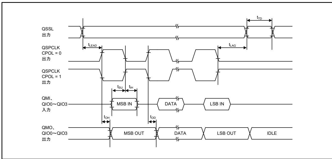
図 61.72 送受信タイミング (CPHA = 1)
