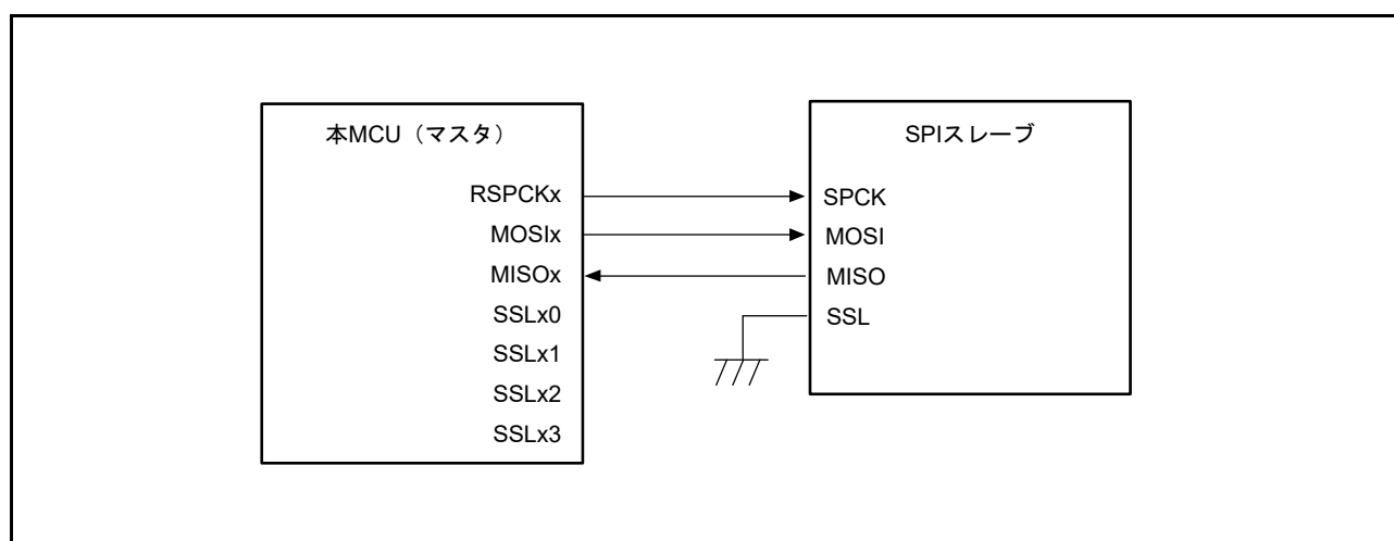
図 43.5 シングルマスタ / シングルスレーブの構成例 (本 MCU = マスタ)
