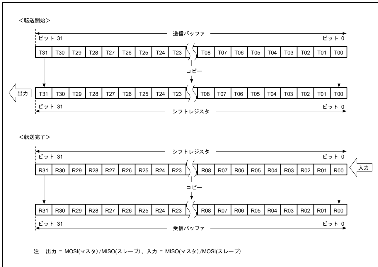
図 43.14 MSB ファースト転送 (32 ビットデータ / パリティ機能無効)
