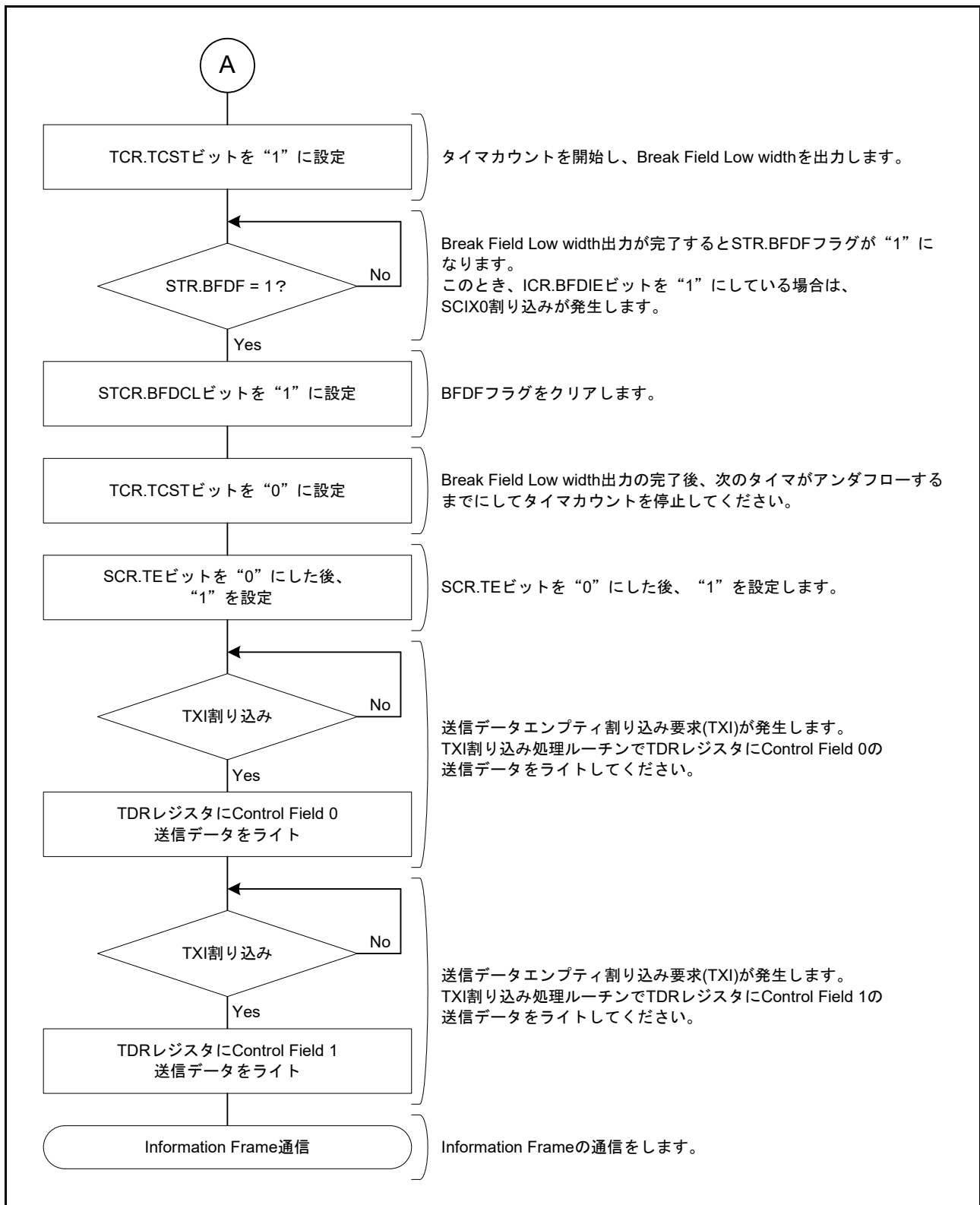
図 40.67 Start Frame 送信フローチャート例 (2)
