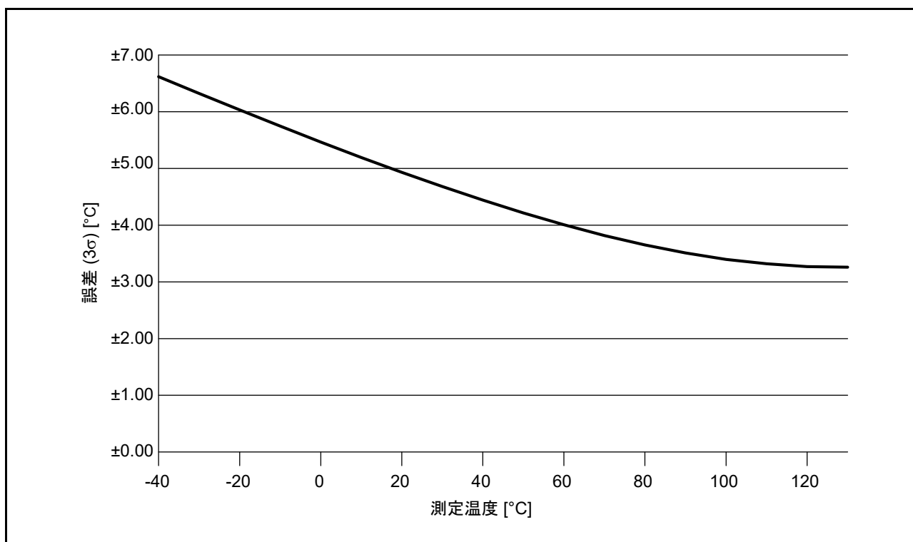
図 56.2 製品の測定温度誤差
