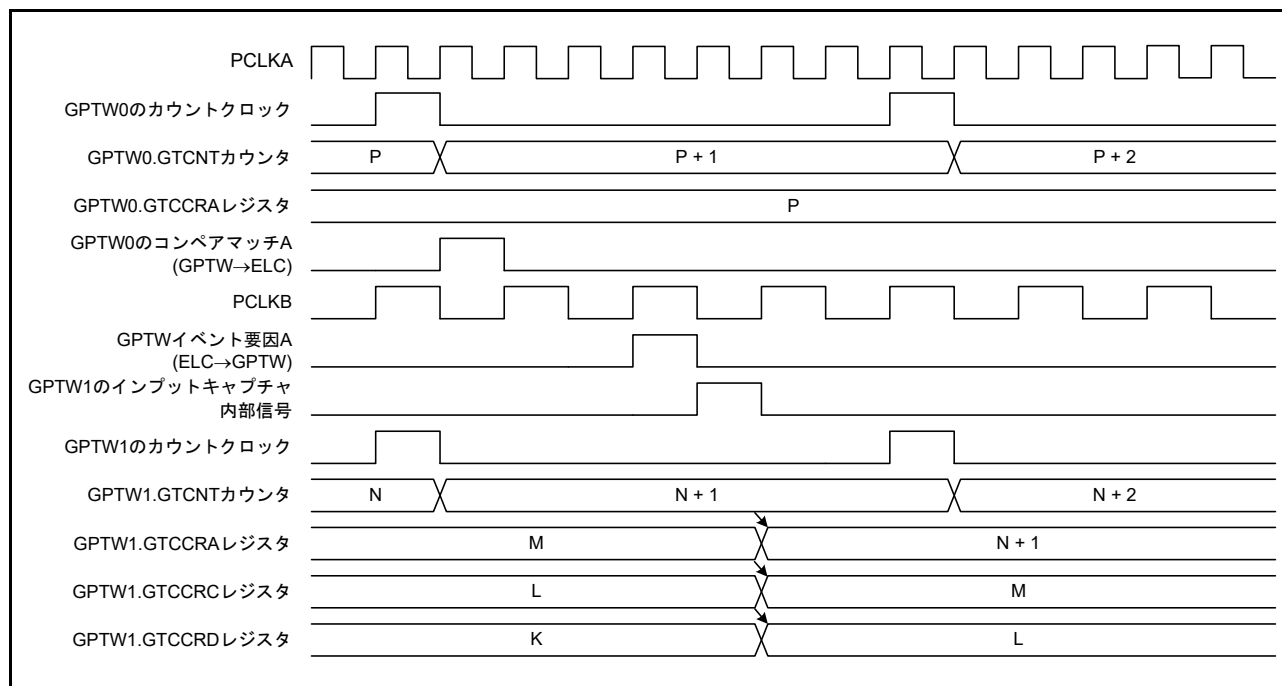
図 26.21 ELCA イベント入力によるインプットキャプチャ動作タイミング例
