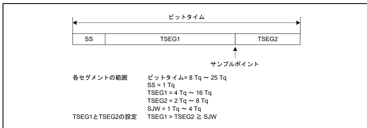
図 42.12 ビットタイミング図
