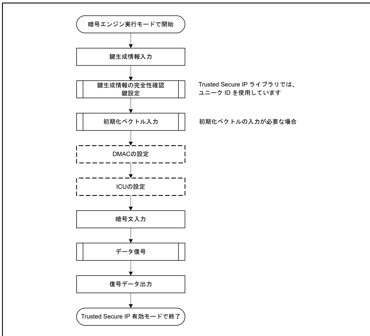
図 53.8 復号フロー
