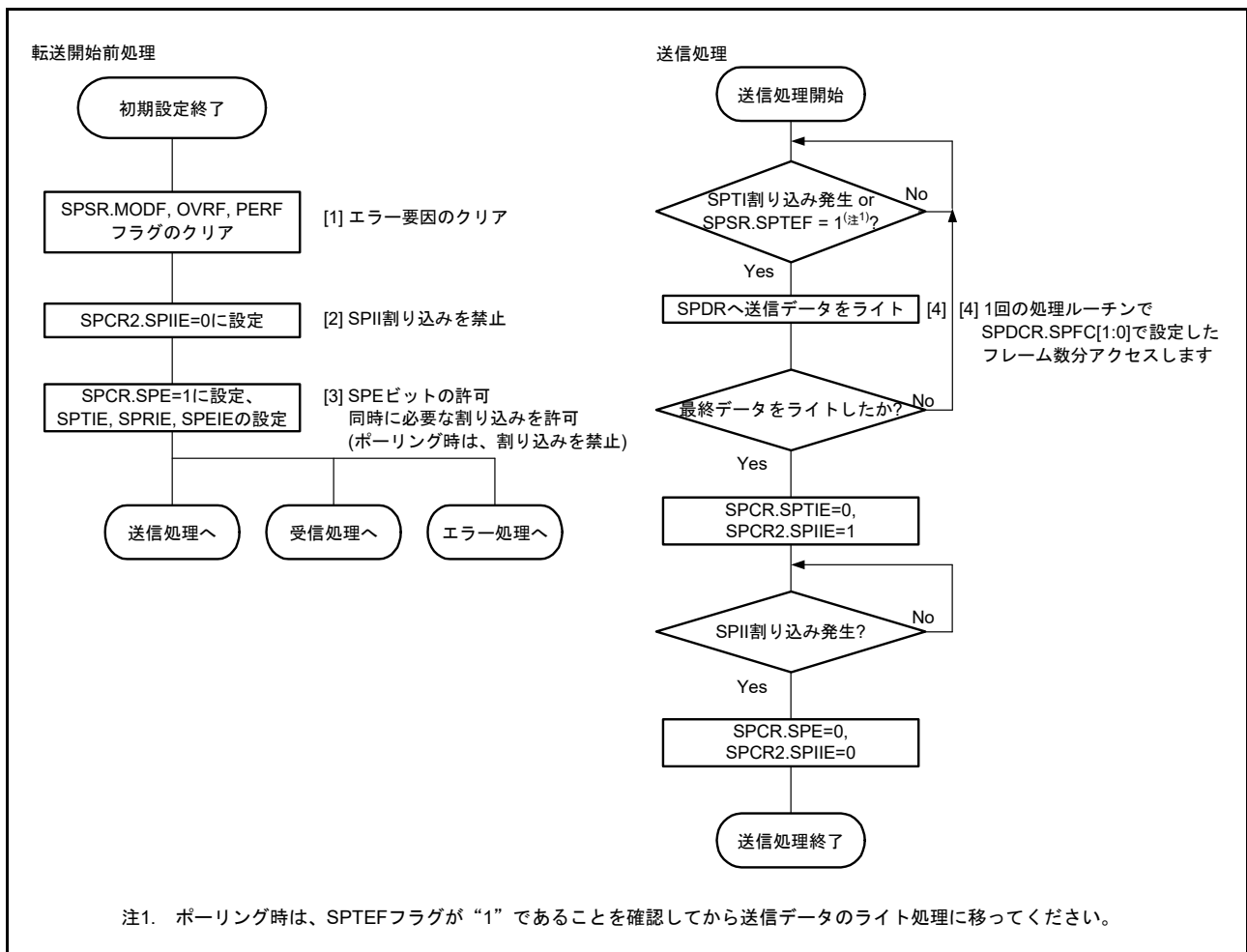
図 43.38 マスタモード時のフローチャート (送信)
