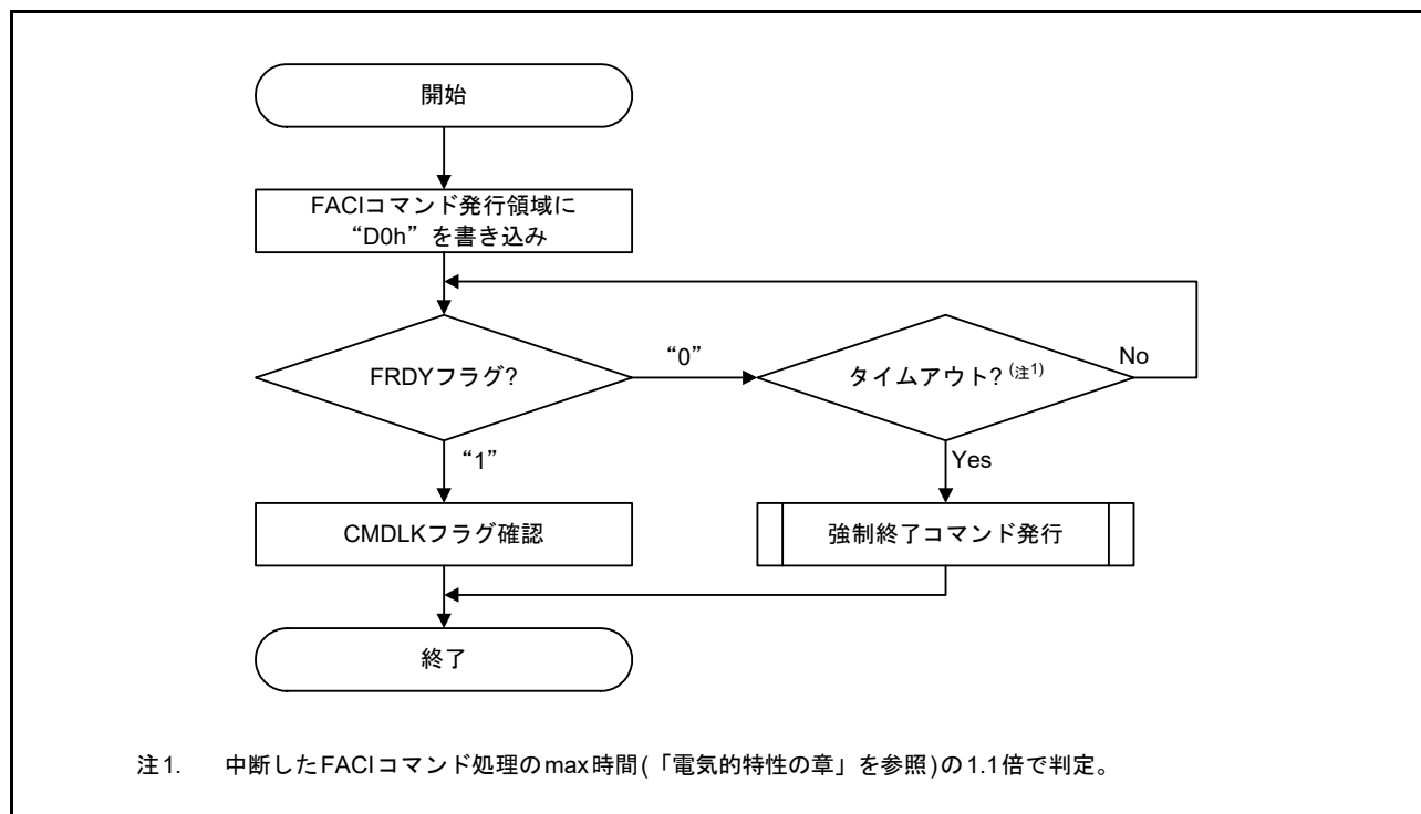
図 60.21 P/E レジュームコマンドの使用方法
