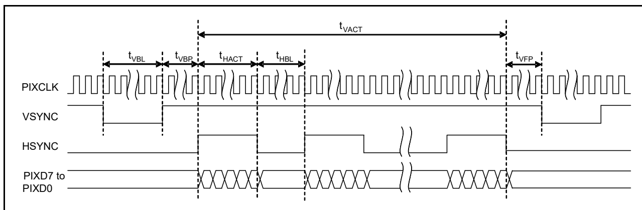
図49.8 PDCの通信タイミング図
