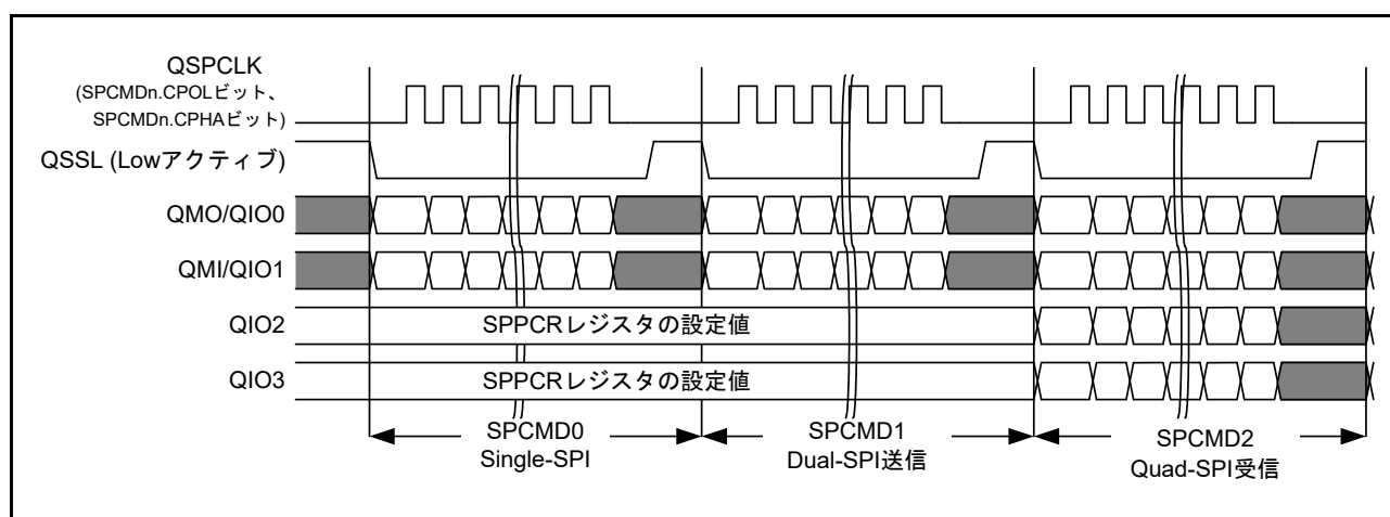
図 44.18 転送モードを切り替えたシーケンス構成の例 ( n=0\sim 3 )
