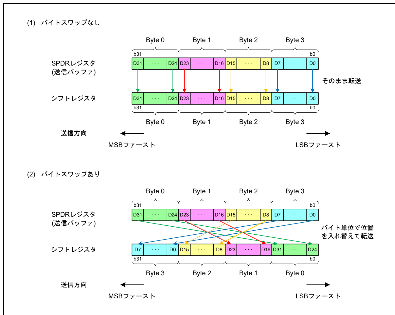
図 43.22 MSB/LSB ファーストとバイトスワップあり/なしの設定と送信データ変換
