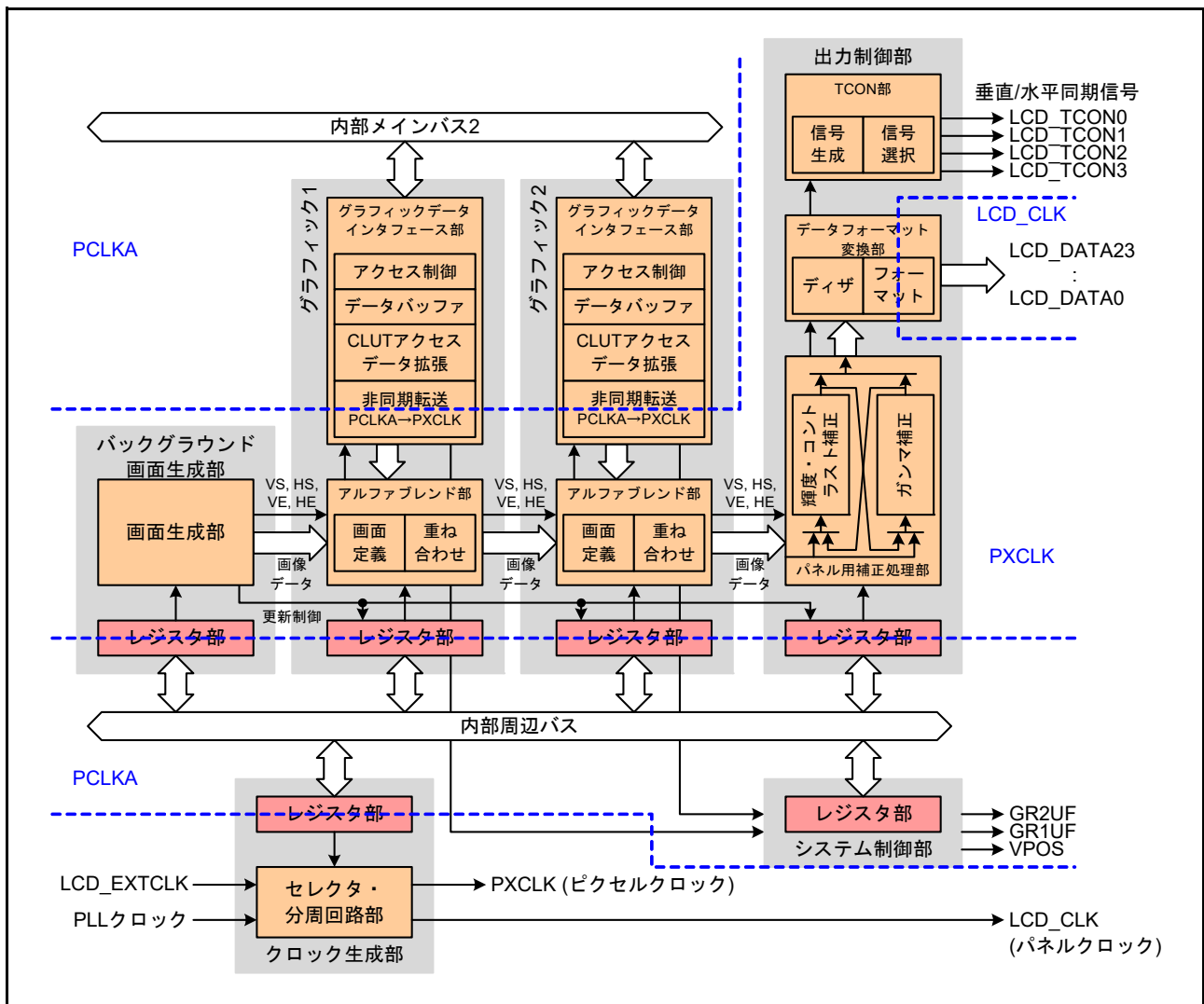
図 50.2 GLCDC の構成
