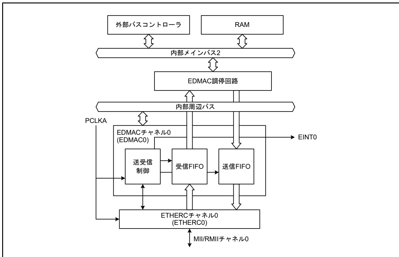
図 37.1 EDMAC の構成
