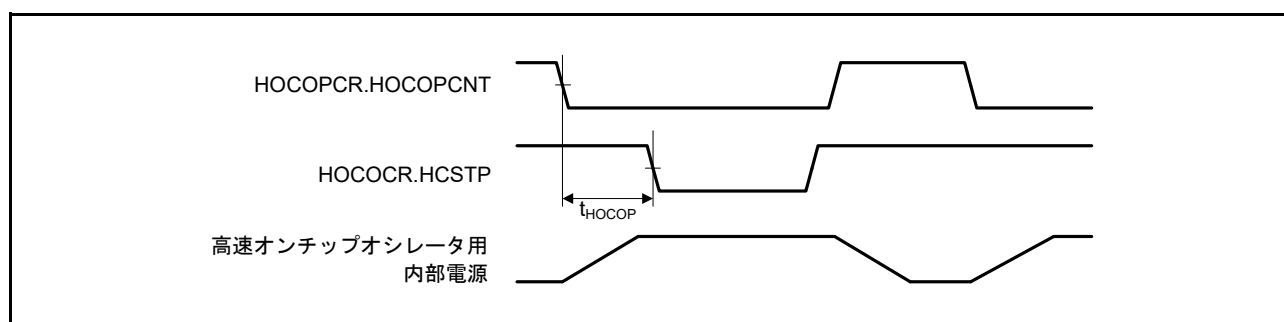
図 61.9 高速オンチップオシレータ電源制御タイミング
