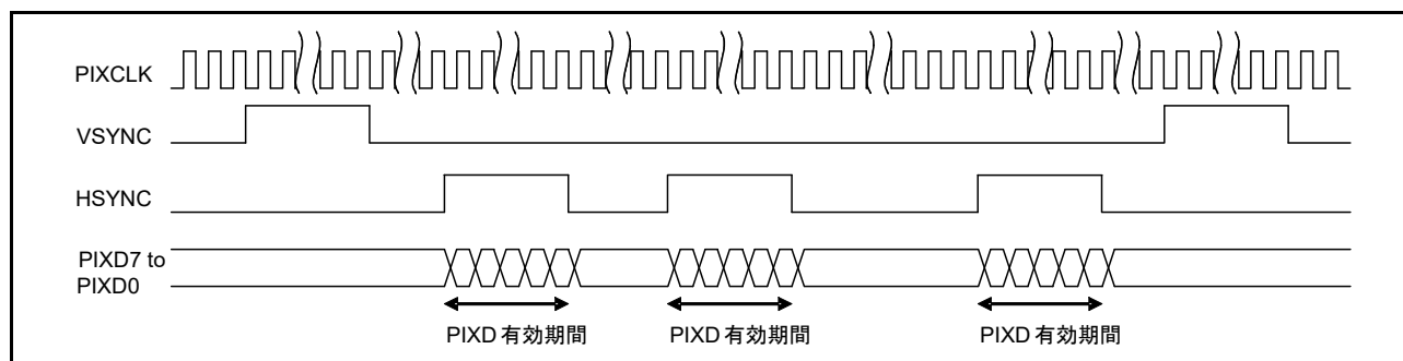
図 49.5 PDC 通信フォーマット (VPS = 1, HPS = 0)
