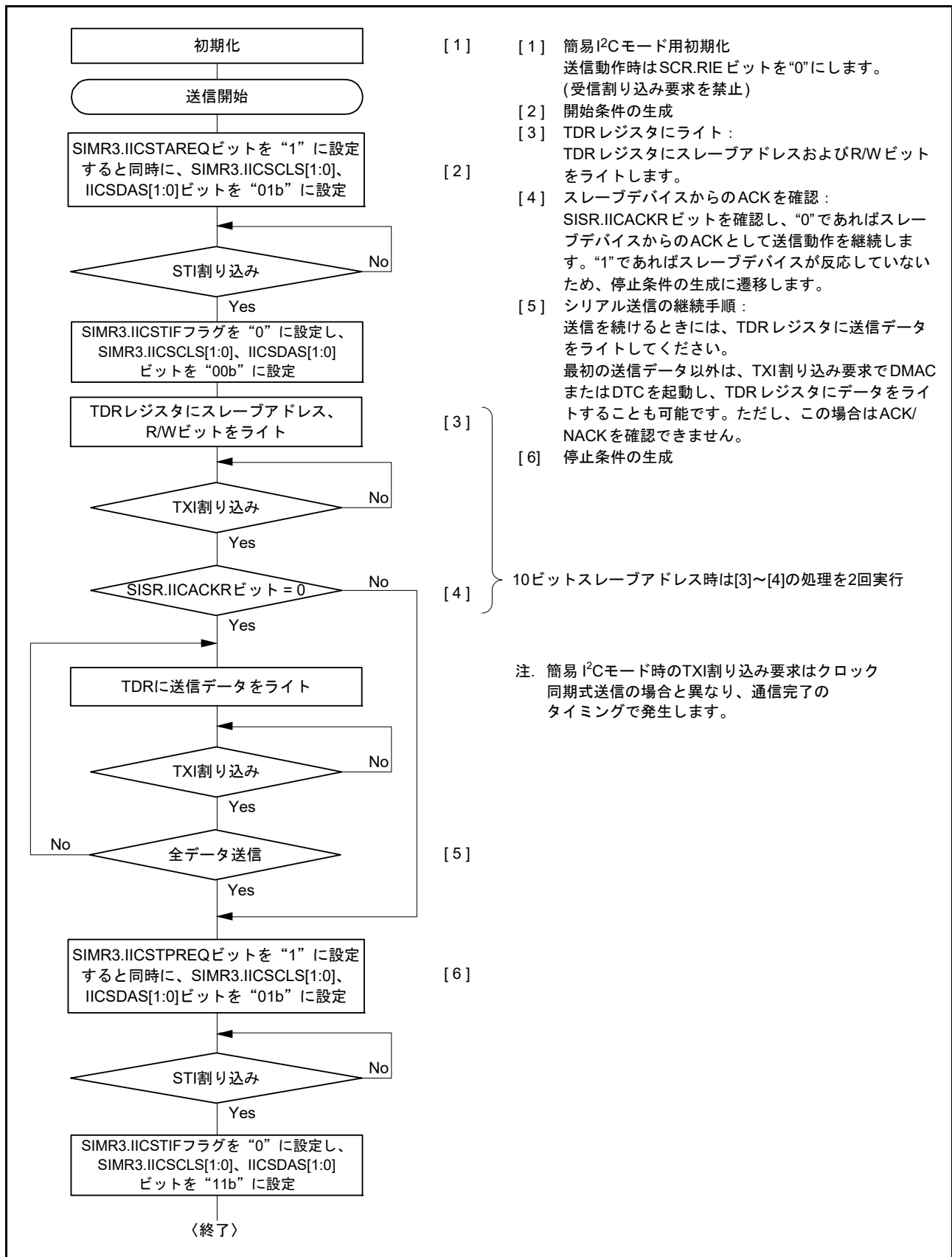
図 40.58 簡易 I 2 C モードのマスタ送信動作のフローチャート例 (送信割り込み、受信割り込み使用時)
