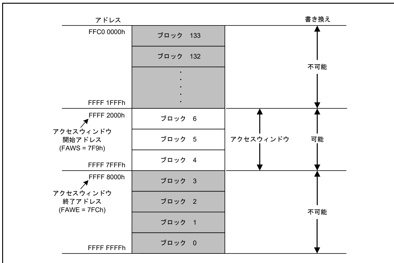
図 60.30 エリアプロテクションの概念 (コードフラッシュメモリ容量が4Mバイトの製品でブロック4からブロック6をアクセスウィンドウに設定した場合の例)
