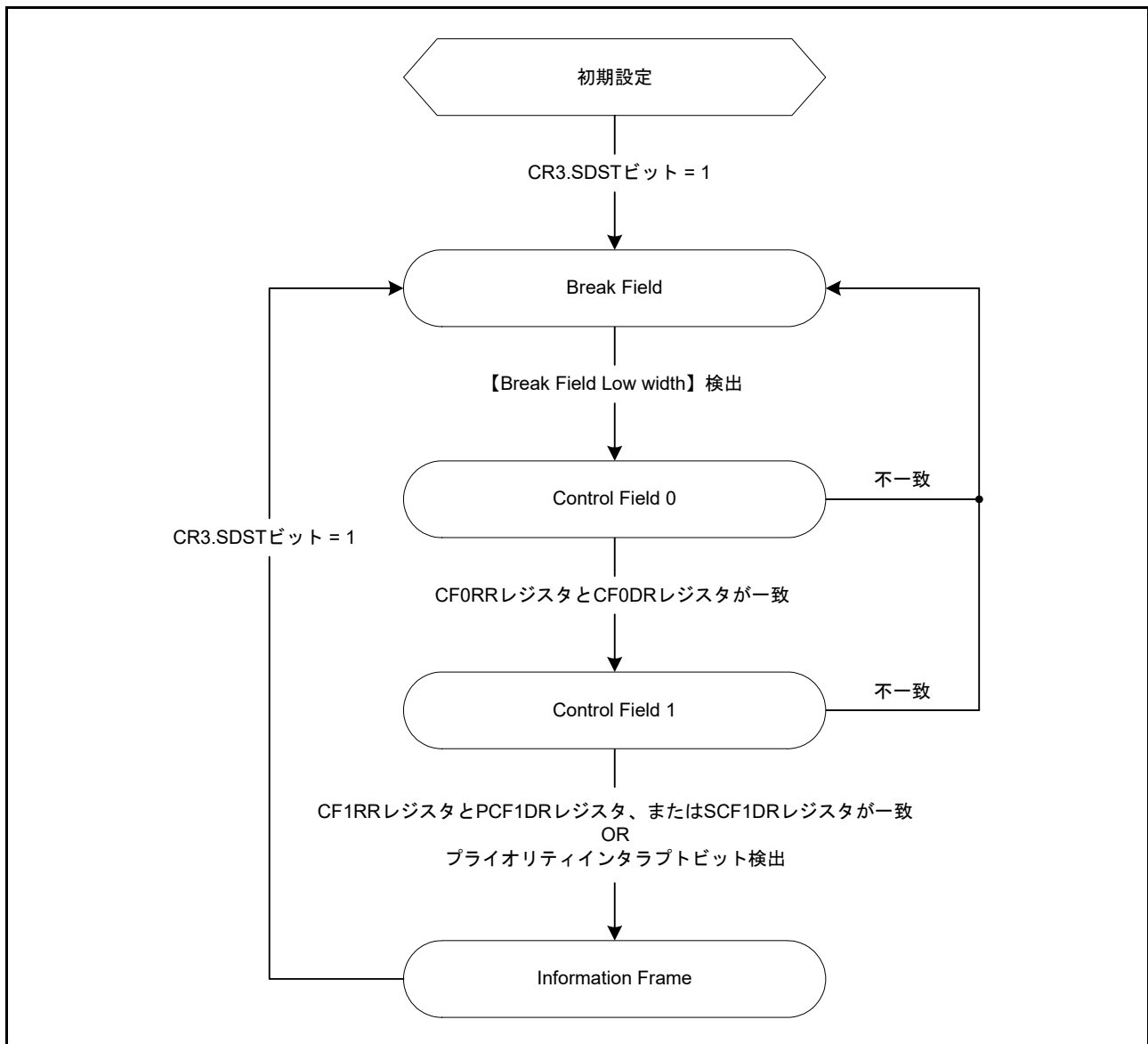
図 40.71 Start Frame 受信時の状態遷移図
