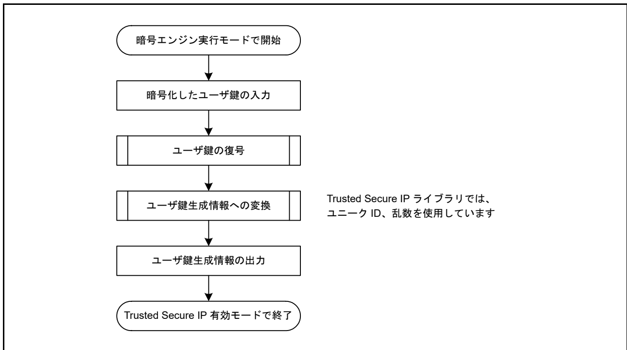
図 53.5 鍵インストールフロー
