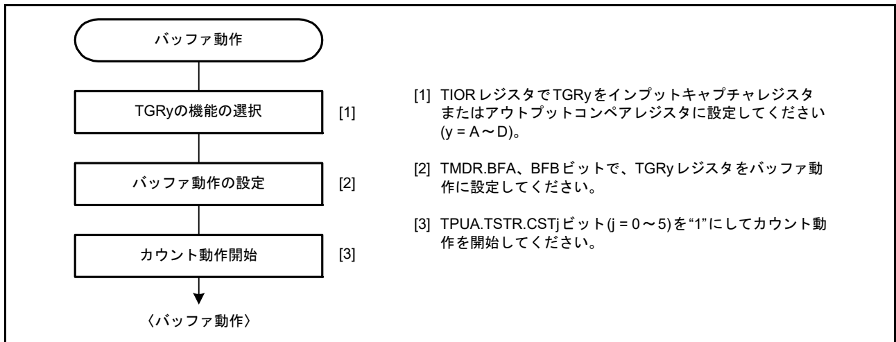
図 28.14 バッファ動作の設定手順例
