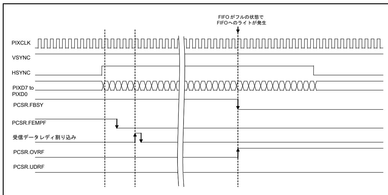
図 49.14 オーバラン
