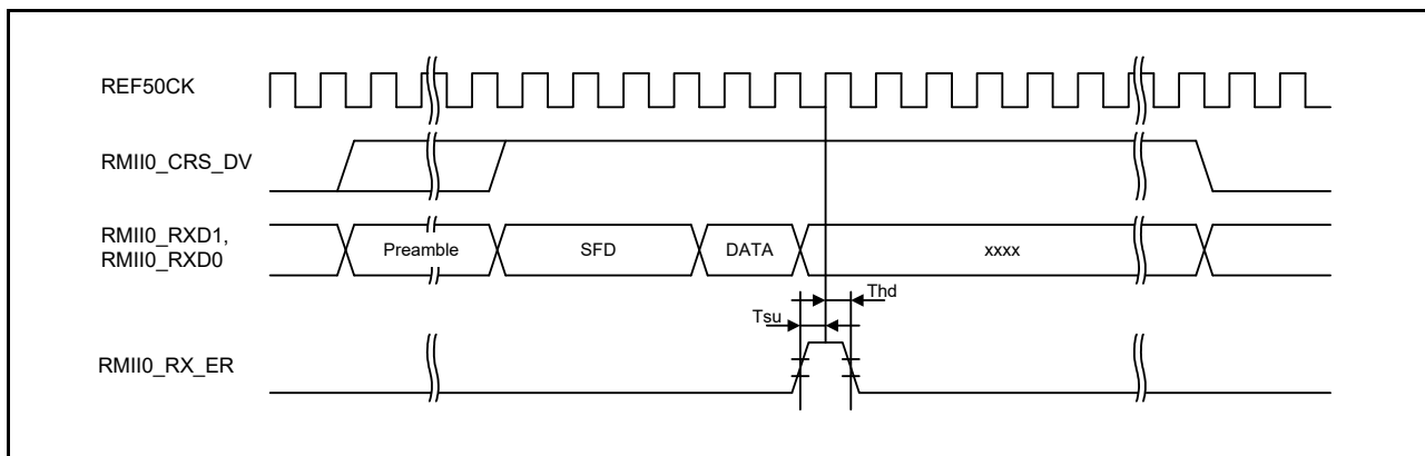
図 61.84 RMIIC 受信タイミング (エラー発生ケース)
