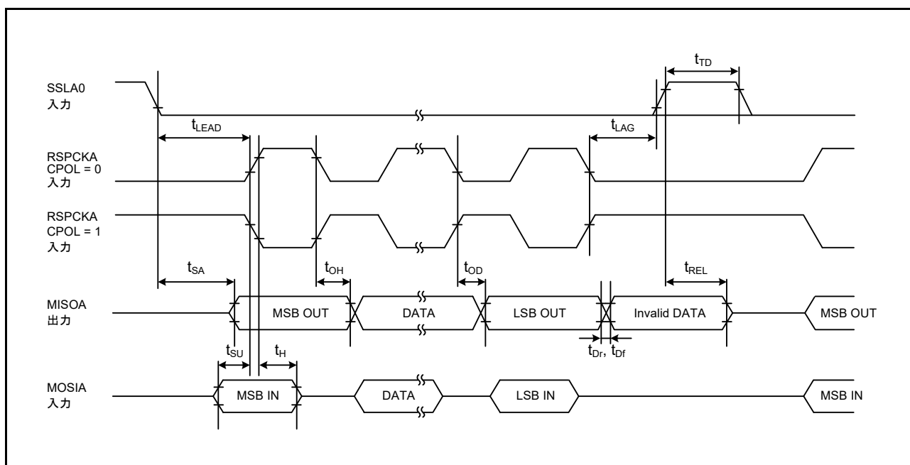
図 61.68 RSPi タイミング (スレーブ、CPHA = 0)
