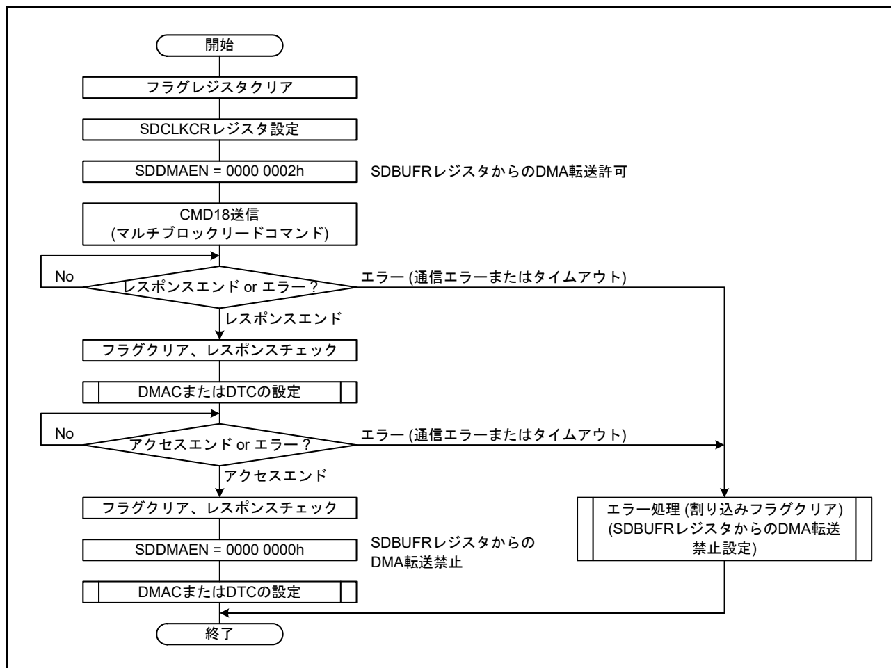
図 47.21 マルチブロックリードコマンド (CMD18) を送信した後、DMA 転送で SDBUFR レジスタから転送する例
