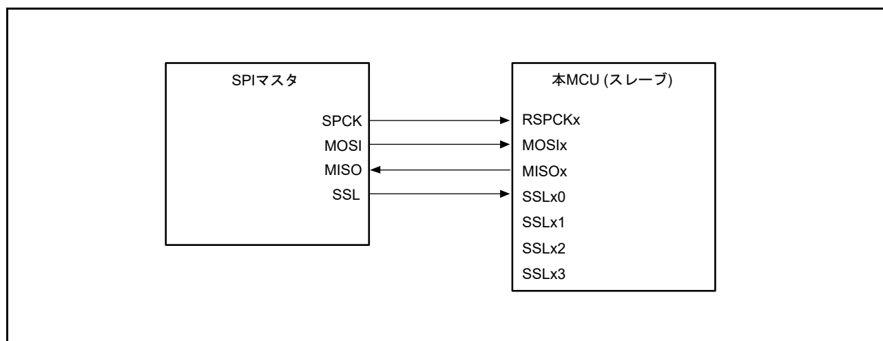
図 43.6 シングルマスタ / シングルスレーブの構成例 (本 MCU = スレーブ、CPHA = 0)
