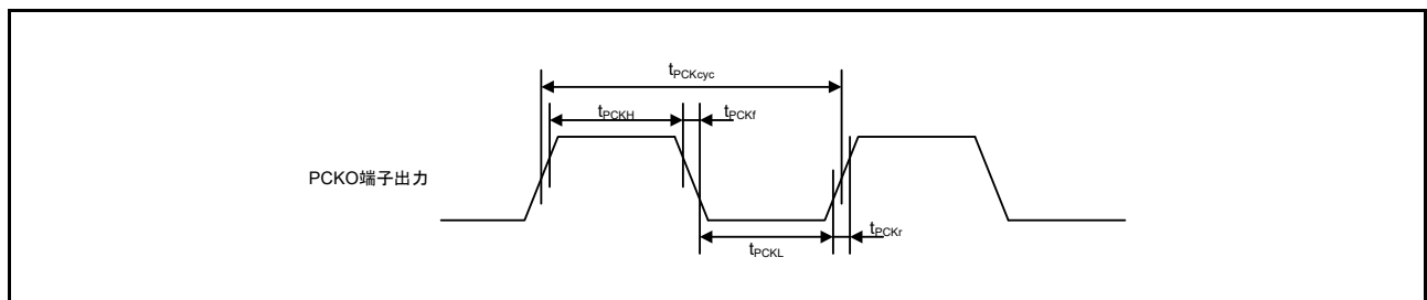
図 61.92 PDC 出力クロックタイミング
