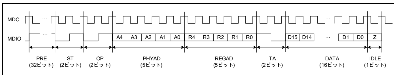
図 38.3 ライトアクセスのデータフォーマット
