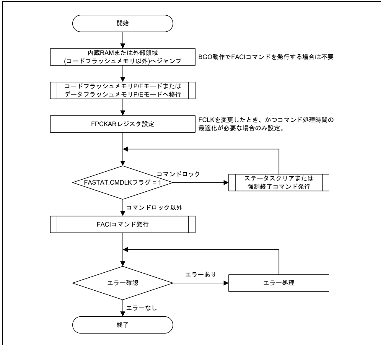
図 60.12 FACI コマンド使用時の概略フロー
