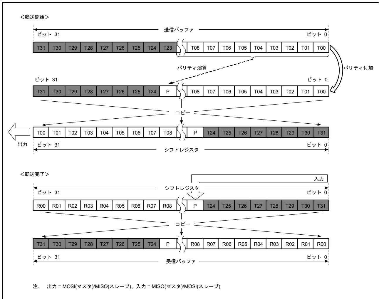
図 43.21 LSB ファースト (24 ビットデータ / パリティ機能有効)
