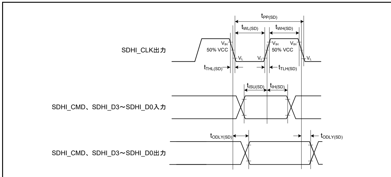
図 61.80 SD ホストインタフェース入出力信号タイミング
