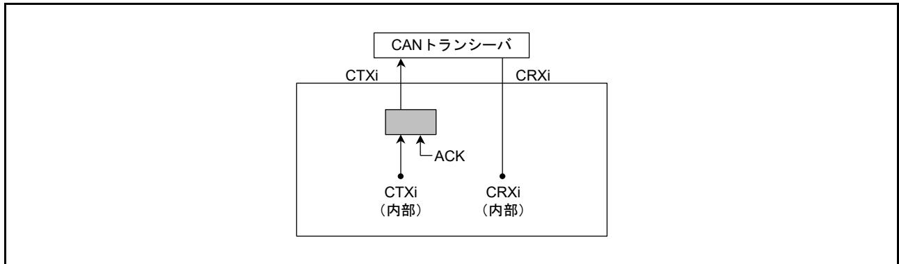
図42.7 セルフテストモード0選択時の接続 (i=0~2)
