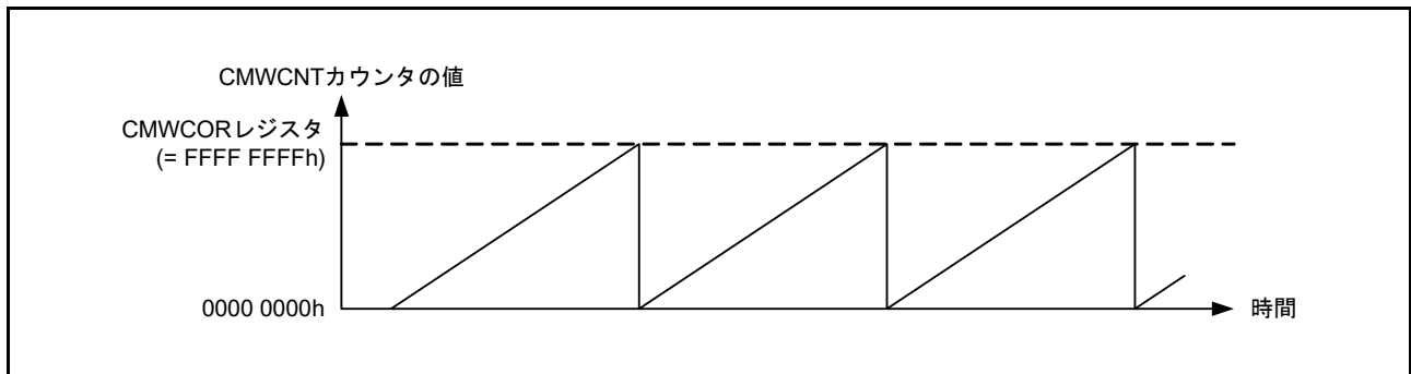
図 32.5 コンペアマッチ動作例 (オーバフロー検出時)
