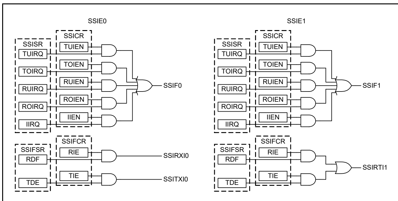
図 46.26 割り込みのブロック図
