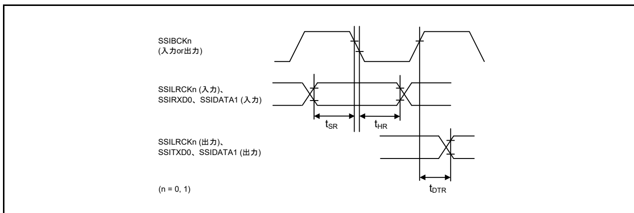
図 61.76 SSICR.BCKP = 1 の場合の SSIE データ送受信タイミング
