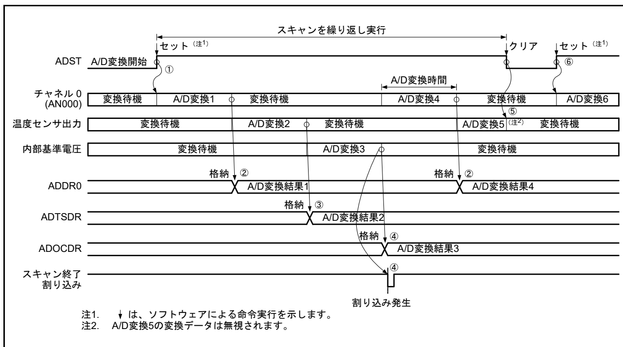
図 54.21 連続スキャンモードの動作例 (基本動作 : AN000、温度センサ出力、内部基準電圧選択)
