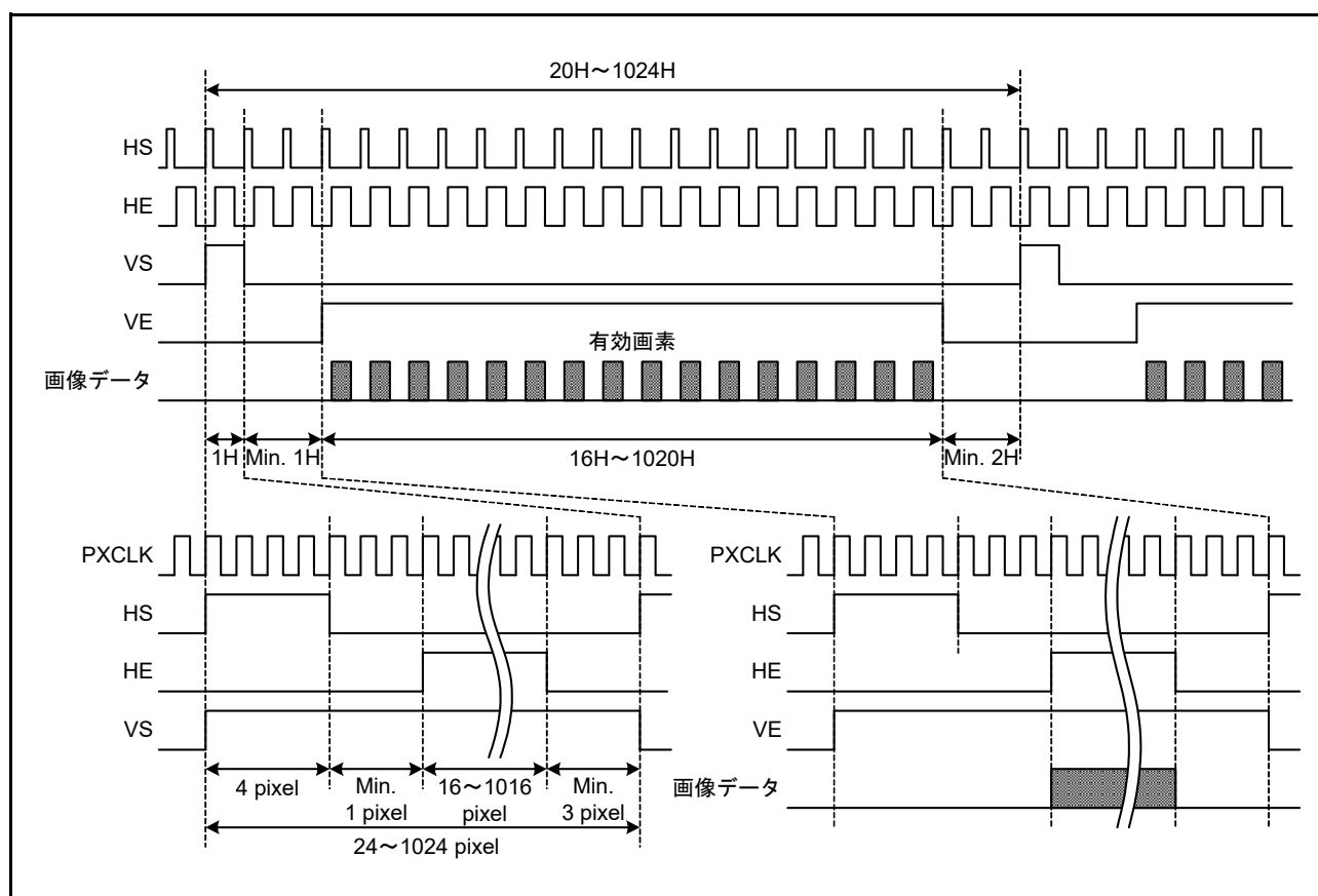
図 50.21 GLCDC の画像データ搬送信号
