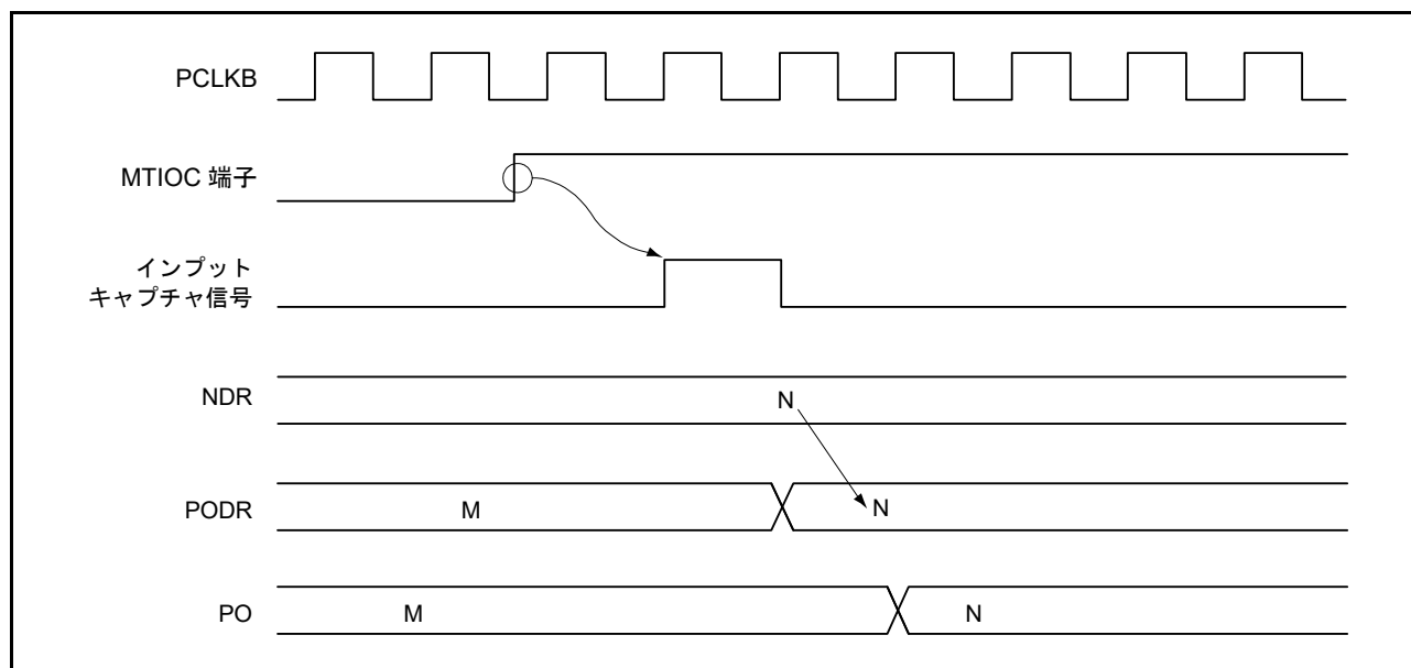
図 29.15 インプットキャプチャによるパルス出力例
