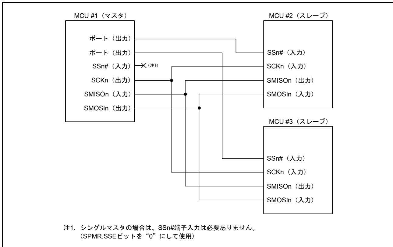
図 40.61 簡易 SPI モードの接続例 (シングルマスタ時 (SPMR.SSE ビット = 0))
