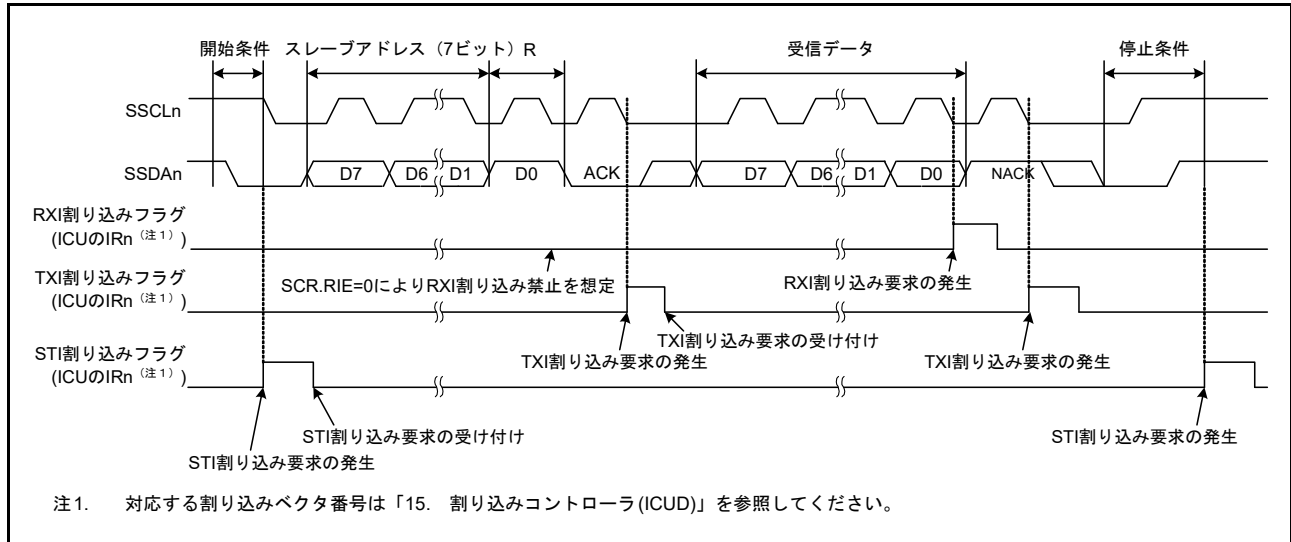
図 40.59 簡易 I 2 C バスモードのマスタ受信の動作例 (7 ビットスレーブアドレス、送信割り込み、受信割り込み使用時)
