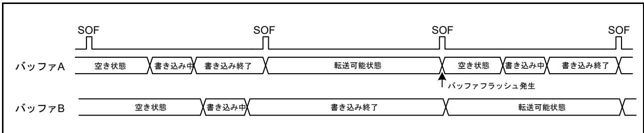
図 39.21 バッファフラッシュ機能動作例
