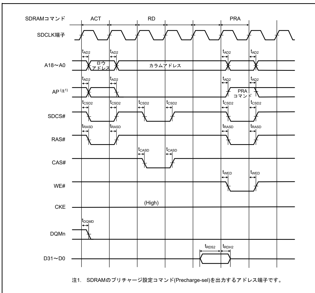
図 61.25 SDRAM 空間シングルリードバスタイミング
