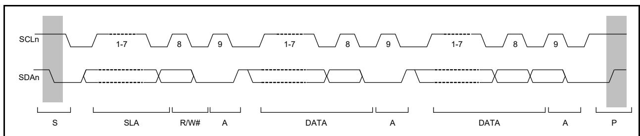
図 41.3 I 2 C バスタイミング (SLA = 7 ビットの場合)
