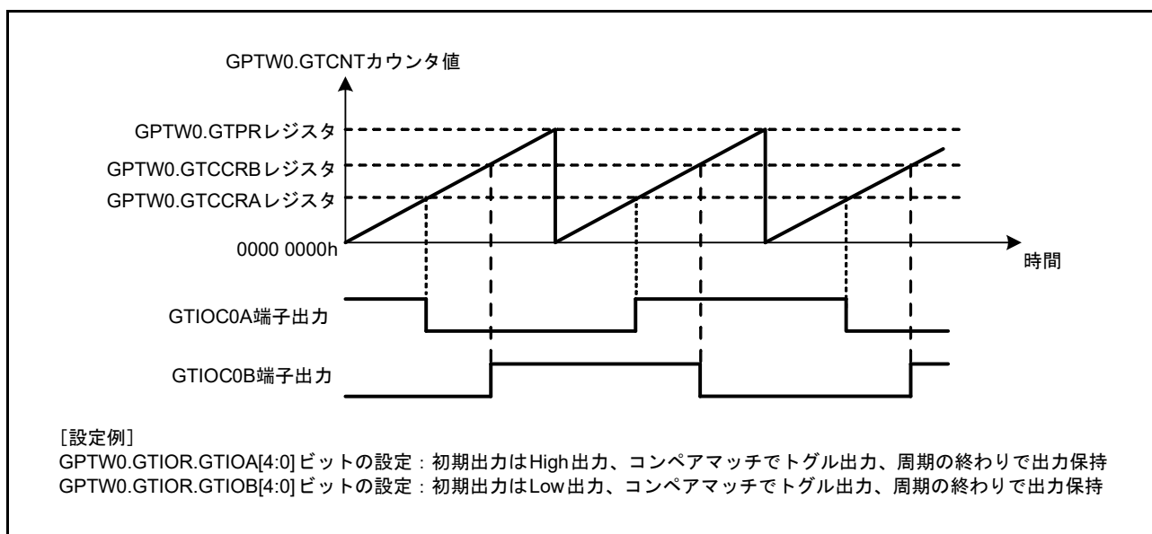
図 26.14 トグル出力動作例 (1)
