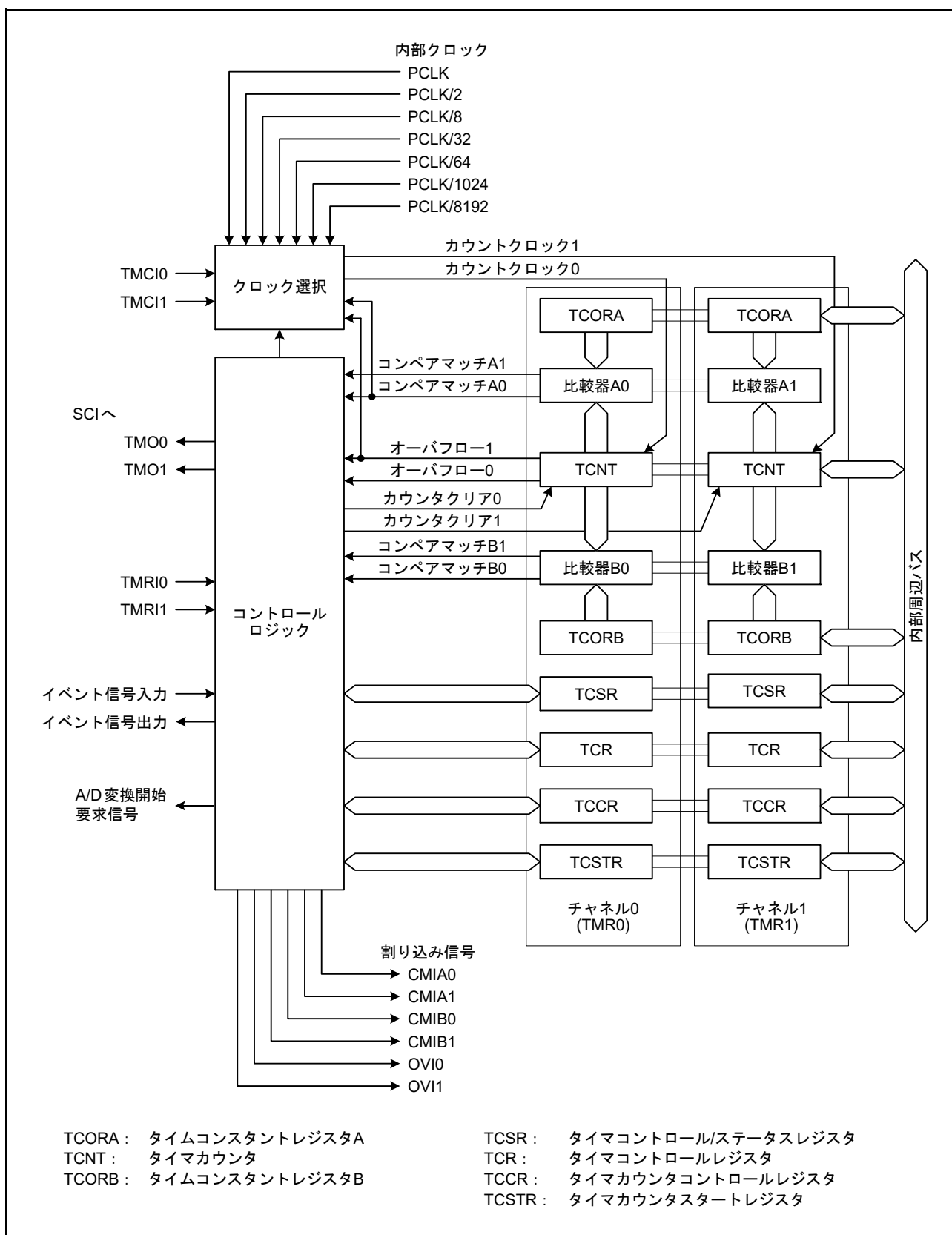
図 30.1 TMR (ユニット0) のブロック図
