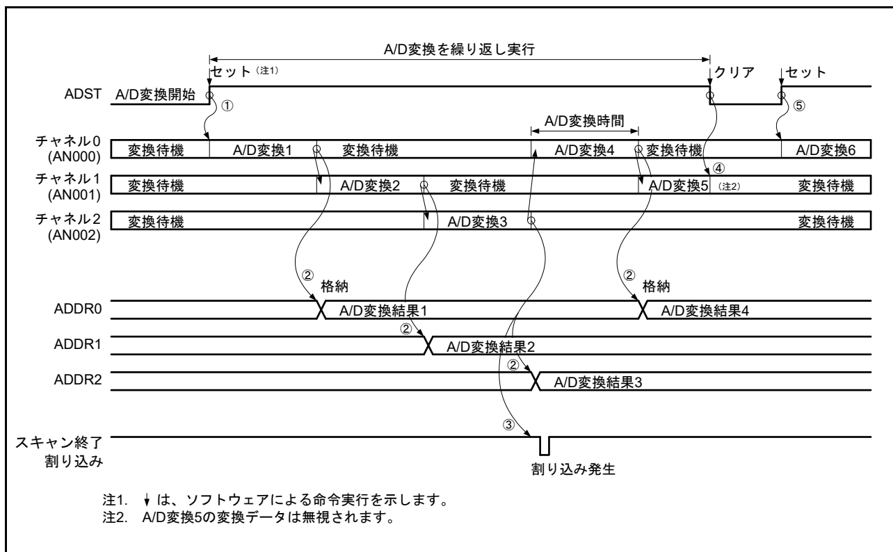
図 54.15 連続スキャンモードの動作例 (基本動作 : AN000, AN001, AN002 選択)
