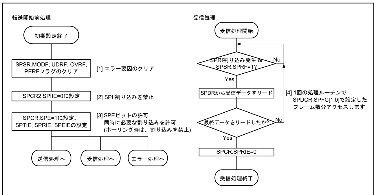
図 43.43 スレーブモード時のフローチャート (受信)
