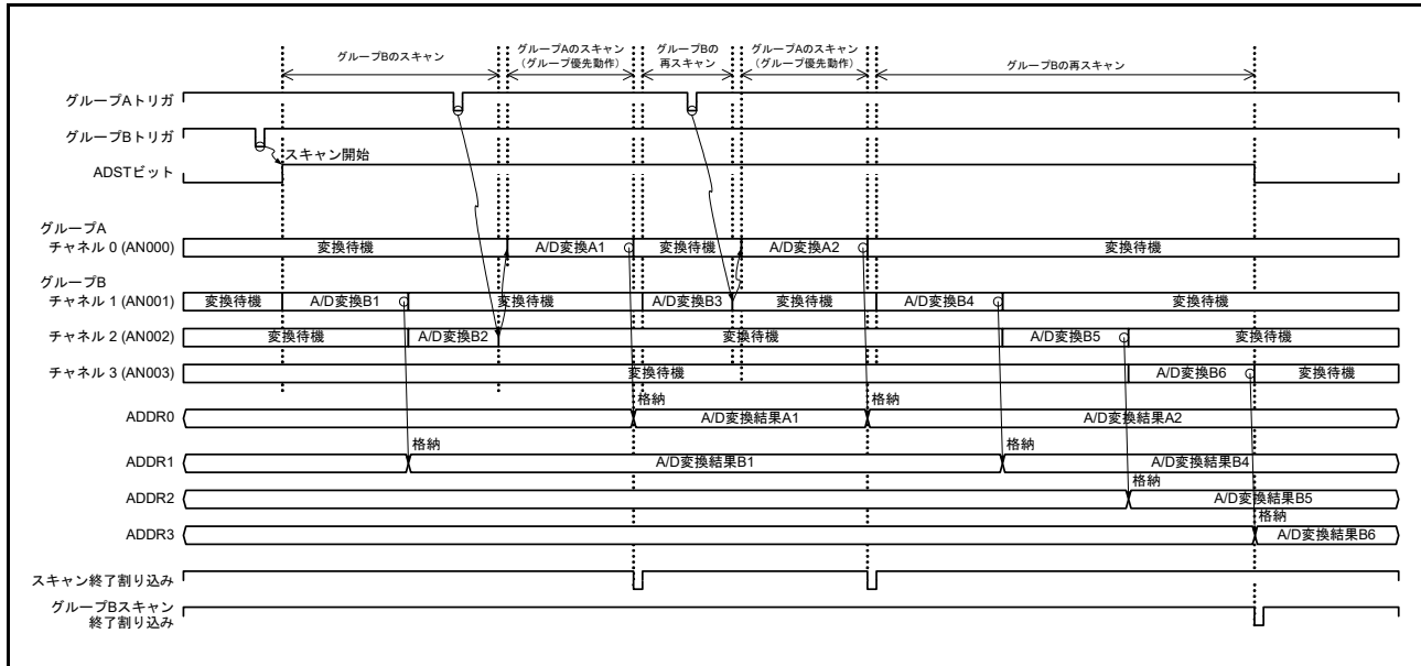
図 54.26 グループ優先動作の例2 「グループB再スキャン中のグループAトリガ入力」再スキャンあり (ADGSPCR.GBRSCN = 1, ADGSPCR.GBRP = 0, ADGSPCR.LGRRS = 0 設定時)
