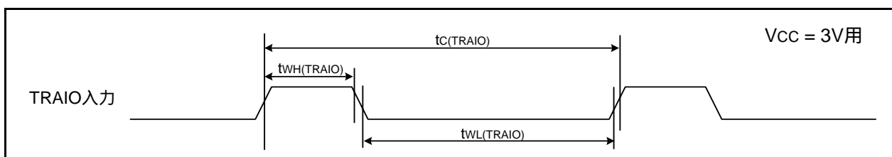
図33.13 Vcc = 3V時のTRAIO入力タイミング
