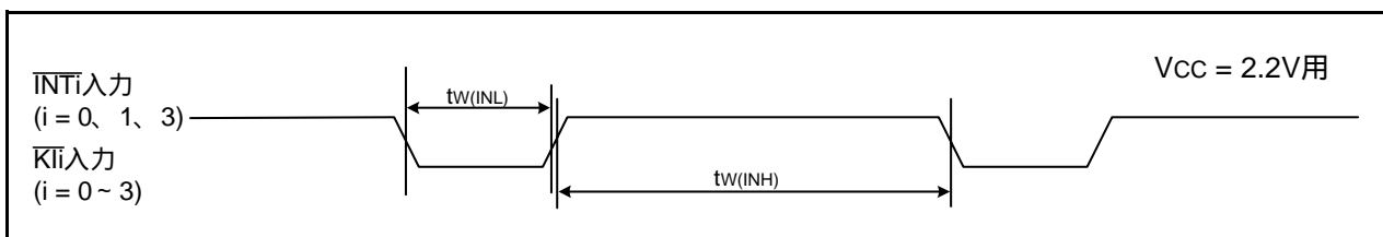
図33.19 V_{cc} = 2.2\text{V} 時の外部割り込み \overline{\text{INT}}_i およびキー入力割り込み \overline{\text{K}}_i 入力タイミング
