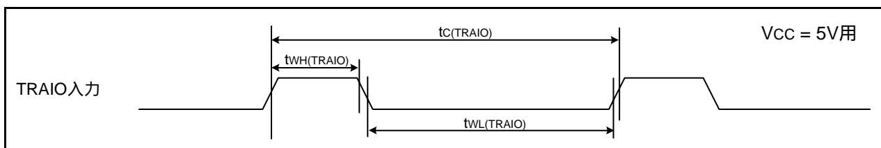
図33.9 V_{CC} = 5V 時のTRAIO入力タイミング
