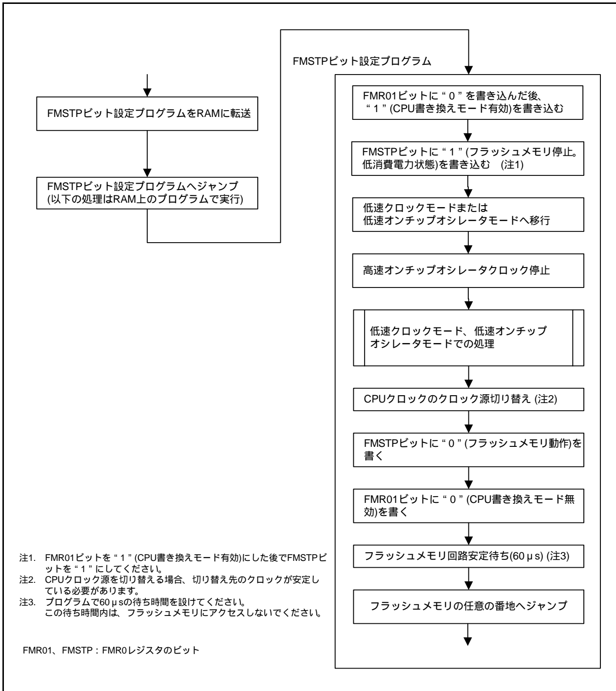
図 32.3 FMSTPビットによる低消費電力操作手順例
