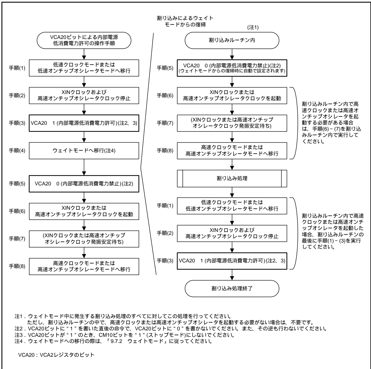
図 32.2 WAIT命令を実行してウェイトモードにする場合のVCA20ビットによる内部電源低消費操作手順
