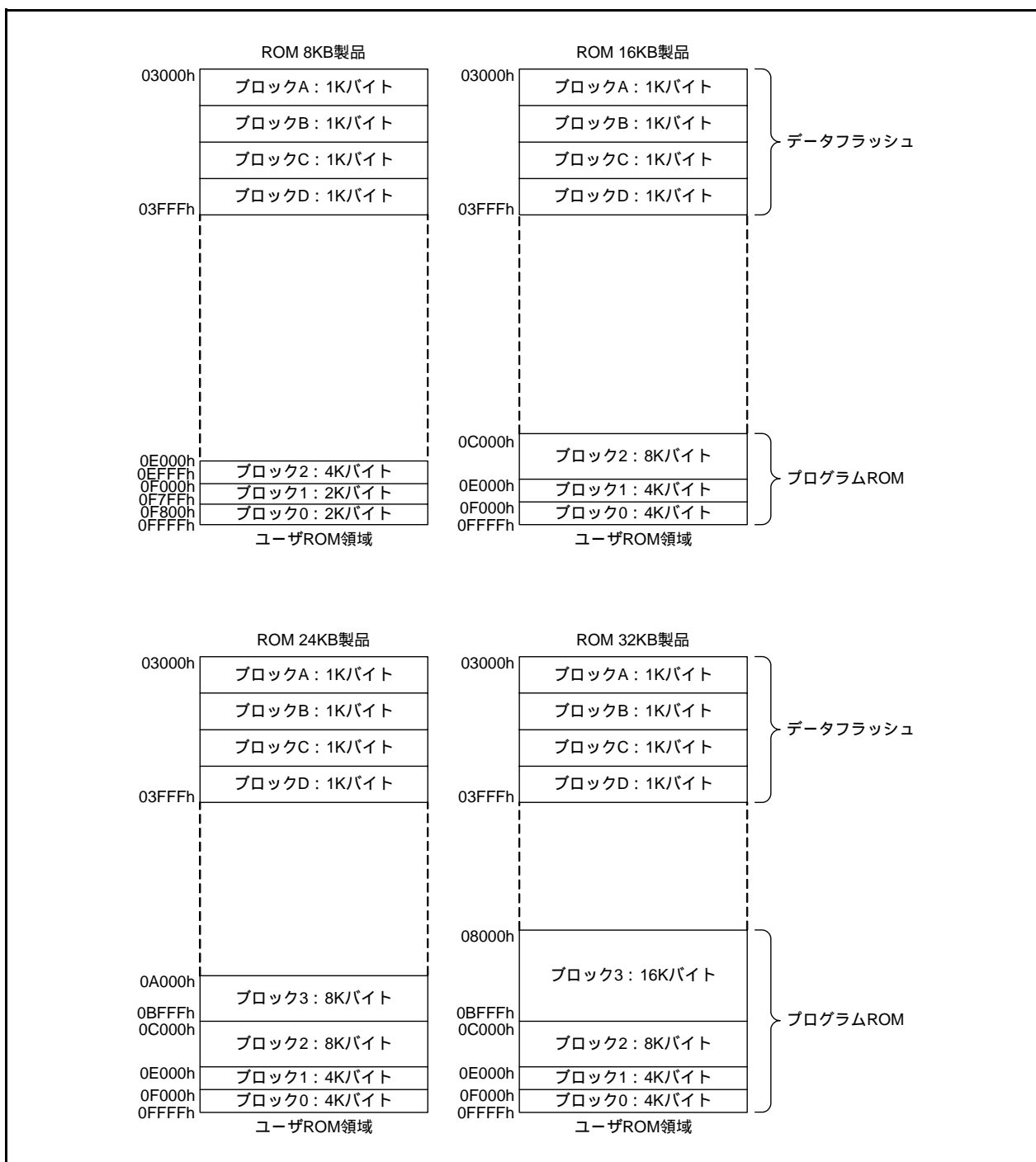
図 31.1 R8C/3GMグループのフラッシュメモリのブロック図
