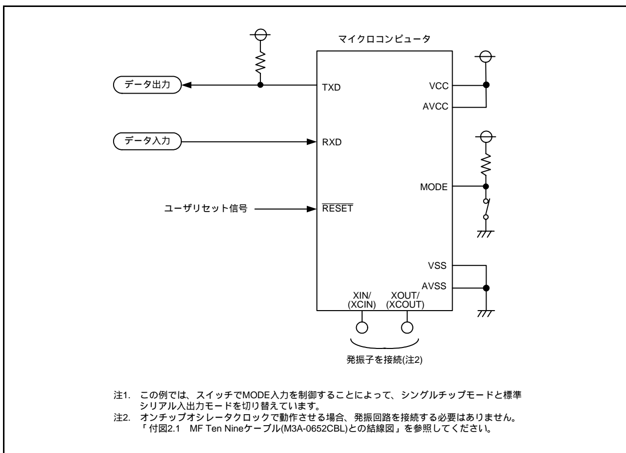
図 31.18 標準シリアル入出力モード2を使用する場合の端子処理例
