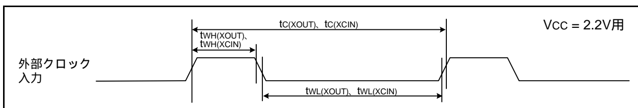
図33.16 VCC = 2.2V時の外部クロック入力タイミング
