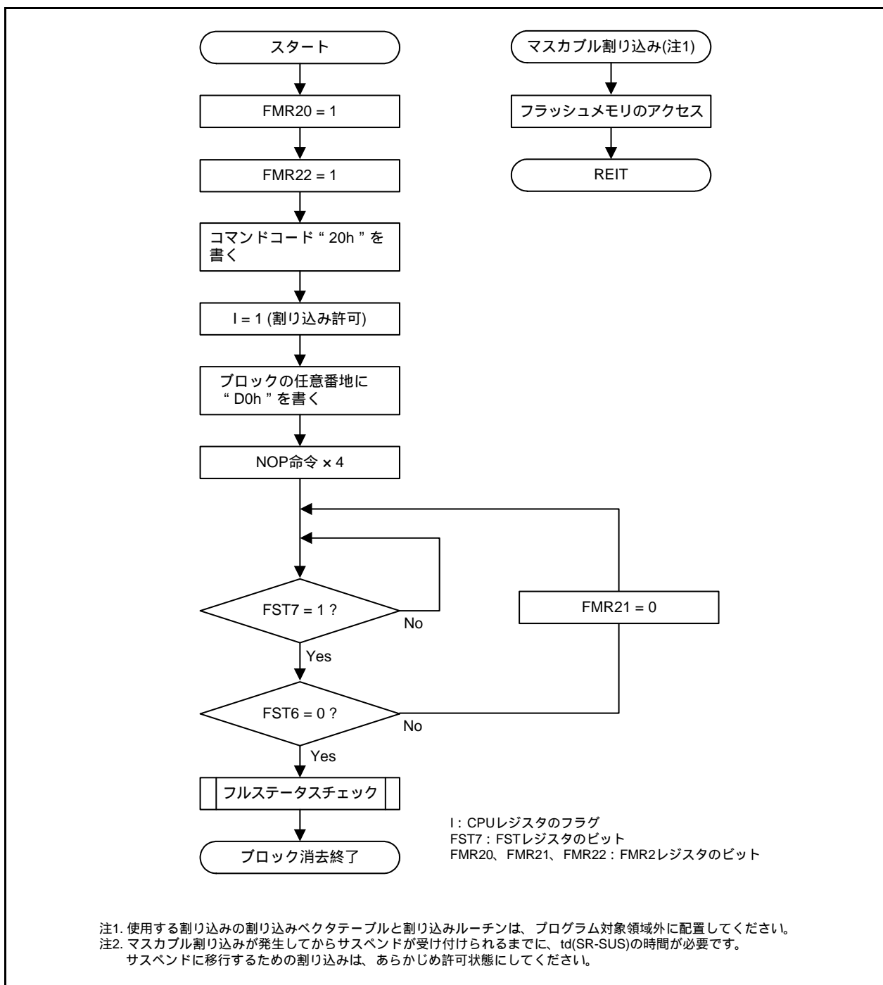
図31.13 EW1モードのブロックイレーズフローチャート(フラッシュレディステータス割り込み禁止かつサスペンド許可)
