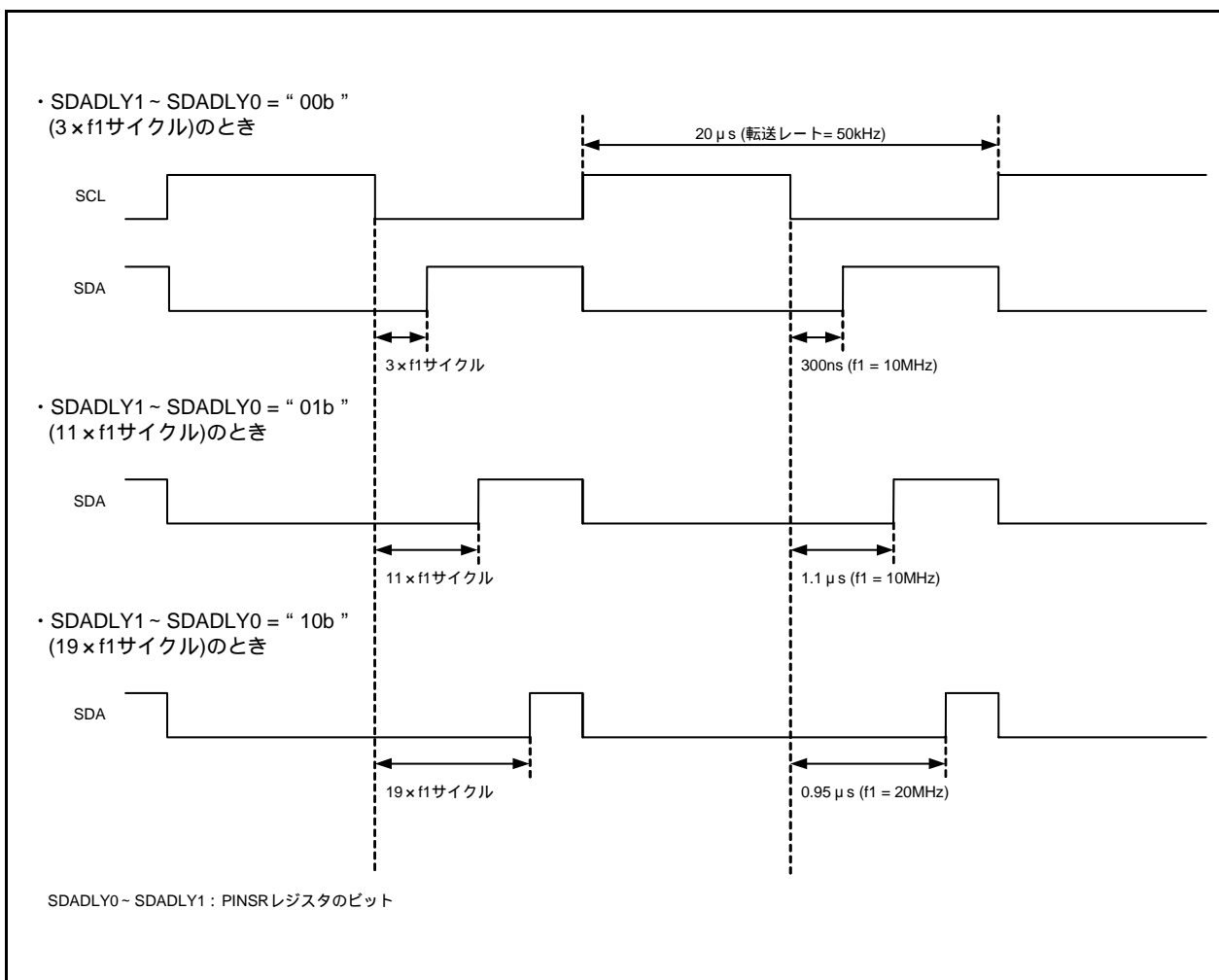
図 25.3 SDA端子のデジタル遅延の動作例
