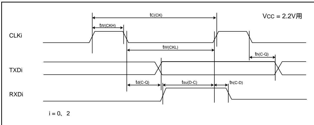
図33.18 V_{cc} = 2.2\text{V} 時のシリアルインタフェースのタイミング
