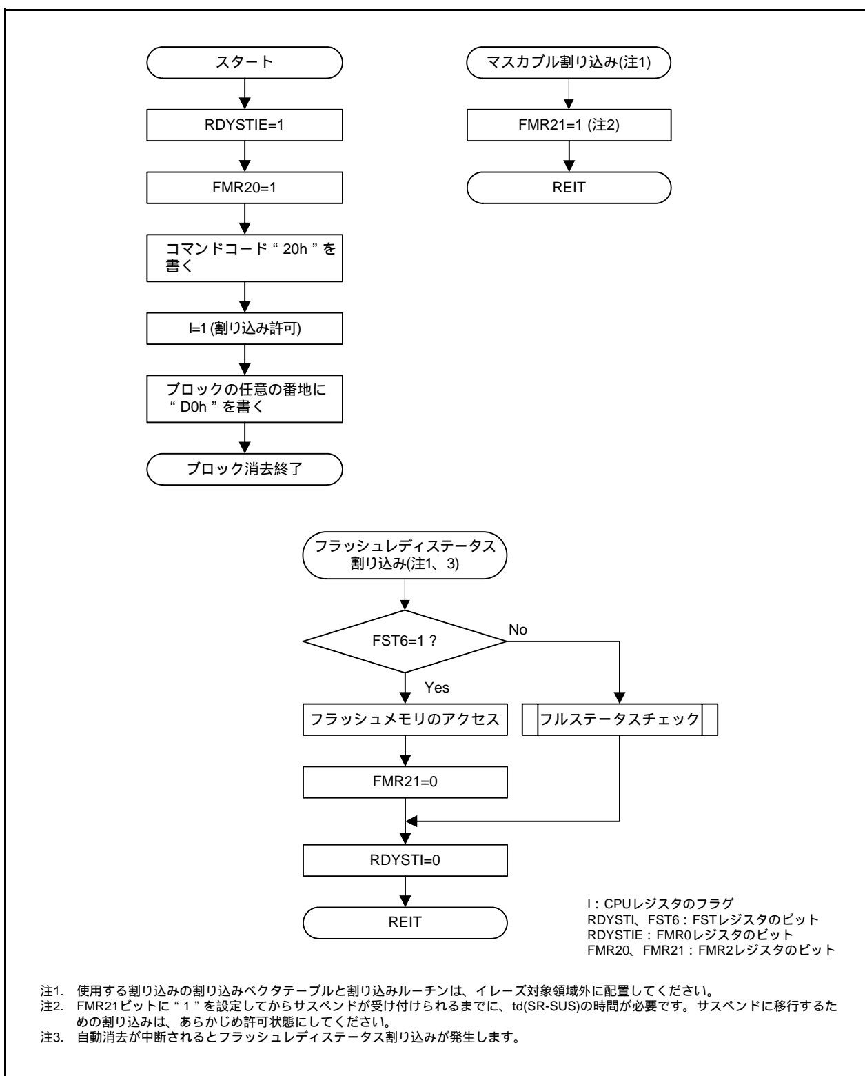
図 31.12 EW0モードのブロックイレーズフローチャート(フラッシュレディステータス割り込み許可かつサスペンド許可)
