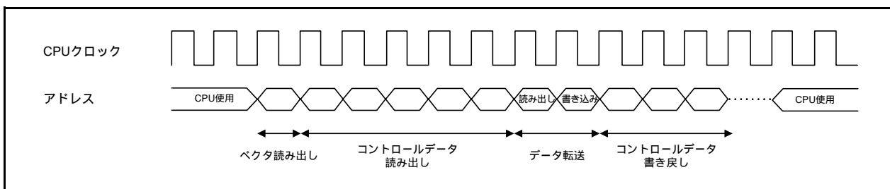
図 15.11 DTCの動作タイミング例
