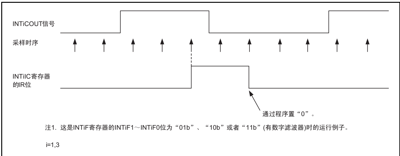
图 28.4 比较电路 Bi 数字滤波器的运行例子
