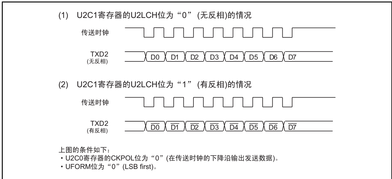
图 22.6 串行数据的逻辑
