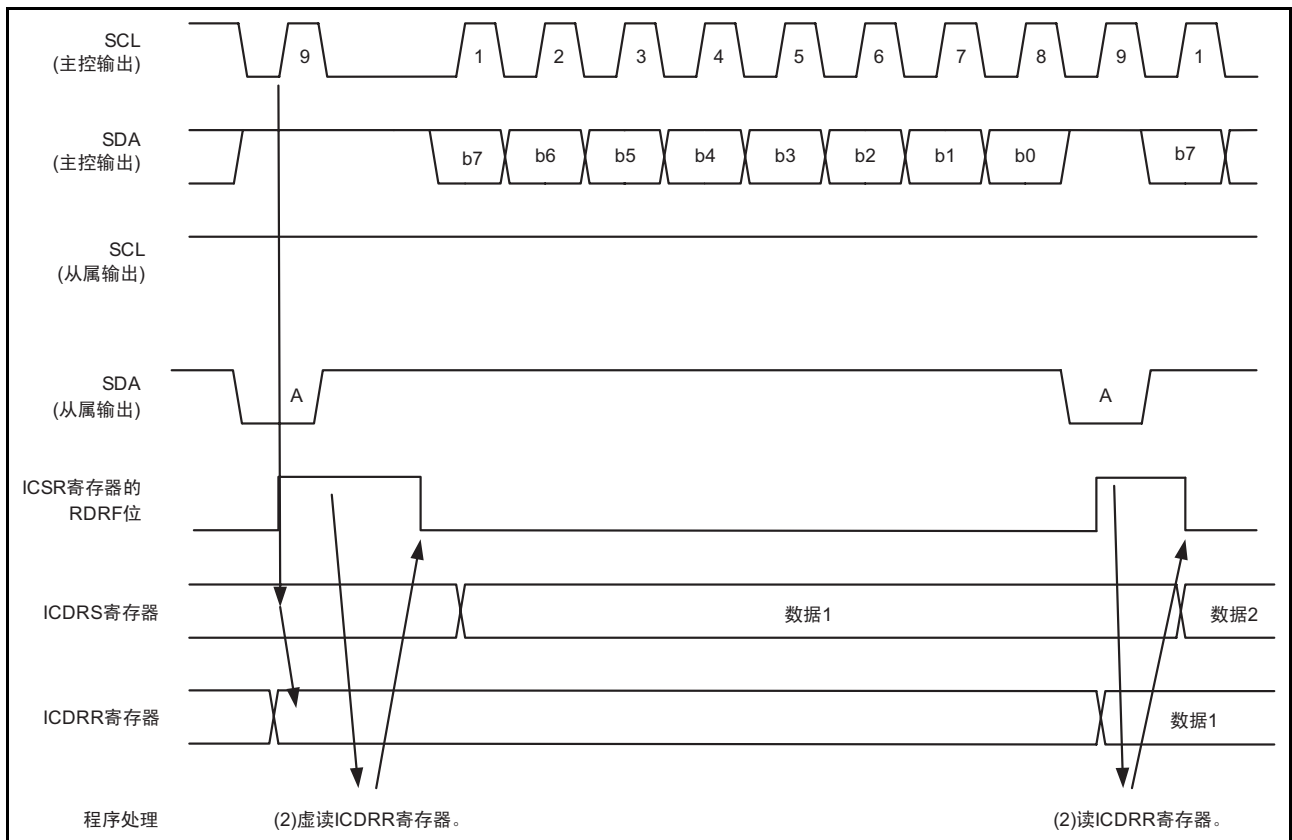
图 25.11 从属接收模式的运行时序 (I 2 C 总线接口模式) (1)
