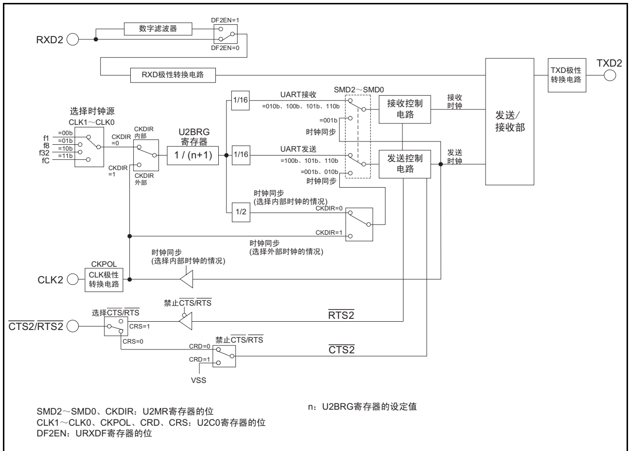
图 22.1 UART2 的框图
