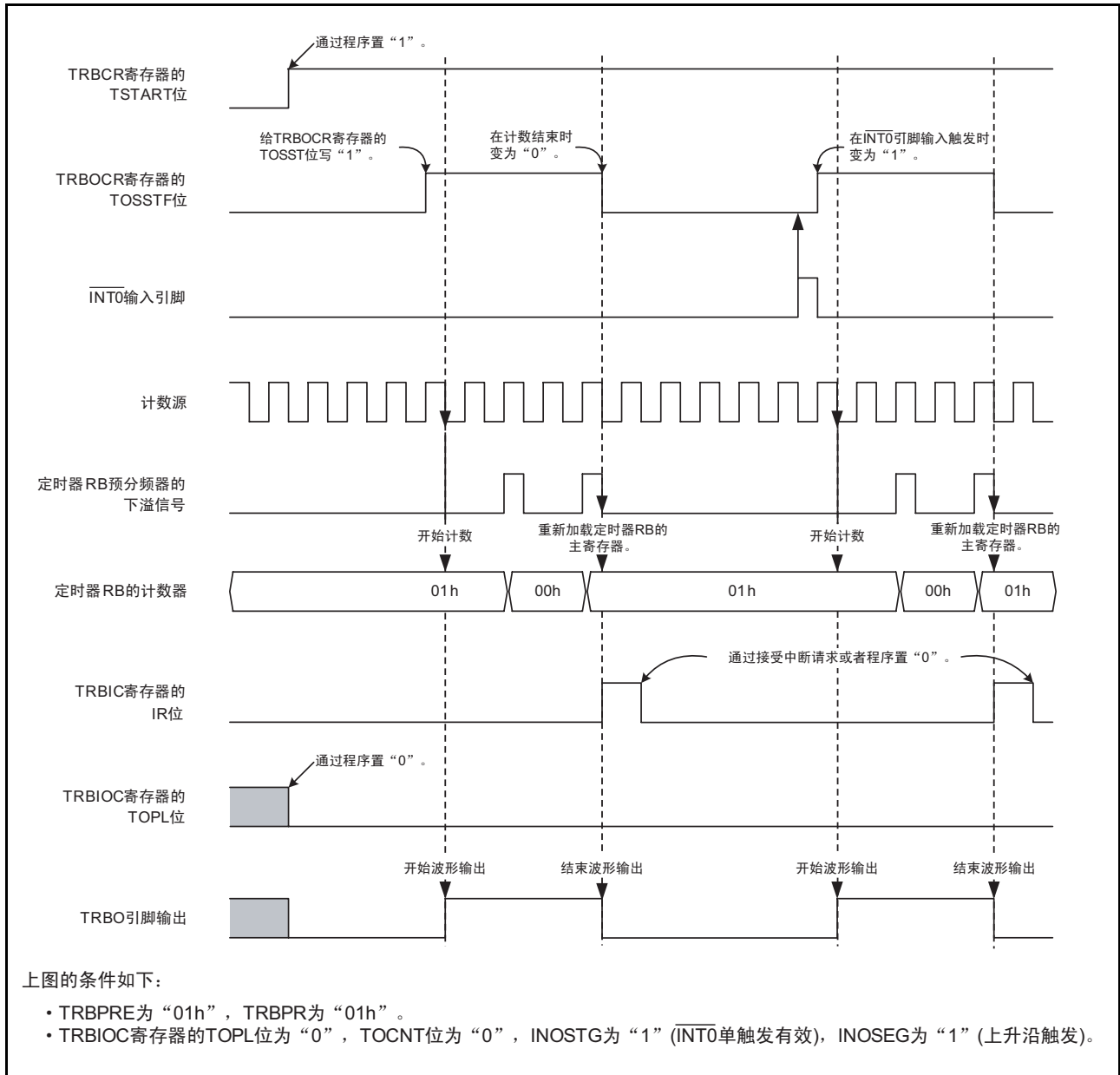
图 18.4 可编程单触发生模式的运行例子
