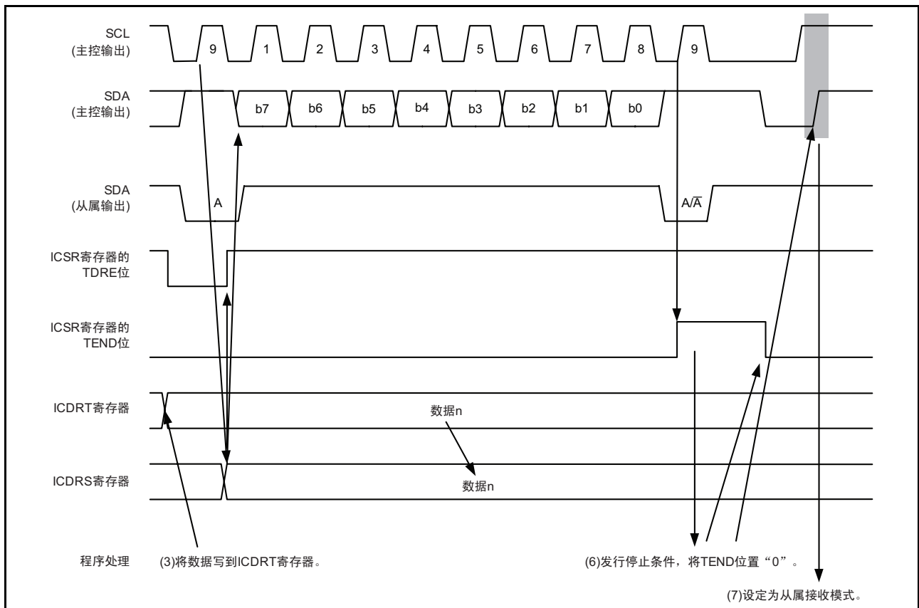
图 25.6 主控发送模式的运行时序（I 2 C 总线接口模式）（2）
