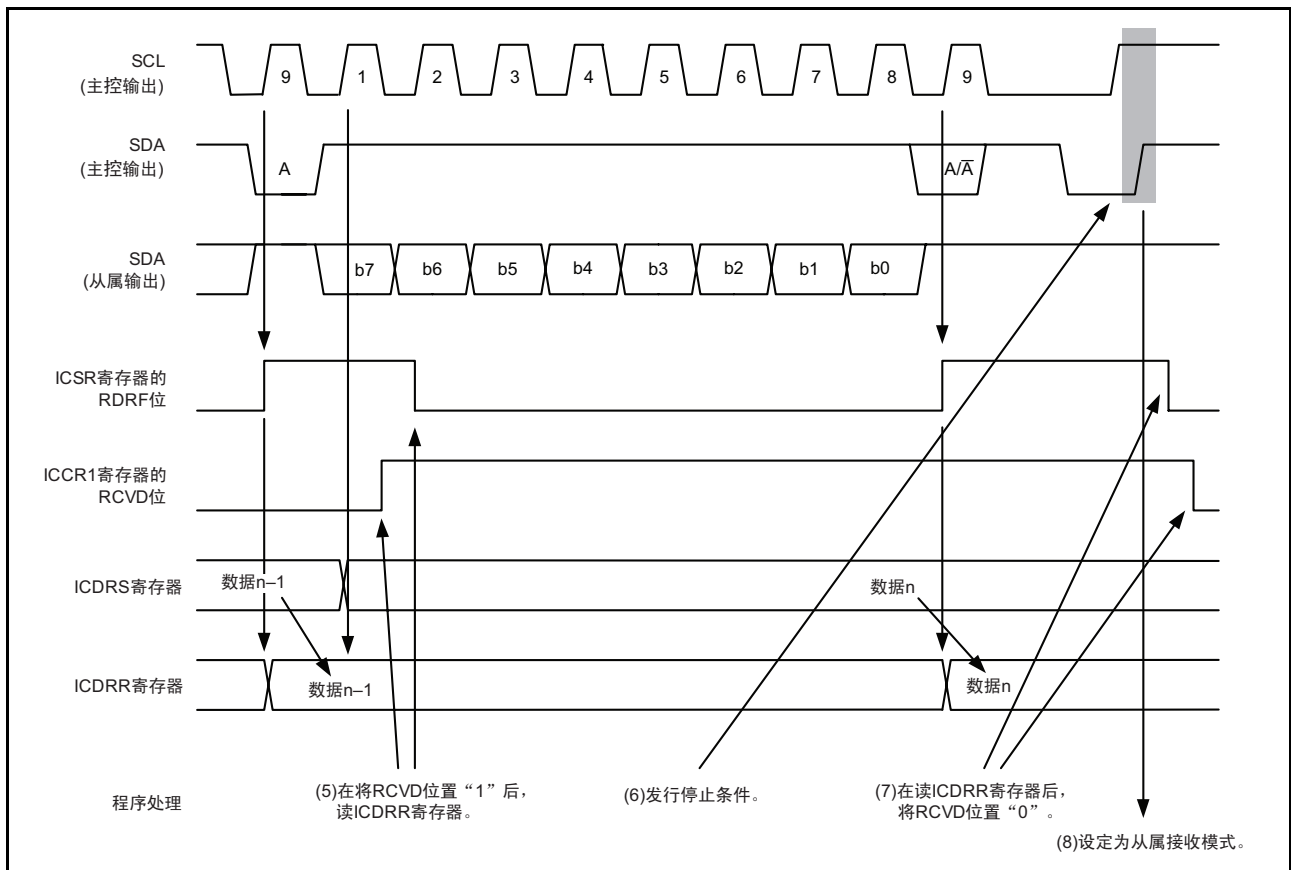
图 25.8 主控接收模式的运行时序 (I 2 C 总线接口模式) (2)
