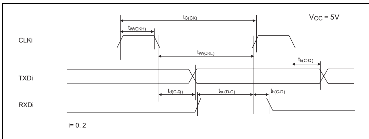
图 31.10 V CC =5V 时的串行接口时序
