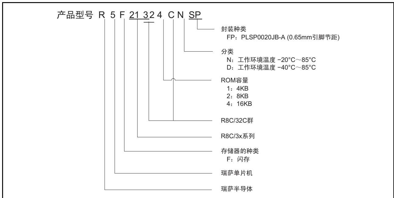
图 1.1 R8C/32C 群的产品型号、存储器容量和封装
