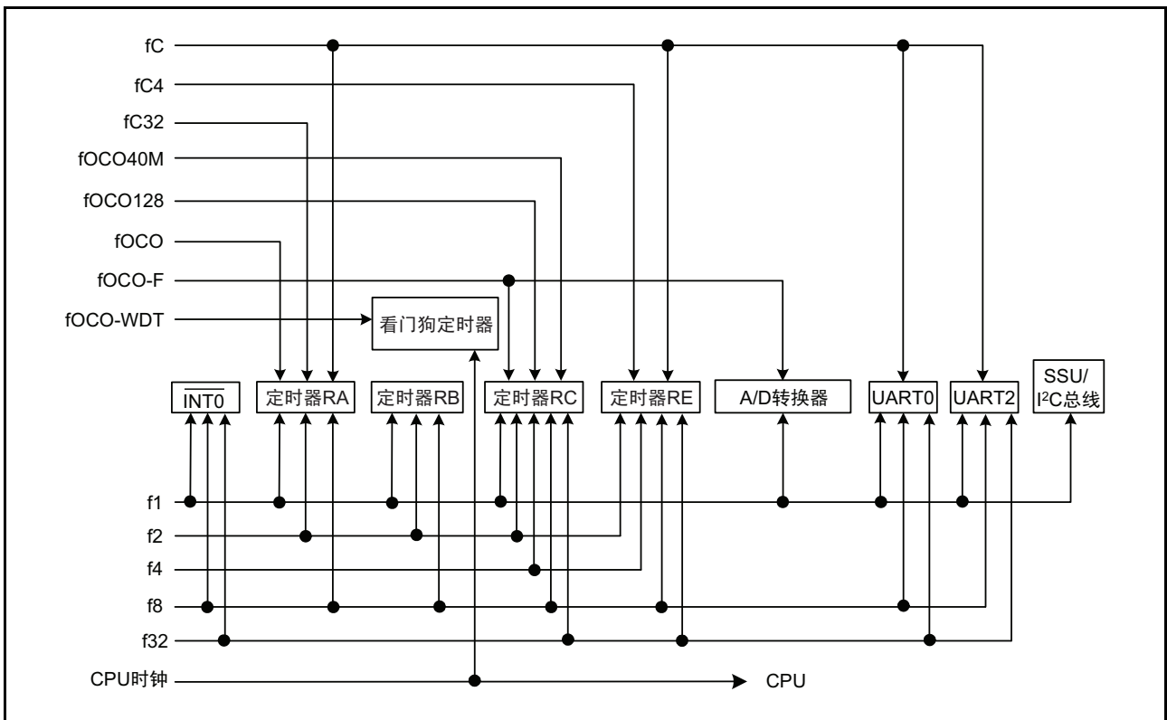
图 9.2 外围功能的时钟
