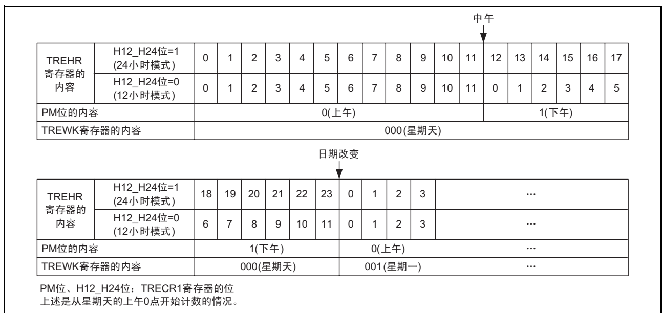
图 20.2 时间表现的定义
