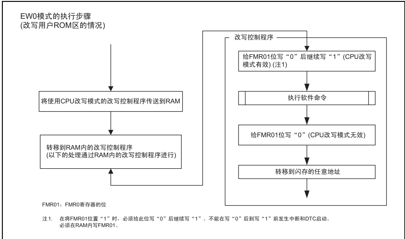
图 29.4 EW0 模式的设定和解除方法
