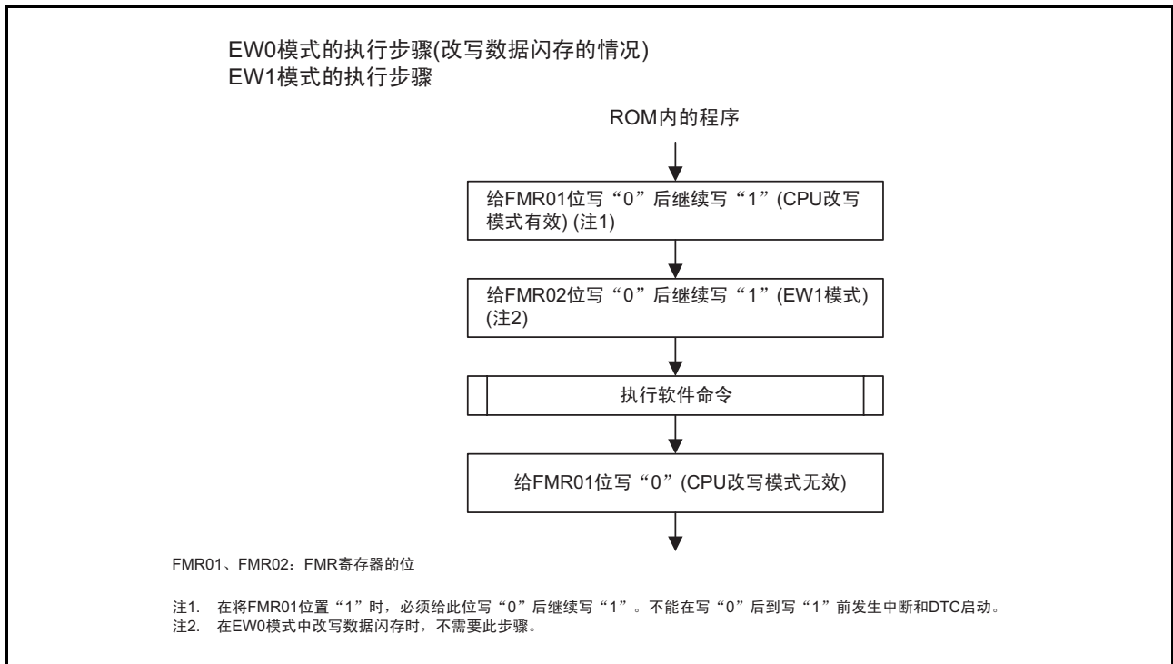
图 29.5 EW0 模式（改写数据闪存的情况）和 EW1 模式的设定和解除方法
