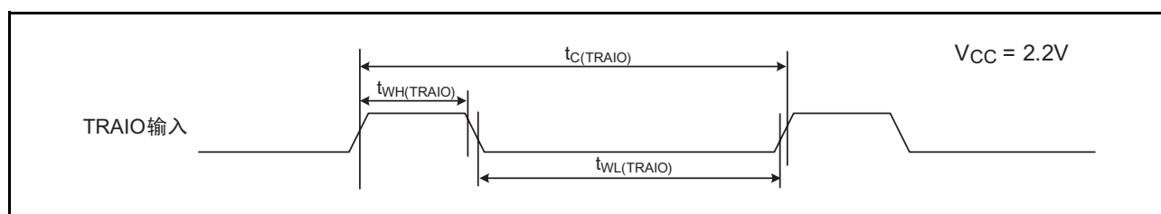
图 31.17 V_{CC}=2.2V 时的 TRAIO 输入时序
