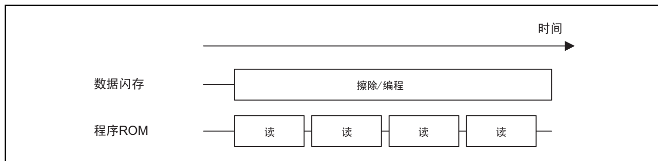
图 29.6 BGO 功能
