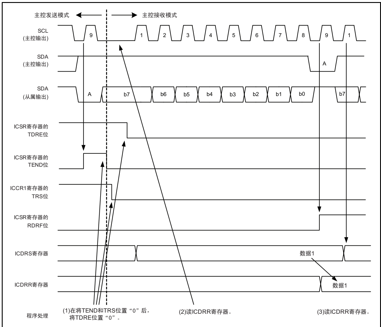
图 25.7 主控接收模式的运行时序 (I 2 C 总线接口模式) (1)
