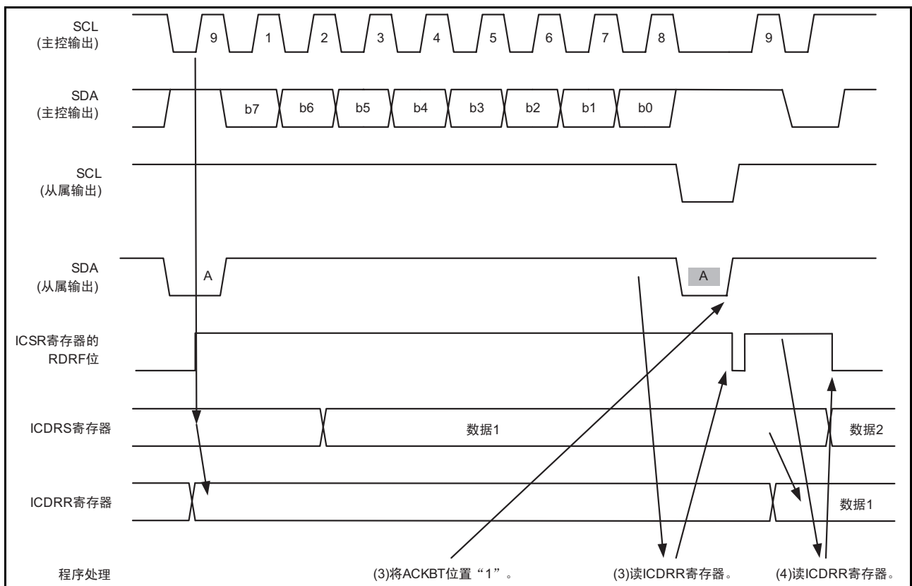
图 25.12 从属接收模式的运行时序 (I 2 C 总线接口模式) (2)
