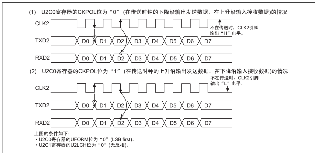
图 22.4 传送时钟的极性
