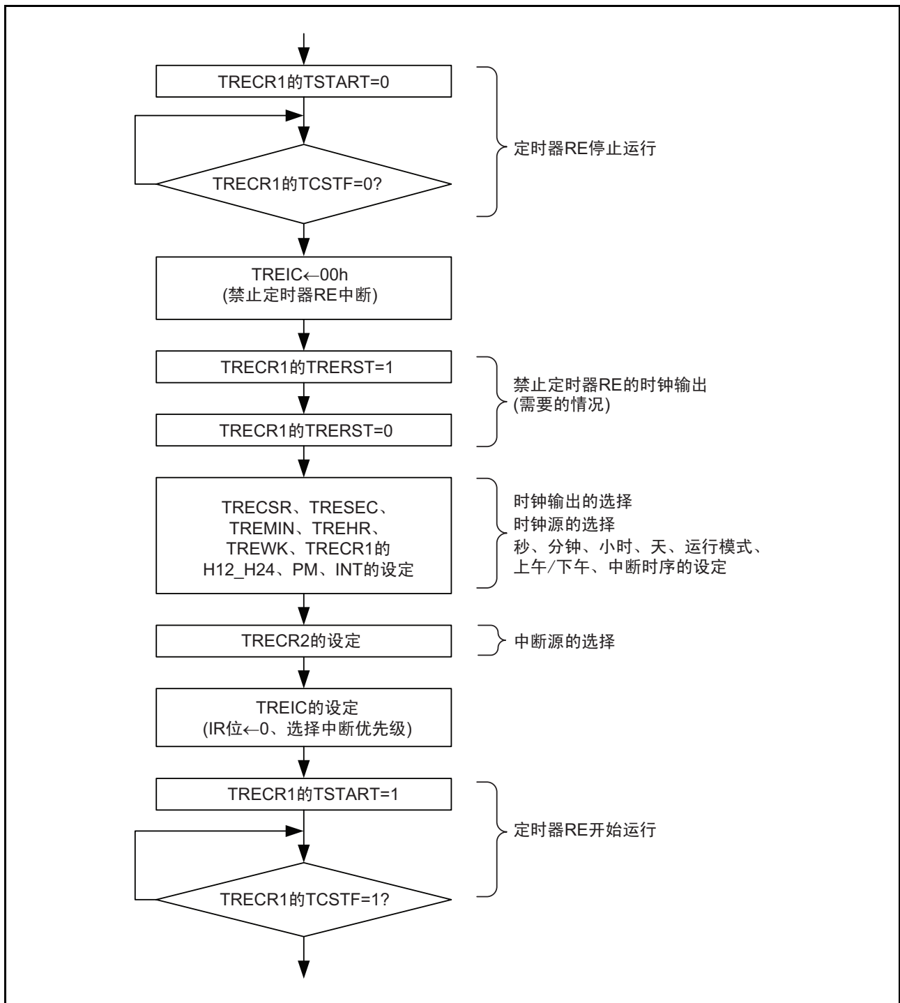
图 20.6 实时时钟模式的设定例子
