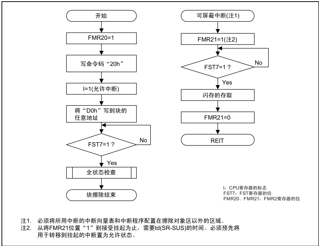
图 29.11 块擦除的流程图（禁止闪存就绪状态的中断而允许挂起）
