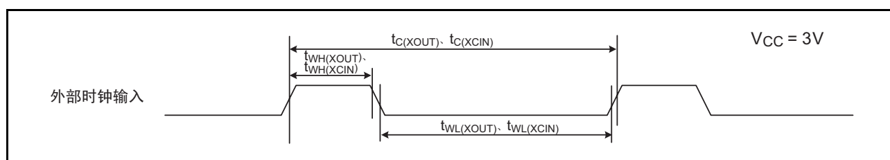
图 31.12 V_{CC}=3V 时的外部时钟输入时序
