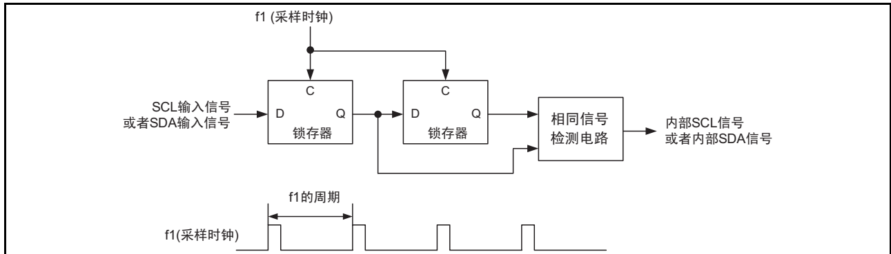
图 25.20 噪声消除电路的框图
