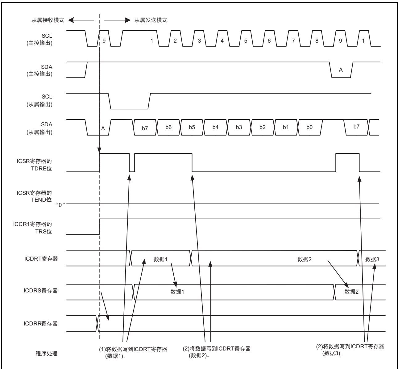
图 25.9 从属发送模式的运行时序 (I 2 C 总线接口模式) (1)
