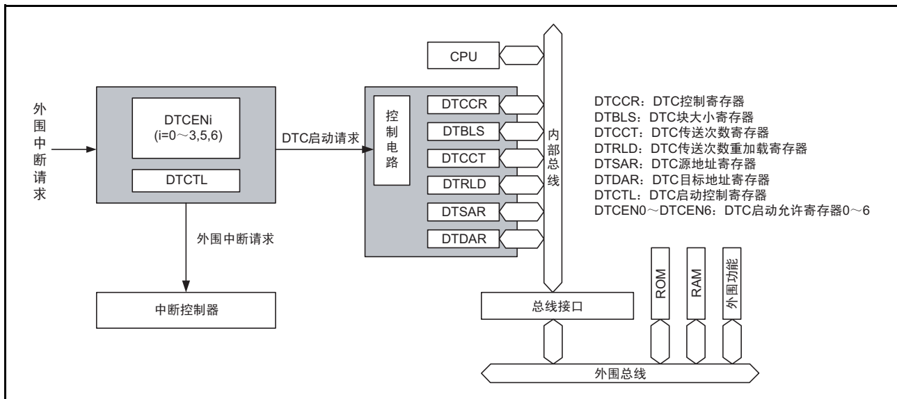
图 15.1 DTC 的框图
