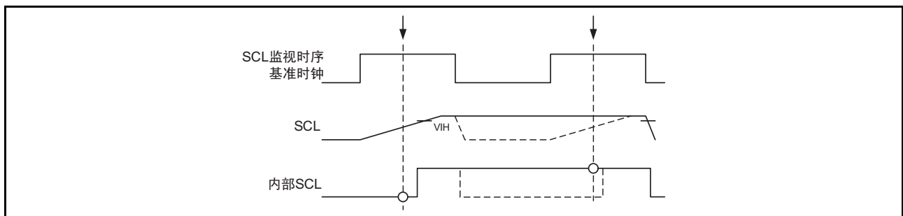
图 25.21 位同步电路的时序
