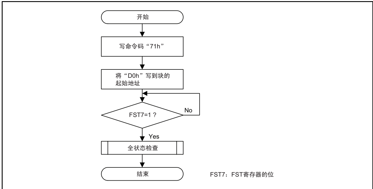
图 29.14 读锁定位状态的流程图
