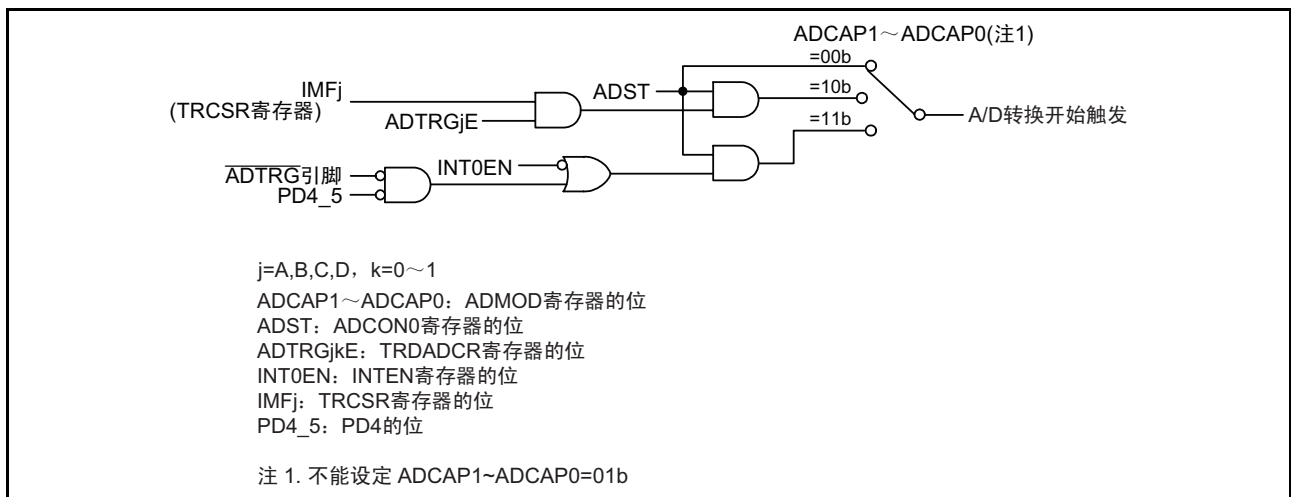
图 27.4 A/D 转换开始控制部的框图
