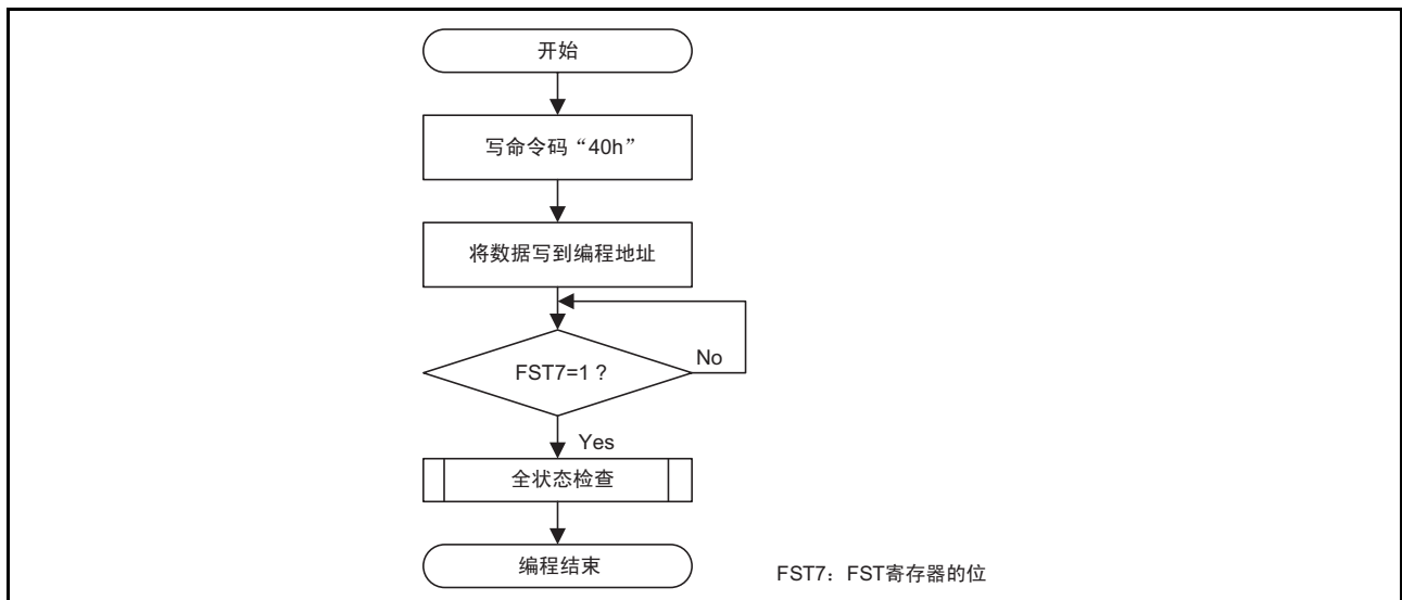
图 29.8 编程的流程图（禁止闪存就绪状态的中断）
