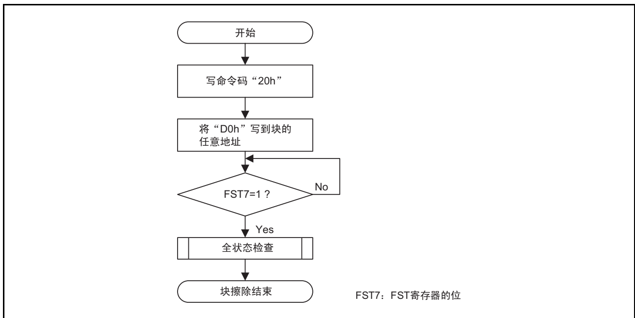
图 29.10 块擦除的流程图（禁止闪存就绪状态的中断）
