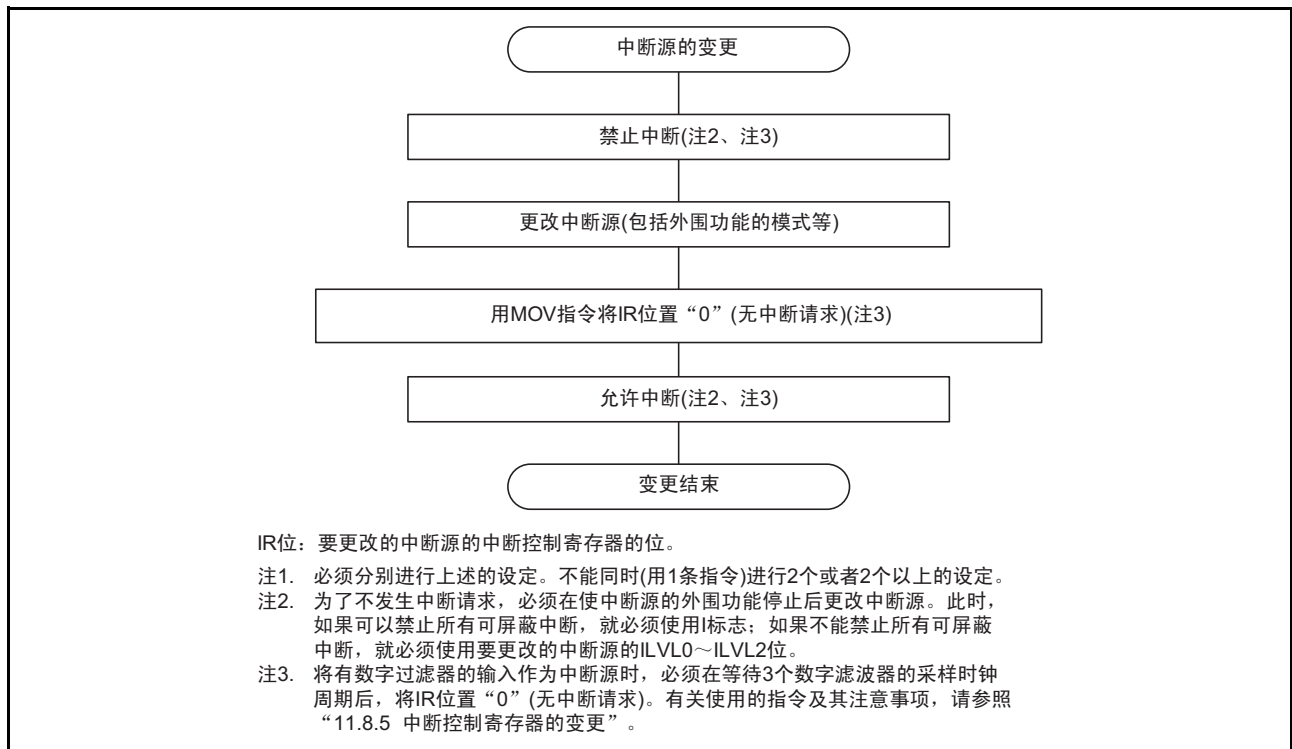
图 32.1 中断源的变更步骤例子
