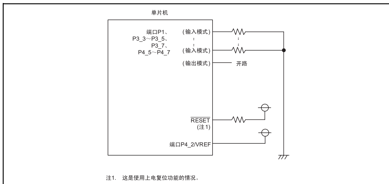
图 7.9 未使用引脚的处理例子
