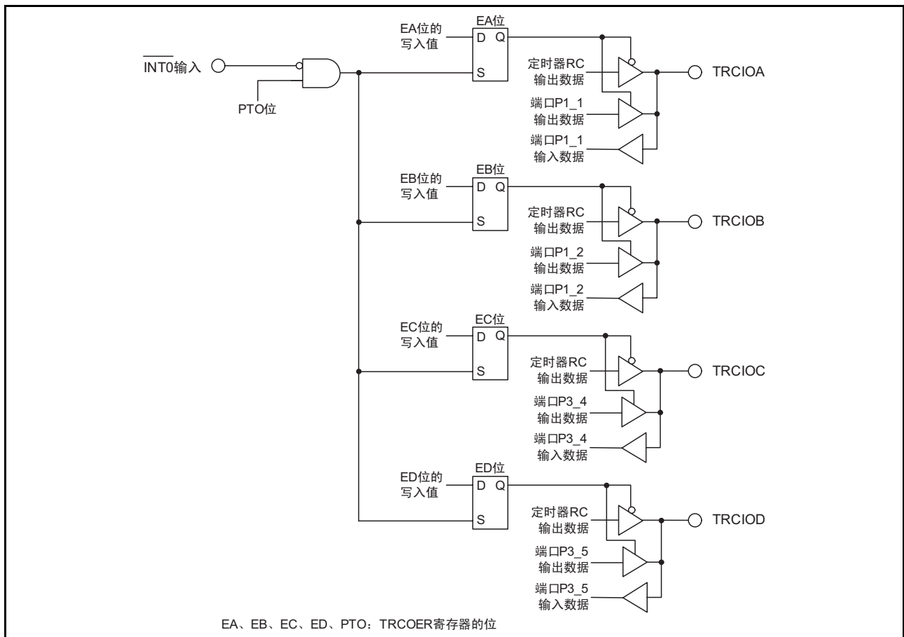
图 19.6 脉冲输出的强制截止
