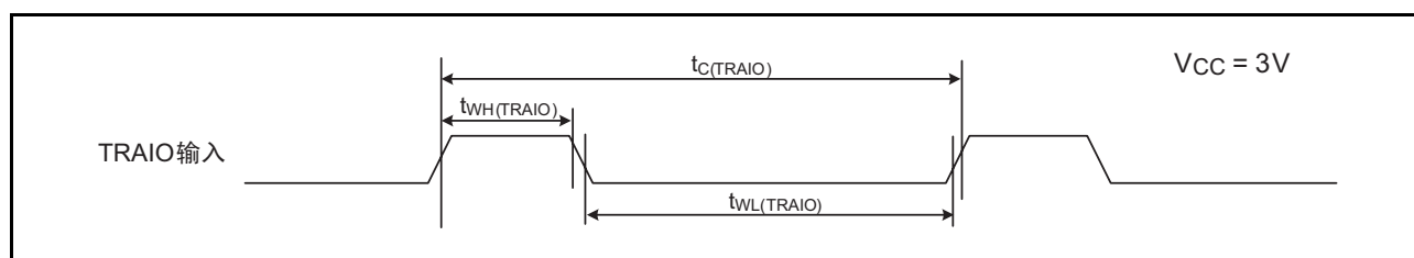
图 31.13 V_{CC}=3V 时的 TRAIO 输入时序
