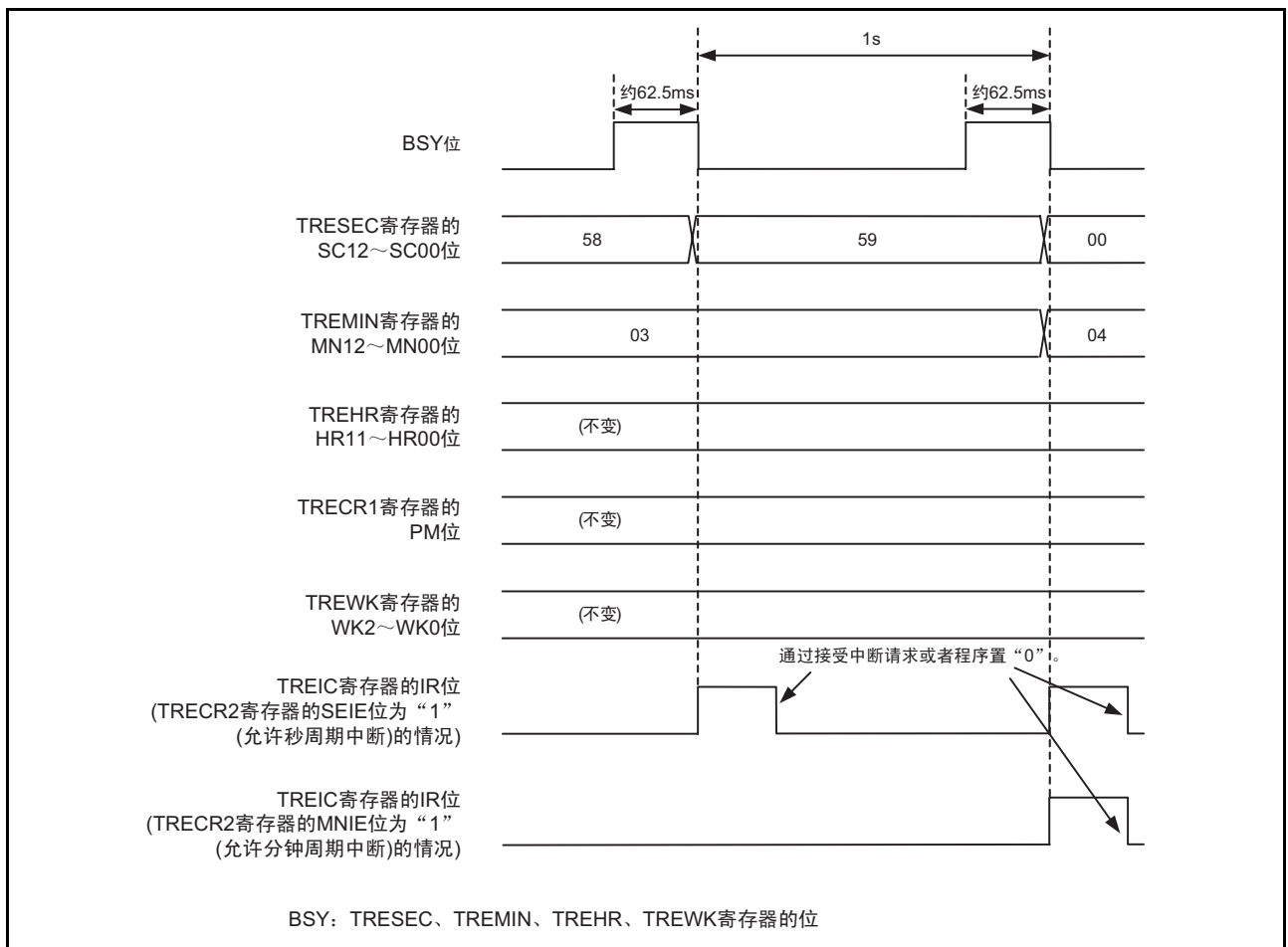
图 20.3 实时时钟模式的运行例子
