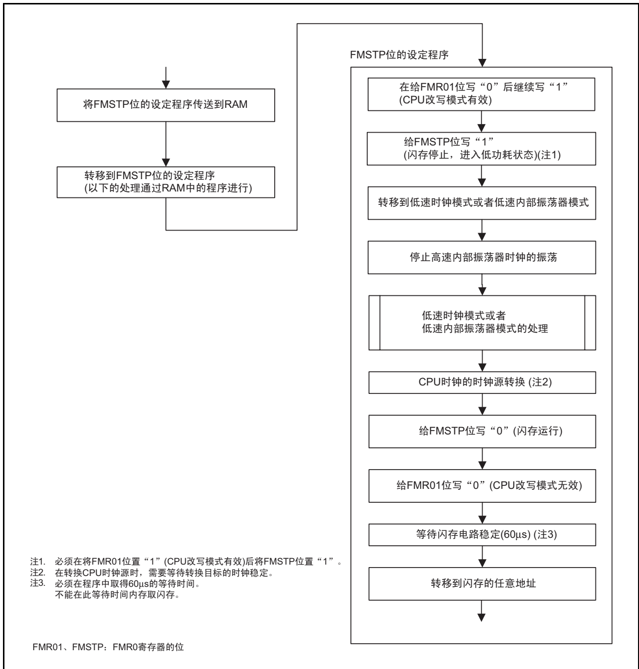
图 30.2 通过 FMSTP 位降低功耗的操作步骤例子
