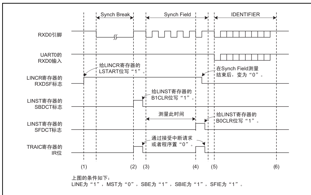
图 26.5 标题字段的接收运行例子
