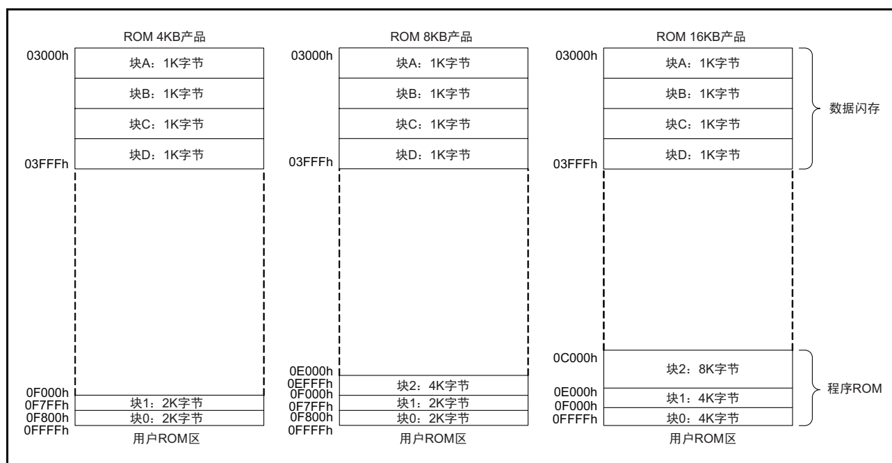
图 29.1 R8C/32C 群的闪存框图
