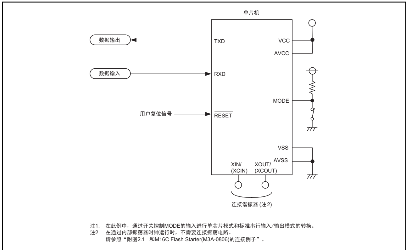
图 29.17 使用标准串行输入 / 输出模式 2 时的引脚处理例子
