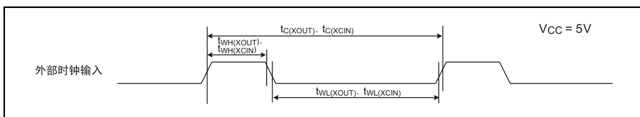
图 31.8 V_{CC}=5V 时的外部时钟输入时序
