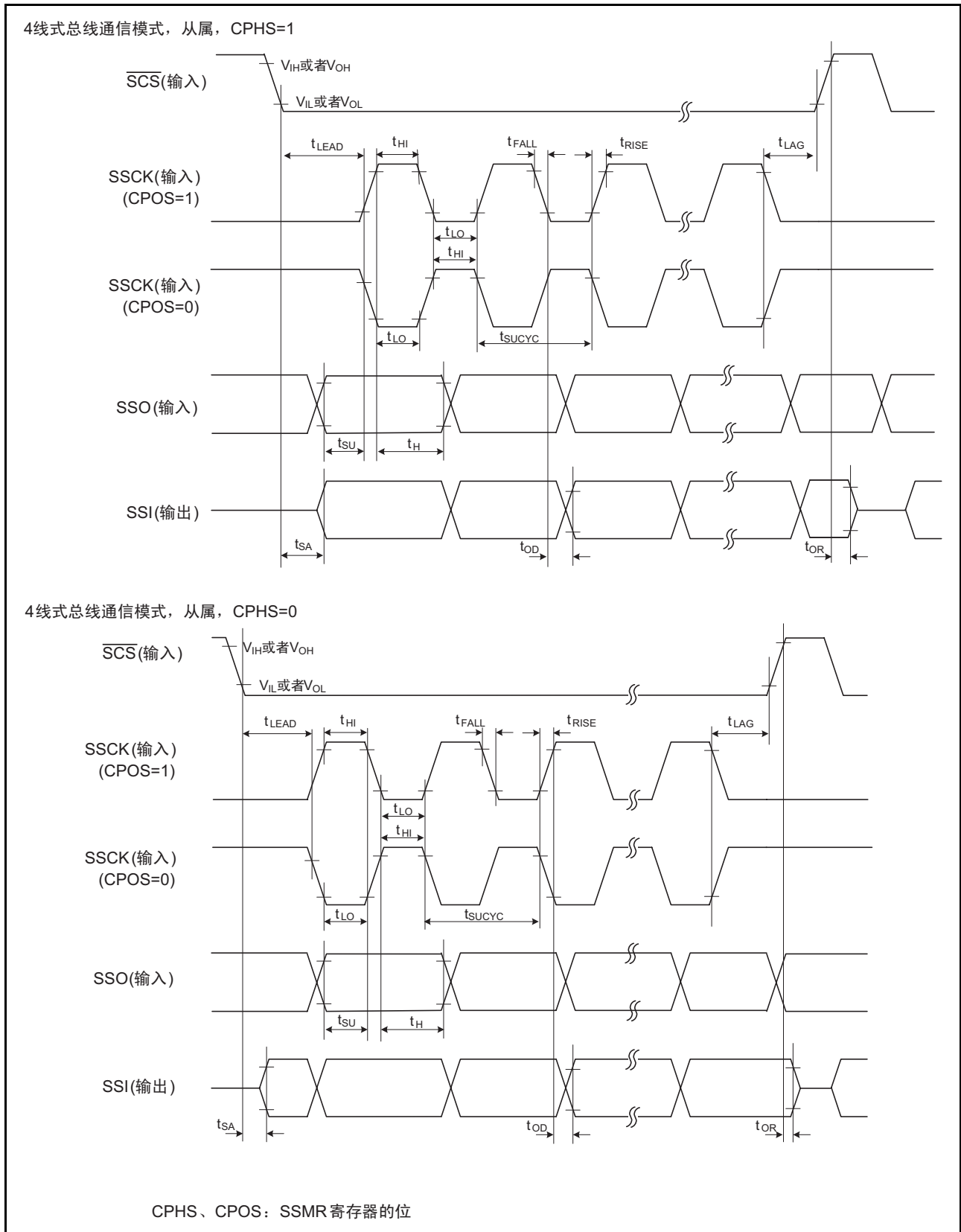
图 31.5 同步串行通信单元 (SSU) 的输入 / 输出时序 (从属)
