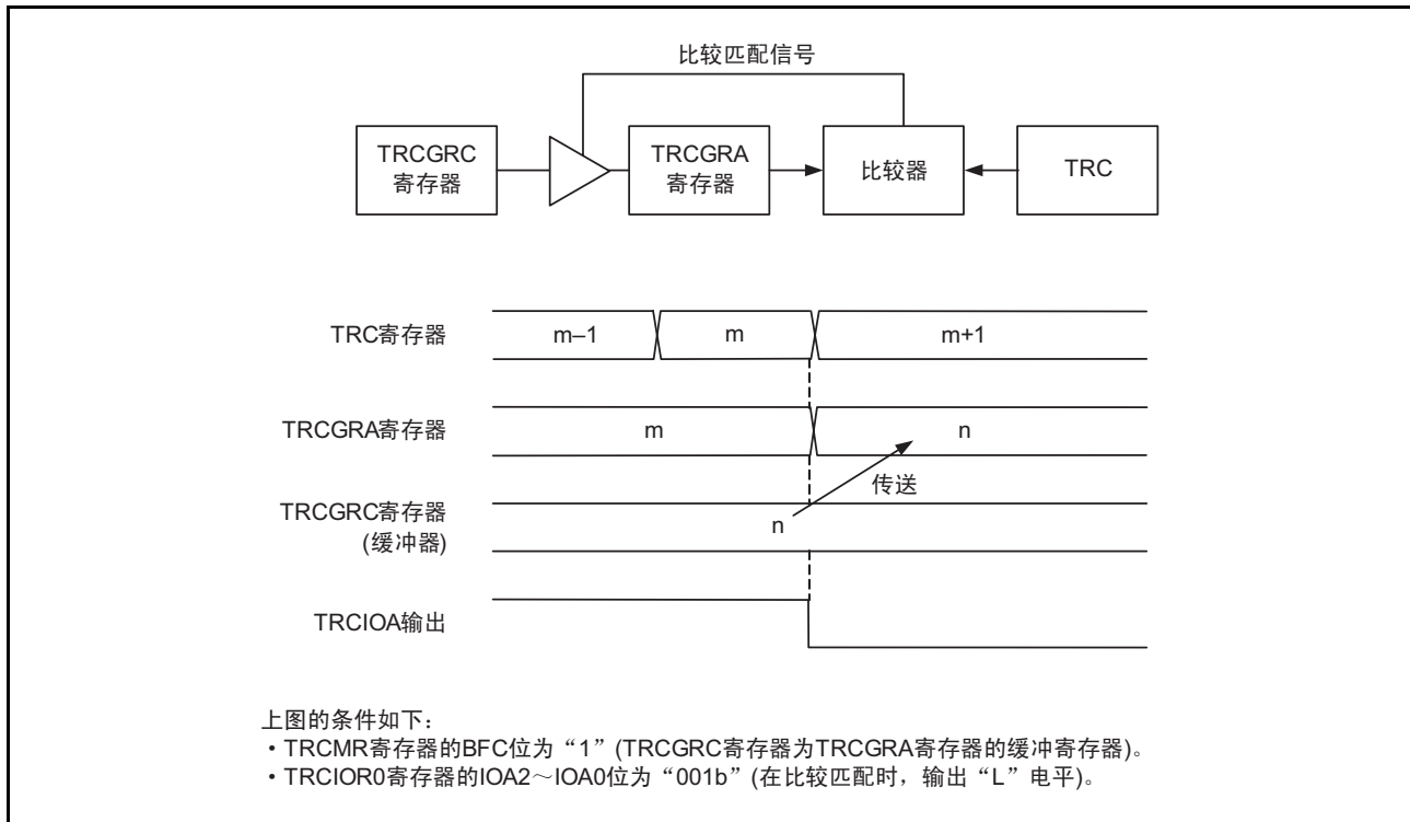
图 19.4 输出比较功能的缓冲器运行
