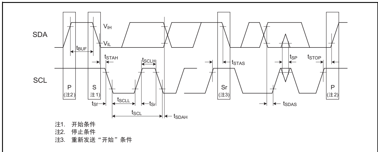
图 31.7 I 2 C 总线接口的输入 / 输出时序
