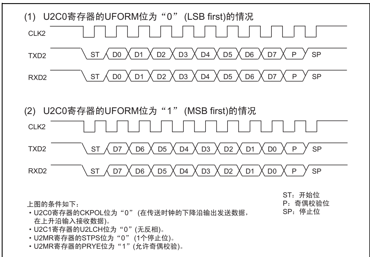
图 22.9 传送格式
