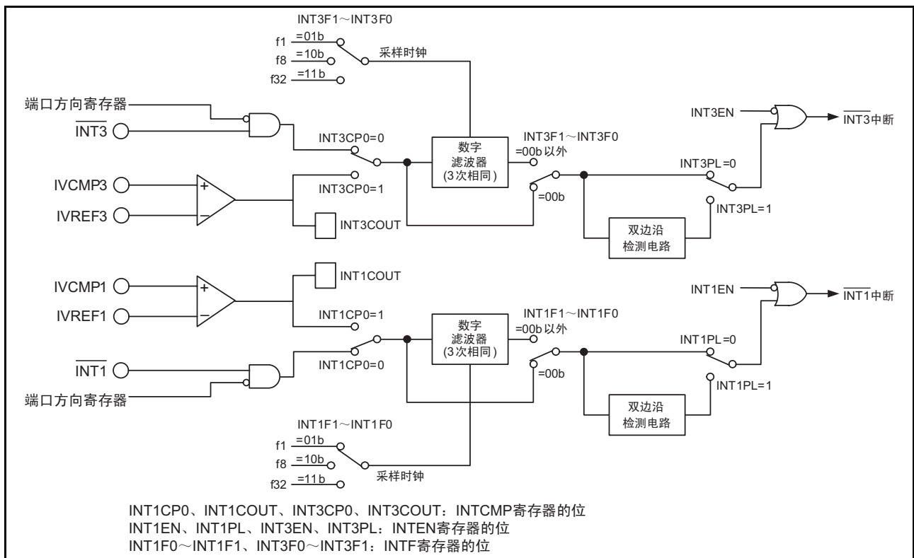
图 28.1 比较电路 B 的框图
