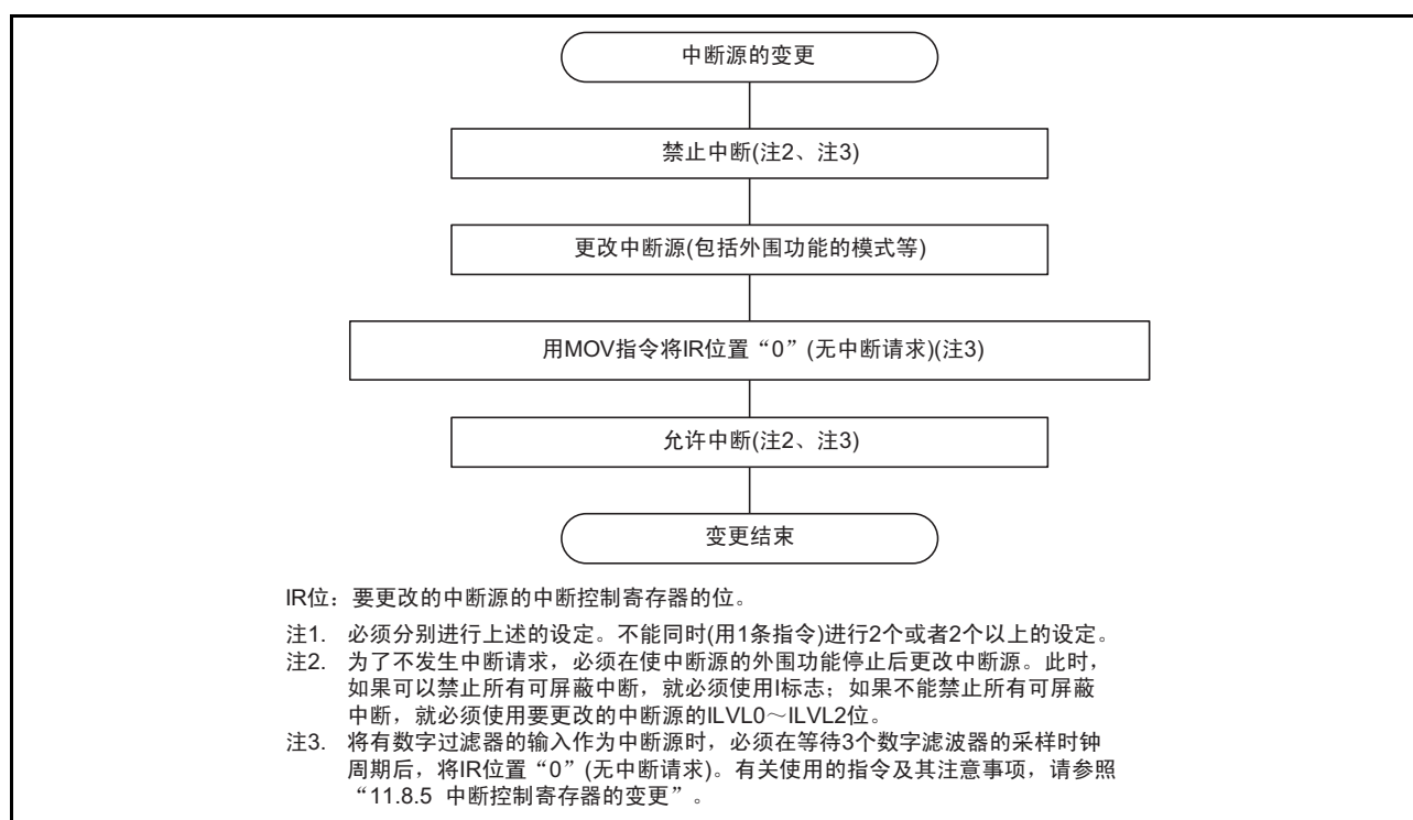
图 11.12 中断源的变更步骤例子
