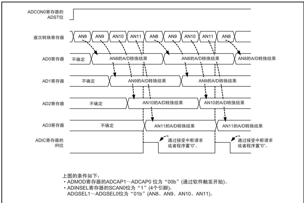
图 27.9 重复扫描模式的运行例子
