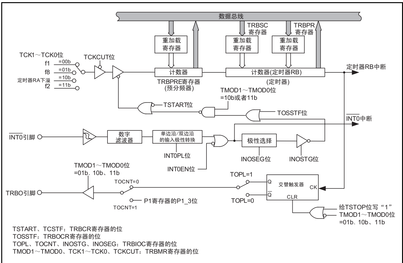
图 18.1 定时器 RB 的框图
