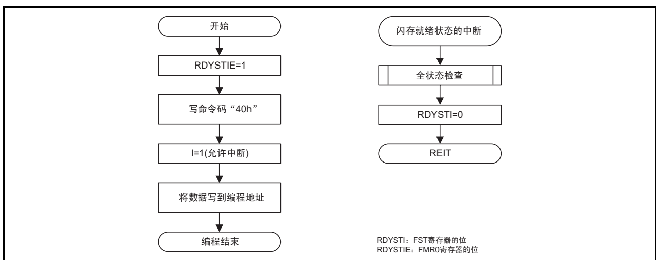
图 29.9 编程的流程图（允许闪存就绪状态的中断）
