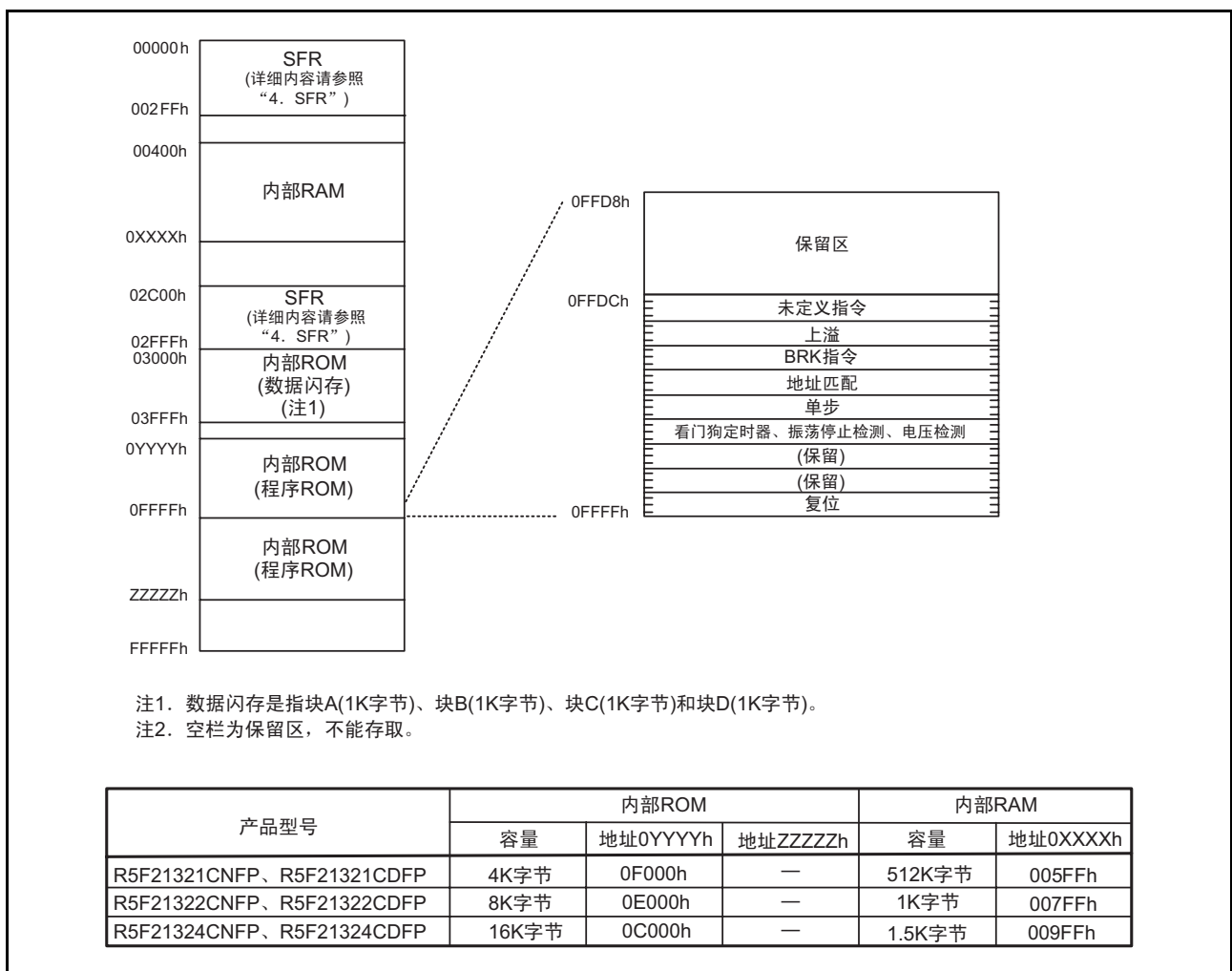
图 3.1 R8C/32C 群的存储器分配图
