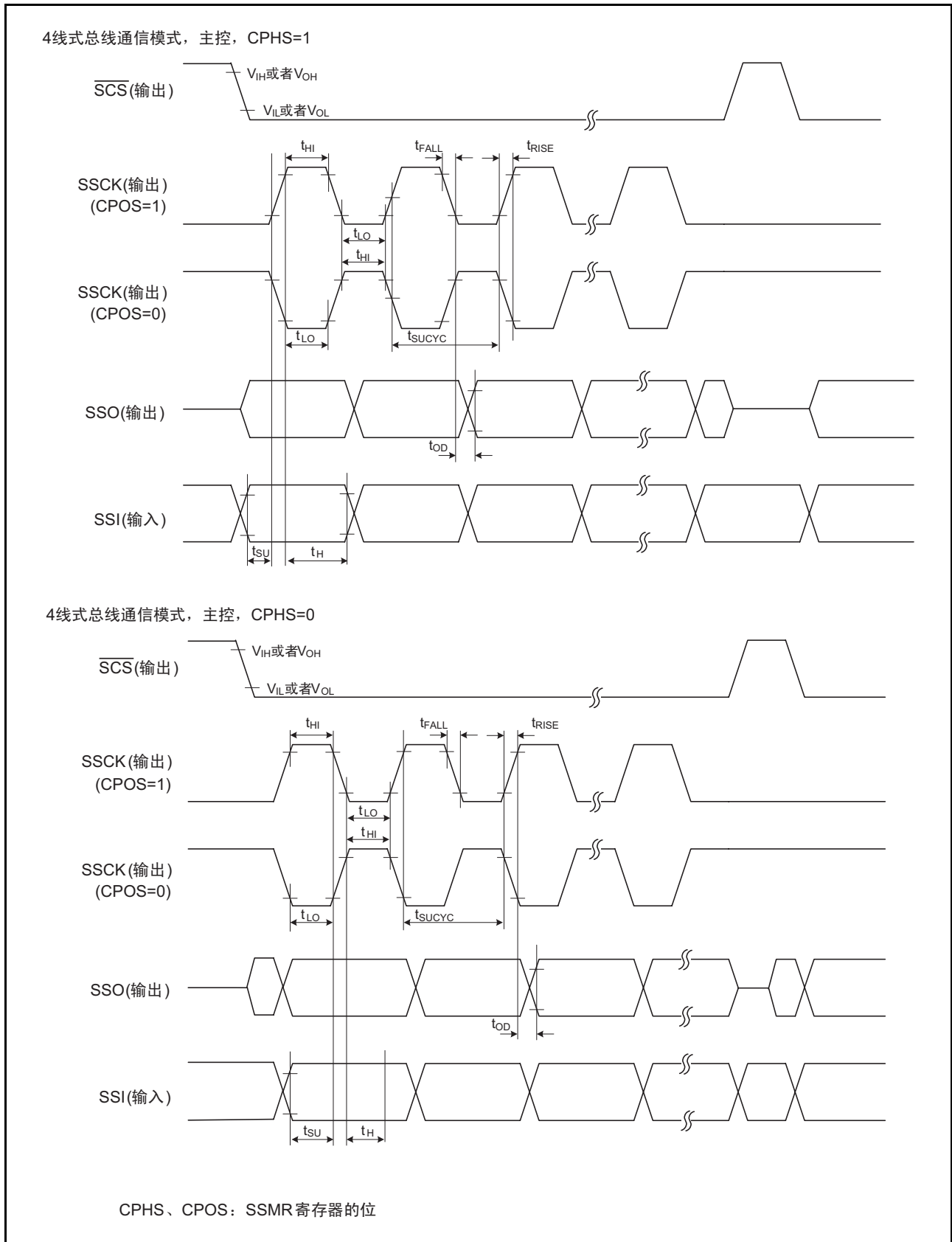
图 31.4 同步串行通信单元 (SSU) 的输入 / 输出时序 (主控)
