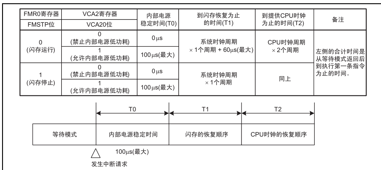
图 9.6 从 CM3 寄存器的 CM30 位被置“1”（转移到等待模式）后的等待模式返回后到执行第一条指令的时间
