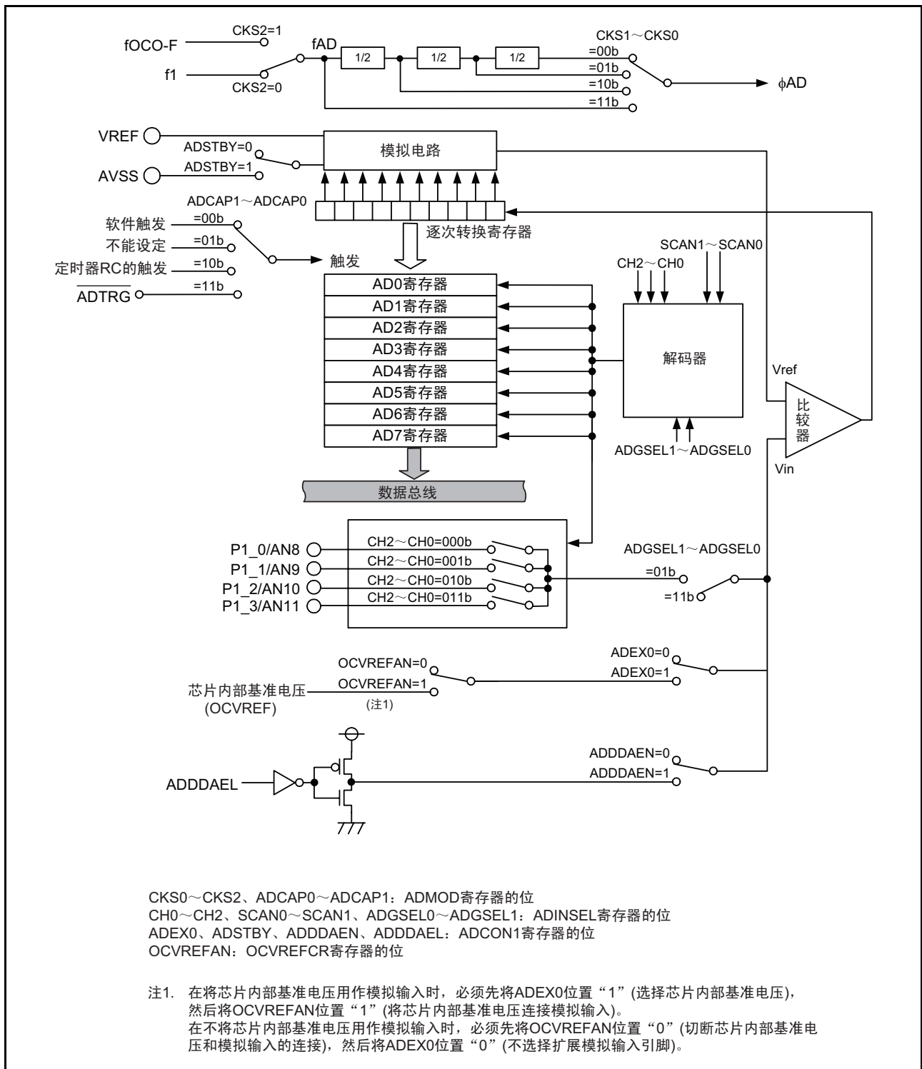
图 27.1 A/D 转换器的框图
