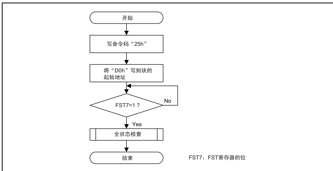
图 29.15 块空白检查的流程图
