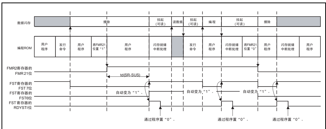
图 29.3 挂起的相关时序
