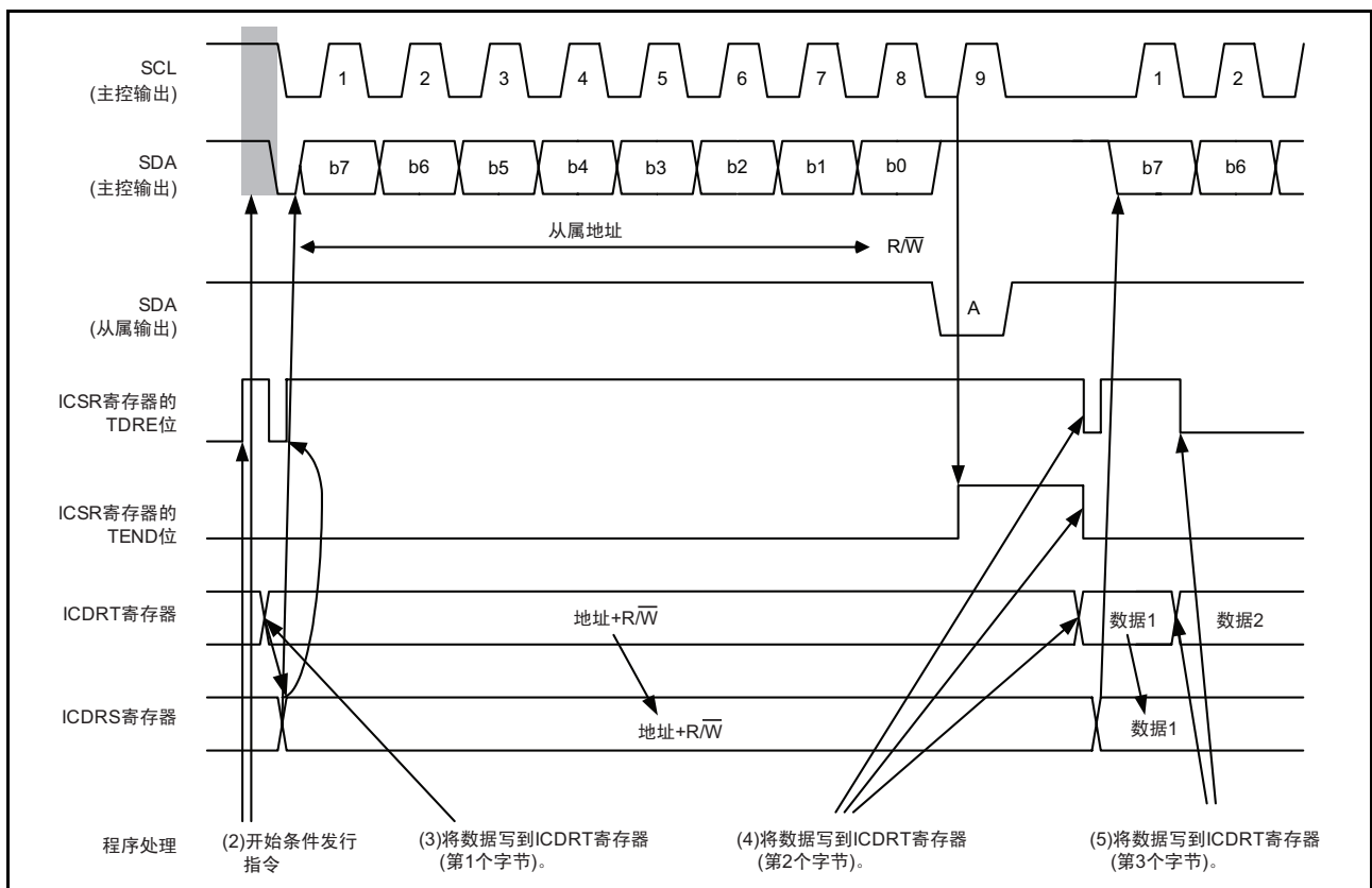
图 25.5 主控发送模式的运行时序（I 2 C 总线接口模式）（1）
