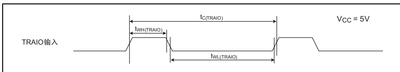
图 31.9 V_{CC}=5V 时的 TRAIO 输入时序
