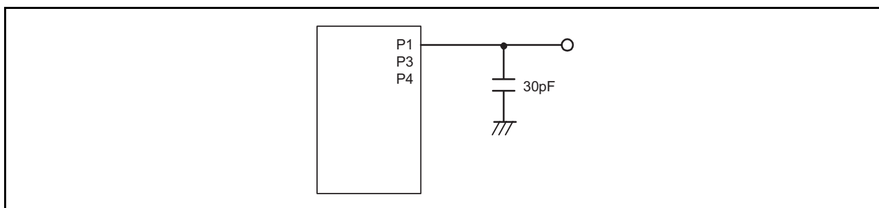
图 31.1 端口 P1、P3、P4 的时序测量电路
