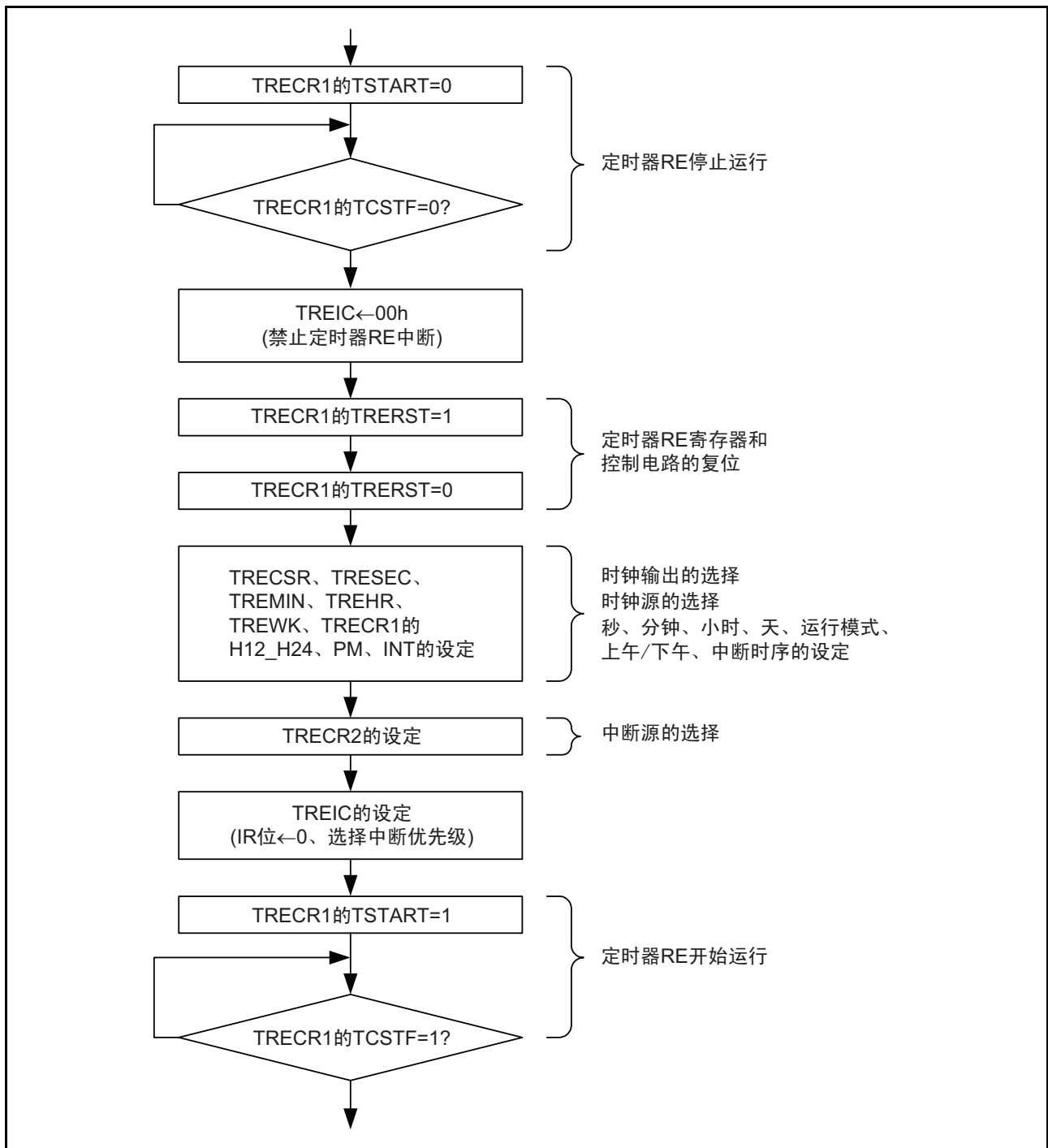
图 32.2 实时时钟模式的设定例子
