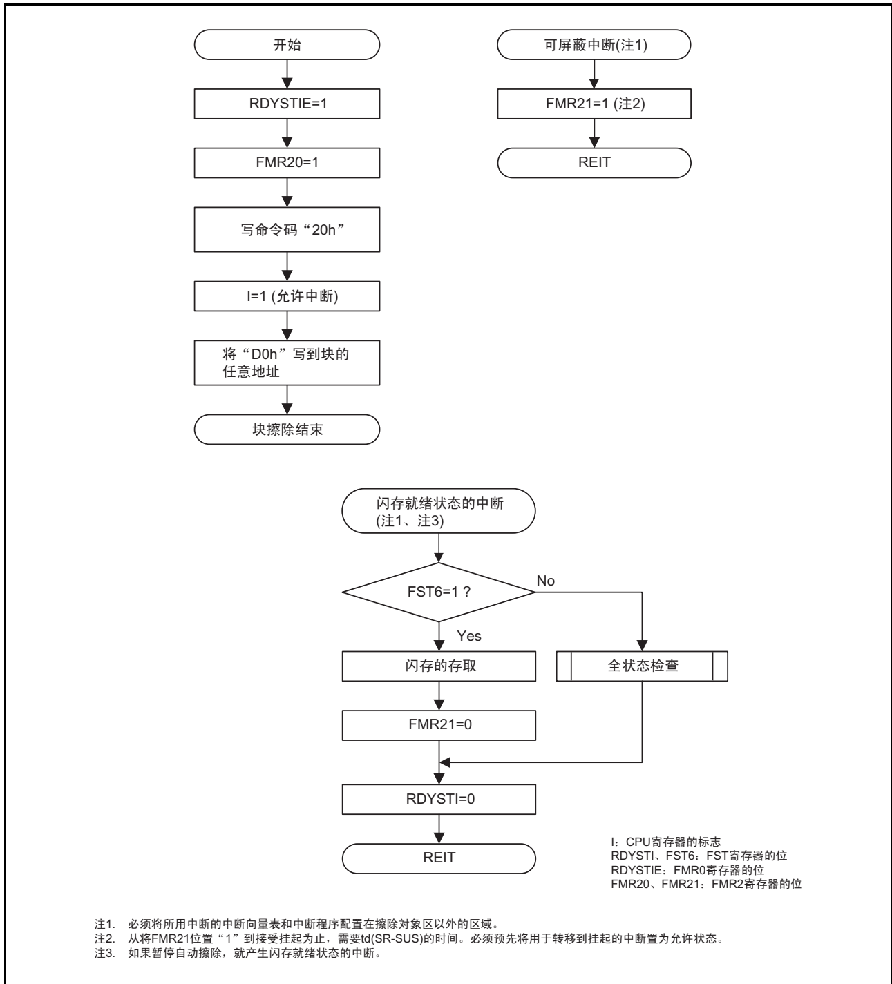
图 29.12 块擦除的流程图（允许闪存就绪状态的中断和挂起）
