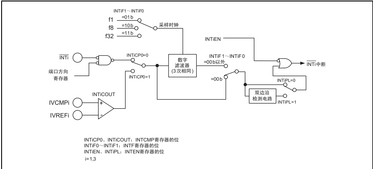
图 28.3 比较电路 Bi 数字滤波器的结构
