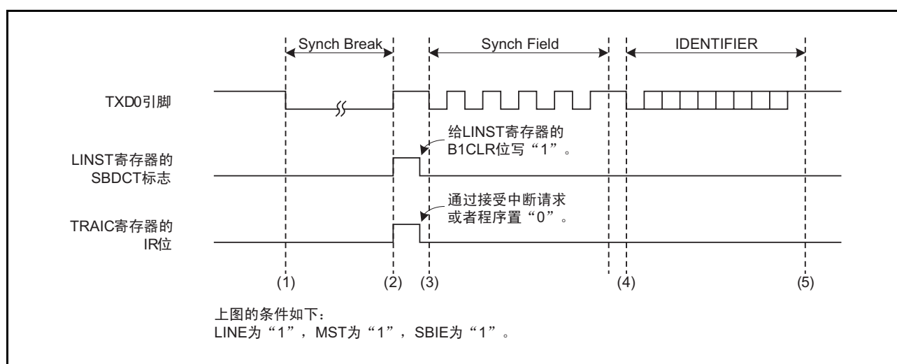
图 26.2 标题字段的发送运行例子
