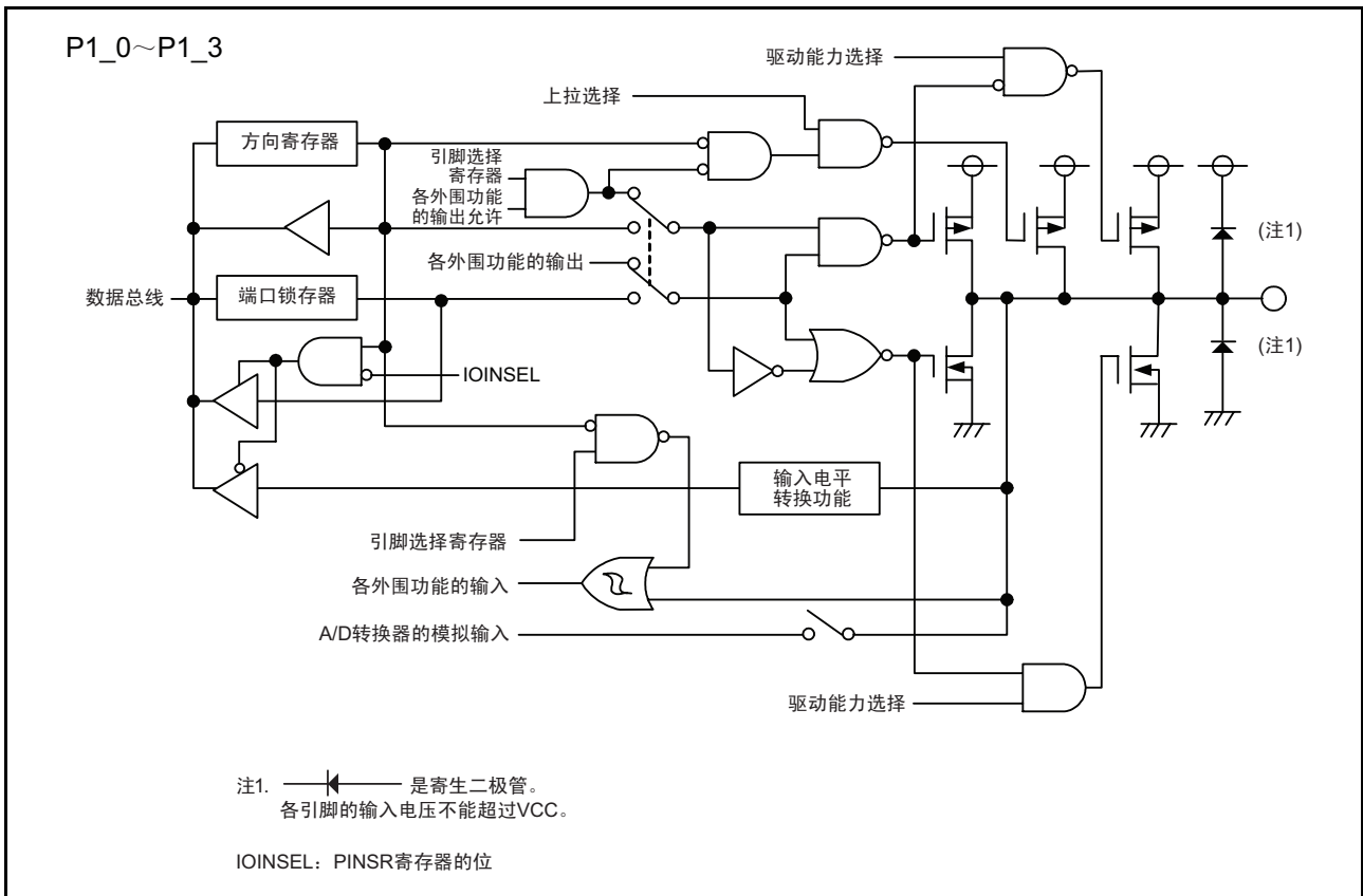
图 7.1 I/O 端口的结构 (1)
