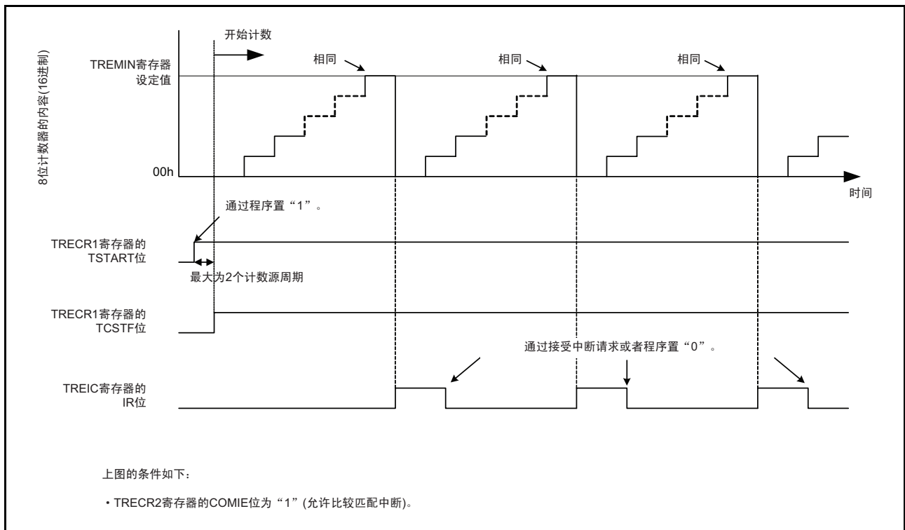
图 20.5 输出比较模式的运行例子
