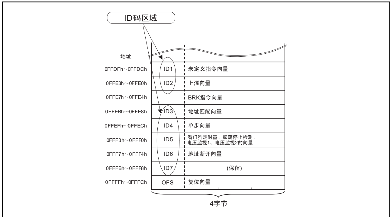
图 12.1 ID 码区域
