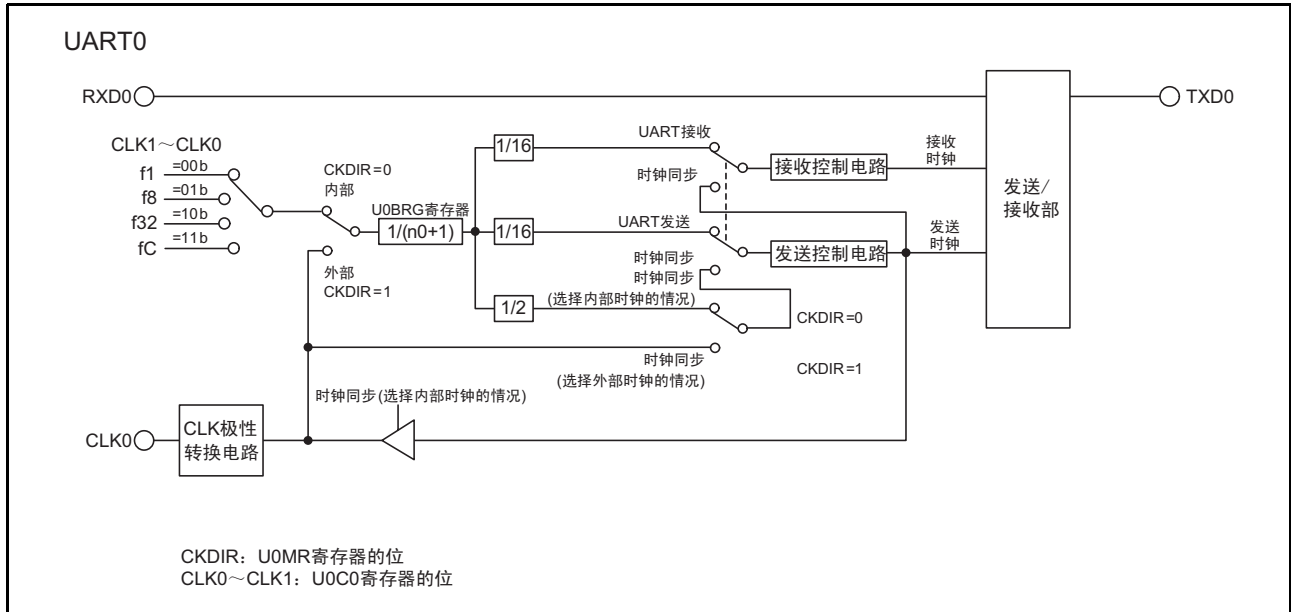
图 21.1 UART0 的框图
