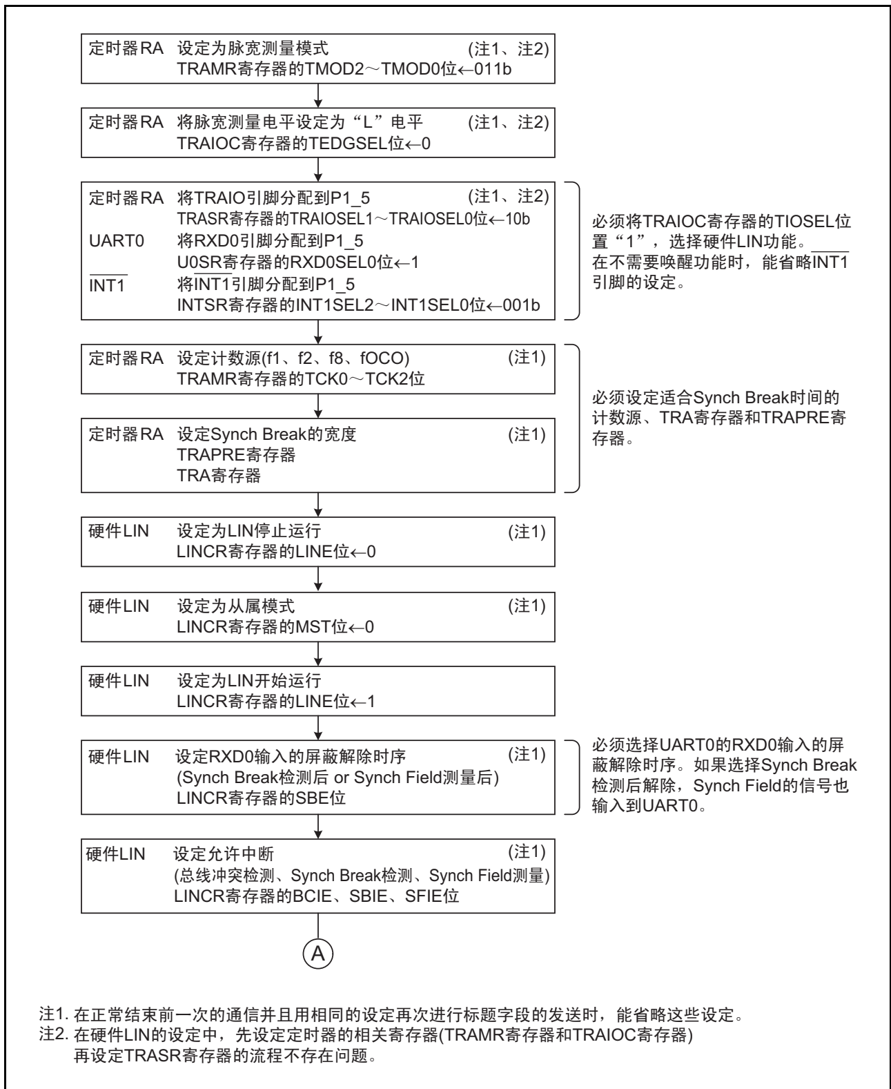
图 26.6 标题字段的接收流程图例子 (1)
