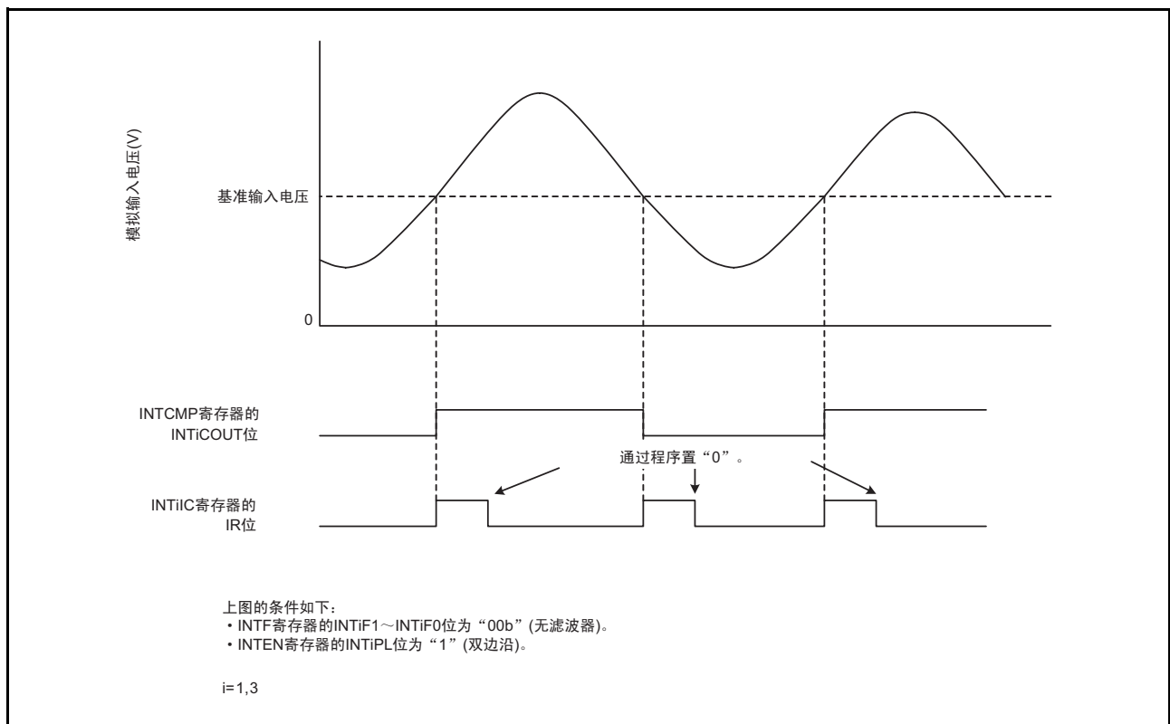
图 28.2 比较电路 Bi（i=1,3）的运行例子
