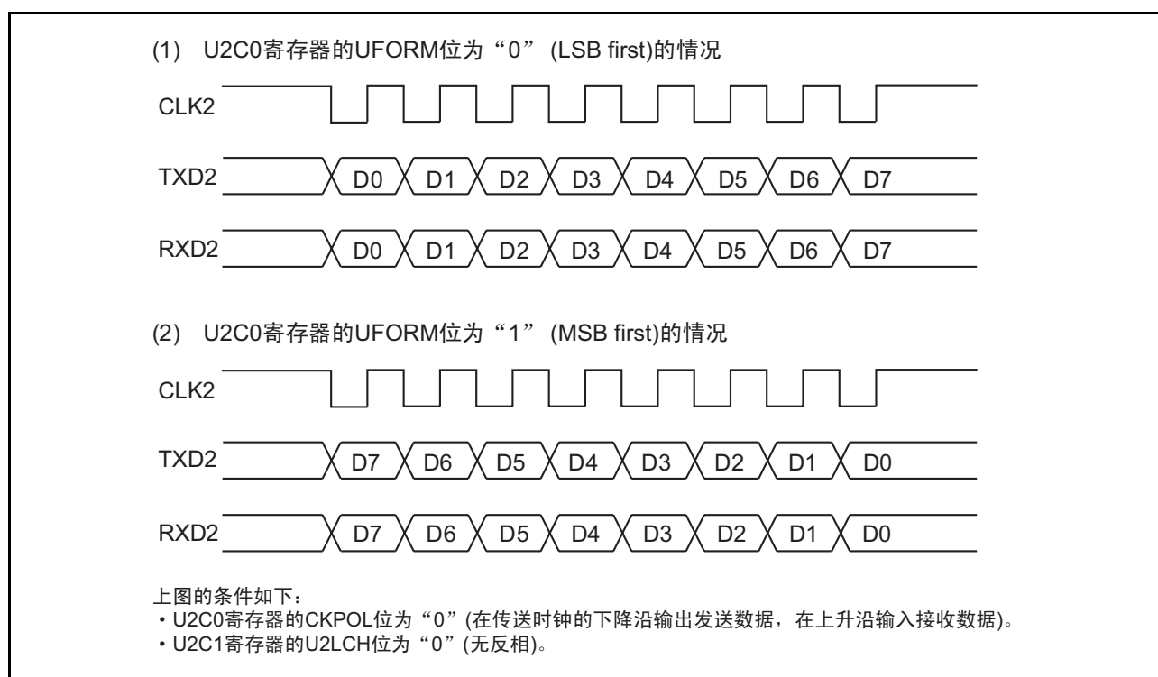
图 22.5 传送格式
