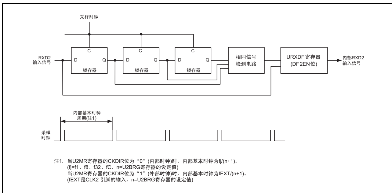
图 22.22 RXD2 数字滤波器电路的框图
