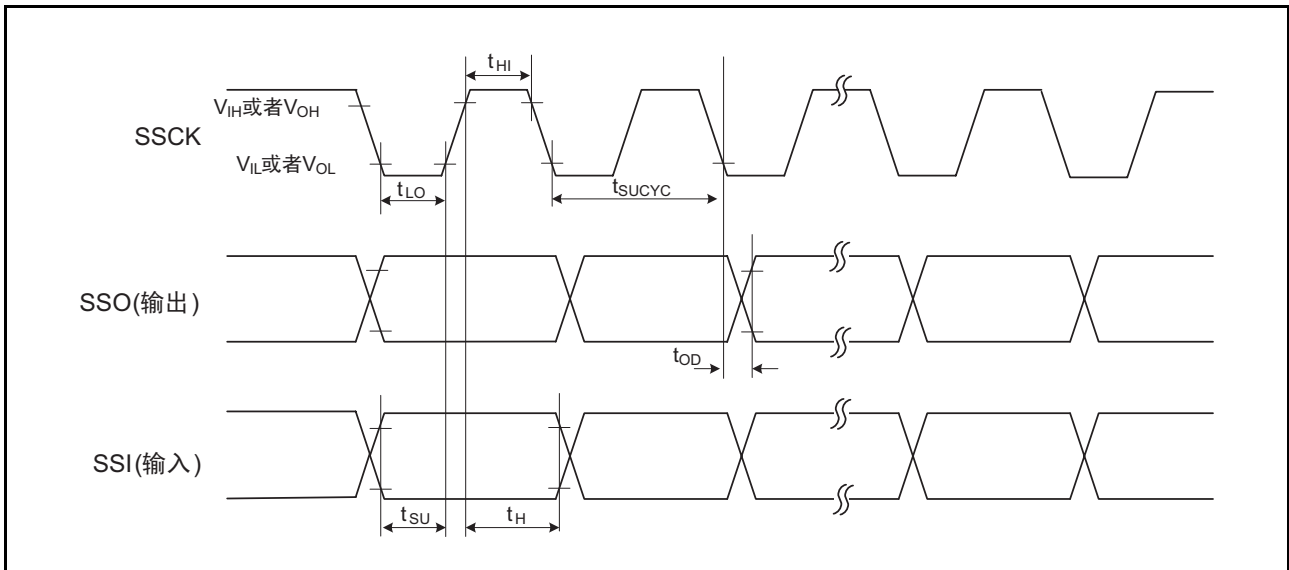
图 31.6 同步串行通信单元 (SSU) 的输入 / 输出时序 (时钟同步通信模式)
