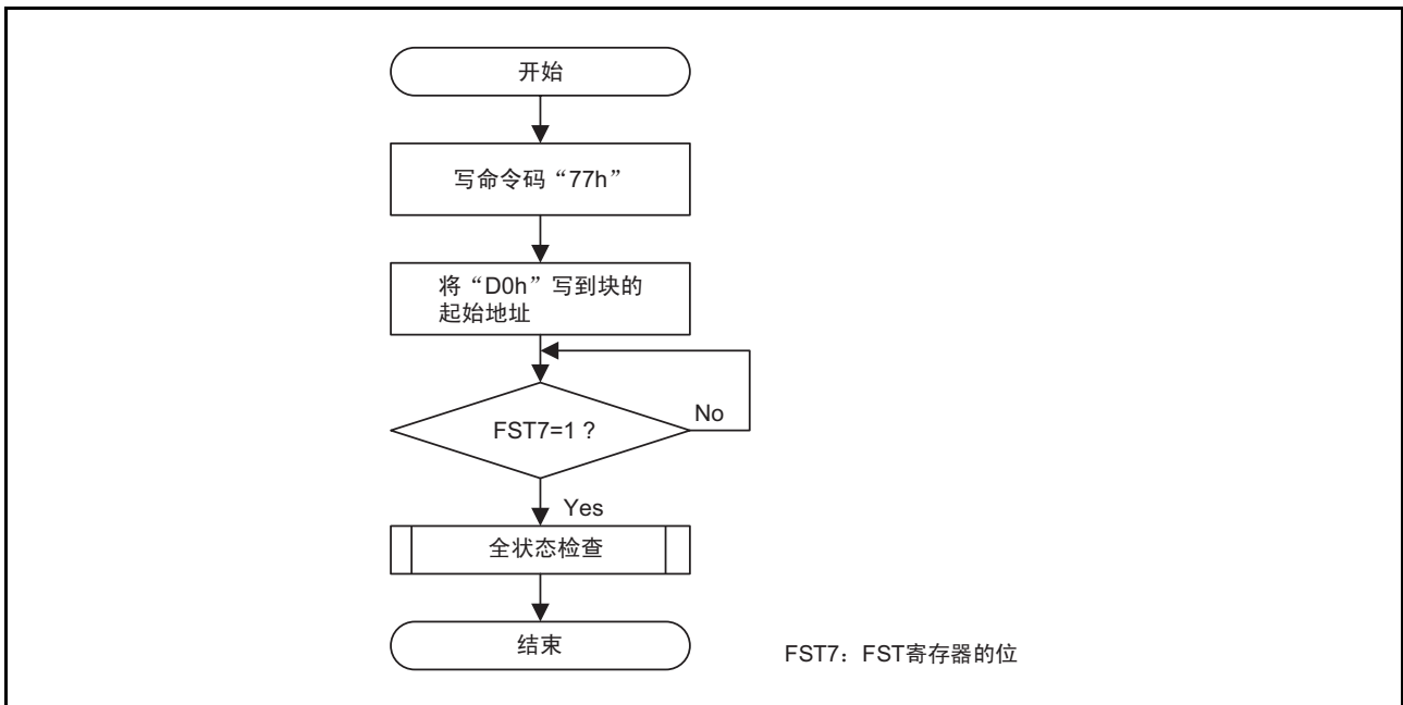
图 29.13 锁定位编程的流程图
