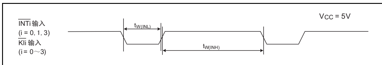
图 31.11 V CC =5V 时的外部中断 \overline{INTi} 和键输入中断 \overline{Kli} 的输入时序
