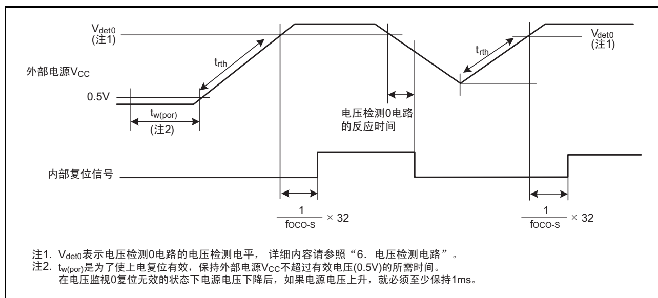
图 31.3 上电复位电路的电特性
