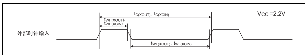
图 31.16 V_{CC}=2.2V 时的外部时钟输入时序
