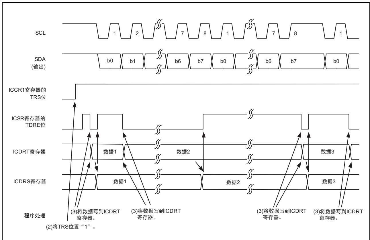
图 25.14 发送模式的运行时序（时钟同步串行模式）
