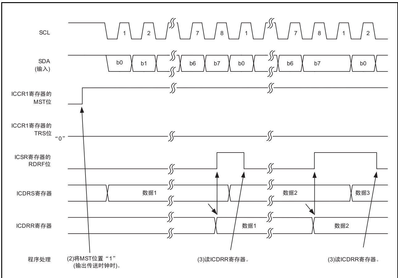
图 25.15 接收模式的运行时序（时钟同步串行模式）
