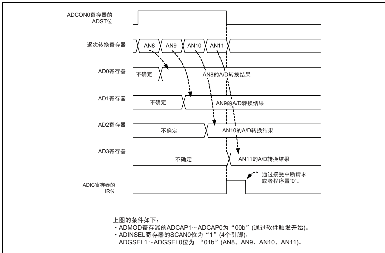
图 27.8 单次扫描模式的运行例子
