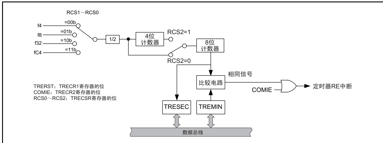
图 20.4 输出比较模式的框图
