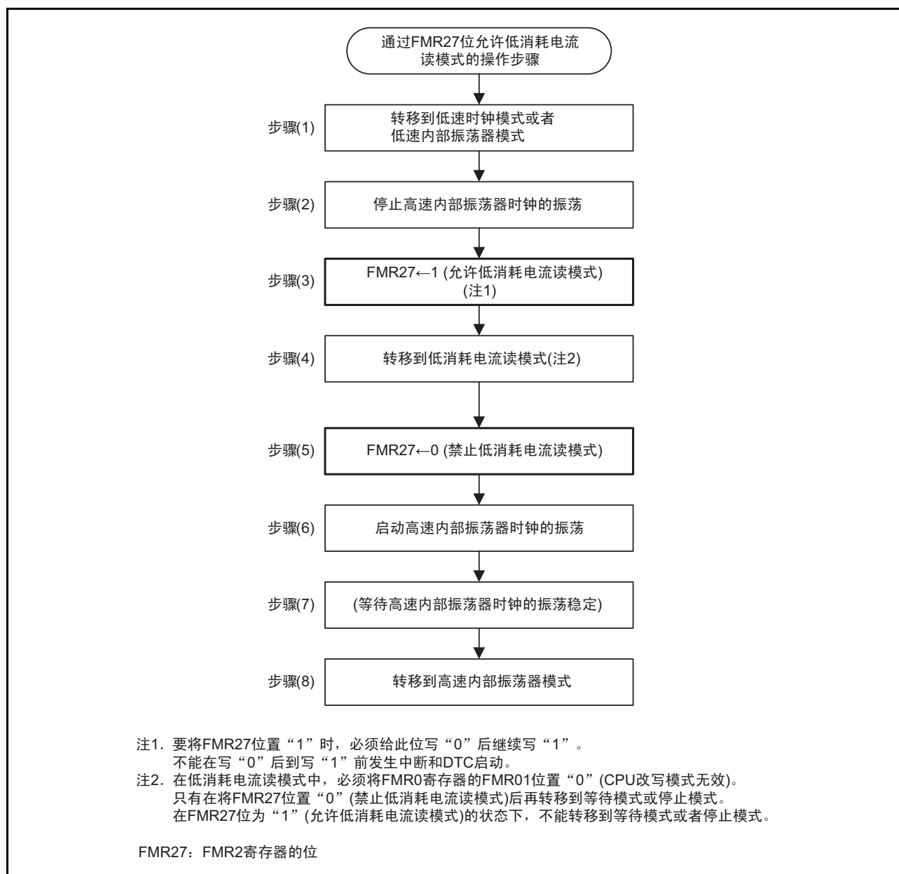
图 30.3 低消耗电流读模式的操作步骤例子
