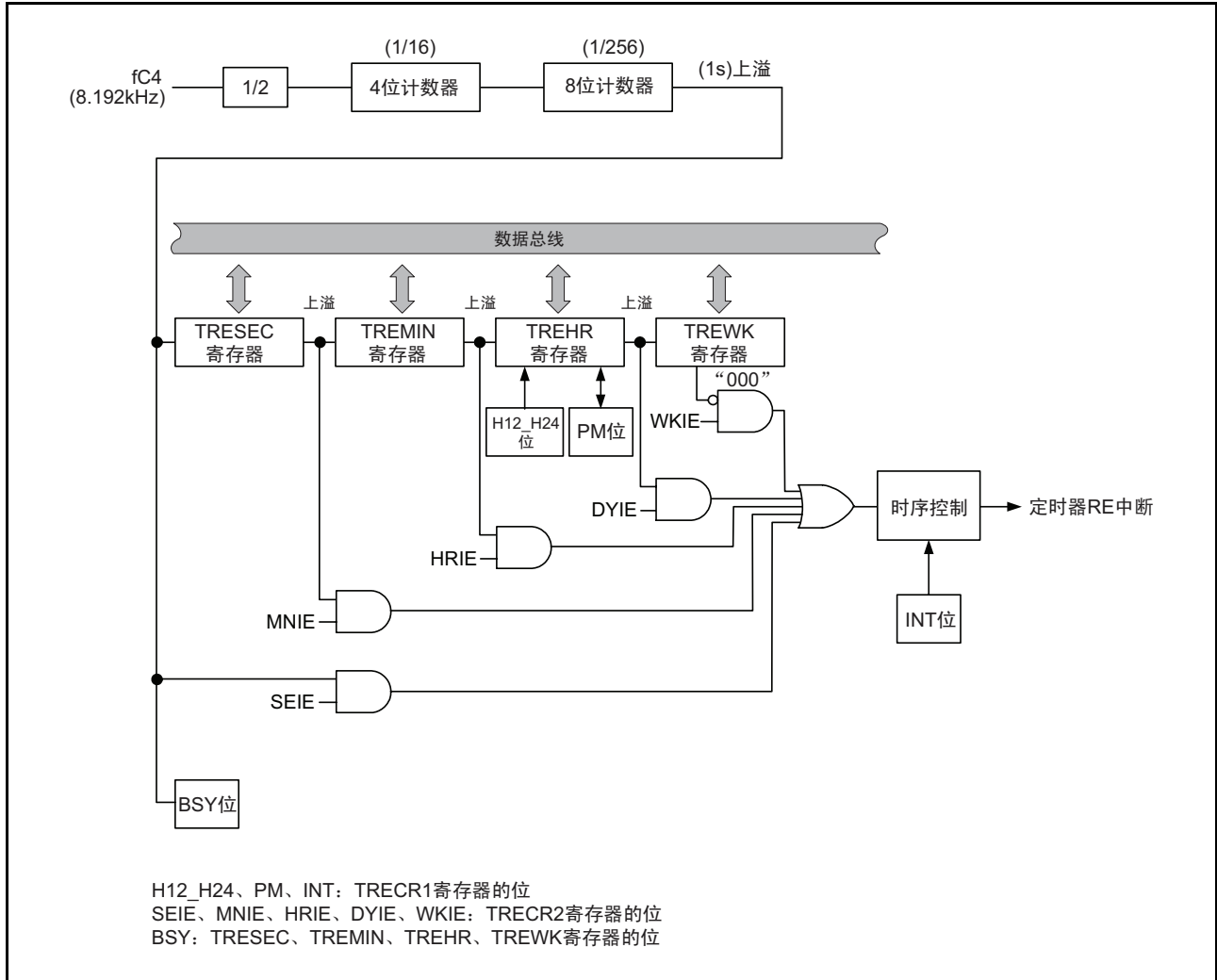
图 20.1 实时时钟模式的框图
