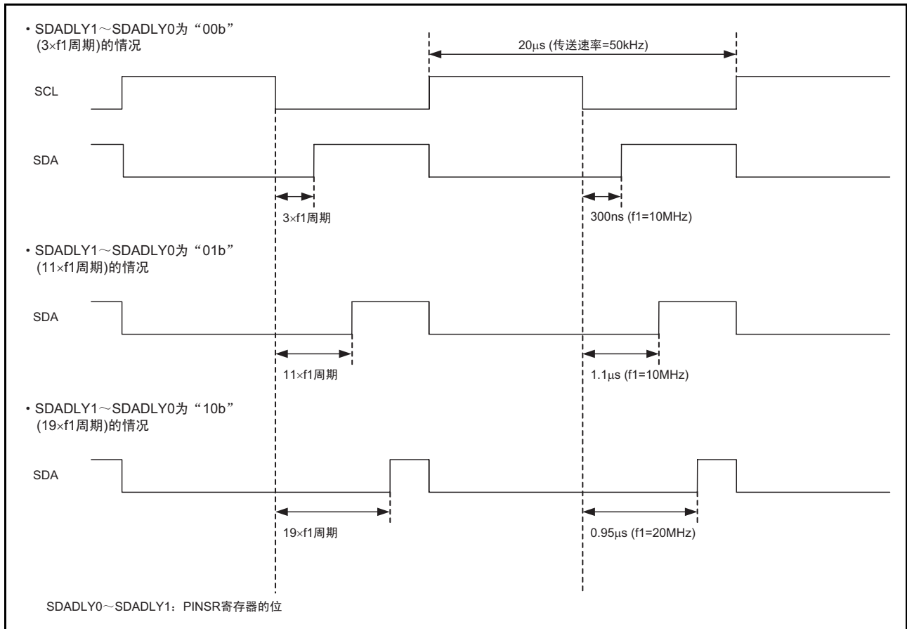
图 25.3 SDA 引脚的数字延迟的运行例子
