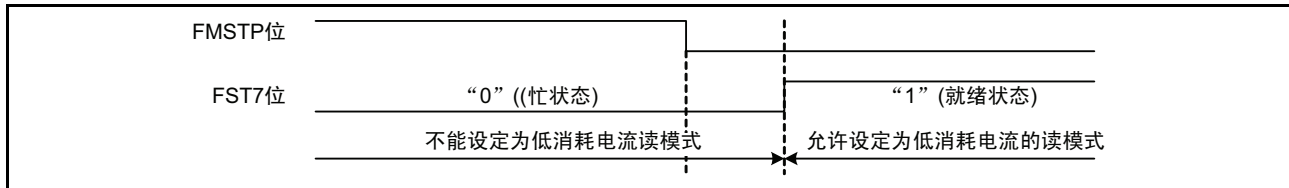
图 29.2 转移到低消耗电流读模式
