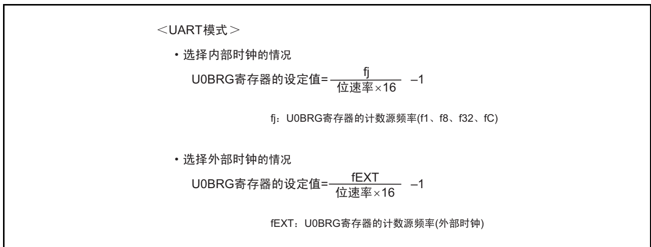
图 21.8 U0BRG 寄存器的设定值的计算式
