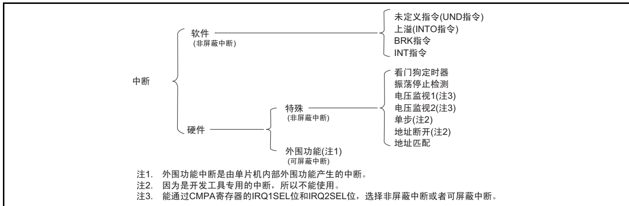
图 11.1 中断的分类
