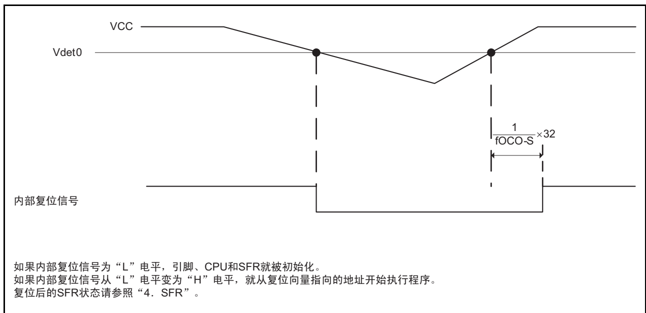
图 6.5 电压监视 0 复位的运行例子
