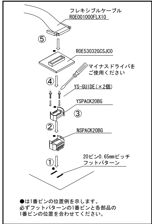
図3 ROE53032GCSJCO装着手順
