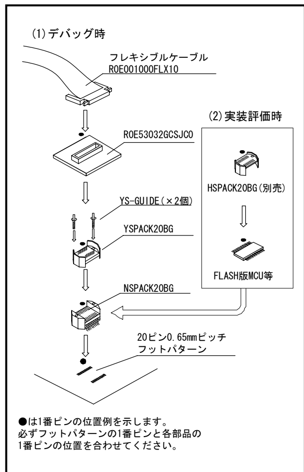
図2 ROE53032GCSJCOの用途
