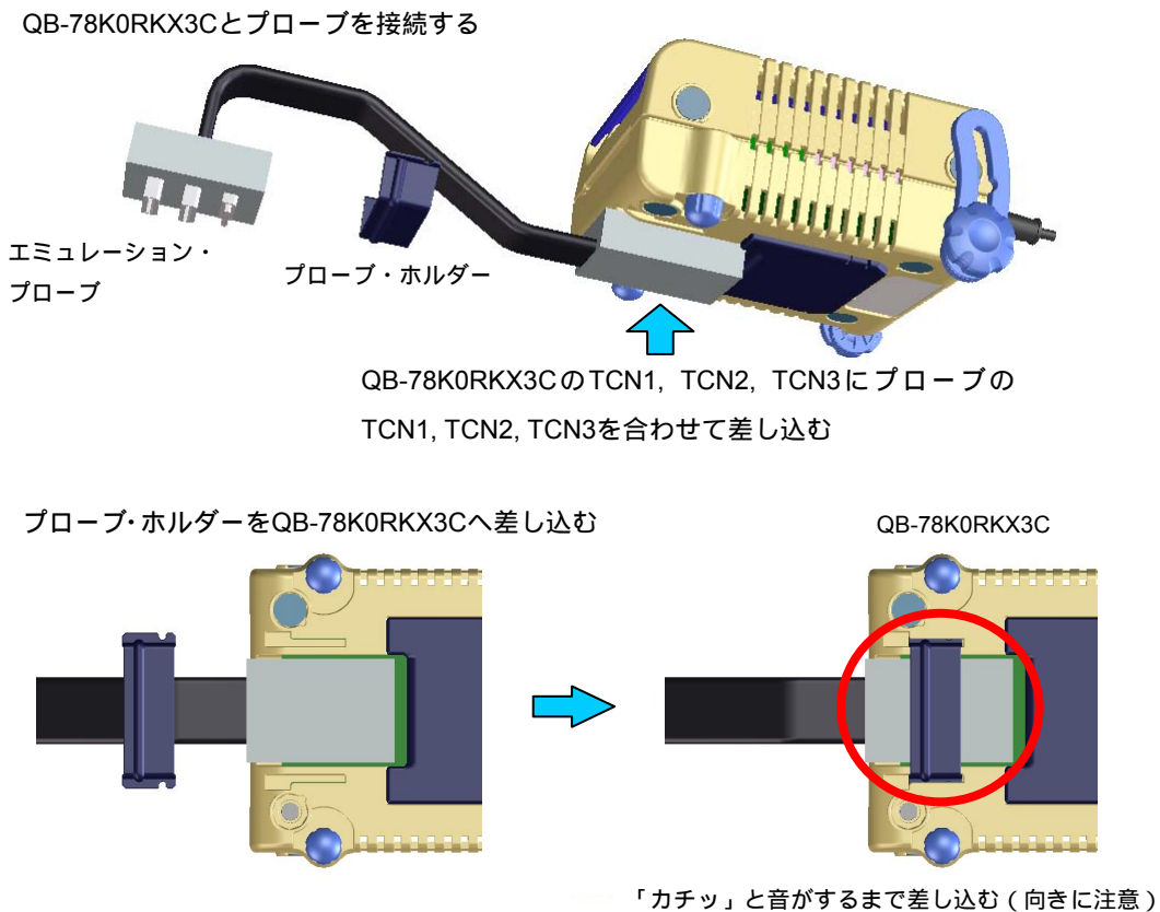
図2 - 5 QB-78K0RKX3Cとプローブの接続
