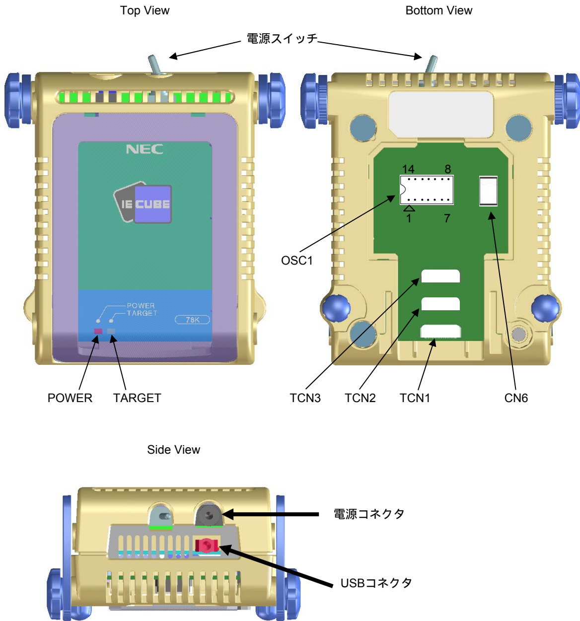
図2 - 1 QB-78K0RKX3Cの各部の名称
