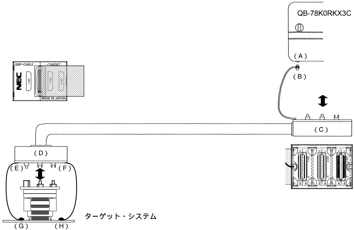
図2-6 GND線
