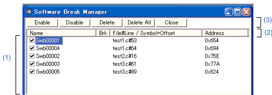
図 6 - 57 ソフトウェア・ブレイク・マネージャ
