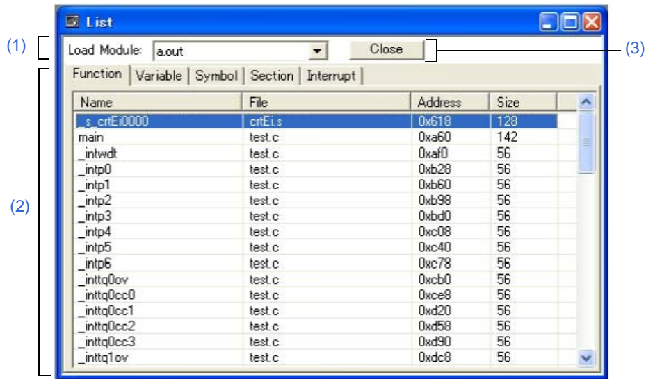
図 6 - 26 リスト・ウィンドウ
