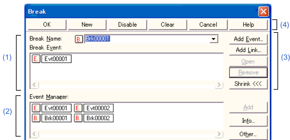
図 6 - 61 ブレーク・ダイアログ
