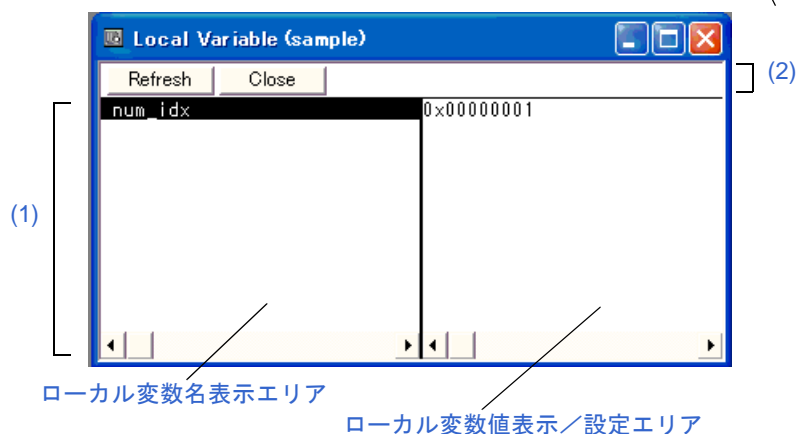
図 6 - 31 ローカル変数ウィンドウ
