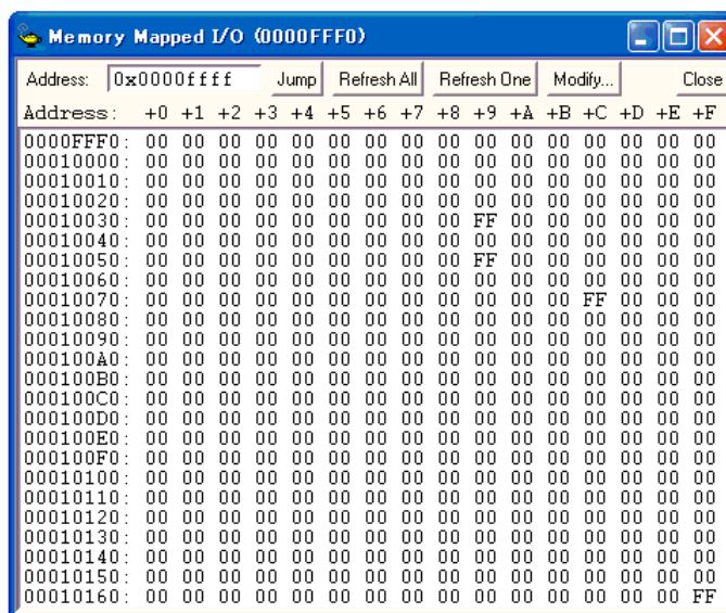
図 A - 5 Memory Mapped I/O ウインドウ
