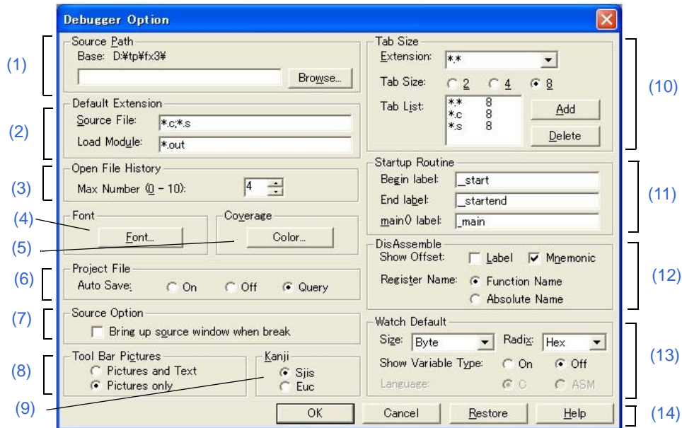
図 6 - 11 デバッガ・オプション設定ダイアログ
