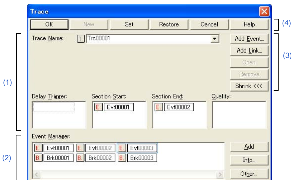
図 6 - 52 トレース・ダイアログ
