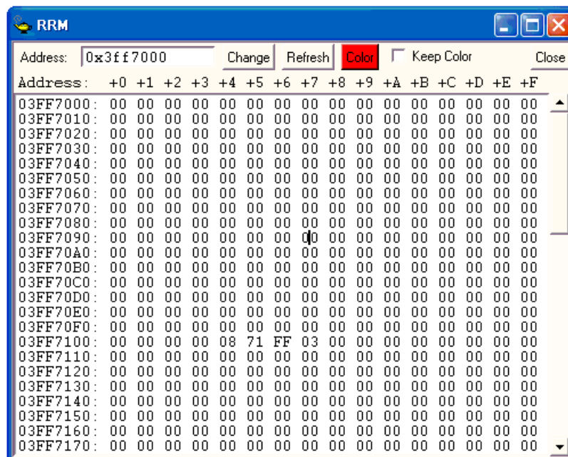
図 A - 3 RRM ウインドウ
