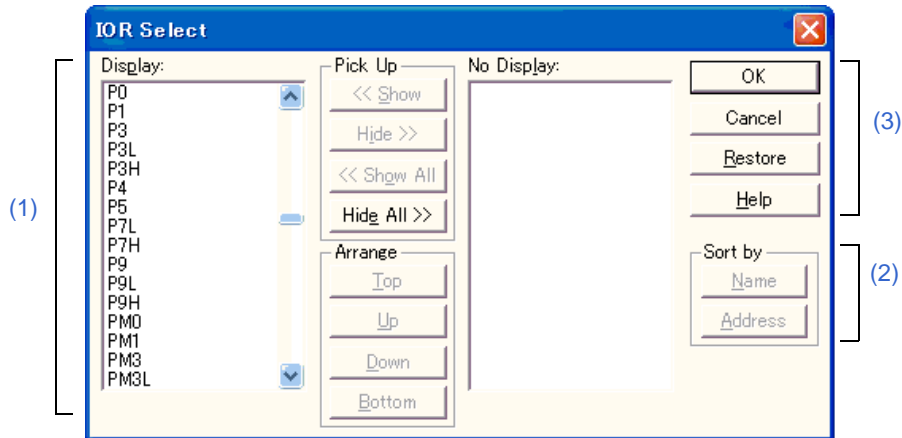
図 6 - 44 周辺 I/O レジスタ選択ダイアログ
