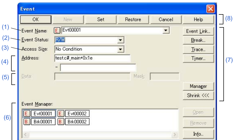
図 6 - 59 イベント・ダイアログ
