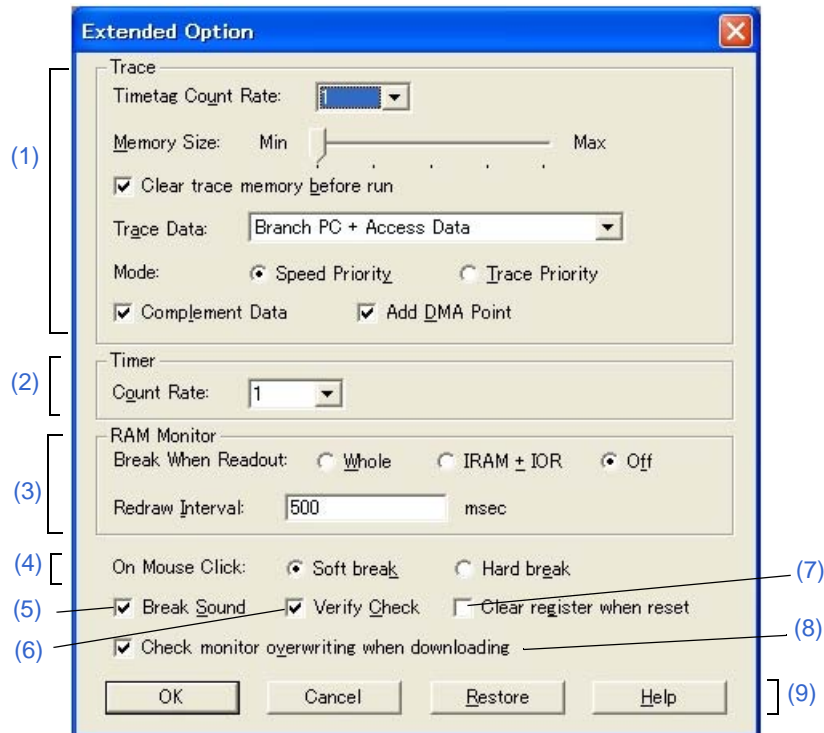
図 6 - 6 拡張オプション設定ダイアログ
