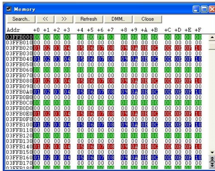
図6-34 メモリ・ウィンドウ (RRM 機能選択時)
