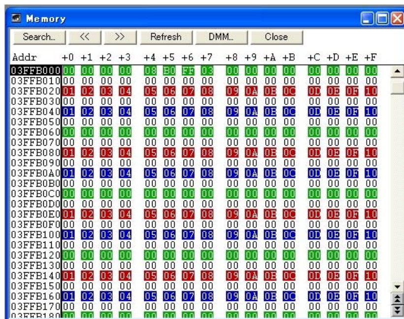
図 5-14 アクセス・モニタ機能（メモリ・ウインドウ）
