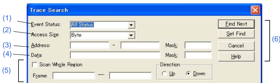
図 6 - 49 トレース・サーチ・ダイアログ
