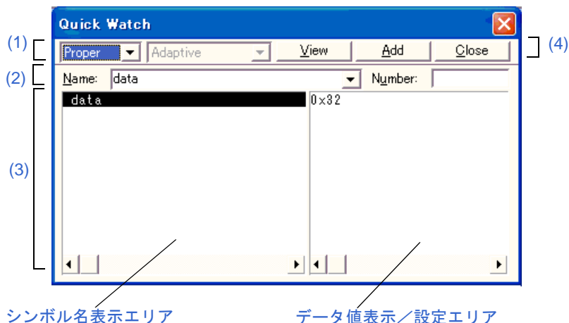
図 6 - 28 クイック・ウォッチ・ダイアログ
