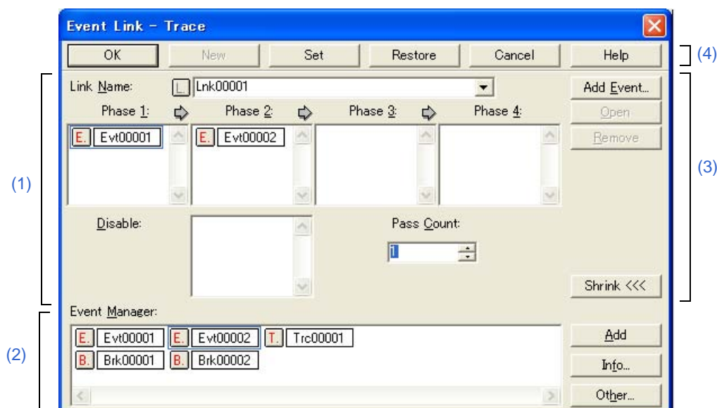
図 6 - 60 イベント・リンク・ダイアログ
