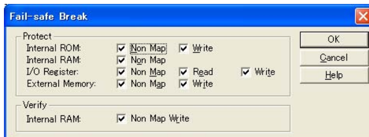
図 5-4 フェイルセーフ・ブレイク設定
