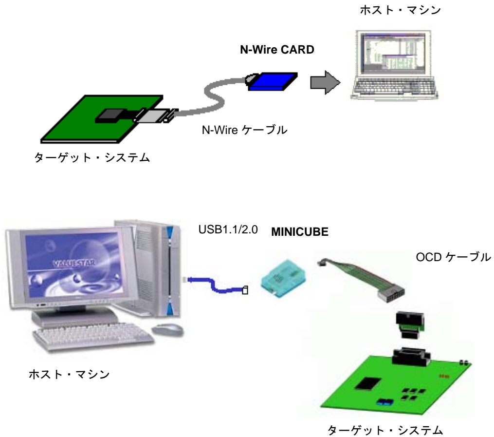
図 1-3 システム構成例 [MINICUBE]
