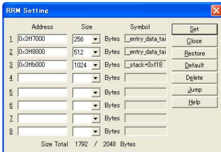
図 5-25 RRM 設定ダイアログ
