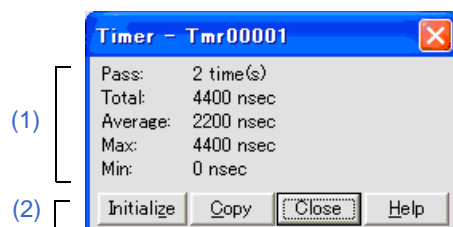
図 6 - 47 タイマ測定結果ダイアログ
